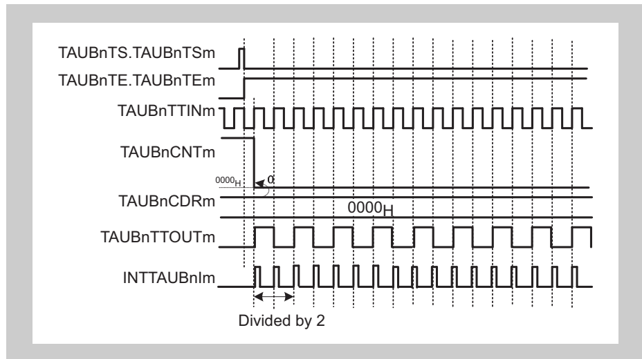
Figure 13-56 TAUBnCDRm = 0000 H , TAUBnCMORm.TAUBnMD0 = 1, TAUBnCMURm.TAUBnTIS[1:0] = 01 B
