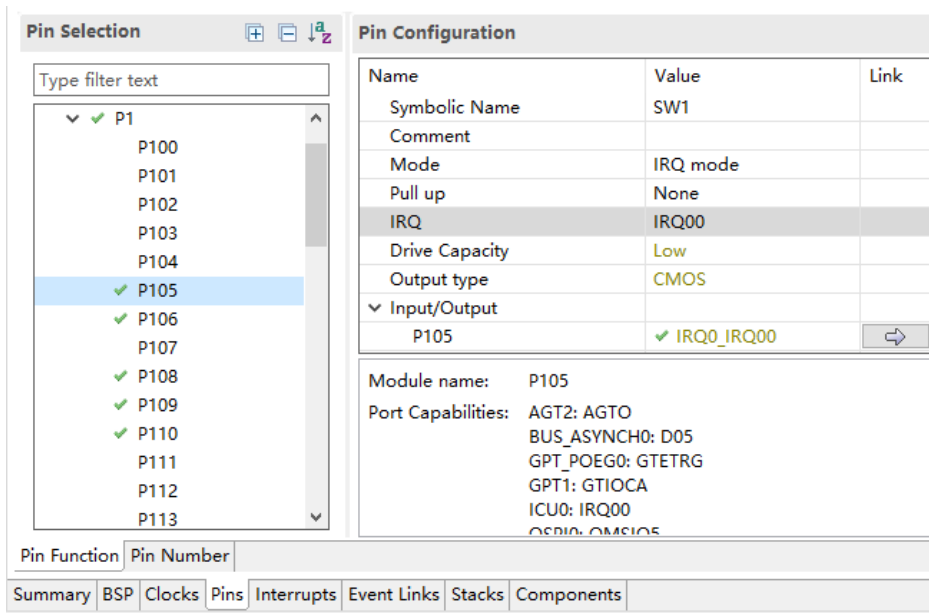
图 4-6: 应已为 IRQ00 正确配置了端口 P105
