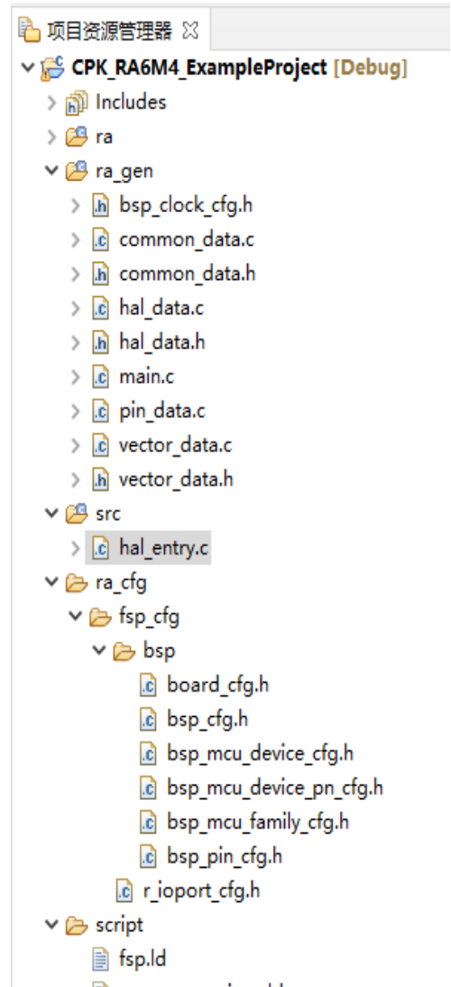
图 3-9: FSP 配置器创建所需文件后的项目树
