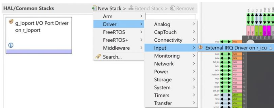
图 5-1: 首先添加 S1 中断的驱动程序
