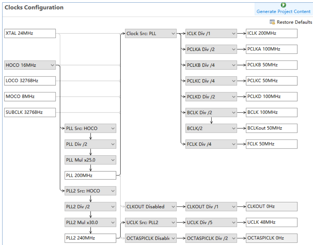
图 5-4: USB FS 需要使用 48 MHz 的时钟，因此需要相应地更改时钟生成电路。必要的更改已突出显示
