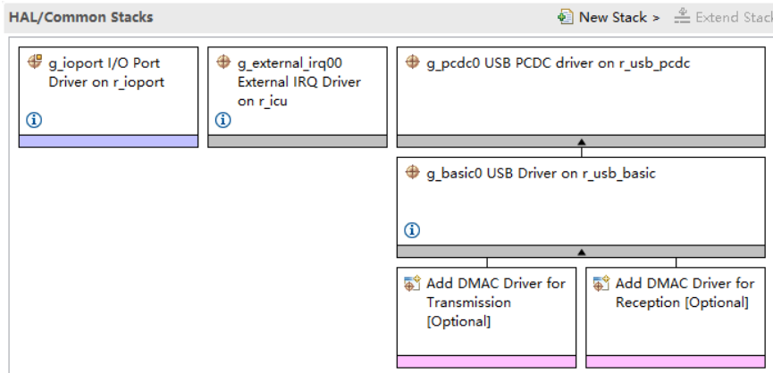
图 5-5: 添加 USB 驱动程序后“堆”窗格的外观
