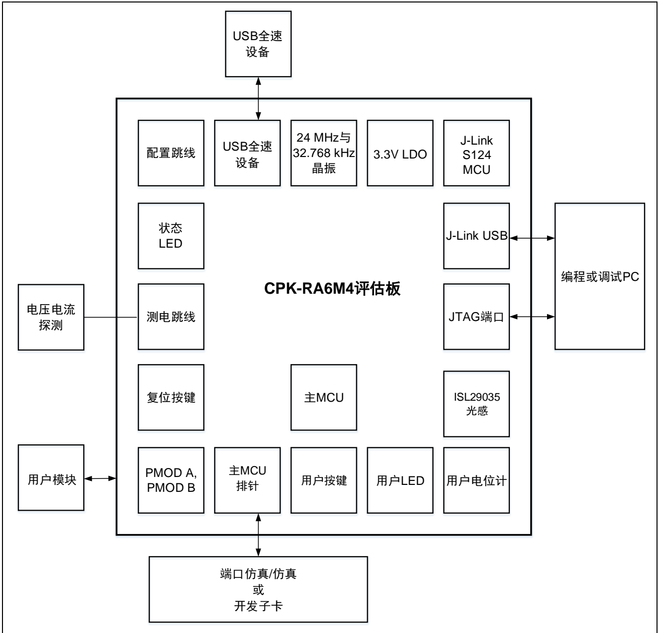
图 3-1: CPK-RA6M4 评估板的框图
