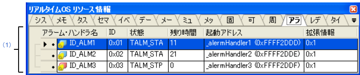
図 A—26 [アラーム・ハンドラ] タブ
