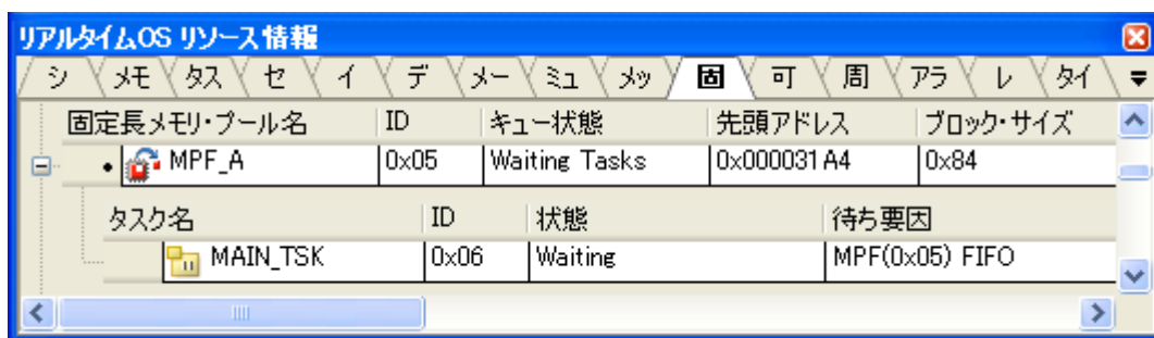
図 A—22 [固定長メモリ・プール] タブ (待ちタスク情報)
