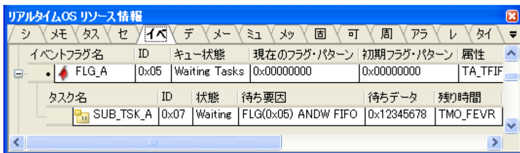
図 A—9 [イベントフラグ] タブ (待ちタスク情報)
