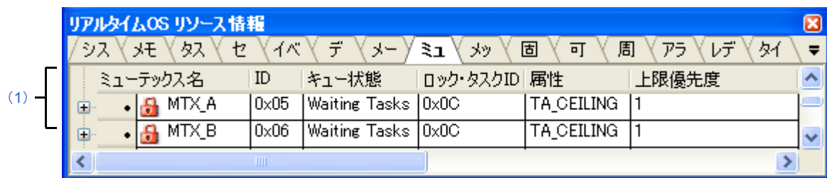
図 A—17 [ミューテックス] タブ
