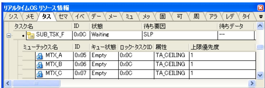
図 A-5 [タスク] タブ（ロック・ミューテックス情報）
