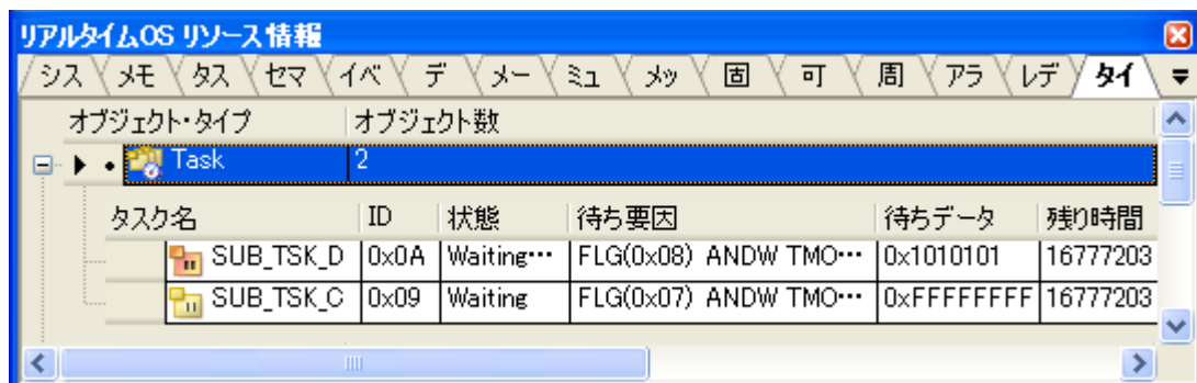
図 A—30 [タイマ・キュー] タブ (待ちタスク情報)
