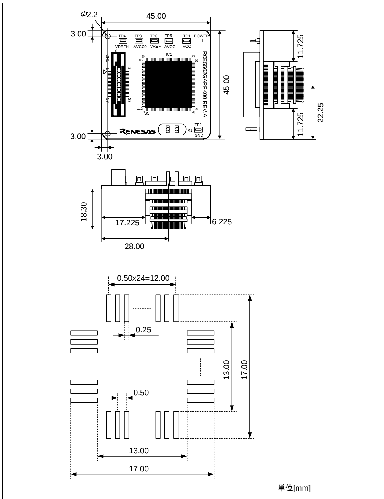
図4 本製品（R0E5562GAPFK00）の寸法図及び参考フットパターン
