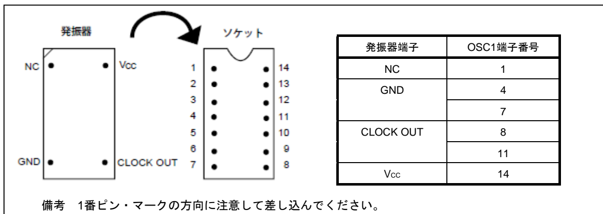
図2-3 発振器とソケットの対応
