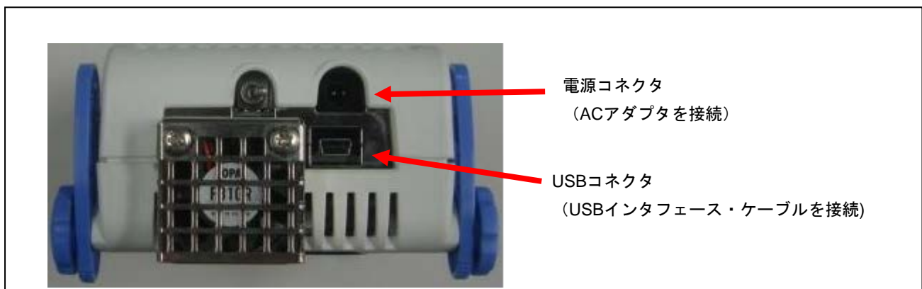
図2-10 コネクタ位置
