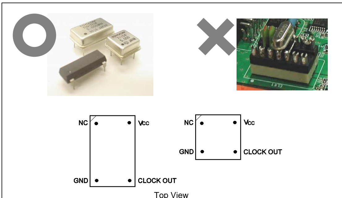
図2-2 発振器形状
