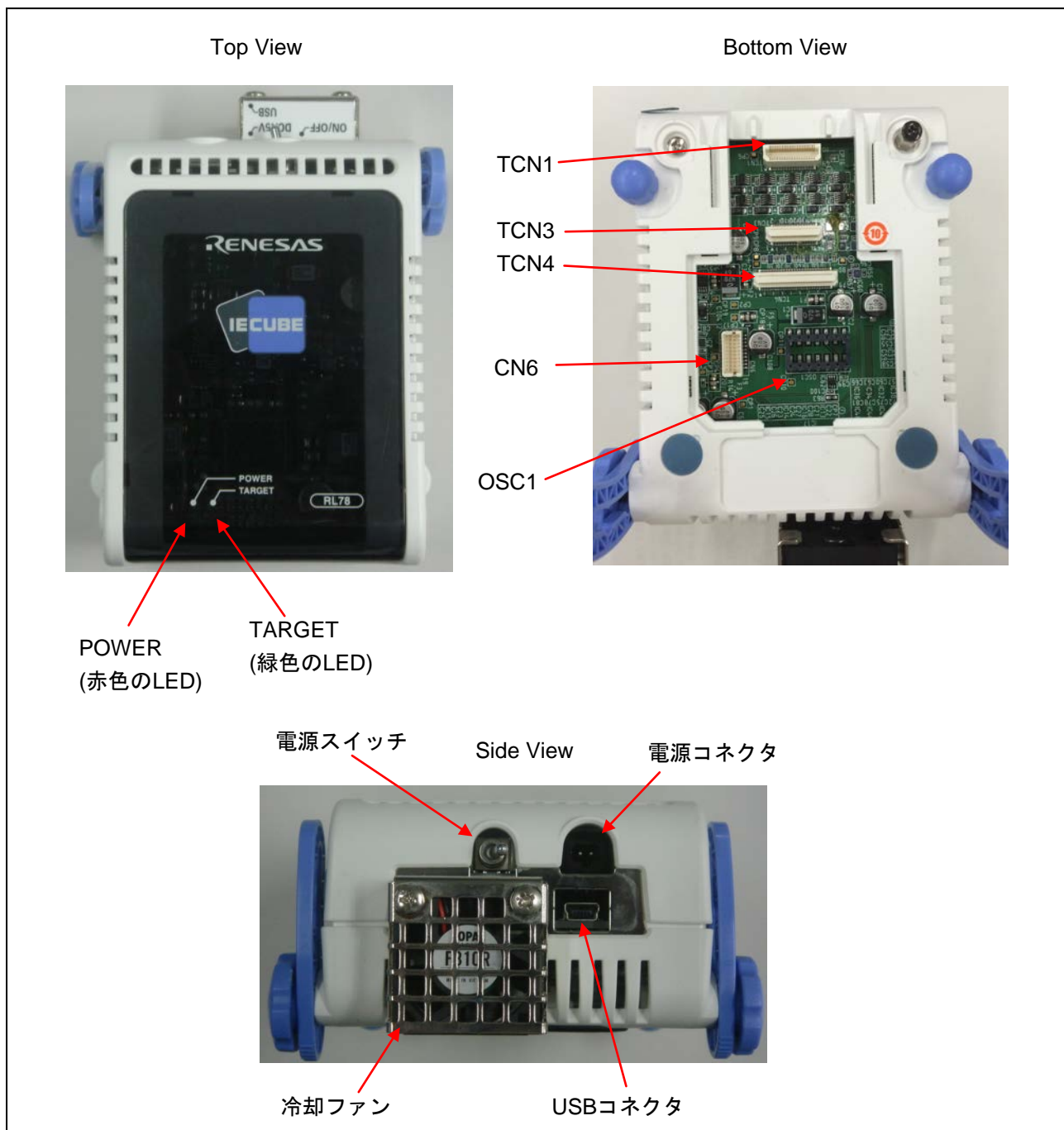
図1-2 QB-RL78G1Fの各部の名称
