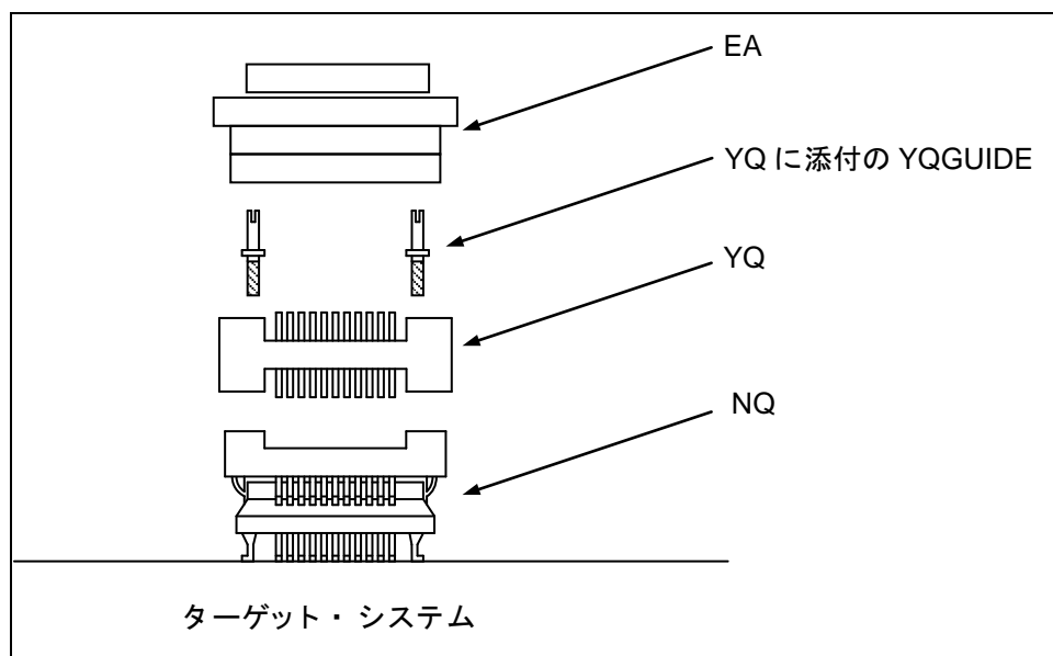
図2-6 EA, YQ, NQの実装図
