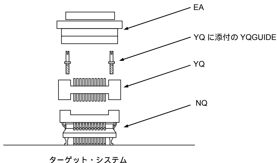
図2-6 EA,YQ,NQの実装図
