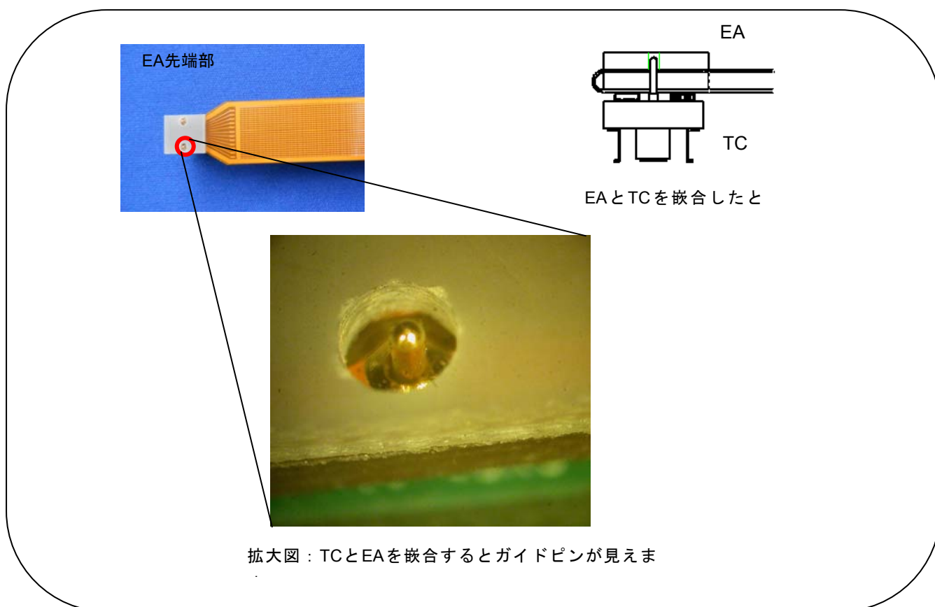
図2-5 TCとEAを嵌合したときのガイド穴拡大図と嵌合図
