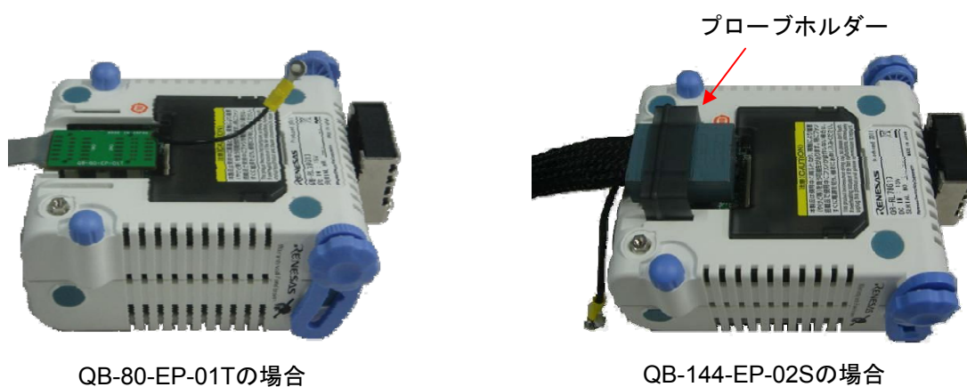
図2-7 エミュレーション・プローブの接続方法
