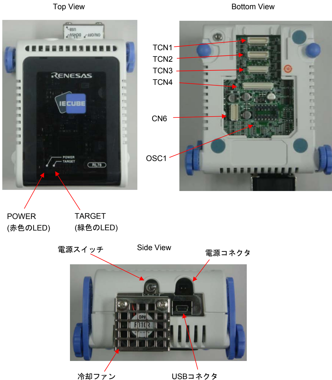
図1-1 QB-RL78F14の各部の名称
