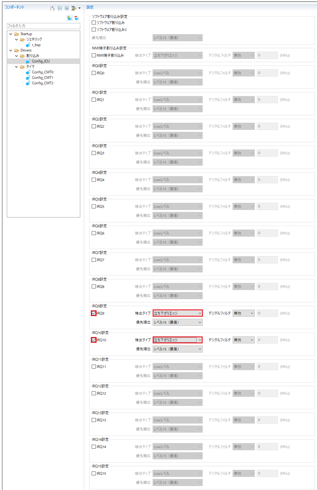
図 4-22: Config_ICU 設定
