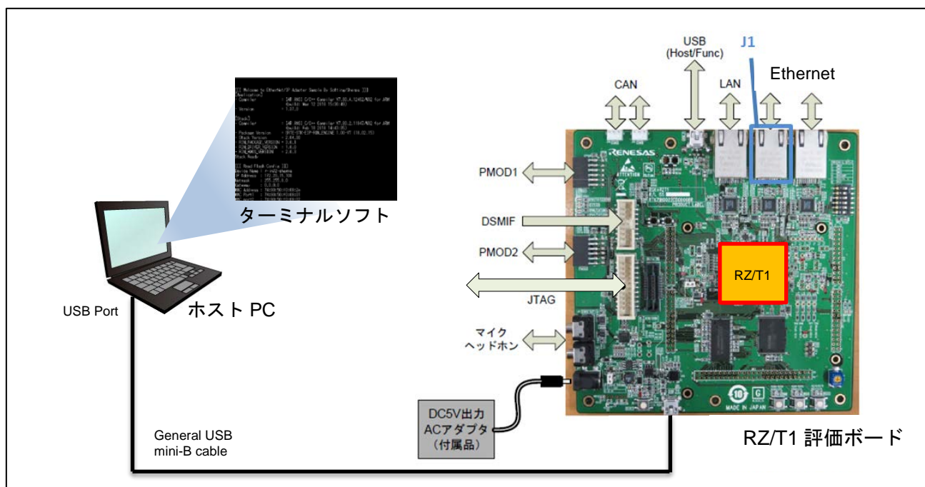
図 A.1 システム構成図
