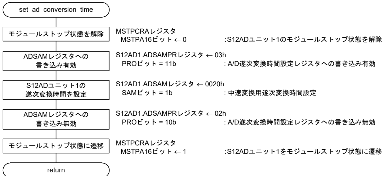
図 3.19 A/D 逐次変換時間の設定
