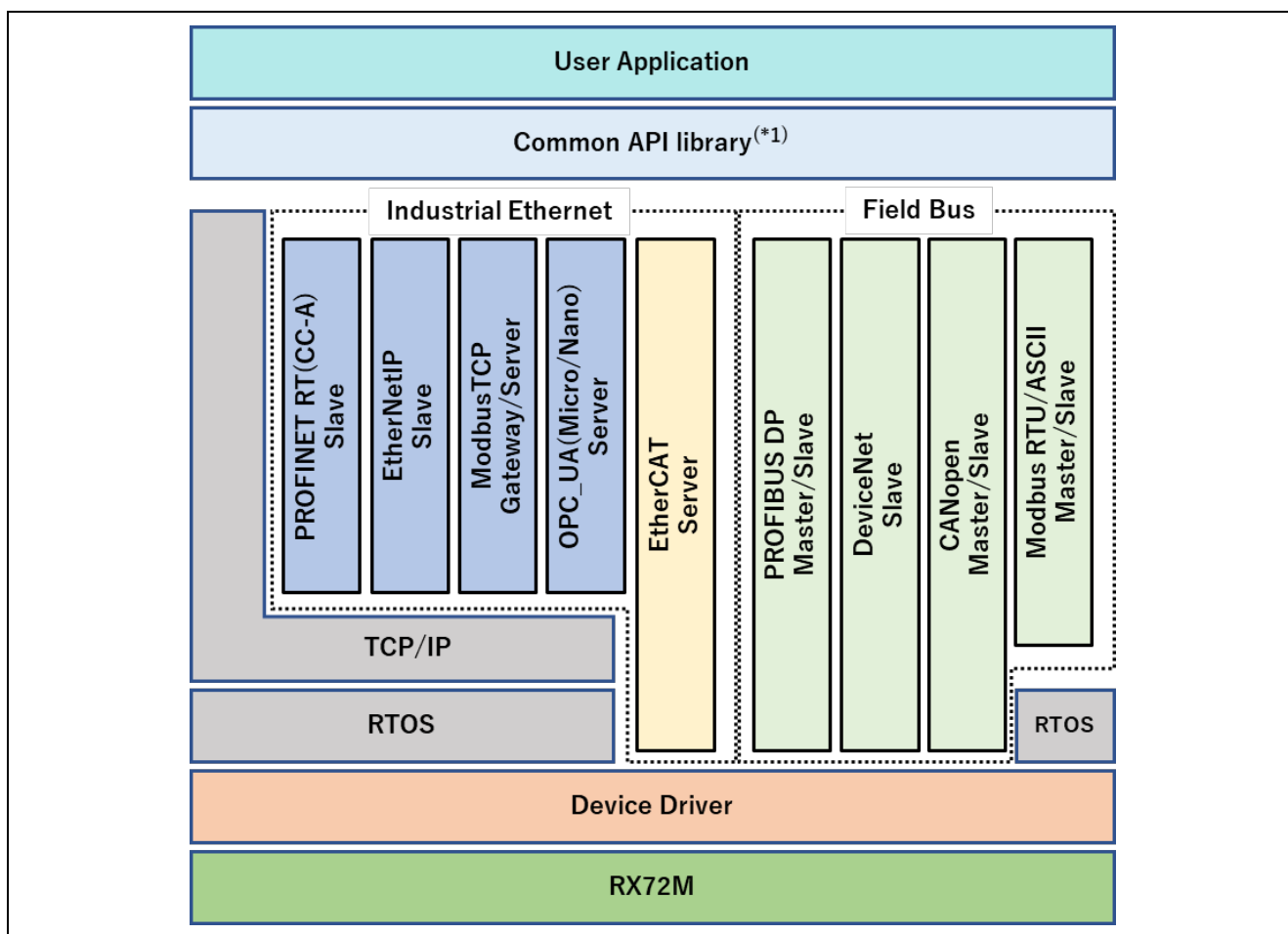
図 2.1 RX72M プロトコルスタックソフトウェア全体構成
