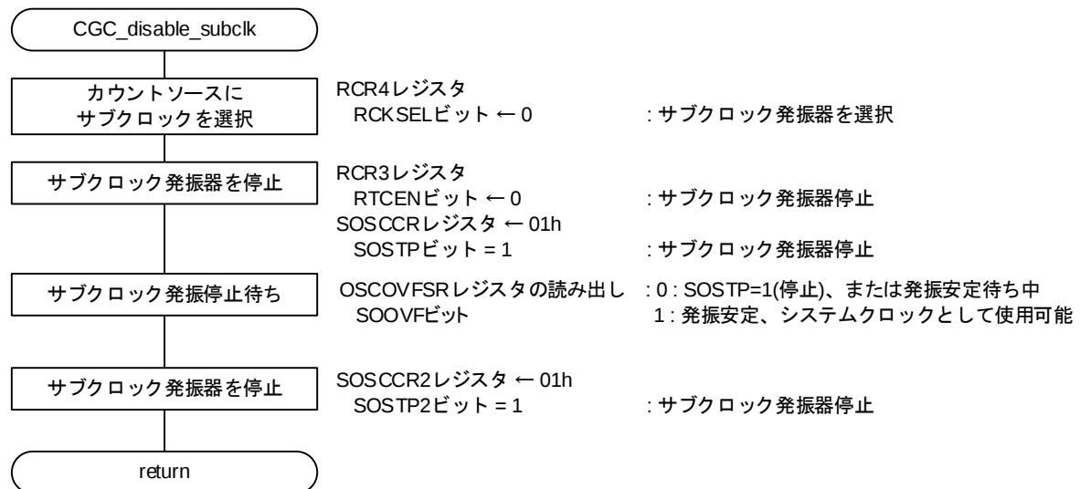
図 3.13 サブクロックの停止設定
