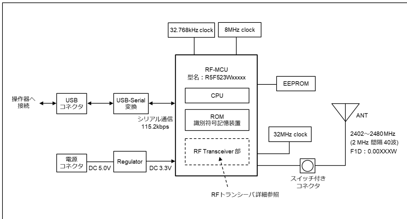
図 2-1 無線設備系統図（記載例）
