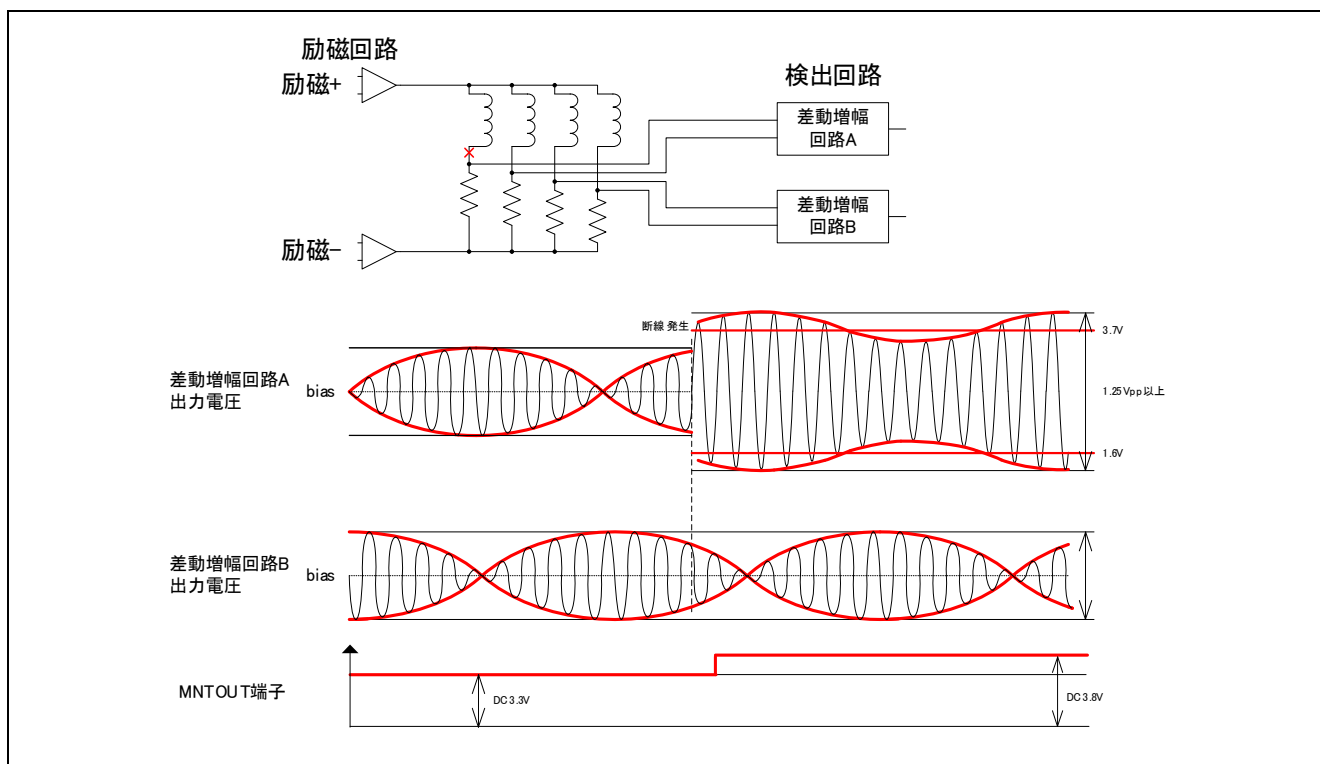
図 10.11 0 度一側断線
