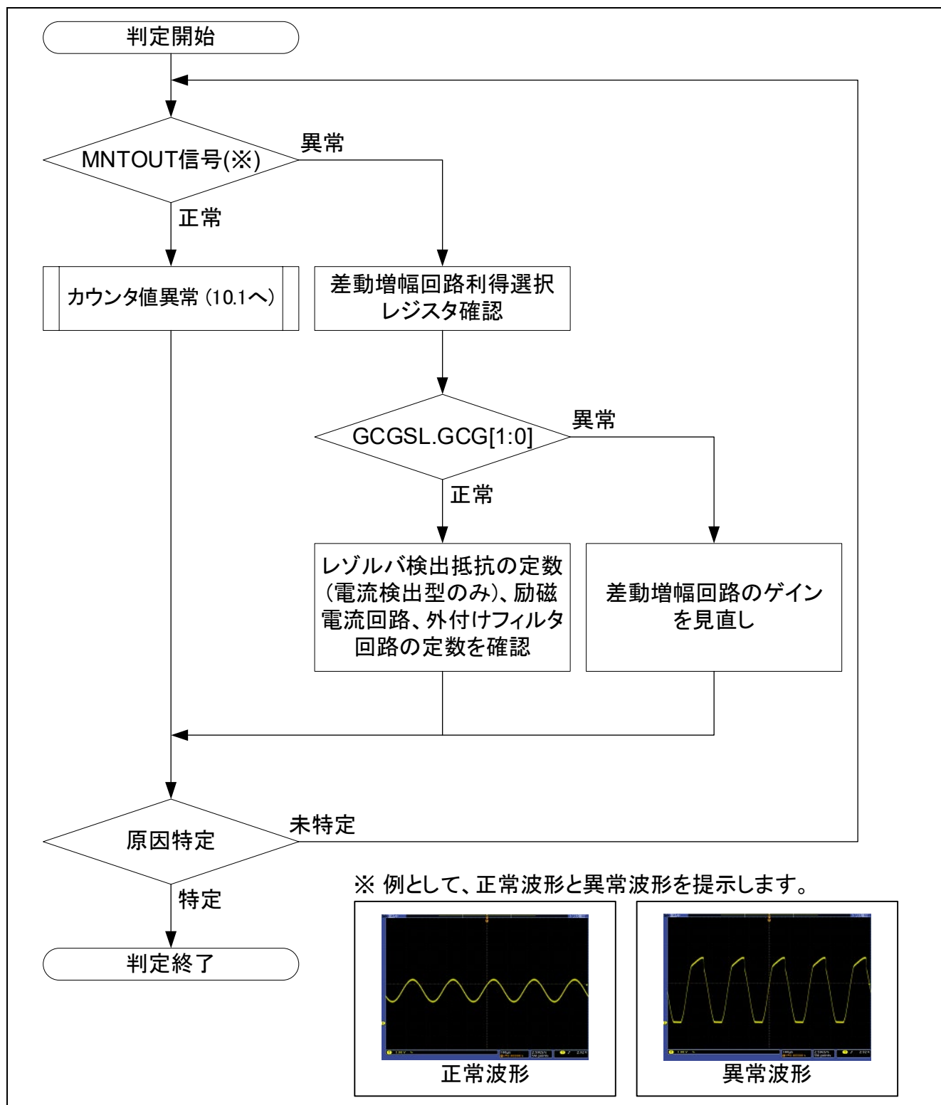
図 10.4 角度異常
