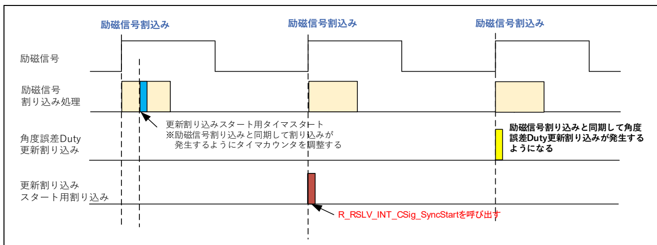
図 9.2 解消方法例
