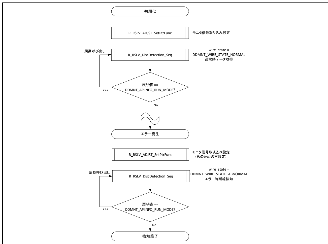
図 7.20 断線検知シーケンス例
