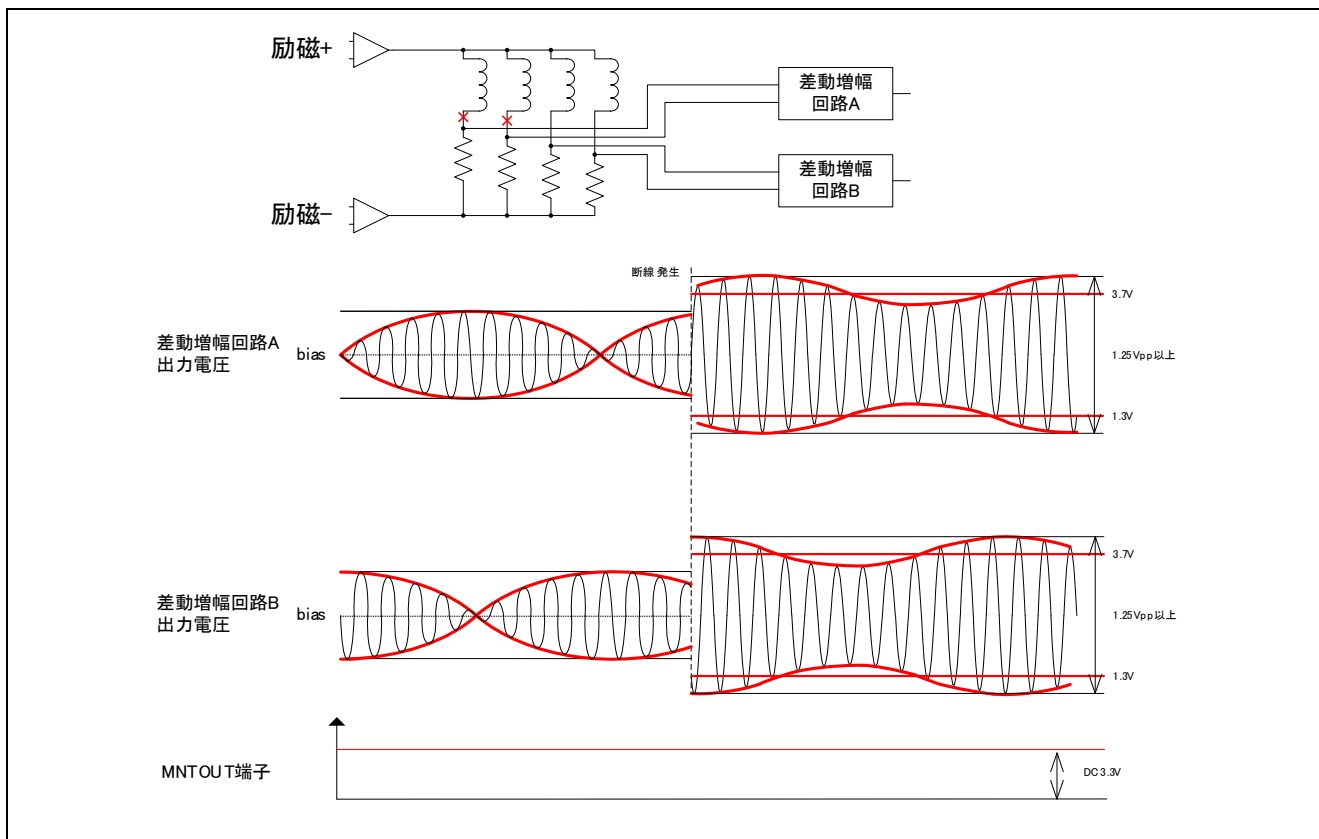
図 10.13 0 度、90 度一側断線
