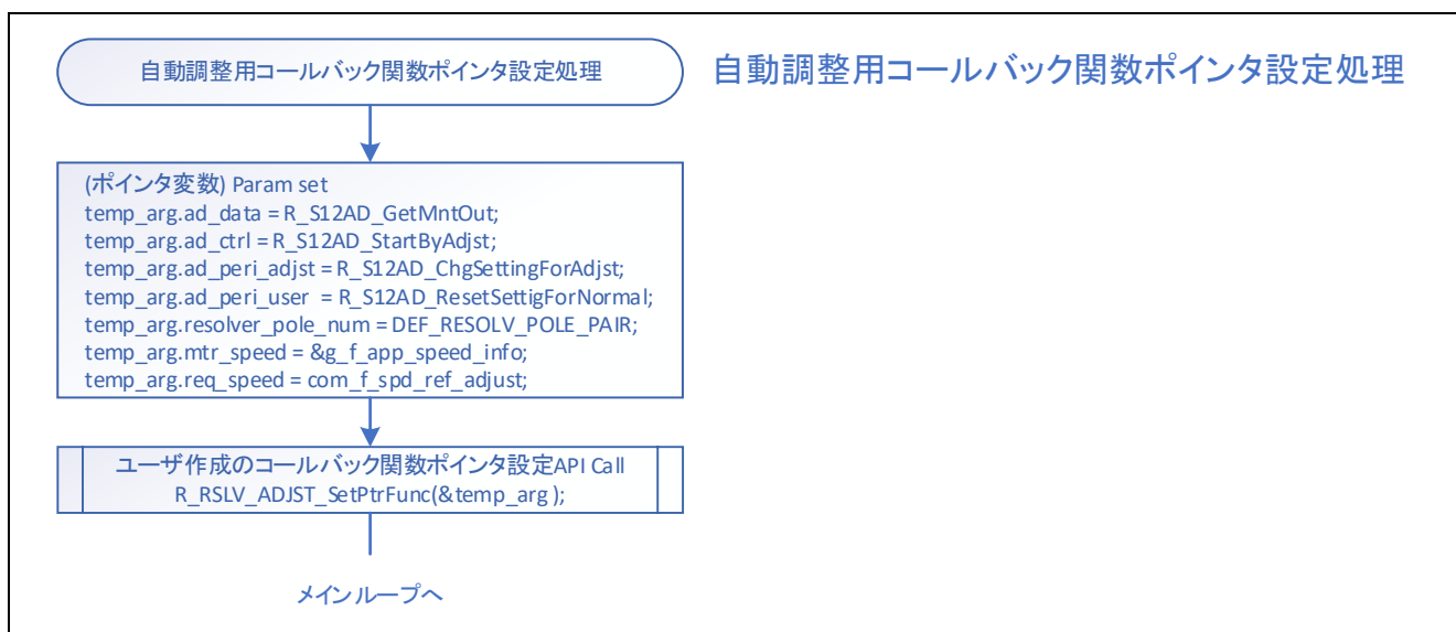
図 7.5 自動調整用初期設定（関数ポインタ設定）処理
