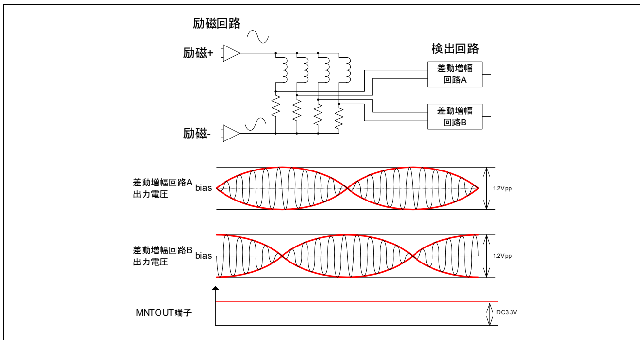
図 10.9 通常時
