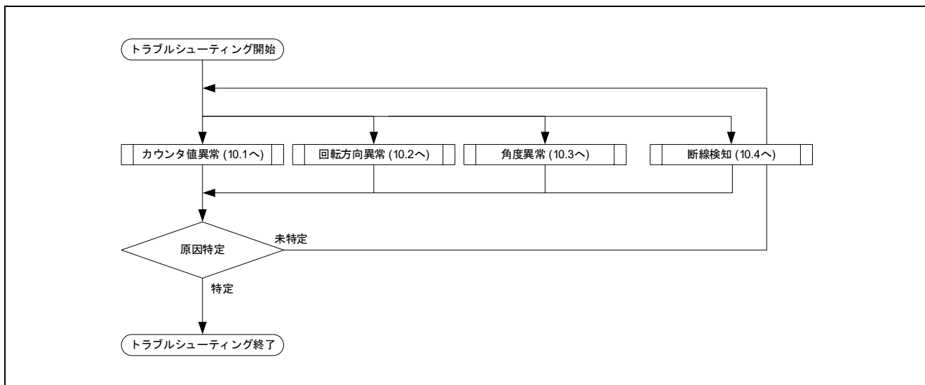
図 10.1 トラブルシューティング全体フロー
