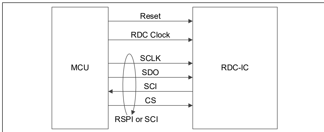
図 3.4 RDC-IC 通信ブロックシステム概要
