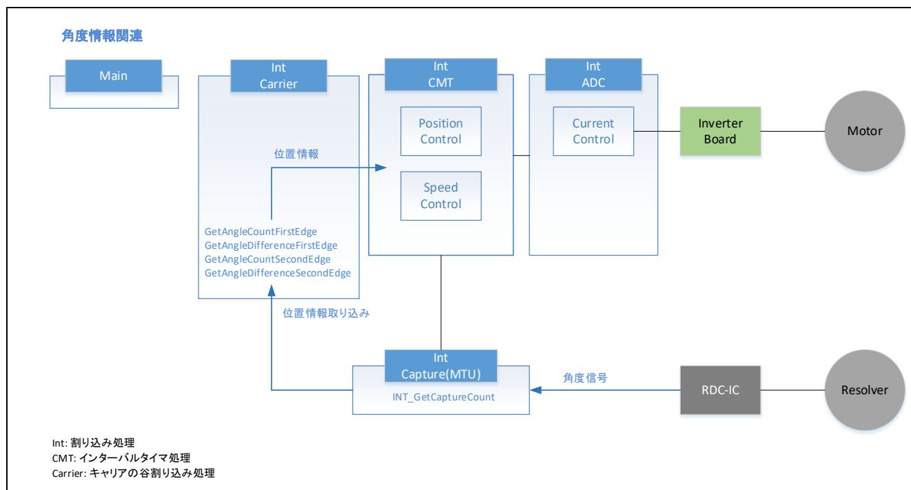
図 7.11 角度信号入力実装例
