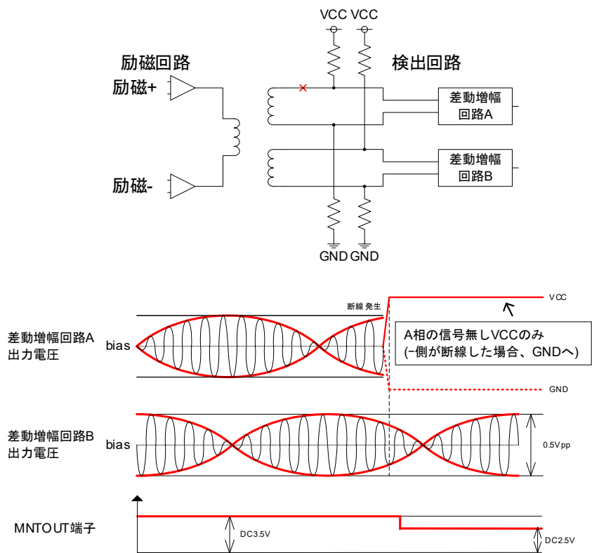
図 10.7 SIN+側断線
