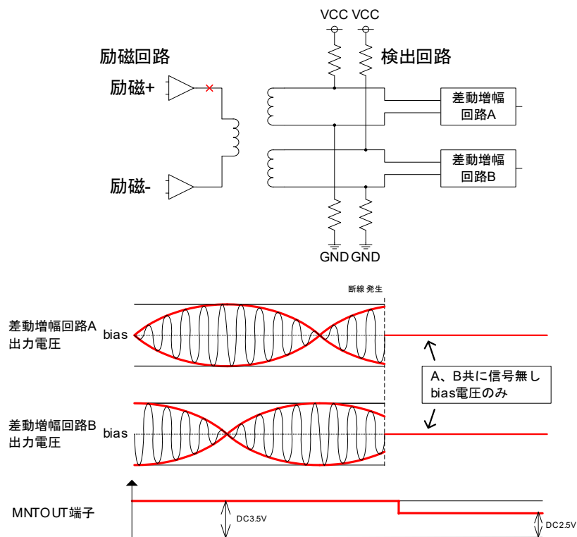
図 10.6 励磁側断線
