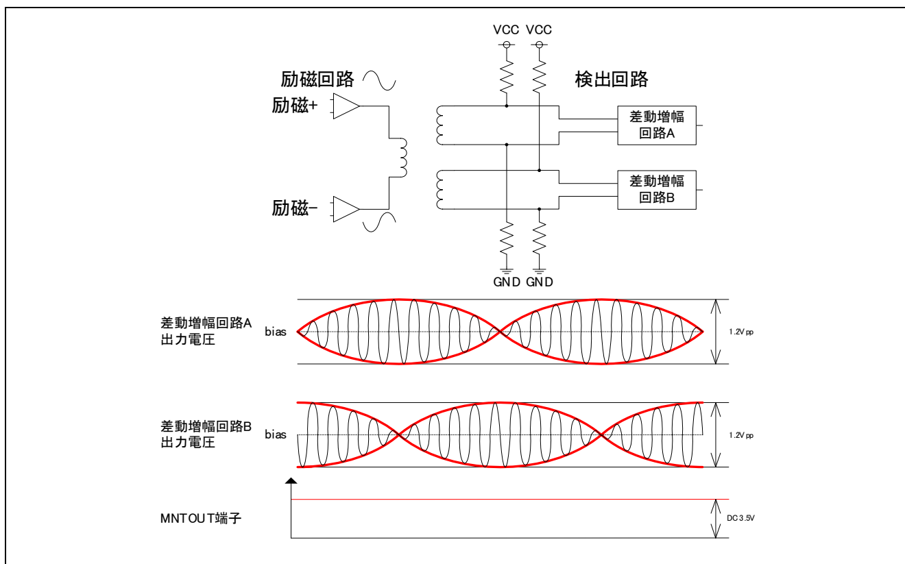
図 10.5 通常状態
