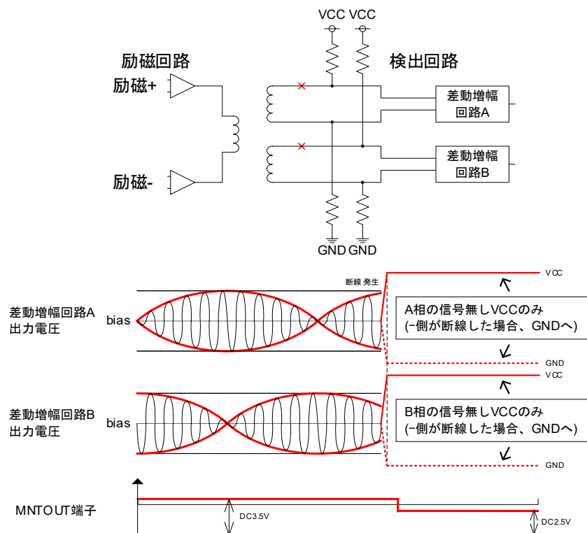
図 10.8 SIN+、COS+側断線
