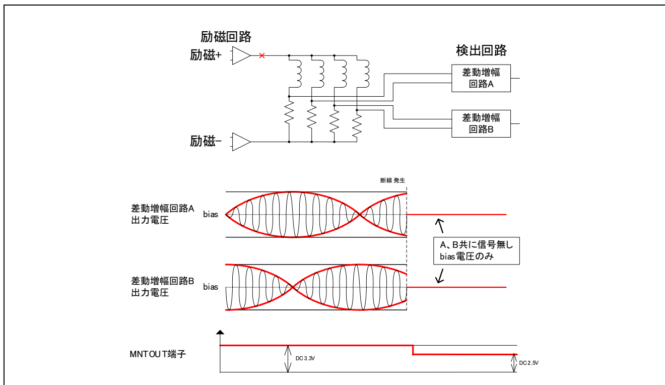
図 10.10 励磁側断線
