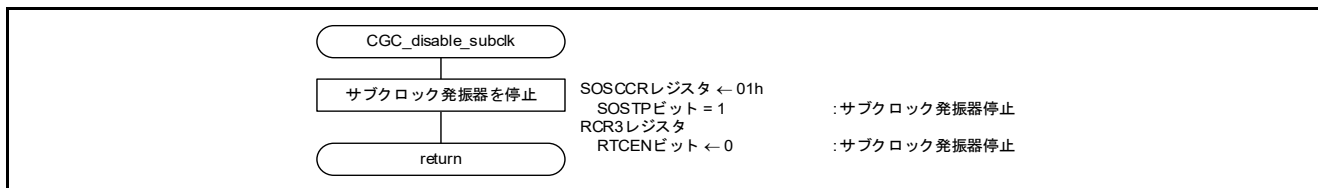
図4.12 サブクロックの停止設定
