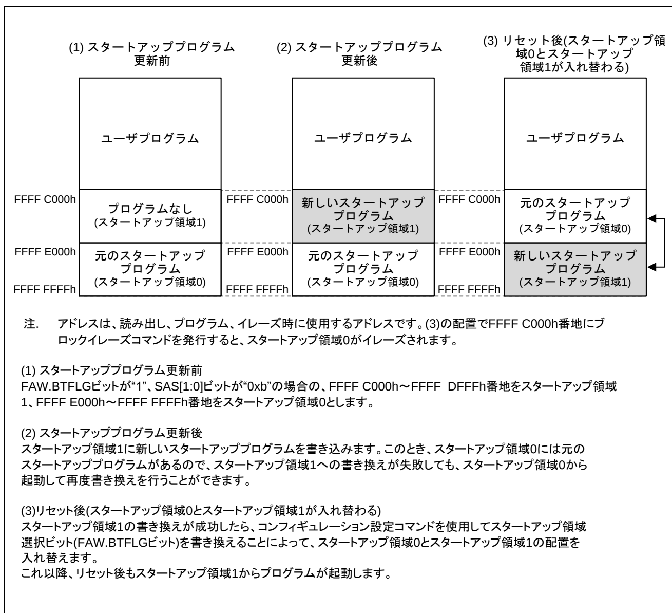
図 2.10 スタートアッププログラム保護機能の概念 (RX72M の場合)
