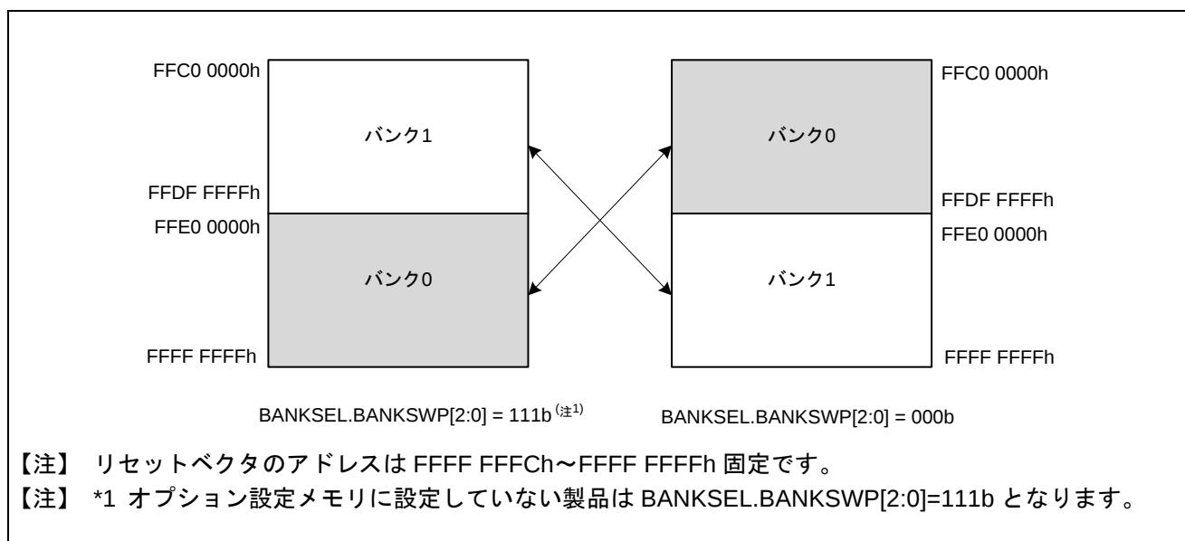
図 2.12 起動バンク選択例 (RX72M の場合)
