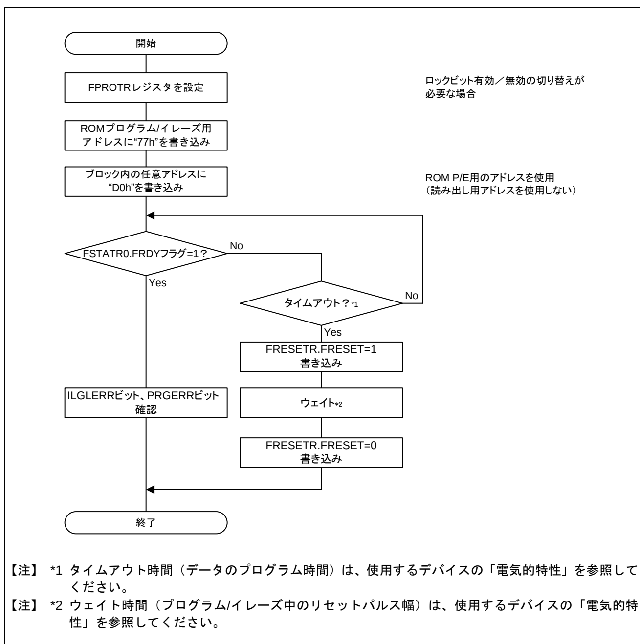
図 2.1 ロックビットプログラムコマンドの発行フロー1
