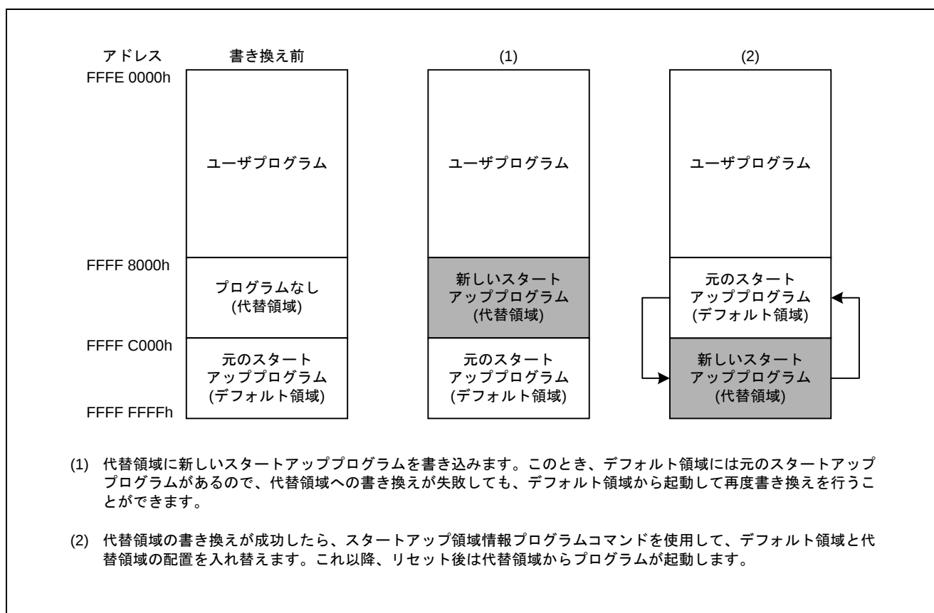
図 2.7 スタートアッププログラム保護機能の概念 (RX140 の場合)
