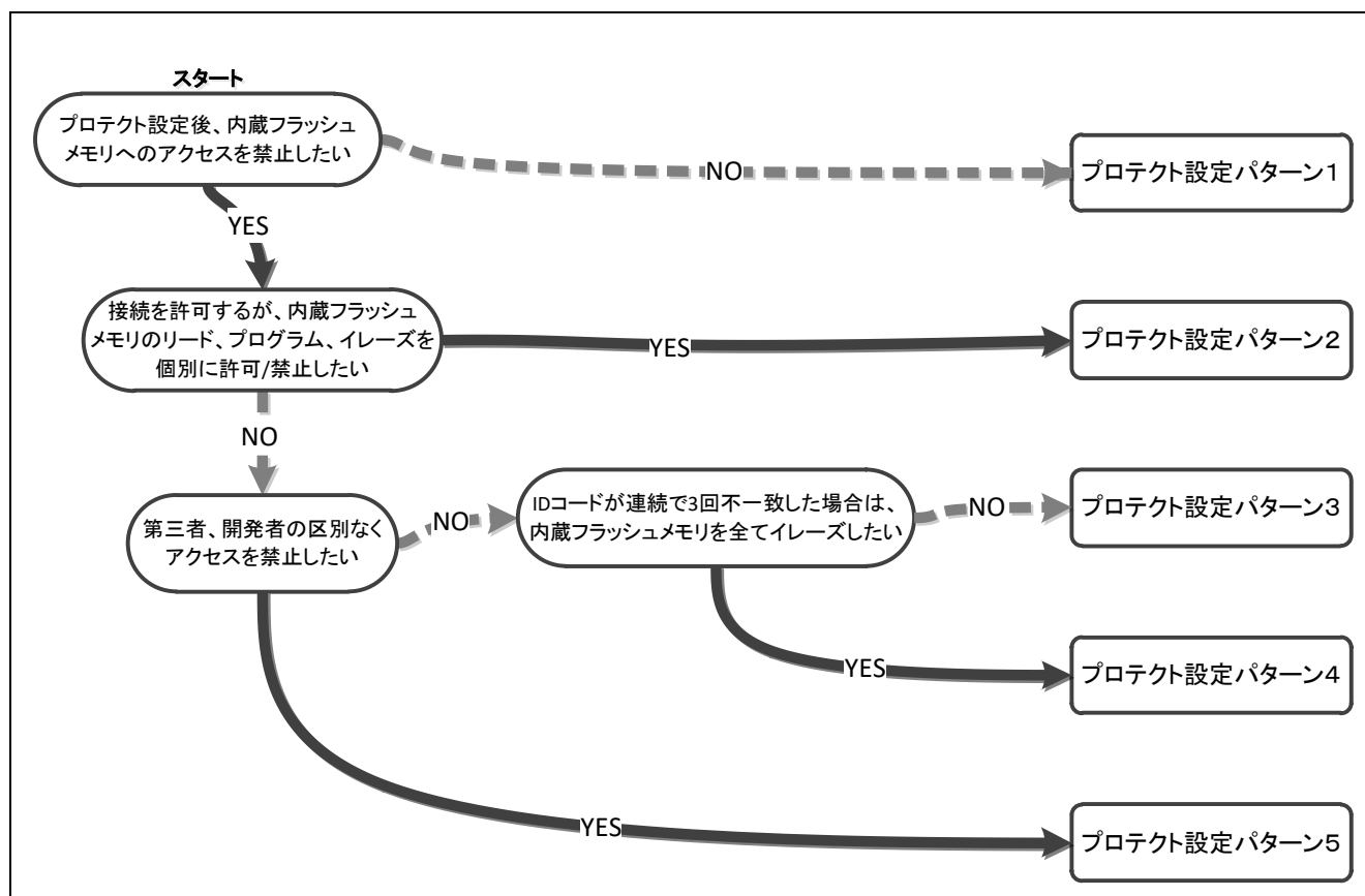
図 1.16 プロテクト設定パターン選択チャート
