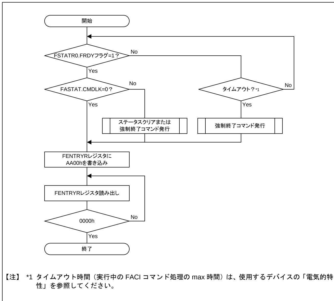
図 2.9 リードモードへの移行フロー
