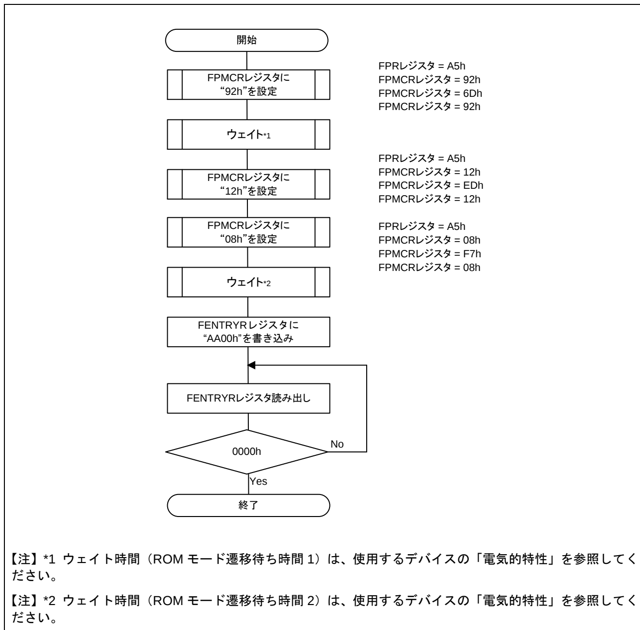
図 2.5 ROM P/E モードからリードモードへの移行フロー
