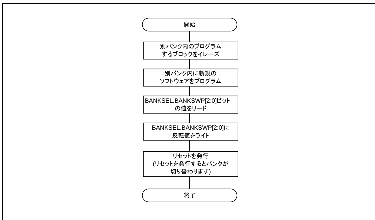
図 2.13 起動バンク切り替えフロー
