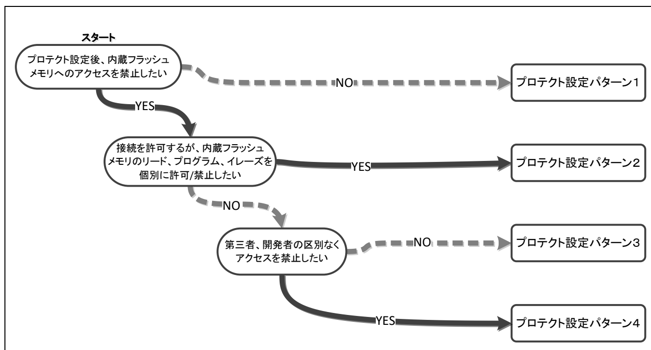
図 1.10 プロテクト設定パターン選択チャート
