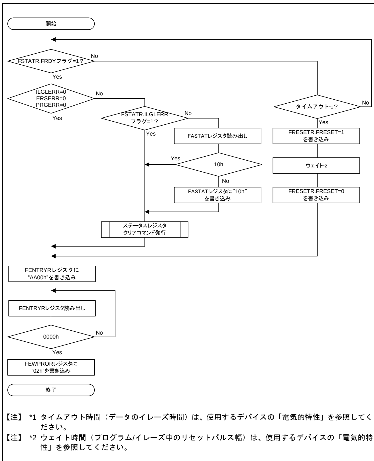
図 2.3 リードモードへの移行フロー1
