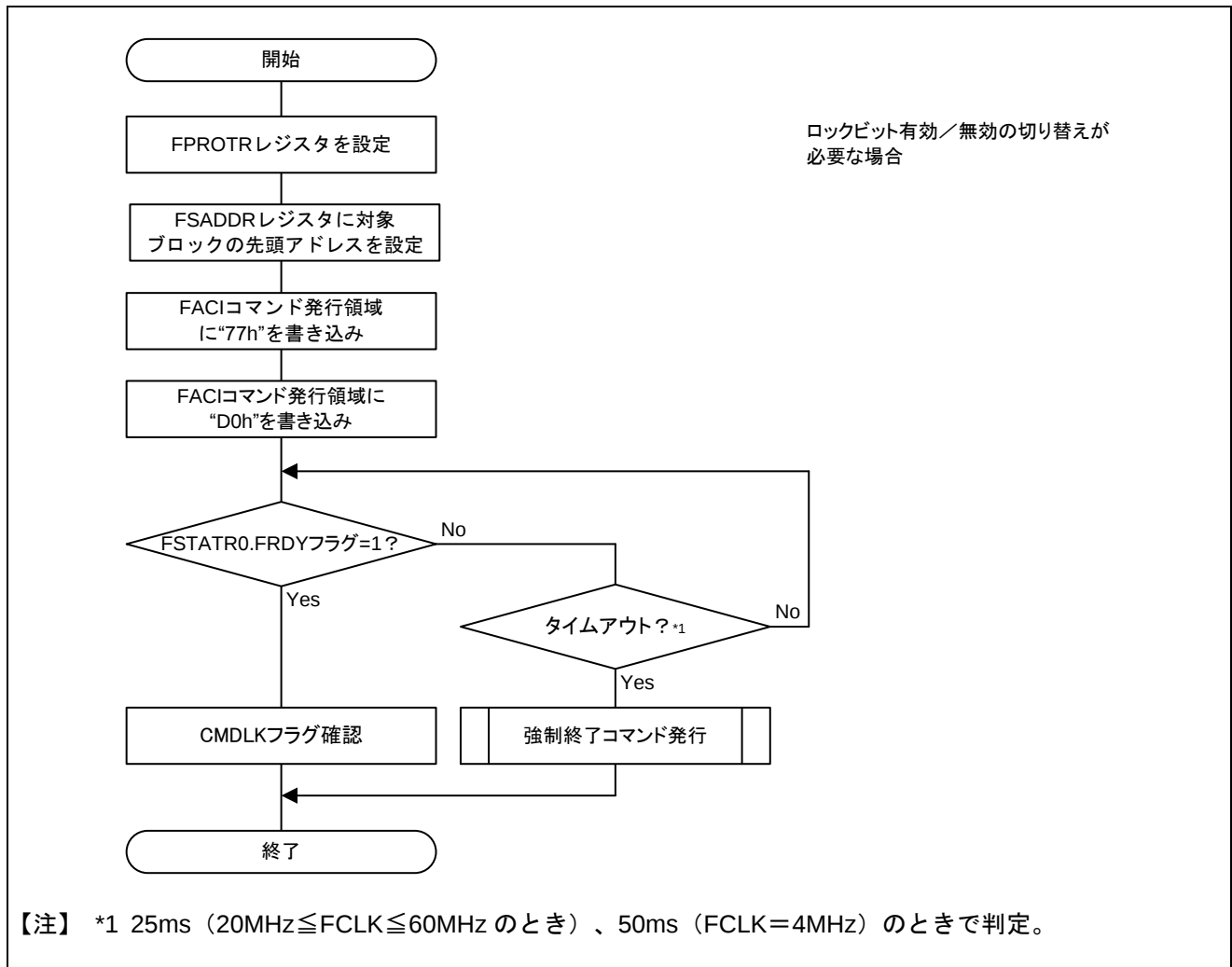
図 2.2 ロックビットプログラムコマンドの発行フロー2
