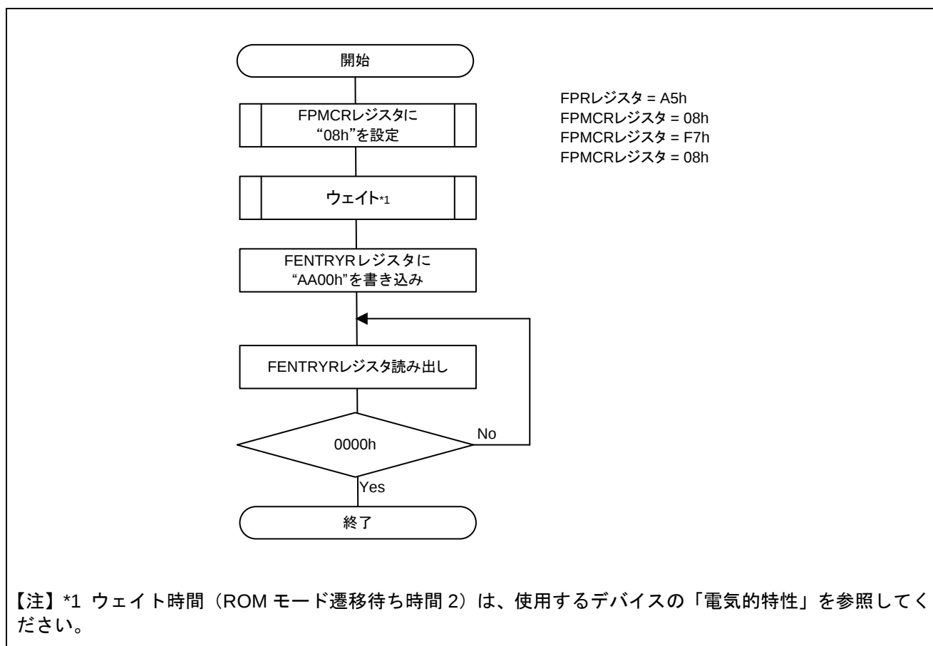
図 2.6 E2 データフラッシュ P/E モードからリードモードへの移行フロー
