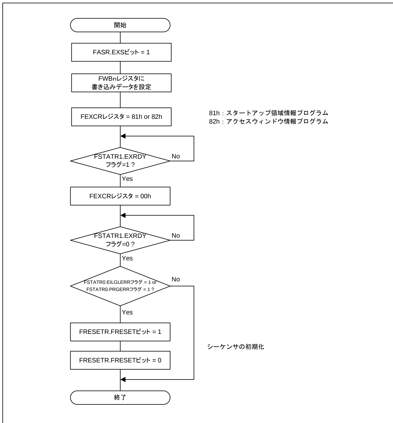
図 2.8 スタートアップ領域情報プログラムコマンド /アクセスウィンドウ情報プログラムコマンドの発行フロー
