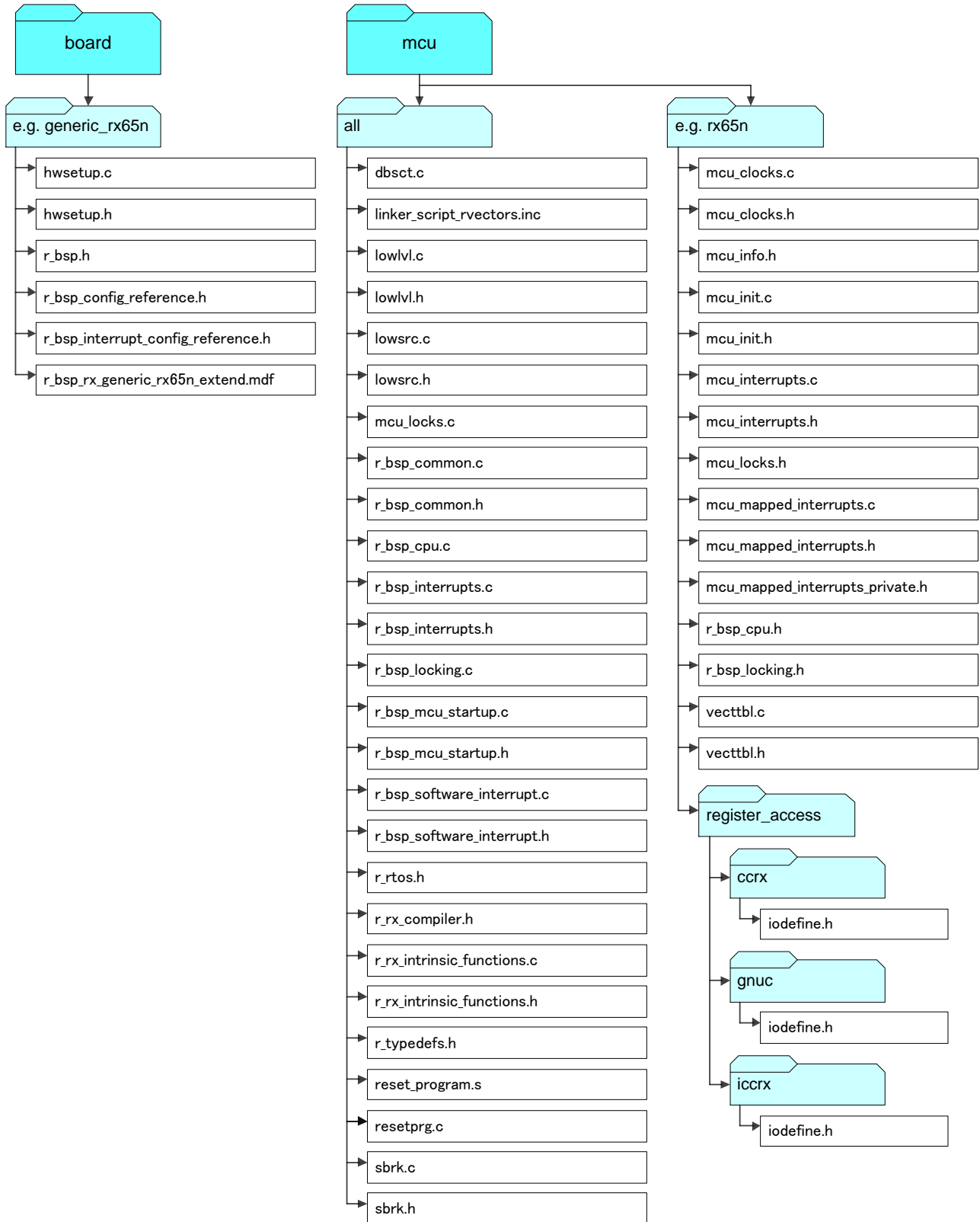
図 1.2 generic フォルダの構成
