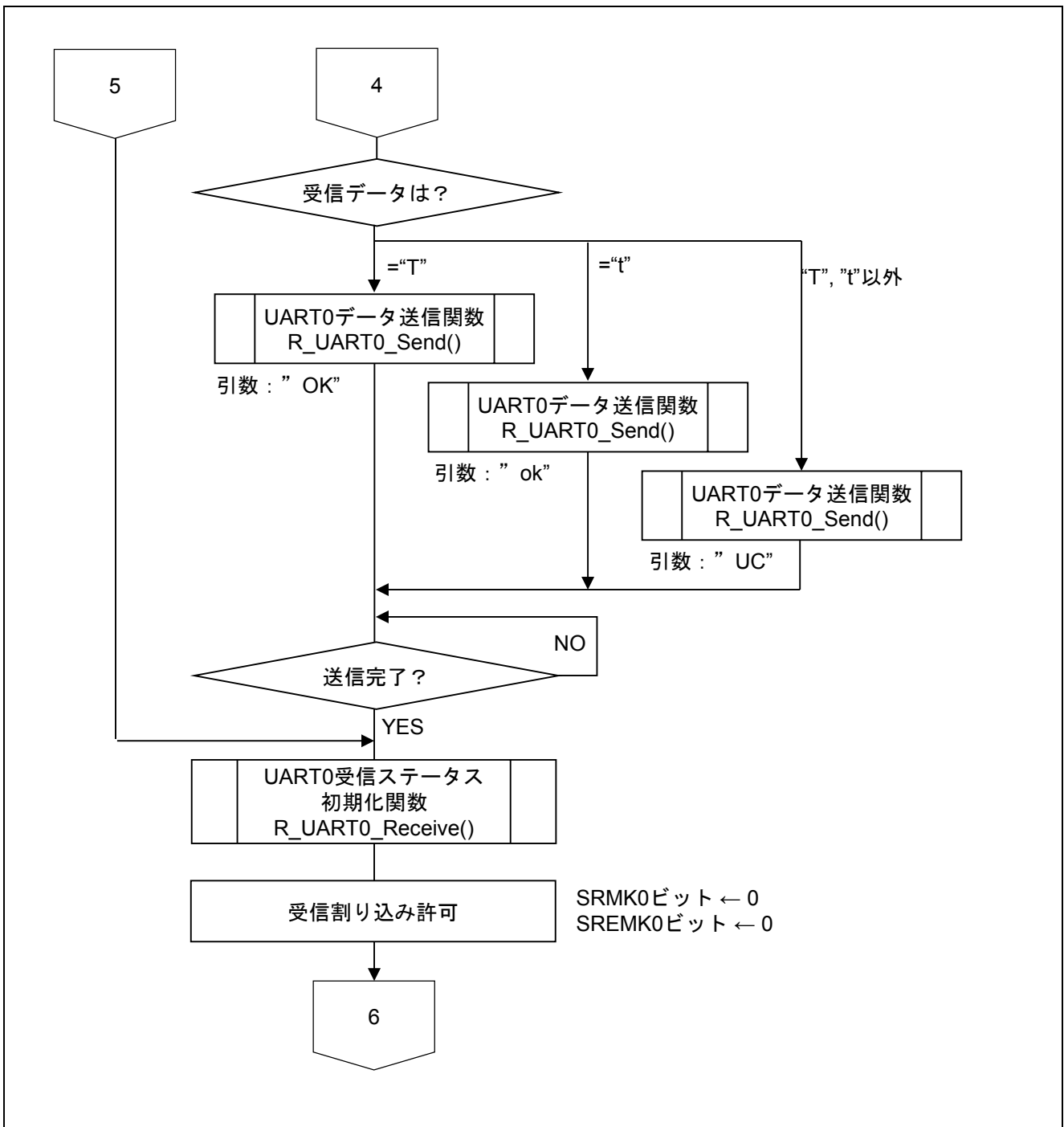
図 5.12 メイン関数 (3/3)
