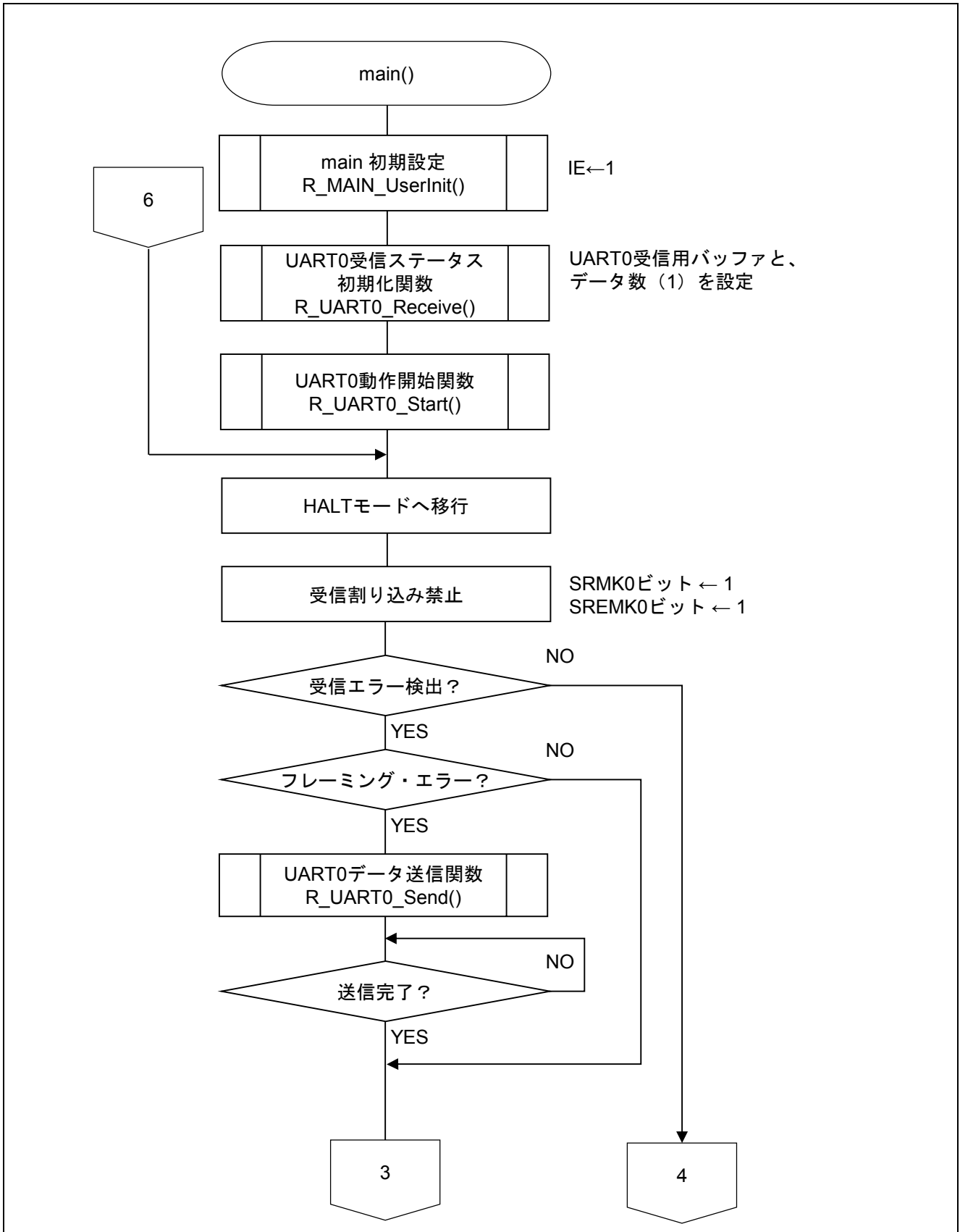
図 5.10 メイン関数 (1/3)
