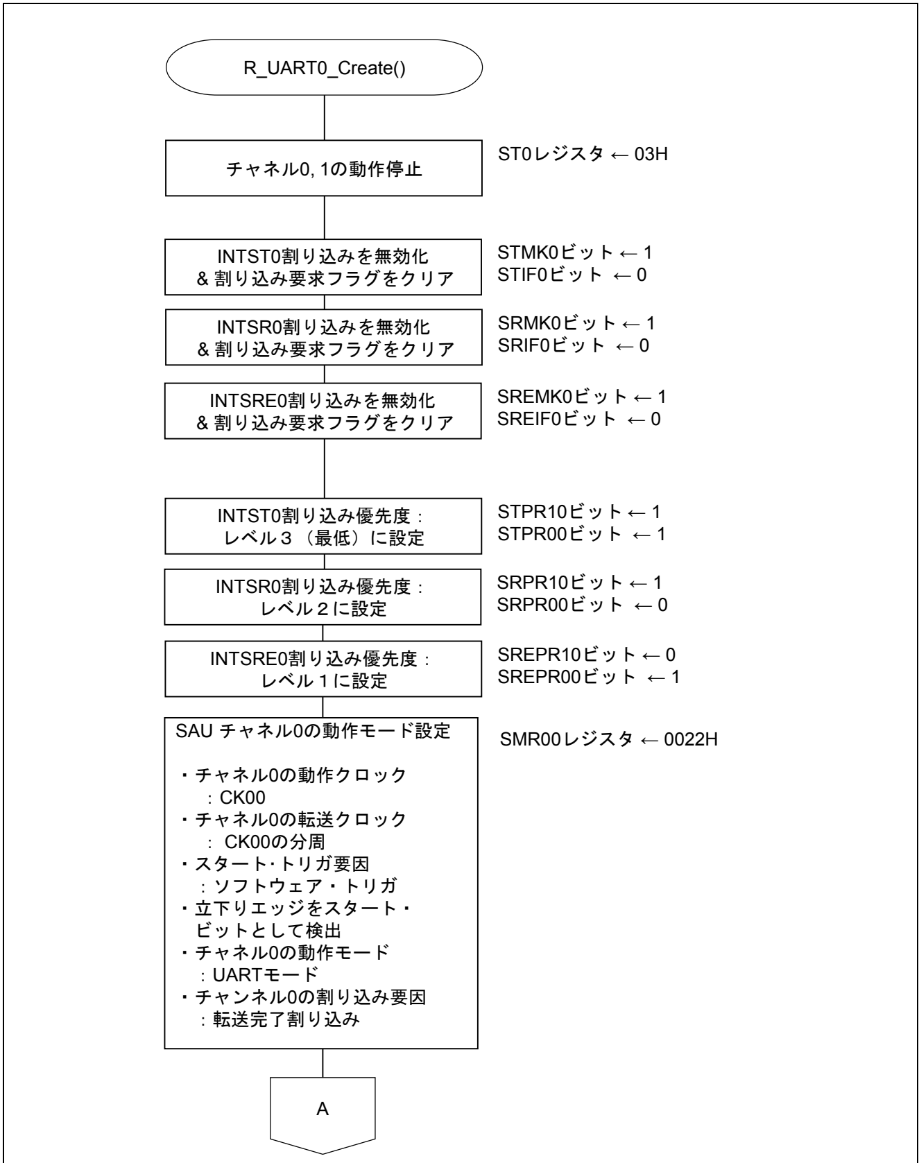
図 5.7 UART0 の設定 (1/3)
