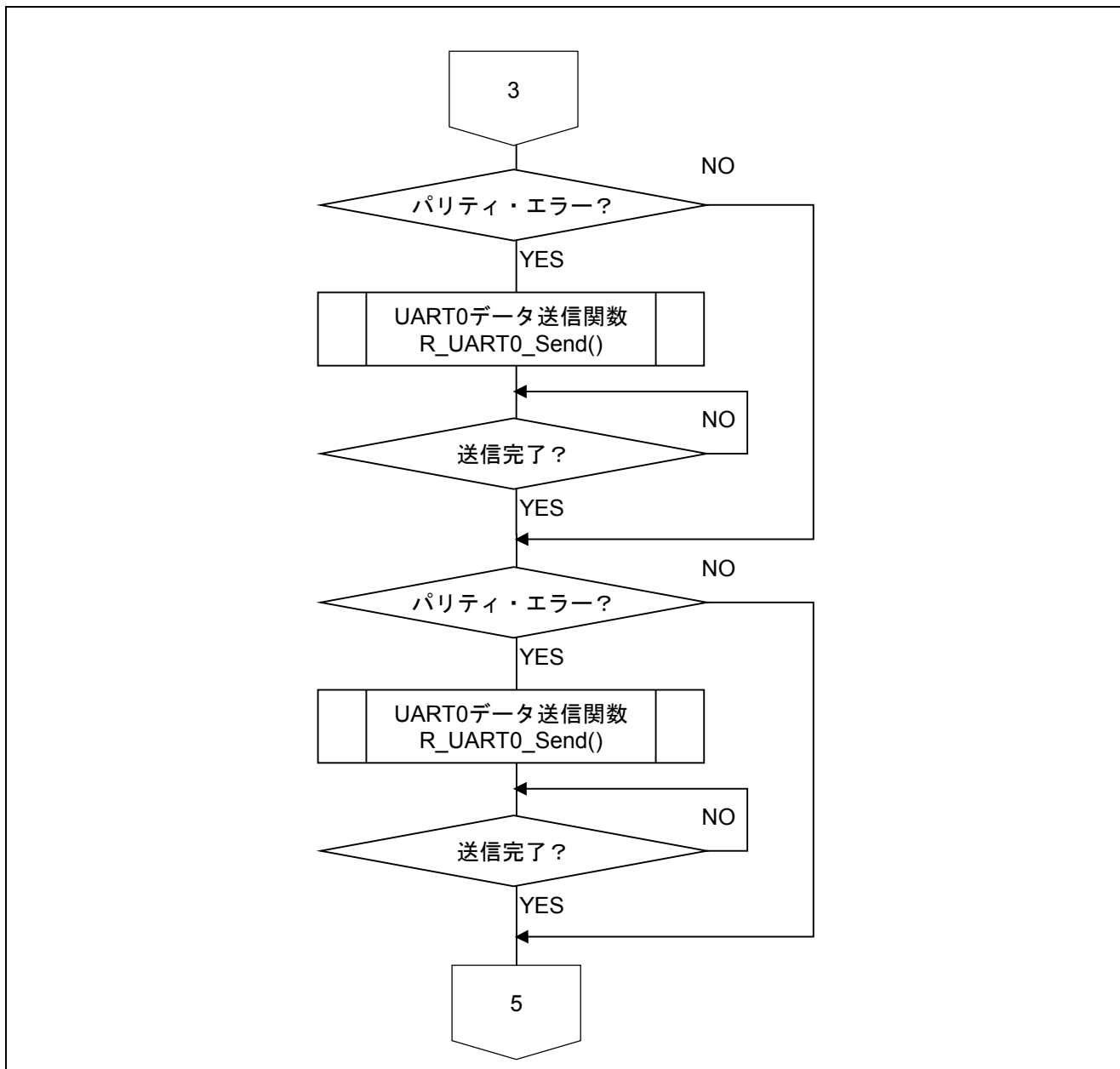
図 5.11 メイン関数 (2/3)
