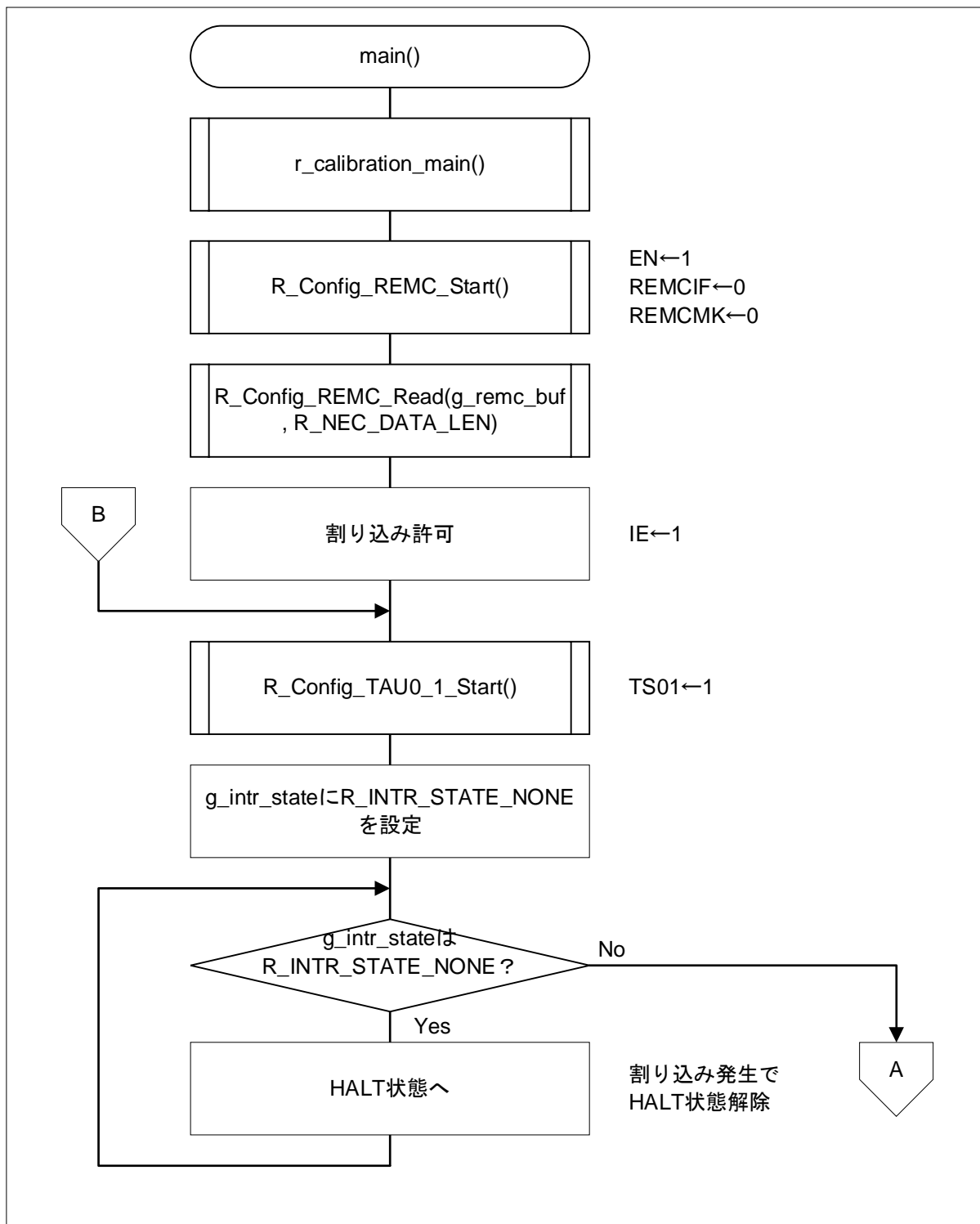
図 4-1 メイン処理 (1/2)
