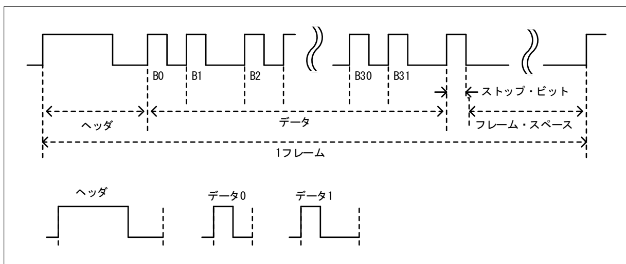
図 1-2 リモコン信号受信タイミング
