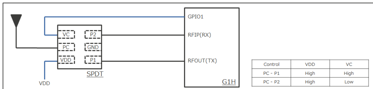
図 7 RL78/G1H との接続 (SPDT_1-control)
