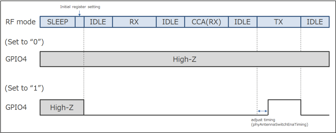
図 3 phyAntennaSwitchEna 設定値と GPIO4 タイミング
