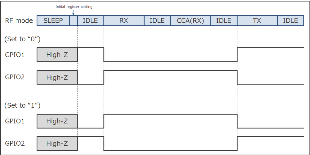
図 2 phyAntennaSelectTx 設定値と GPIO1/2 タイミング
