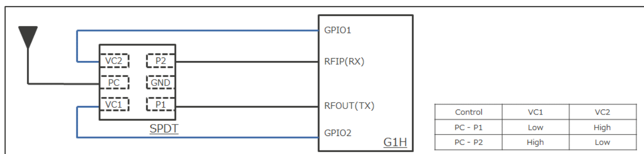
図 6 RL78/G1H との接続 (SPDT_2-control)
