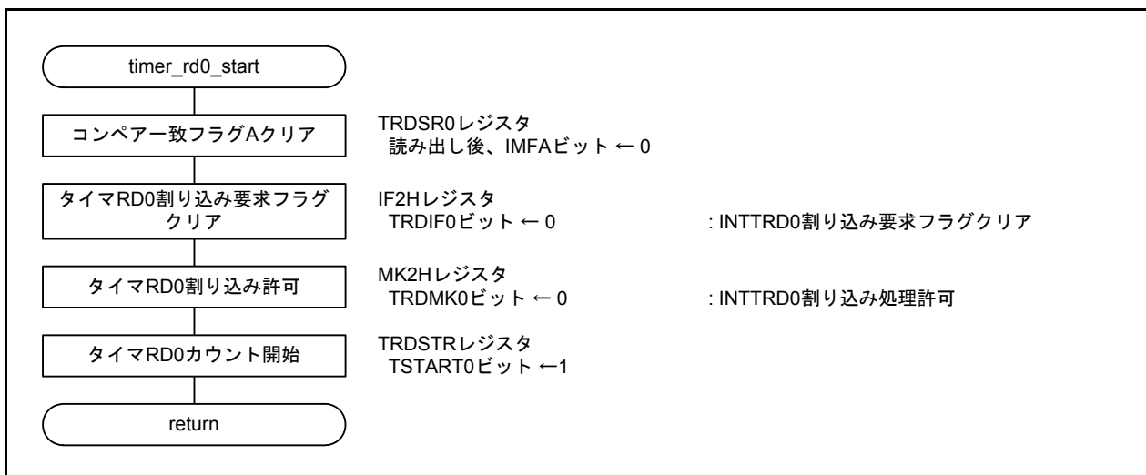
図 4.9 タイマRDカウント開始設定
