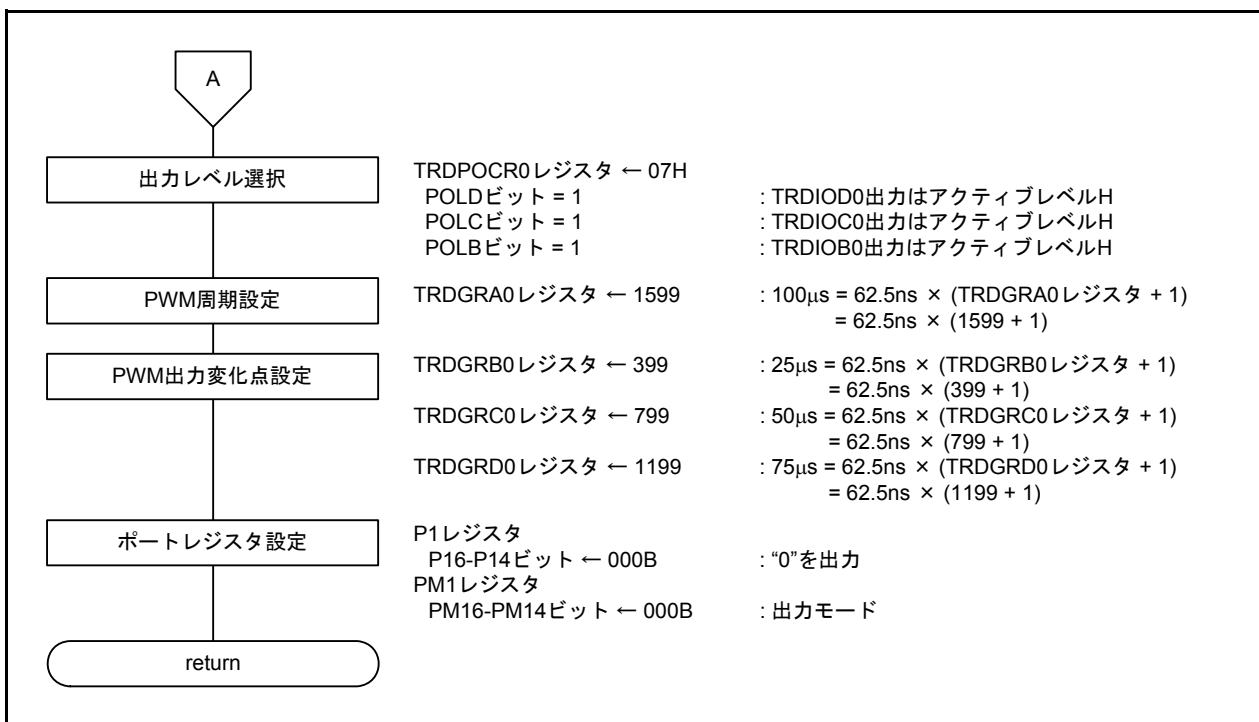
図 4.7 タイマRD初期設定(2/2)
