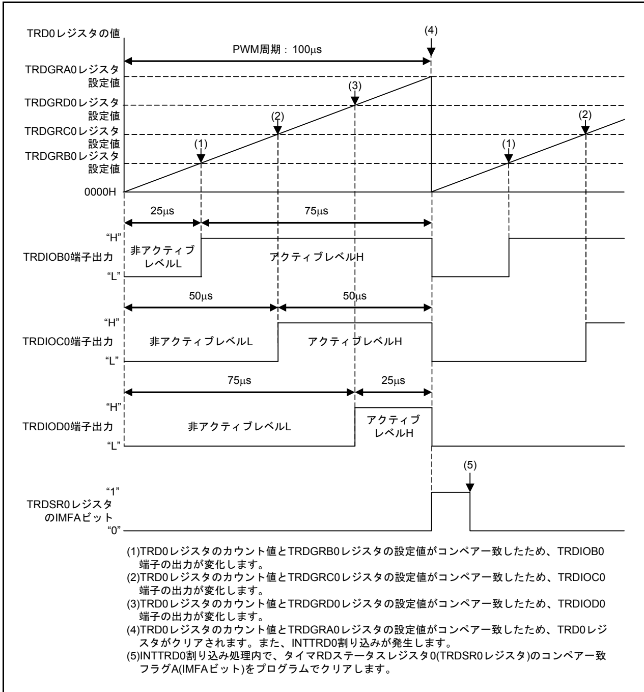
図 4.1 PWMの出力波形
