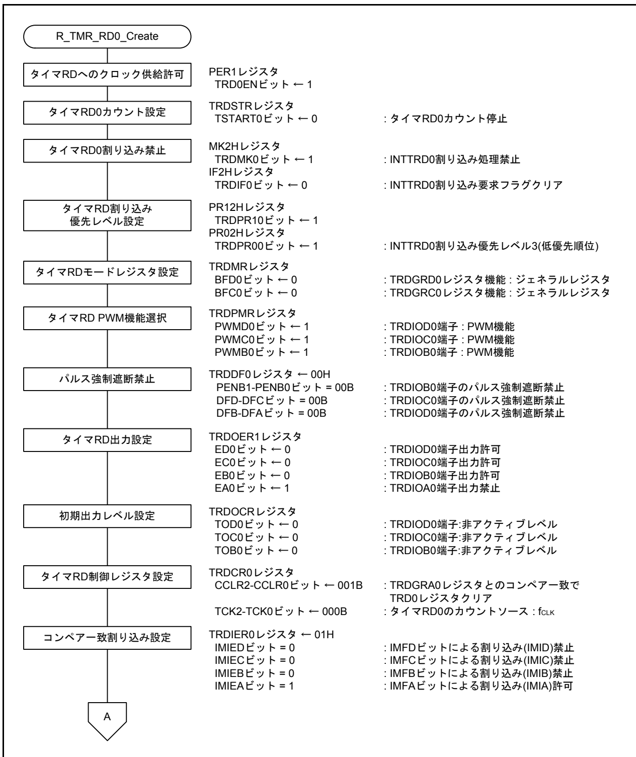
図 4.6 タイマRD初期設定(1/2)
