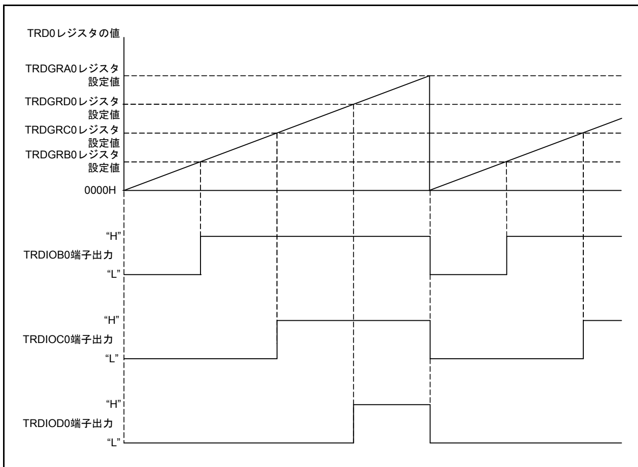
図 1.1 出力タイミング図
