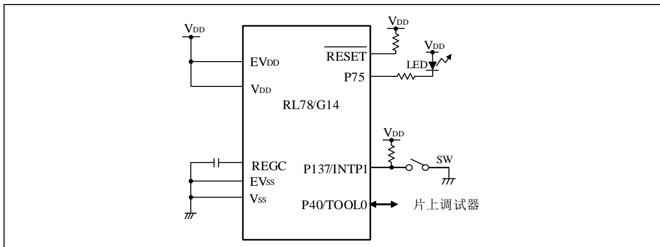
图 4.1 硬件配置
