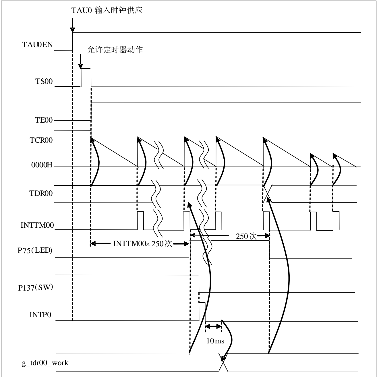
图 1.1 定时器及中断的动作概要
