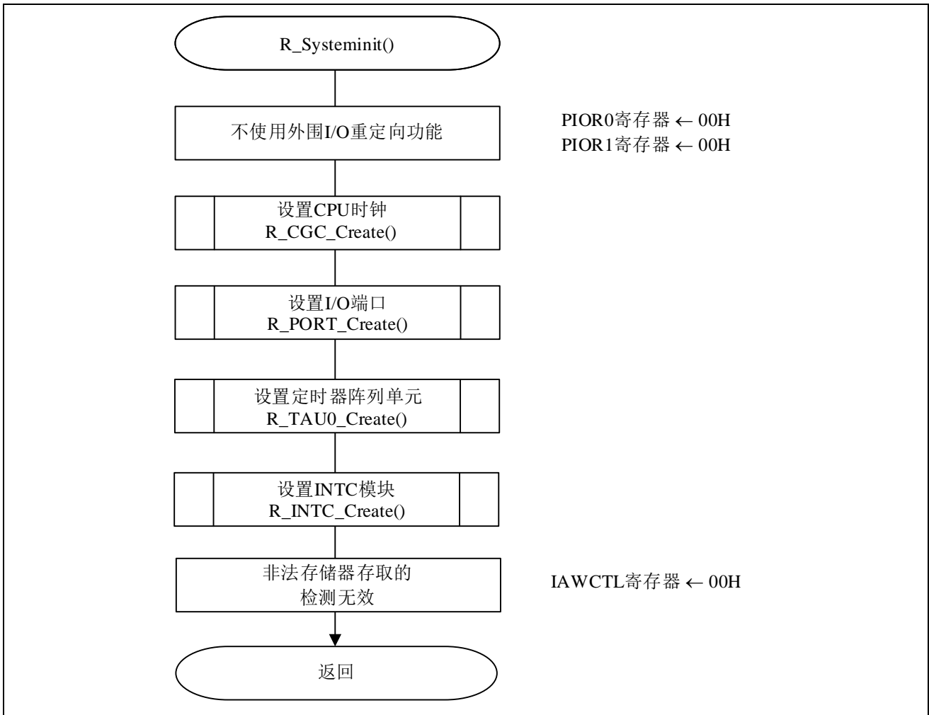
图 5.3 系统函数
