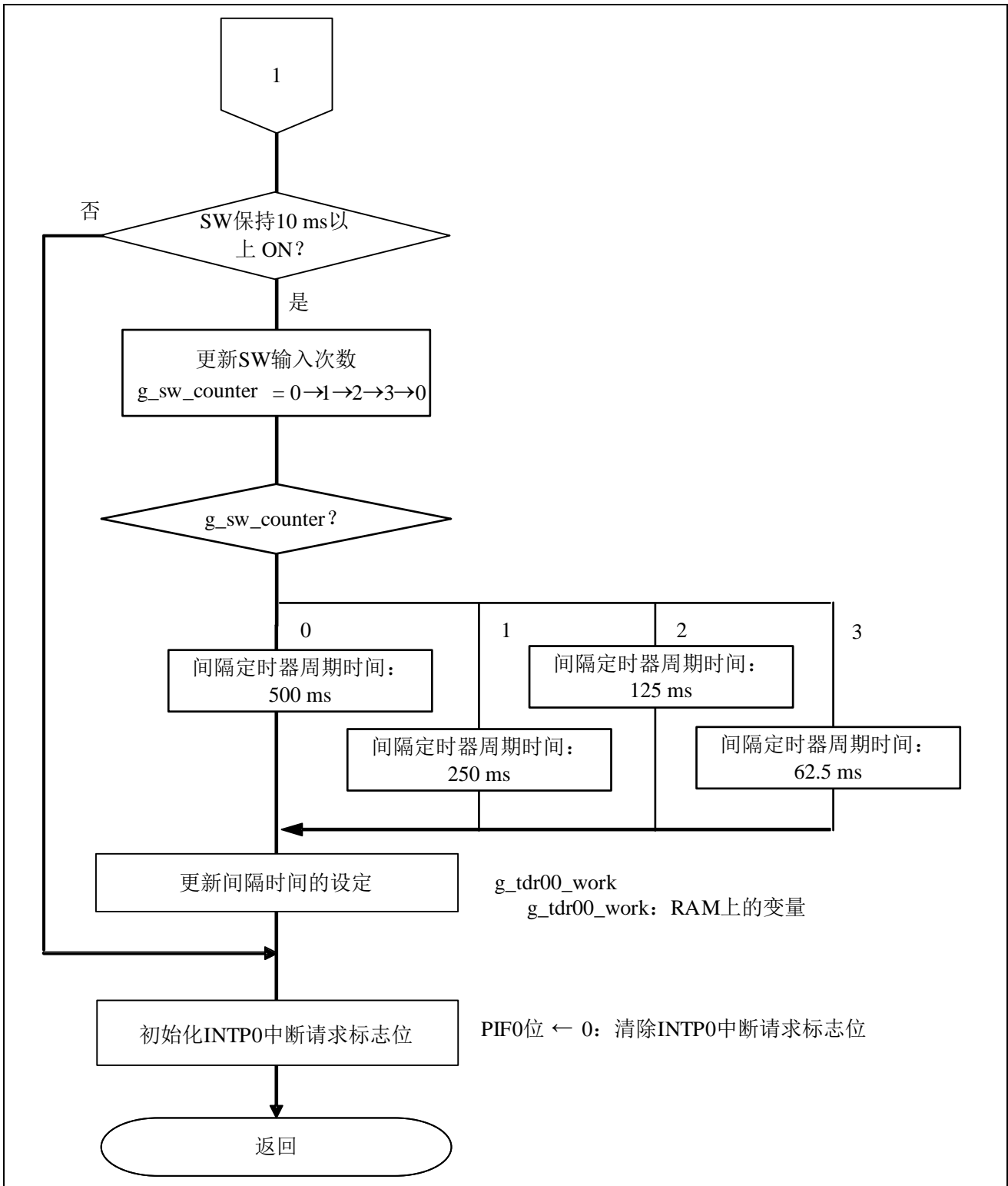
图 5.15 INTPO 中断处理 (2/2)
