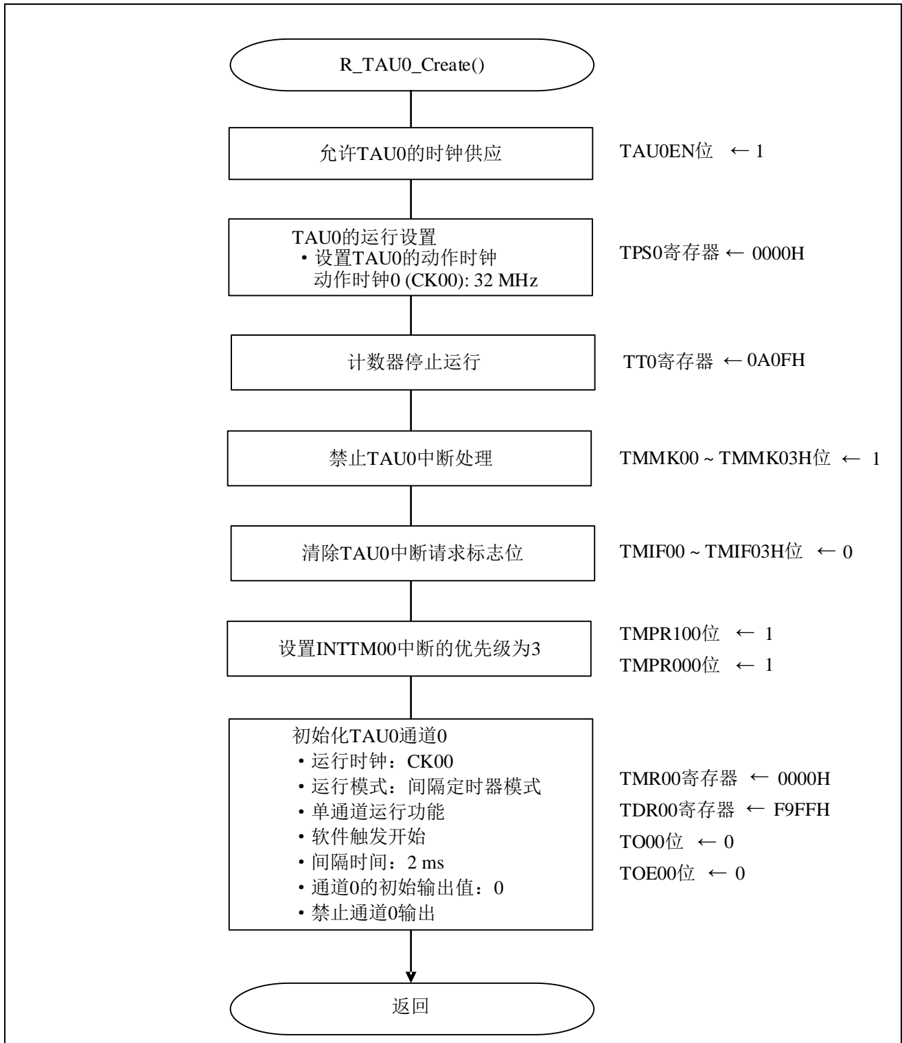
图 5.6 定时器阵列单元的设置
