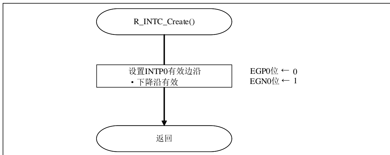
图 5.7 INTPO 的初始化函数
