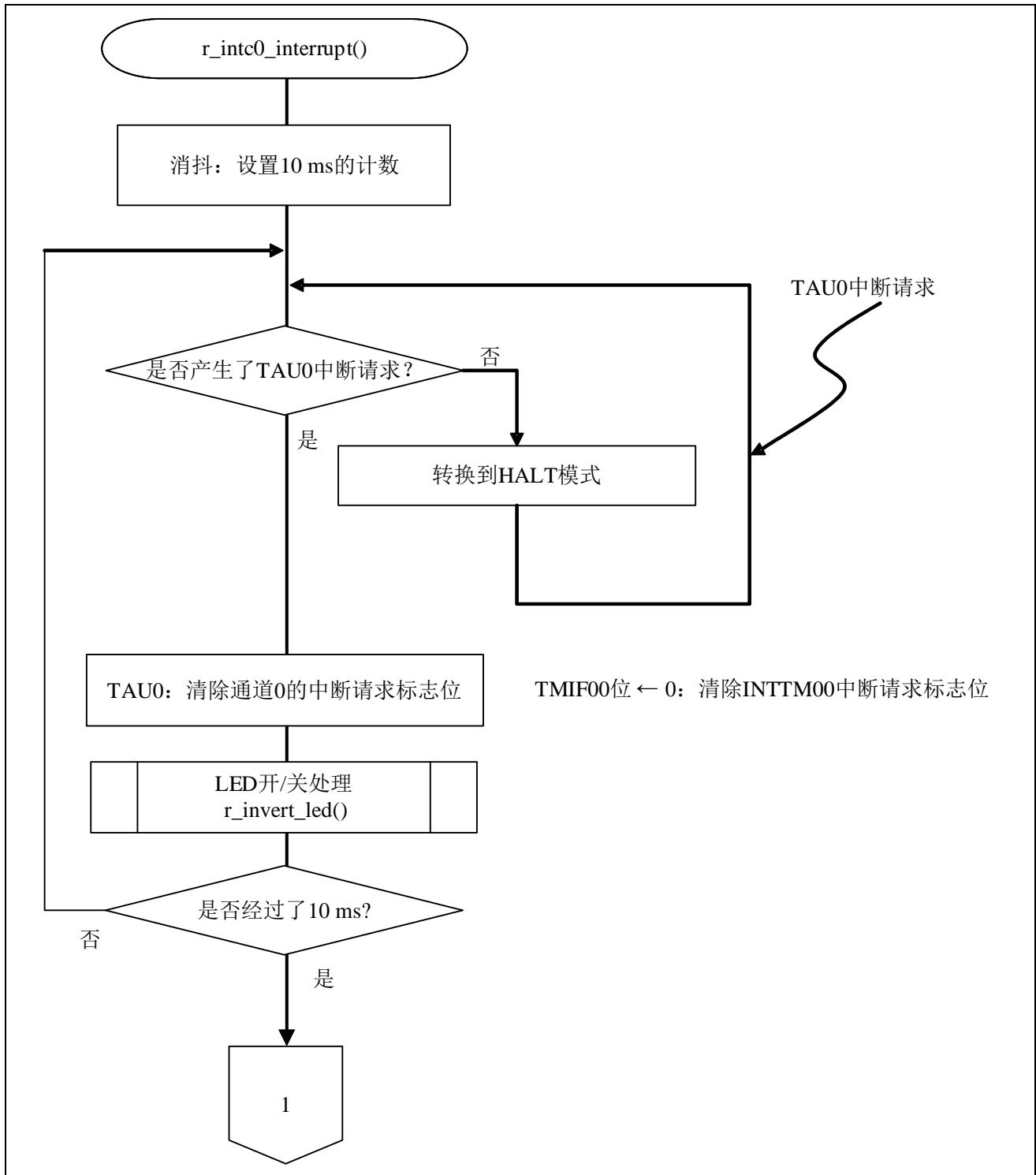
图 5.14 INTP0 中断处理（1/2）
