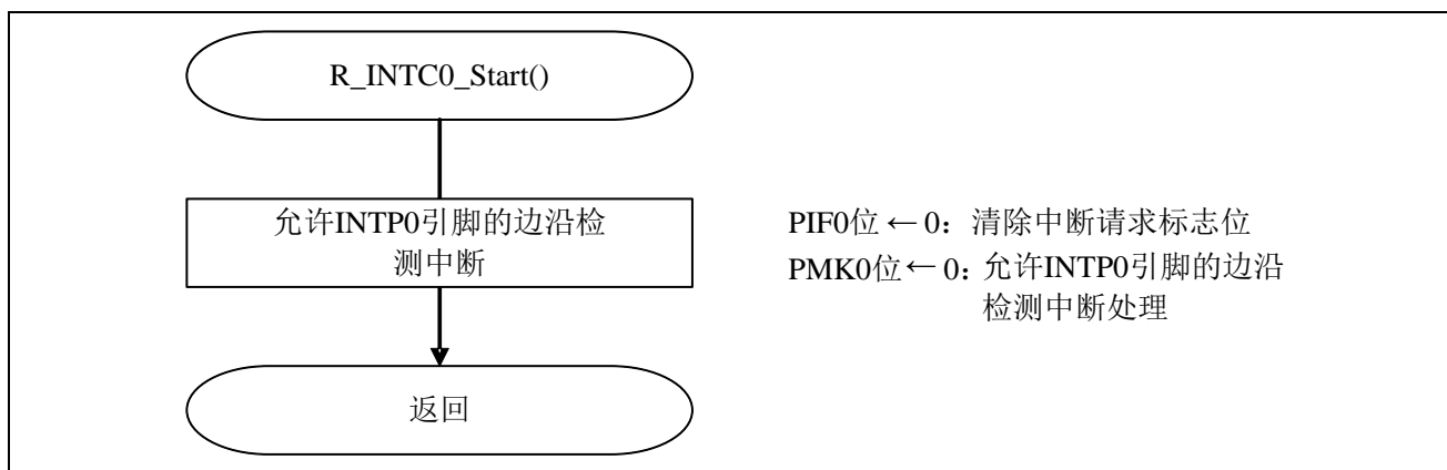
图 5.10 INTP0 运行开始
