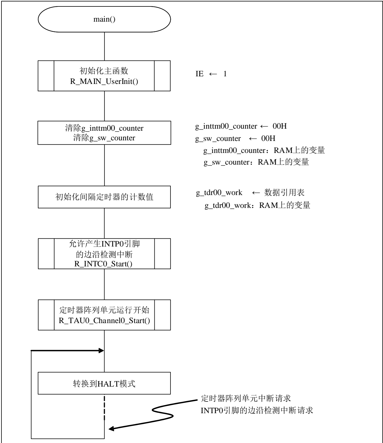
图 5.8 主函数处理
