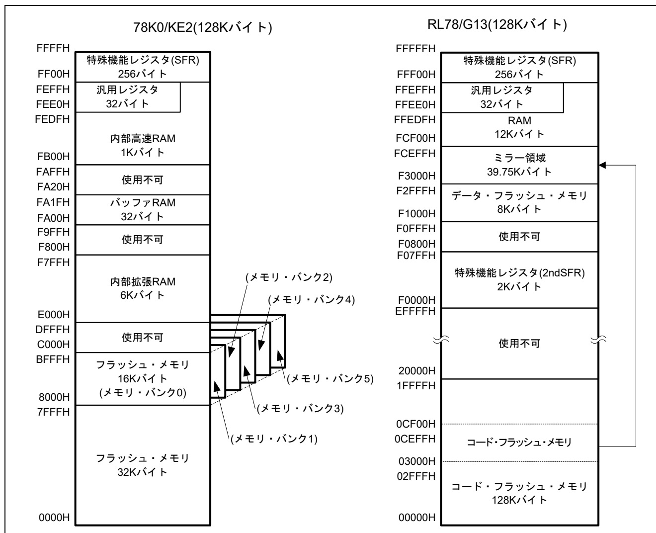
図 1.1 78K0/KE2 と RL78/G13 の 128K バイトのメモリ・マップ
