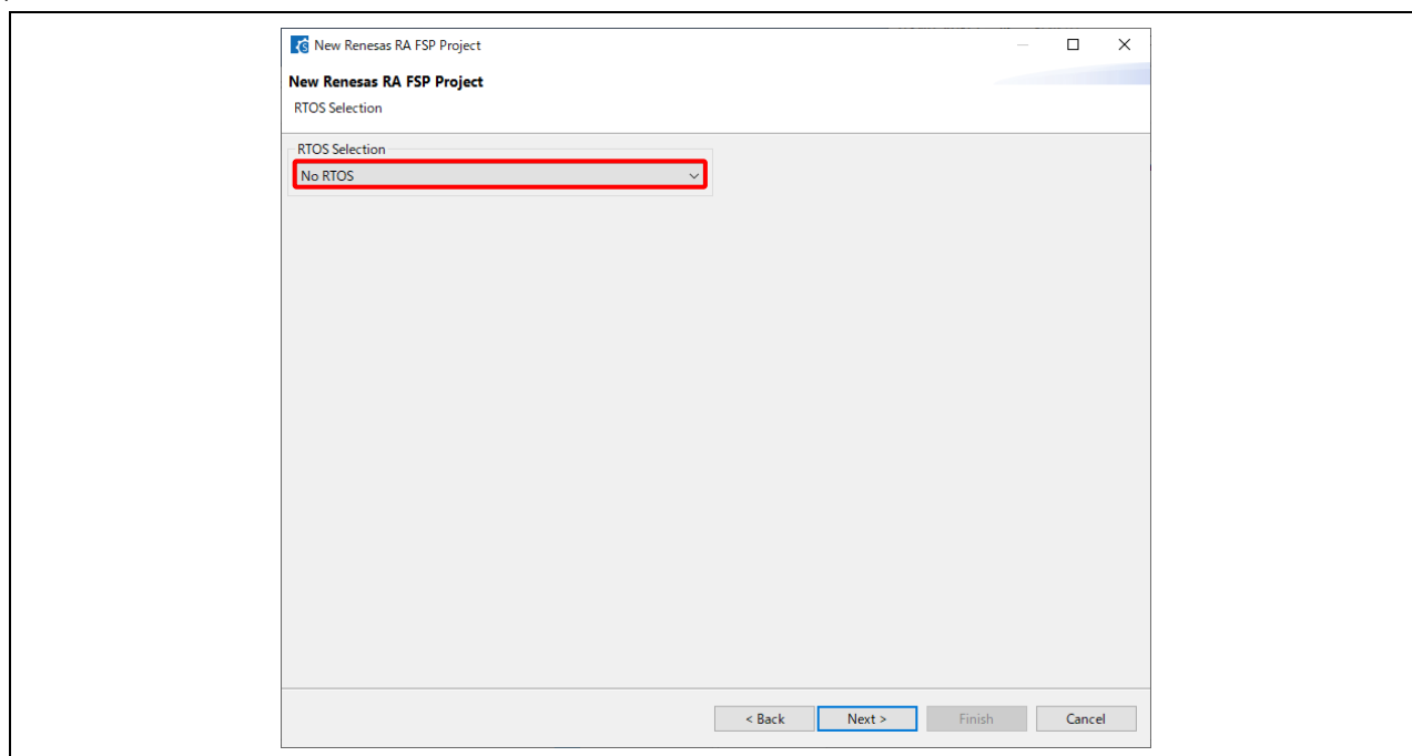
図 17 RTOS の選択
