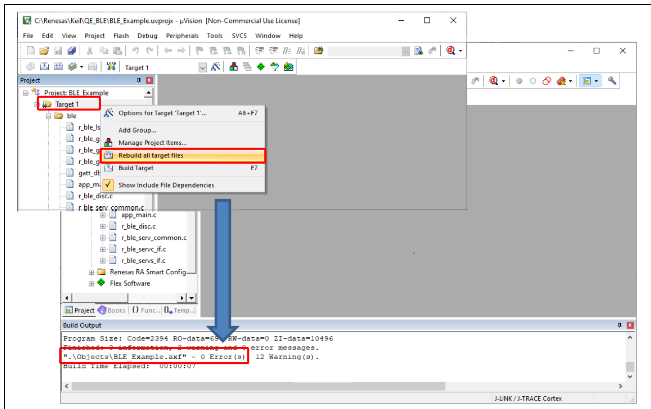
図 36 ビルド成功
