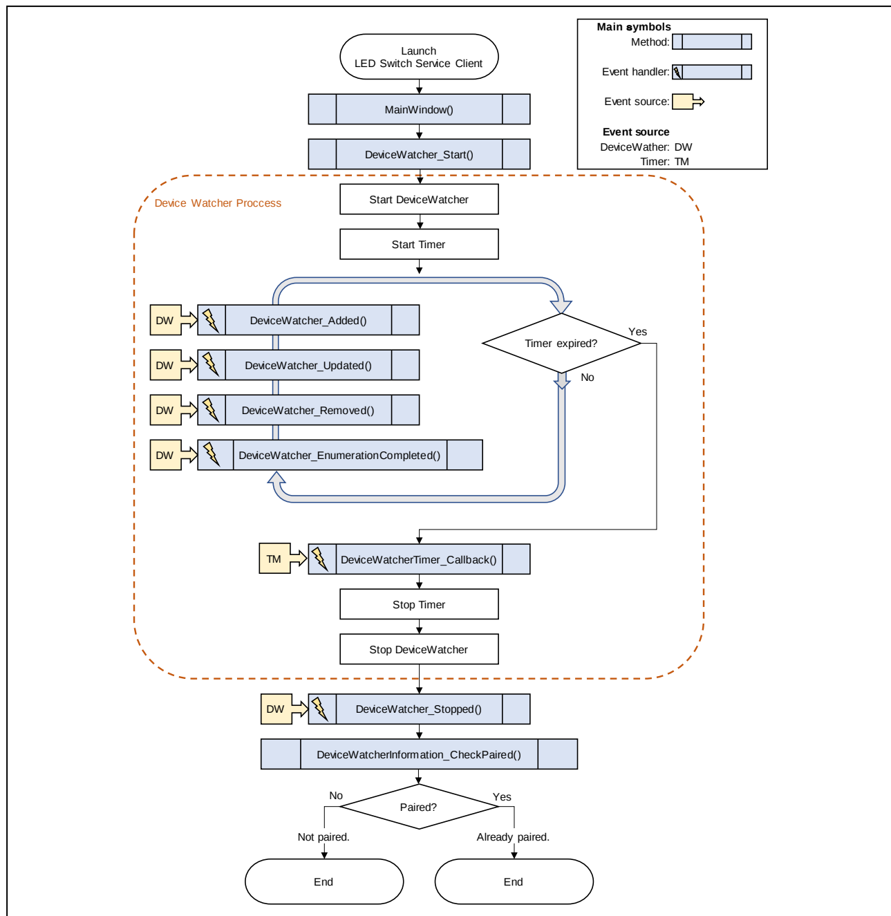
図 4-1 アプリケーション起動フローチャート
