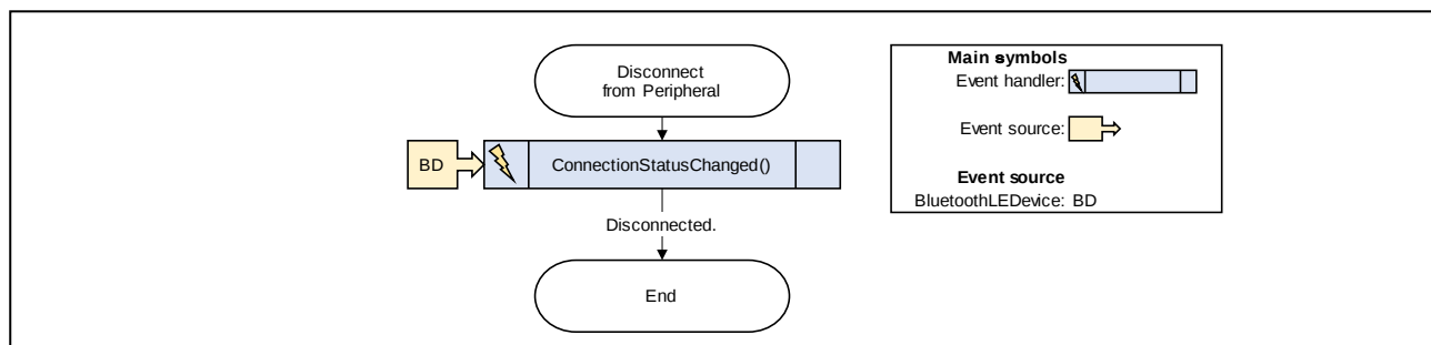
図 4-7 評価ボードからの切断フローチャート
