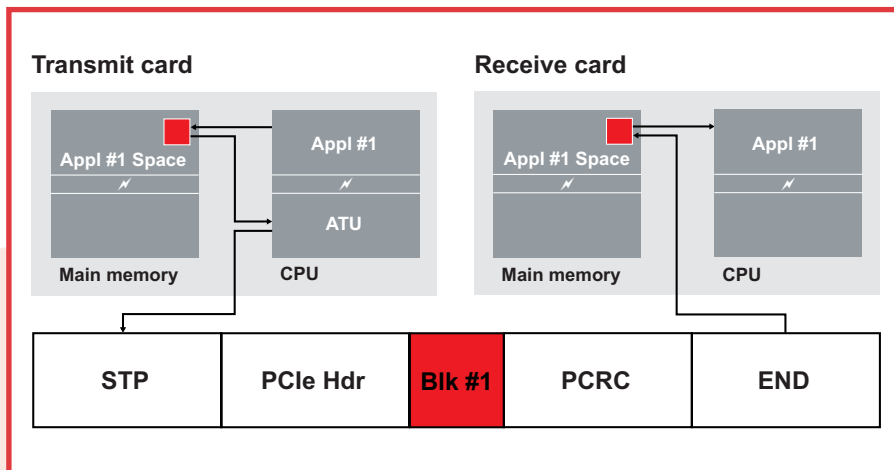
Bild 3. Direkte Speicherzugriffskonzepte wie PCIe erzeugen keine zusätzlichen Datenkopien
