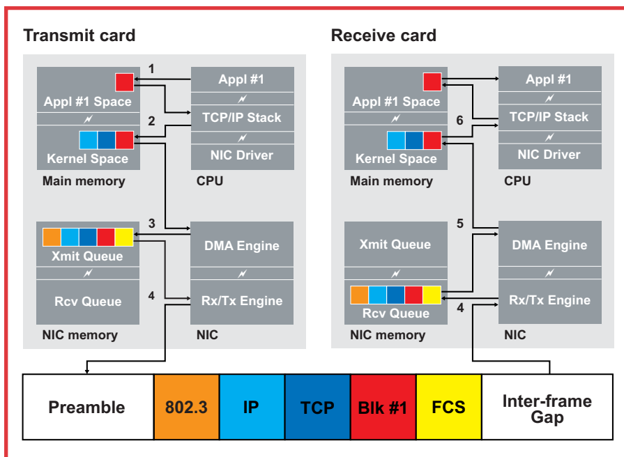
Bild 2. Beim Einsatz von Ethernet als Datenübertragungsmechanismus werden zahlreiche Daten-Kopien benötigt
