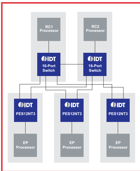
Bild 1. PCIe-Konfiguration für Upstream-Redundanz
