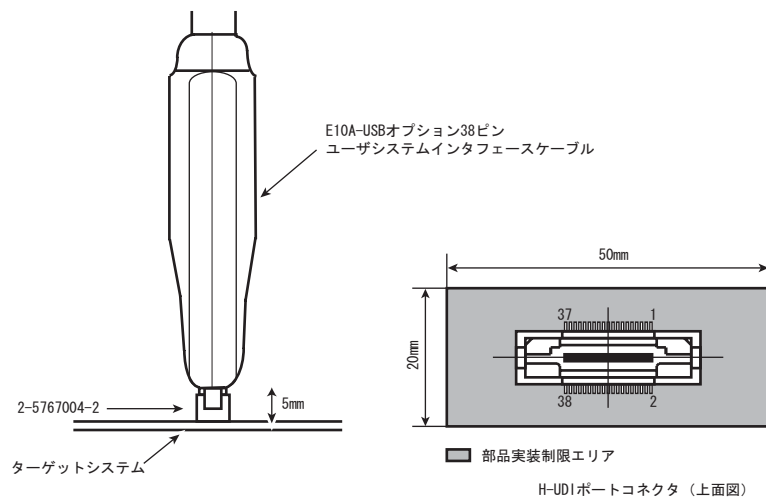
図 1.1 部品高さ制限
