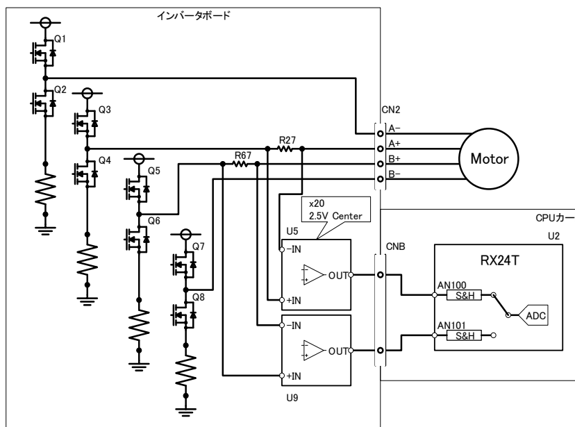
図 3-6 電流検出回路
