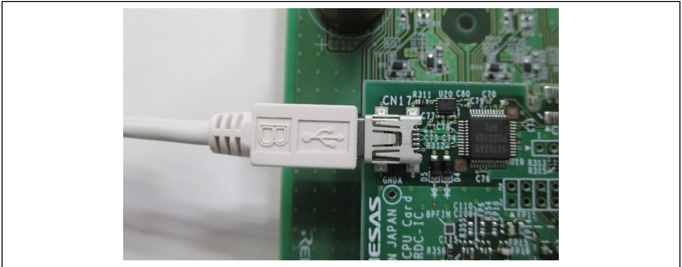
図 4-1 PC と接続
