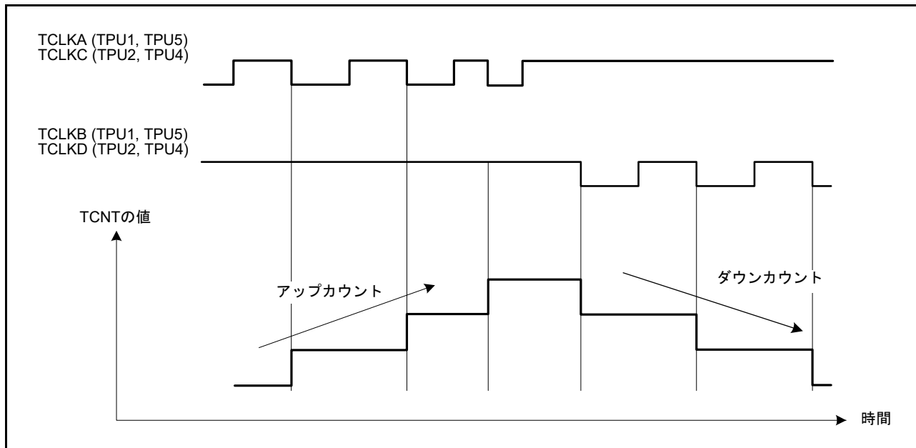
図 28.27 位相計数モード3の動作例
