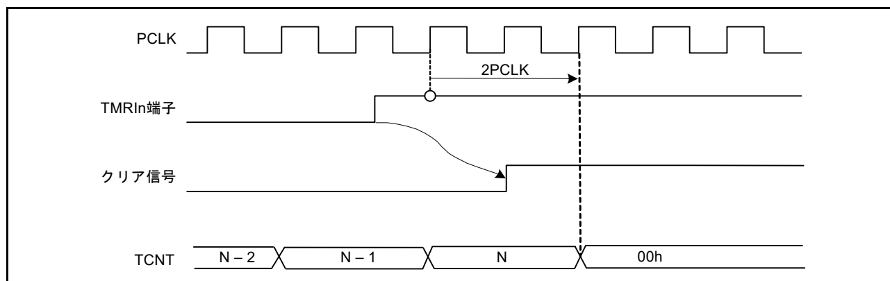
図 30.11 外部カウンタリセット信号によるクリアタイミング (High)
