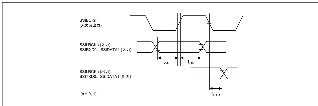
図 63.75 SSICR.BCKP = 0 の場合の SSIE データ送受信タイミング
