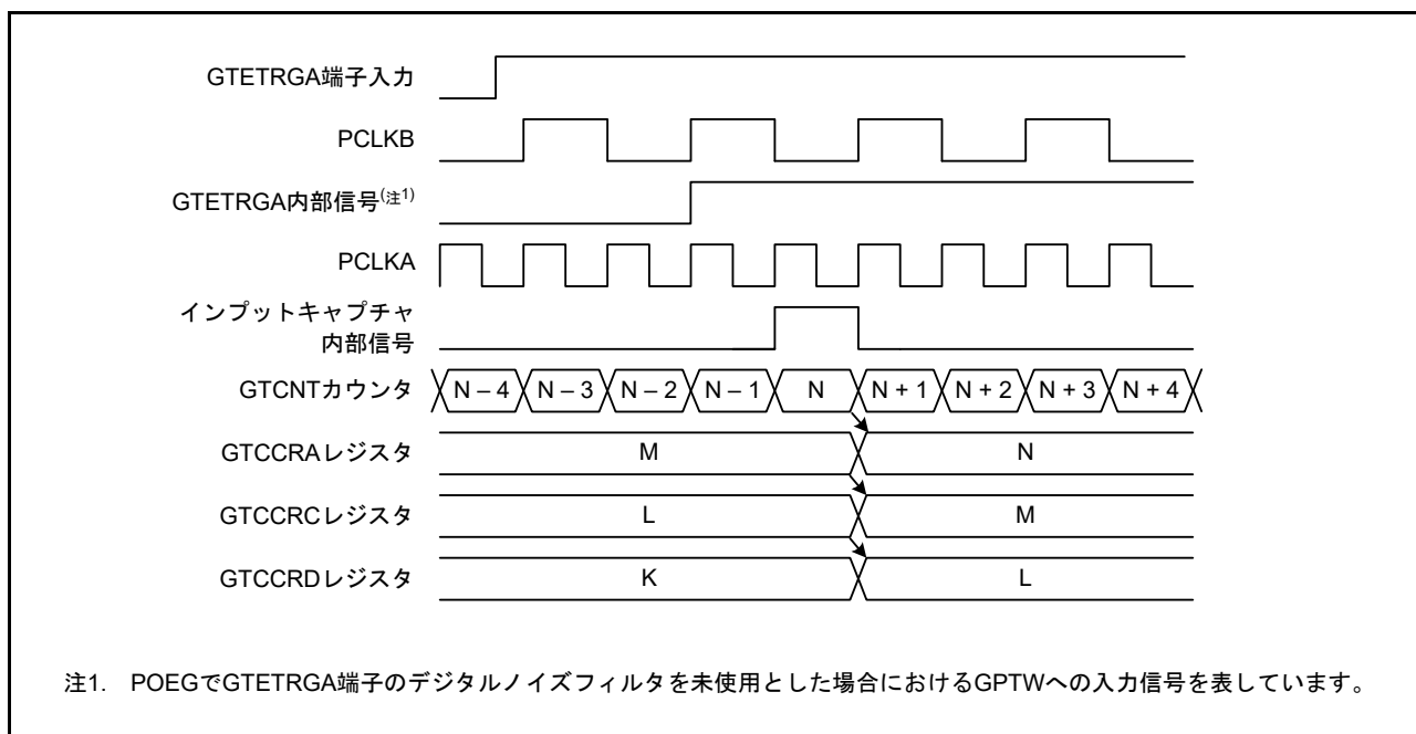
図 26.19 GTETRGA 端子入力立ち上がりによるインプットキャプチャ動作タイミング例
