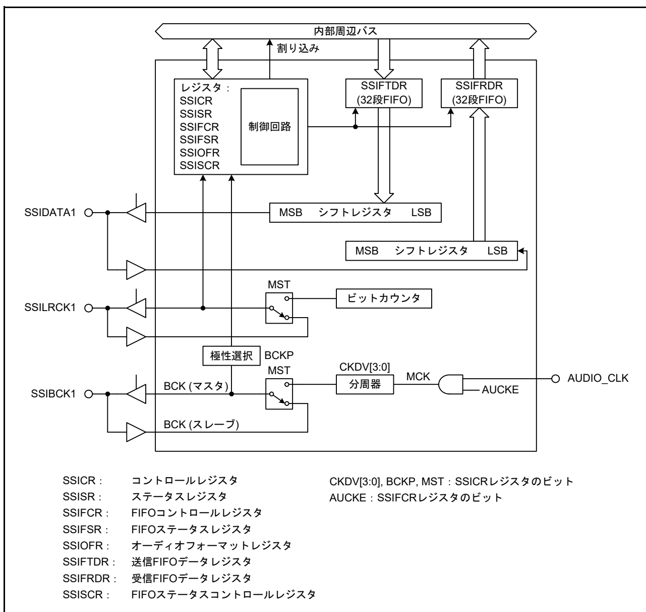
図 47.3 SSIE1 ブロック図
