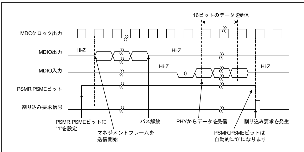
図 39.6 PHYレジスタリードの動作例
