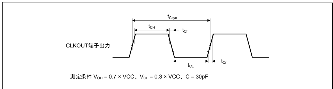
図 63.12 CLKOUT 端子出力タイミング
