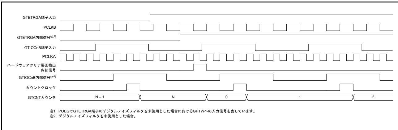
図 26.74 GTETRGA 端子入力の立ち上がりによるカウンタクリア動作タイミング例 (ハードウェア要因によるカウント動作時)
