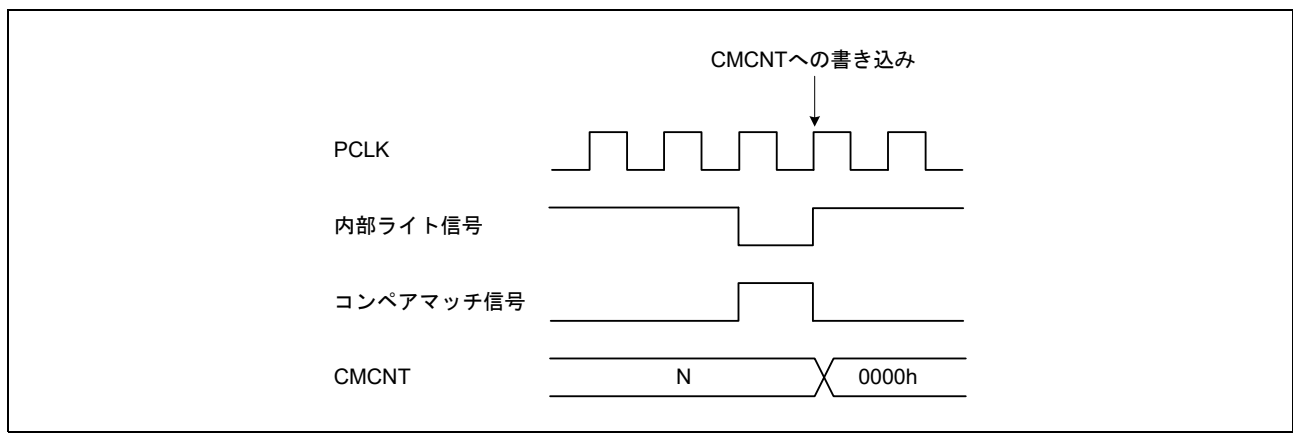
図 31.5 CMCNTカウンタへの書き込みとコンペアマッチの競合
