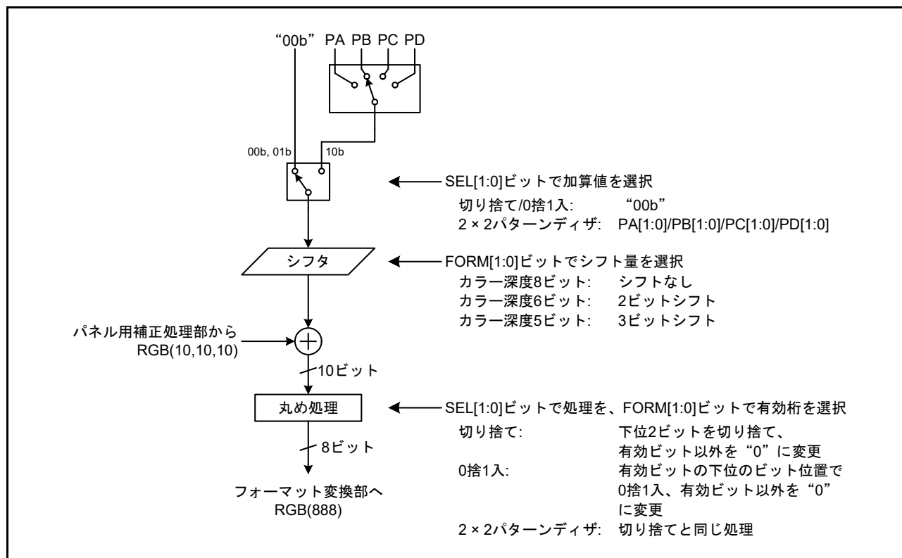
図 51.12 ディザ処理部の構成
