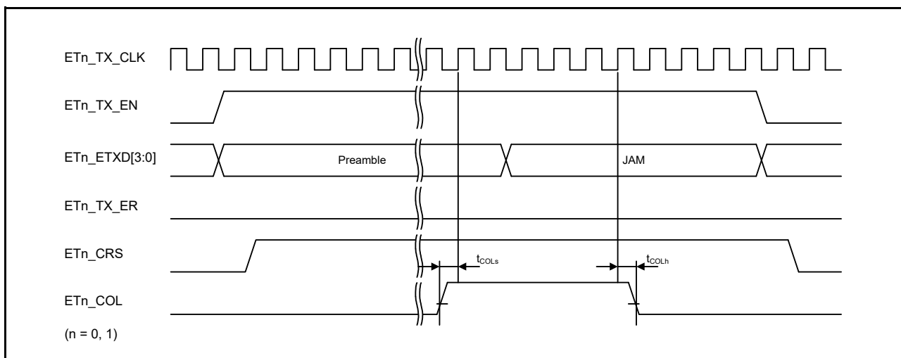
図 63.87 MII 送信タイミング (衝突発生ケース)
