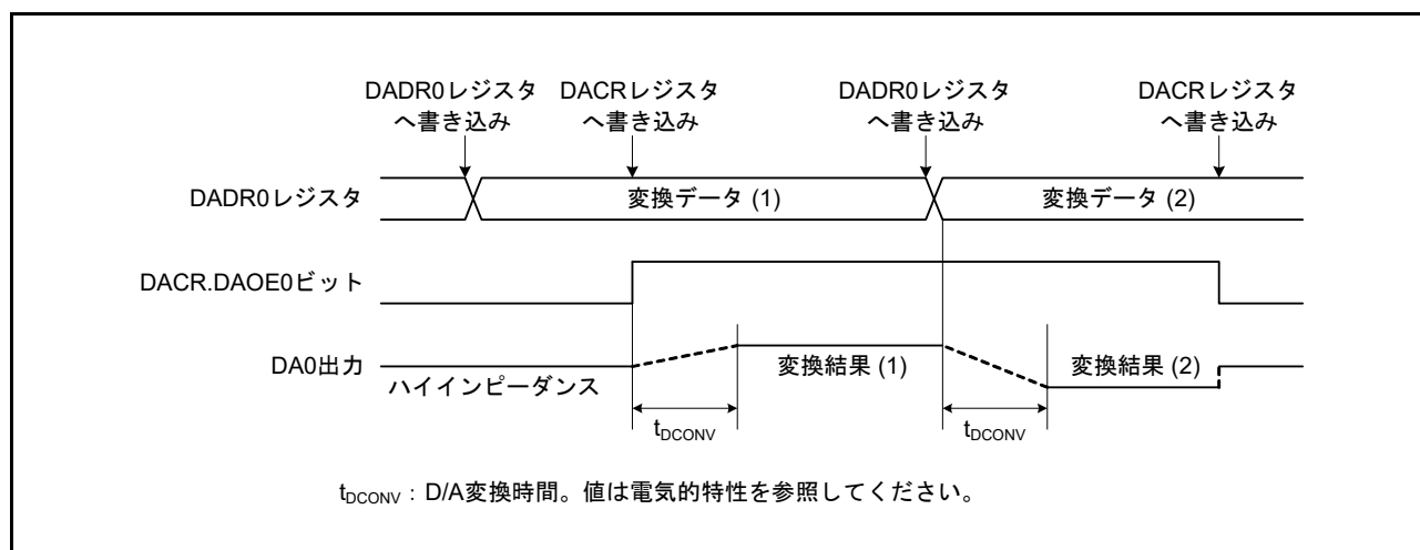
図 57.2 12ビットD/Aコンバータの動作例
