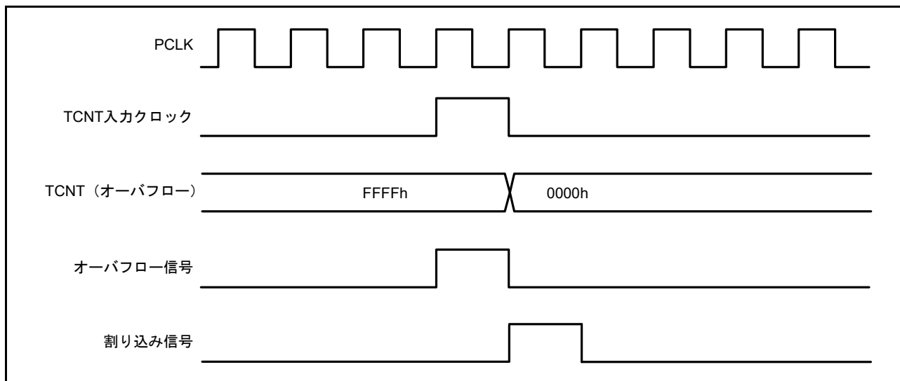
図 28.41 TCImV 割り込みのセットタイミング
