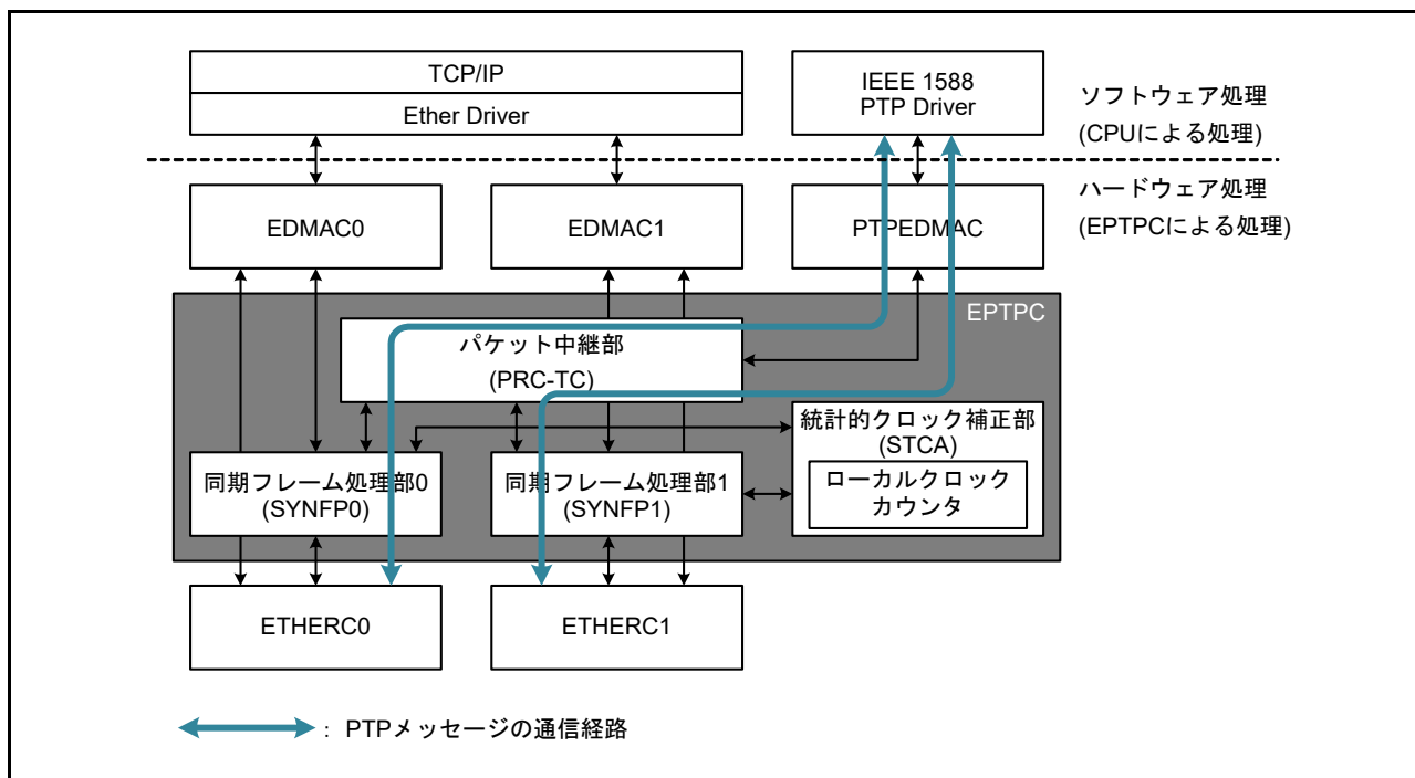
図37.6 ソフトウェア処理が必要なPTPメッセージの通信経路
