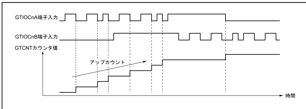
図 26.95 位相計数モード5の動作例 (n = 0 ~ 3)
