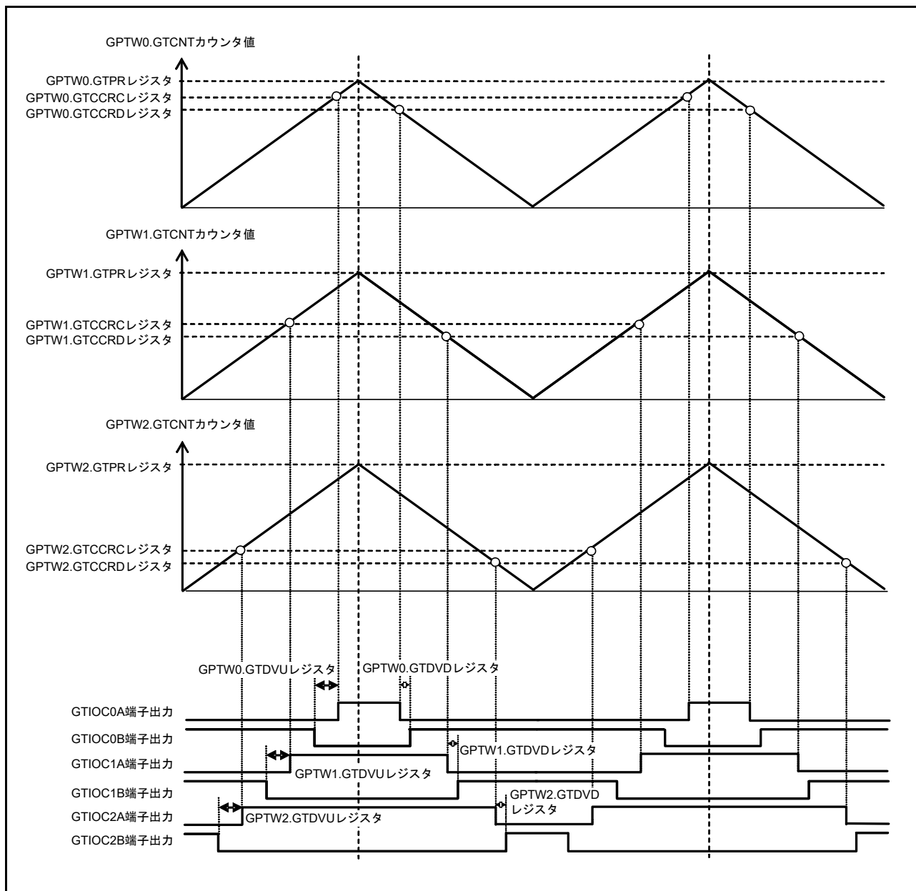
図 26.86 非対称三角波 3 相相補 PWM 出力例 (デッドタイム自動設定)
