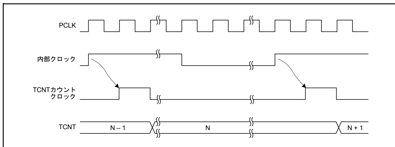
図 30.5 内部クロック動作時のカウンタタイミング
