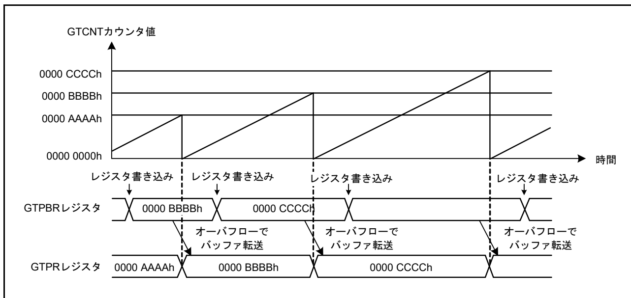
図 26.22 GTPR レジスタのバッファ動作例 (のこぎり波でアップカウントの場合)
