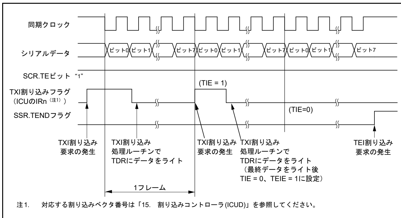
図 41.31 クロック同期式モードのシリアル送信の動作例 (3) (送信中～送信終了時)
