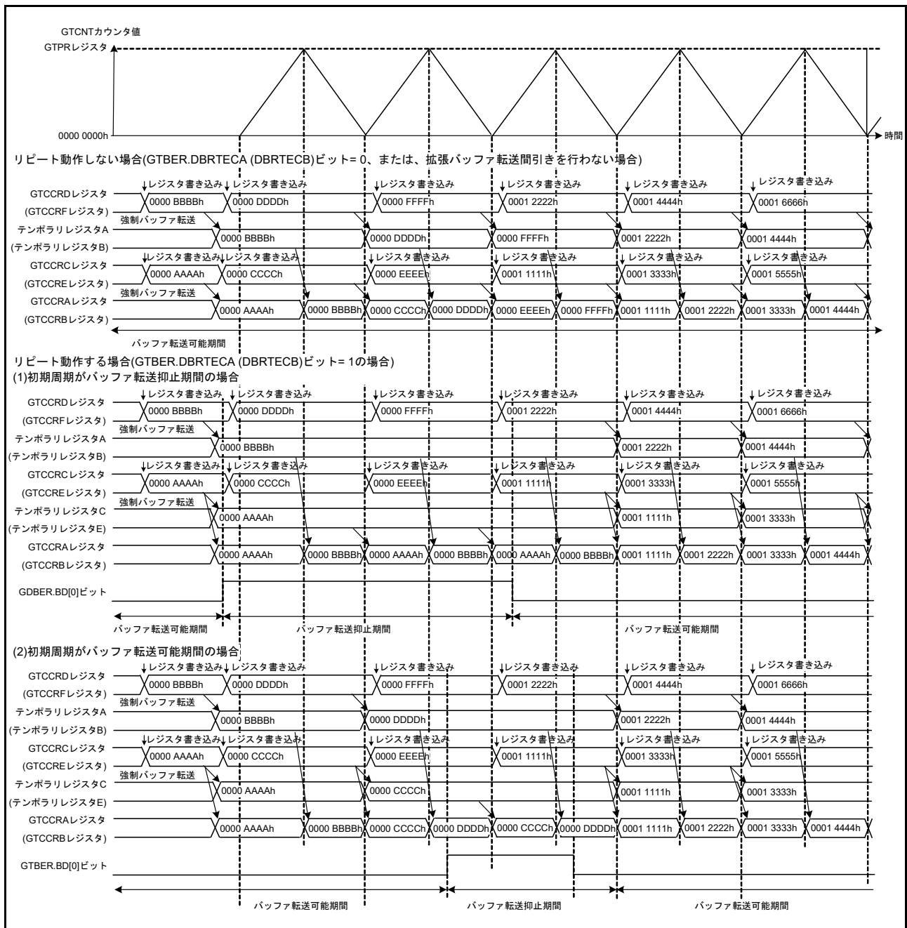
図 26.124 GTCCR バッファ転送抑止時ダブルバッファリポート動作例 (三角波 PWM モード 3、GTBER.BD[0] ビットを更新する場合)
