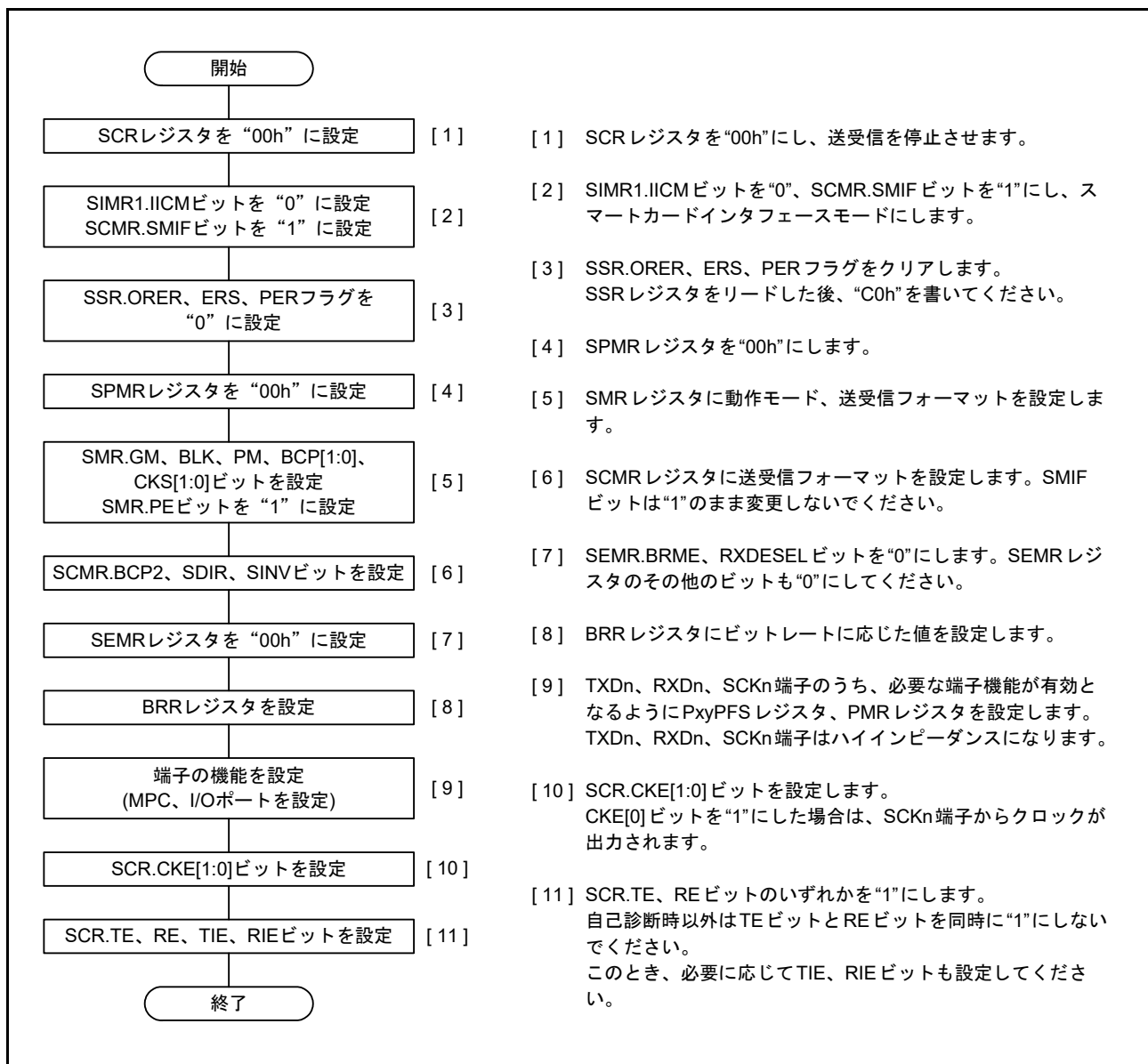
図 41.42 SCIの初期化フローチャートの例 (スマートカードインタフェースモード)
