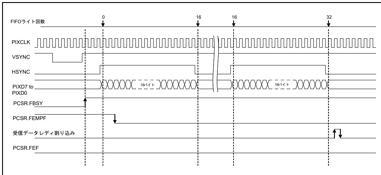
図 50.12 水平ブランキング期間中の動作例
