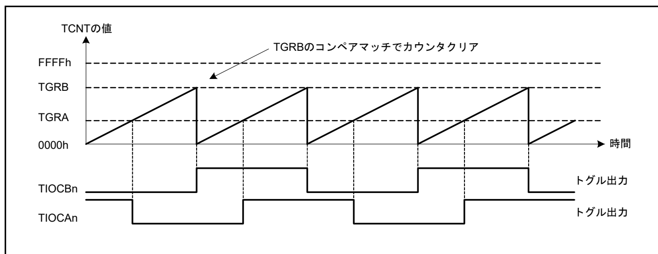
図 28.7 トグル出力の動作例 ( n=0\sim 5 )
