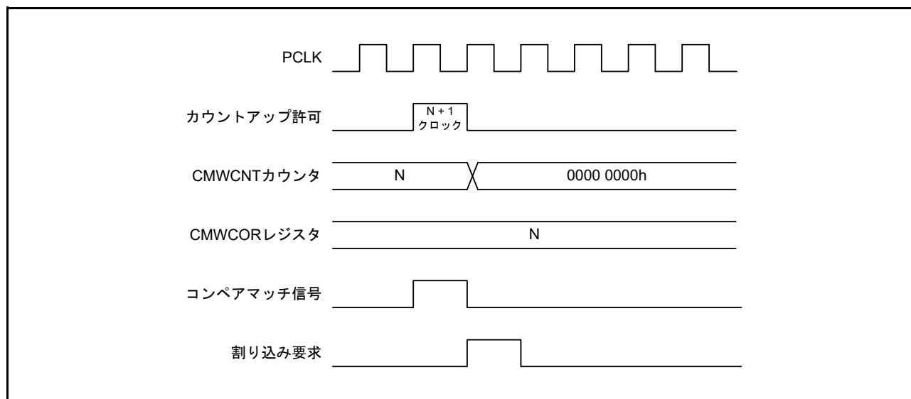
図 32.13 コンペアマッチ割り込みの発生タイミング
