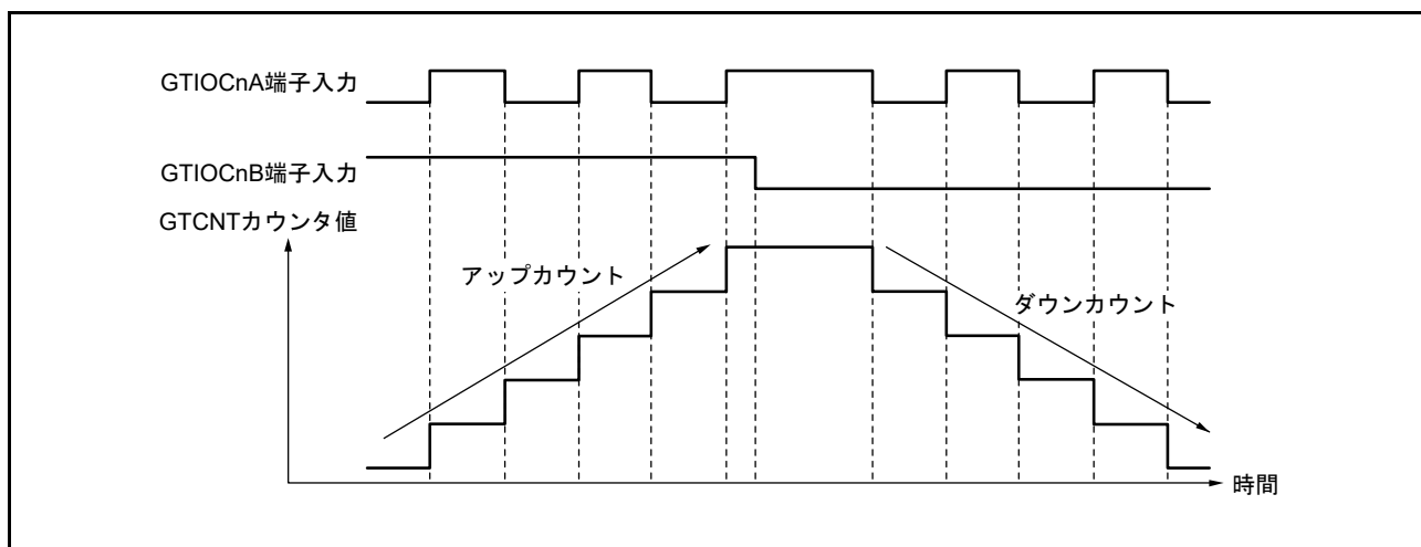
図 26.90 位相計数モード2の動作例 (n = 0 ~ 3)
