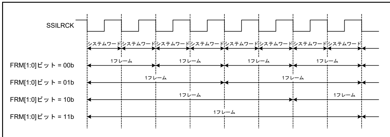
図 47.5 フレームワード長
