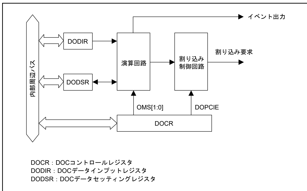
図 59.1 DOC のブロック図
