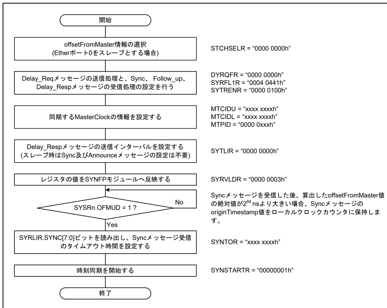
図37.13 E2Eスレーブ動作の開始手順
