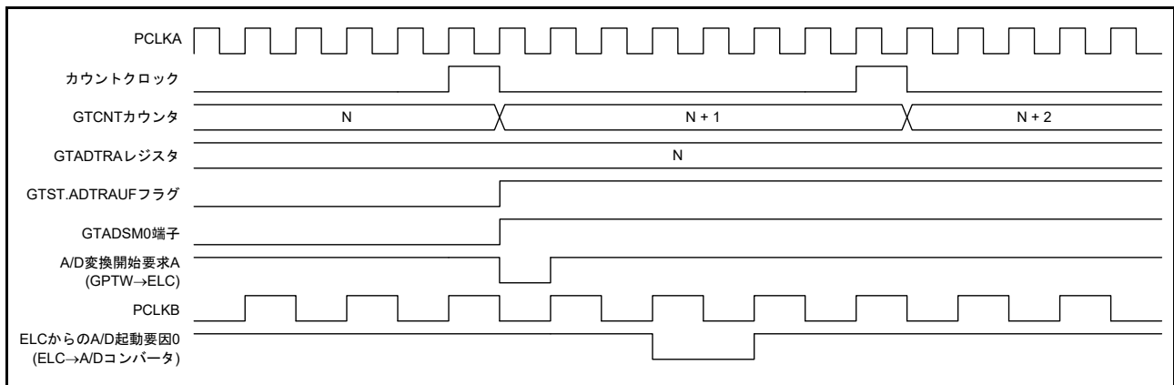
図 26.117 A/D 変換開始要求動作タイミング例
