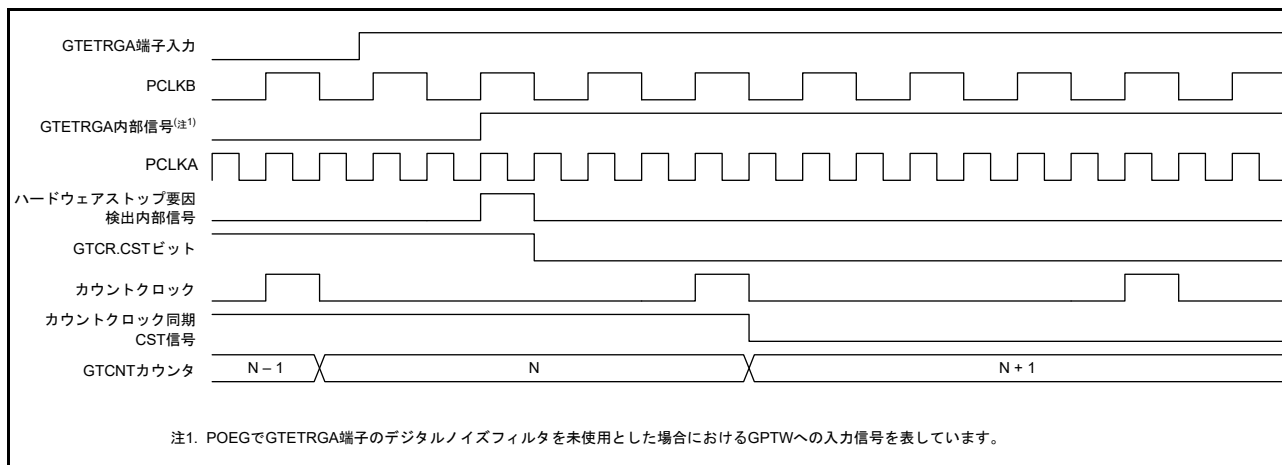
図 26.64 GTETRGA 端子入力の立ち上がりによるカウントストップ動作タイミング例
