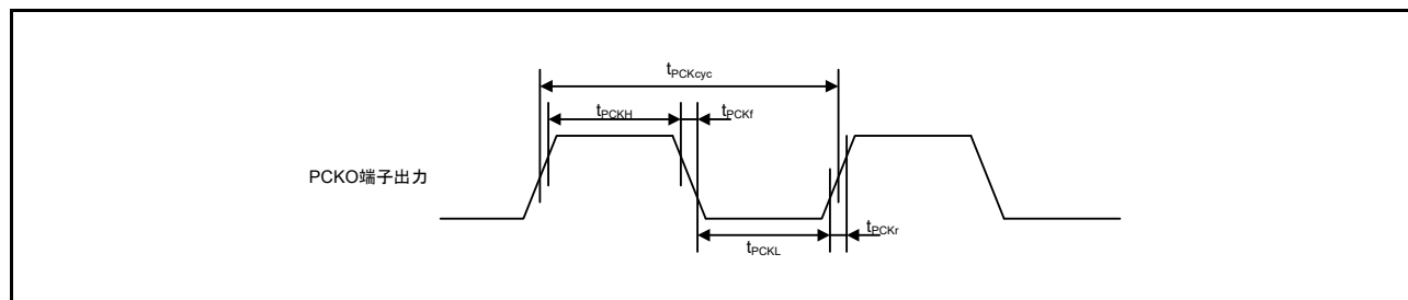
図 63.92 PDC 出力クロックタイミング
