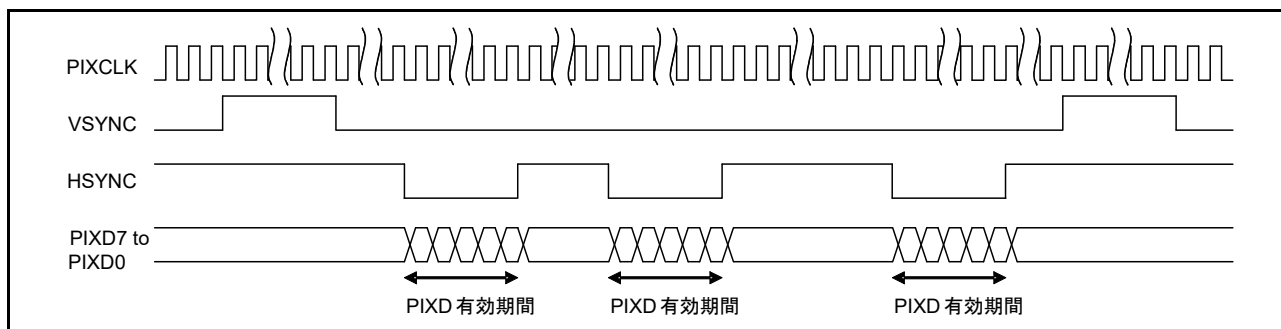
図 50.7 PDC 通信フォーマット (VPS = 1, HPS = 1)
