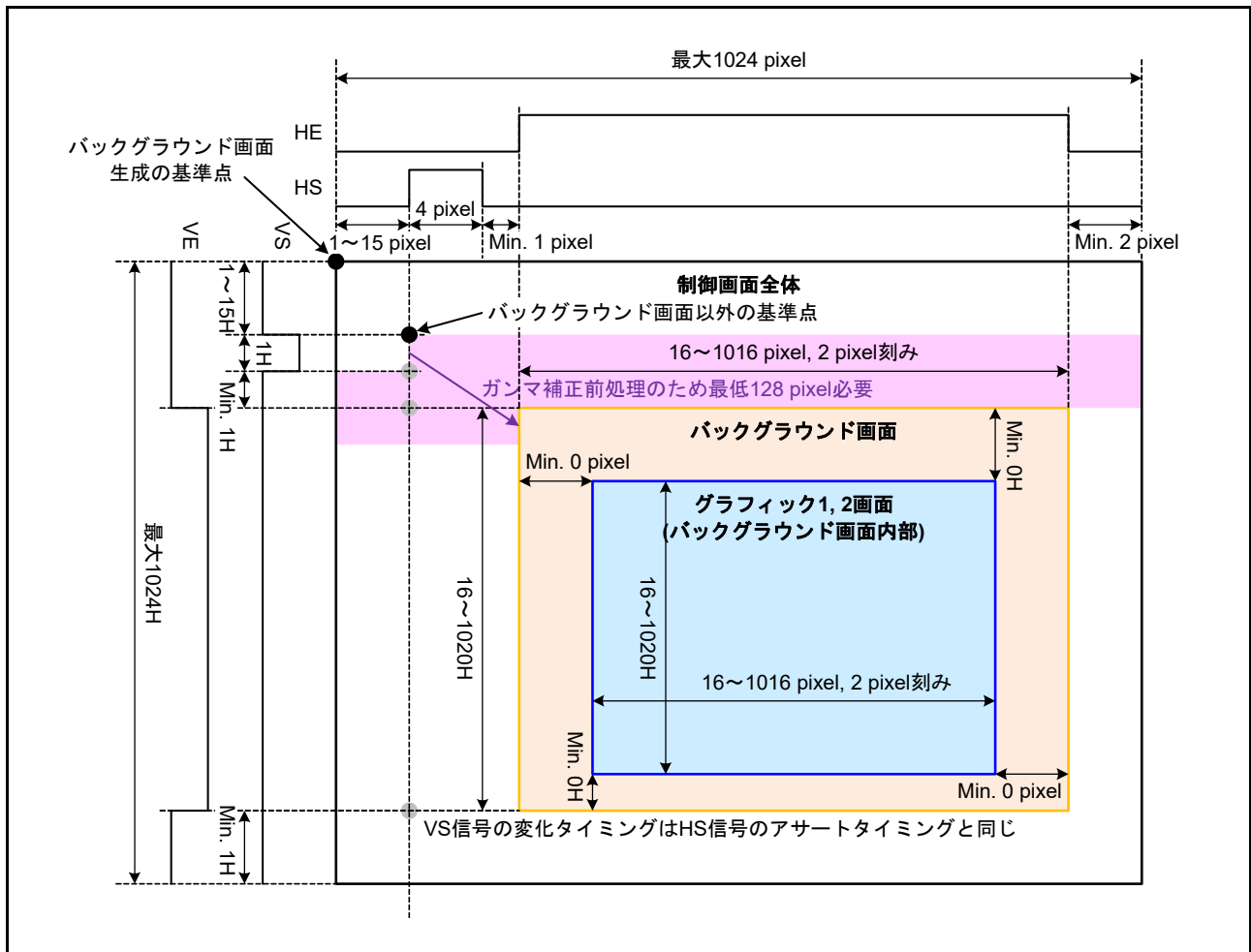
図 51.3 画面フォーマット
