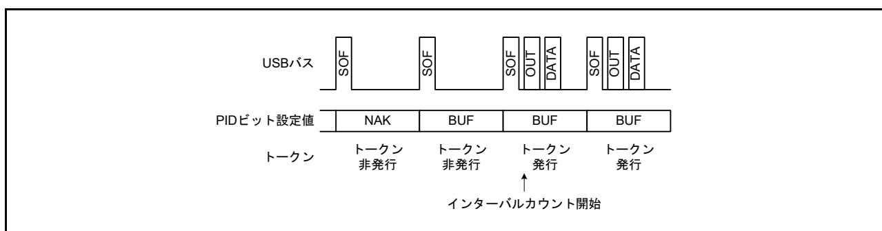
図 40.16 IITV[2:0] = 000b の場合のトークン発行有無
