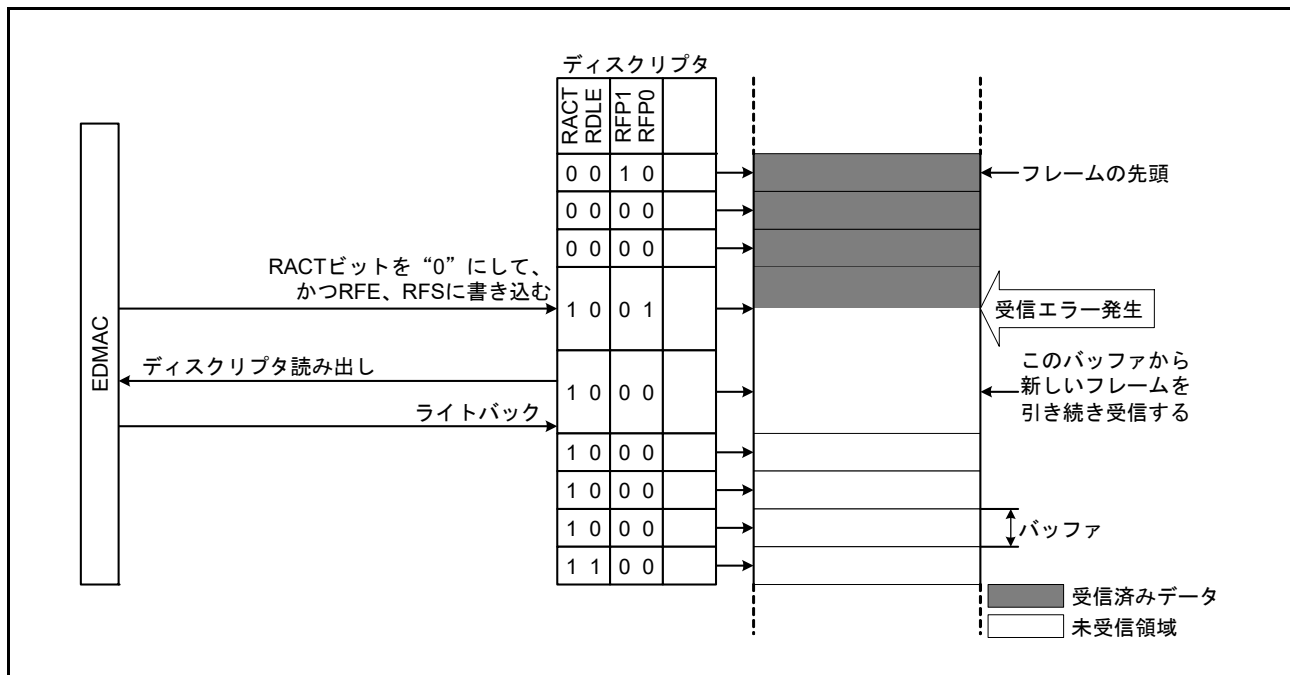
図 38.8 受信エラー発生後のEDMAC動作
