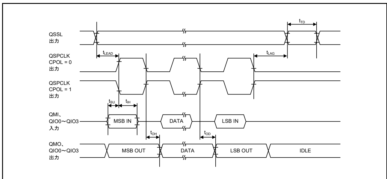
図 63.71 送受信タイミング (CPHA = 0)
