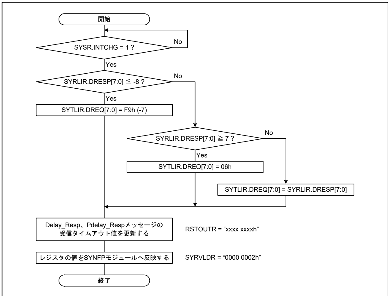
図37.14 Delay_Reqメッセージの送信間隔の変更手順
