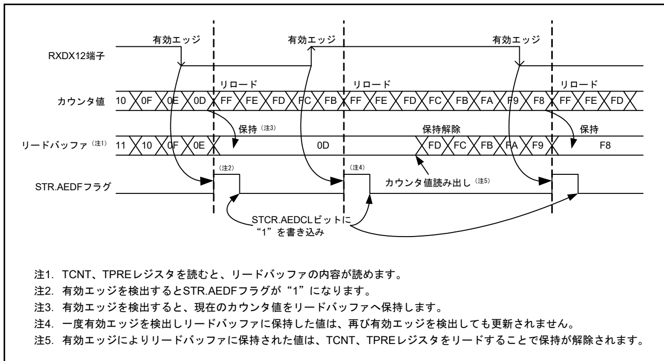
図 41.75 ビットレート測定機能動作例
