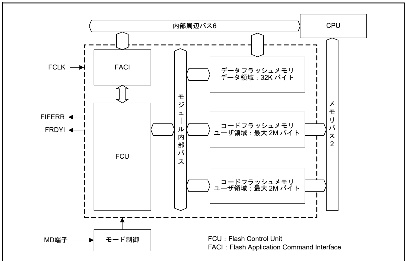
図 62.1 フラッシュメモリ関連のブロック図
