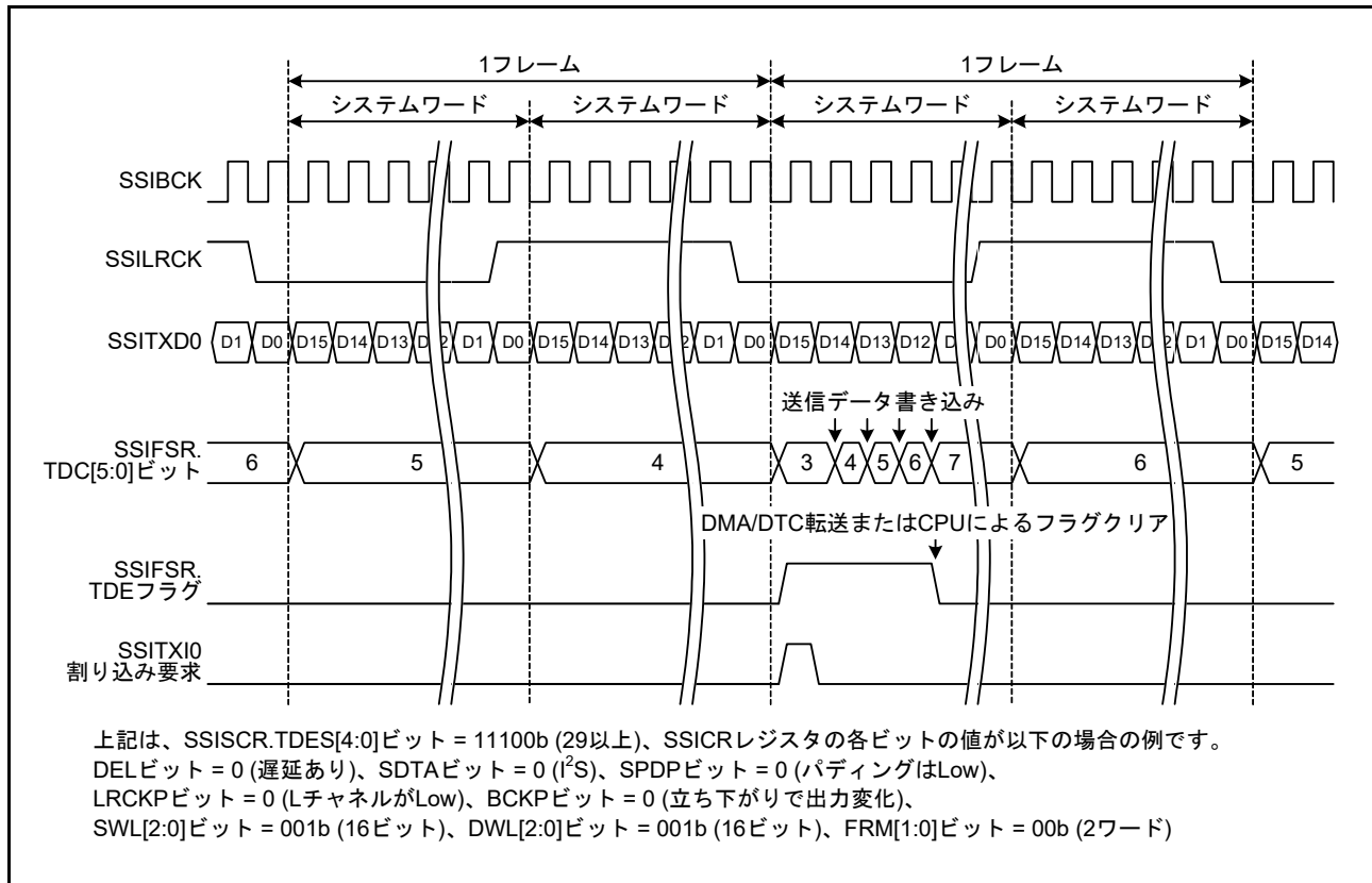
図 47.27 SSITXIO 割り込みのタイミング図
