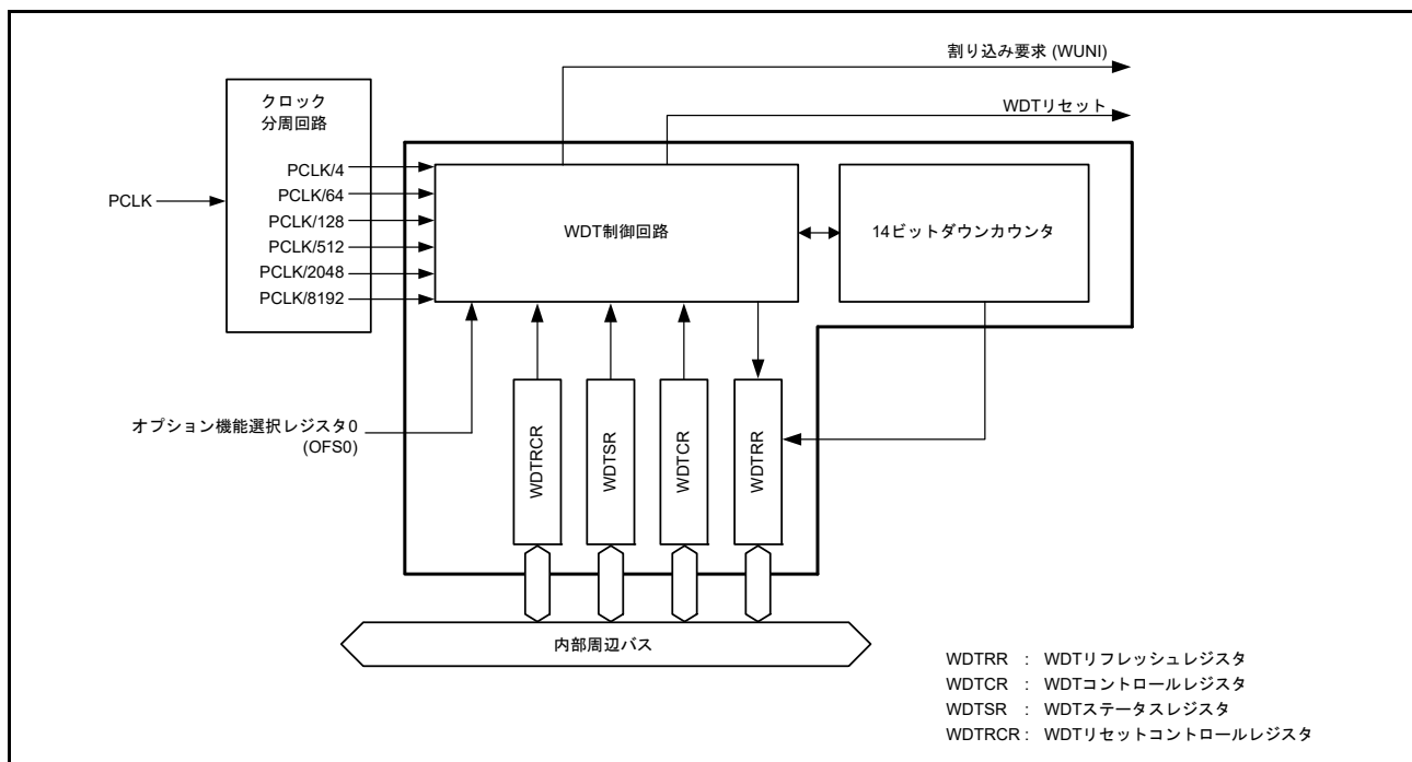
図 34.1 WDT のブロック図
