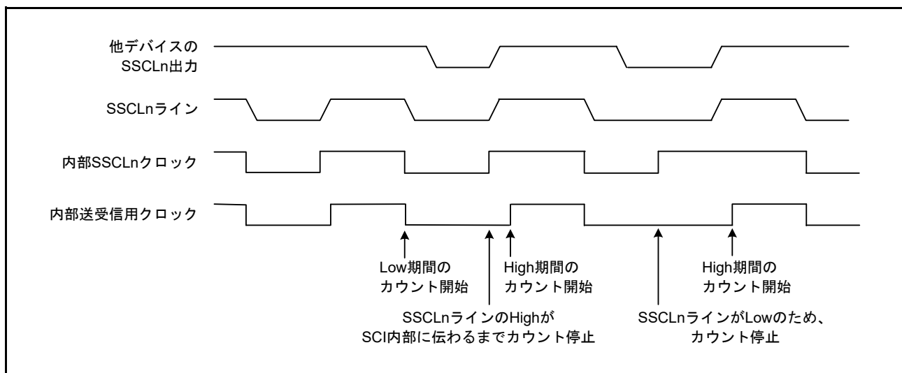
図 41.53 クロック同期化の動作例
