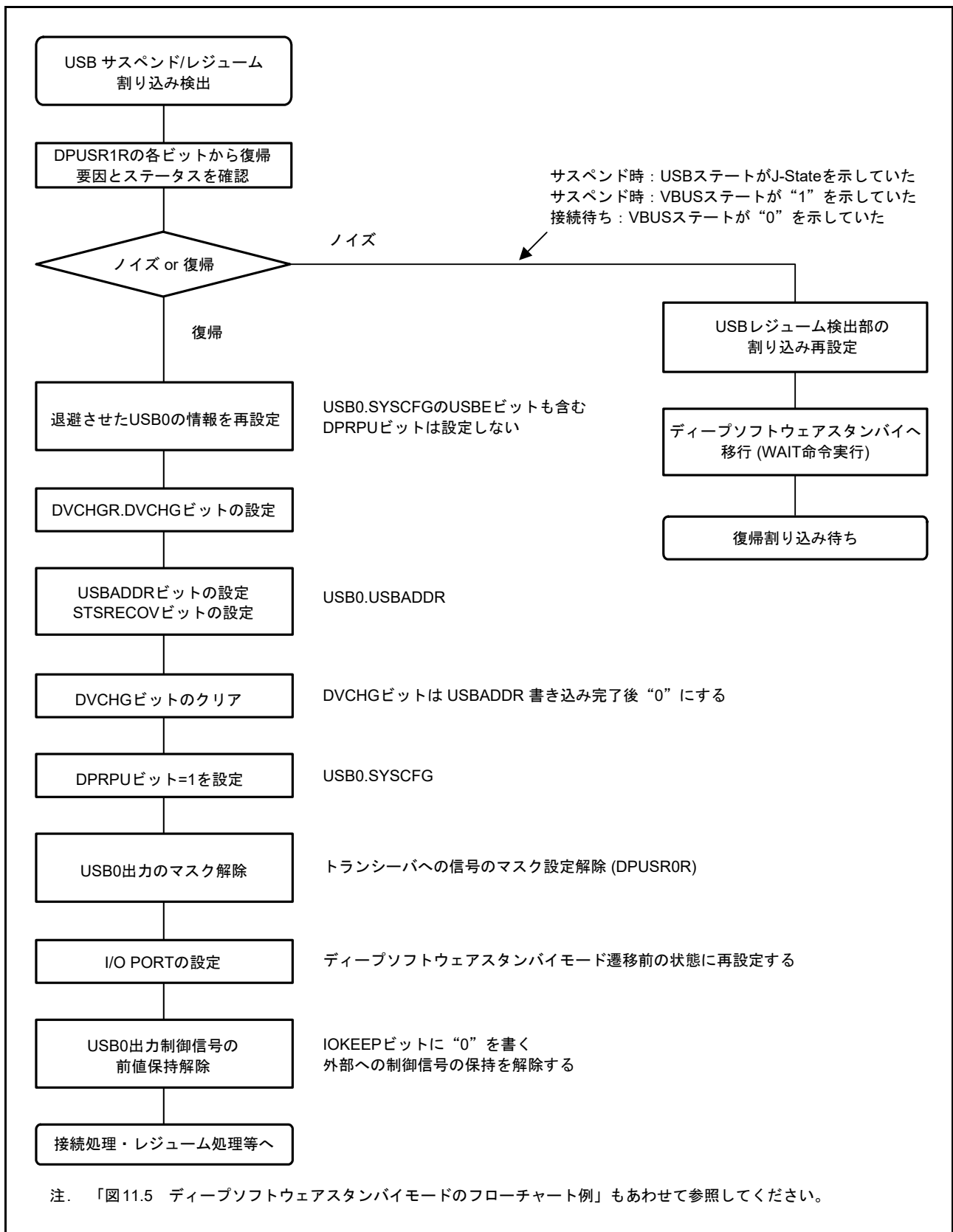
図 40.9 ファンクション時のディープソフトウェアスタンバイ解除時の USB 設定フロー
