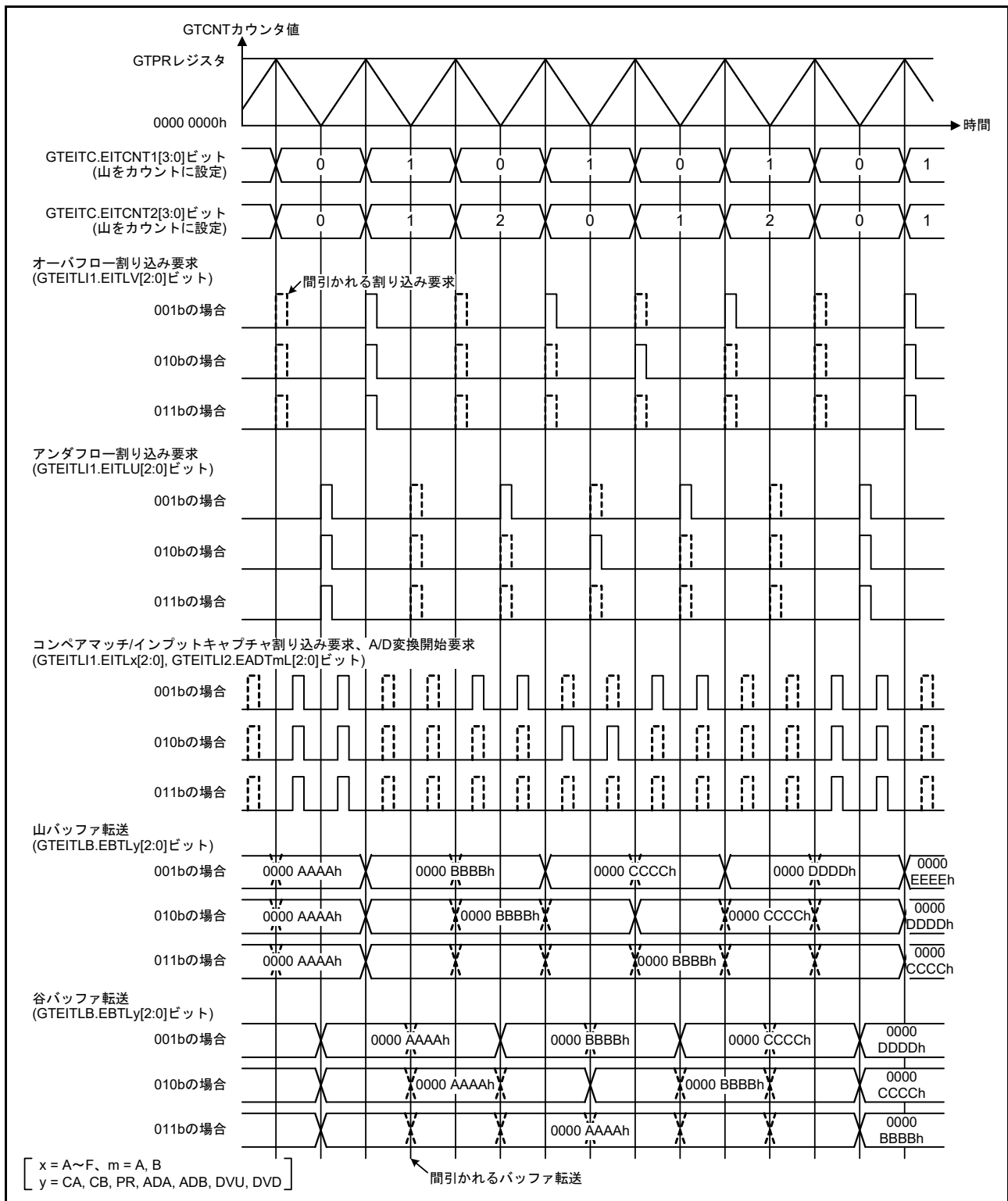
図 26.107 拡張割り込み間引き機能の動作例 (三角波、拡張割り込み間引き 1 間引き回数 1 で山をカウント、拡張割り込み間引き 2 間引き回数 2 で山をカウント、拡張割り込み間引きカウンタ 2 初期値 “0” の場合 GTEITC.EITCNTk ビット (k = 1, 2) が “0” 以外の期間で間引く場合)
