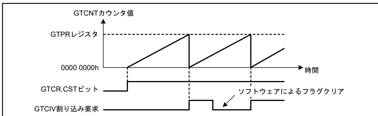
図 26.2 サイクルカウント動作例(カウントクロックによるアップカウント時)
