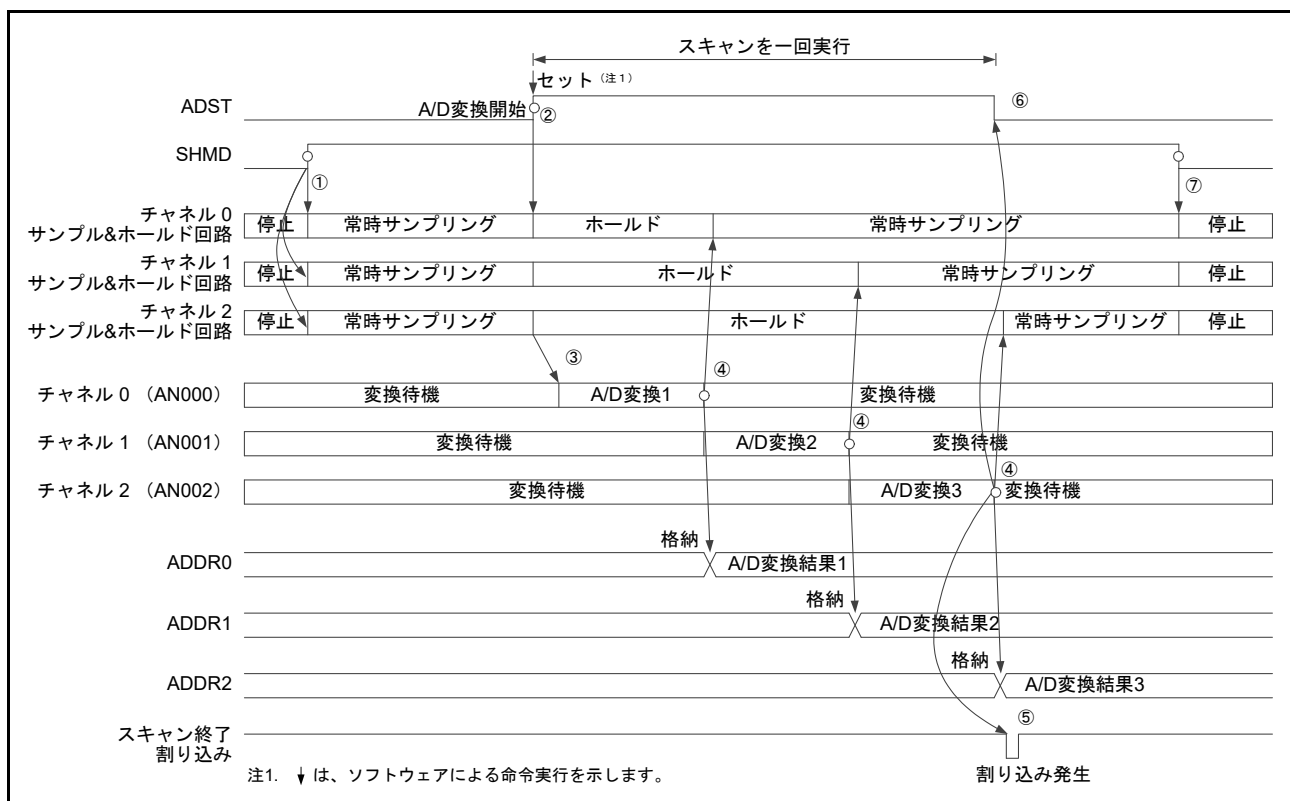
図 56.8 シングルスキャンモードの動作例 (チャンネル専用サンプル & ホールド回路使用 : AN000 ~ AN002 選択、常時サンプリング有効)
