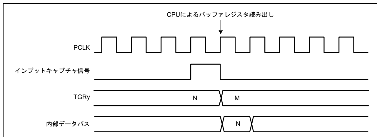
図 28.48 TPUm.TGRy レジスタの読み出しとインプットキャプチャの競合
