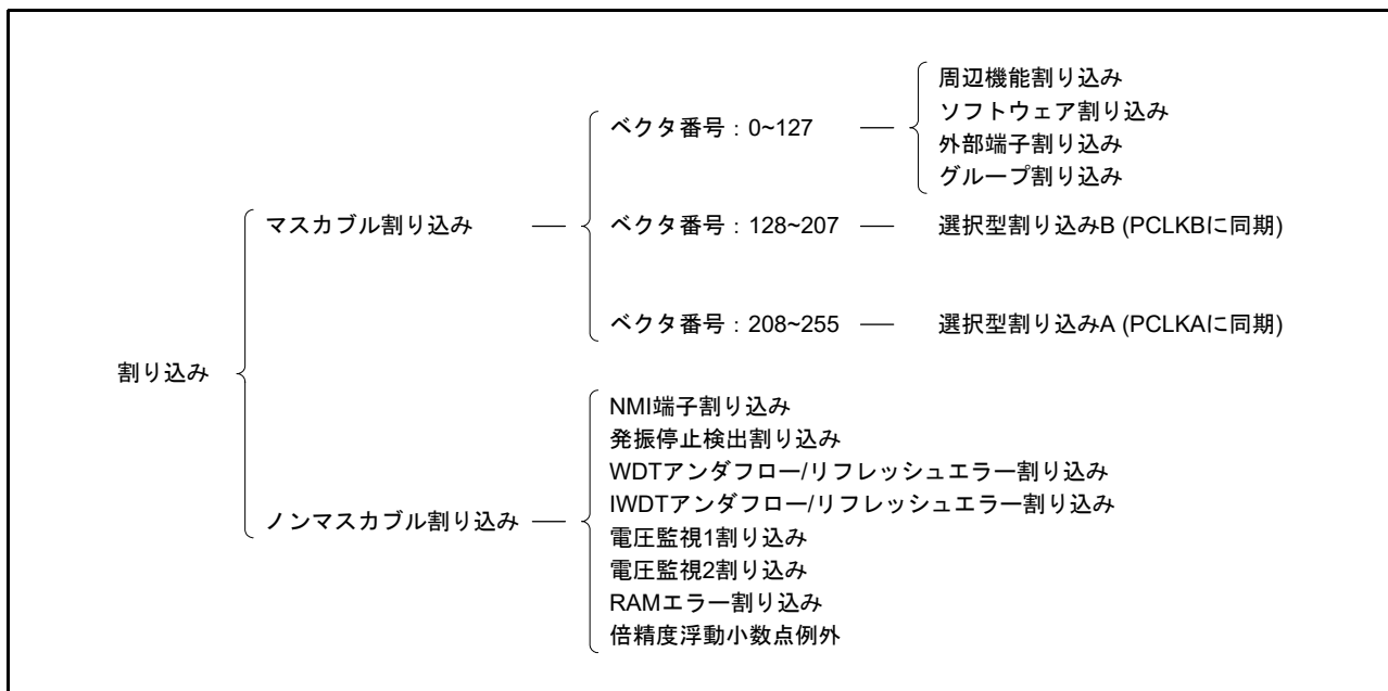
図 15.2 割り込みの種類
