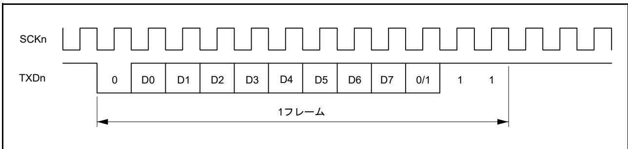
図 41.8 出カクロックと送信データの位相関係 (調歩同期式モード: SEMR.CHR = 0、PE = 1、MP = 0、STOP = 1)
