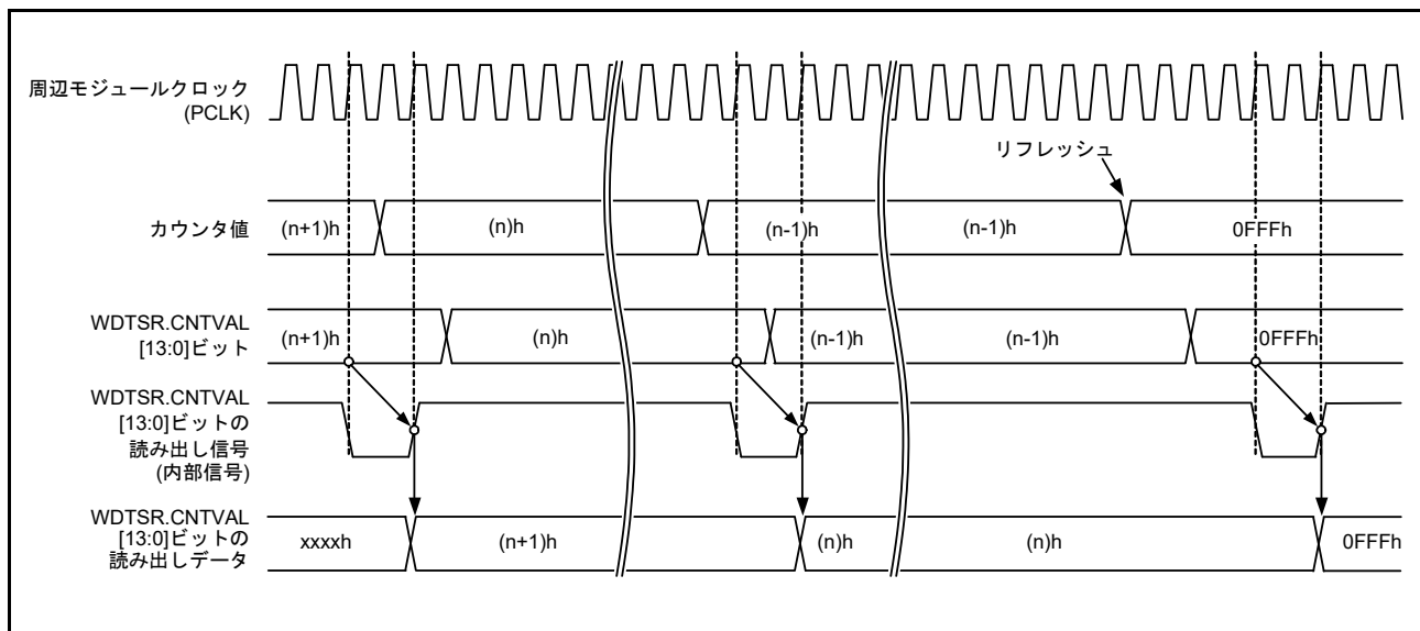
図 34.7 WDT ダウンカウンタ値の読み出し処理 (WDTCR.CKS[3:0] = 0100b、WDTCR.TOPS[1:0] = 01b)
