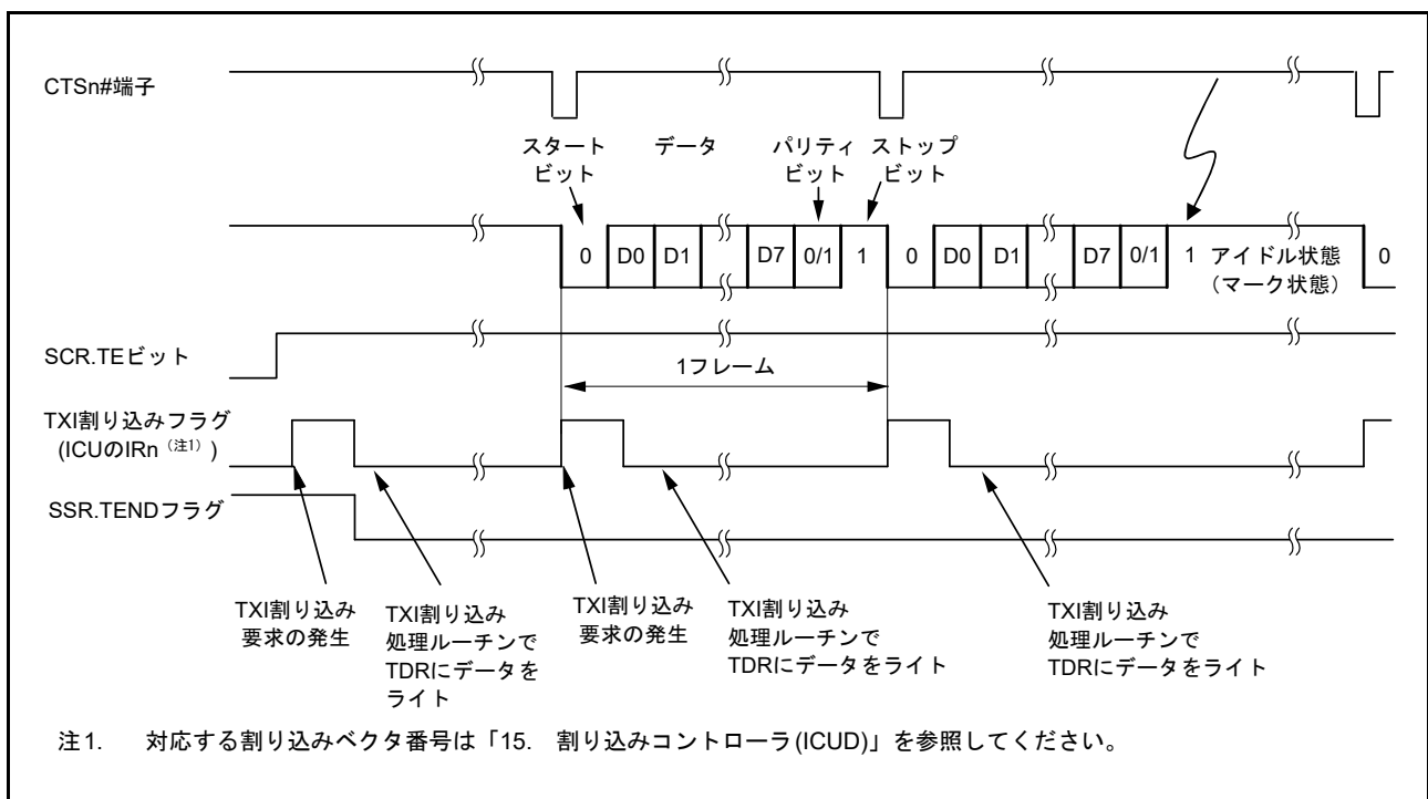
図 41.15 調歩同期式モードのシリアル送信の動作例 (2) (8ビットデータ / パリティあり / 1ストップビット / CTS 機能使用する / 送信開始時)
