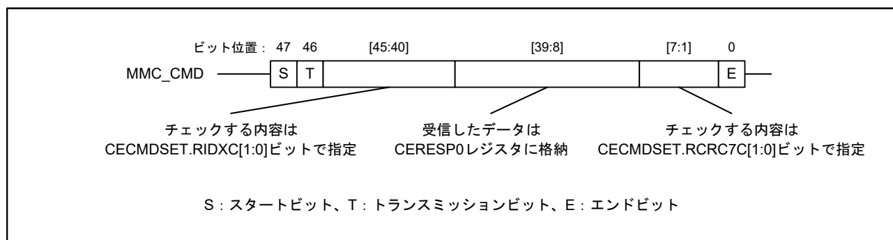
図 49.3 6 バイトのレスポンス (R2 レスポンス以外) のフォーマット
