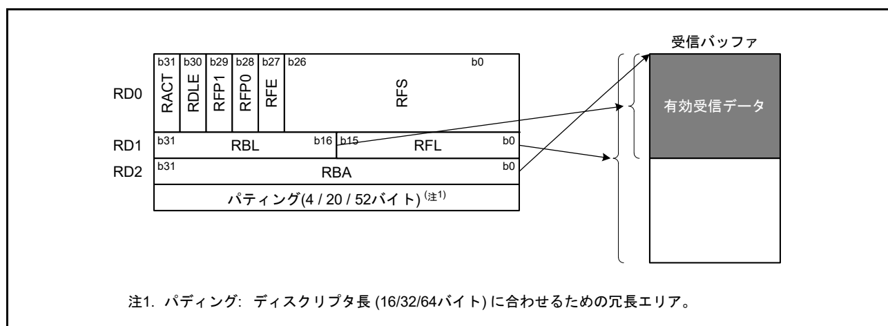
図 38.4 受信ディスクリプタと受信バッファの関係
