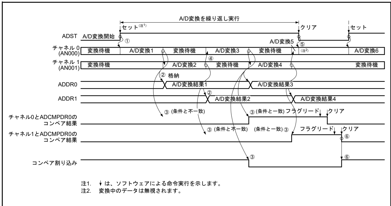
図 56.37 コンペア機能の動作例 (AN000, AN001 コンペア対象)
