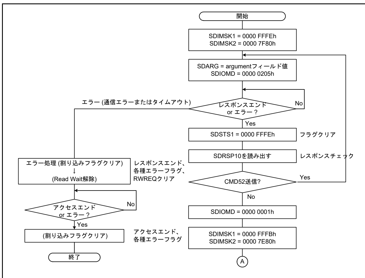
図 48.17 IO_RW_EXTENDED コマンド (CMD53/ マルチブロックリード) のシーケンス中に Read Wait 状態にした後、SDIO none abort コマンド (CMD52) を送信する例
