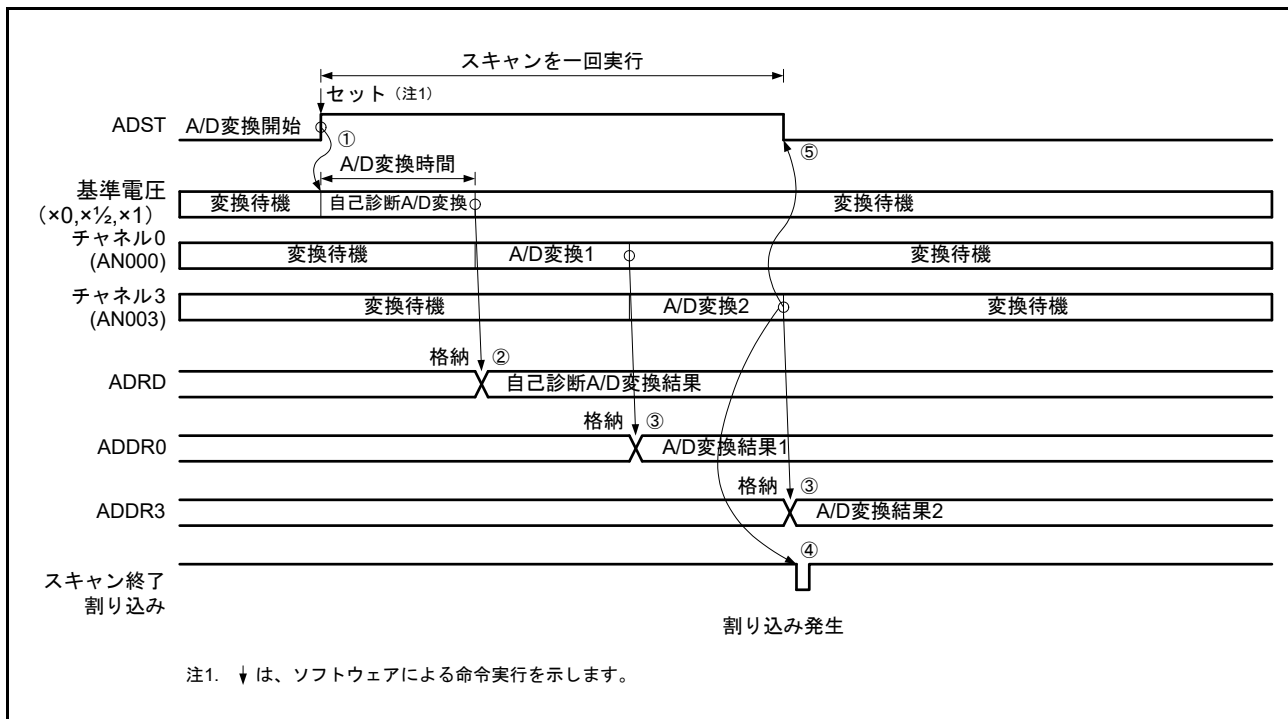
図 56.9 シングルスキャンモードの動作例 (基本動作 : AN000, AN003 選択 + 自己診断)
