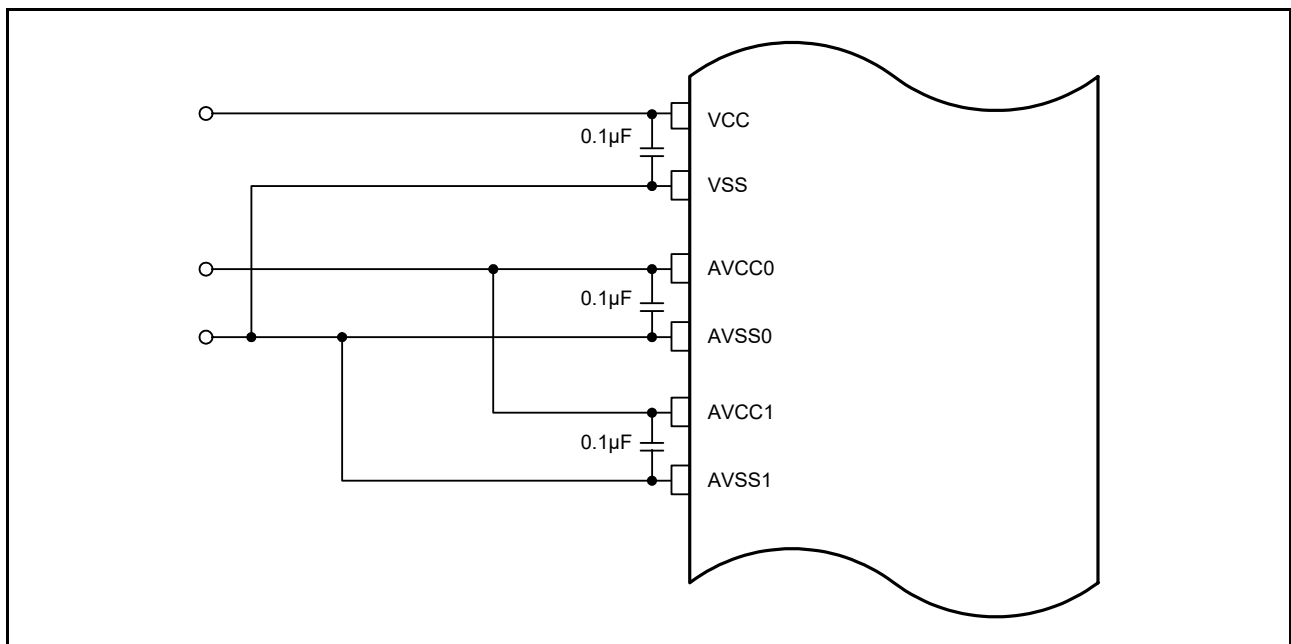
図 56.47 各電源端子の接続例
