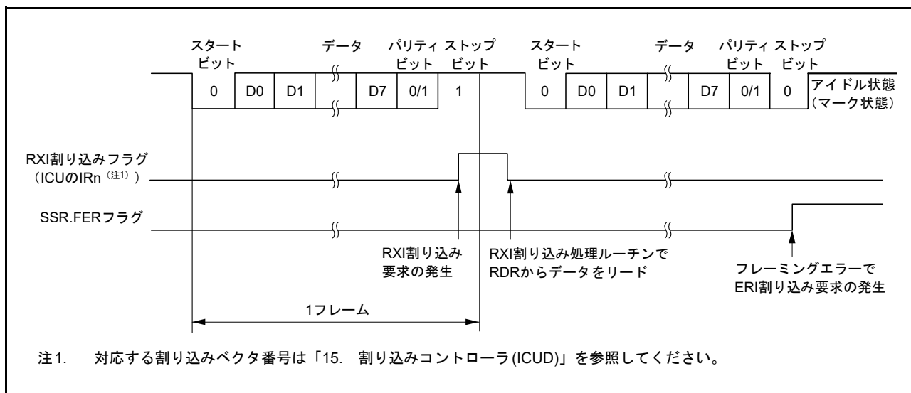
図 41.18 調歩同期式モードのシリアル受信時の動作例 (1) (RTS 機能未使用時) (8 ビットデータ / パリティあり / 1 ストップビットの例)
