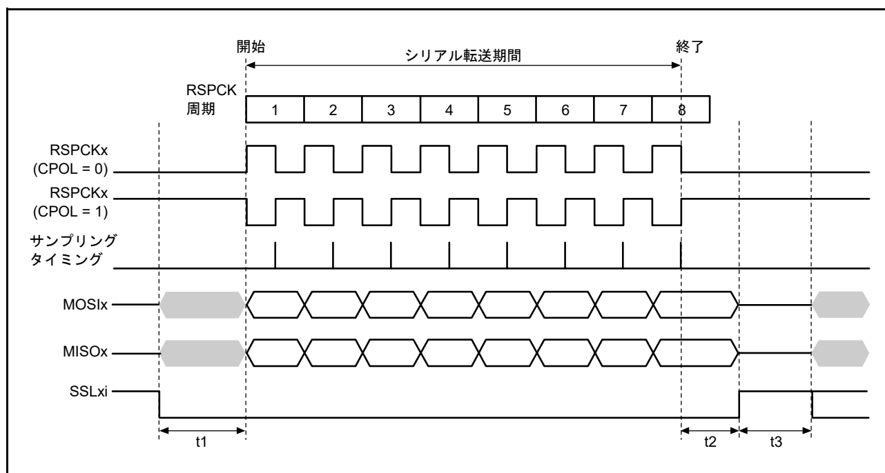
図 44.25 RSPI 転送フォーマット (CPHA ビット = 1)
