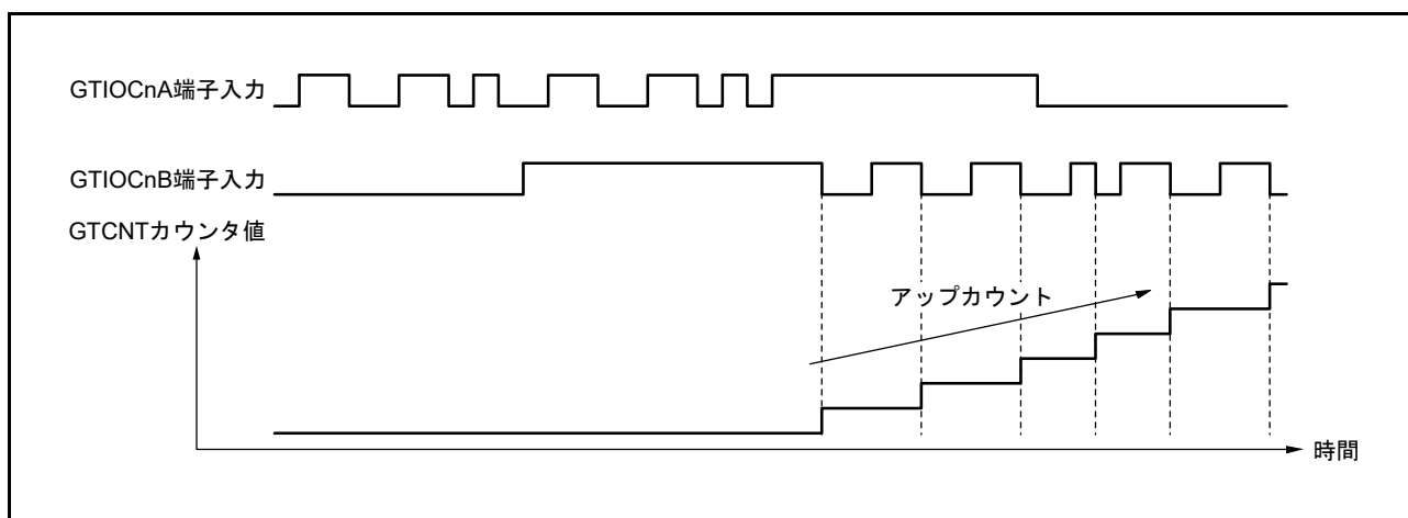
図 26.96 位相計数モード5の動作例 (n = 0 ~ 3)
