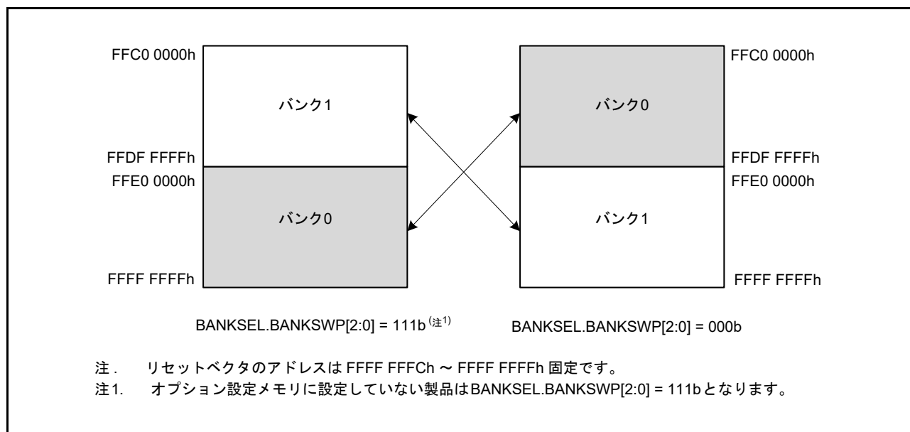
図 62.32 起動バンク選択例 (コードフラッシュメモリ容量が 4M バイトの製品の例)
