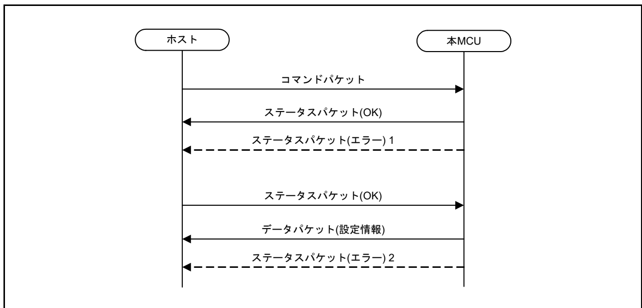
図 62.44 設定情報を取得するコマンドの共通通信シーケンス
