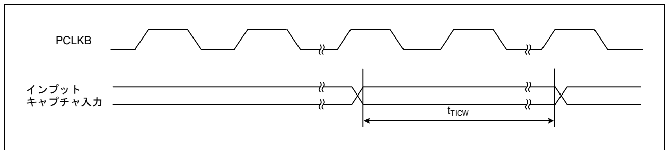
図 63.36 TPU インプットキャプチャ入力タイミング
