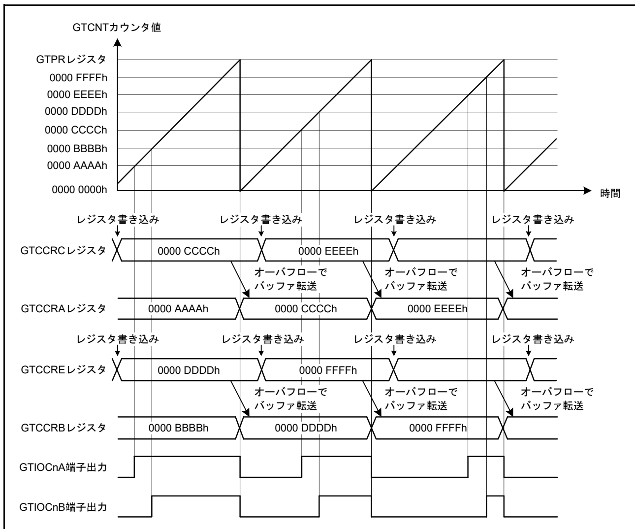
図 26.37 のこぎり波 PWM モード動作例
