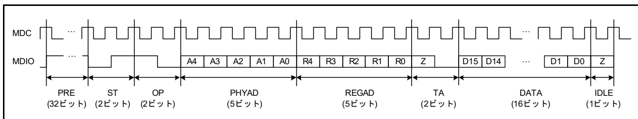
図 39.2 リードアクセスのデータフォーマット
