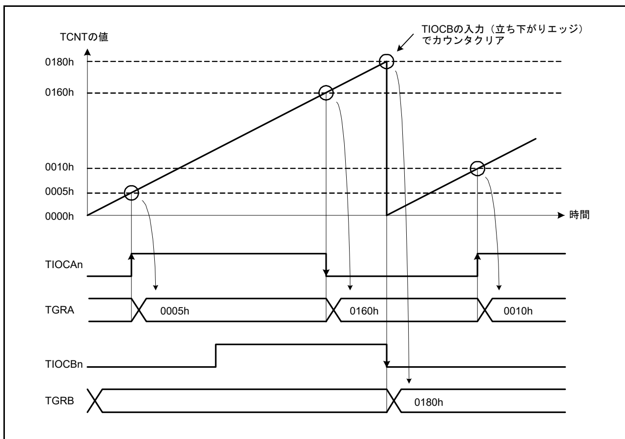
図 28.9 インพุットキャプチャ動作例 (ノイズフィルタ停止) (n = 0 ~ 5)
