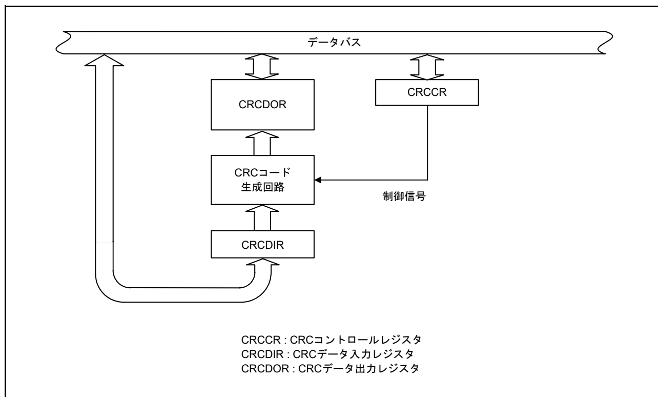
図 46.1 CRC 演算器のブロック図
