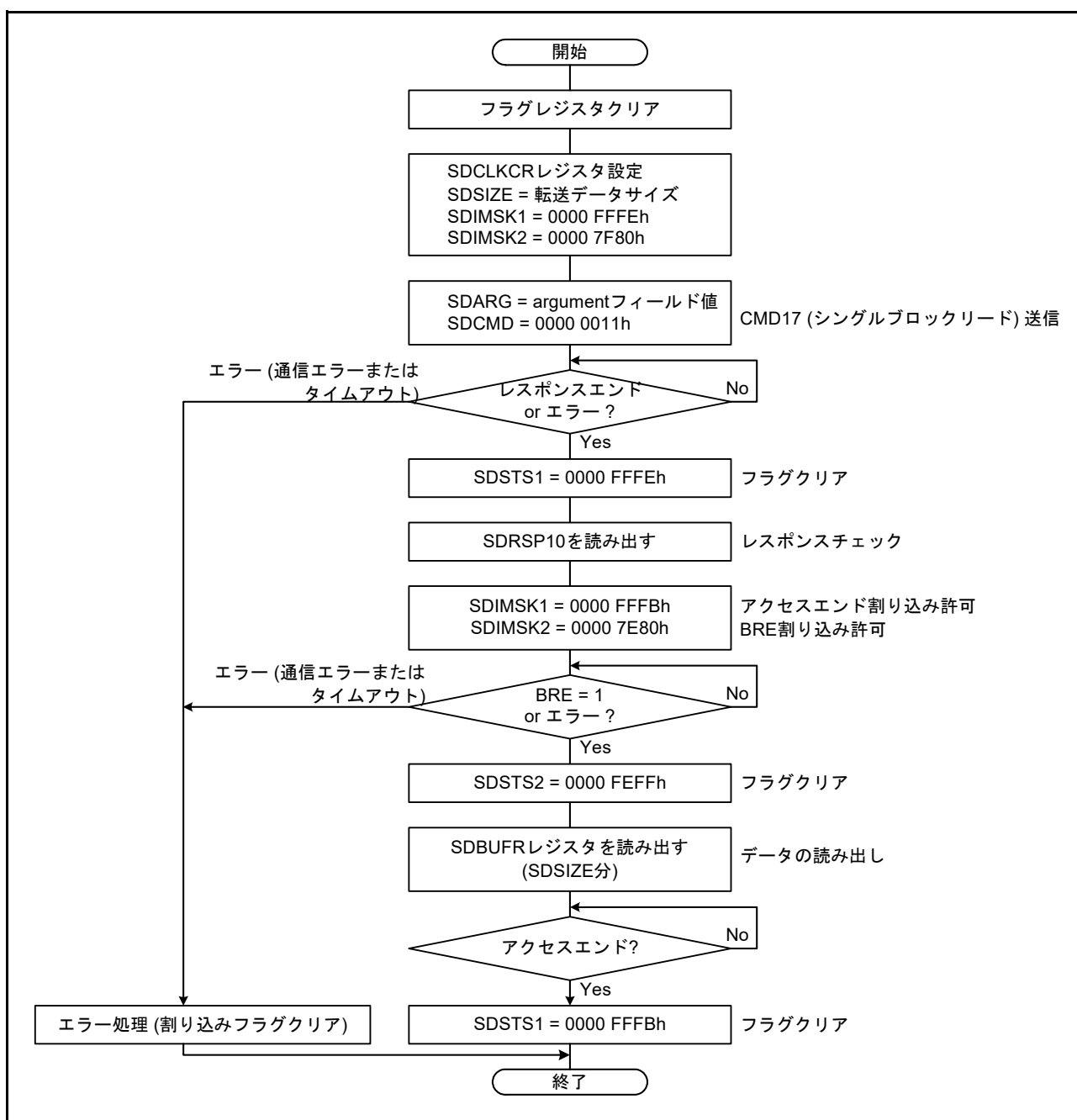
図 48.10 シングルブロックリードコマンドの送信例
