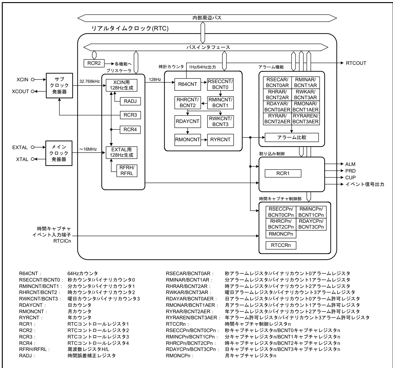
図 33.1 RTC のブロック図 (n = 0 ~ 2)
