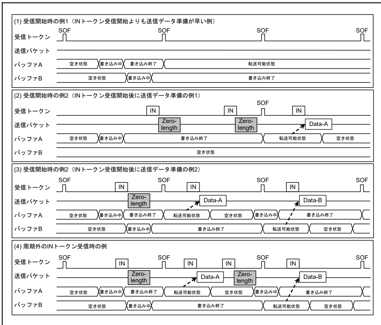
図 40.20 データセットアップ機能動作例
