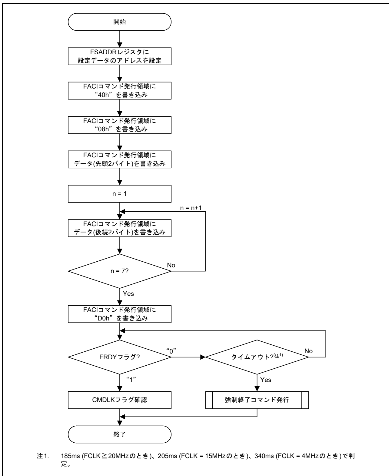
図 62.25 コンフィギュレーション設定コマンドの使用法
