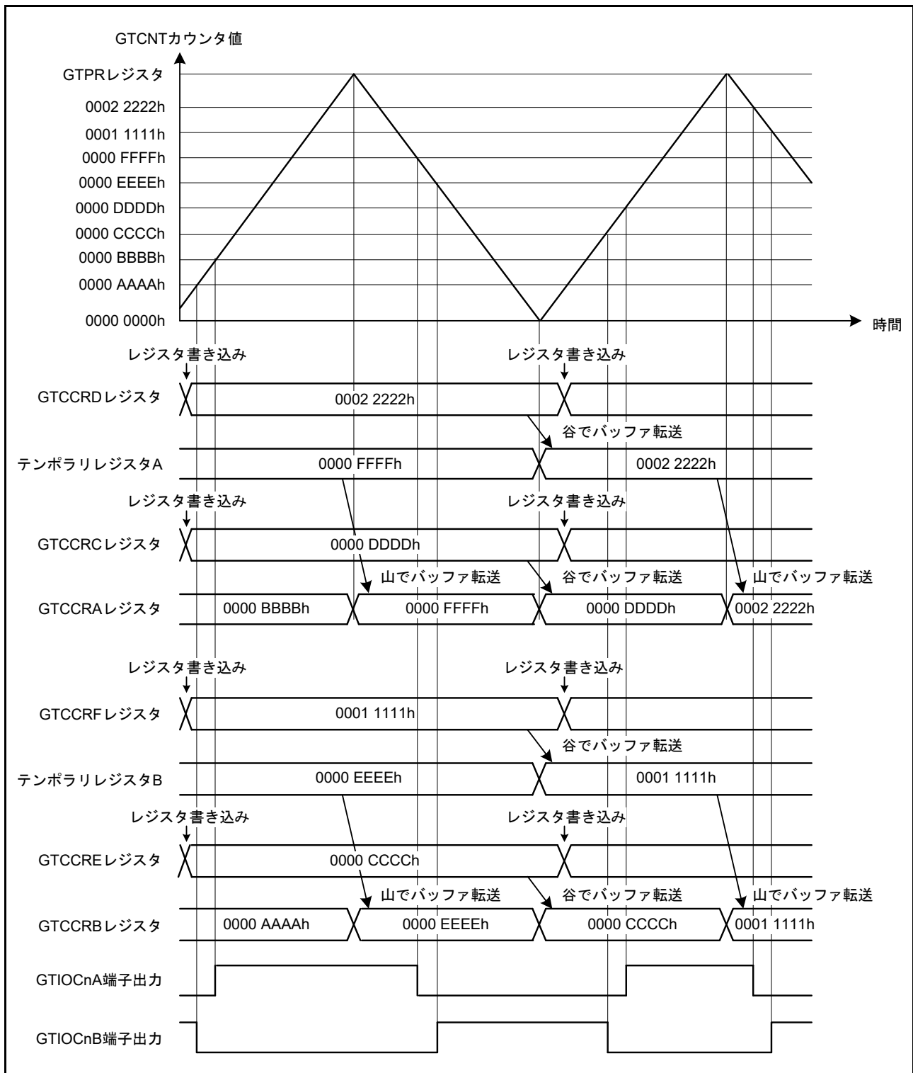
図 26.45 三角波 PWM モード 3 動作例 (初期出力で GTIOCnA 端子 = Low 出力 / GTIOCnB 端子 = High 出力、GTCCRA/GTCCRB レジスタのコンペアマッチでトグル出力、周期の終わりで出力保持の場合) (n = 0 ~ 3)
