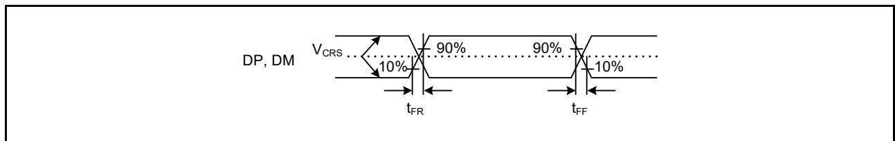
図 63.100 DP, DM 出カタイミング (フルスピード時)
