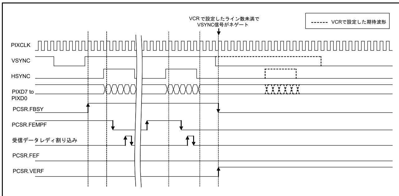
図 50.16 垂直方向ライン数設定エラー検出
