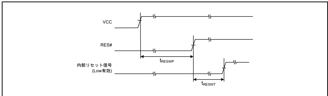
図 63.1 電源投入時リセット入力タイミング
