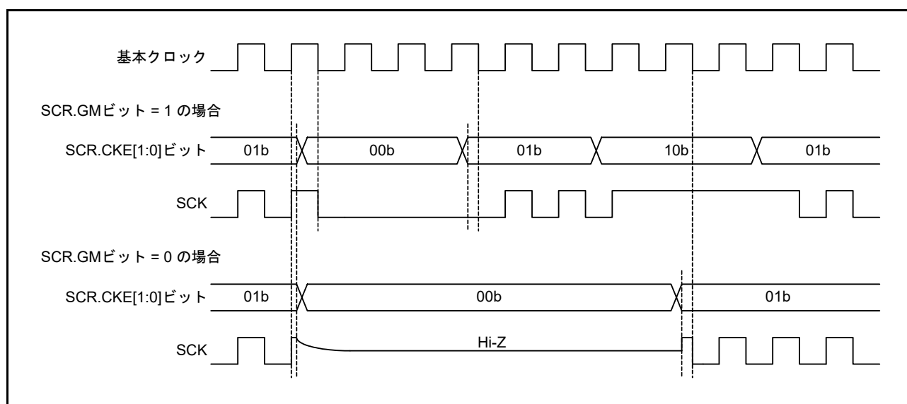
図 41.49 クロック出力制御
