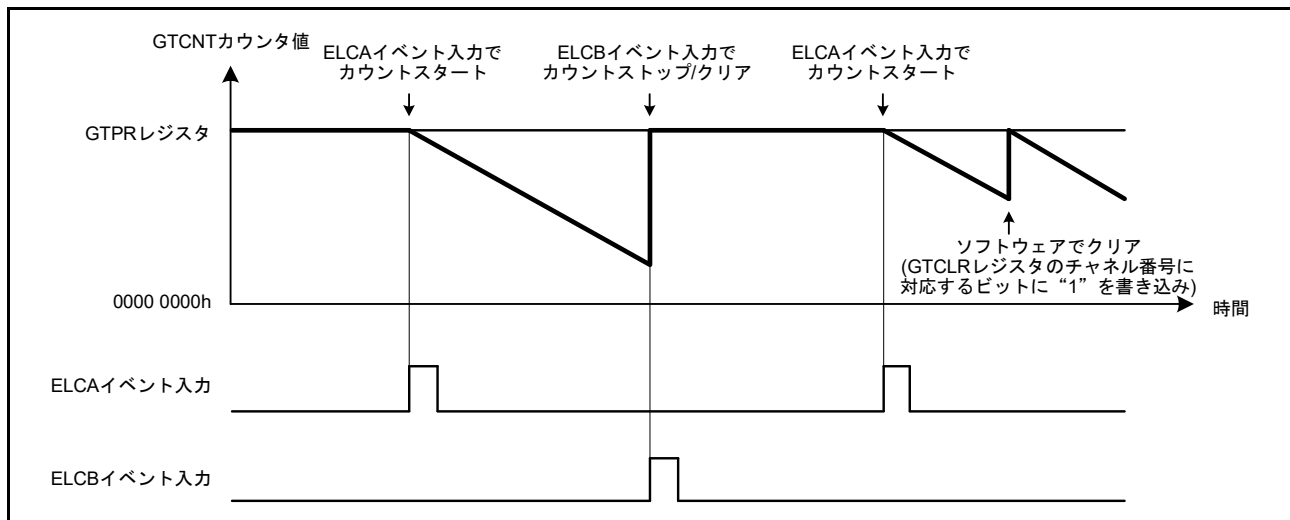
図 26.68 ハードウェア要因によるカウンタクリア動作例 (のこぎり波でダウンカウント、ELCA イベント入力でスタート、ELCB イベント入力でカウントストップ/クリア時)
