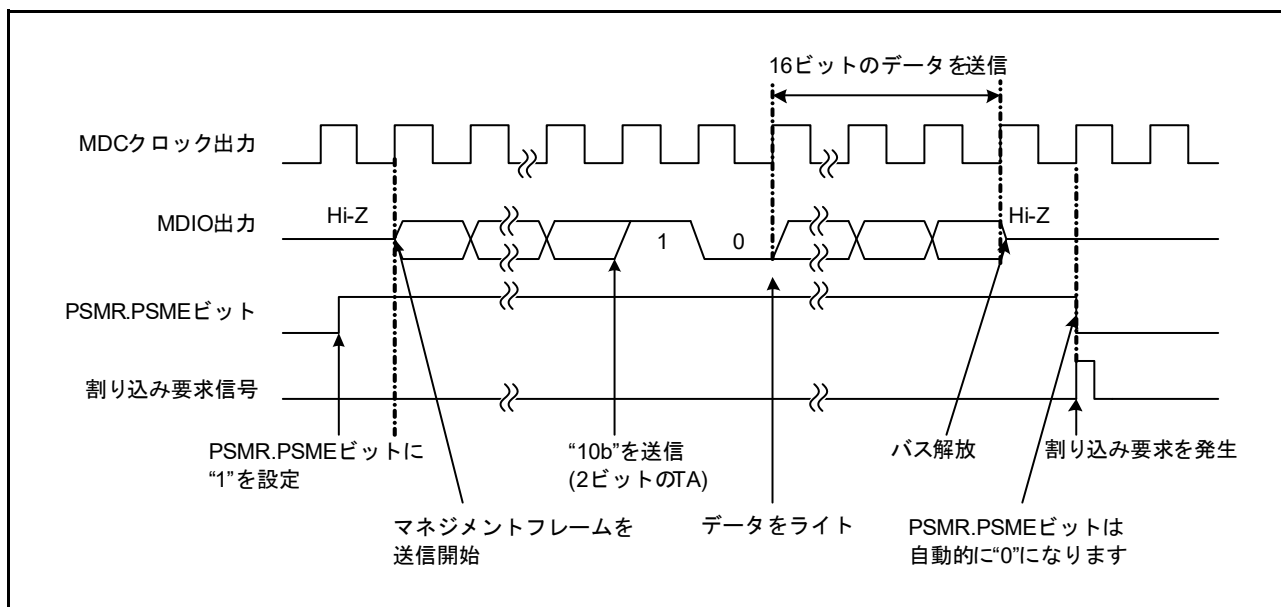
図 39.8 PHYレジスタライトの動作例
