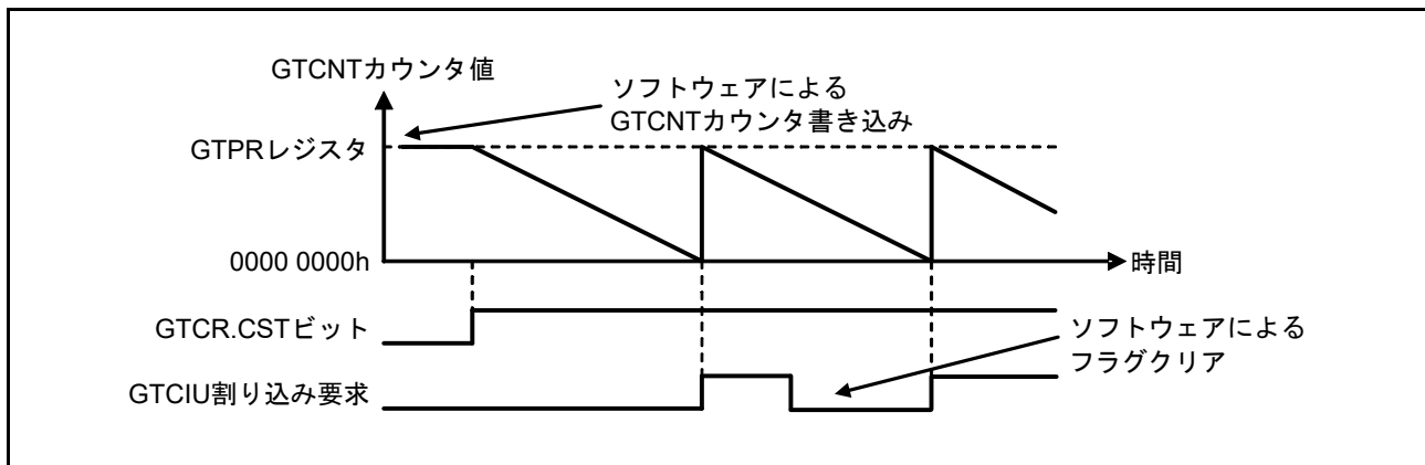
図 26.4 サイクルカウント動作例 (カウントクロックによるダウンカウント時)
