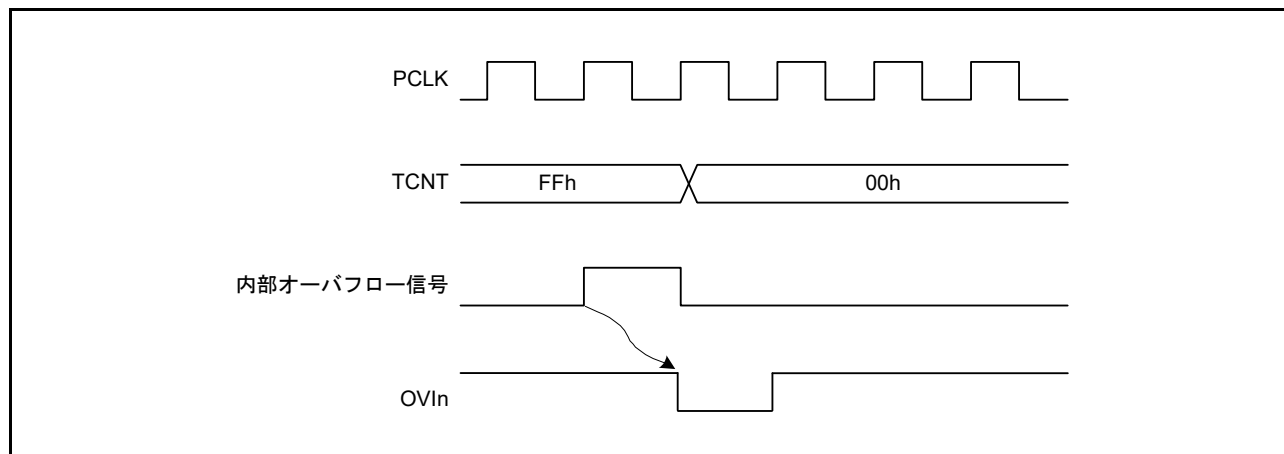
図 30.12 オーバフローによる割り込みタイミング (n = 0 ~ 3)
