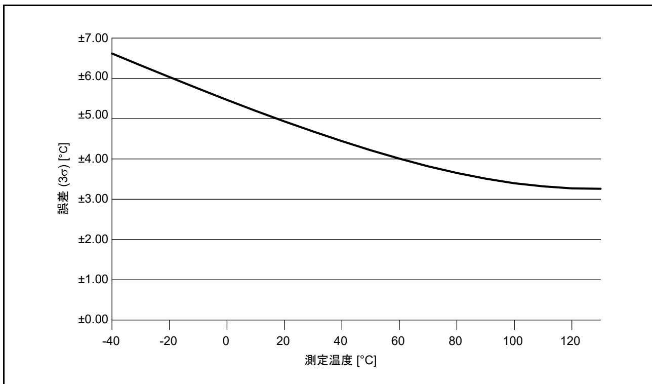
図 58.2 製品の測定温度誤差
