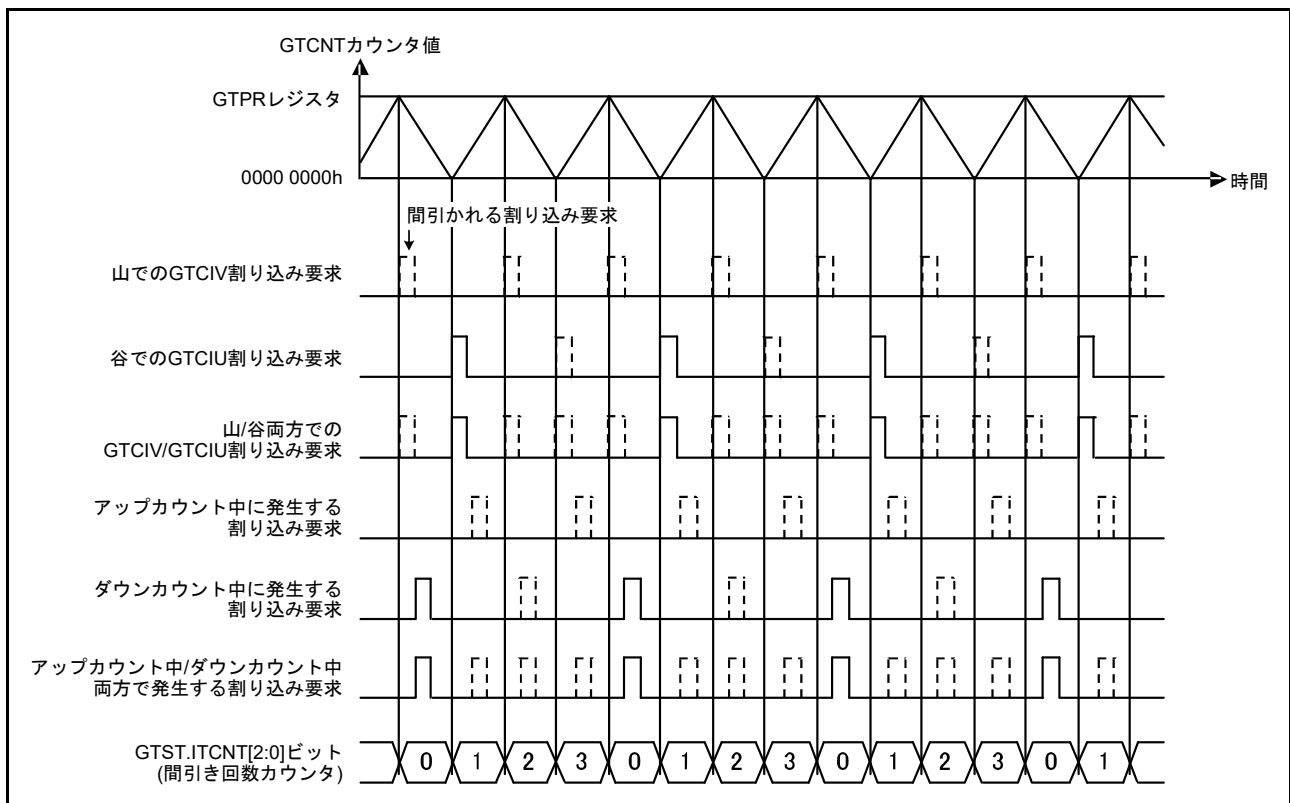
図 26.100 割り込み間引き機能の動作例 (三角波、谷 / 山両方をカウントして間引き、間引き回数 3、アップカウントで間引き開始の場合)
