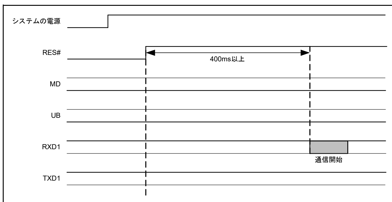
図 62.37 ブートモード (SCI インタフェース) で通信が可能になるまでの各端子の状態
