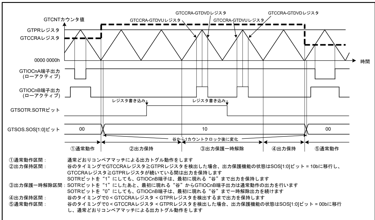
図 26.135 谷のバッファ転送で GTCCR レジスタ \geq GTPR レジスタが設定された場合の出力保護機能一時解除の動作例 (谷のバッファ転送で 0 < GTCCR レジスタ < GTPR レジスタに復帰、アクティブレベルは Low の場合) (n = 0 ~ 3)
