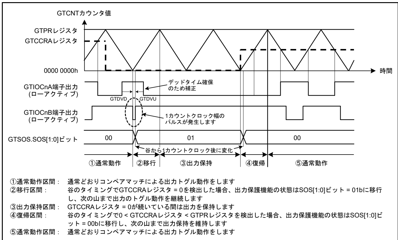
図 26.129 山のバッファ転送で GTCCRA レジスタが “0000 0000h” である場合の出力保護機能の動作例 (谷のバッファ転送で 0 < \text{GTCCRA レジスタ} < \text{GTPR レジスタ} に復帰、アクティブレベルは Low の場合) ( n = 0 \sim 3 )
