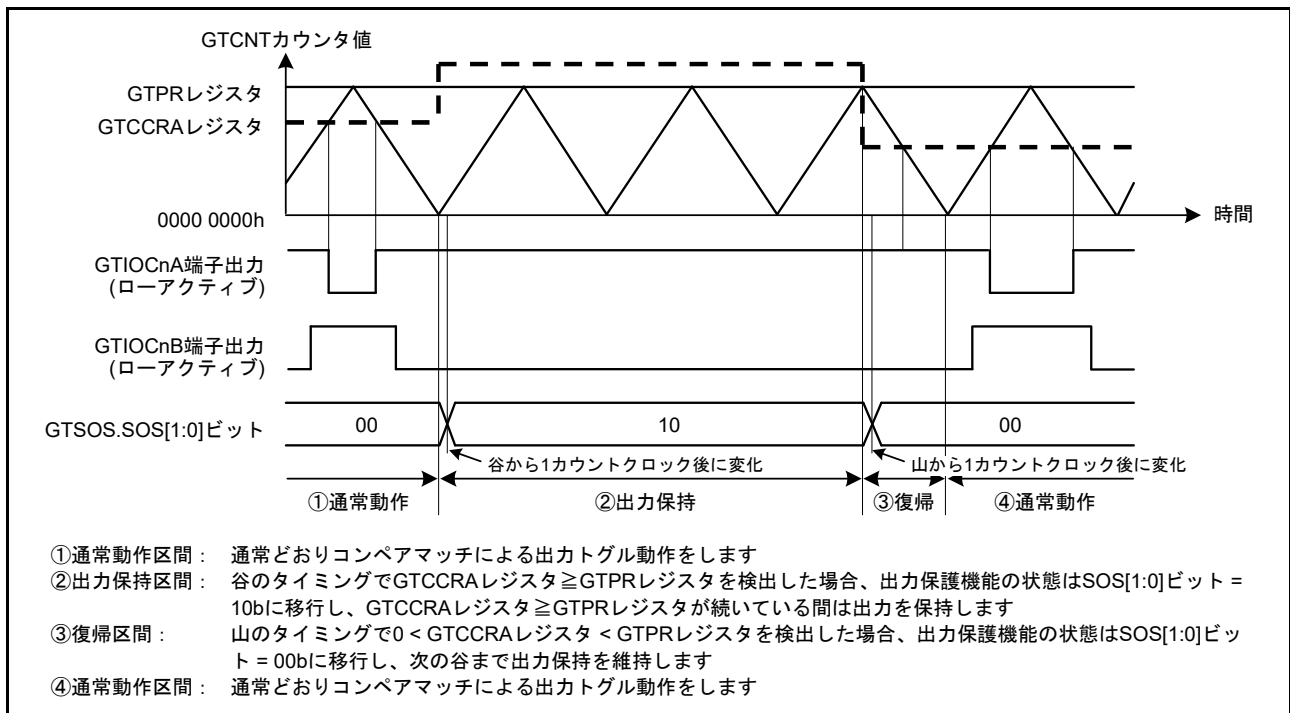
図 26.132 谷のバッファ転送で GTCCRA レジスタ \geq GTPR レジスタが設定された場合の出力保護機能の動作例 (山のバッファ転送で 0 < GTCCRA レジスタ < GTPR レジスタに復帰、アクティブレベルは Low の場合) ( n = 0 \sim 3 )
