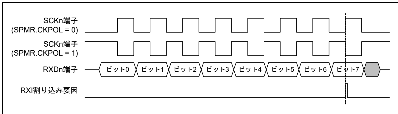
図 41.85 簡易 SPI モード (クロック遅れあり) RXI 割り込み発生タイミング
