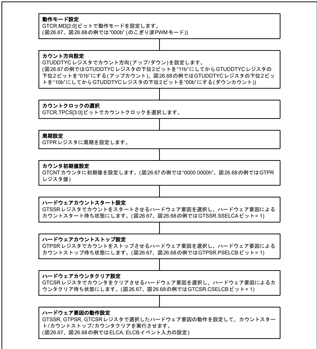
図 26.69 ハードウェア要因によるカウンタクリア動作設定例
