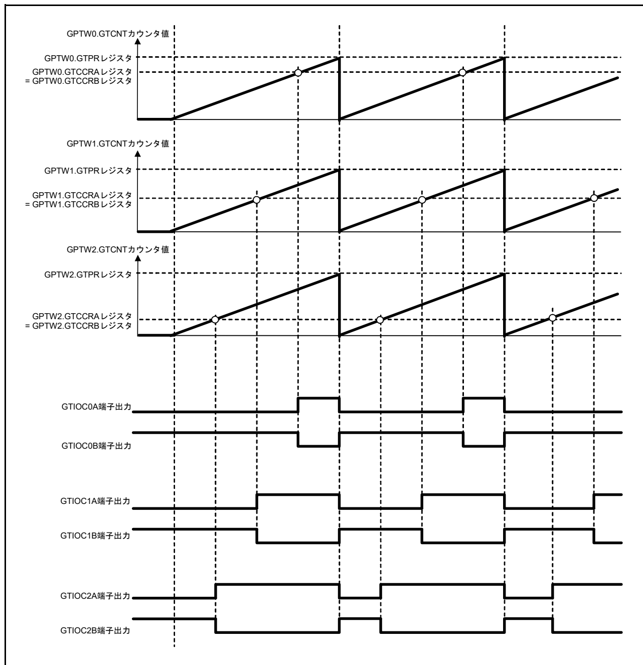
図 26.82 のこぎり波3相相補PWM出力
