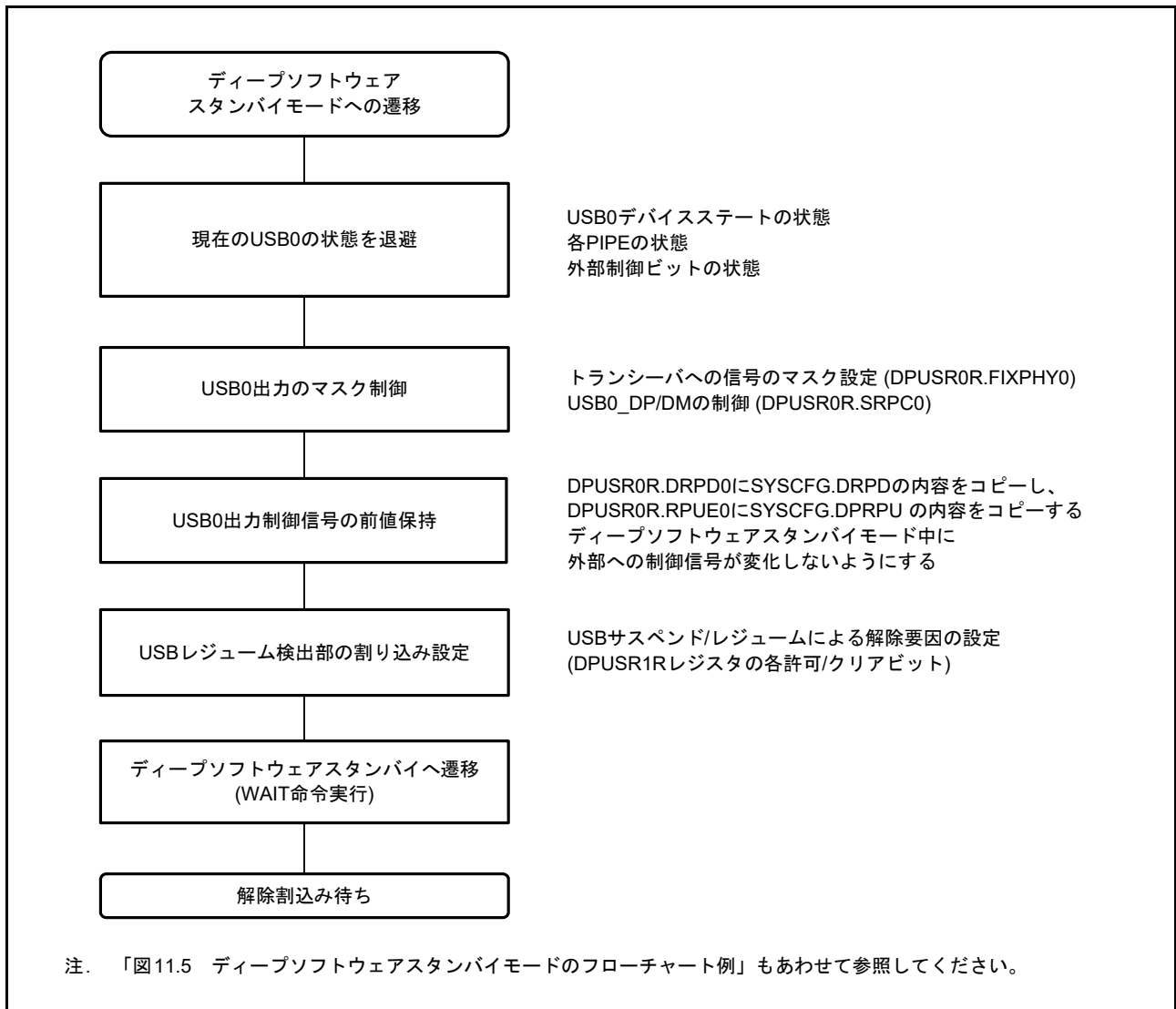
図 40.7 ホスト時またはファンクション時のディープソフトウェアスタンバイ遷移時の USB 設定フロー
