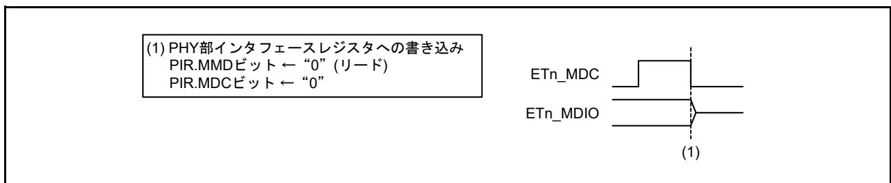
図 36.17 単独バス解放フロー (表 36.3 中のライト時の IDLE)
