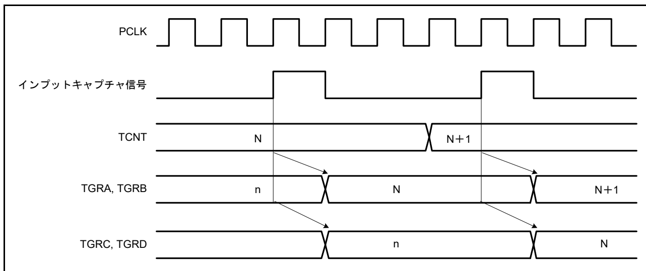
図 28.38 バッファ動作タイミング (インพุットキャプチャ)
