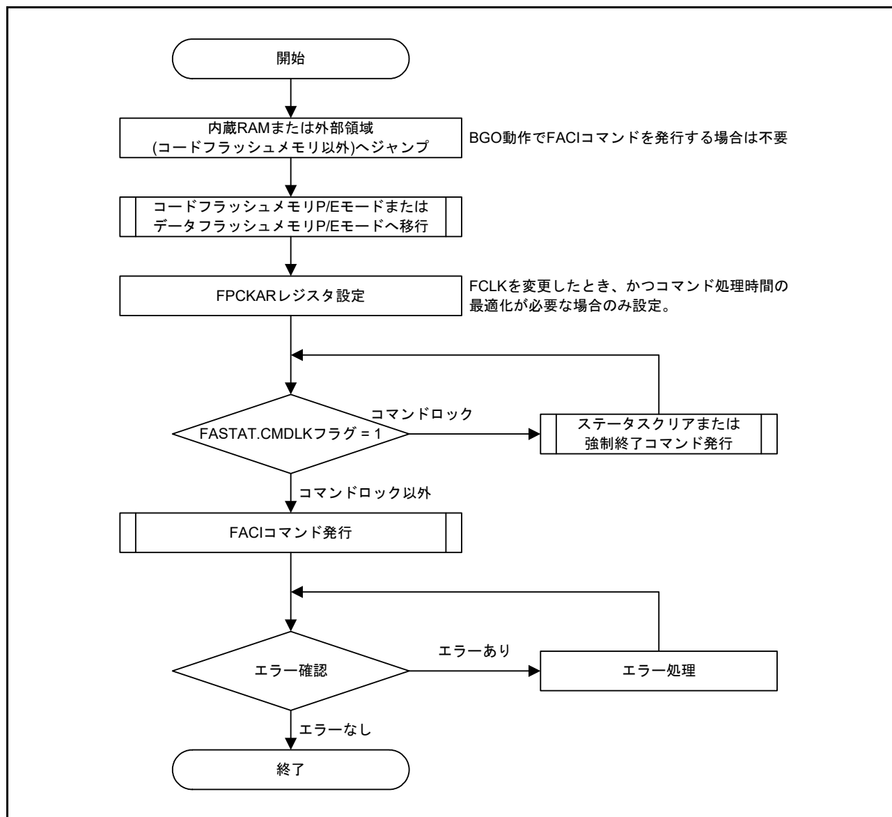
図 62.12 FACL コマンド使用時の概略フロー
