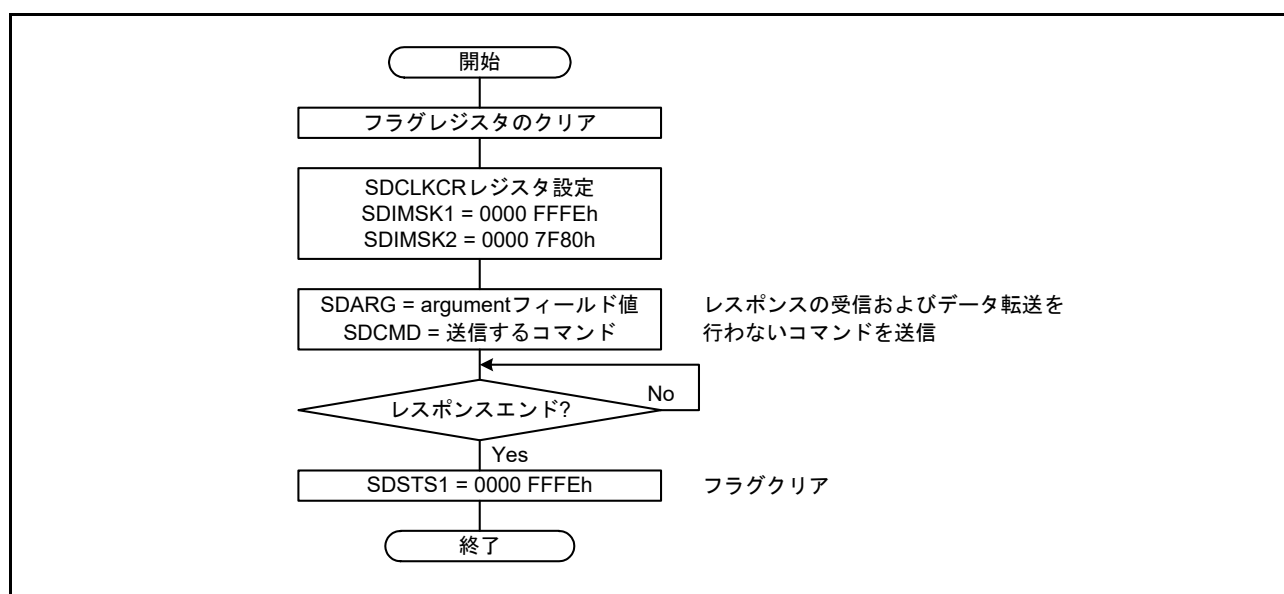
図 48.8 レスポンスの受信とデータ転送のないコマンドの送信例
