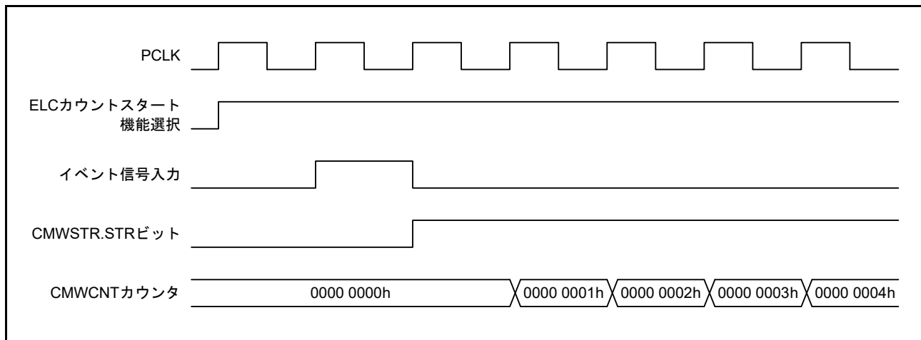
図 32.17 イベント受け付けによるカウントスタート動作
