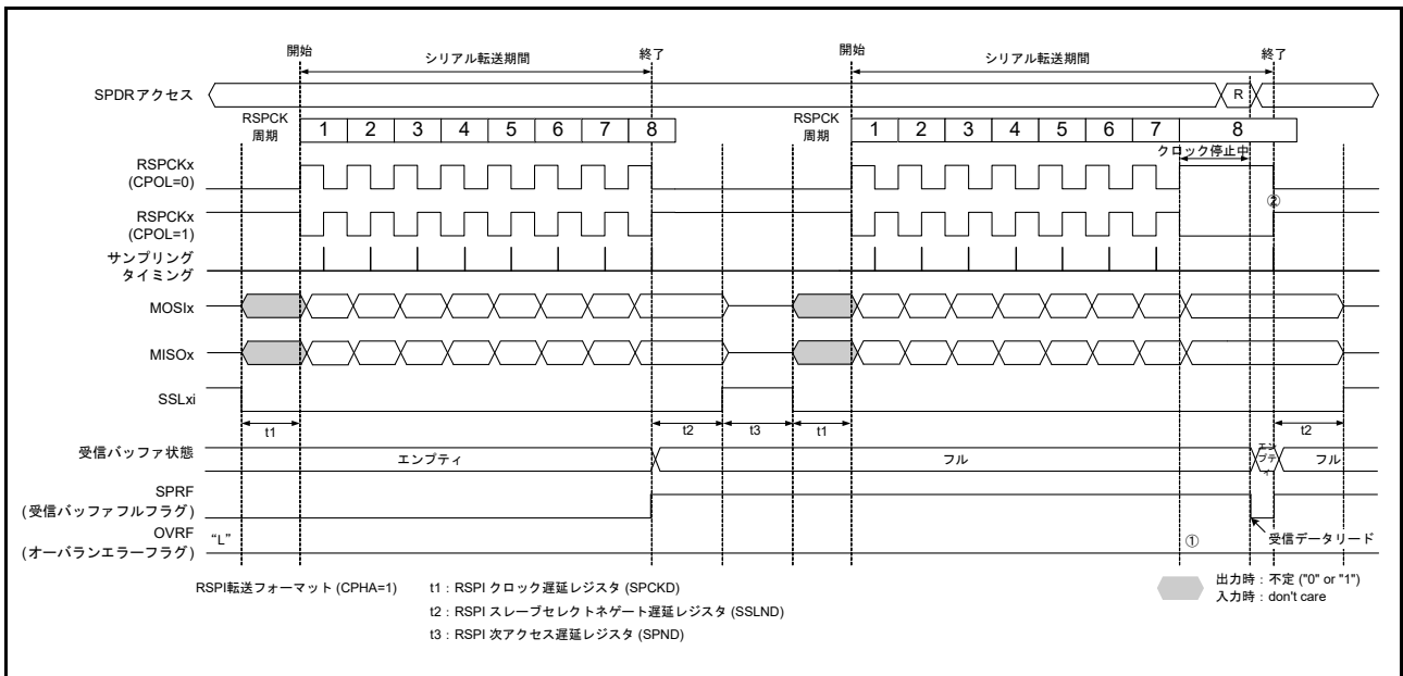
図 44.30 マスタモードの受信バッファフル状態でシリアル転送が継続するときのクロック停止波形 (CPHA = 1)
