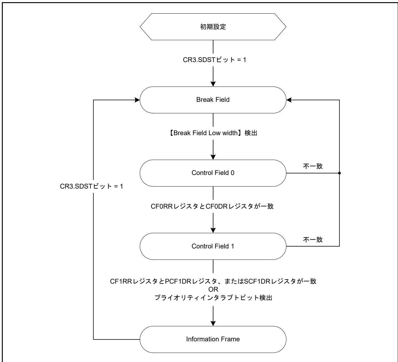
図 41.71 Start Frame 受信時の状態遷移図
