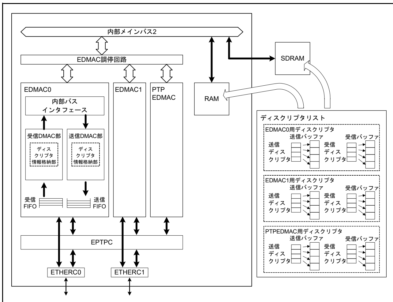
図 38.2 EDMAC とメモリ上のディスクリプタおよび送受信バッファの構成
