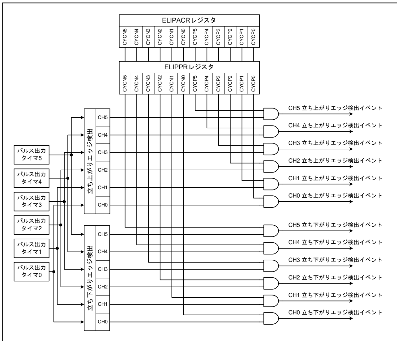
図37.38 パルス出力タイマとELCの関係
