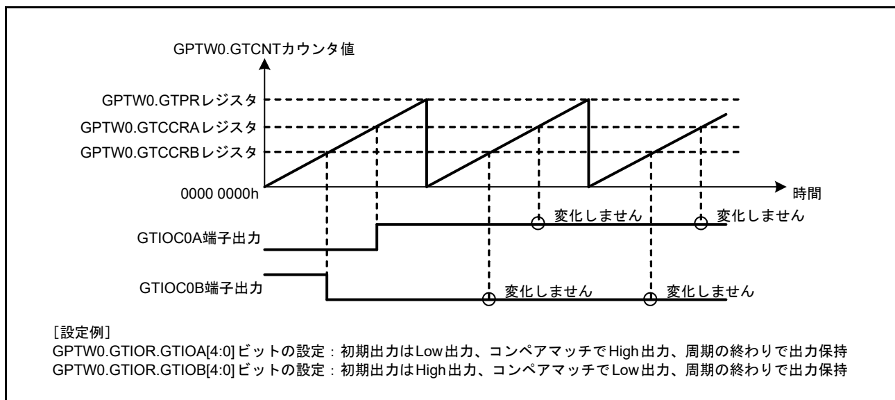
図 26.12 Low 出力 / High 出力動作例
