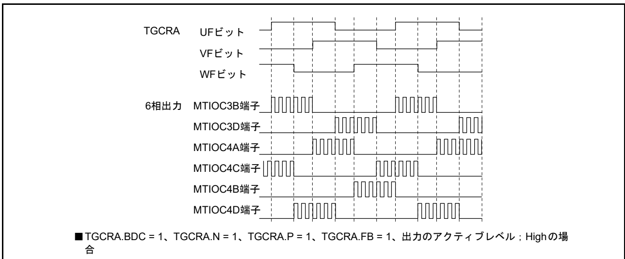
図 24.82 UF、VF、WF ビット設定による出力相の切り替え動作例 (2)
