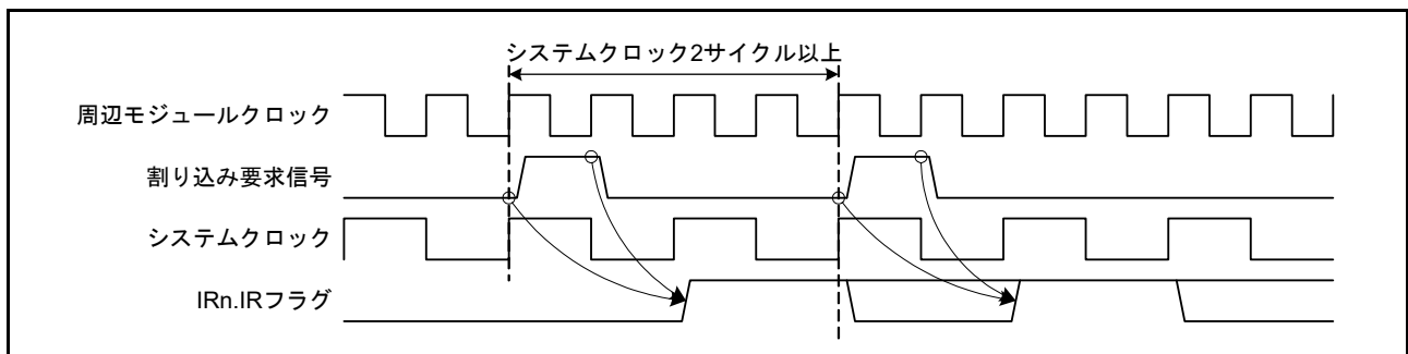
図 15.6 連続した割り込み要求信号の受け付け (システムクロック周波数 &lt; 周辺モジュールクロック周波数の場合)
