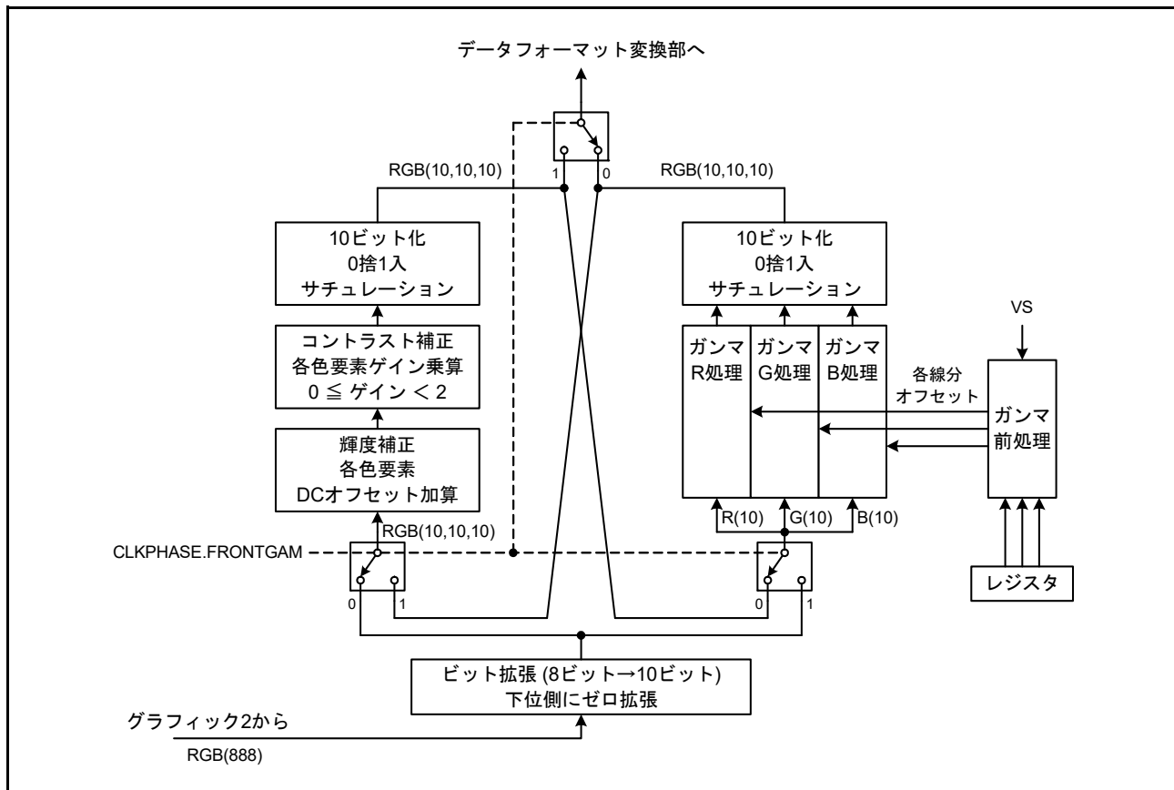
図 51.8 パネル用補正処理回路の構成
