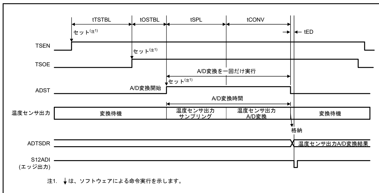
図 58.4 温度センサの動作から A/D 変換完了までのタイミング
