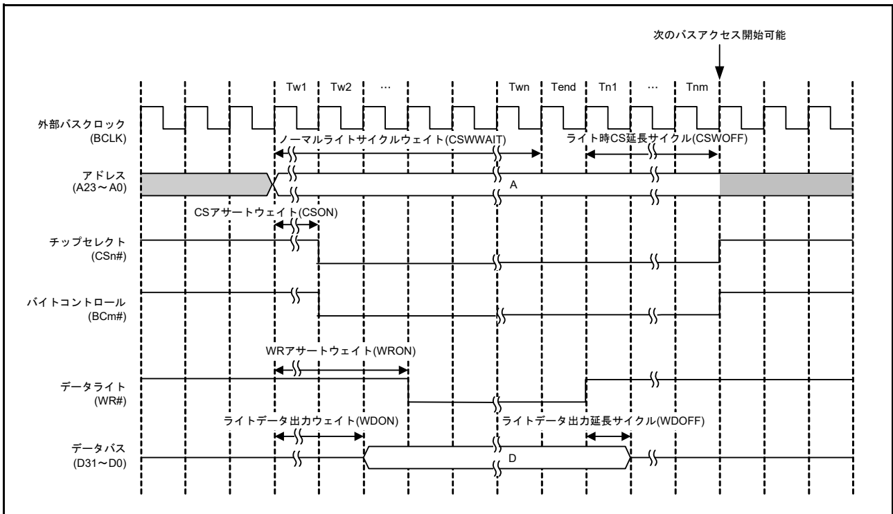
図 16.20 バスタイミング (ノーマルライト、1 ライトストローブモード) (n = 0 ~ 7, m = 0 ~ 3)
