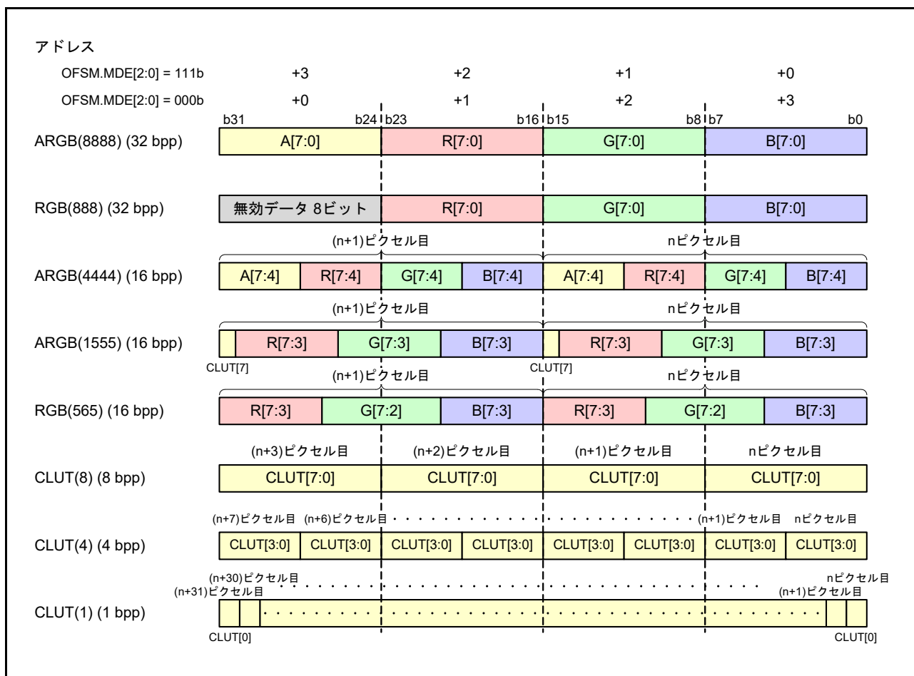
図 51.6 フレームデータのカラーフォーマット
