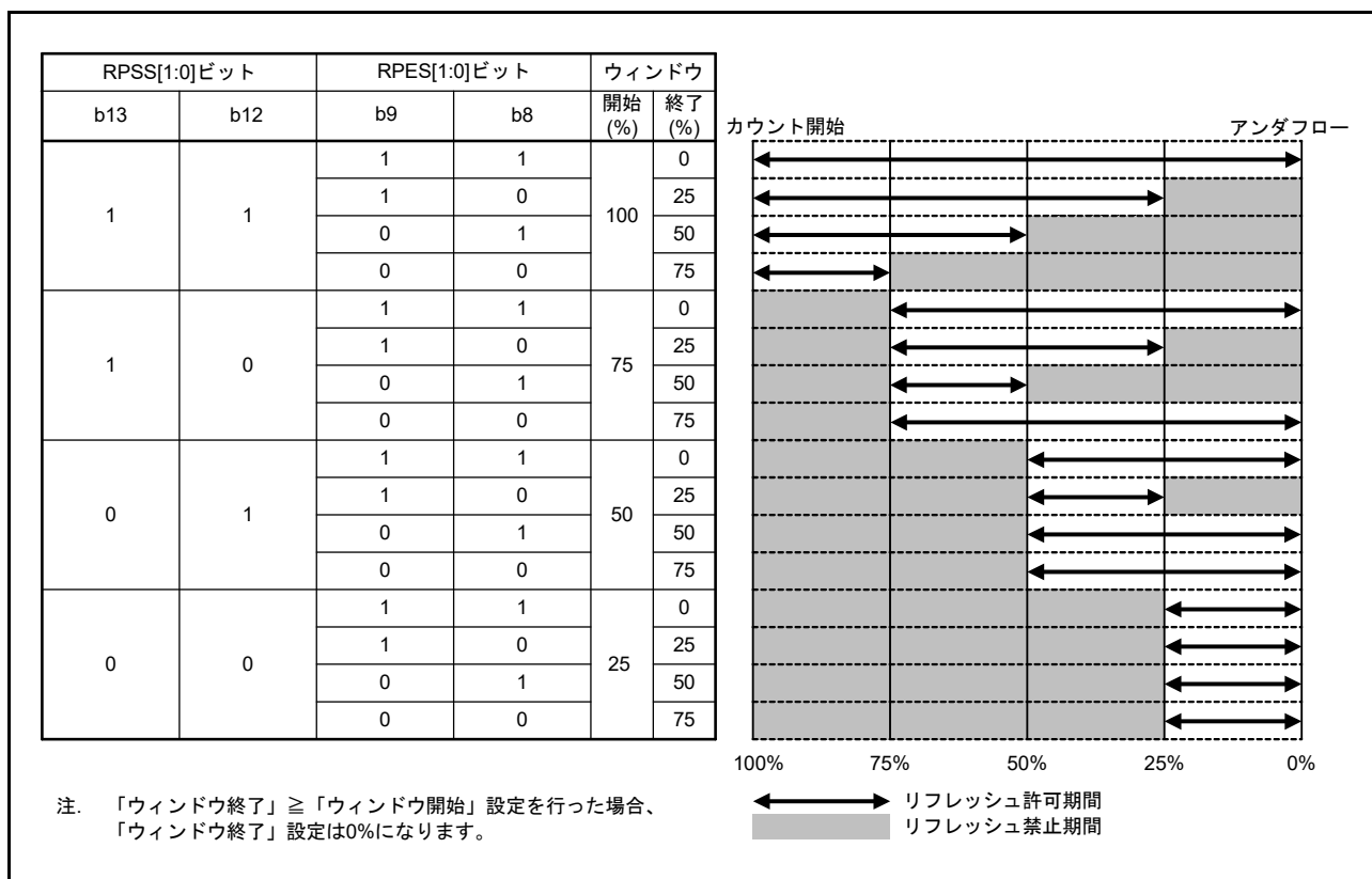
図 35.2 RPSS[1:0] ビット、RPES[1:0] ビットとリフレッシュ許可期間
