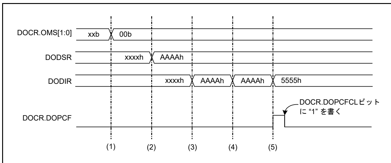
図 59.2 データ比較モードの動作例
