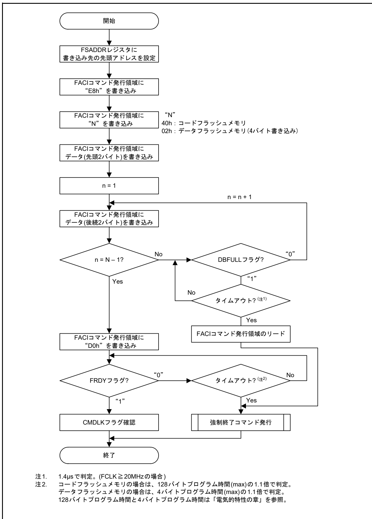
図 62.14 プログラムコマンドの使用方法
