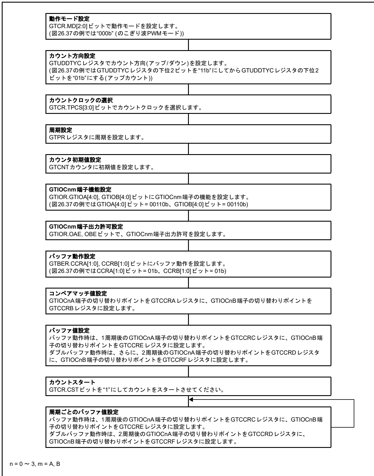
図 26.38 のこぎり波 PWM モード設定例
