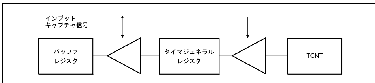
図 28.13 インプットキャプチャバッファ動作
