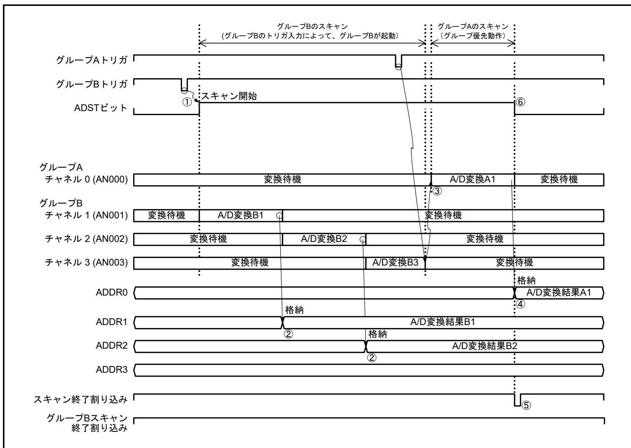
図 56.28 グループ優先動作の例 4 「グループ B スキャン中のグループ A トリガ入力」再スキャンなし (ADGSPCR.GBRSCN = 0, ADGSPCR.GBRP = 0, ADGSPCR.LGRRS = 0 設定時)
