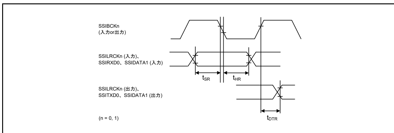
図 63.76 SSICR.BCKP = 1 の場合の SSIE データ送受信タイミング
