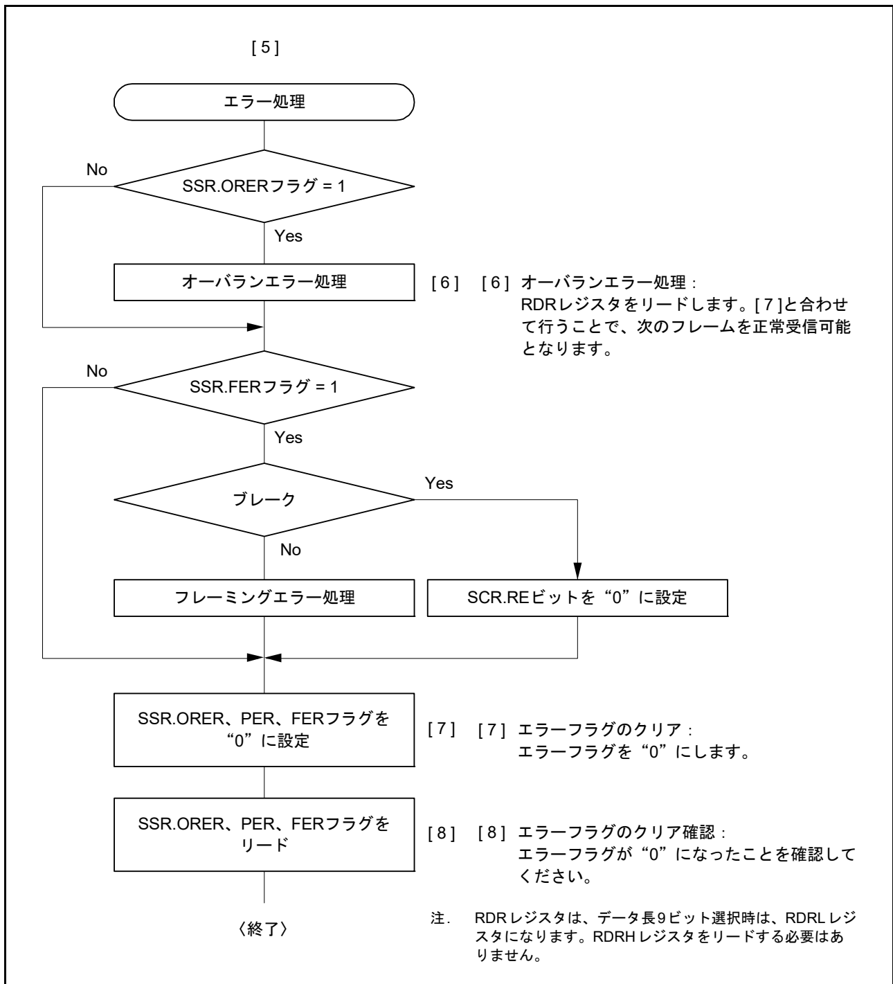
図 41.26 マルチプロセッサシリアル受信のフローチャートの例 (2)
