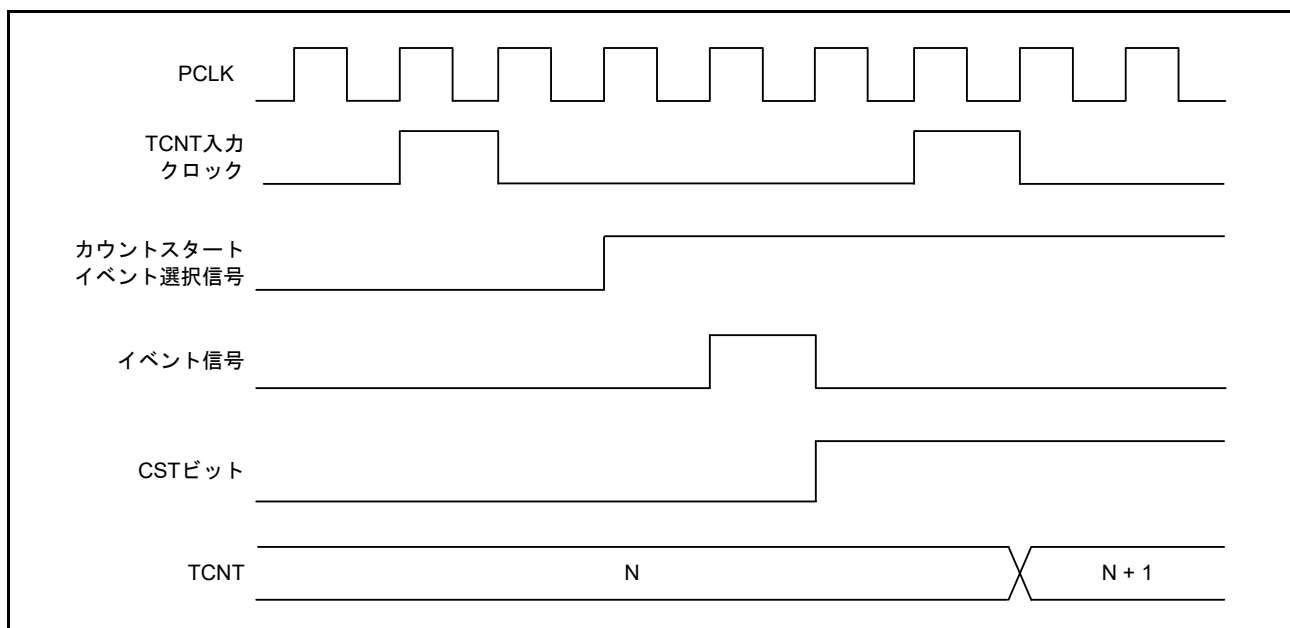
図 28.56 イベント信号入力によるカウントスタート動作
