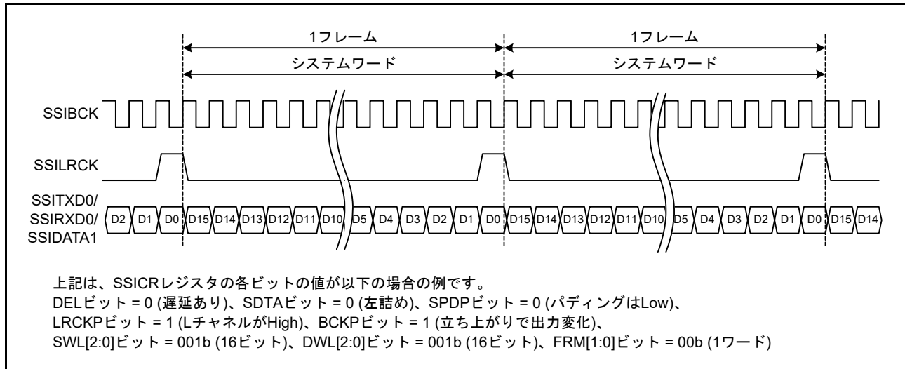
図 47.12 モノラルフォーマットの例 (1) (SSICR.DEL ビット = 0、パディングなし)
