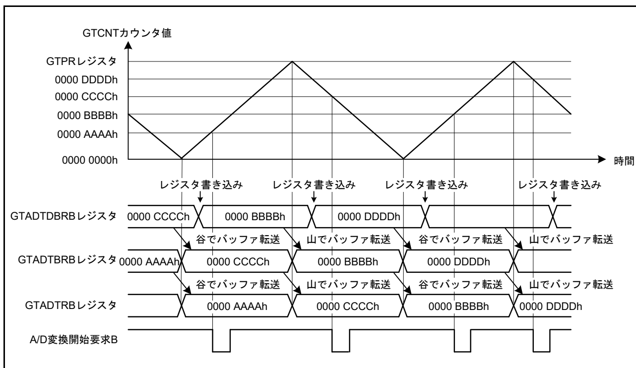
図 26.35 GTADTRA, GTADTRB レジスタのダブルバッファ動作例 (三角波、谷/山両方でバッファ転送、アップカウント/ダウンカウント両方で A/D 変換開始要求発生の場合)
