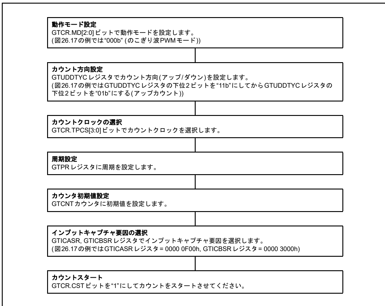
図 26.18 インプットキャプチャ動作設定例
