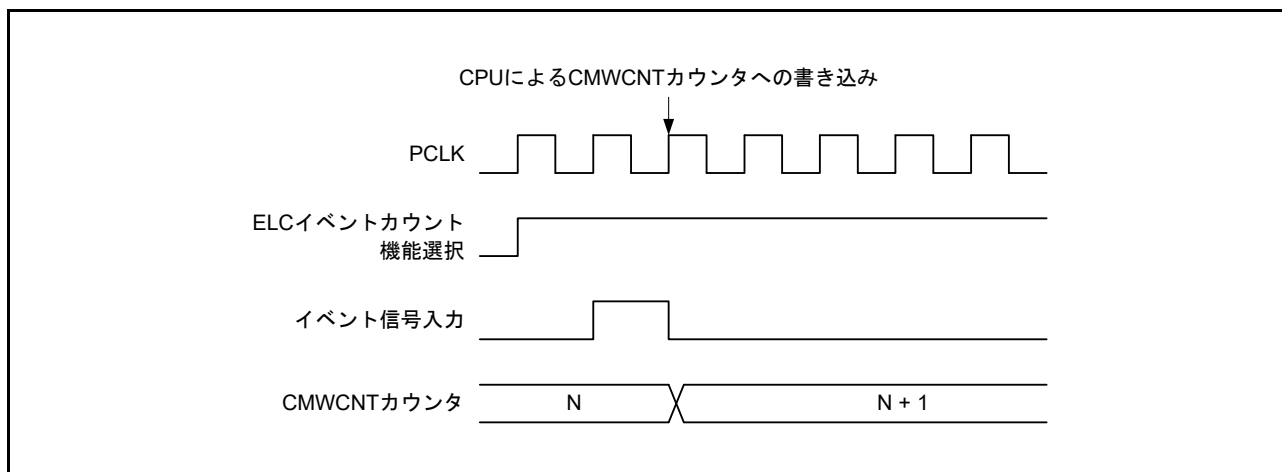
図 32.21 イベントカウント動作でのイベント受け付けとレジスタアクセスの競合
