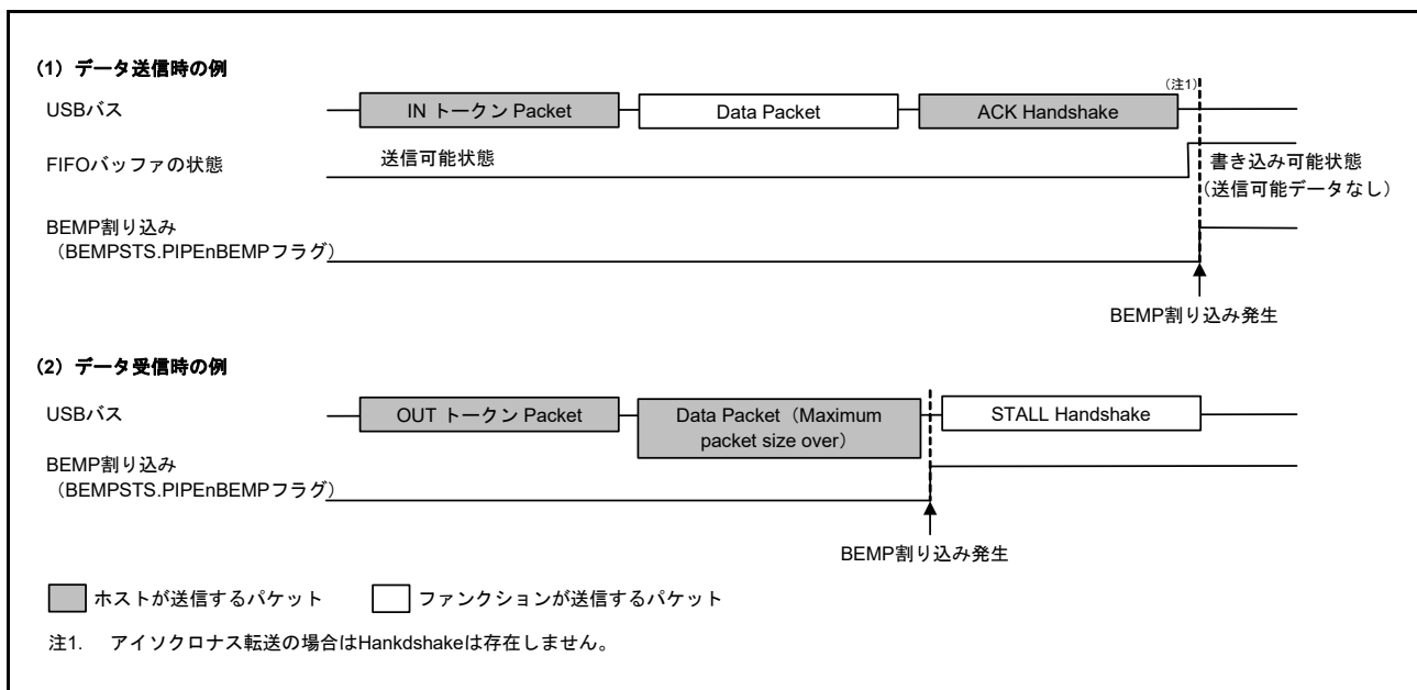
図 40.13 ファンクションコントローラ機能選択時の BEMP 割り込み発生タイミング図
