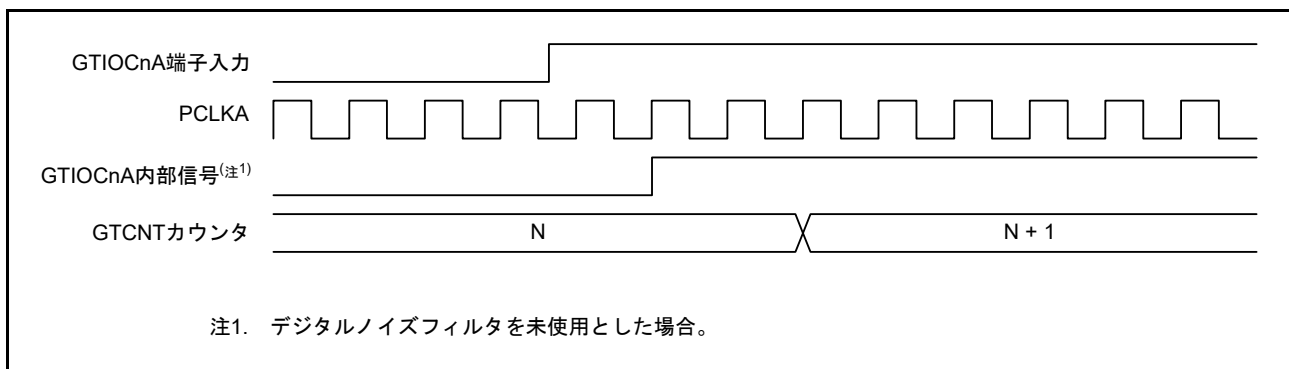
図 26.7 イベントカウント動作例 (GTIOCnA 端子入力の立ち上がりによるアップカウント)
