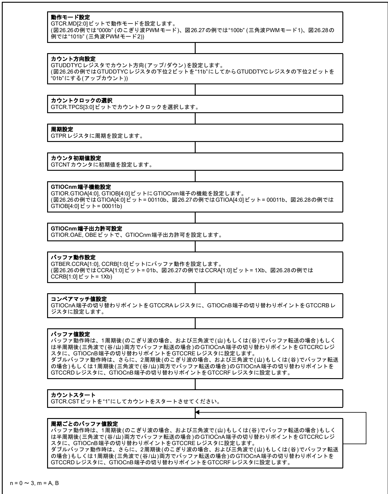
図 26.29 GTCCRA, GTCCRB レジスタのバッファ動作設定例 (アウトプットコンペア時)
