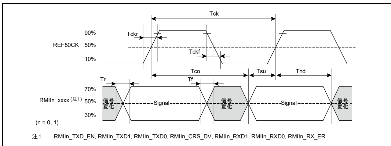
図 63.81 REF50CK と RMII 信号とのタイミング
