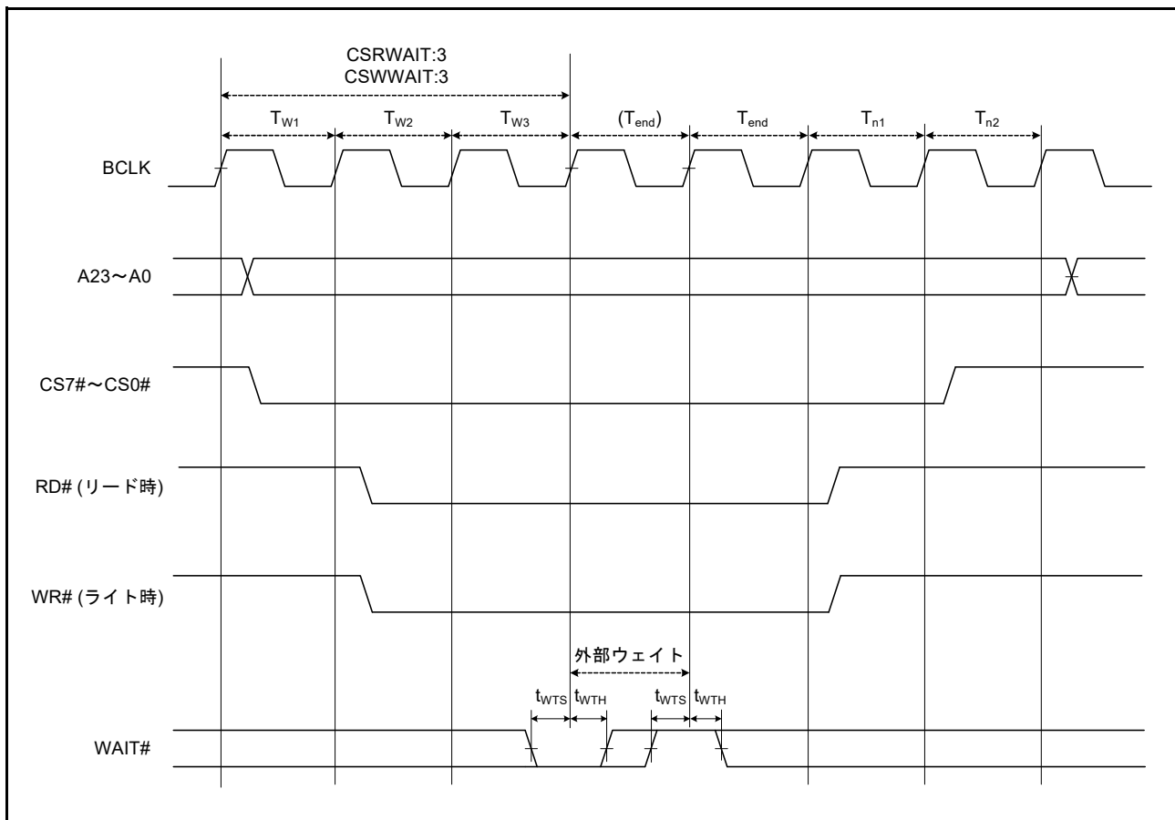
図 63.24 外部バスタイミング / 外部ウェイト制御
