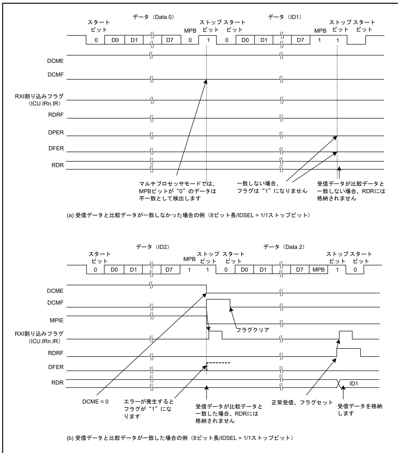
図 41.10 データ一致検出の例 (2) マルチプロセッサモード
