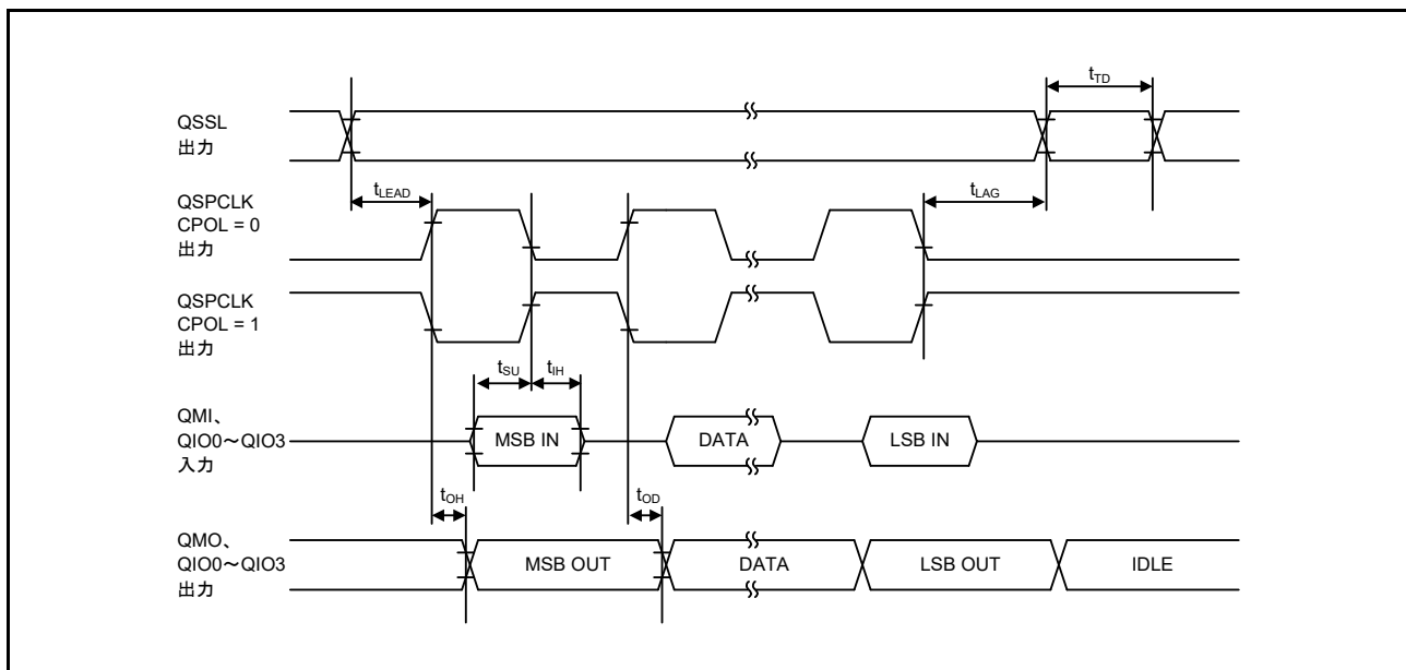
図 63.72 送受信タイミング (CPHA = 1)
