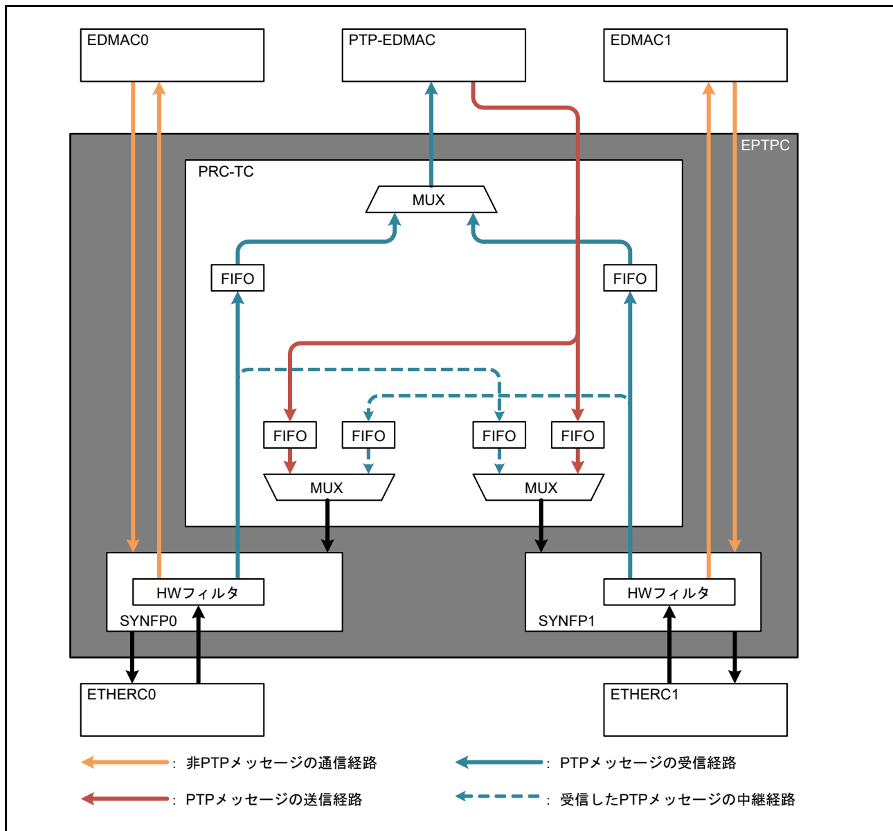
図37.4 フレームの転送および中継に関するモジュールのブロック図
