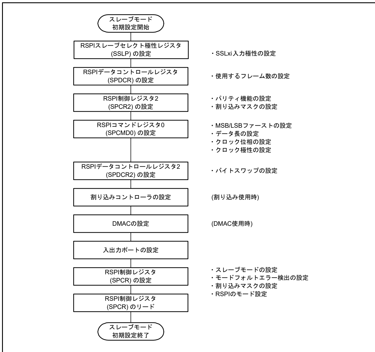
図 44.41 スレーブモード時の初期化フロー例 (SPI 動作)
