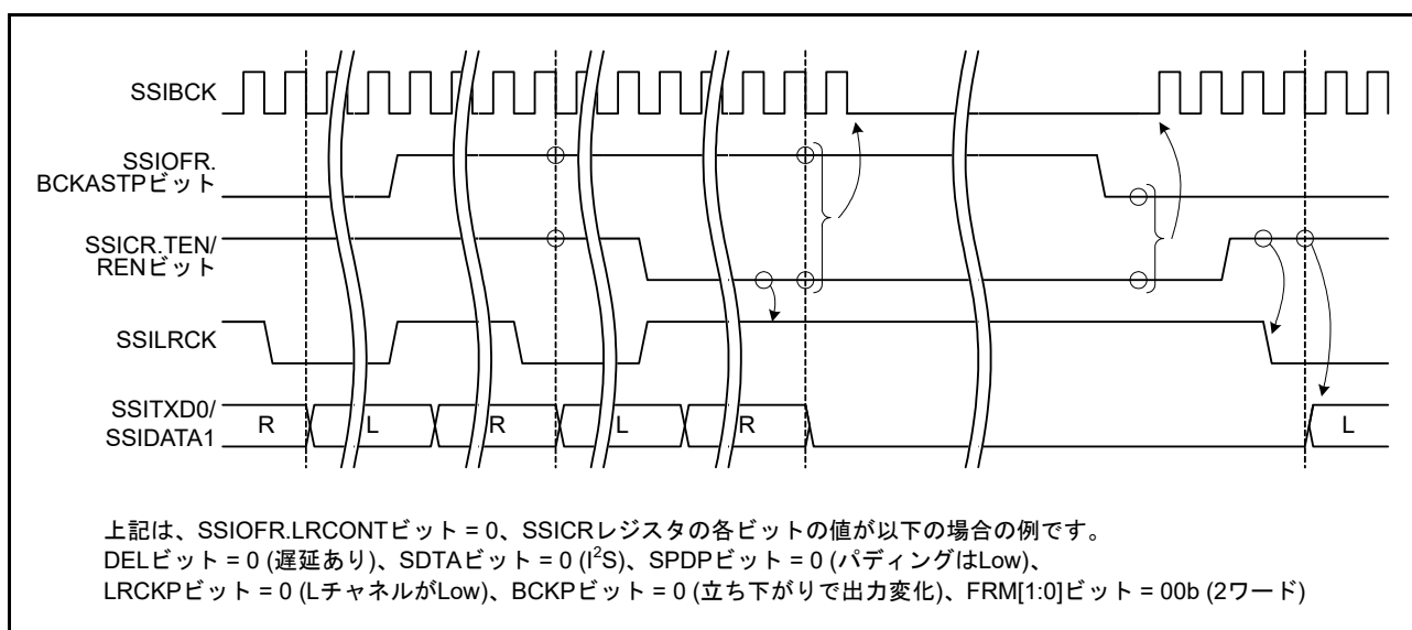
図 47.19 BCK 連続出力停止機能の動作例
