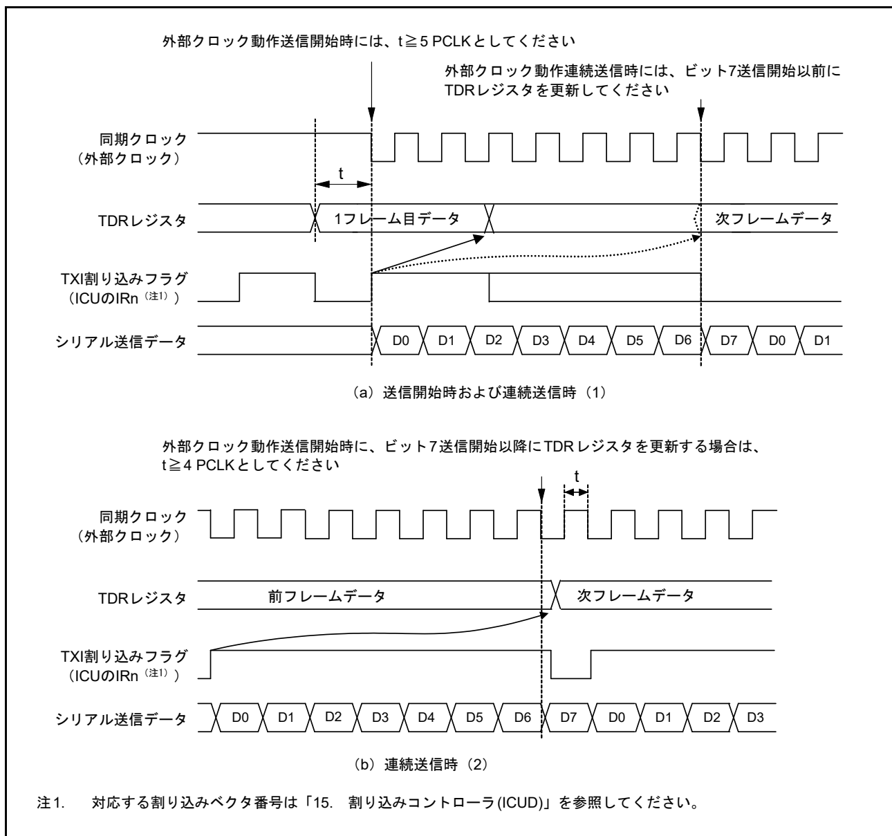
図 41.80 クロック同期式モード送信での外部クロック使用の制約事項
