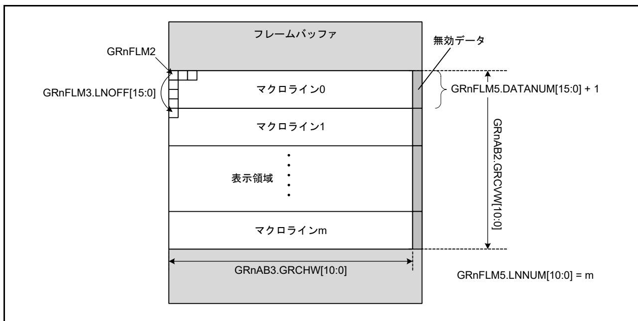
図 51.5 マクロラインを使用する場合のフレームバッファ設定例
