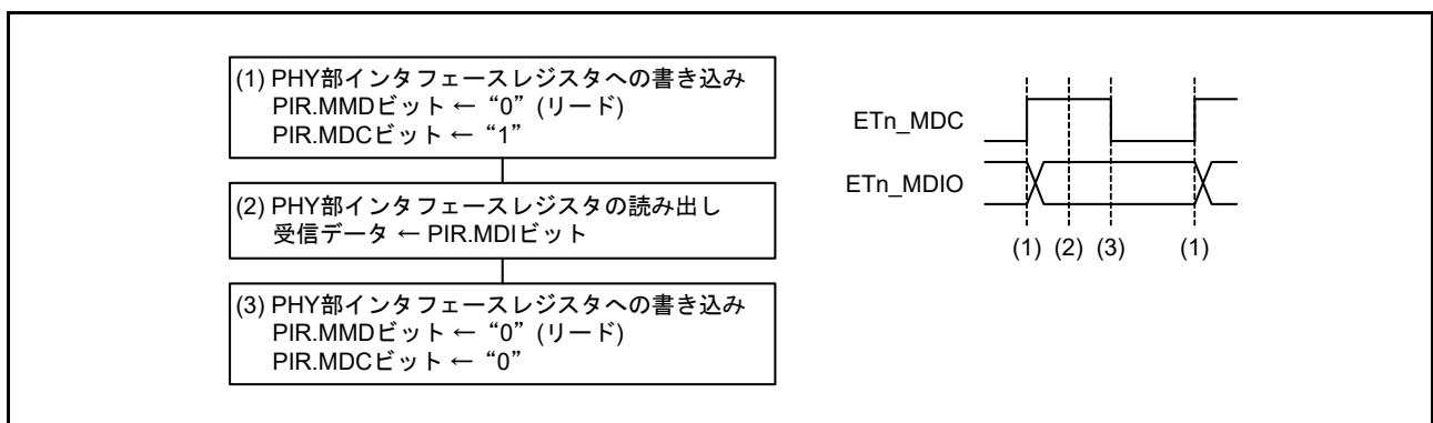
図 36.16 1ビットデータのリードフロー
