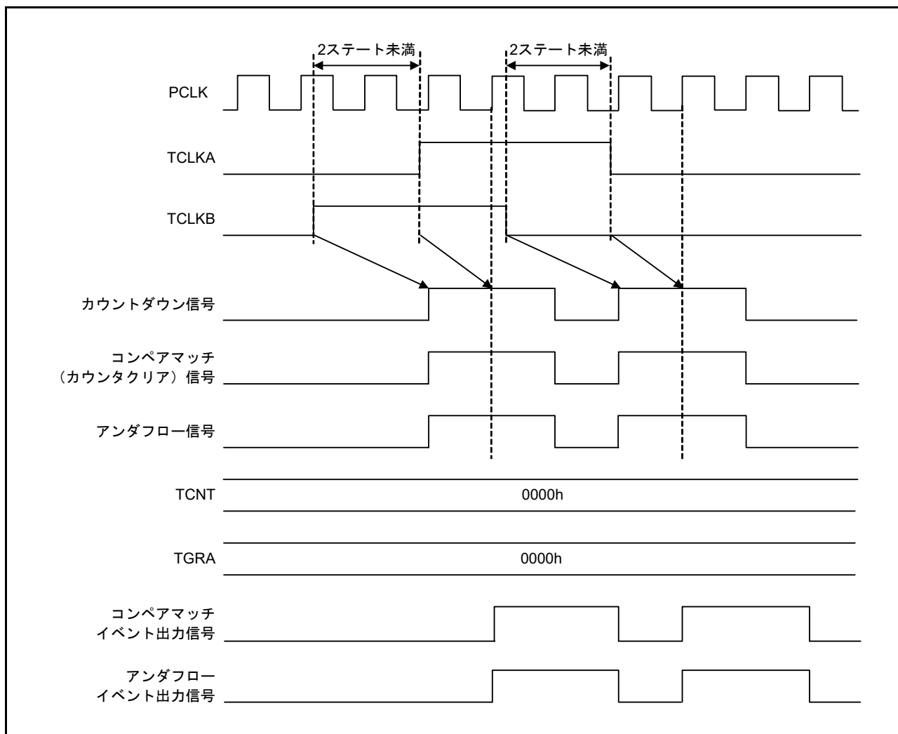
図 28.64 アンダフローイベント出力信号の連続出力
