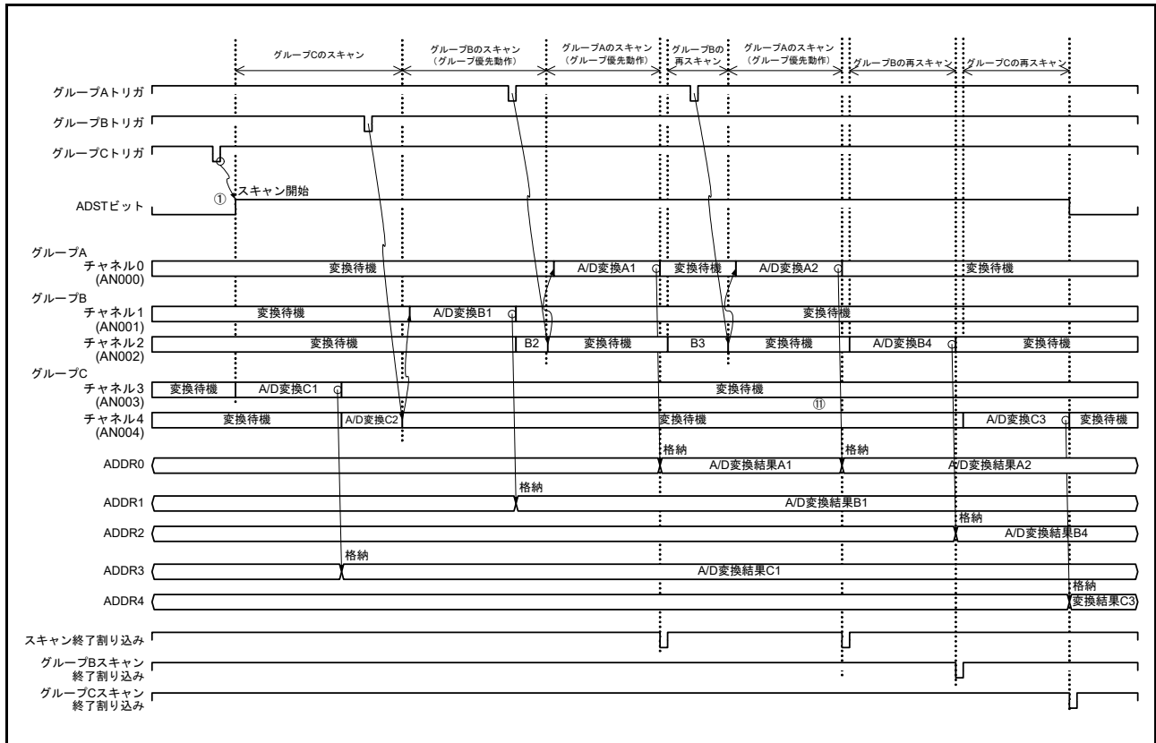
図 56.31 グループ優先動作の例 2 「低優先グループ再スキャン中の優先グループトリガ入力」再スキャンあり (ADGSPCR.GBRSCN = 1, ADGSPCR.GBRP = 0, ADGSPCR.LGRRS = 1 設定時)
