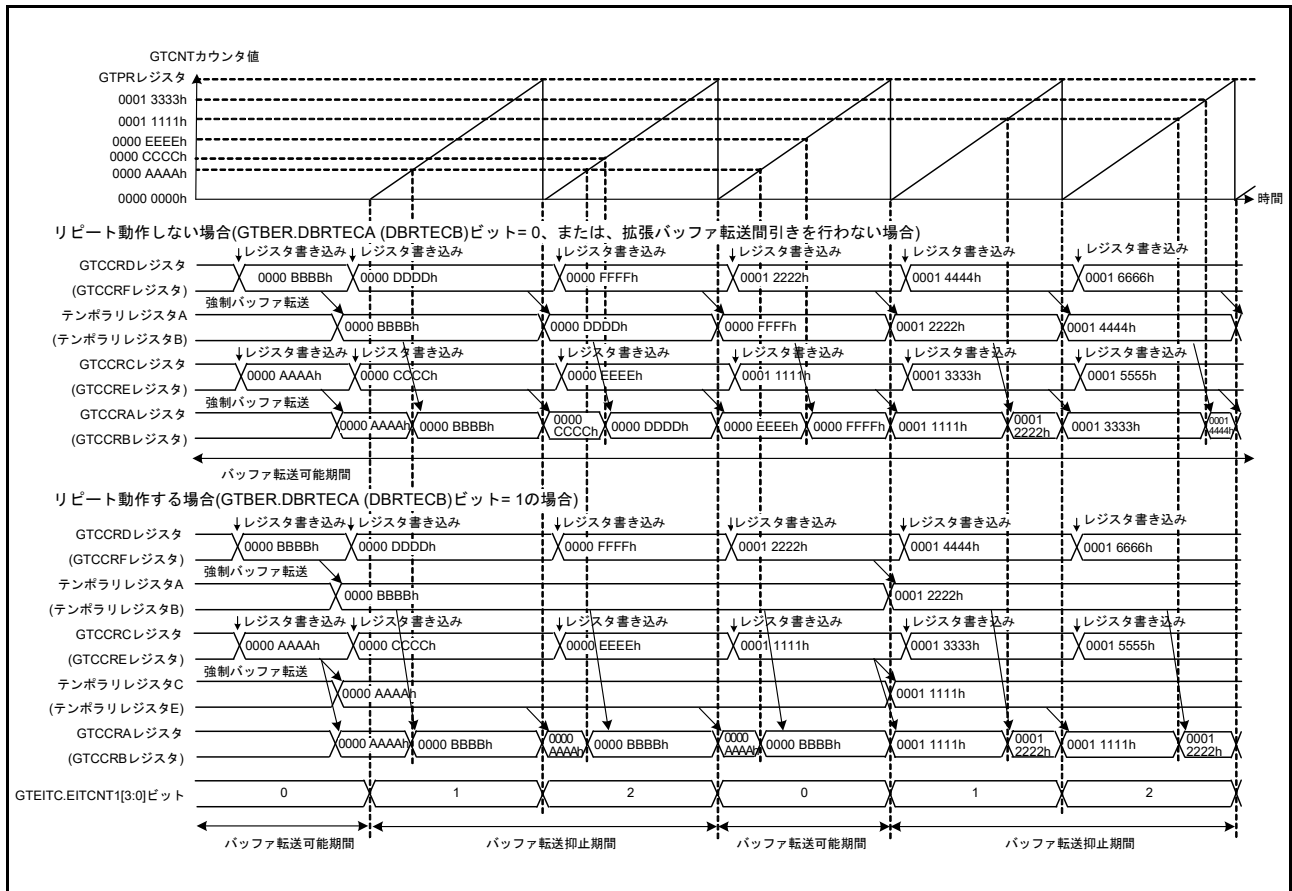
図 26.121 GTCCR バッファ転送抑制時ダブルバッファリポート動作例 (のこぎり波ワンショットパルスモード、拡張バッファ転送間引き使用、GTBER.BD[0] ビットは常時“0”の場合)
