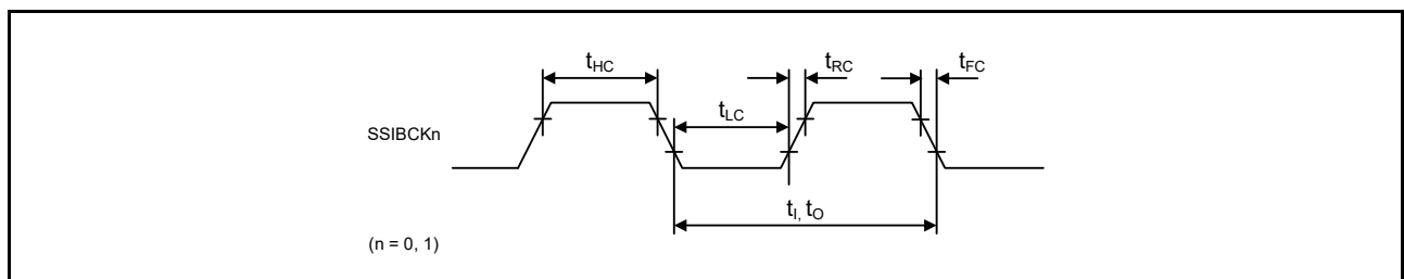
図63.74 SSIE クロック入出力タイミング
