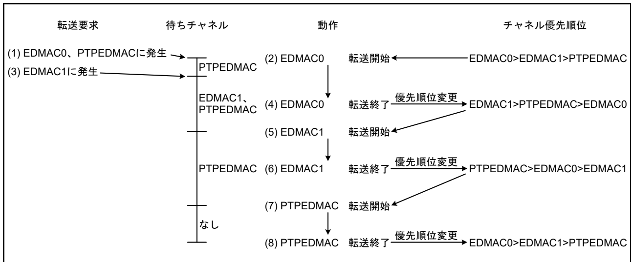
図 38.10 ラウンドロビン方式でのチャンネル優先順位
