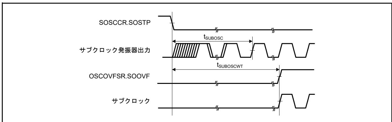
図 63.11 サブクロック発振開始タイミング
