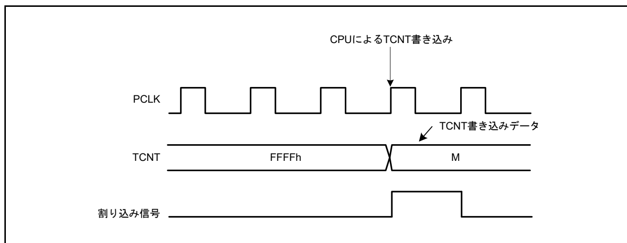
図 28.52 TPUm.TCNT への書き込みとオーバフローの競合
