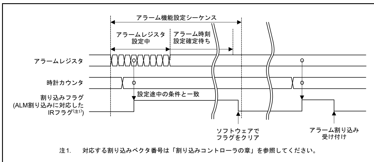
図 33.11 アラーム割り込み (ALM) のタイミングチャート
