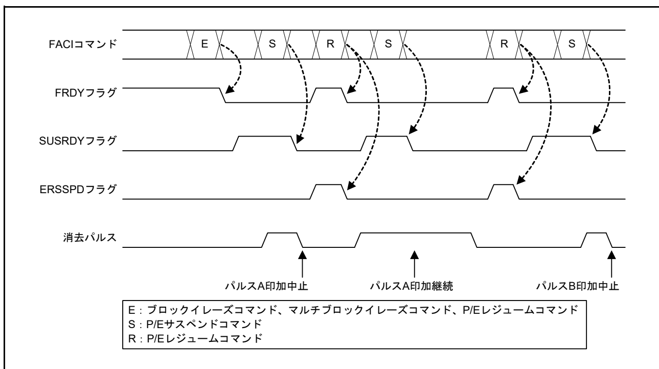
図 62.19 イレーズ処理の中断動作 (サスペンド優先モード)
