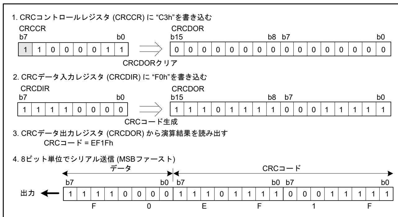
図 46.3 MSB ファーストでのデータ送信
