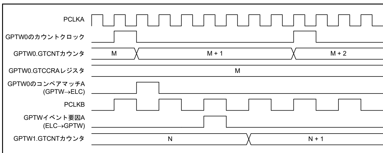
図 26.8 イベントカウンタ動作例 (ELCA イベント入力によるアップカウント)
