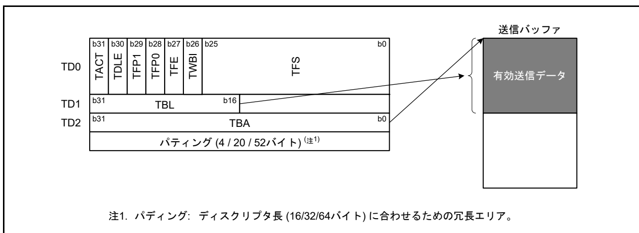
図 38.3 送信ディスクリプタと送信バッファの関係
