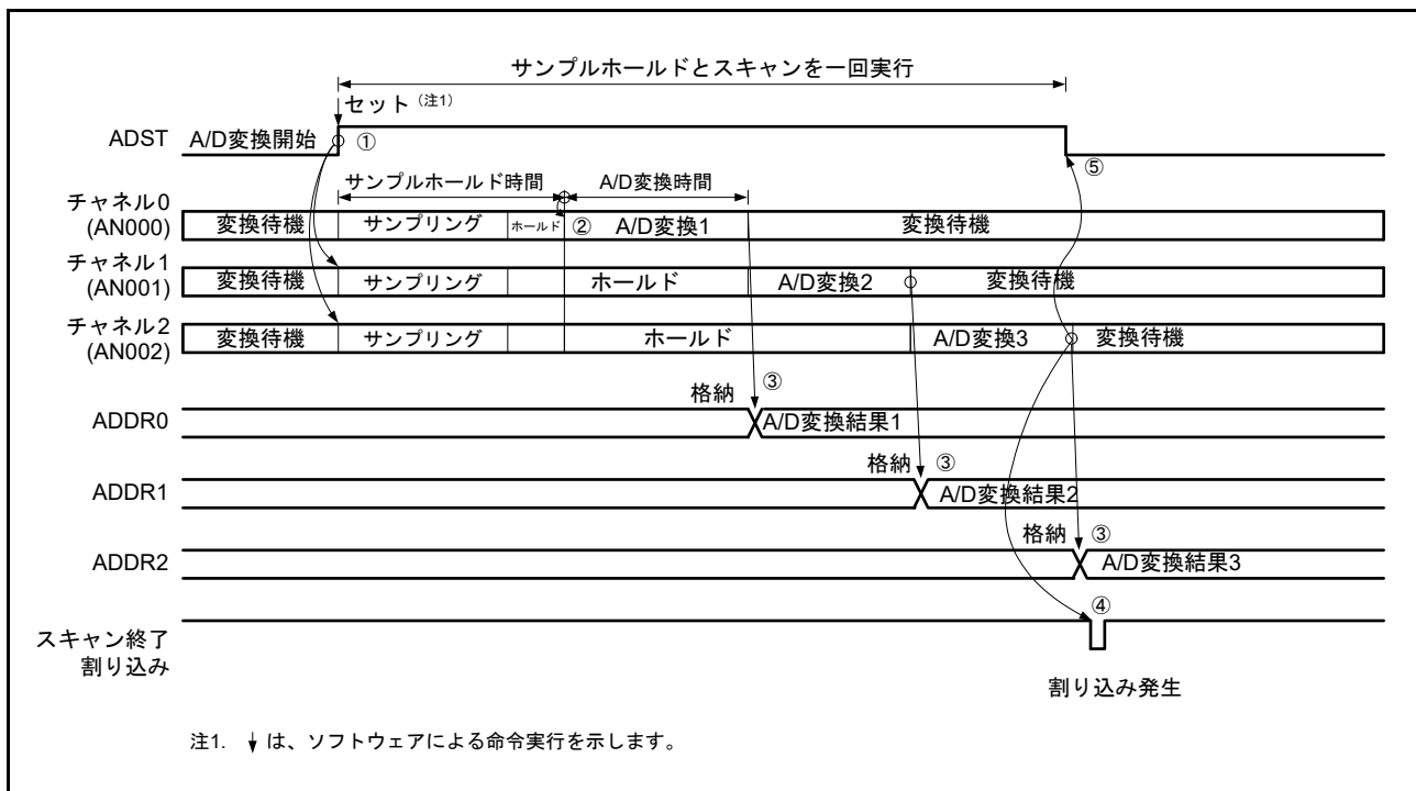
図 56.7 シングルスキャンモードの動作例 (チャンネル専用サンプル & ホールド回路使用チャンネル AN000, AN001, AN002 選択、常時サンプリング無効)
