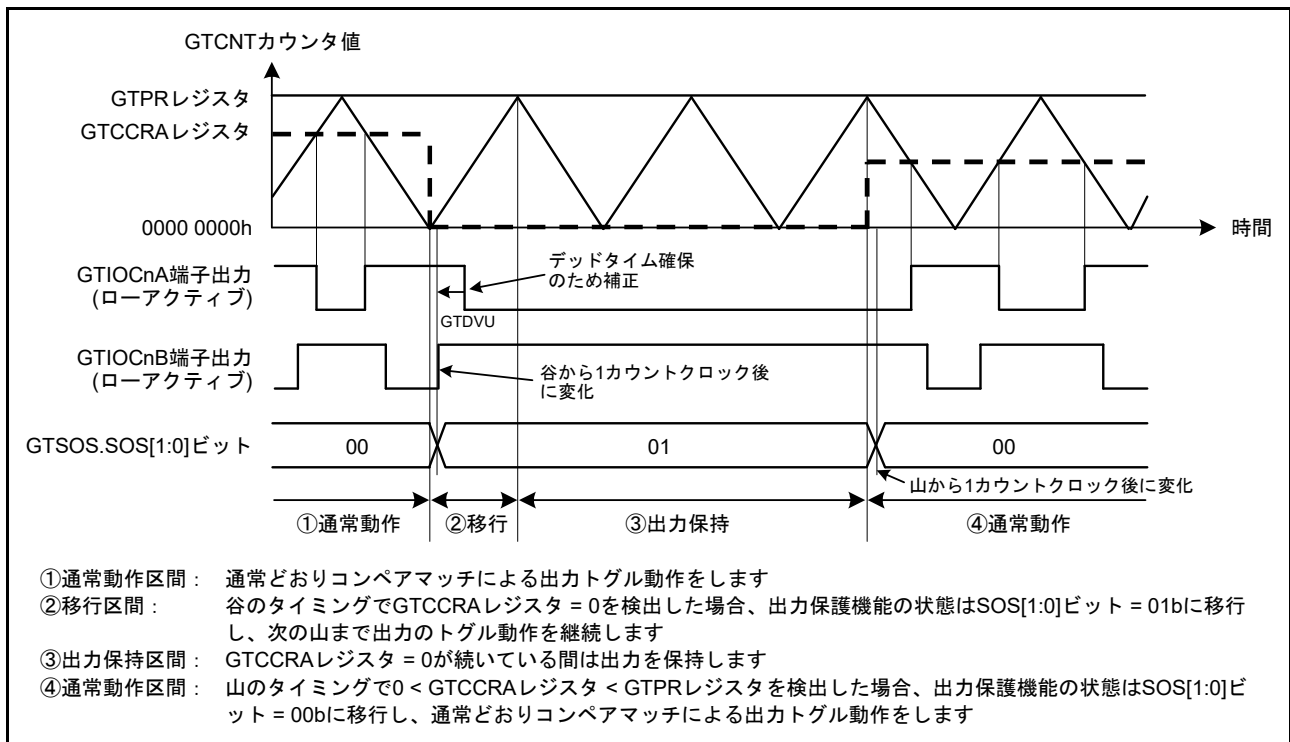
図 26.128 谷のバッファ転送で GTCCRA レジスタが “0000 0000h” である場合の出力保護機能の動作例 (山のバッファ転送で 0 < \text{GTCCRA レジスタ} < \text{GTPR レジスタ} に復帰、アクティブレベルは Low の場合) ( n = 0 \sim 3 )
