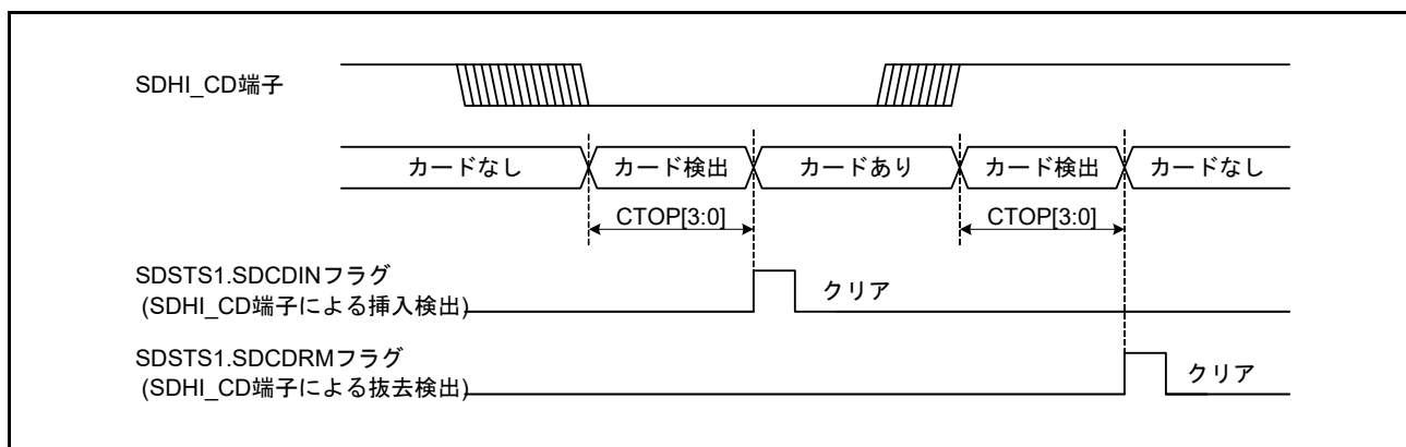
図48.6 SDHI_CD端子によるカード検出例
