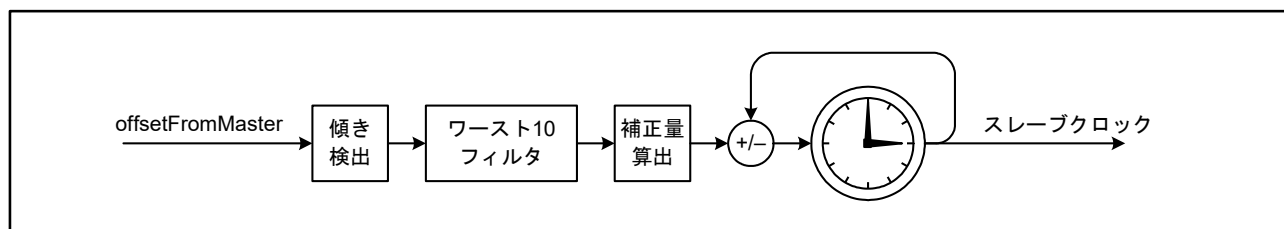
図 37.24 時刻補正回路の構成
