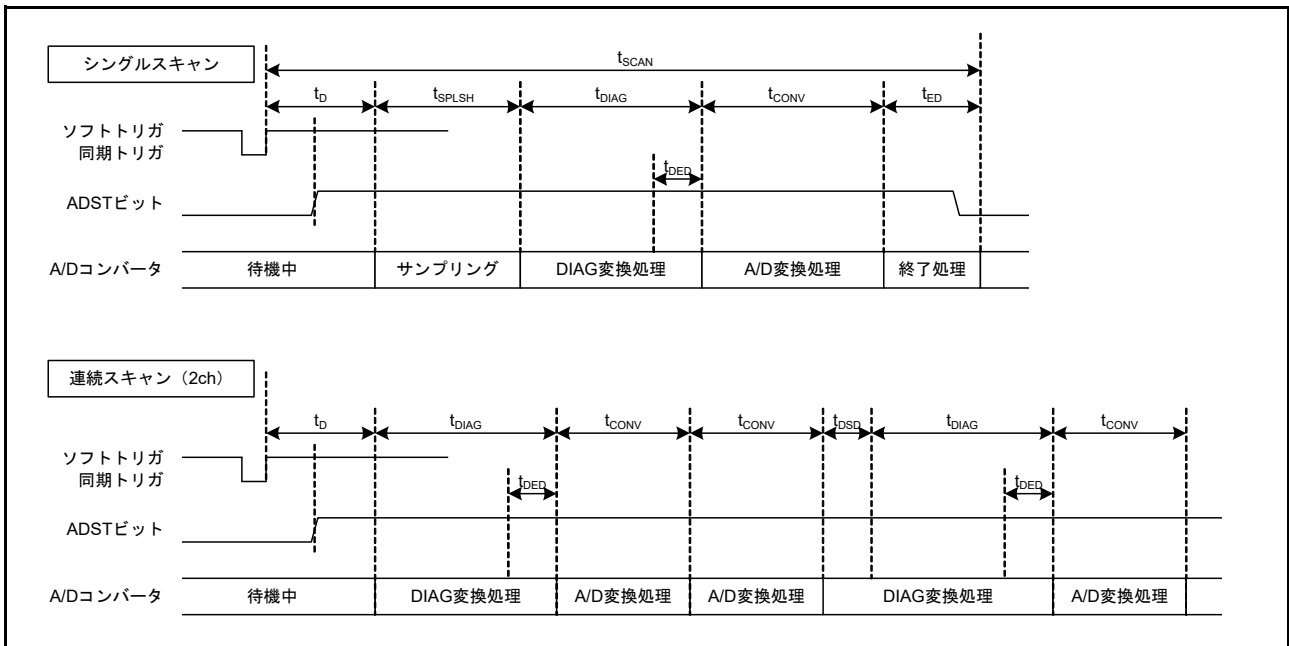
図 56.38 スキャン変換のタイミング (ソフトウェア起動、同期トリガ起動の場合)
