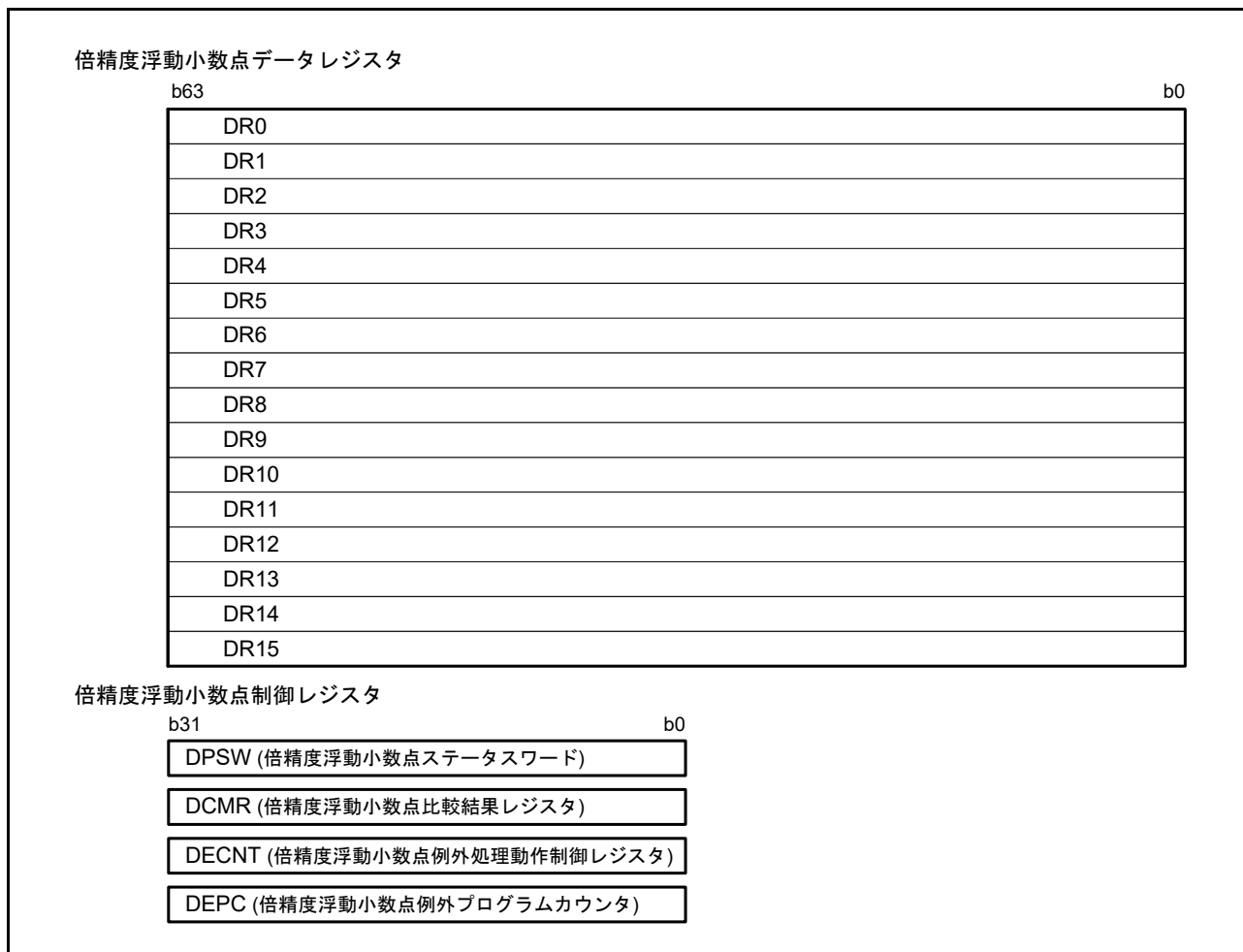
図 2.11 倍精度浮動小数点レジスタセット
