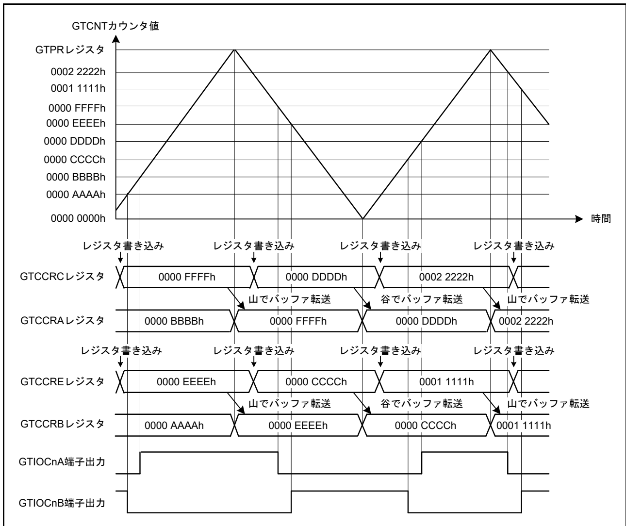
図 26.43 三角波 PWM モード 2 動作例 (バッファ動作、初期出力で GTIOCnA 端子 = Low 出力 / GTIOCnB 端子 = High 出力、GTCRA/GTCRB レジスタのコンペアマッチでトグル出力、周期の終わりで出力保持の場合) (n = 0 ~ 3)
