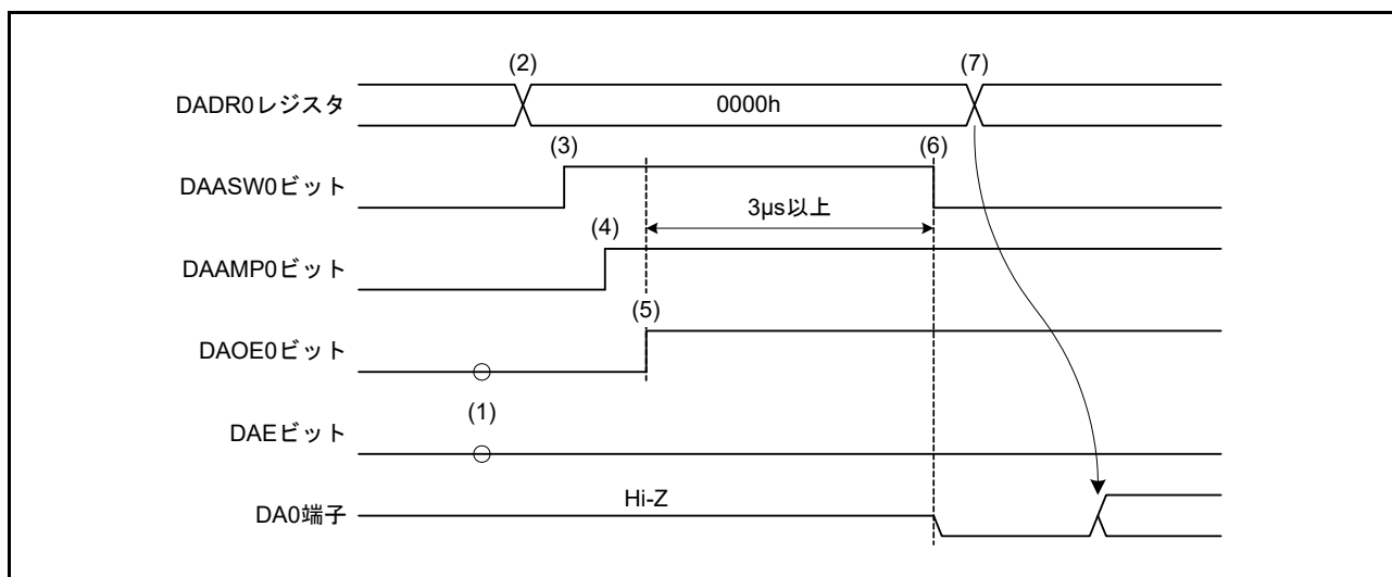
図 57.4 出力バッファアンプの初期設定手順
