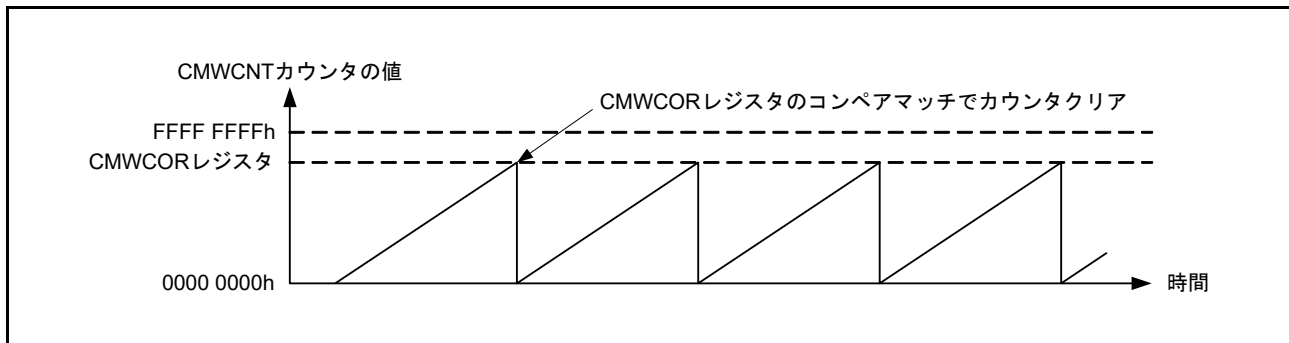
図 32.4 コンペアマッチ動作例
