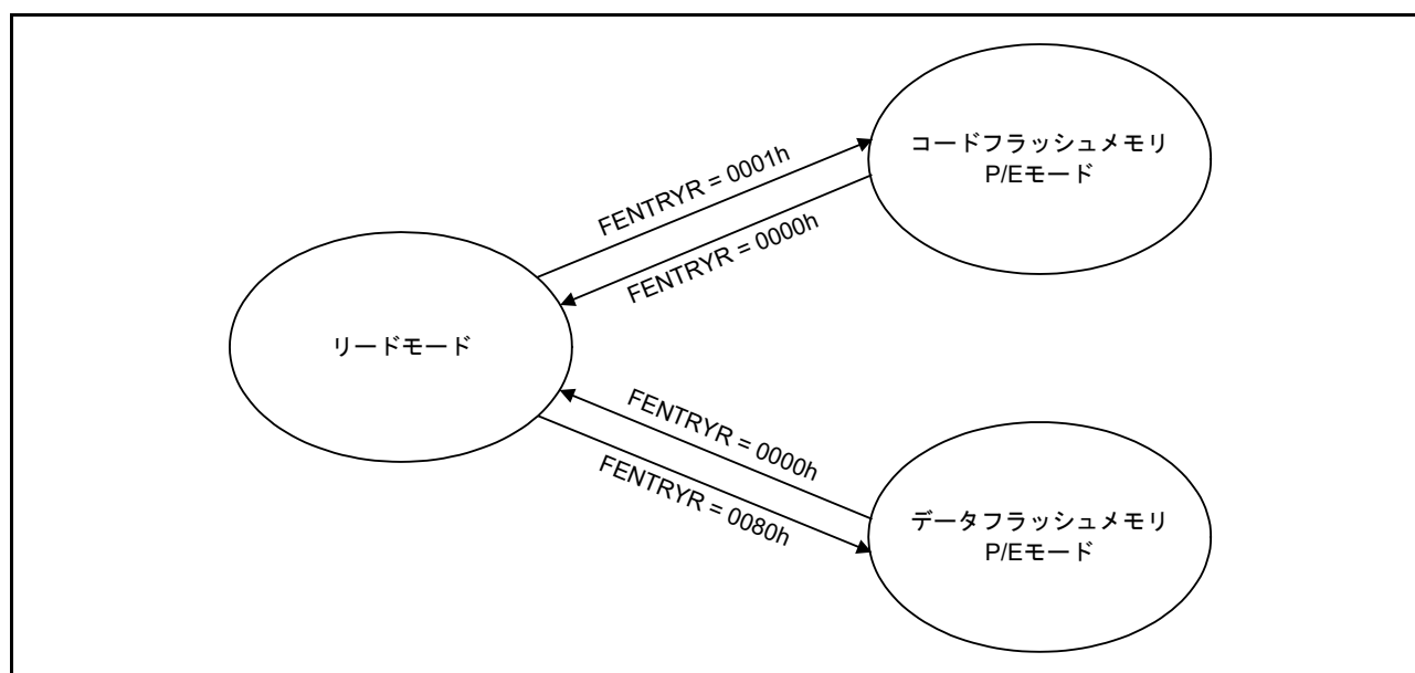
図 62.7 フラッシュシーケンサのモード
