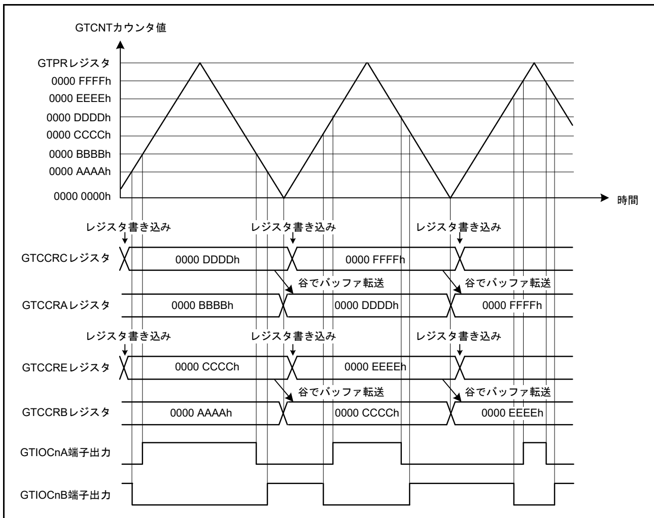
図 26.41 三角波 PWM モード 1 動作例 (バッファ動作、初期出力で GTIOCnA 端子 = Low 出力 / GTIOCnB 端子 = High 出力、GTCCRA/GTCCRB レジスタのコンペアマッチでトグル出力、周期の終わりで出力保持の場合) (n=0~3)
