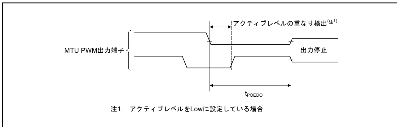
図 63.44 POE 出力ディセーブル時間 (出力端子の短絡)
