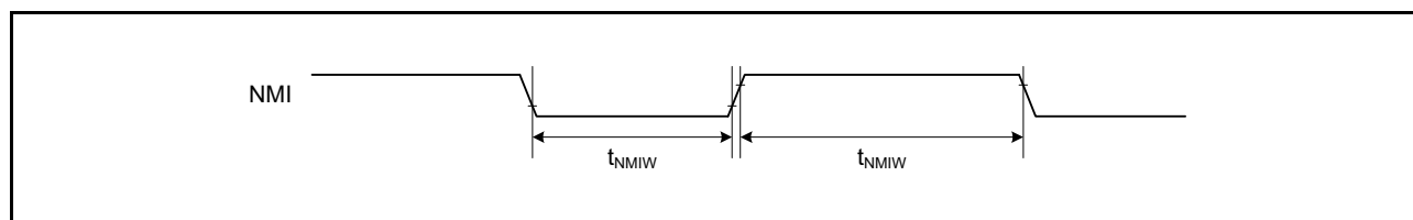
図 63.16 NMI 割り込み入カタイミング
