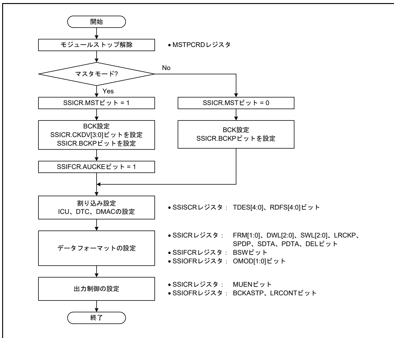
図 47.22 初期設定フロー例
