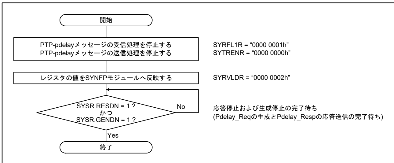
図37.17 P2P動作の停止手順
