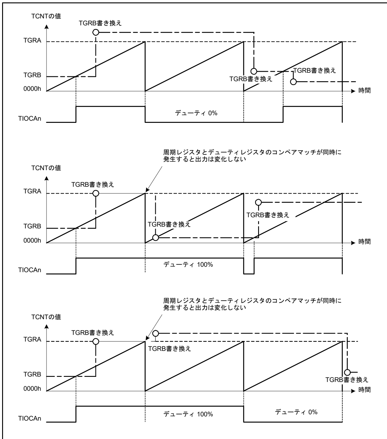
図 28.23 PWM モード動作例 (3) (n = 0 ~ 5)
