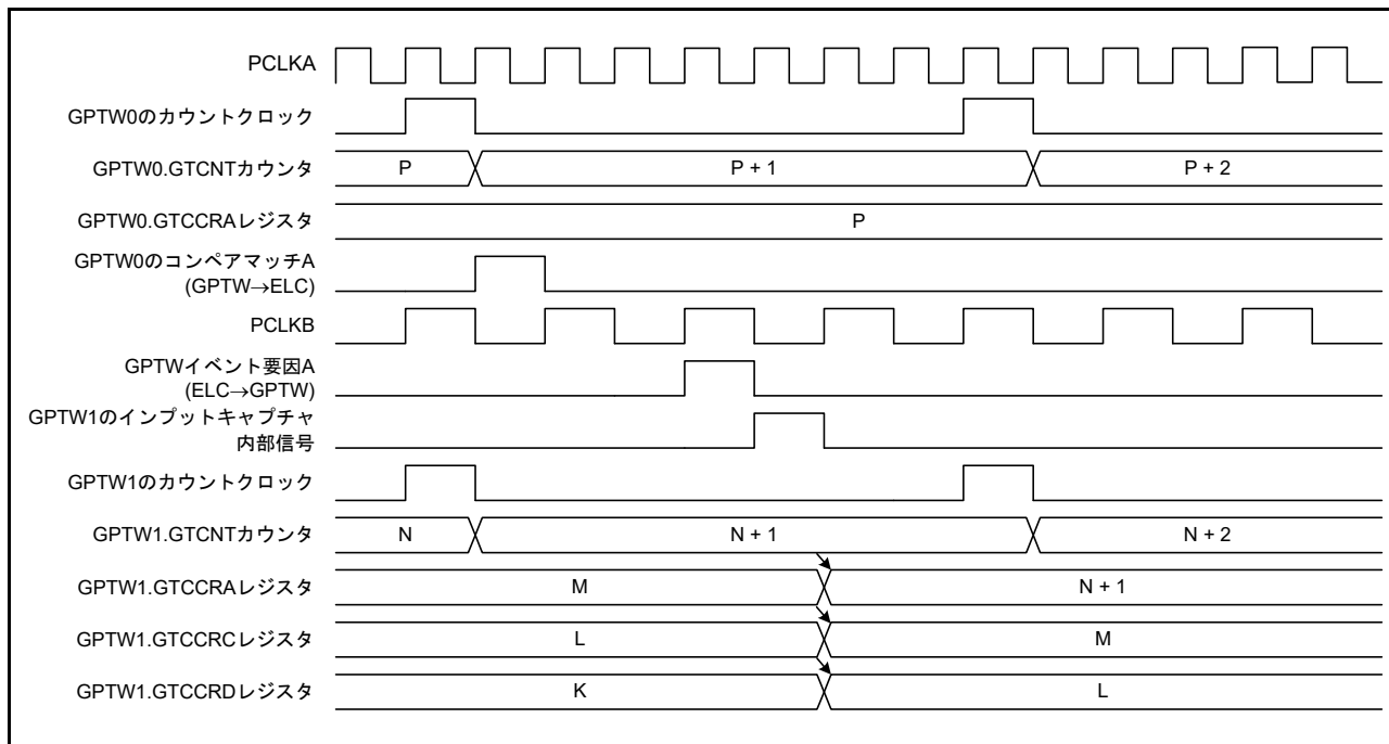
図 26.21 ELCA イベント入力によるインプットキャプチャ動作タイミング例
