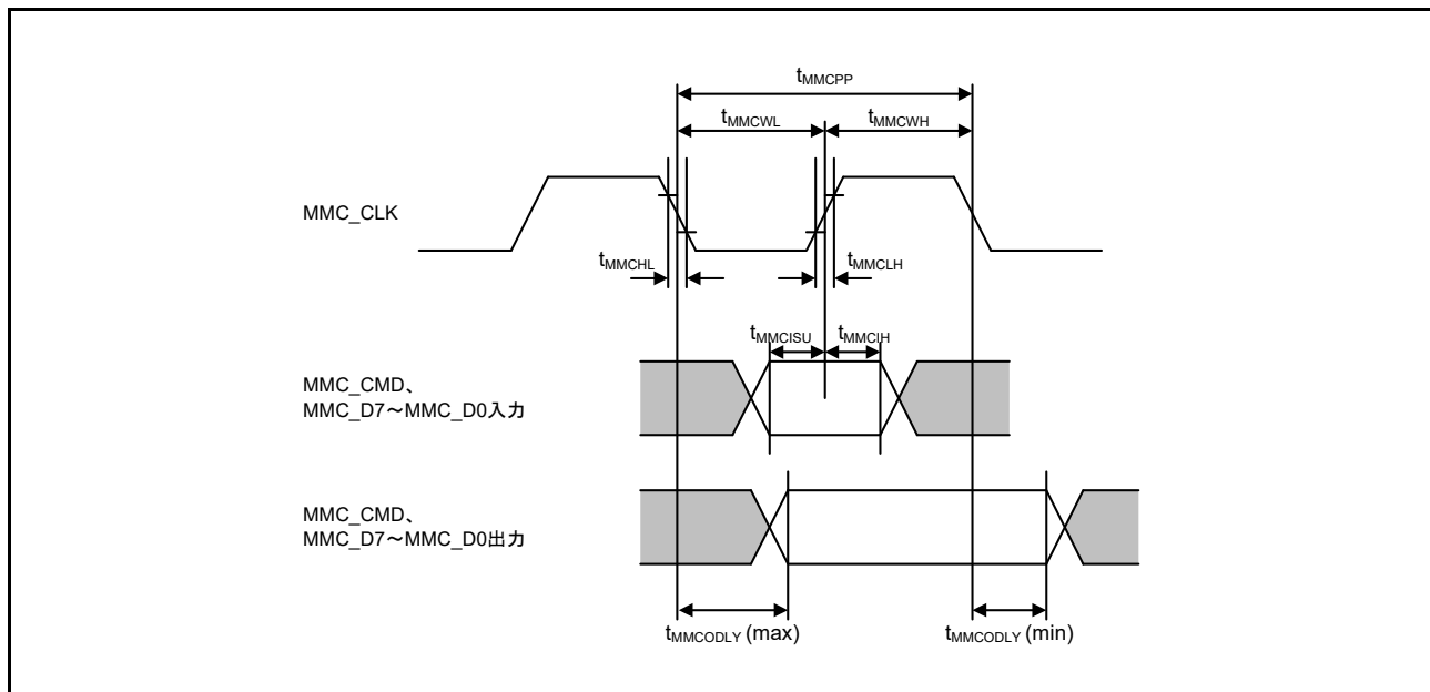
図 63.79 MMC インタフェース
