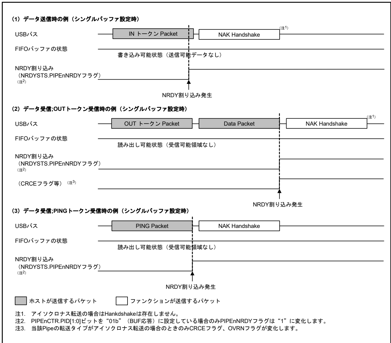
図 40.12 NRDY 割り込み発生タイミング図 (ファンクションコントローラ機能選択時)
