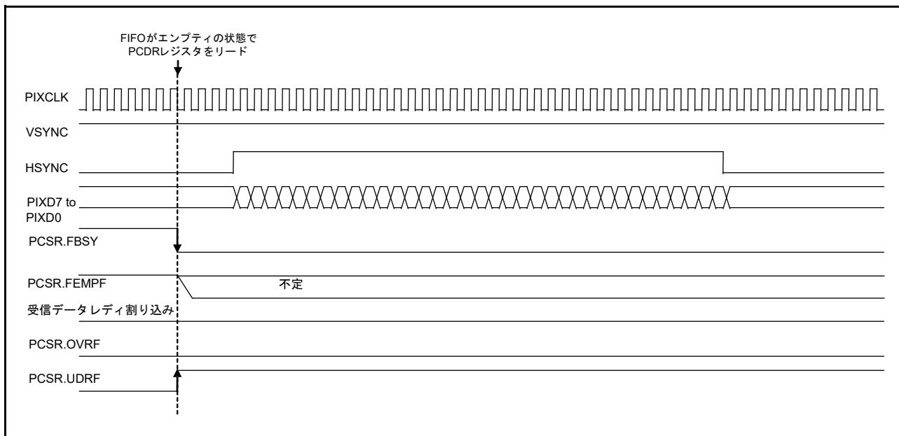
図 50.15 アンダラン検出
