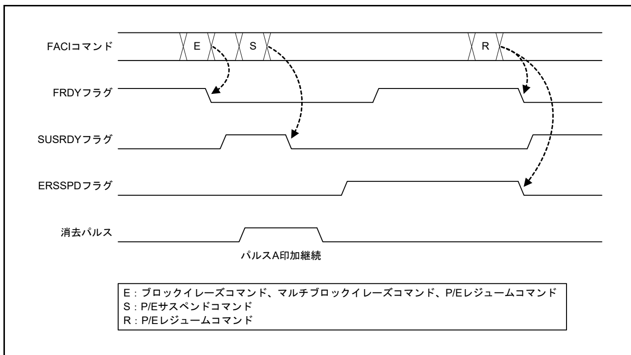
図 62.20 イレーズ処理の中断動作 (イレーズ優先モード)
