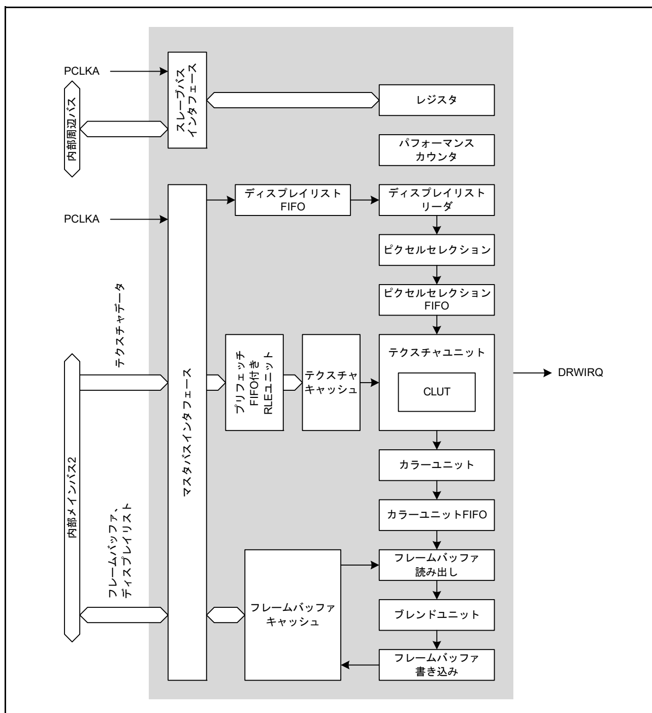
図 52.2 DRW2D のブロック図
