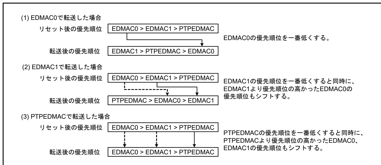
図 38.9 ラウンドロビン方式の動作
