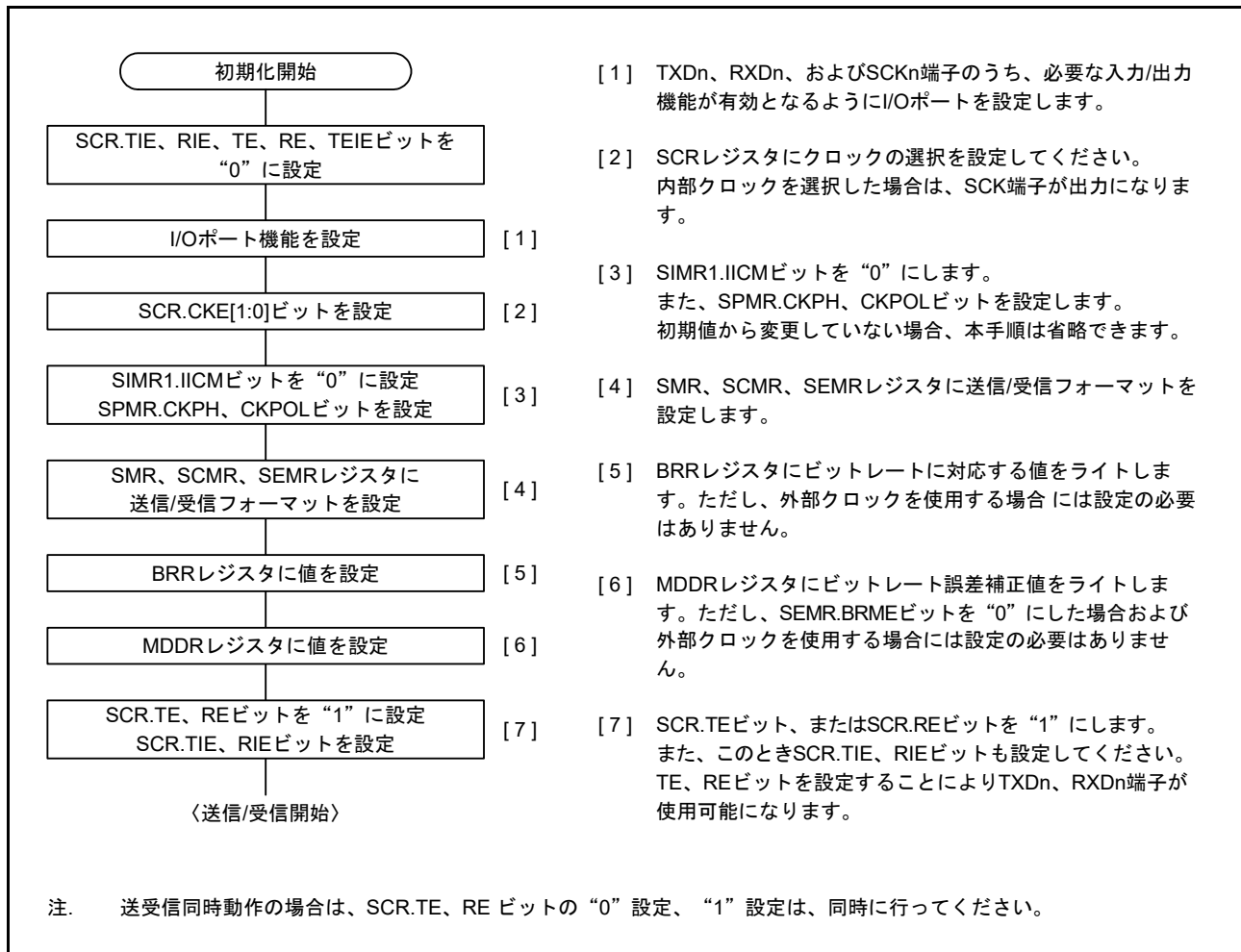
図 41.28 SCIの初期化フローチャートの例(クロック同期式モード)
