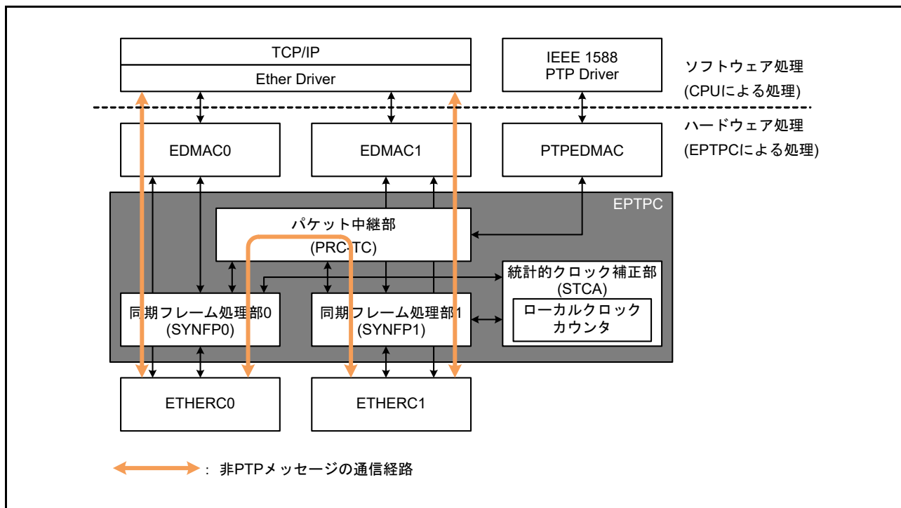
図37.5 非PTPメッセージの送受信と中継の経路
