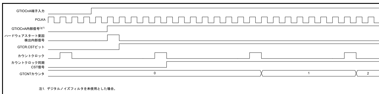
図 26.58 GTIOCnA 端子入力の立ち上がりによるカウントスタート動作タイミング例
