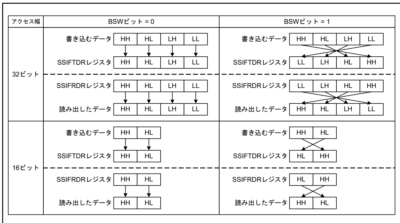
図 47.6 バイトスワップの動作例
