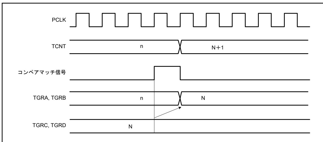
図 28.37 バッファ動作タイミング (コンペアマッチ)
