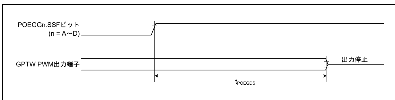
図 63.50 POEG 出力ディセーブル時間 (レジスタ設定)
