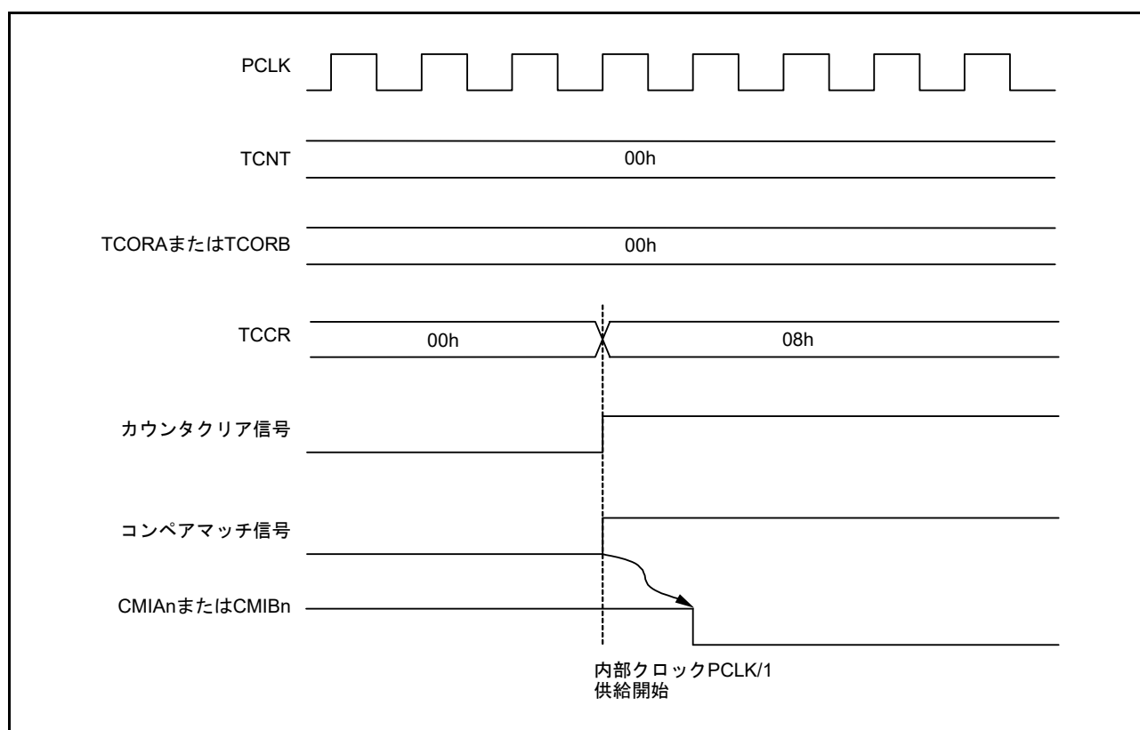
図 30.16 コンペアマッチ割り込みの連続出力 (n = 0 ~ 3)
