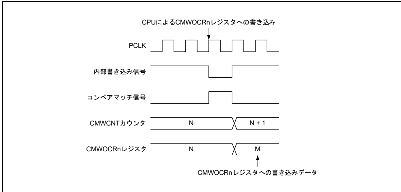
図 32.26 CMWOCRn レジスタへの書き込みとコンペアマッチの競合
