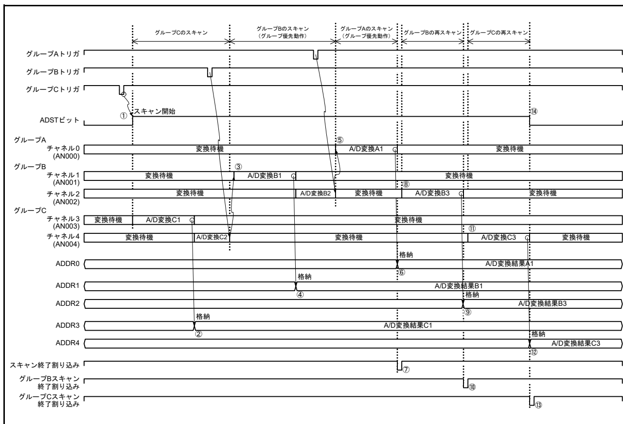
図 56.30 グループ優先動作の例 1 「低優先グループスキャン中の優先グループトリガ入力」再スキャンあり (ADGSPCR.GBRSCN = 1, ADGSPCR.GBRP = 0, ADGSPCR.LGRRS = 1 設定時)
