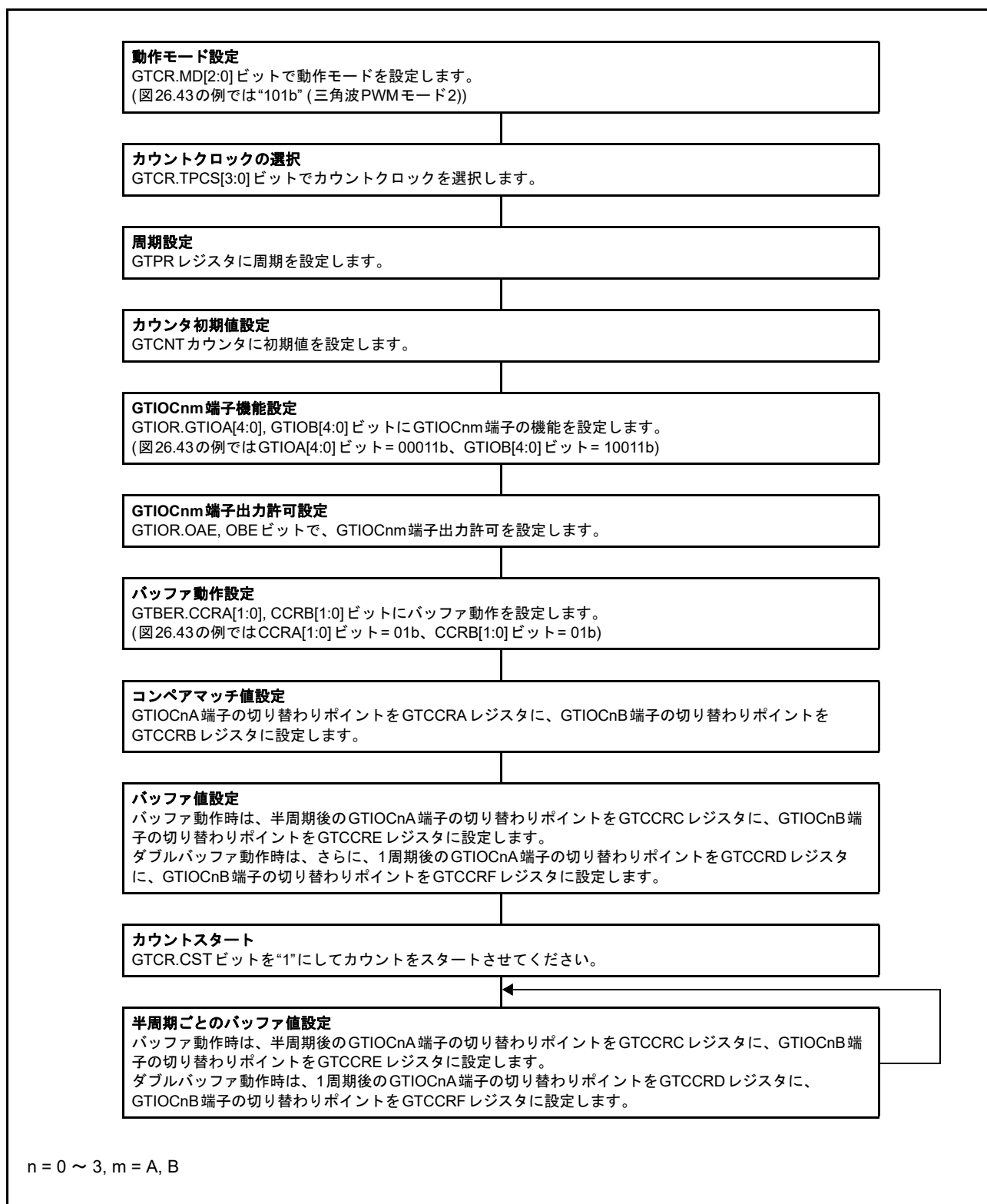
図 26.44 三角波 PWM モード 2 設定例
