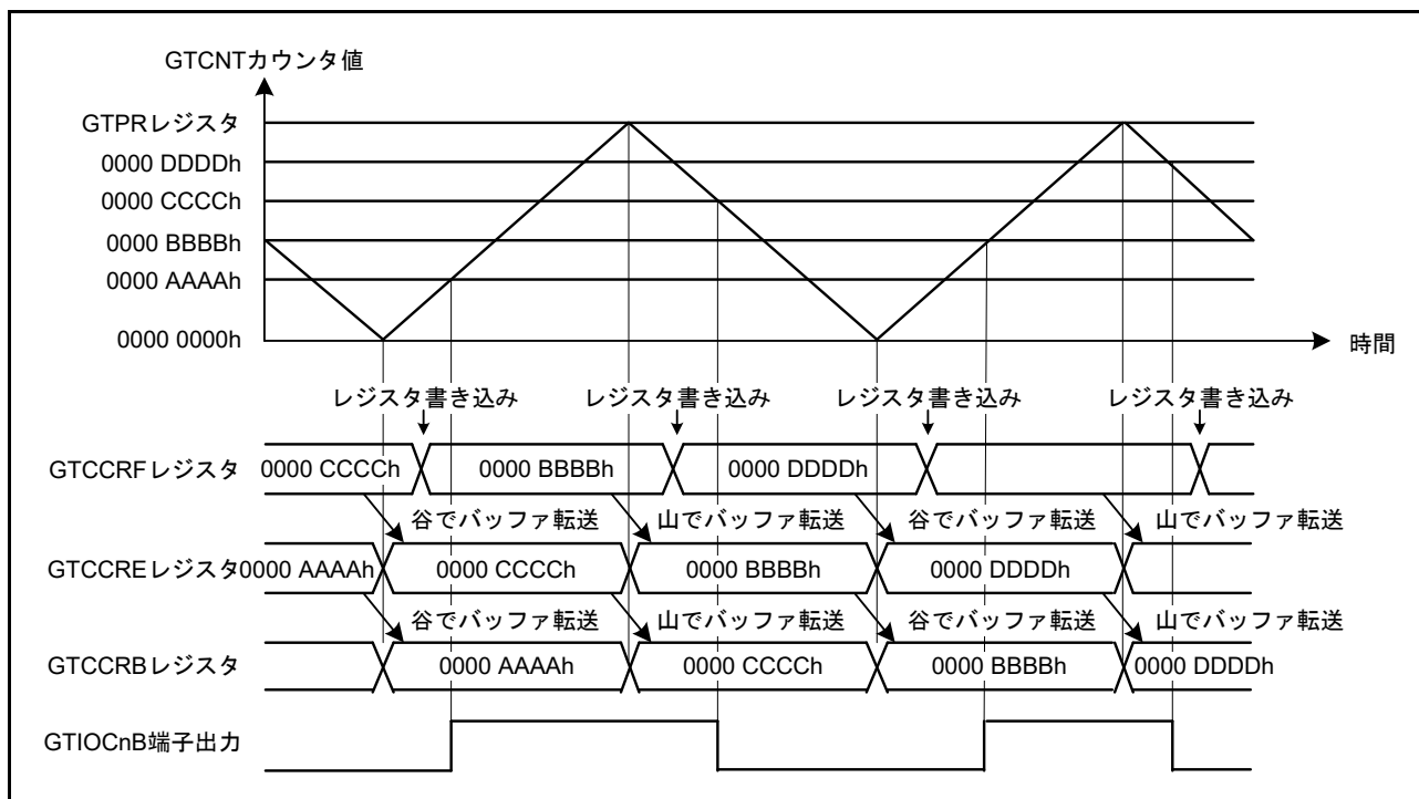
図 26.28 GTCCRA, GTCCRB レジスタのダブルバッファ動作例 (アウプットコンペア、三角波、谷 / 山両方でバッファ転送、GTCCRB レジスタコンペアマッチでトグル出力、周期の終わりで出力保持の場合) (n = 0 ~ 3)
