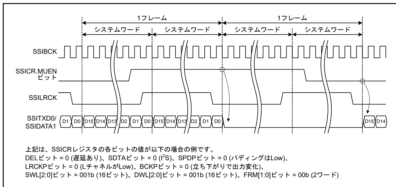
図 47.17 ミュート機能の動作例
