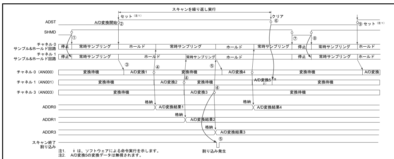
図 56.17 連続スキャンモードの動作例 (チャンネル専用サンプル & ホールド回路使用 : AN000, AN001, AN003 選択、常時サンプリング有効)
