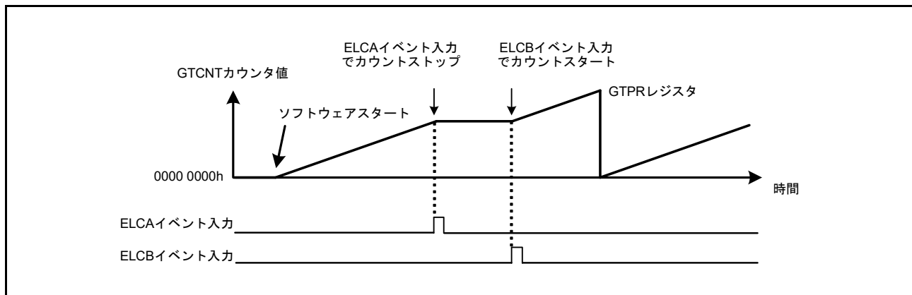
図 26.60 ハードウェア要因によるカウントストップ動作例 (ソフトウェアでスタート、ELCA イベント入力でストップ、ELCB イベント入力 で再スタート時)
