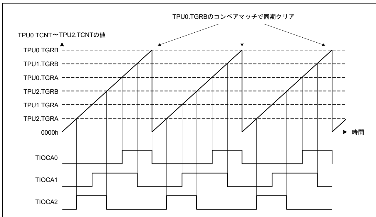
図 28.11 同期動作の動作例
