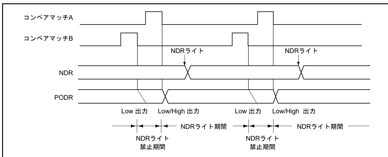
図 29.10 ノンオーバーラップ動作と PPGn.NDRH, PPGn.NDRL, PPGn.NDRH2, PPGn.NDRL2 レジスタ書き込みタイミング
