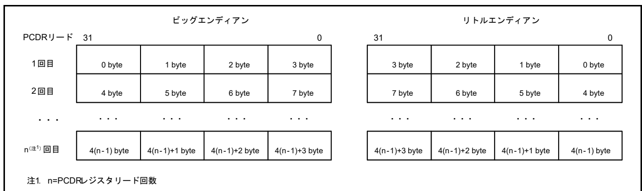
図 50.3 エンディアンフォーマット
