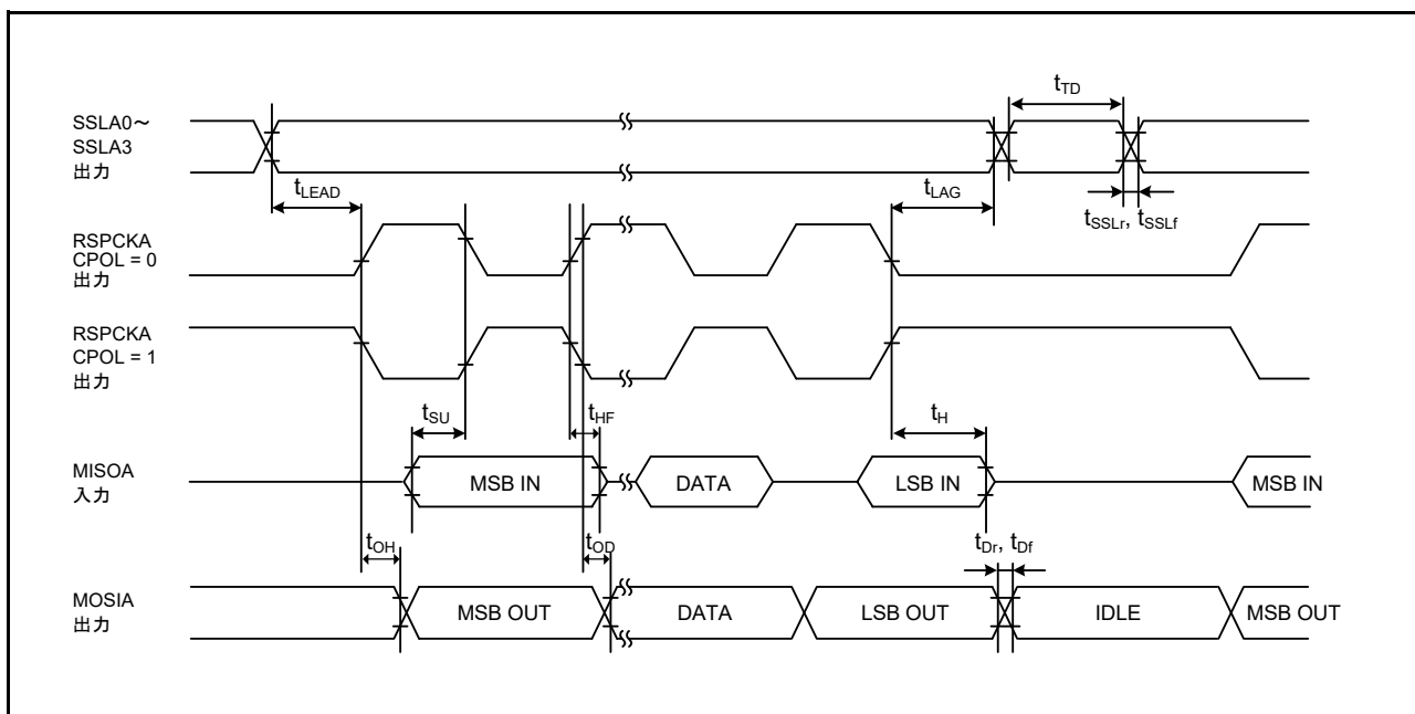
図 63.67 RSPI タイミング ( マスタ、CPHA = 1) ( ビットレート : PCLKA を 2 分周に設定 )
