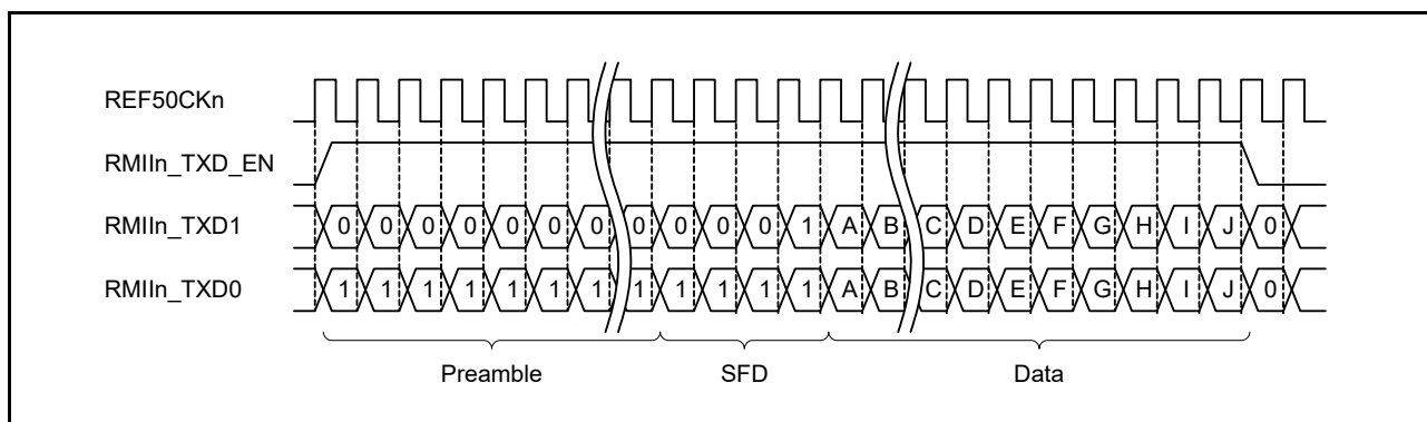
図 36.11 RMII フレーム送信タイミング (正常送信)
