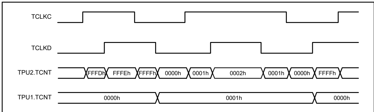
図 28.19 カスケード接続動作例 (2)
