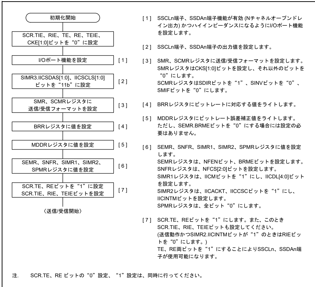
図 41.55 SCIの初期化フローチャート例 (簡易 I 2 C モード)
