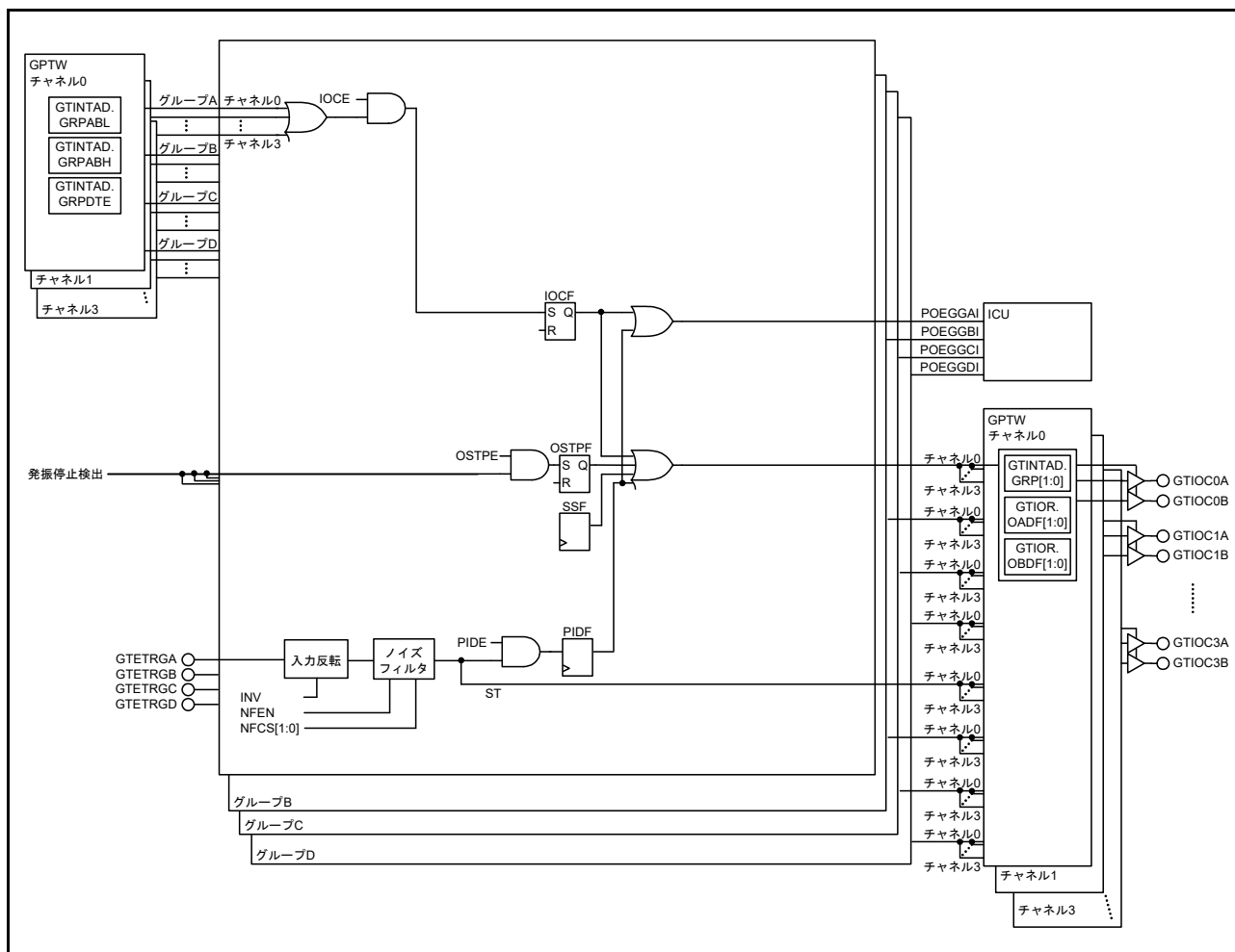
図 27.2 POEG のブロック図
