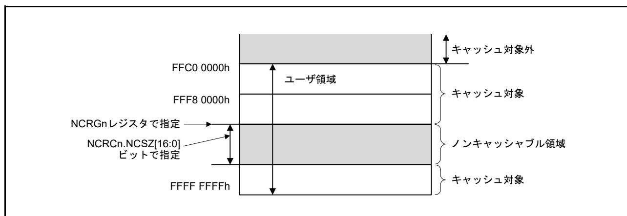
図 62.8 ノンキャッシュャブル領域指定 (n = 0, 1)
