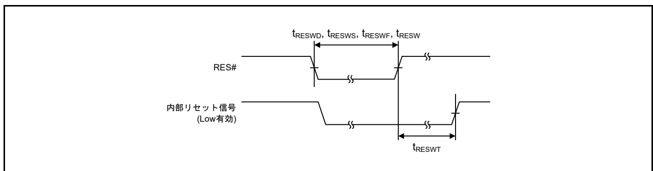
図 63.2 リセット入力タイミング
