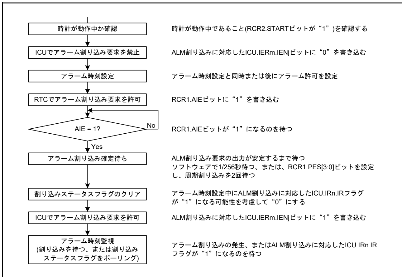
図 33.7 アラーム機能の使用方法
