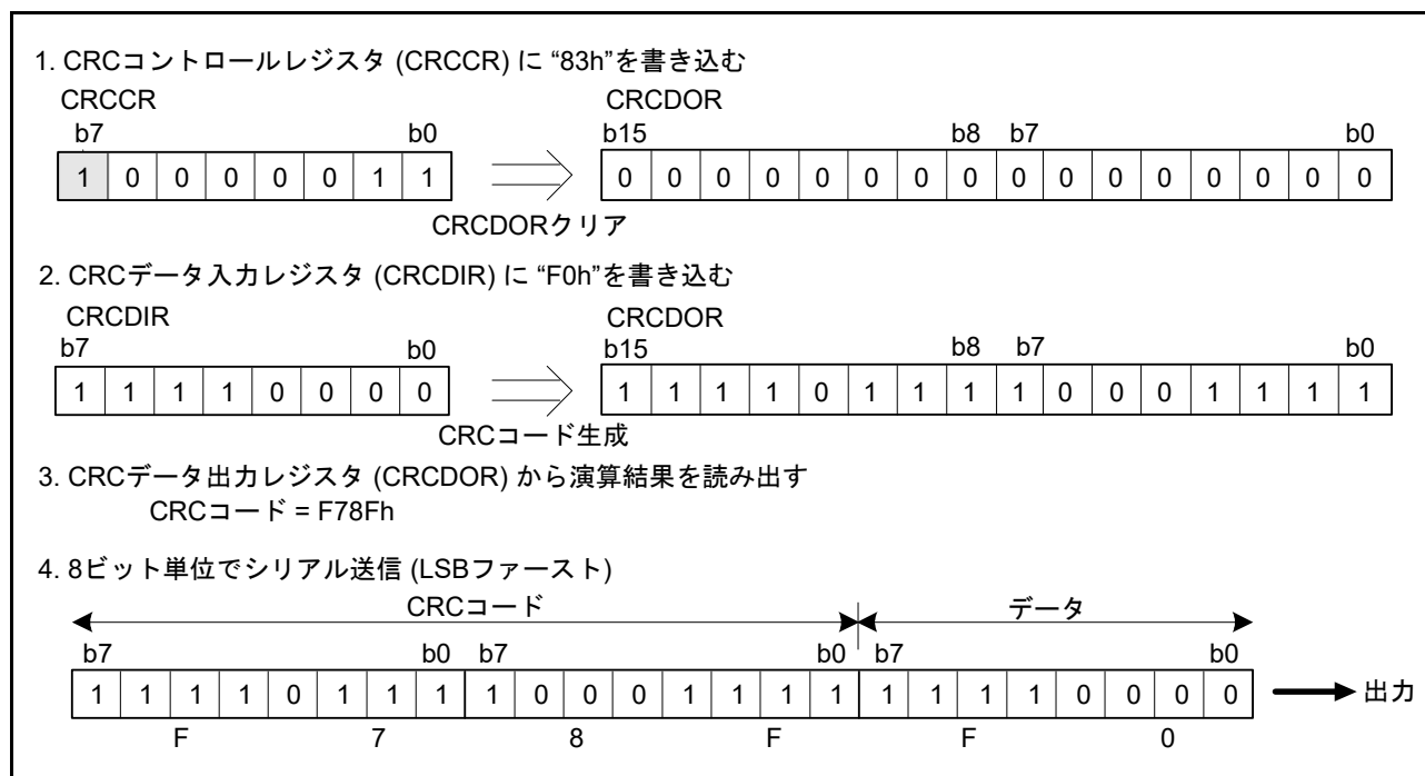
図 46.2 LSB ファーストでのデータ送信
