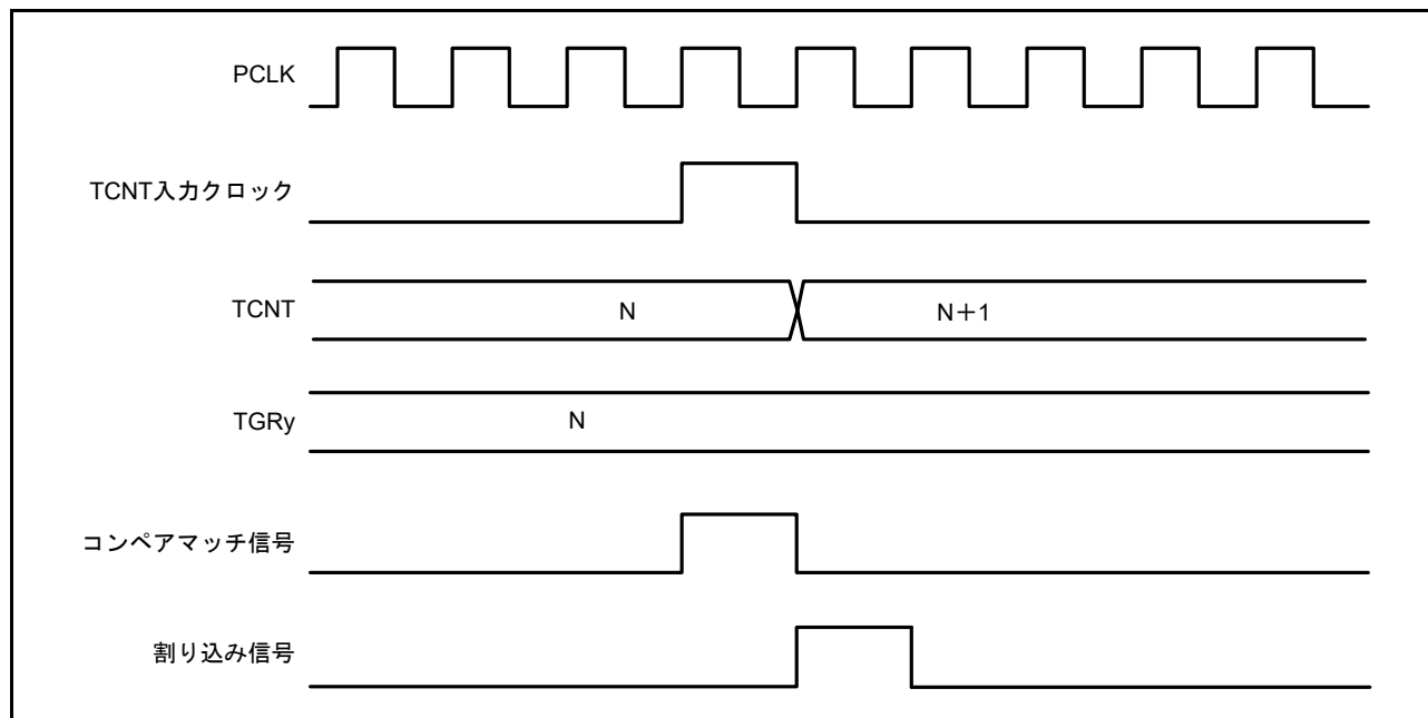
図 28.39 TGI my 割り込みタイミング (コンペアマッチ)
