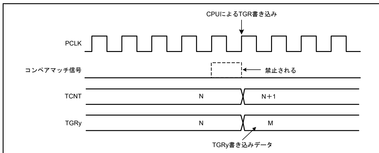
図 28.46 TPUm.TGRy レジスタへの書き込みとコンペアマッチの競合
