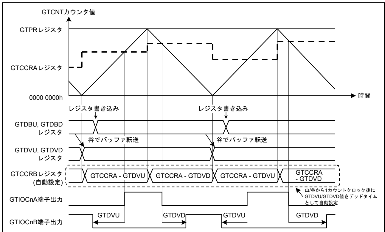
図 26.50 デッドタイム付きコンペアマッチ値の自動設定機能の動作例 ( 三角波 PWM モード 2/3、GTDVU/GTDDVD レジスタはバッファ動作、アクティブレベルは High の場合 ) (n = 0 ~ 3)
