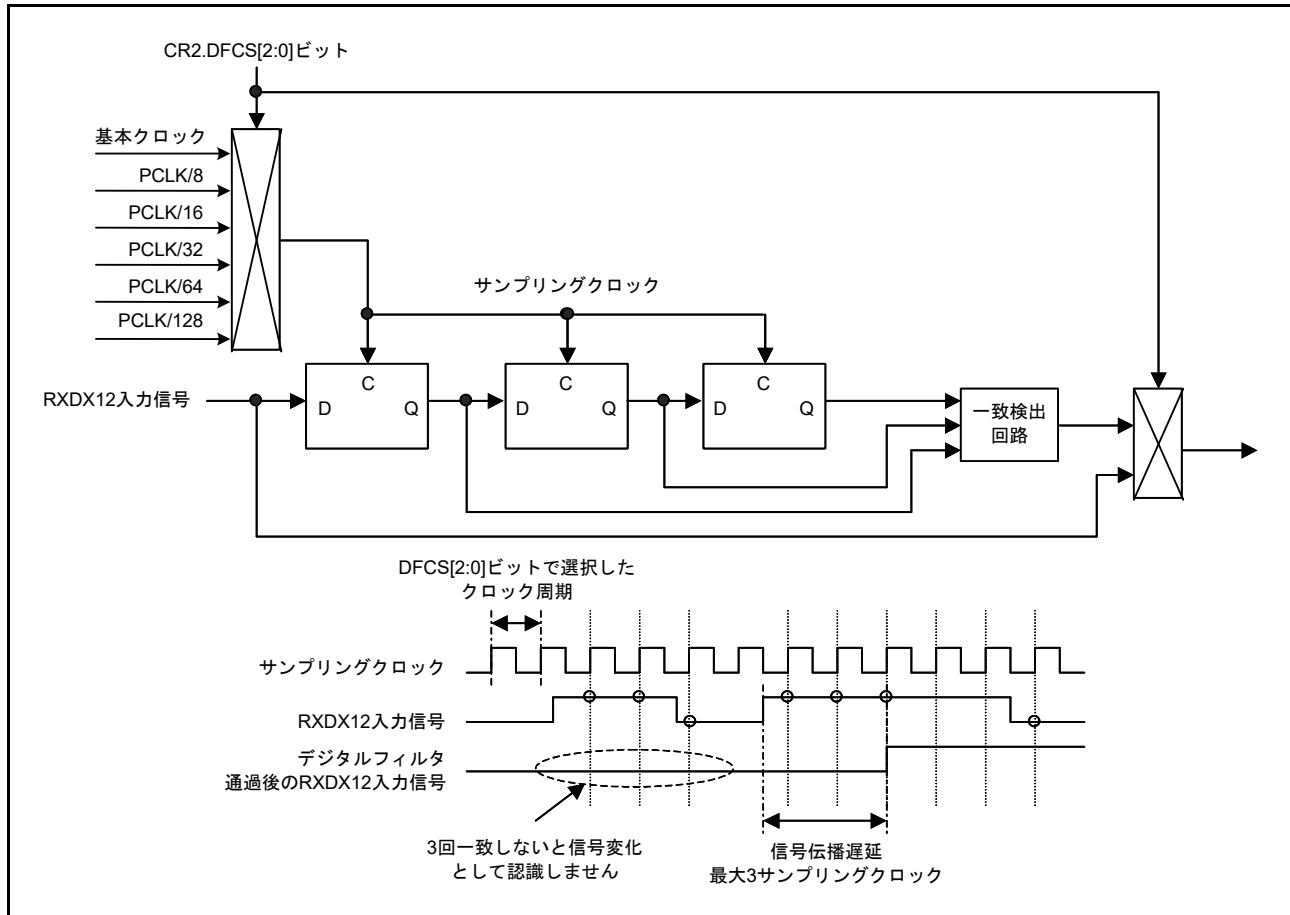
図 41.74 デジタルフィルタ機能の動作例
