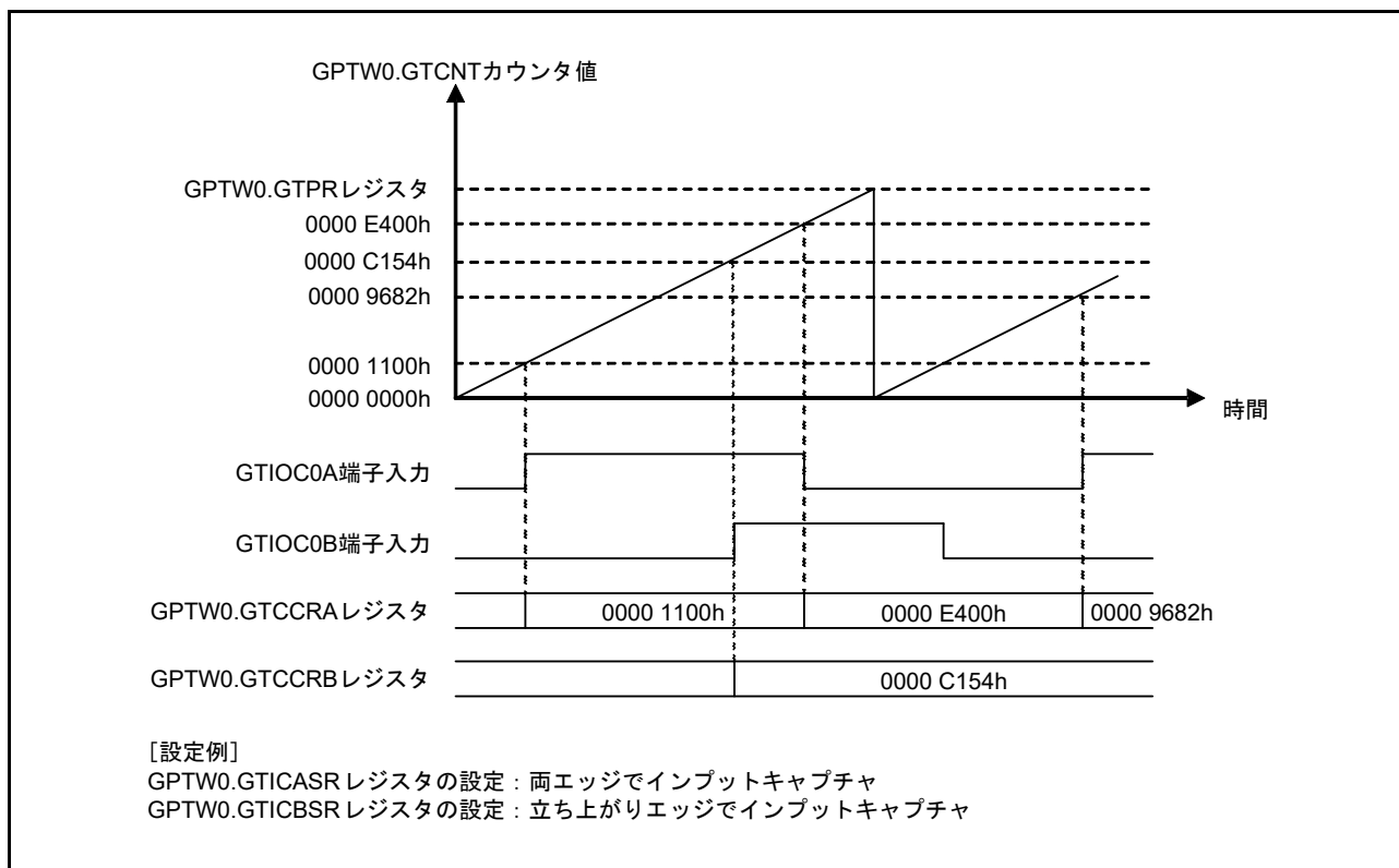
図 26.17 インพุットキャプチャ動作例
