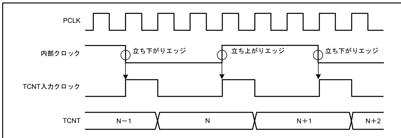
図 28.31 内部クロック動作時のカウントタイミング
