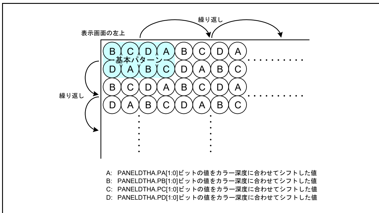
図 51.13 2×2 パターンディザの加算値選択方法
