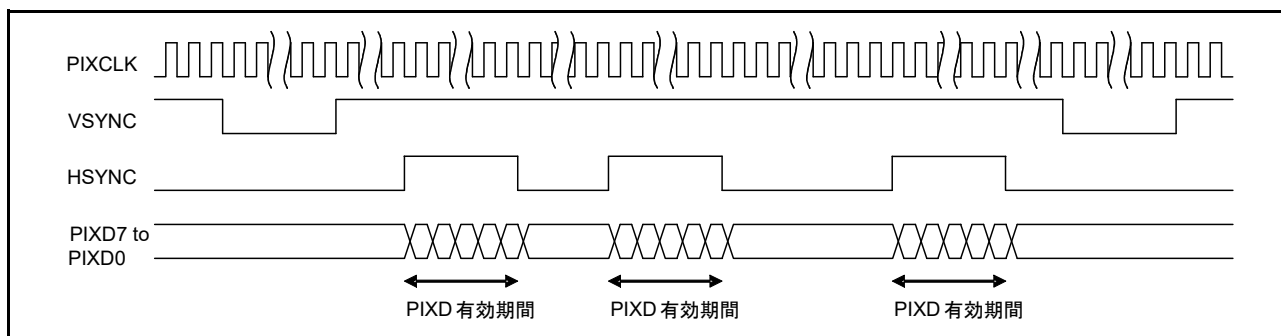
図 50.4 PDC 通信フォーマット (VPS = 0, HPS = 0)
