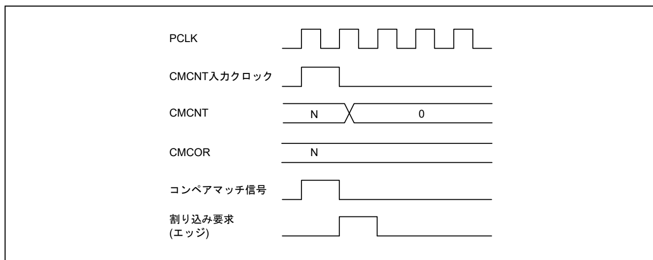
図 31.4 コンペアマッチ割り込みタイミング
