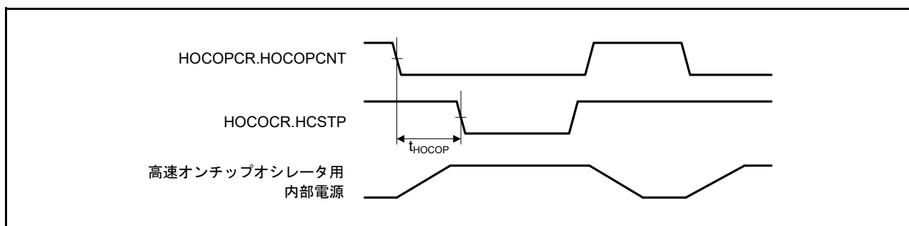
図 63.9 高速オンチップオシレータ電源制御タイミング
