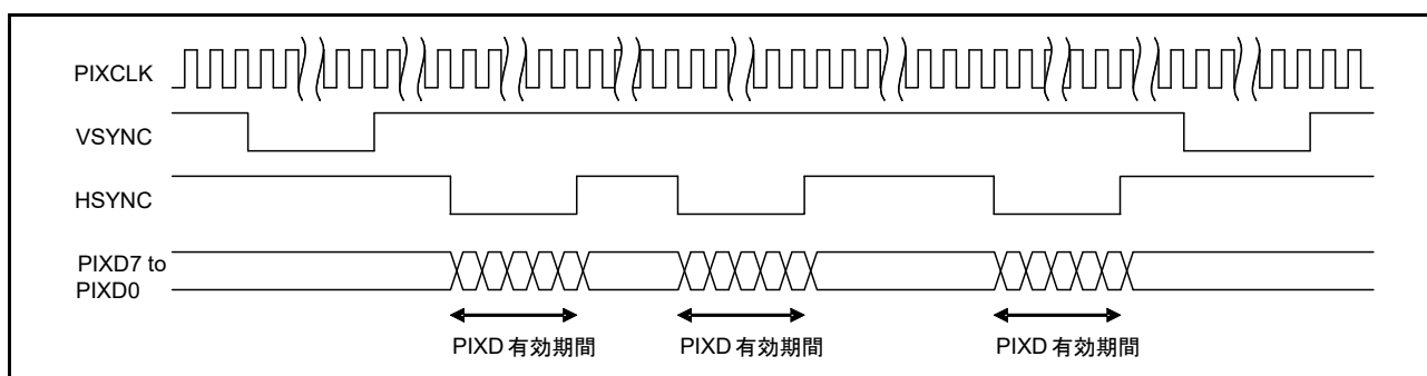
図 50.6 PDC 通信フォーマット (VPS = 0, HPS = 1)
