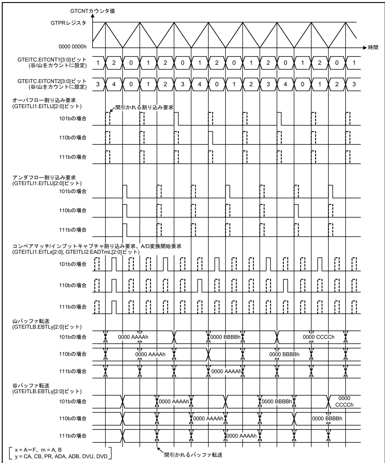
図 26.110 拡張割り込み間引き機能の動作例 ( 三角波、拡張割り込み間引き 1 間引き回数 2 で谷 / 山両方をカウント、拡張割り込み間引き 2 間引き回数 4 で谷 / 山両方をカウント、拡張割り込み間引きカウンタ 2 初期値 "0"、GTEITC.EITCNTk ビット (k = 1, 2) が GTEITC.EIVTTk ビット以外の期間で間引く場合 )
