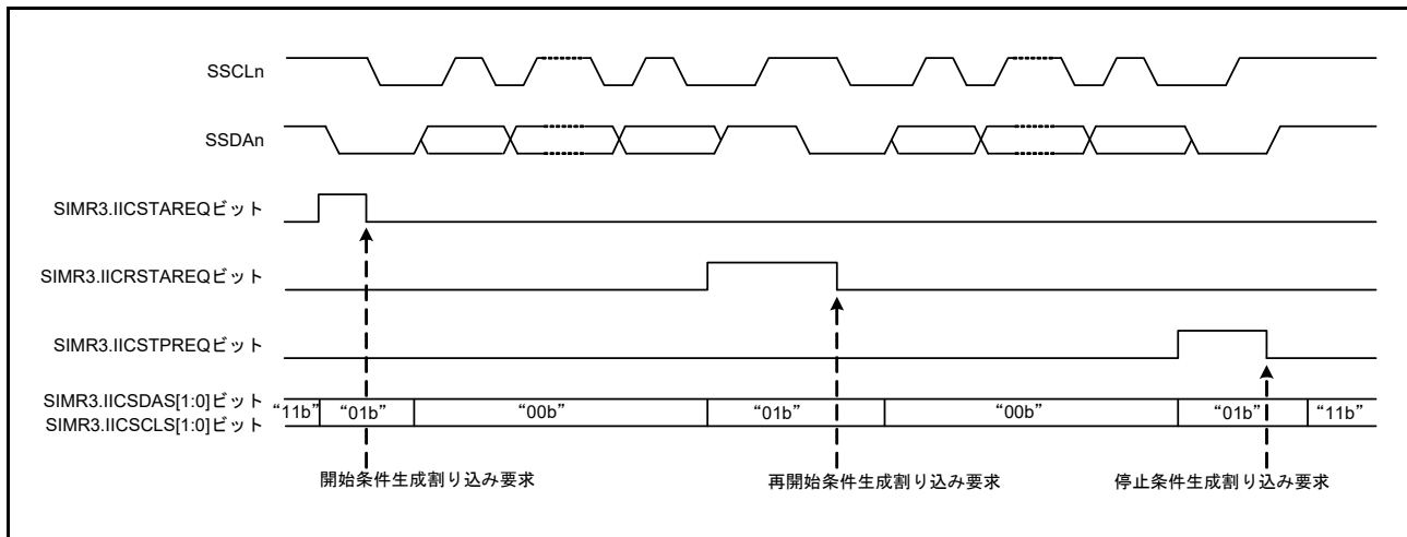
図 41.52 開始条件、再開条件、停止条件生成の動作タイミング
