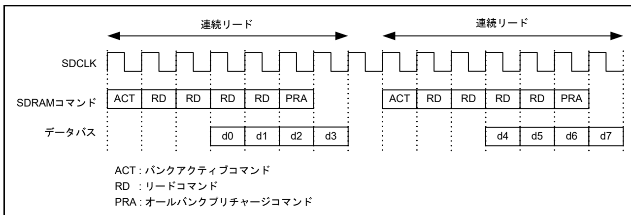
図 16.61 連続リードタイミング例 (SDAMOD.BE = 1, SDTR.CL[2:0] = 010b : 2 サイクルの場合)
