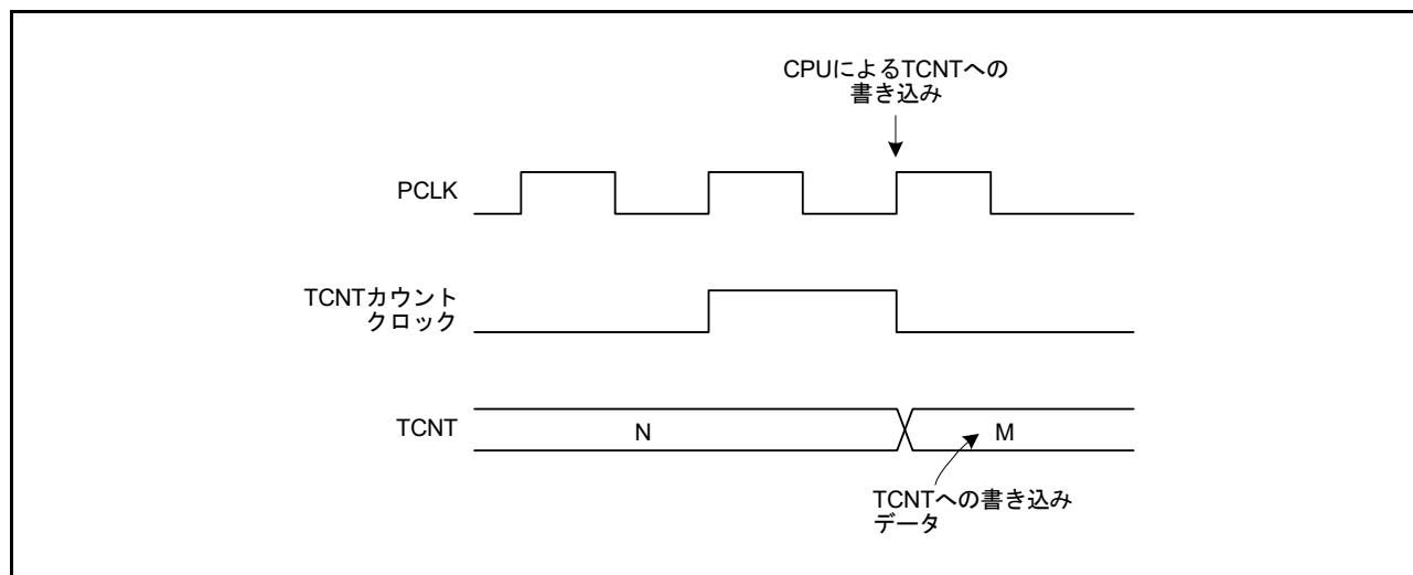
図 30.14 TCNT カウンタへの書き込みとカウントアップの競合
