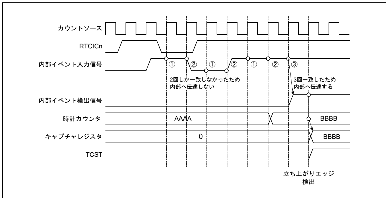
図 33.10 時間キャプチャ機能動作タイミング (フィルタ ON) (n = 0 ~ 2)
