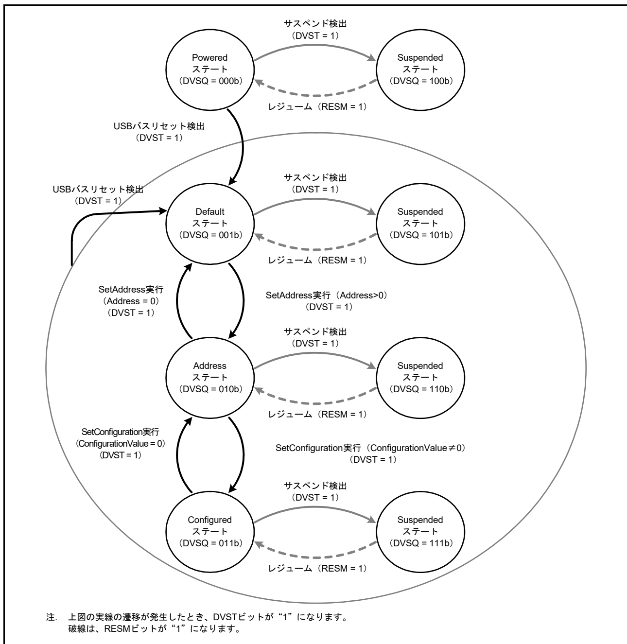
図 40.14 デバイスステート遷移図
