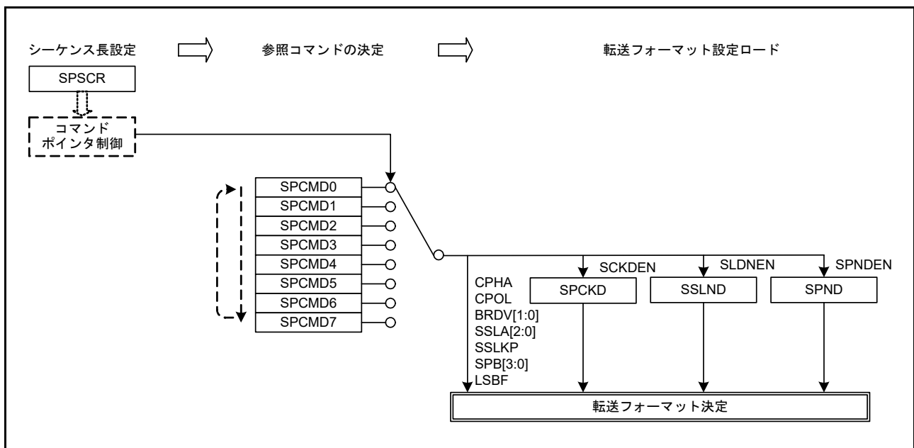
図 44.33 マスタモードでのシリアル転送方式の決定方法
