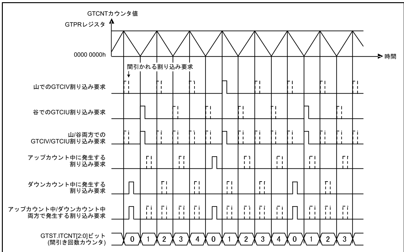
図 26.99 割り込み間引き機能の動作例 (三角波、谷 / 山両方をカウントして間引き、間引き回数 4 の場合)
