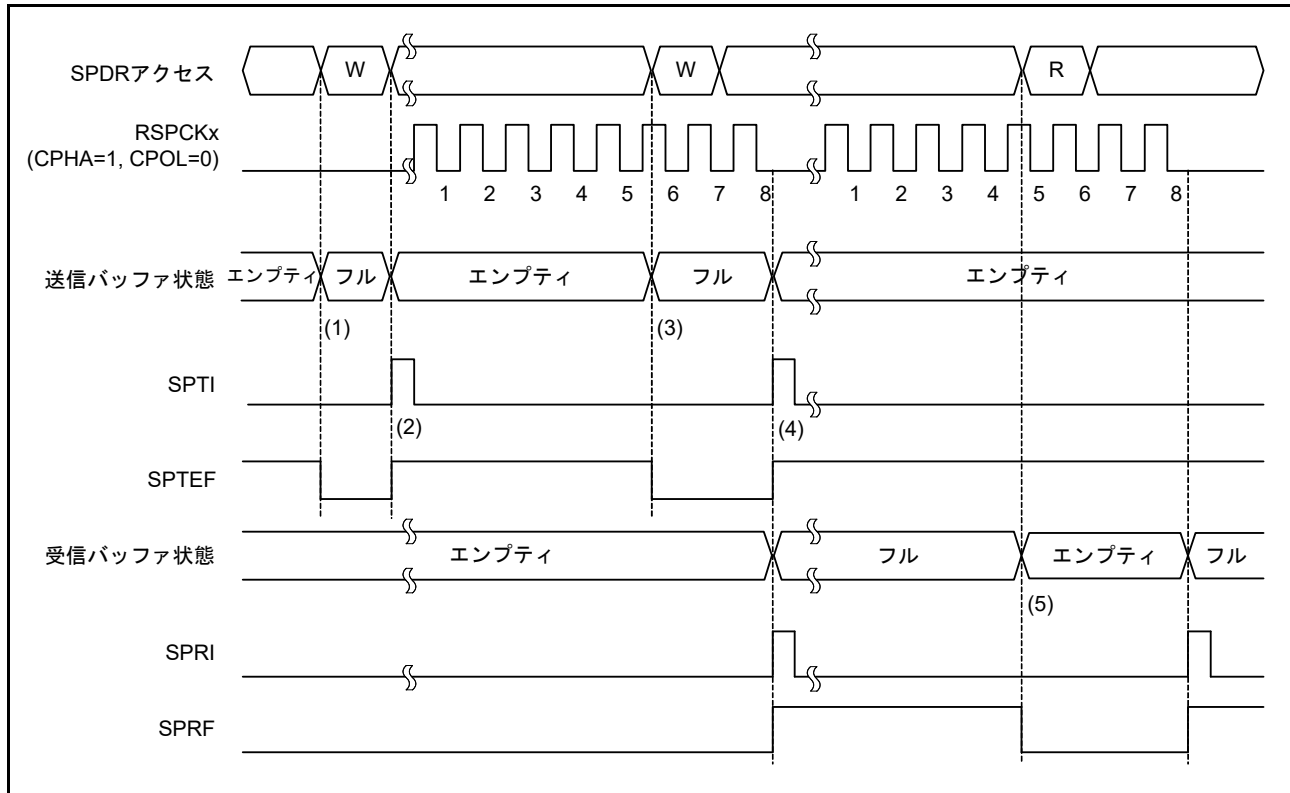
図 44.28 SPTI、SPRI 割り込みの動作例
