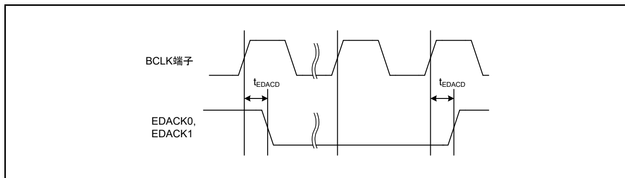
図 63.33 EDACK0、EDACK1 シングルアドレス転送タイミング (CS 領域)
