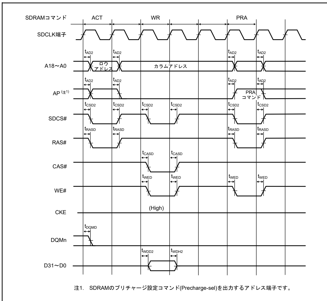
図 63.26 SDRAM 空間シングルライトバスタイミング
