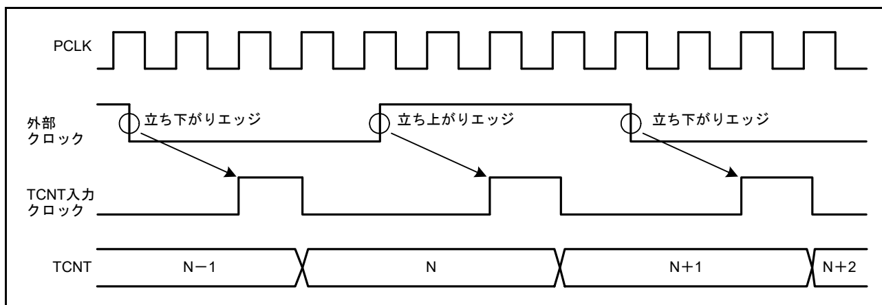
図 28.32 外部クロック動作時のカウントタイミング
