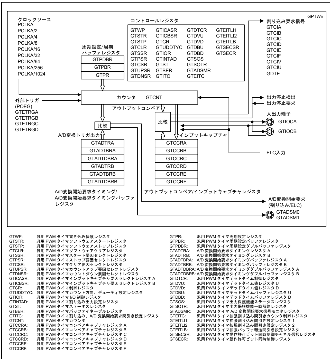
図 26.1 GPTW のブロック図 (n = 0 ~ 3)
