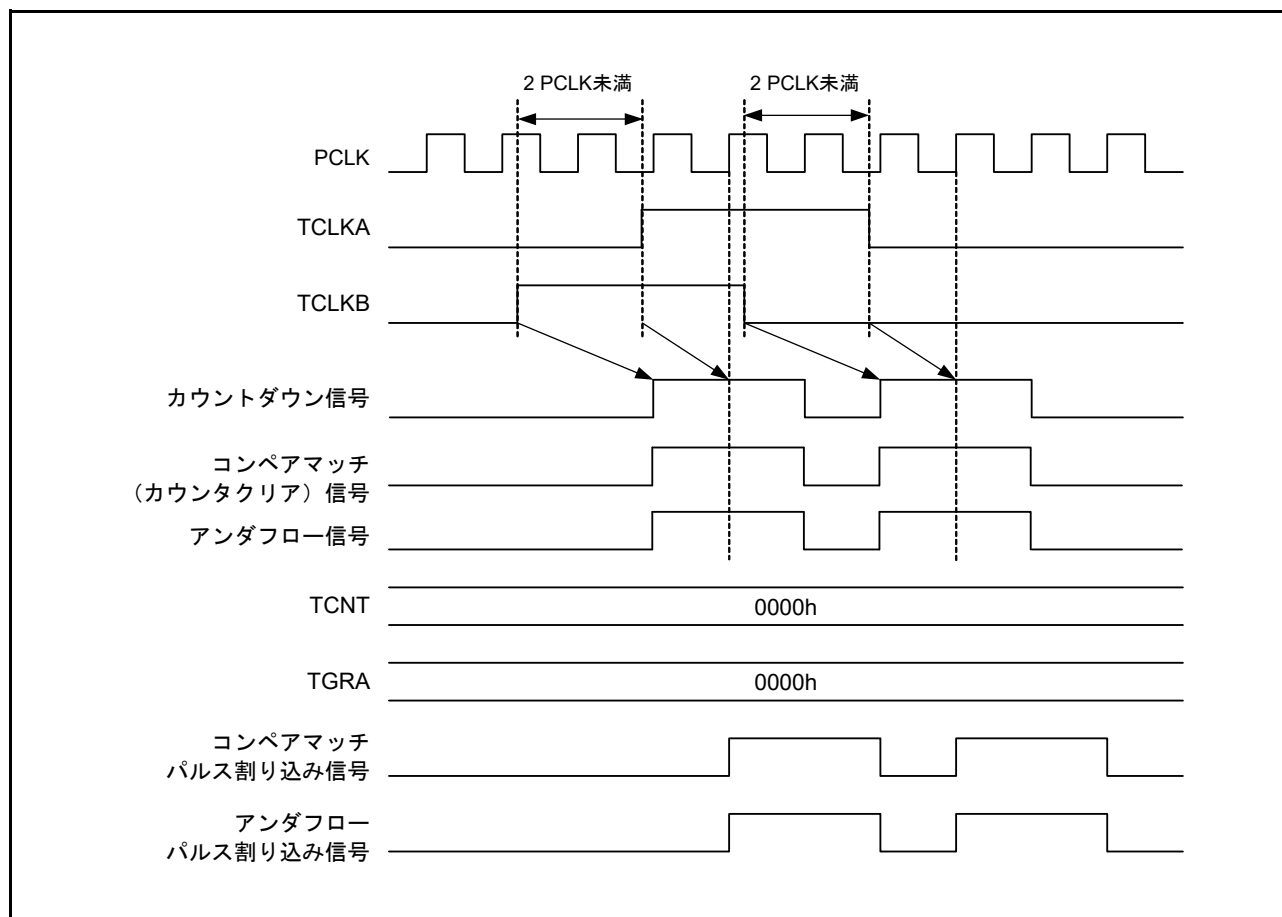
図 28.55 アンダフローパルス割り込みの連続出力
