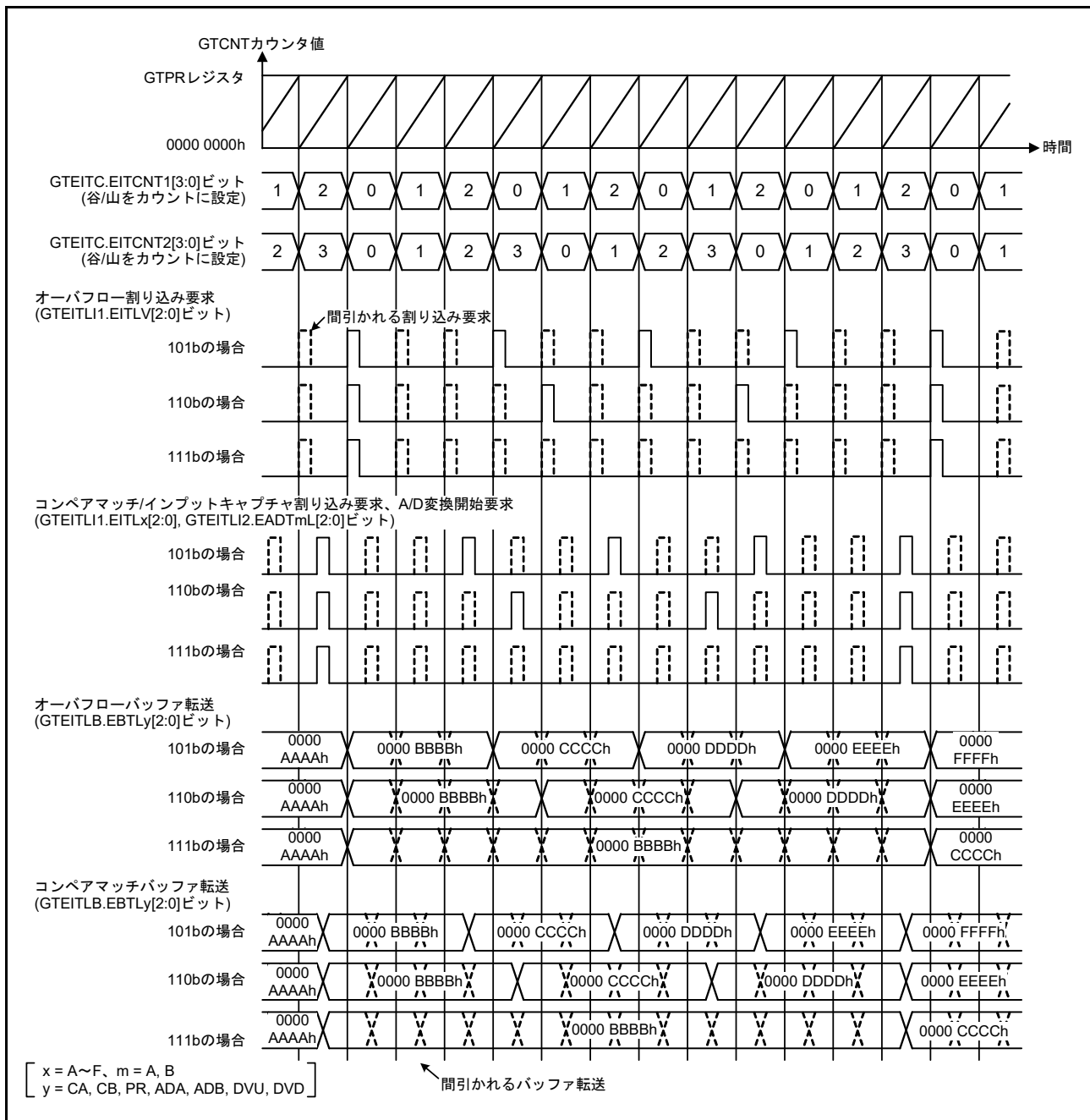
図 26.112 拡張割り込み間引き機能の動作例 (のこぎり波アップカウント、拡張割り込み間引き 1 間引き回数 2 でオーバーフローをカウント、拡張割り込み間引き 2 間引き回数 3 でオーバーフローをカウント、拡張割り込み間引きカウンタ 2 初期値 “0”、GTEITC.EITCNTk ビット (k = 1, 2) が GTEITC.EIVTTk ビット以外の期間で間引く場合)
