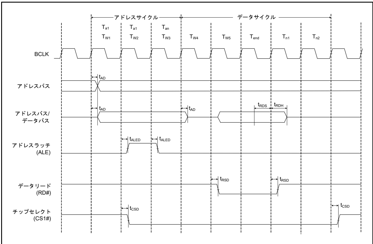
図 63.18 アドレス/データマルチプレクスバスのリードアクセスタイミング
