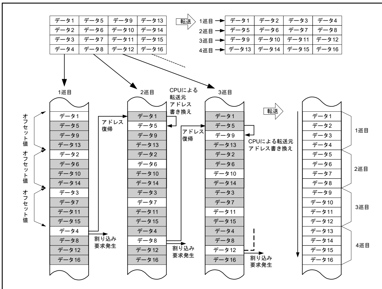
図 18.8 リピータ転送モード + オフセット加算による XY 変換のときの動作
