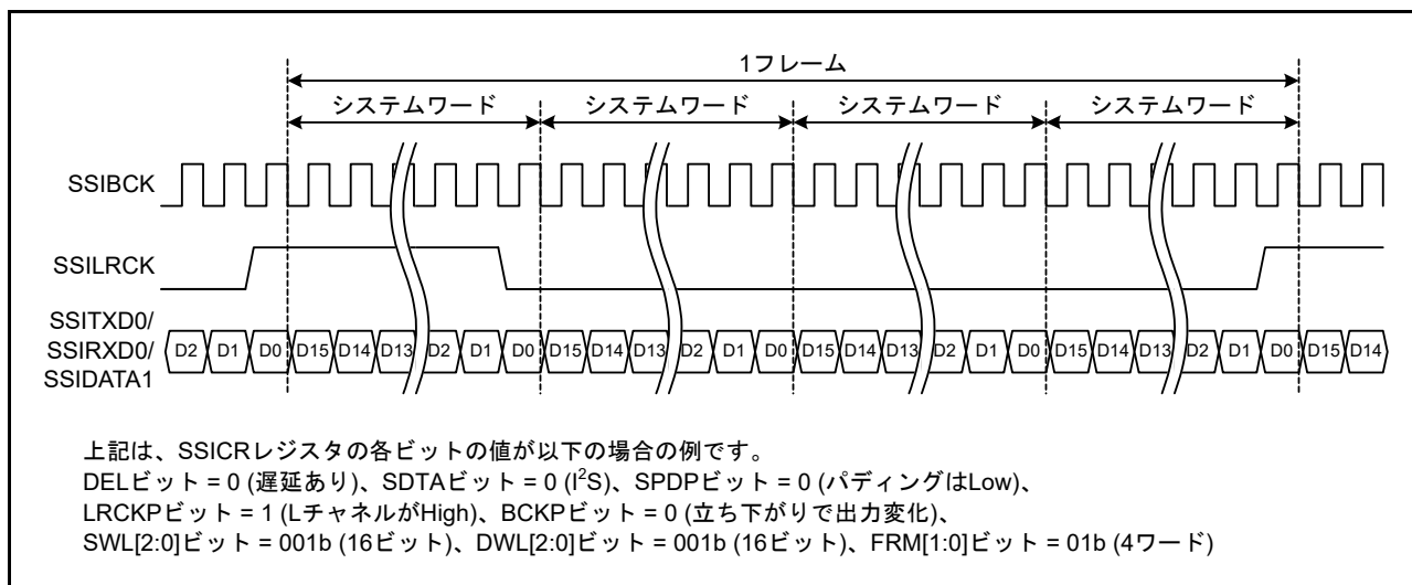
図 47.15 TDM フォーマットの例 (1) (SSICR.DEL ビット = 0、パディングなし)
