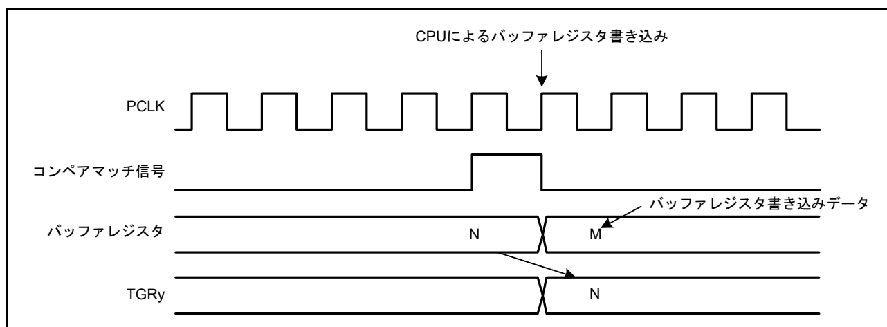
図 28.47 バッファレジスタへの書き込みとコンペアマッチの競合
