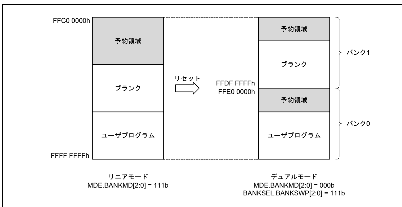
図 62.52 リセット前後のメモリマップ (コードフラッシュメモリ容量が4M バイト未満の製品の例)
