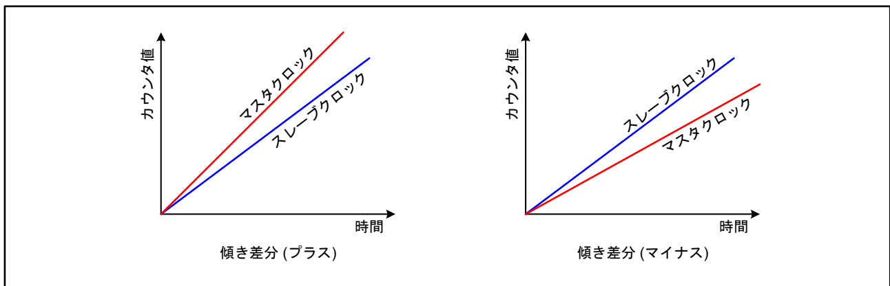
図 37.27 傾き差分の概念
