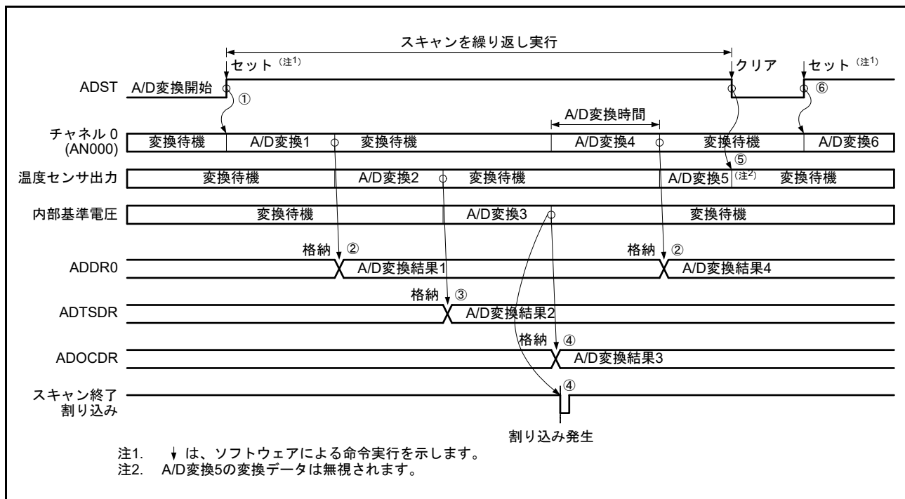
図 56.21 連続スキャンモードの動作例 (基本動作 : AN000、温度センサ出力、内部基準電圧選択)
