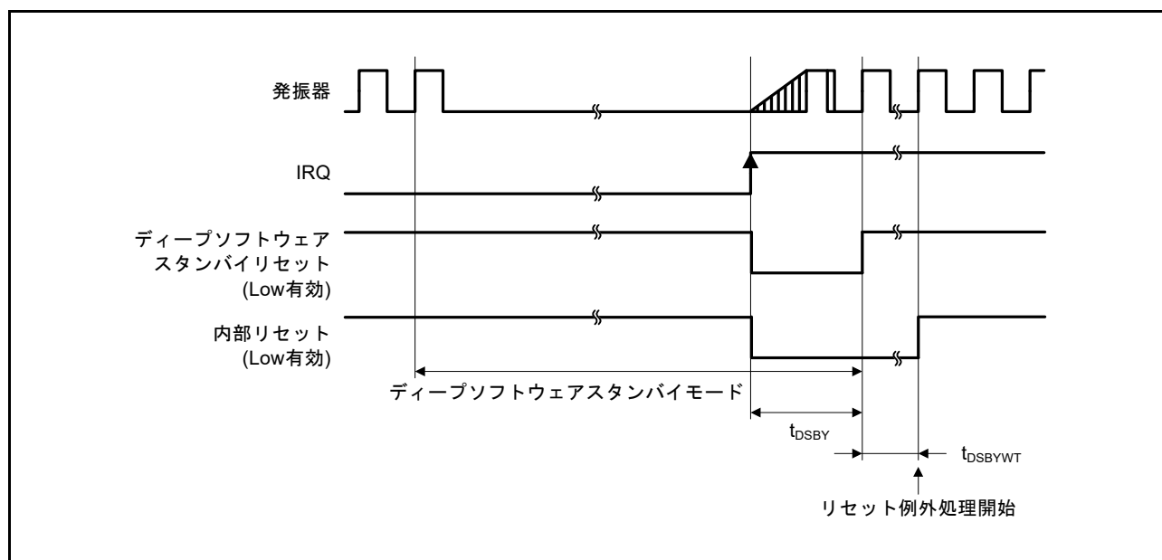
図 63.15 ディープソフトウェアスタンバイモード解除タイミング
