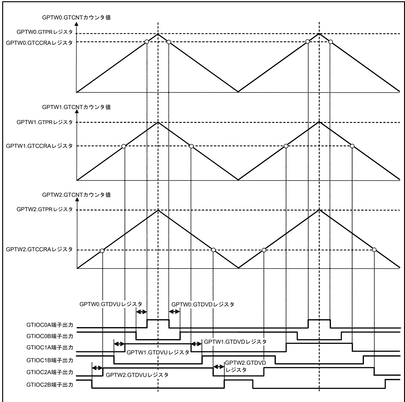
図 26.85 三角波3相相補PWM出力例(デッドタイム自動設定)
