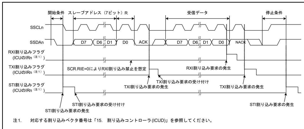
図 41.59 簡易 I 2 C バスモードのマスタ受信の動作例 (7 ビットスレーブアドレス、送信割り込み、受信割り込み使用時)
