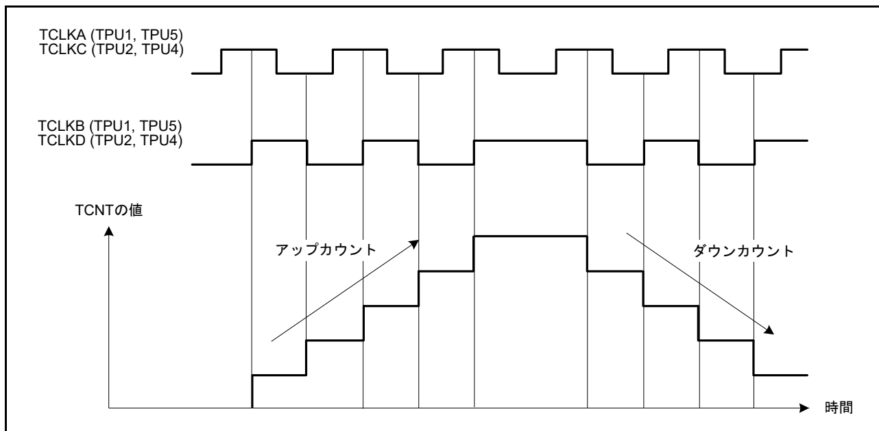
図 28.28 位相計数モード4の動作例
