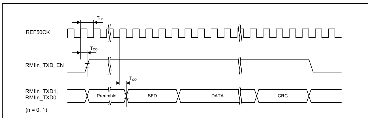
図 63.82 RMII 送信タイミング
