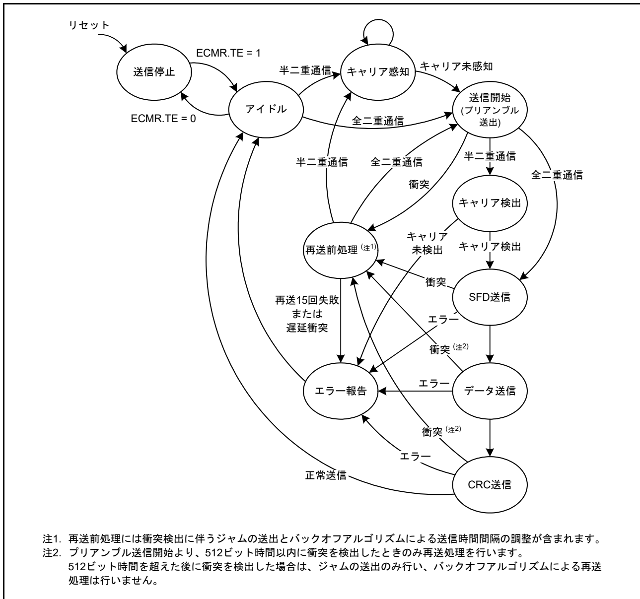
図 36.4 ETHERC 送信部状態遷移図
