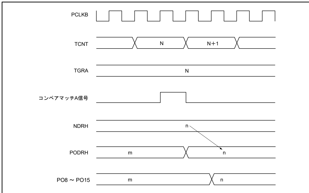
図 29.5 NDR の内容が転送・出力されるタイミング例
