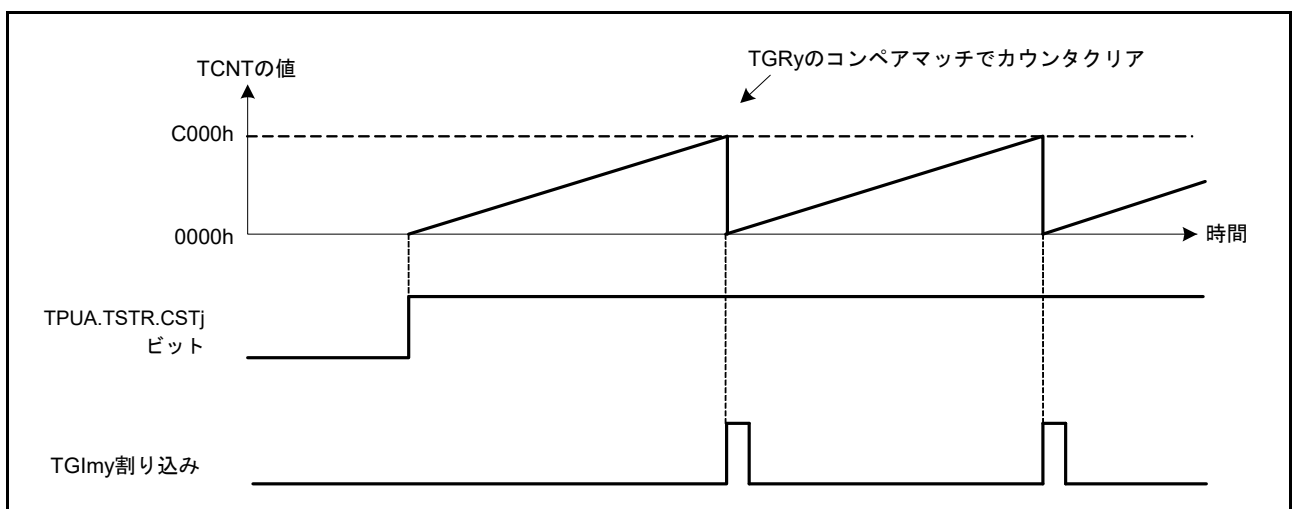
図 28.4 周期カウンタの動作
