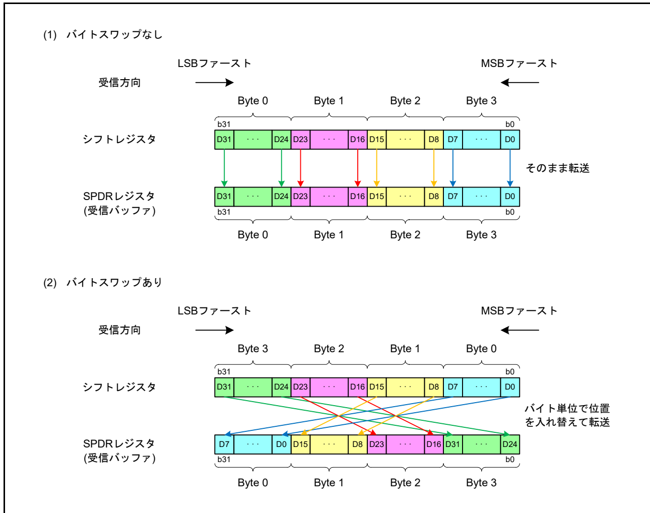
図 44.23 MSB/LSB ファーストとバイトスワップあり/なしの設定と受信データ変換
