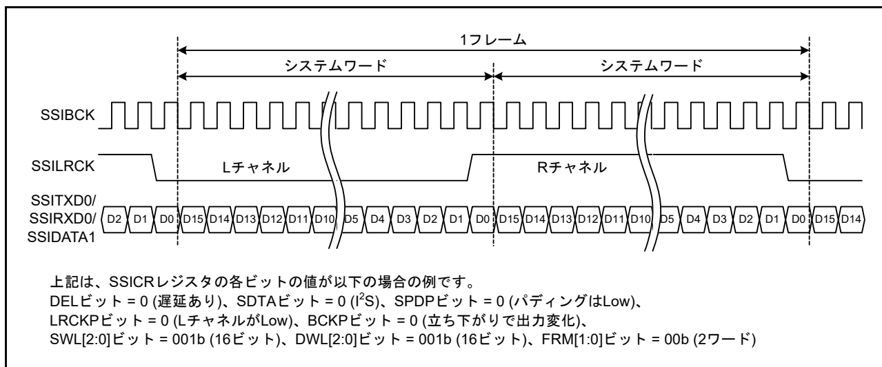
図47.9 I 2 S フォーマットの例
