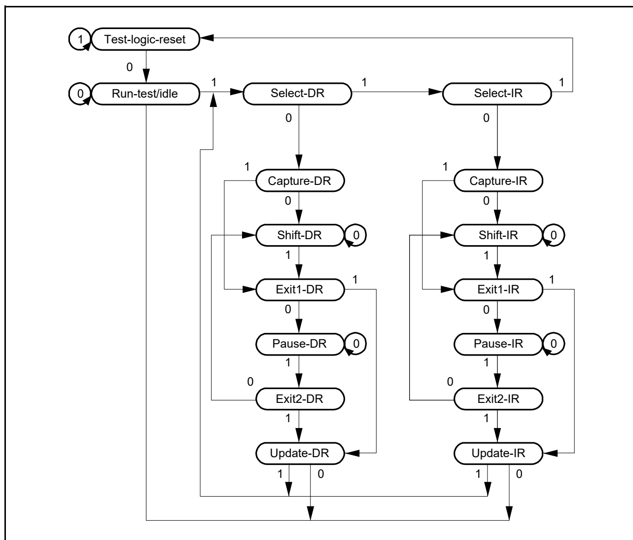
図 53.2 TAP コントローラの状態遷移図
