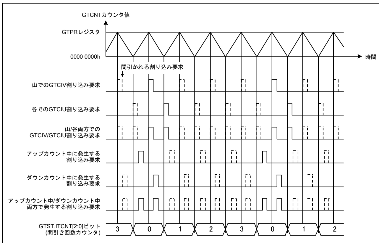
図 26.98 割り込み間引き機能の動作例 (三角波、谷をカウントして間引き、間引き回数 3 の場合)
