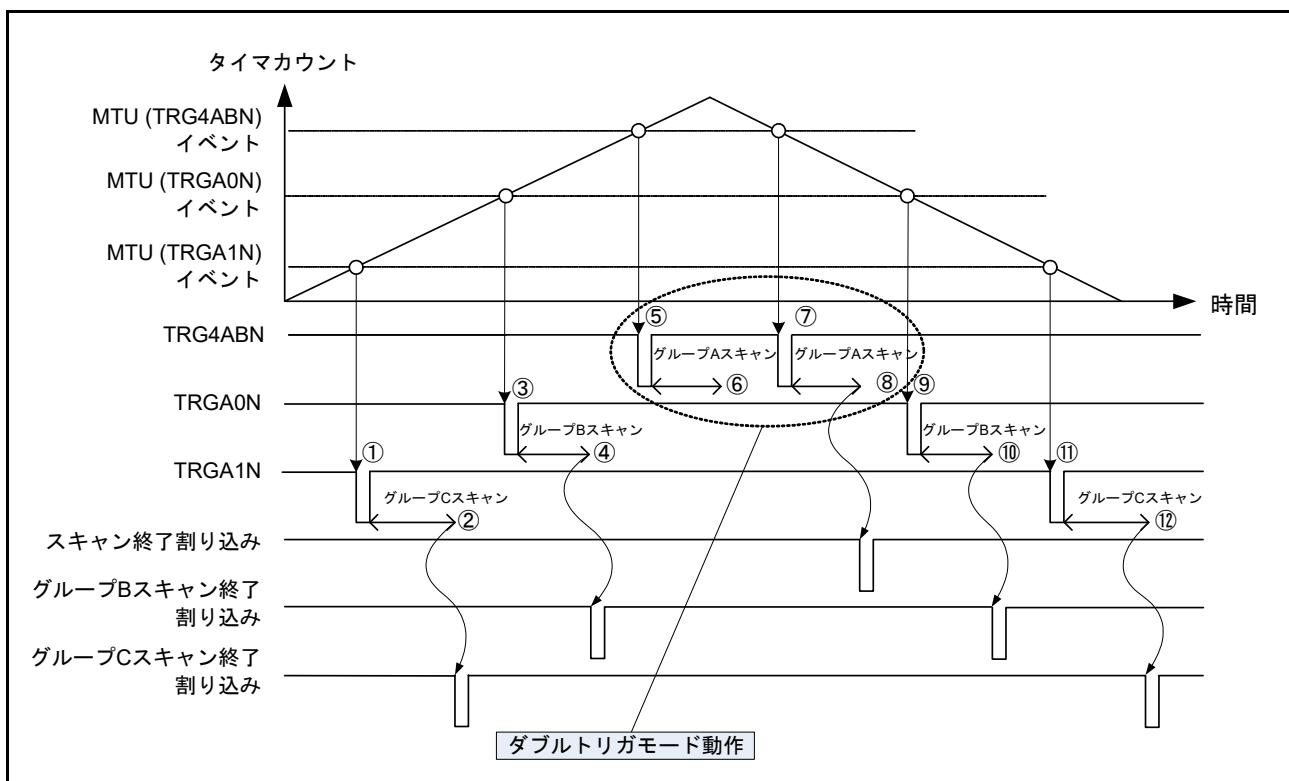
図 56.23 グループスキャンモードでダブルトリガモード選択時の動作例 (MTUからの同期トリガ発生による基本動作)
