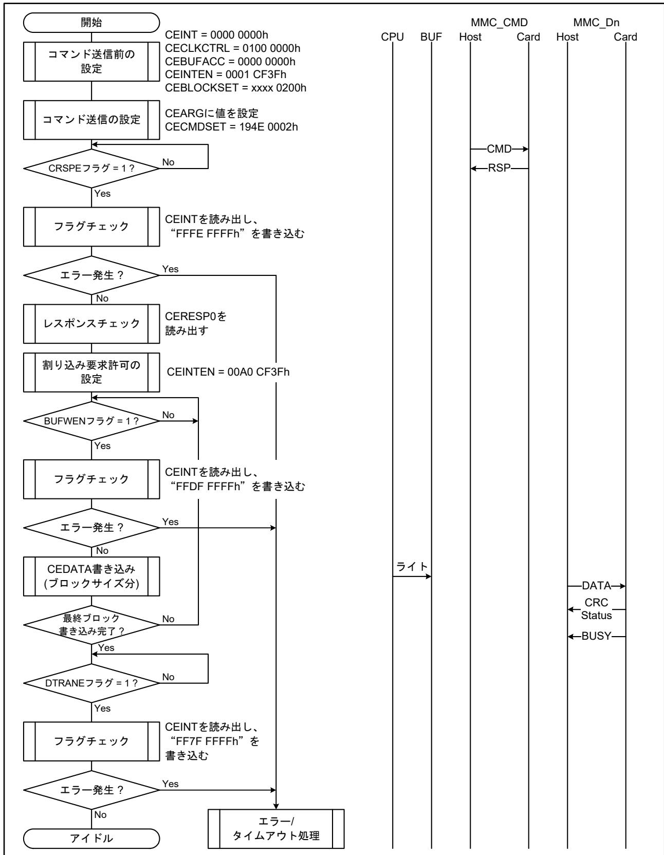
図 49.19 マルチブロックライトコマンドの送信例 (CMD25 Pre-defined)
