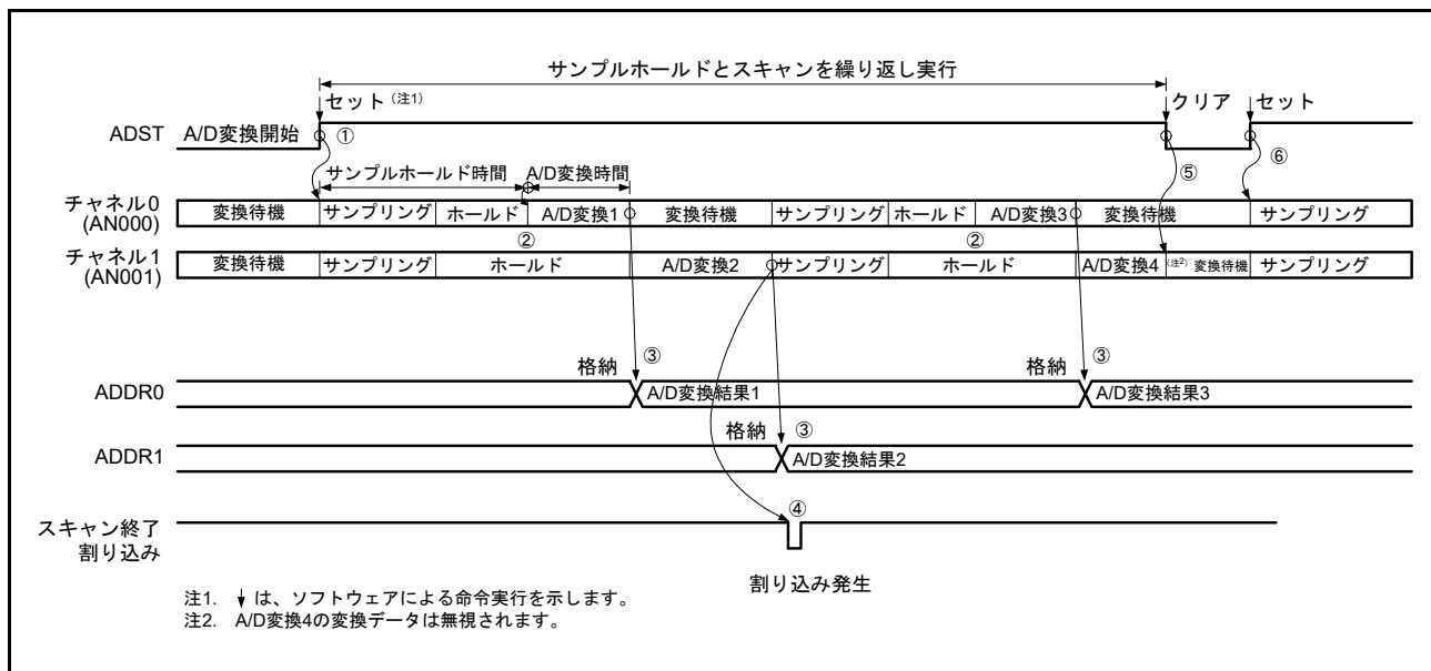
図 56.16 連続スキャンモードの動作例 (チャンネル専用サンプル & ホールド回路使用 : AN000, AN001 選択、常時サンプリング無効)
