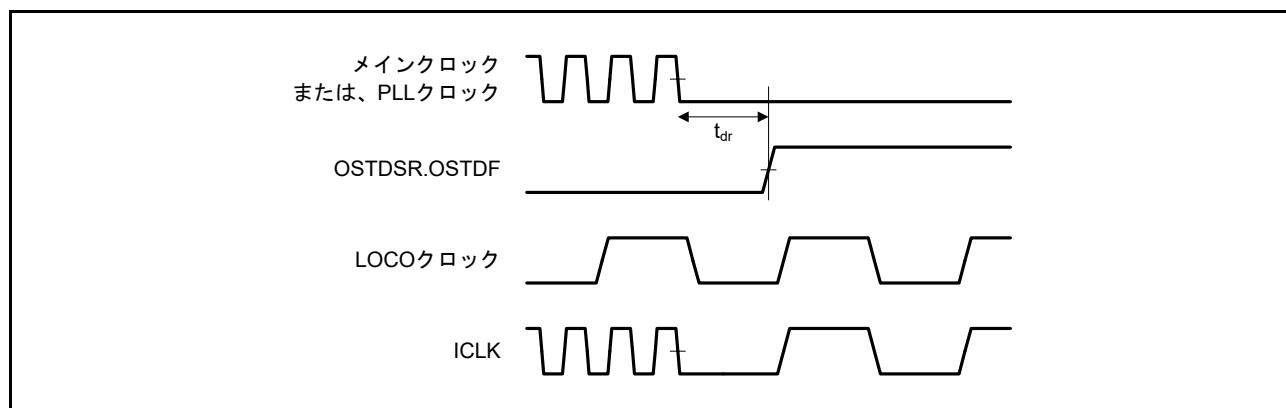
図 63.106 発振停止検出タイミング
