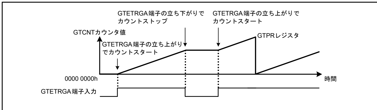
図 26.62 ハードウェア要因によるカウントスタート/ストップ動作例 (GTETRGA 端子入力の立ち上がりでスタート、GTETRGA 端子入力の立ち下がりでストップ時)
