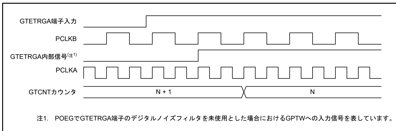
図 26.10 イベントカウント動作例 (GTETRGA 端子入力の立ち上がりによるダウンカウント)
