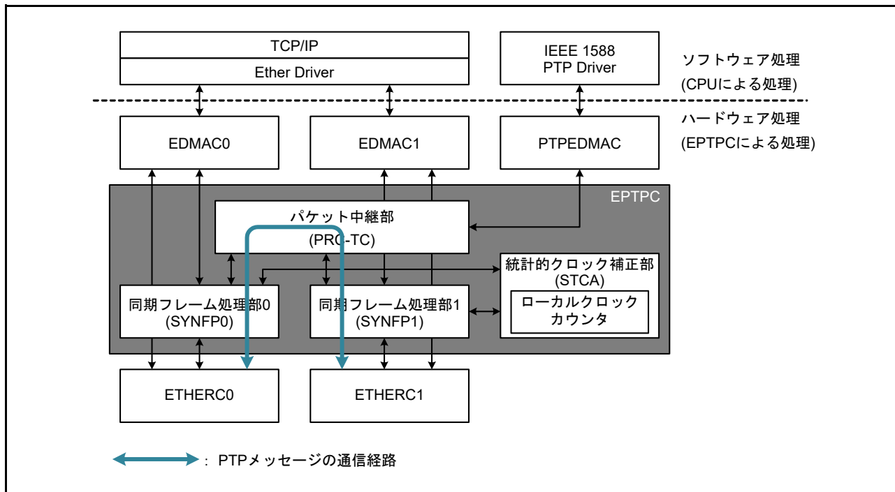
図37.8 ハードウェアによるPTPメッセージの中継経路
