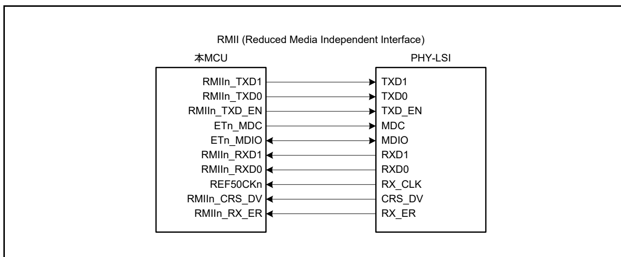
図 36.3 PHY-LSI との接続例 (RMII)
