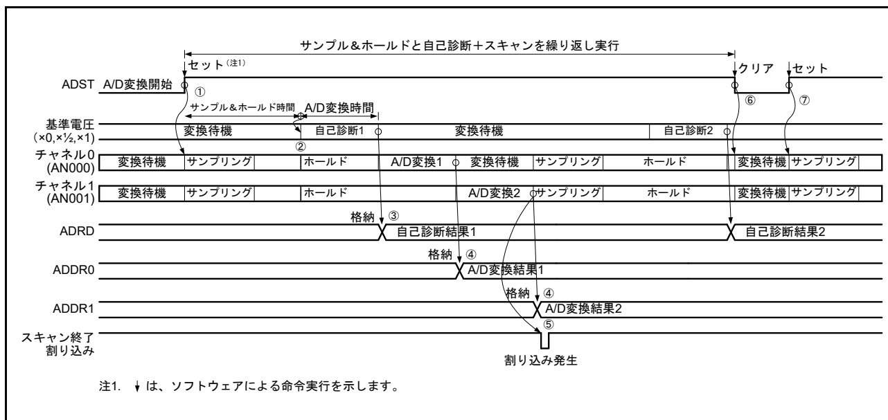
図 56.19 連続スキャンモードの動作例 (チャネル専用サンプル & ホールド回路使用 : AN000, AN001 選択 + 自己診断)
