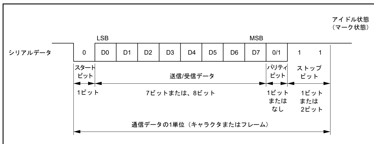
図 41.6 調歩同期式シリアル通信のデータフォーマット (8 ビットデータ / パリティあり / 2 ストップビットの例)
