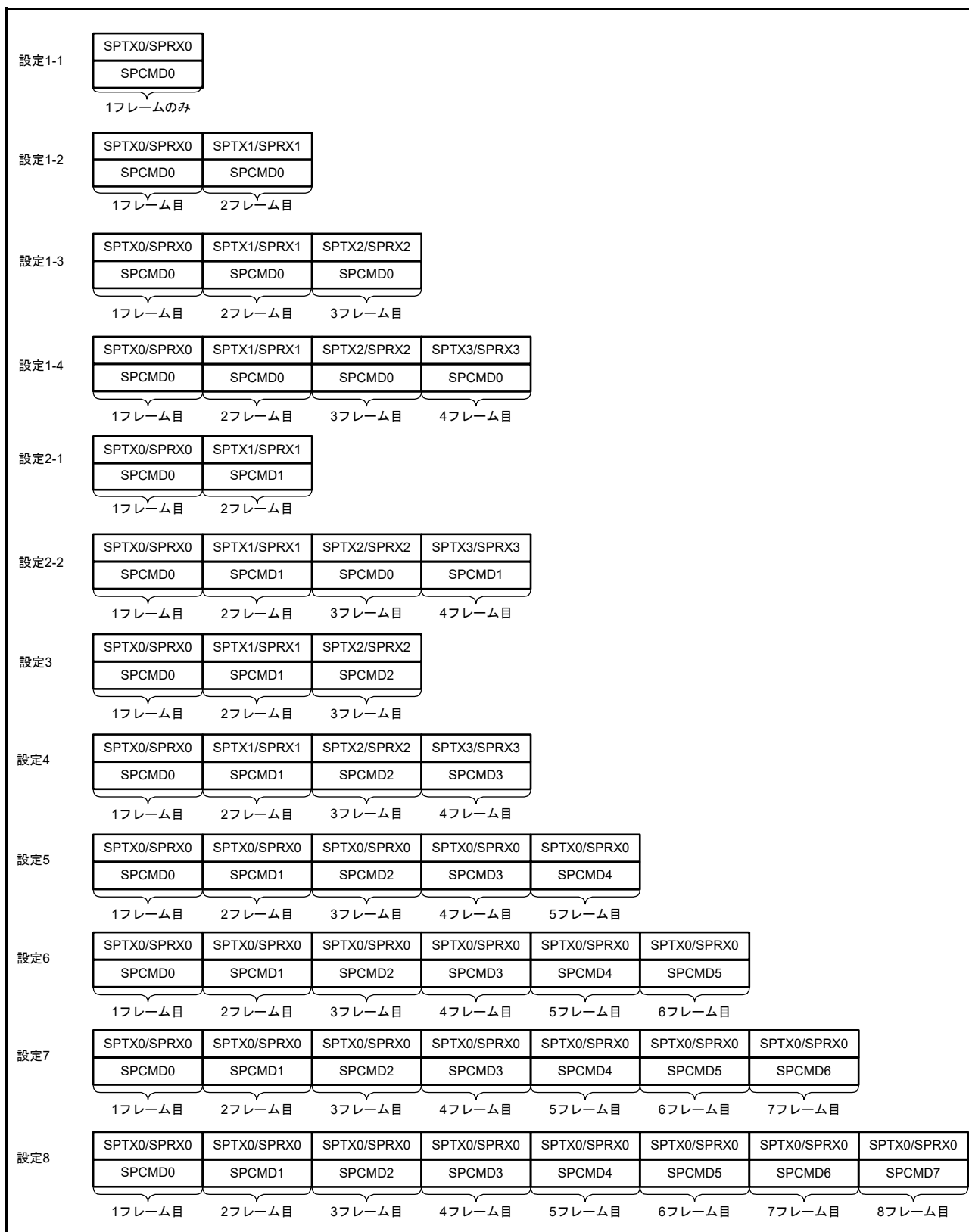
図 44.47 シーケンス動作時の RSPI コマンドレジスタと送受信バッファの対応
