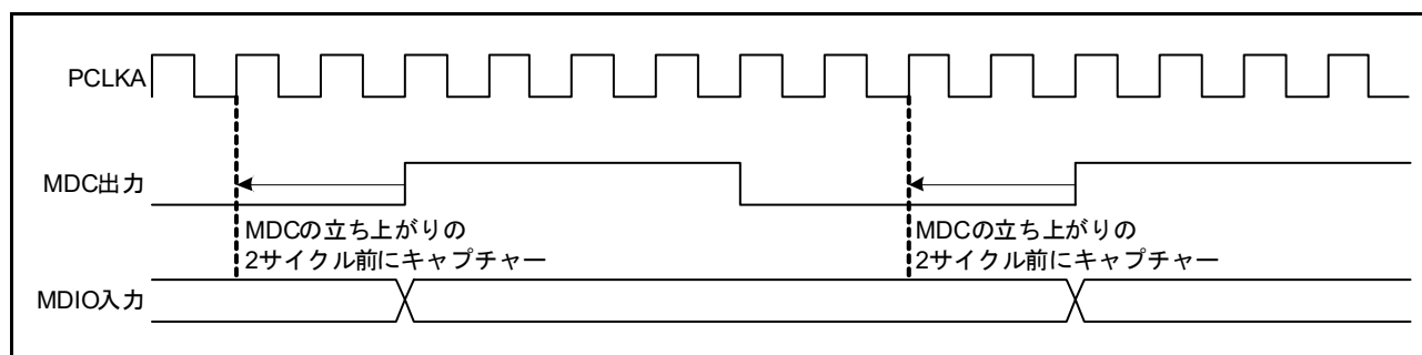
図 39.10 PCLKA の 2 サイクル前にキャプチャー時のタイミング
