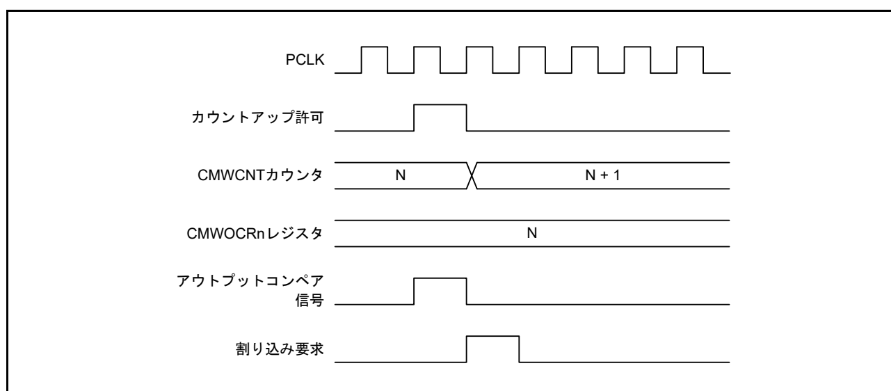
図 32.14 アウトプットコンペア割り込みの発生タイミング ( n = 0, 1 )
