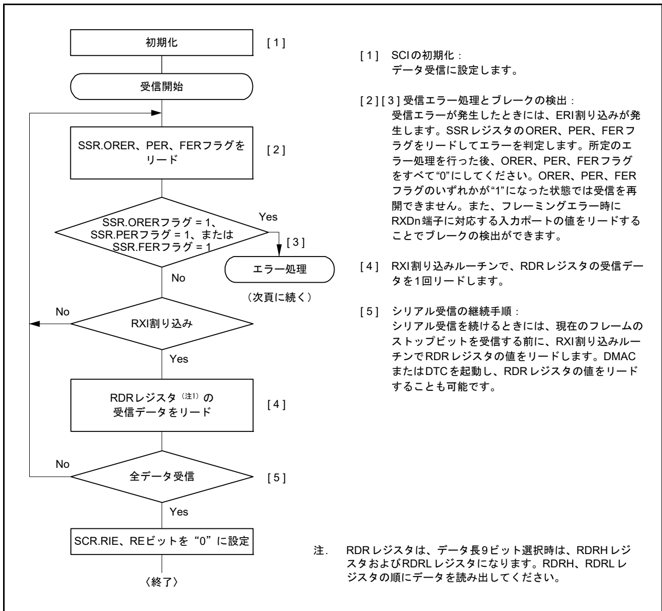
図 41.20 調歩同期式モードのシリアル受信のフローチャート例 (1)
