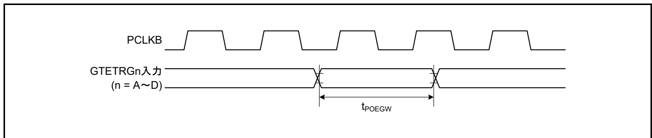
図 63.47 POEG 入力タイミング
