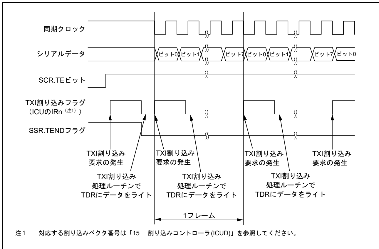
図 41.29 クロック同期式モードのシリアル送信の動作例 (1) (送信開始・CTS 機能使用しない)
