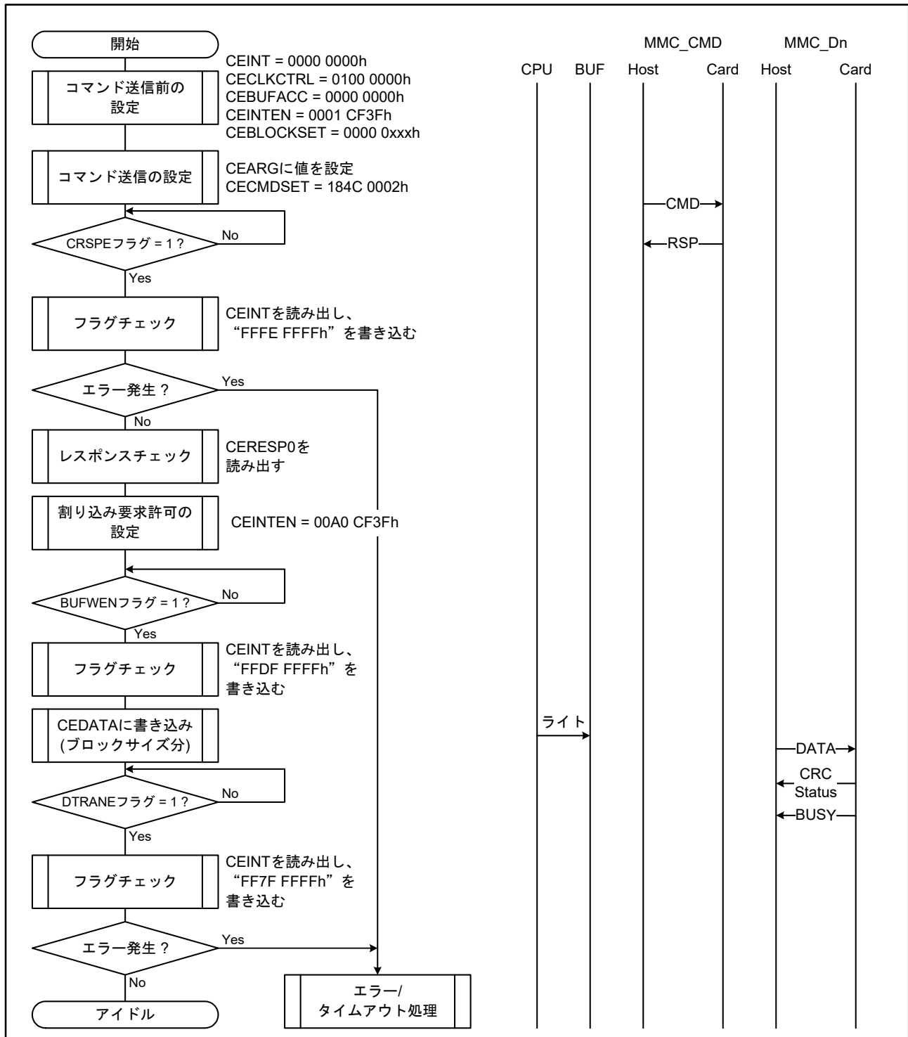
図 49.18 シングルブロックライトコマンドの送信例 (CMD24)
