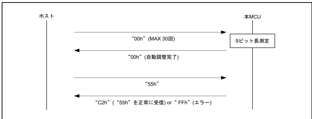
図 62.42 ホストと本 MCU 間の通信シーケンス
