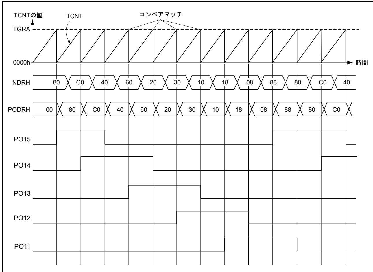
図 29.8 パルス出力通常動作例 (5相パルス出力例)
