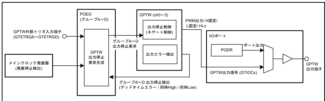
図 27.1 POEG のシステム概要図
