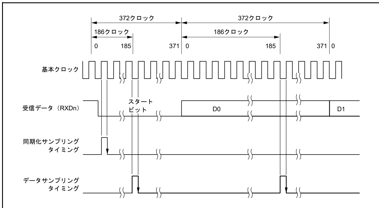
図 41.41 スマートカードインタフェースモード時の受信データサンプリングタイミング (372 倍のクロック使用時)
