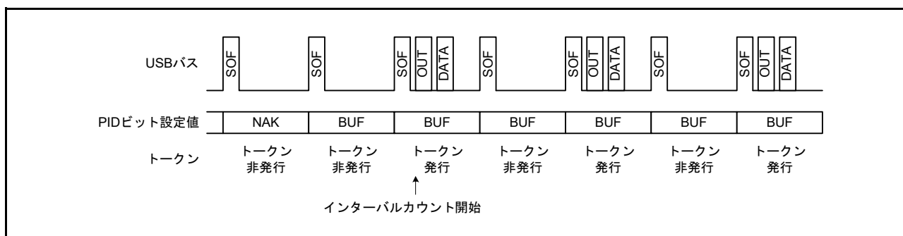
図 40.17 IITV[2:0] = 001b の場合のトークン発行有無
