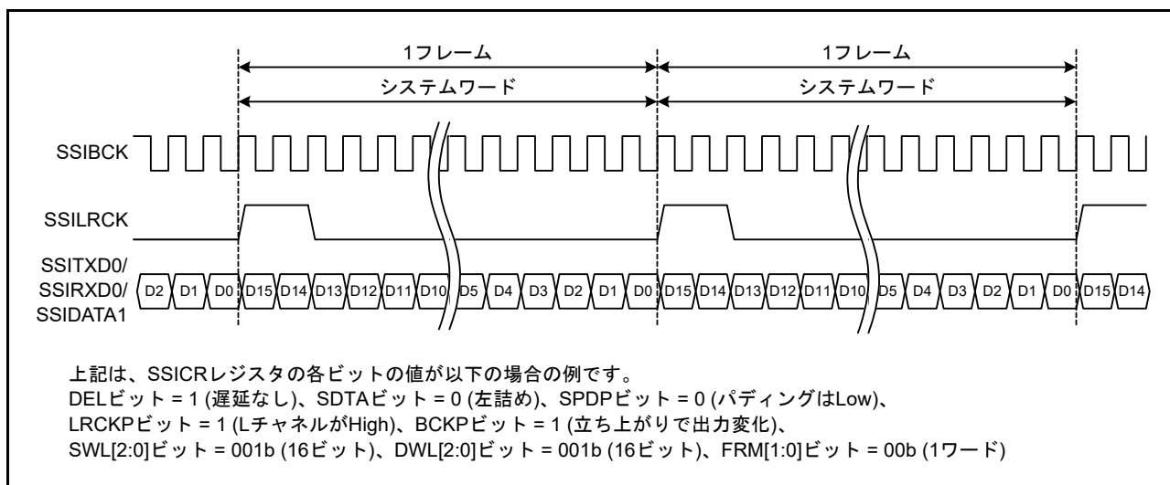
図 47.14 モノラルフォーマットの例 (3) (SSICR.DEL ビット = 1、パディングなし)
