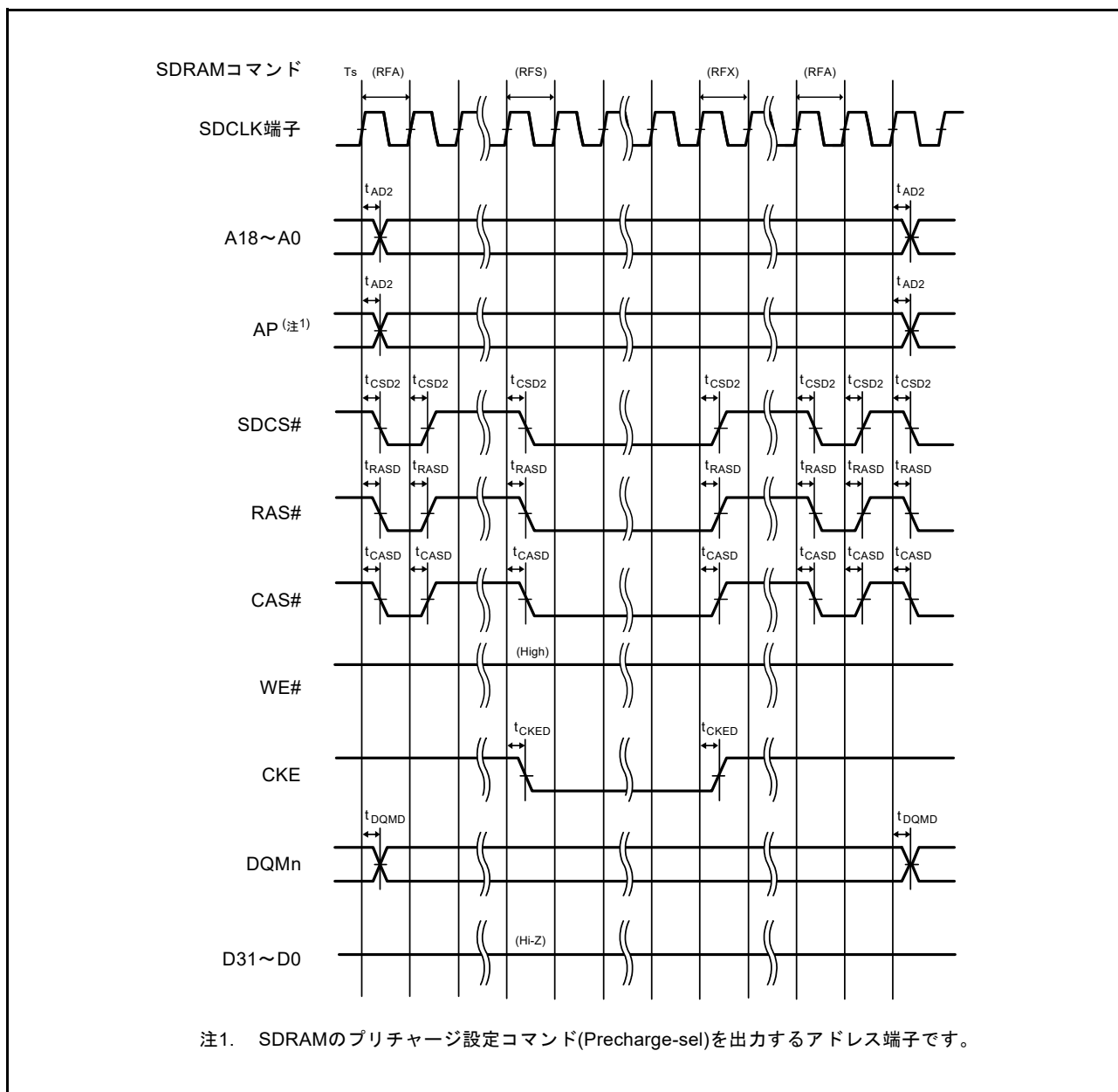
図 63.31 SDRAM 空間セルフリフレッシュバスタイミング
