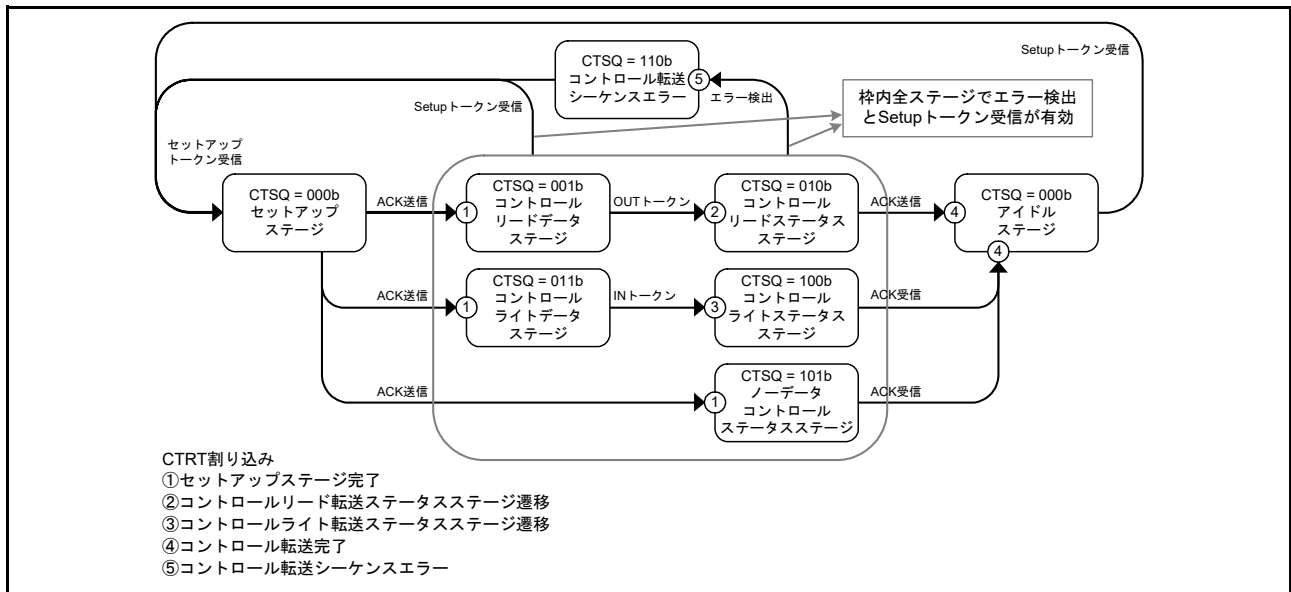
図 40.15 コントロール転送ステージ遷移図
