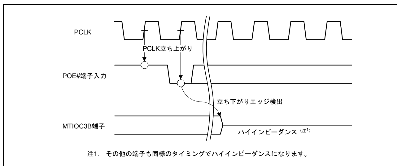
図 25.3 立ち下がりエッジ検出を選択した場合の動作
