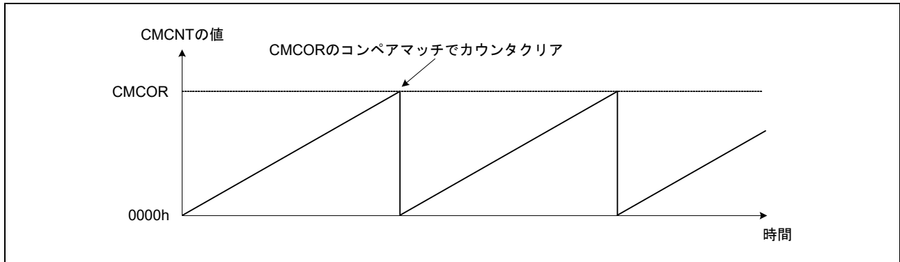
図 31.2 CMCNT カウンタの動作
