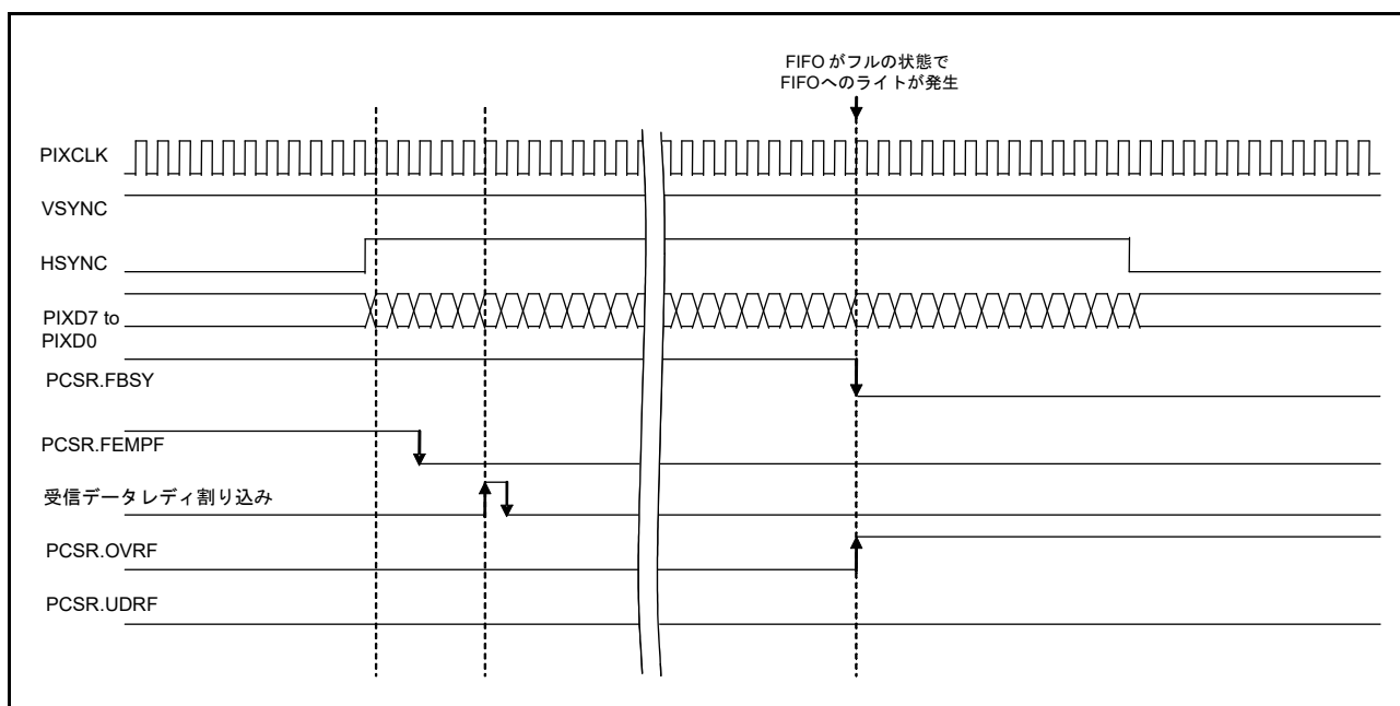
図 50.14 オーバラン
