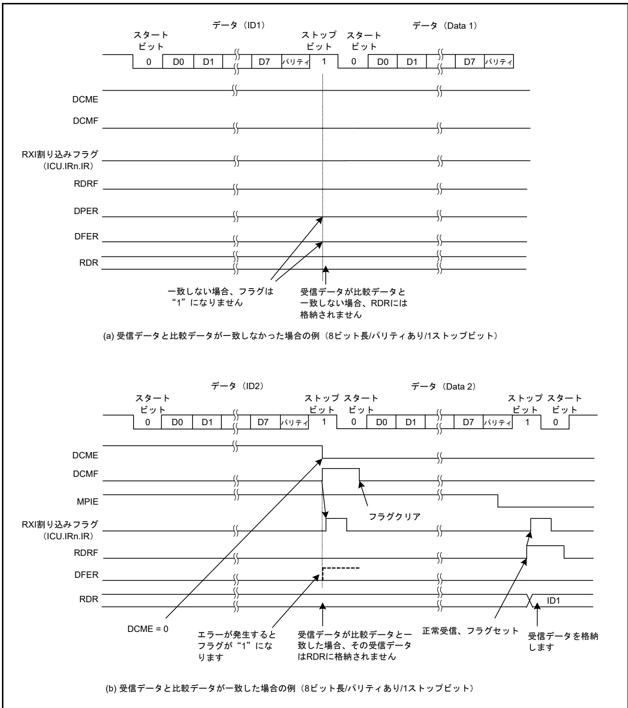
図 41.9 データ一致検出の例 (1) 非マルチプロセッサモード
