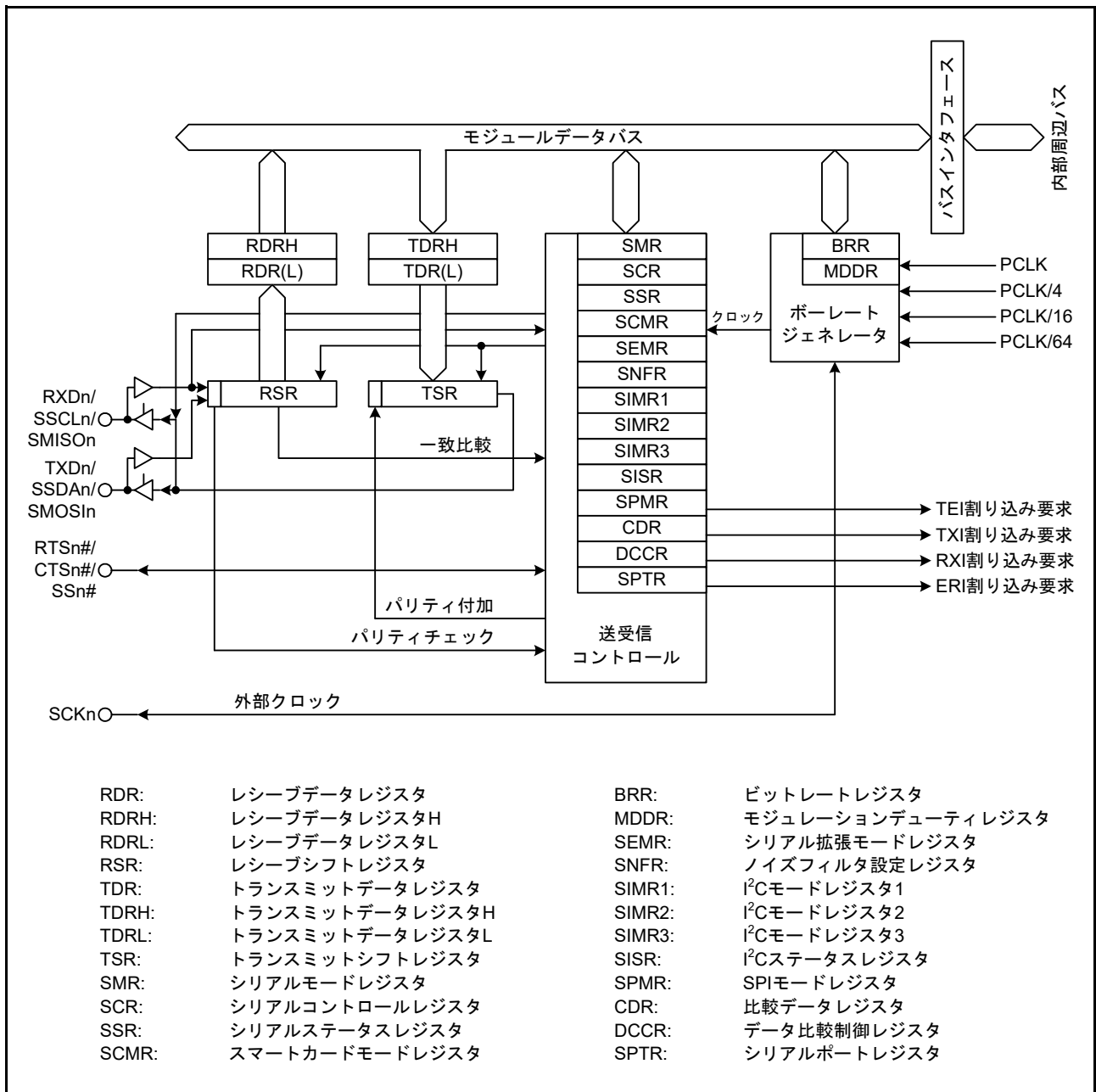
図 41.1 SCIj (SCI0 ~ SCI4) のブロック図
