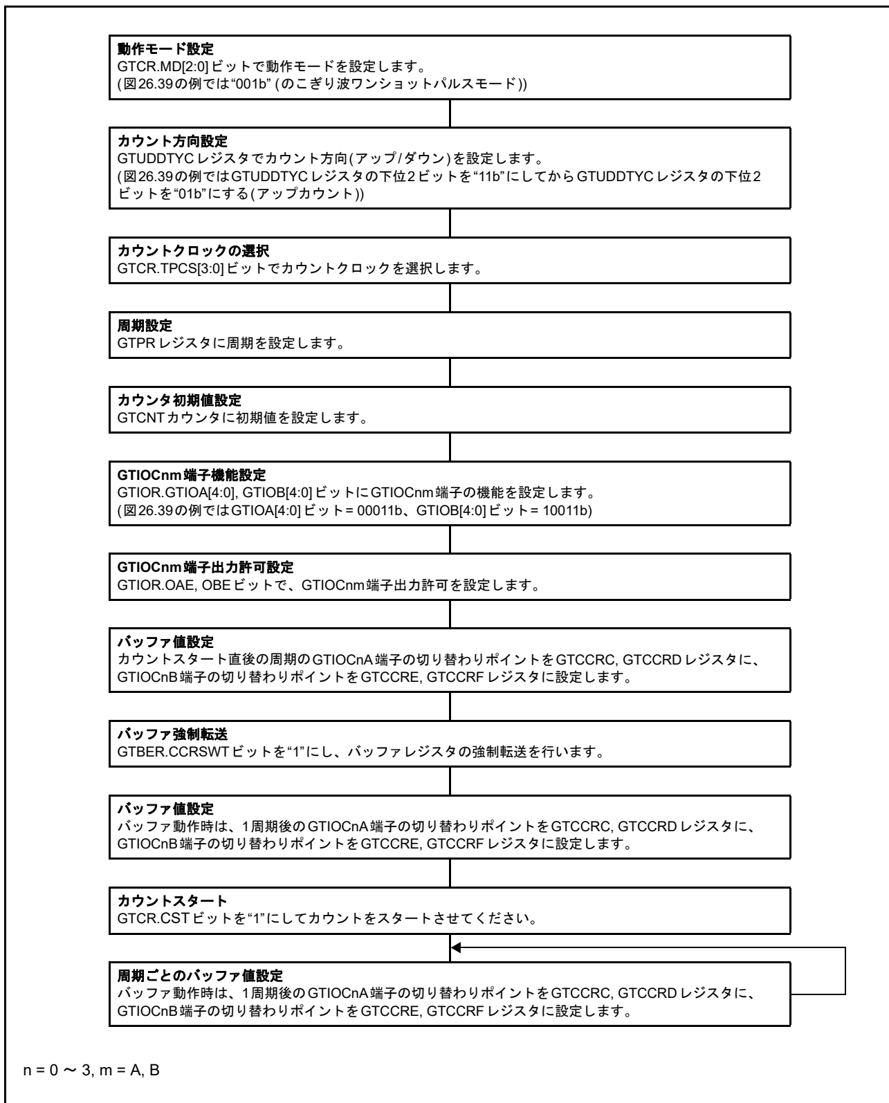
図 26.40 のこぎり波ワンショットパルスモード設定例
