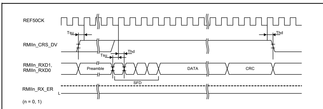
図 63.83 RMII 受信タイミング (正常動作時)
