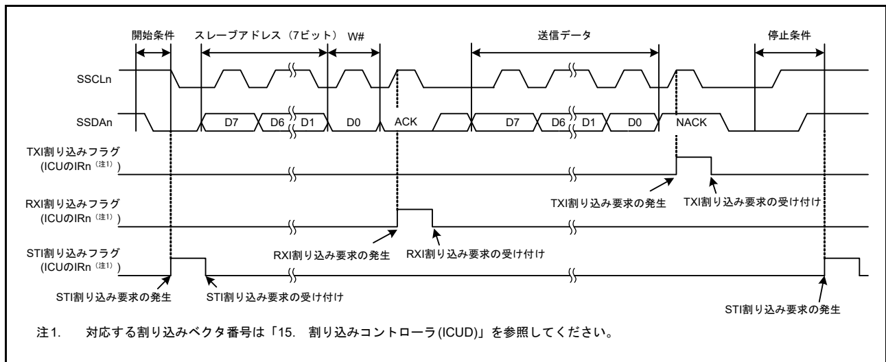
図 41.57 簡易 I 2 C バスモードのマスタ送信の動作例 2 (7 ビットスレーブアドレス、ACK 割り込み、NACK 割り込み使用時)
