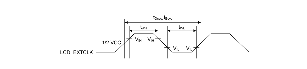
図 63.94 LCD_EXTCLK クロック入カタイミング
