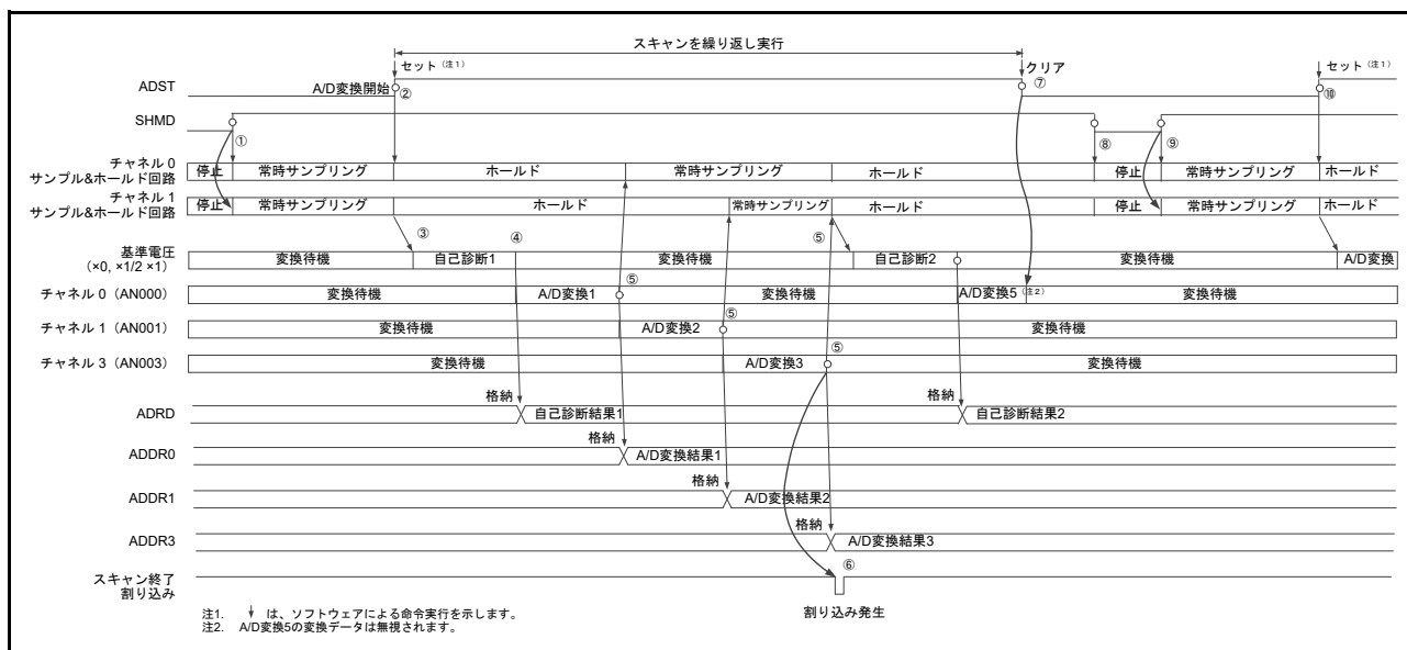
図 56.20 連続スキャンモードの動作例 (チャンネル専用サンプル & ホールド回路使用 : AN000, AN001, AN003 選択 + 自己診断、常時サンプリング有効)
