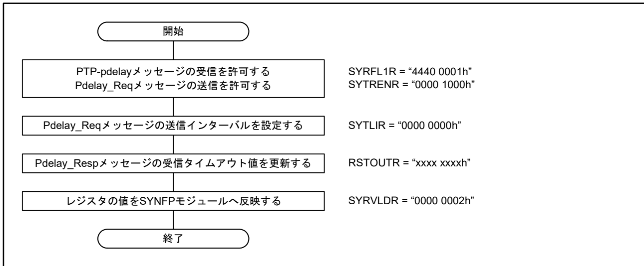
図37.16 P2P動作の開始手順
