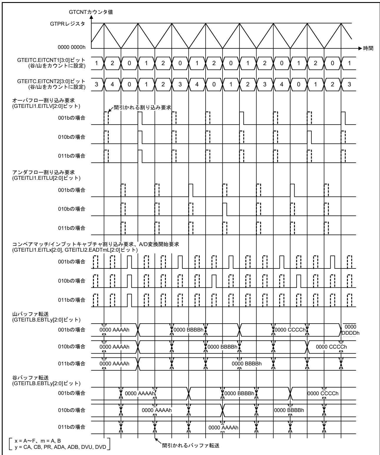
図 26.109 拡張割り込み間引き機能の動作例 (三角波、拡張割り込み間引き 1 間引き回数 2 で谷 / 山両方をカウント、拡張割り込み間引き 2 間引き回数 4 で谷 / 山両方をカウント、拡張割り込み間引きカウンタ 2 初期値 “0”、GTEITC.EITCNTk ビット (k = 1, 2) が “0” 以外の期間で間引く場合)
