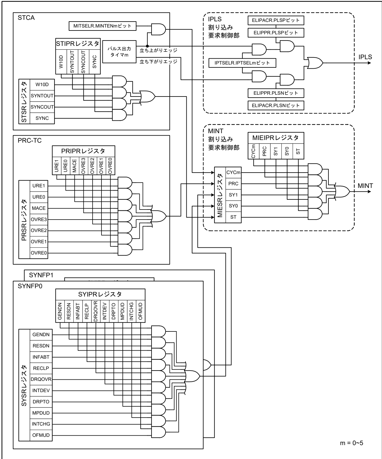
図37.36 MINT割り込み要求とIPLS割り込み要求
