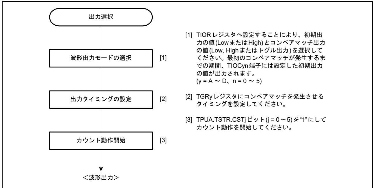
図 28.5 コンペアマッチによる波形出力動作の設定手順例
