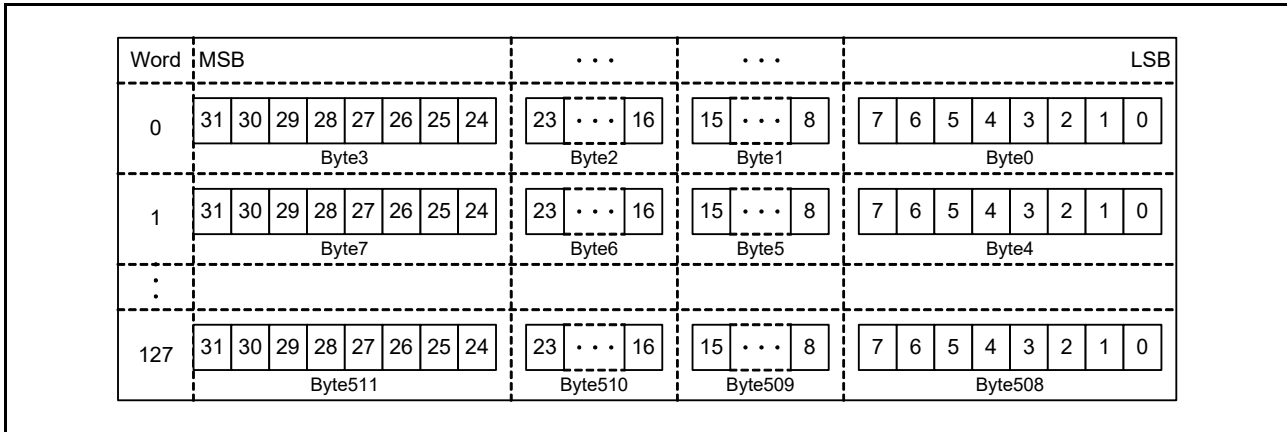
図 48.4 SDバッファのデータ構造(ダブルバッファのうちのひとつ)
