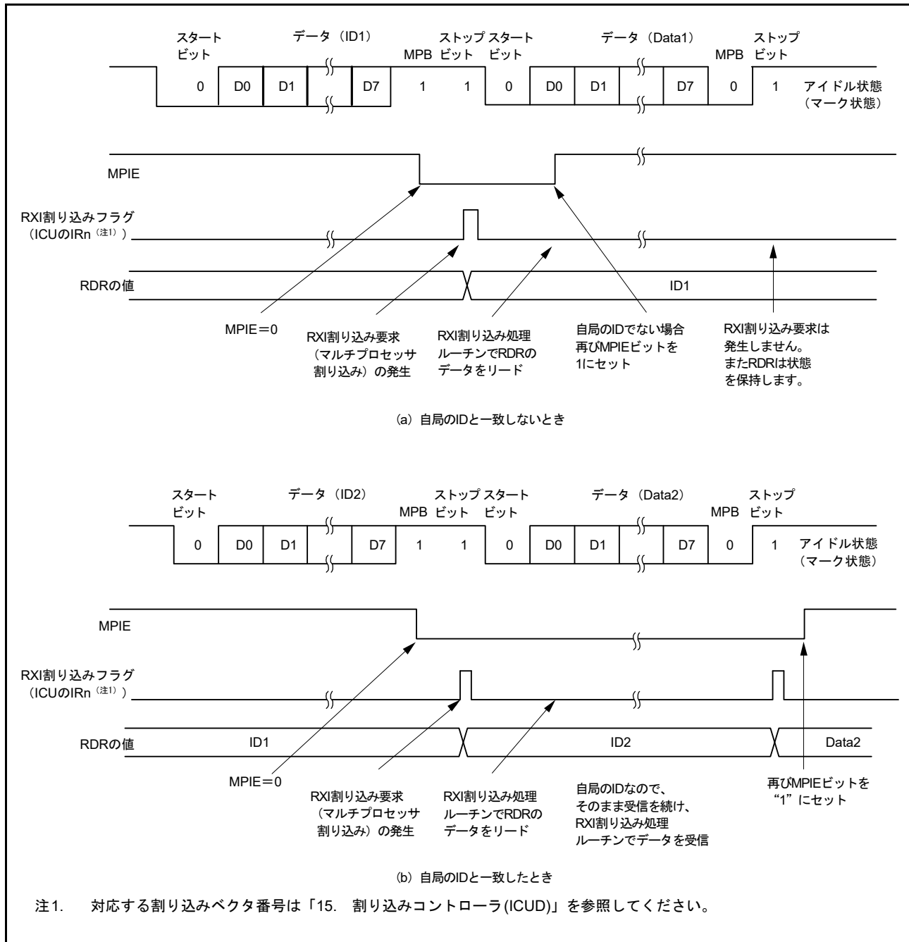
図 41.24 SCI の受信時の動作例 (8 ビットデータ / マルチプロセッサビットあり / 1 ストップビットの例)
