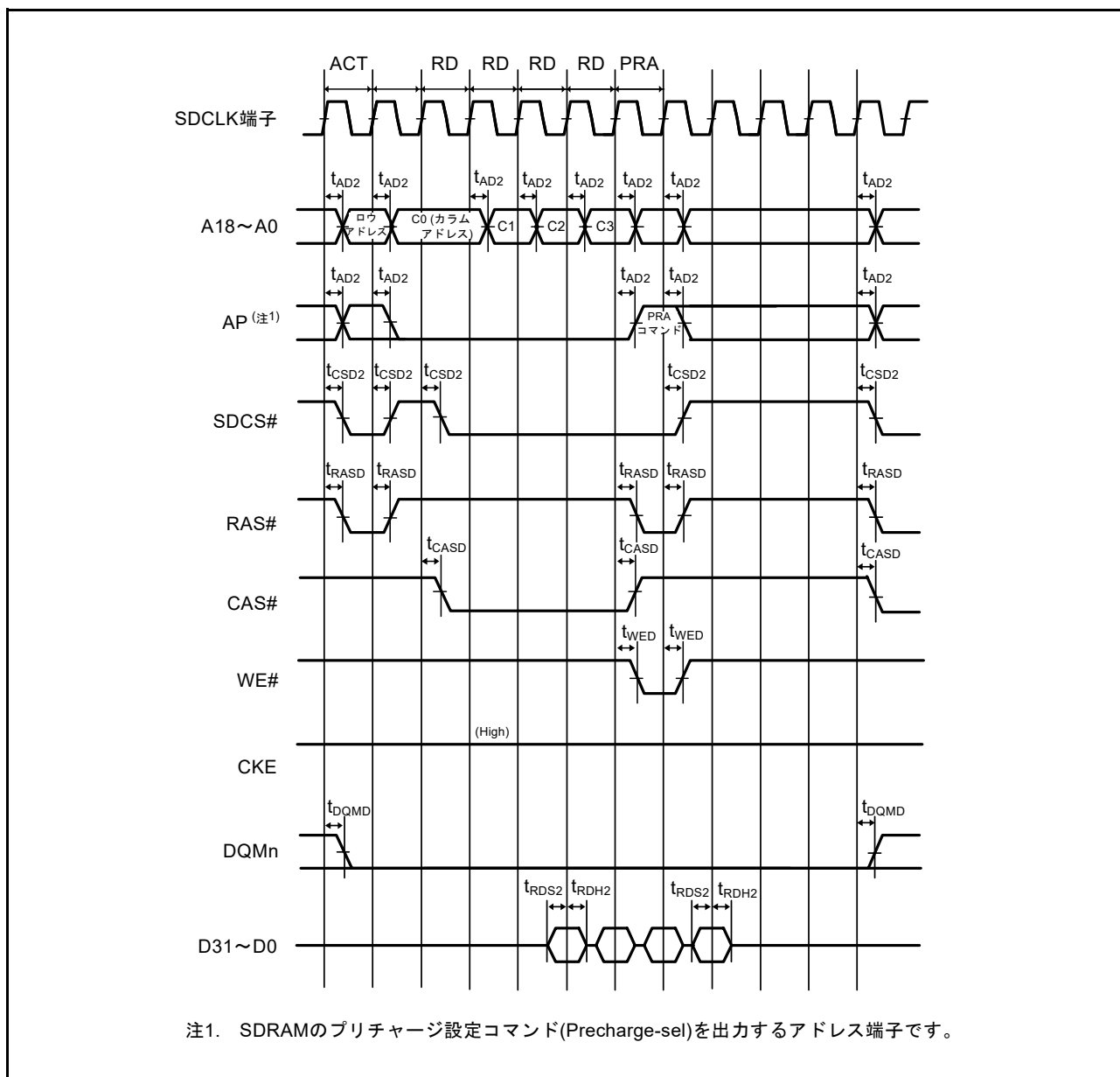
図 63.27 SDRAM 空間複数リードバスタイミング
