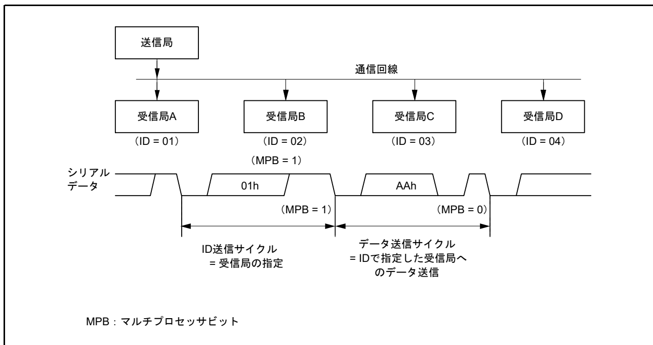
図 41.22 マルチプロセッサフォーマットを使用した通信例 (受信局 A へのデータ“AAh”の送金の例)
