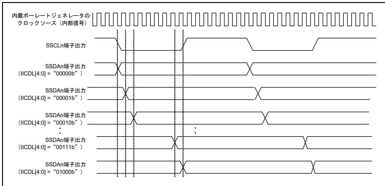
図 41.54 SSSDA 出力遅延のタイミング
