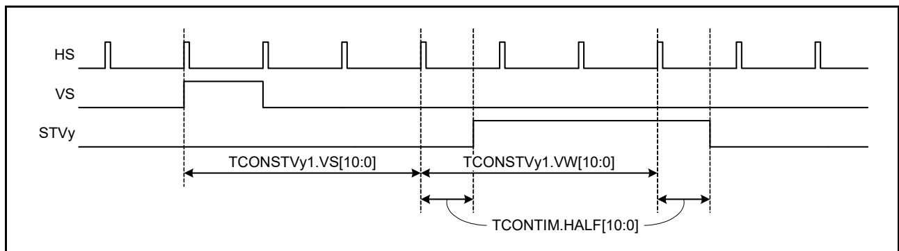
図 51.17 STVy 信号の生成 (y = A, B)
