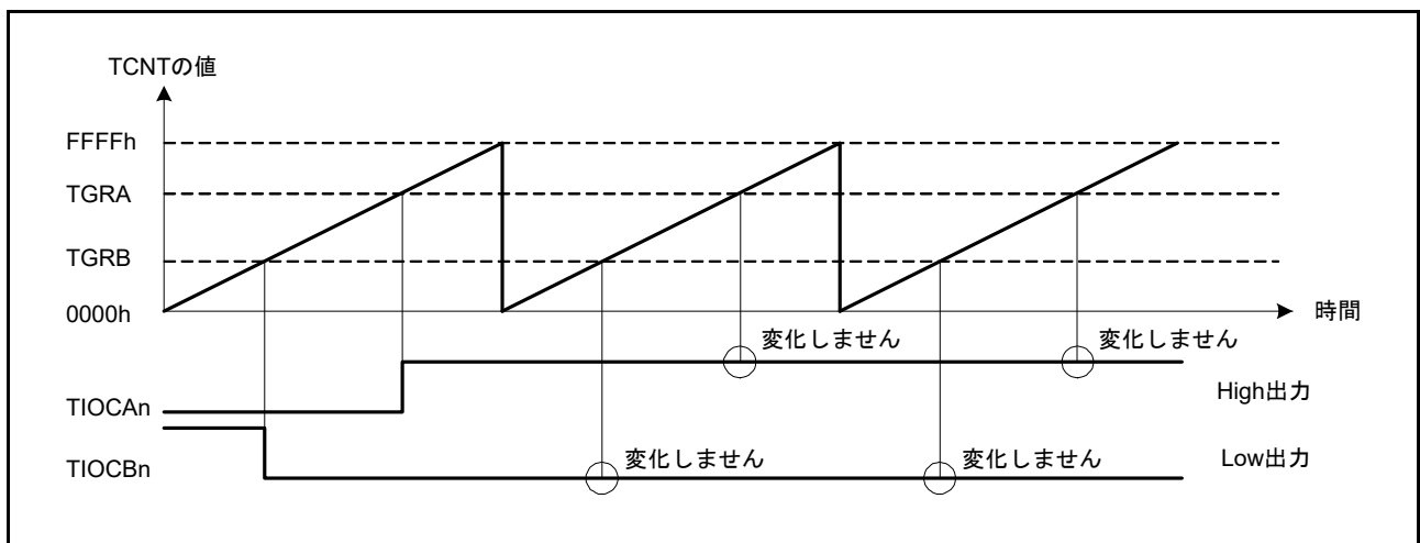
図 28.6 Low出力/High出力の動作例 (n = 0 ~ 5)
