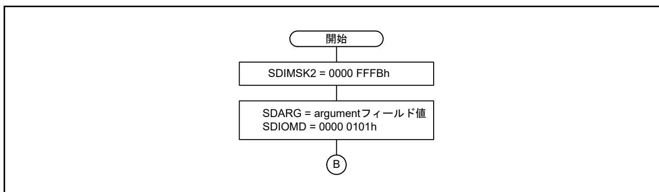
図 48.19 IO_RW_EXTENDED コマンド (CMD53) のシーケンス中に SDIO abort (CMD52) を送信する例
