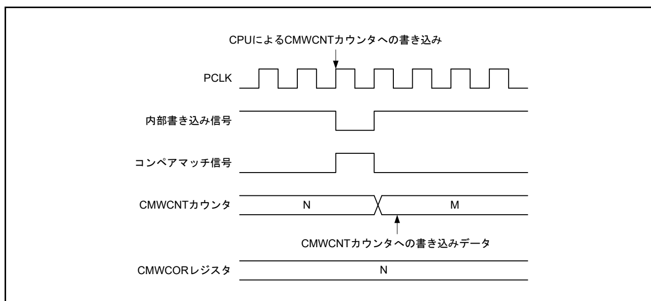
図 32.23 CMWCNT カウンタへの書き込みとコンペアマッチの競合
