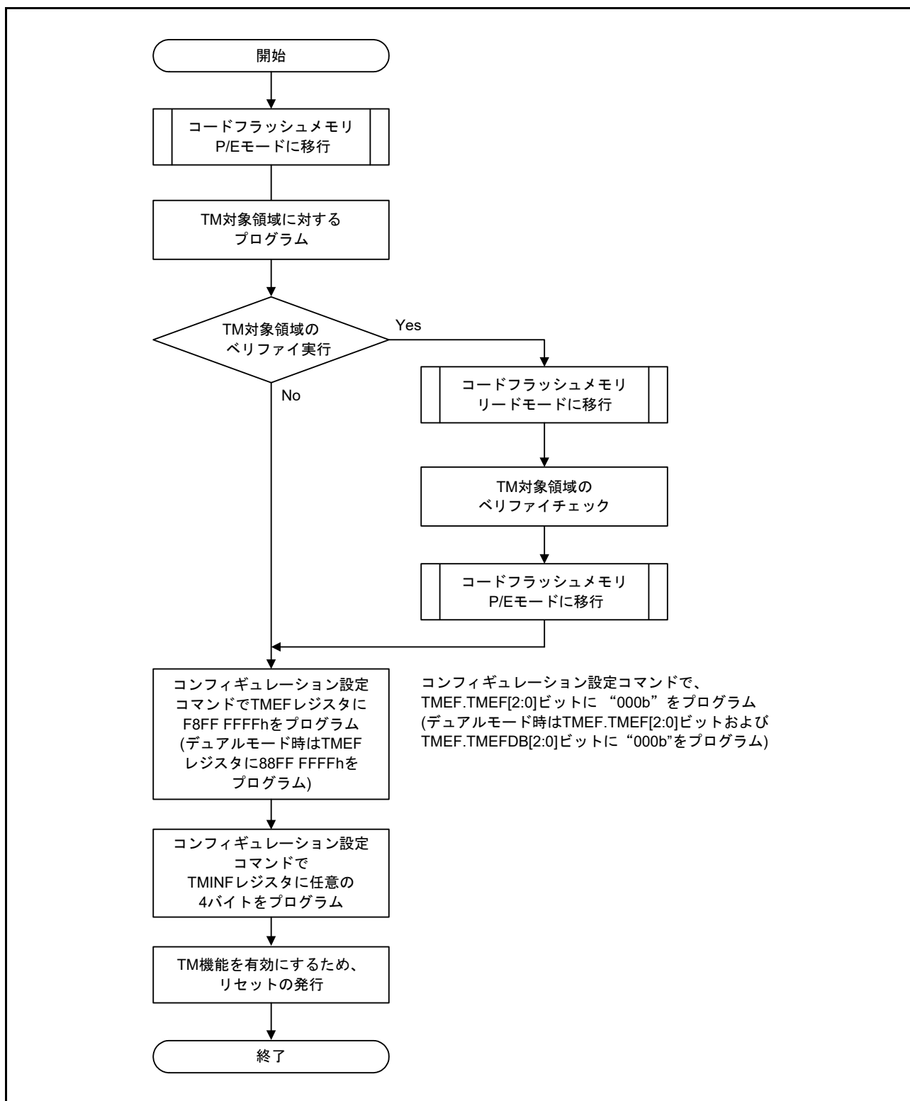
図 62.56 セルフプログラミングによる TM 機能を有効にするためのフロー
