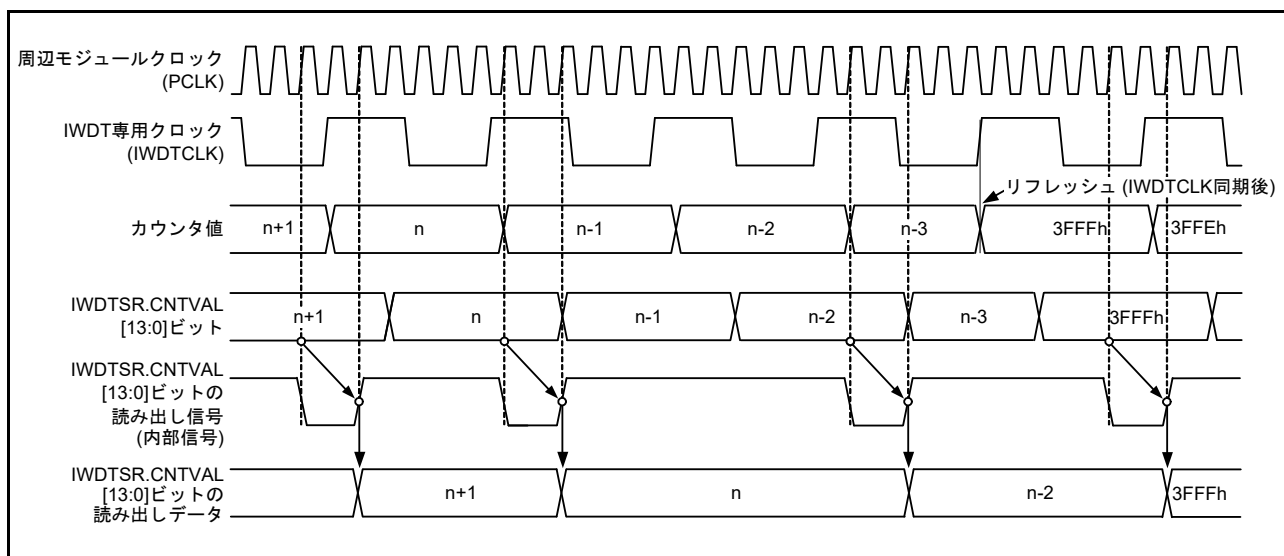
図 35.7 IWDT カウンタ値の読み出し処理 (IWDTCR.CKS[3:0] = 0000b、IWDTCR.TOPS[1:0] = 11b)
