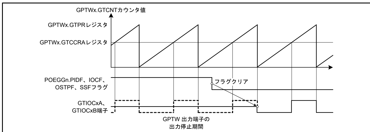
図 27.4 出力停止要求の解除による GPTW の出力端子の停止解除タイミング
