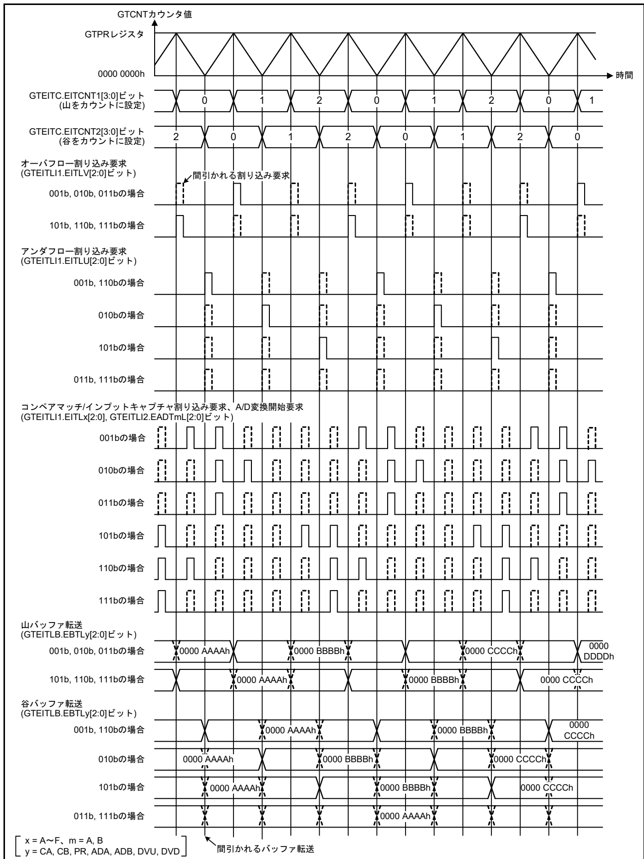
図 26.105 拡張割り込み間引き機能の動作例 (三角波、拡張割り込み間引き 1 間引き回数 2 で山をカウント、拡張割り込み間引き 2 間引き回数 2 で谷をカウント、拡張割り込み間引きカウンタ 2 初期値 “0” の場合)
