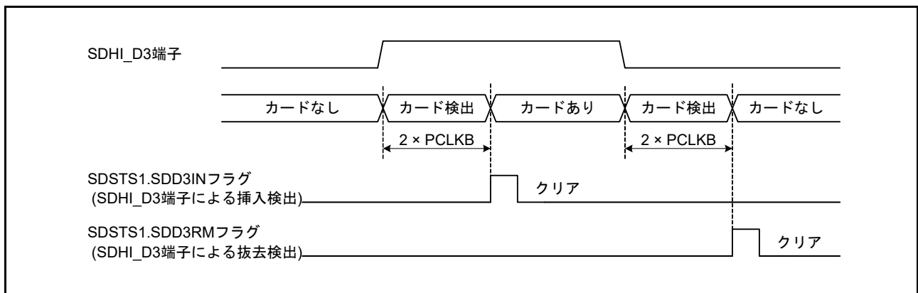
図 48.7 SDHI_D3 端子による SD カード検出
