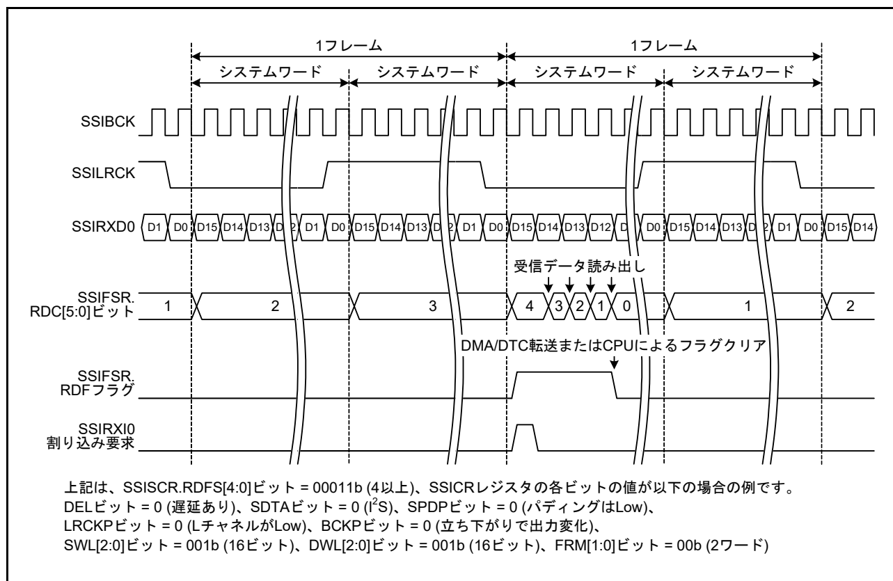
図 47.28 SSIRXIO 割り込みのタイミング図
