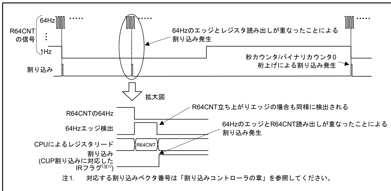
図 33.12 桁上げ割り込み (CUP) のタイミングチャート
