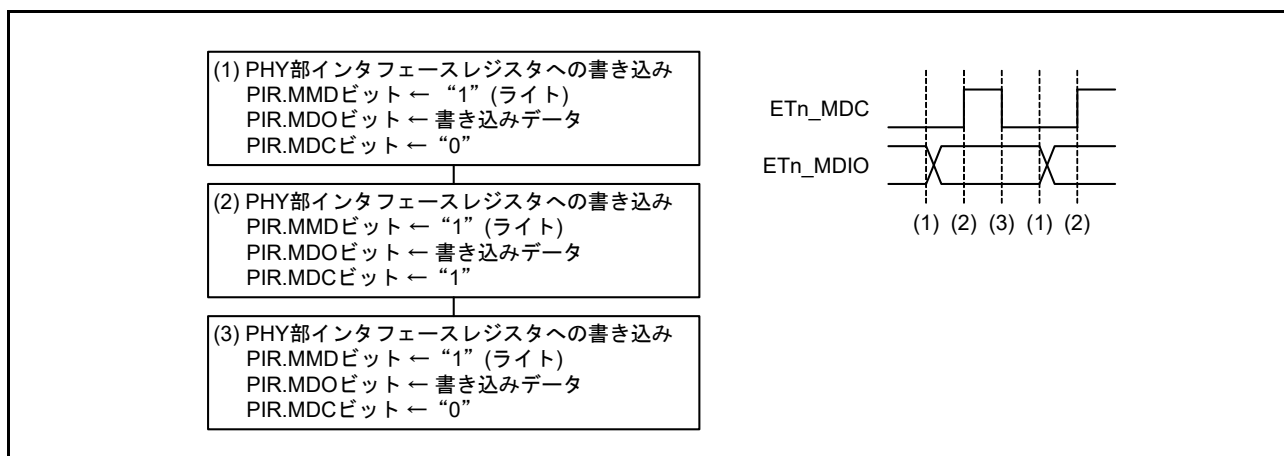
図 36.14 1 ビットデータのライトフロー
