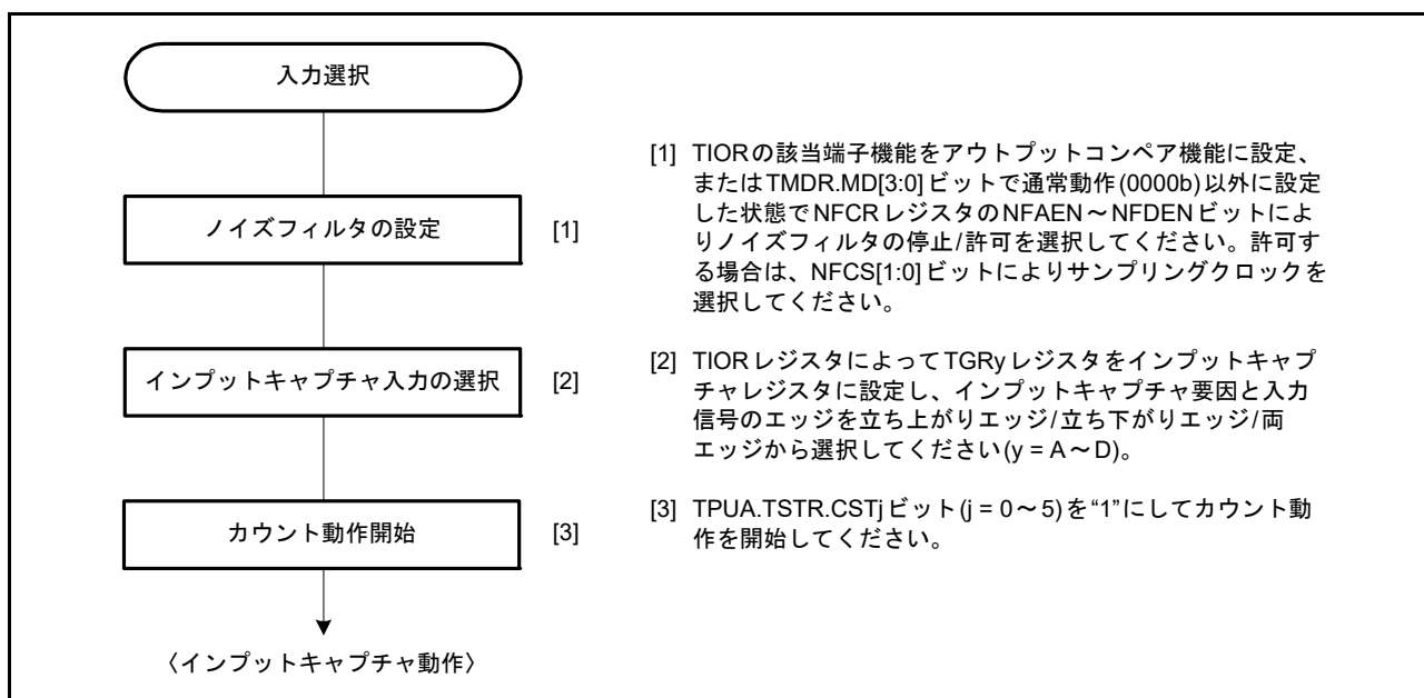
図 28.8 インพุットキャプチャ動作の設定手順例
