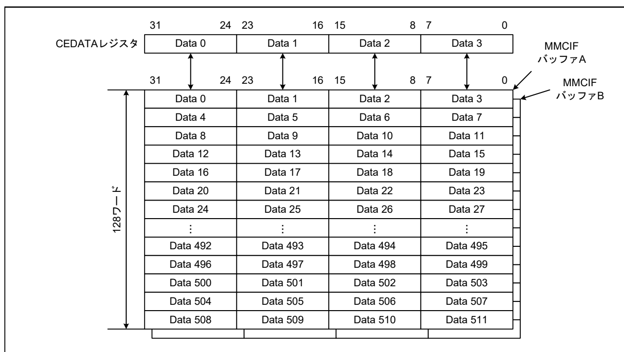
図 49.6 MMCIF バッファの構成 (32 ビットアクセス)
