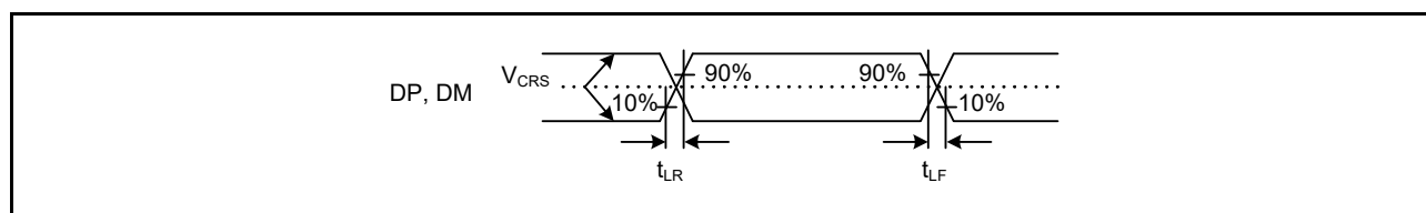
図 63.98 DP, DM 出力タイミング (ロースピード時)
