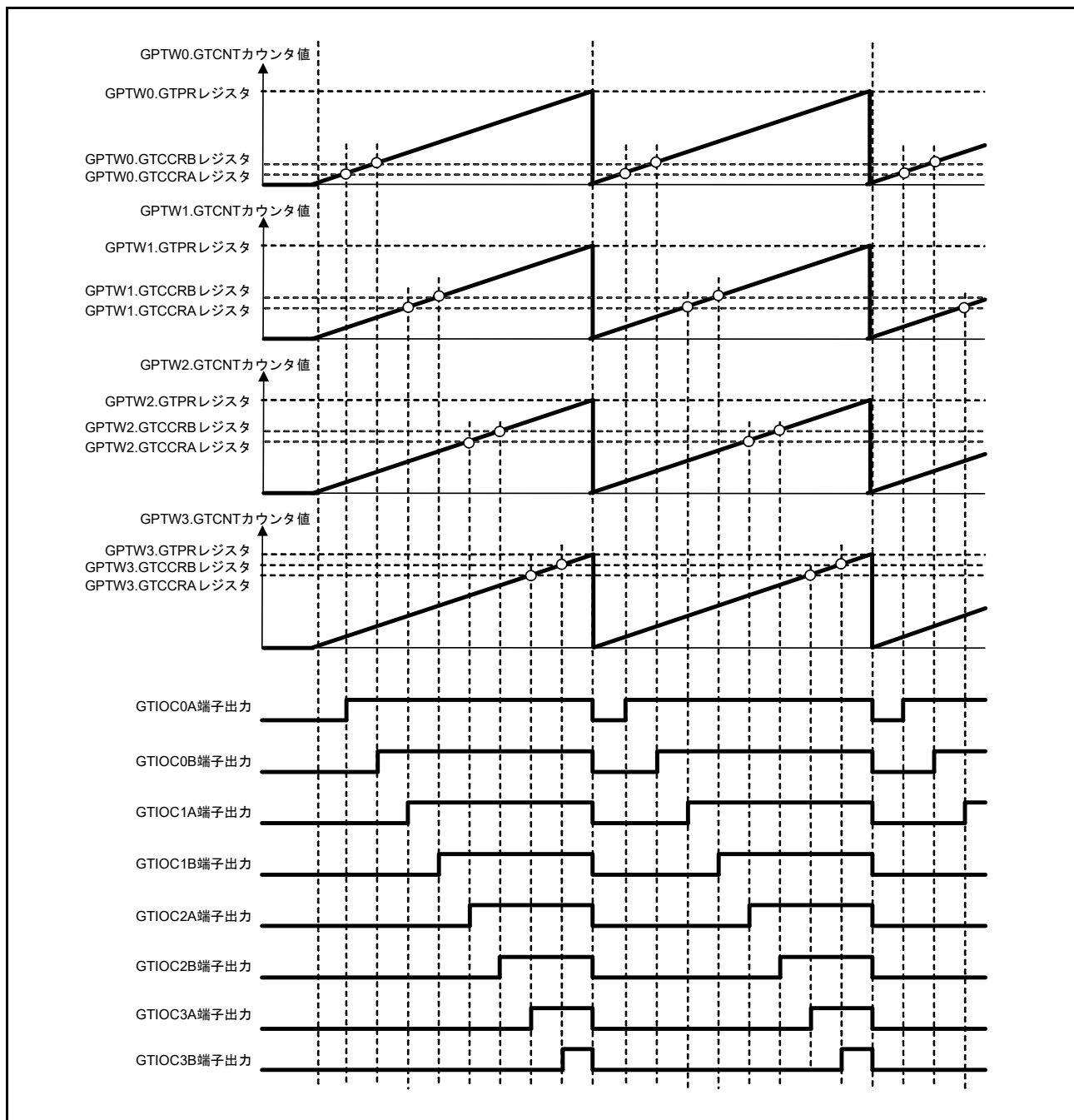
図 26.81 同期PWM出力例
