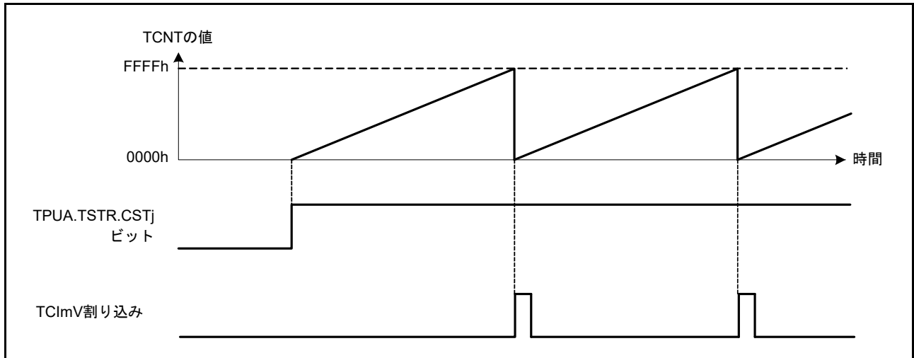
図 28.3 フリーランカウンタの動作
