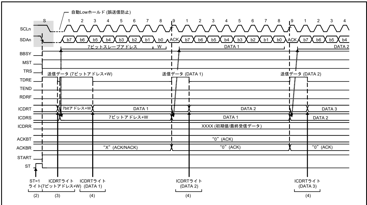
図 42.6 マスタ送信の動作タイミング (1) (7ビットアドレスフォーマットのとき)
