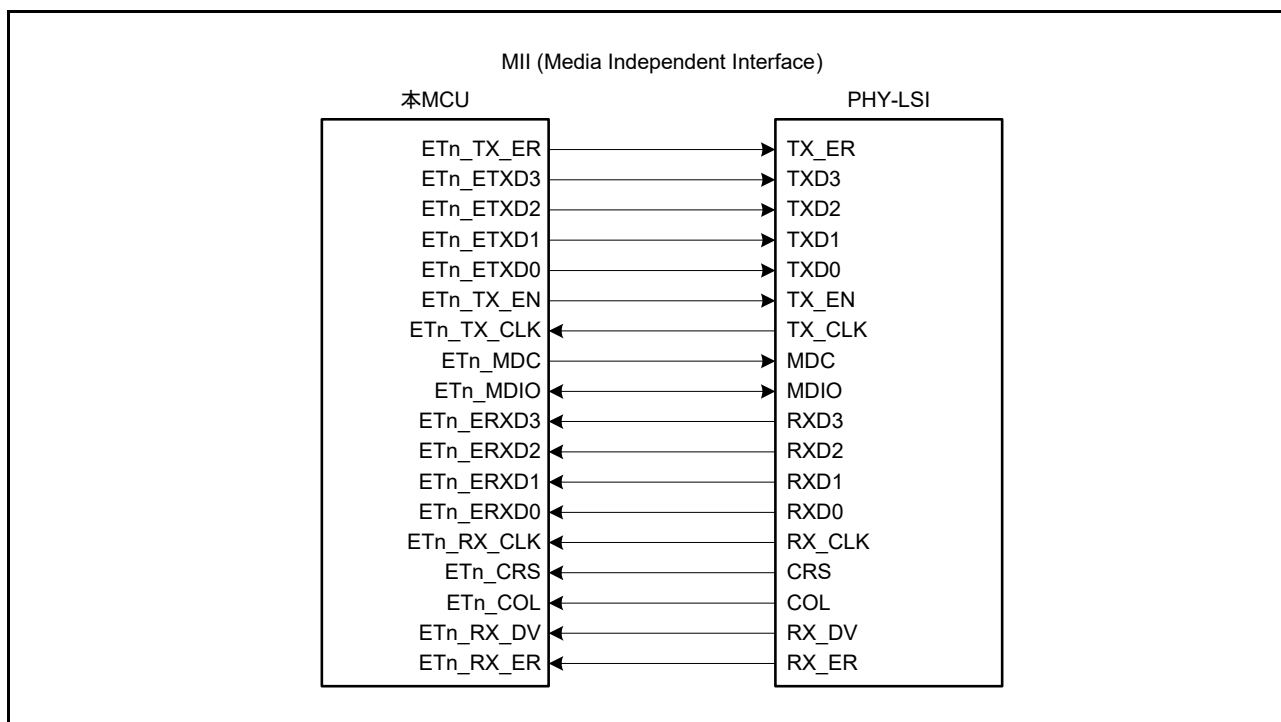
図 36.2 PHY-LSI との接続例 (MII)
