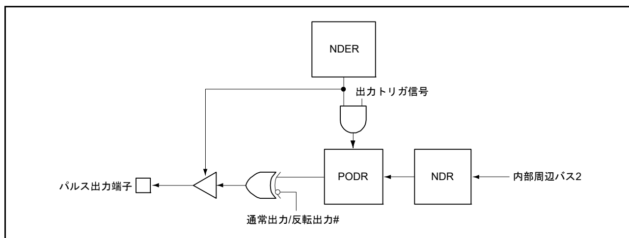
図 29.4 PPG 概要図
