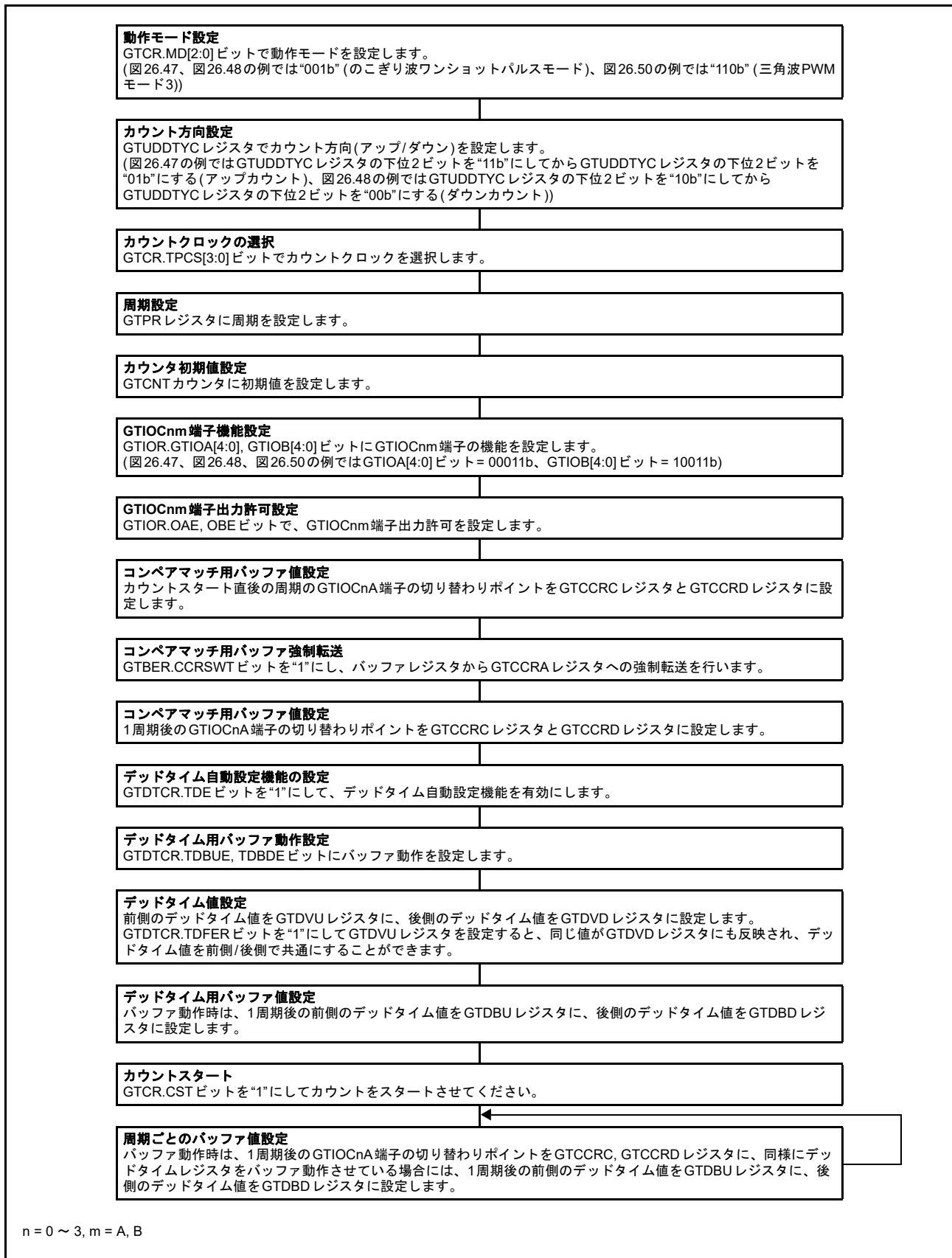
図 26.51 デッドタイム自動設定機能の設定例 (のこぎり波ワンショットパルスモード、三角波 PWM モード 3 時)
