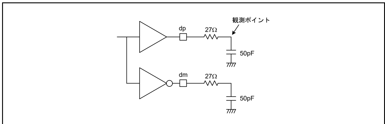
図 63.101 測定回路 (フルスピード時)
