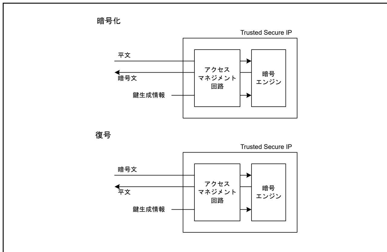
図 55.3 暗号エンジン概念図
