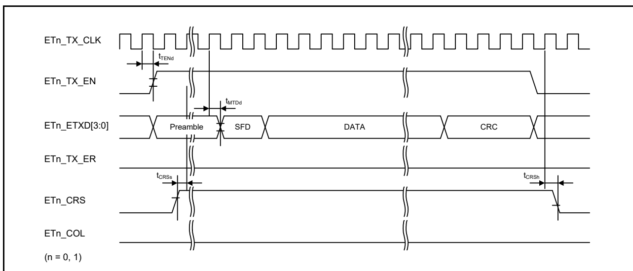
図 63.86 MII 送信タイミング (正常動作時)
