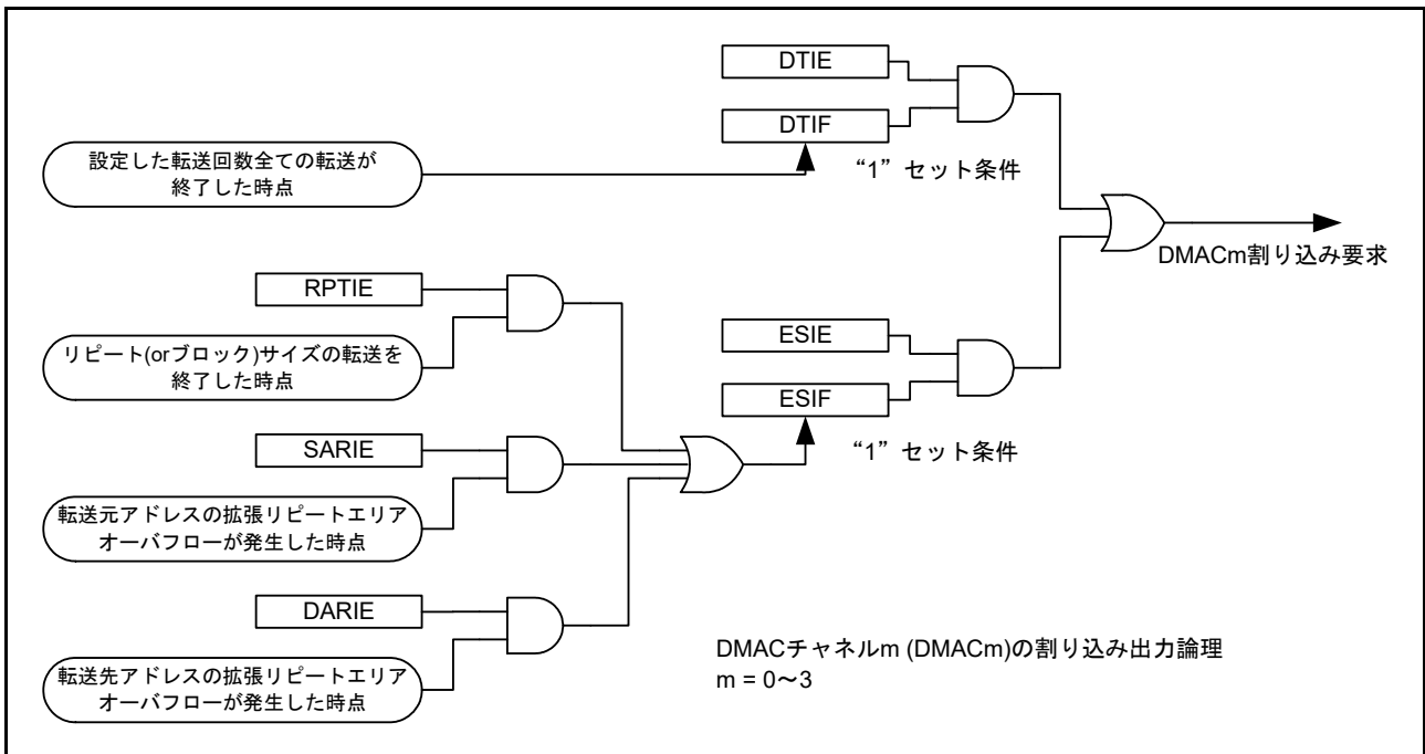
図 18.13 割り込み出力の概略論理図 (DMAC0 ~ DMAC3)
