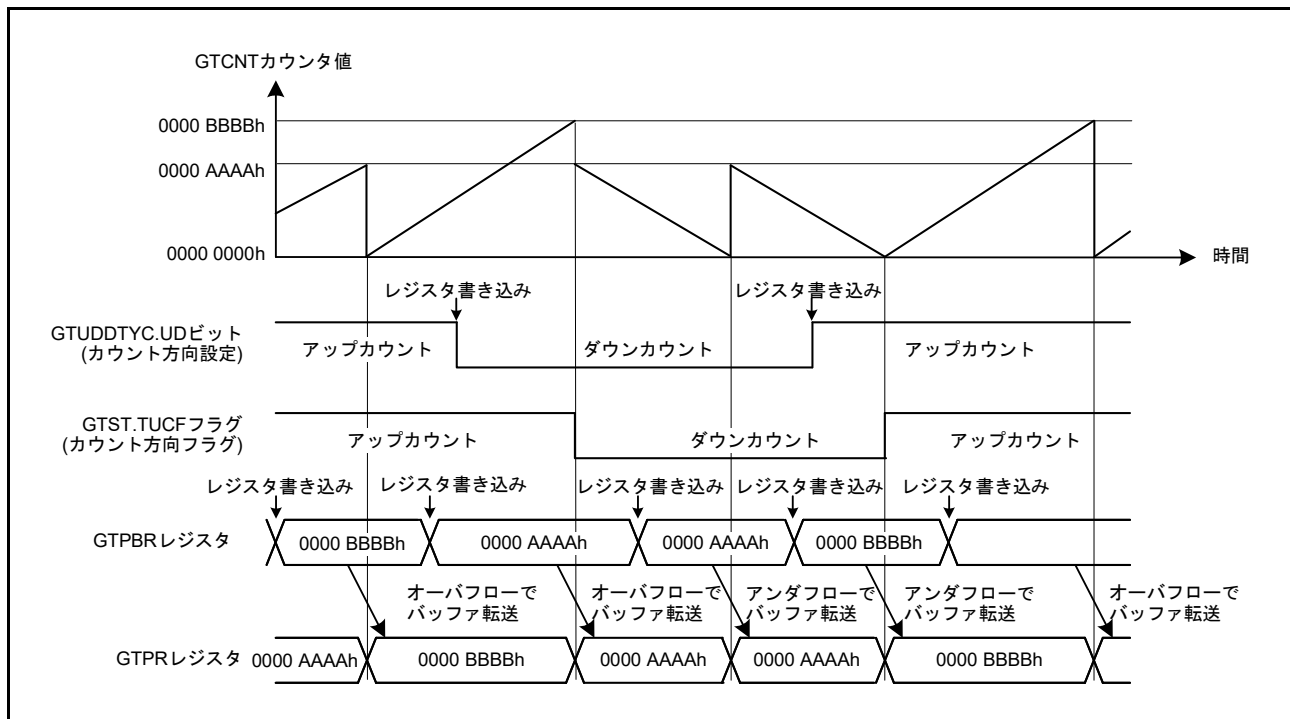
図 26.53 カウント方向切り替え機能の動作例 (バッファ動作時)
