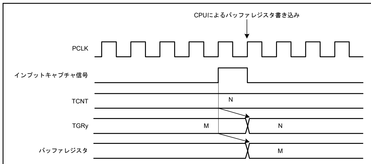
図 28.50 バッファレジスタへの書き込みと入力キャプチャの競合
