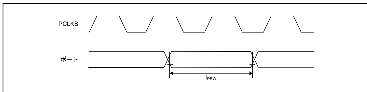
図 63.35 I/Oポート入力タイミング
