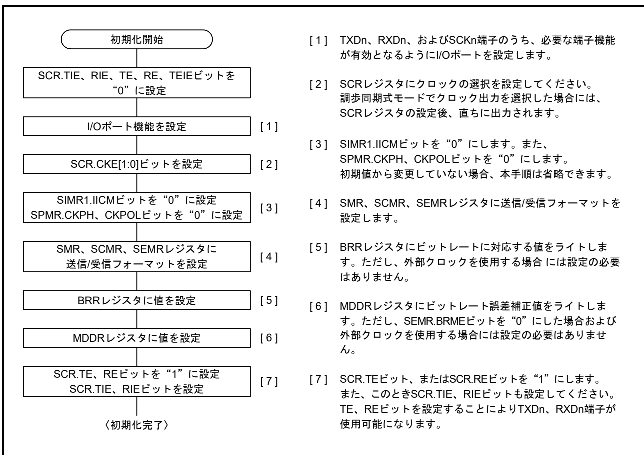
図 41.11 SCIの初期化フローチャートの例 (調歩同期式モード) (SCI0 ~ SCI6, SCI12)
