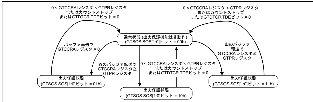
図 26.126 出力保護機能
