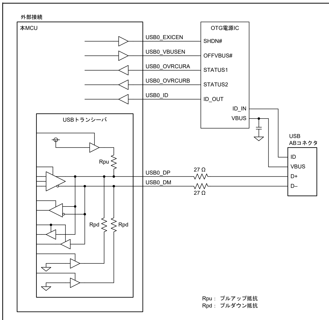
図 40.2 セルフパワー時の OTG デバイスと USB コネクタとの接続例
