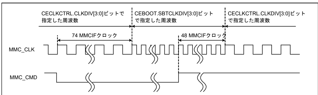
図 49.10 Boot Operation 時の MMCIF クロック周波数切り替え
