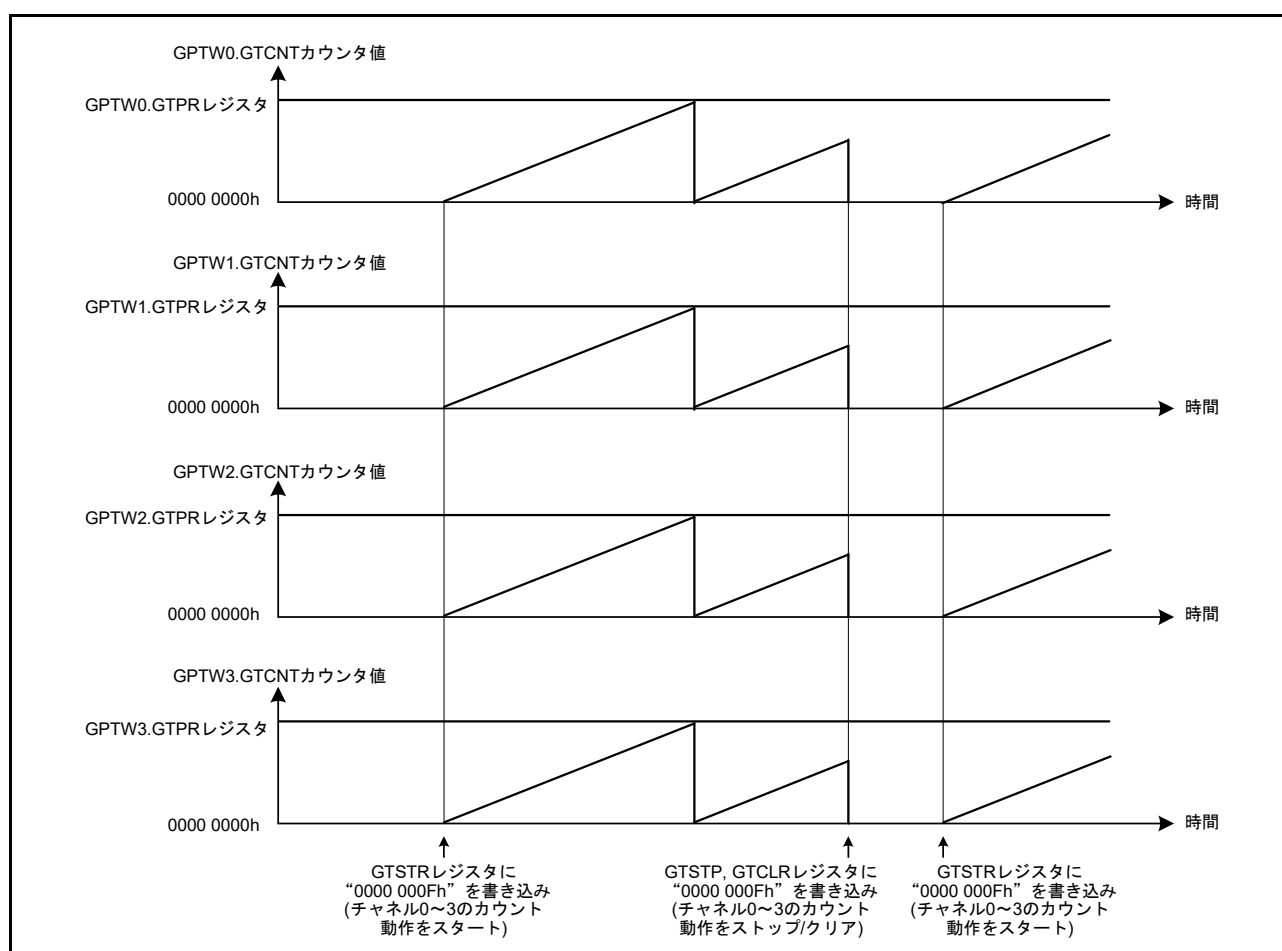
図 26.77 ソフトウェアによる同時スタート/ストップ/クリア動作例 (カウント周期(GTPRレジスタ値)が同一のとき)
