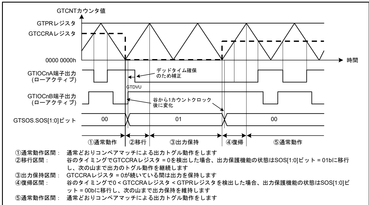
図 26.127 谷のバッファ転送で GTCRA レジスタが “0000 0000h” である場合の出力保護機能の動作例 (谷のバッファ転送で 0 < GTCRA レジスタ < GTPR レジスタに復帰、アクティブレベルは Low の場合) (n = 0 ~ 3)
