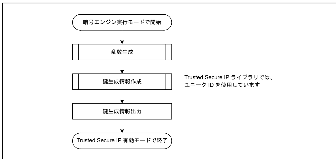
図 55.9 鍵生成情報作成フロー (乱数使用)
