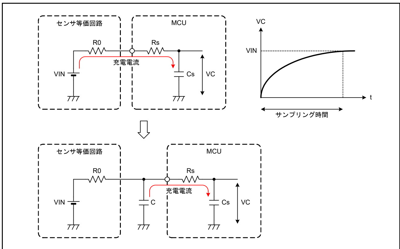
図 56.45 アナログ入力端子と外部センサの等価回路
