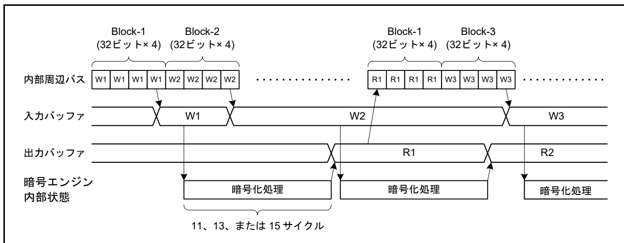
図 55.6 AES 暗号 / 復号処理タイミング図
