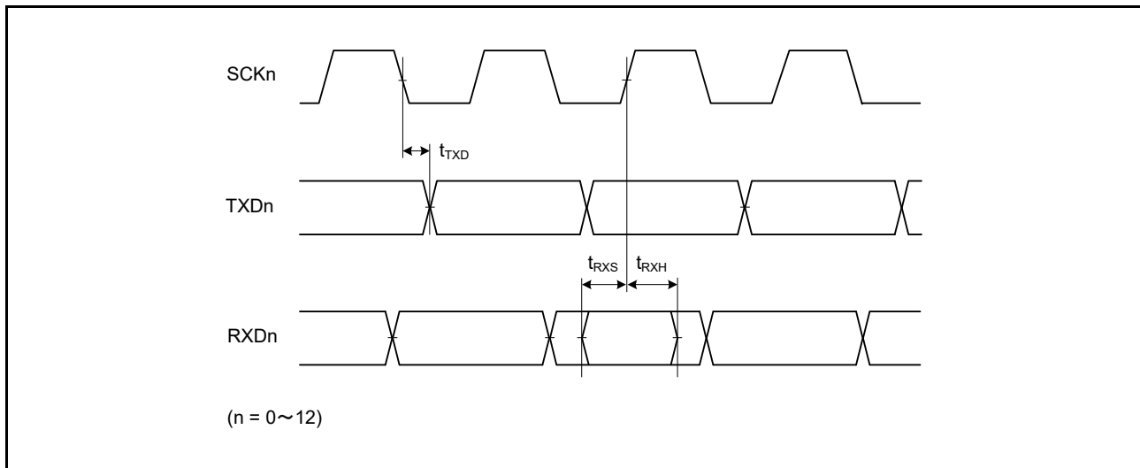
図 63.55 SCI 入出力タイミング/クロック同期式モード
