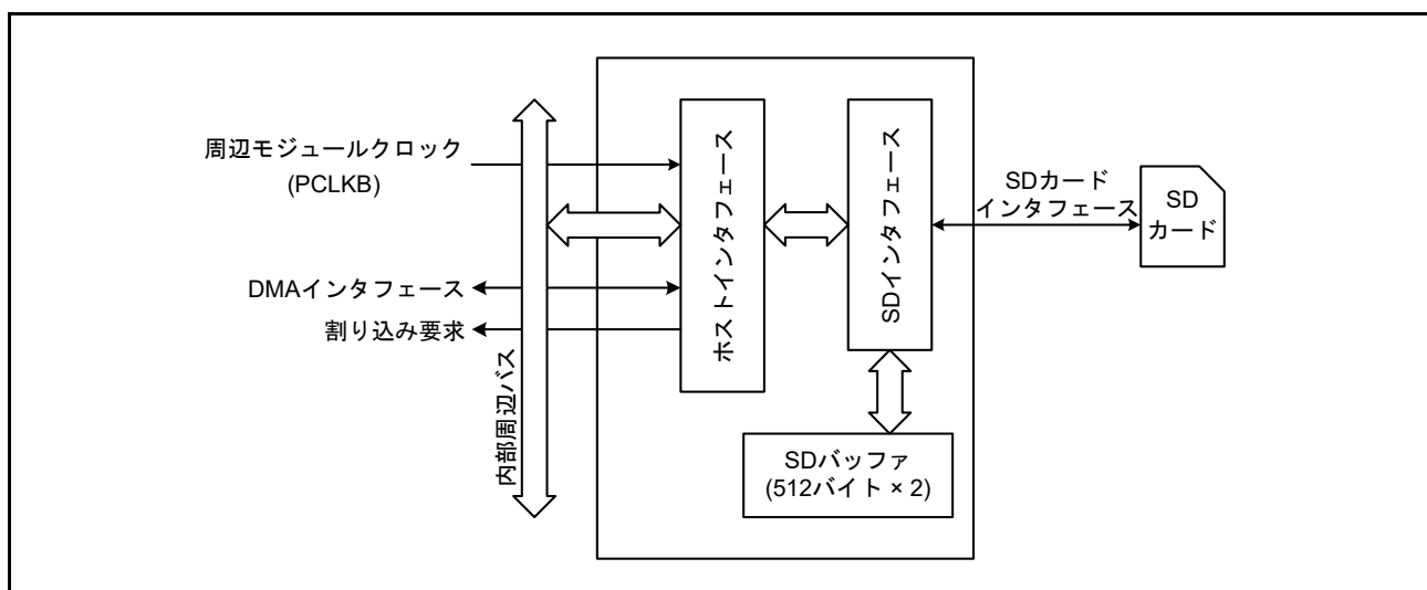
図 48.1 SDHIのブロック図
