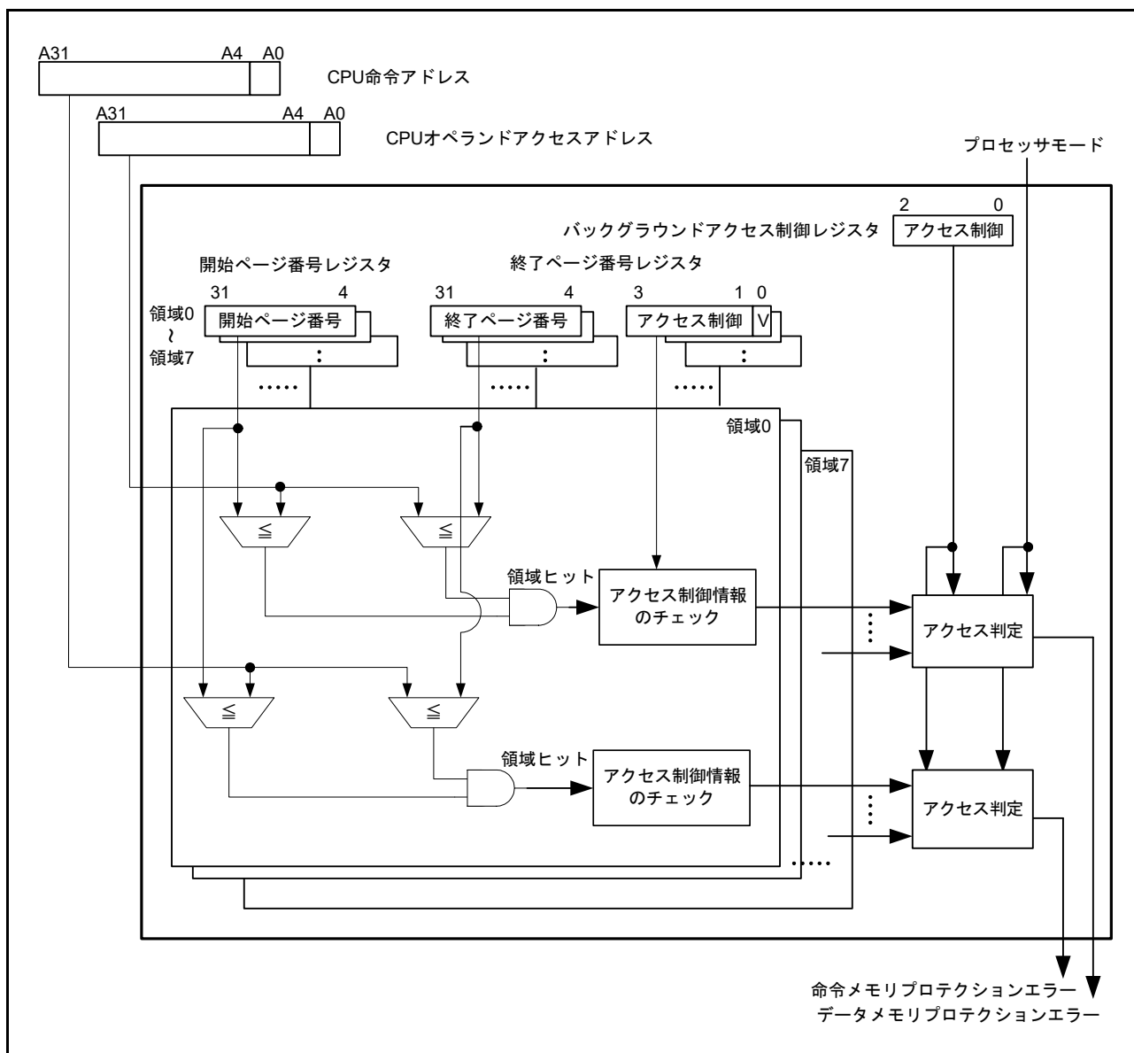
図 17.1 メモリプロテクションユニットブロック図
