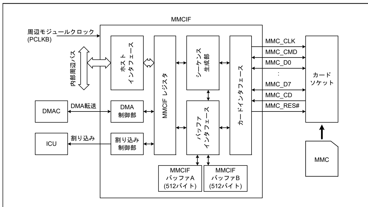
図 49.1 MMCIF のブロック図
