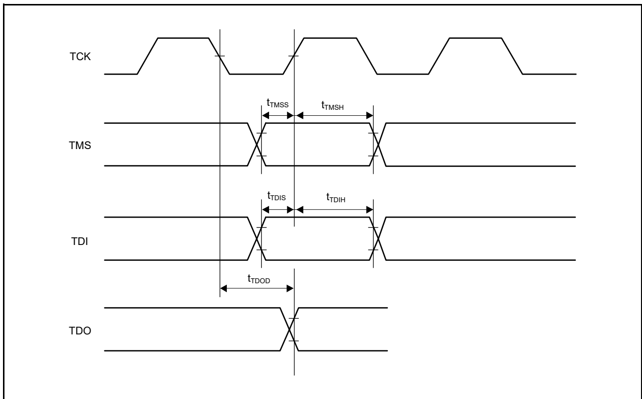
図 63.111 バウンダリスキャン入出力タイミング
