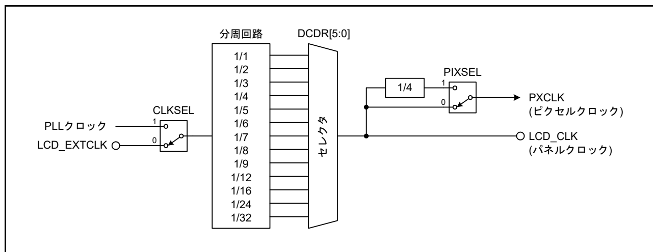
図 51.19 クロック生成部の構成
