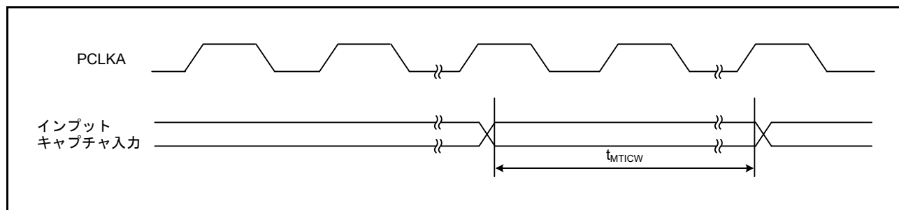
図 63.40 MTU インプットキャプチャ入力タイミング
