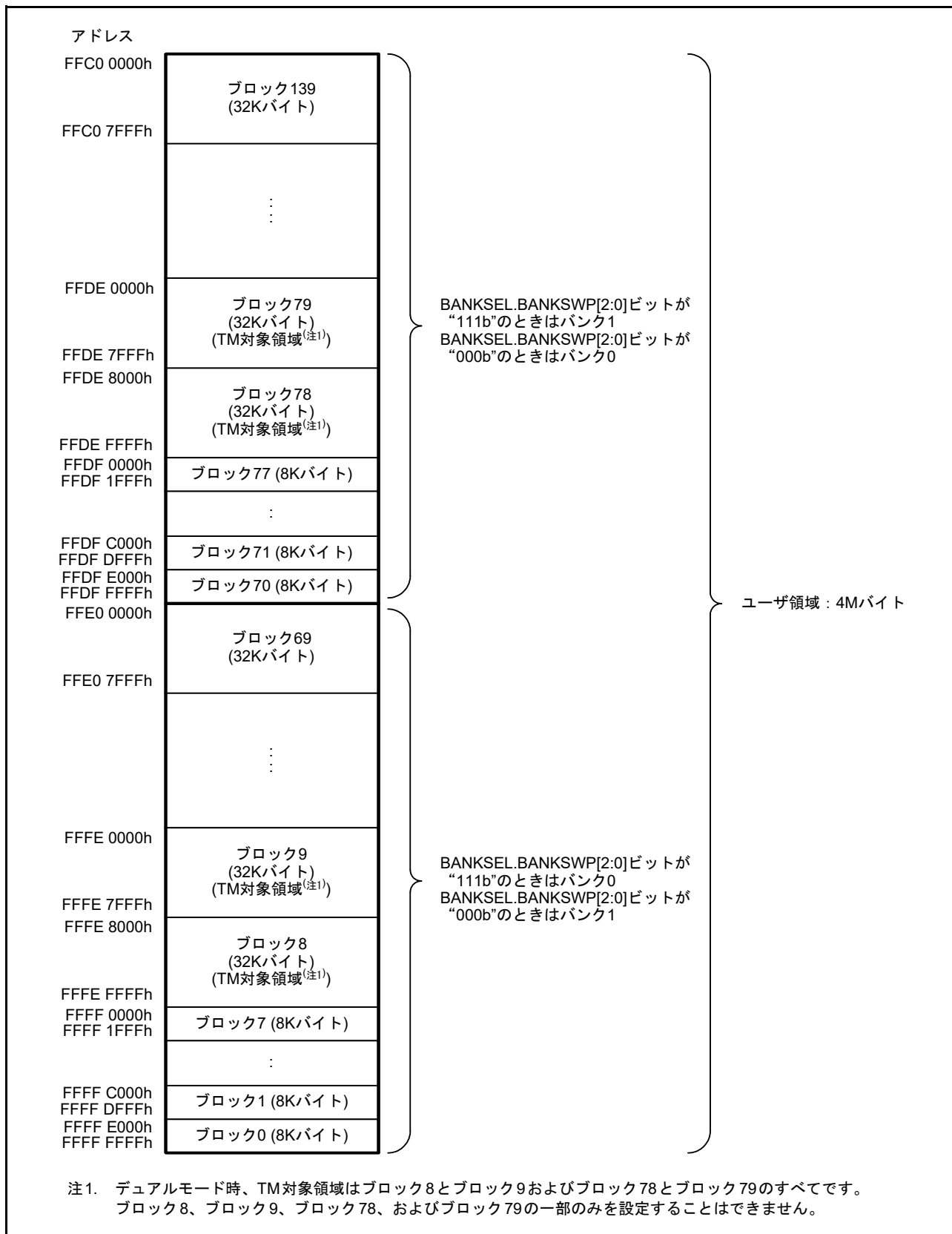
図 62.3 デュアルモード時のコードフラッシュメモリマッピング (コードフラッシュメモリ容量が4Mバイトの製品)
