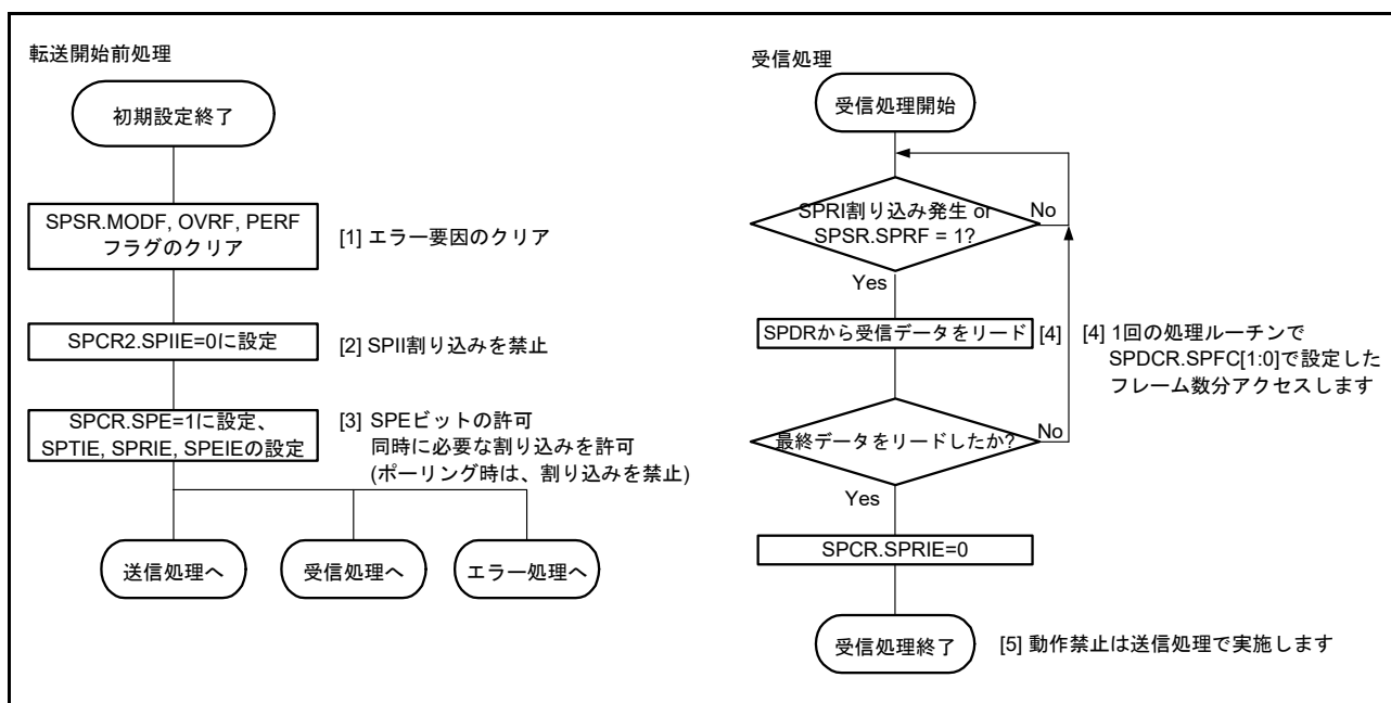
図 44.39 マスタモード時のフローチャート (受信)
