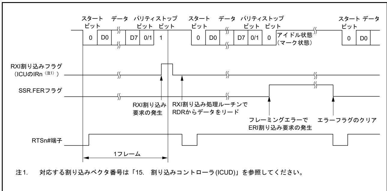
図 41.19 調歩同期式モードのシリアル受信時の動作例 (2) (RTS 機能使用時) (8 ビットデータ / パリティあり / 1 ストップビットの例)
