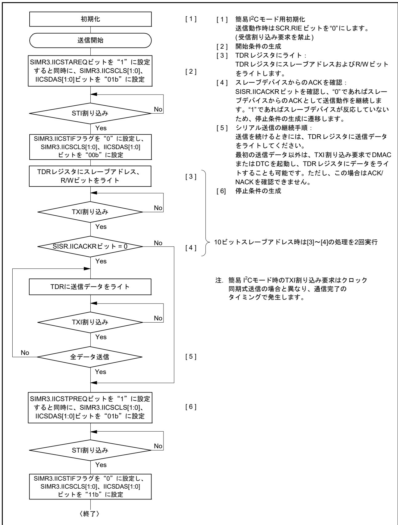
図 41.58 簡易 I 2 C モードのマスタ送信動作のフローチャート例 (送信割り込み、受信割り込み使用時)
