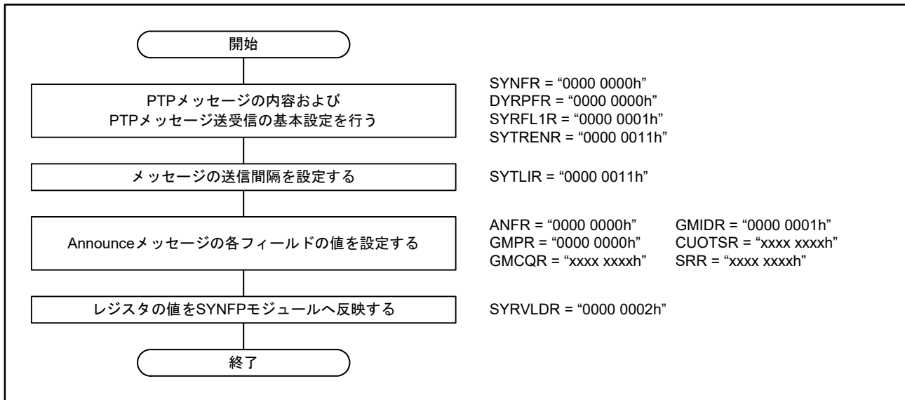
図37.10 E2Eマスタ動作の開始手順
