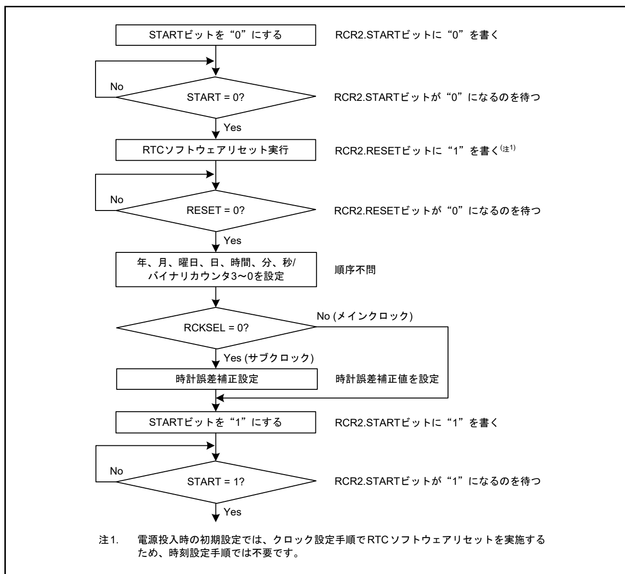
図 33.4 時刻設定手順
