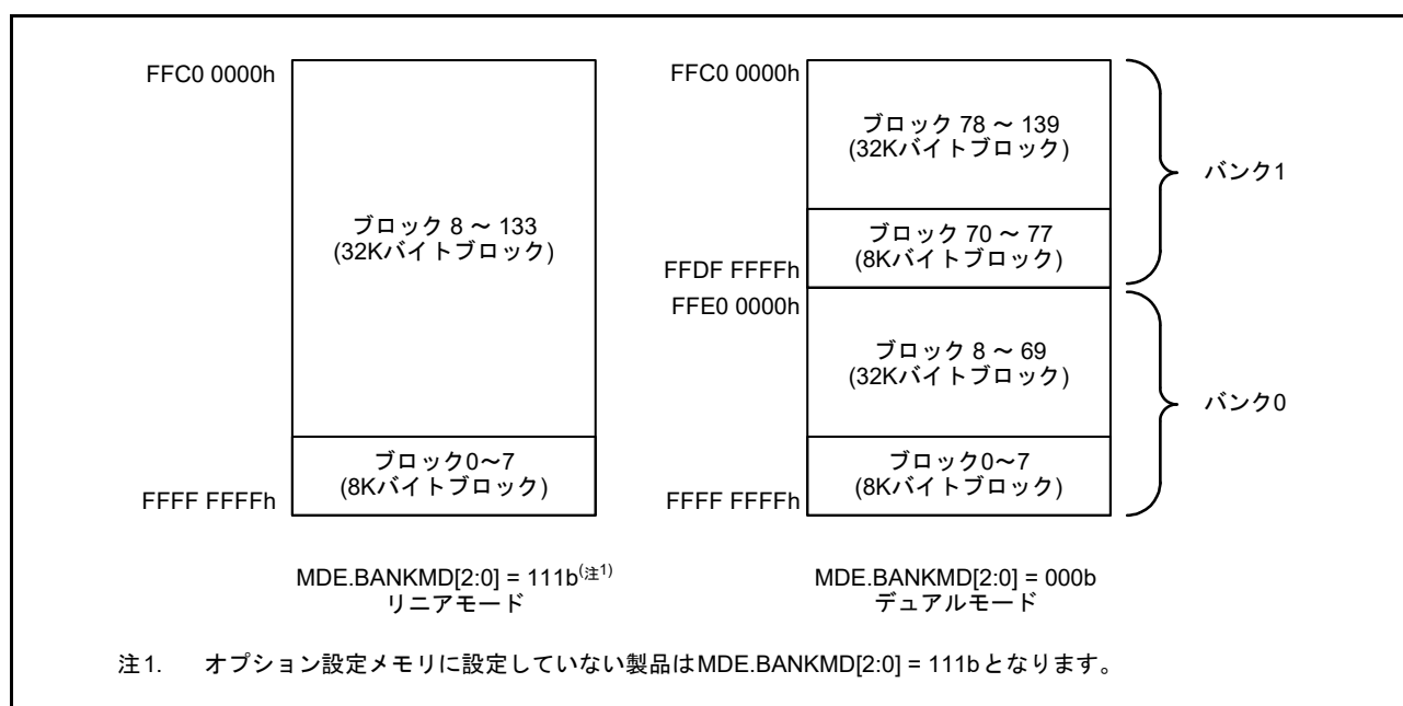
図 62.31 バンクモード切り替え例 (コードフラッシュメモリ容量が4Mバイトの製品の例)
