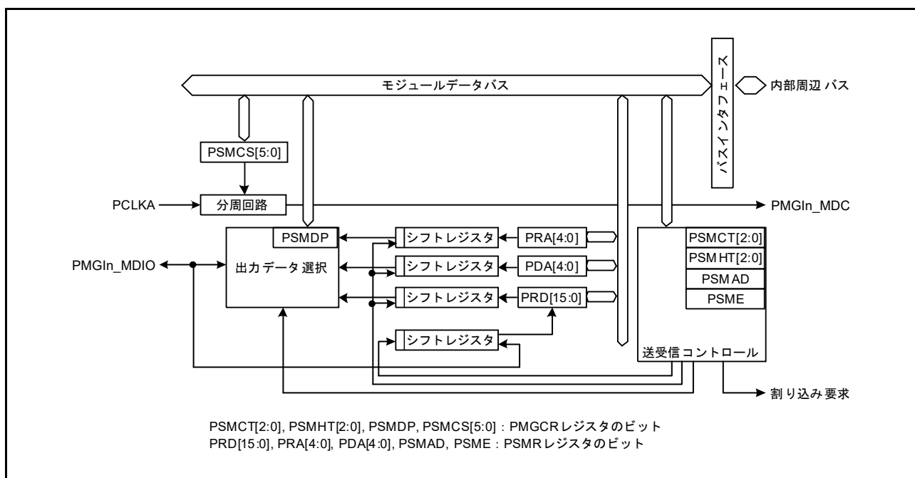
図 39.1 PMGI のブロック図 (n = 0, 1)
