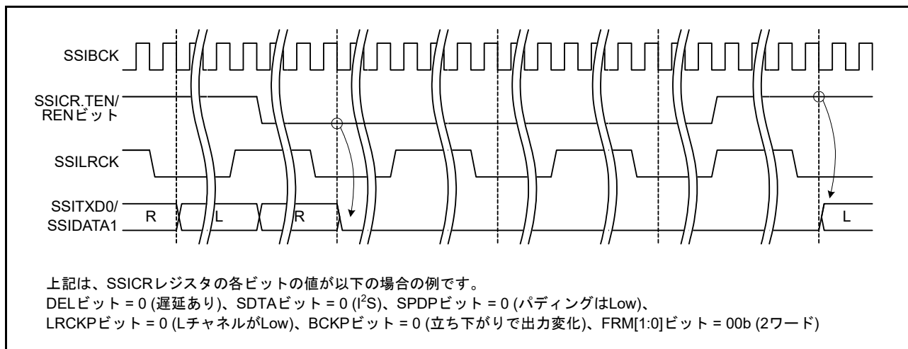
図 47.18 LRCK 連続出力機能の動作例
