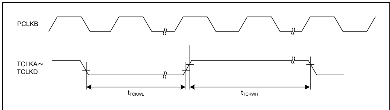
図 63.37 TPU クロック入力タイミング
