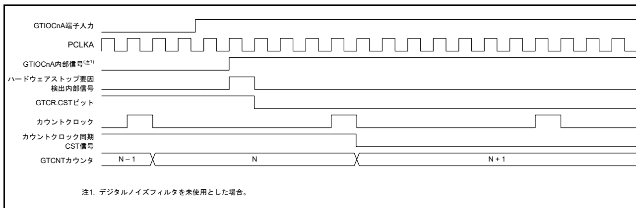
図 26.65 GTIOCnA 端子入力の立ち上がりによるカウントストップ動作タイミング例
