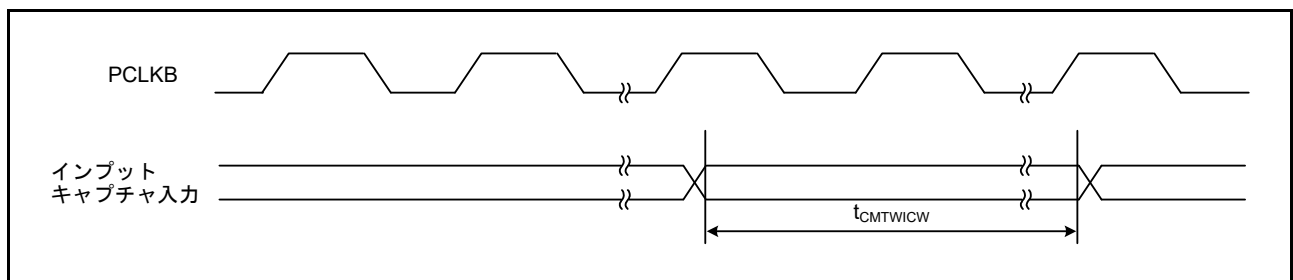
図 63.39 CMTW インプットキャプチャ入力タイミング
