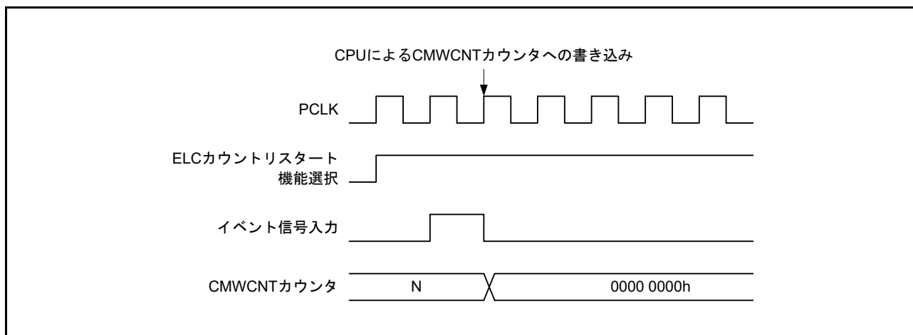
図 32.22 カウントリスタート動作でのイベント受け付けとレジスタアクセスの競合
