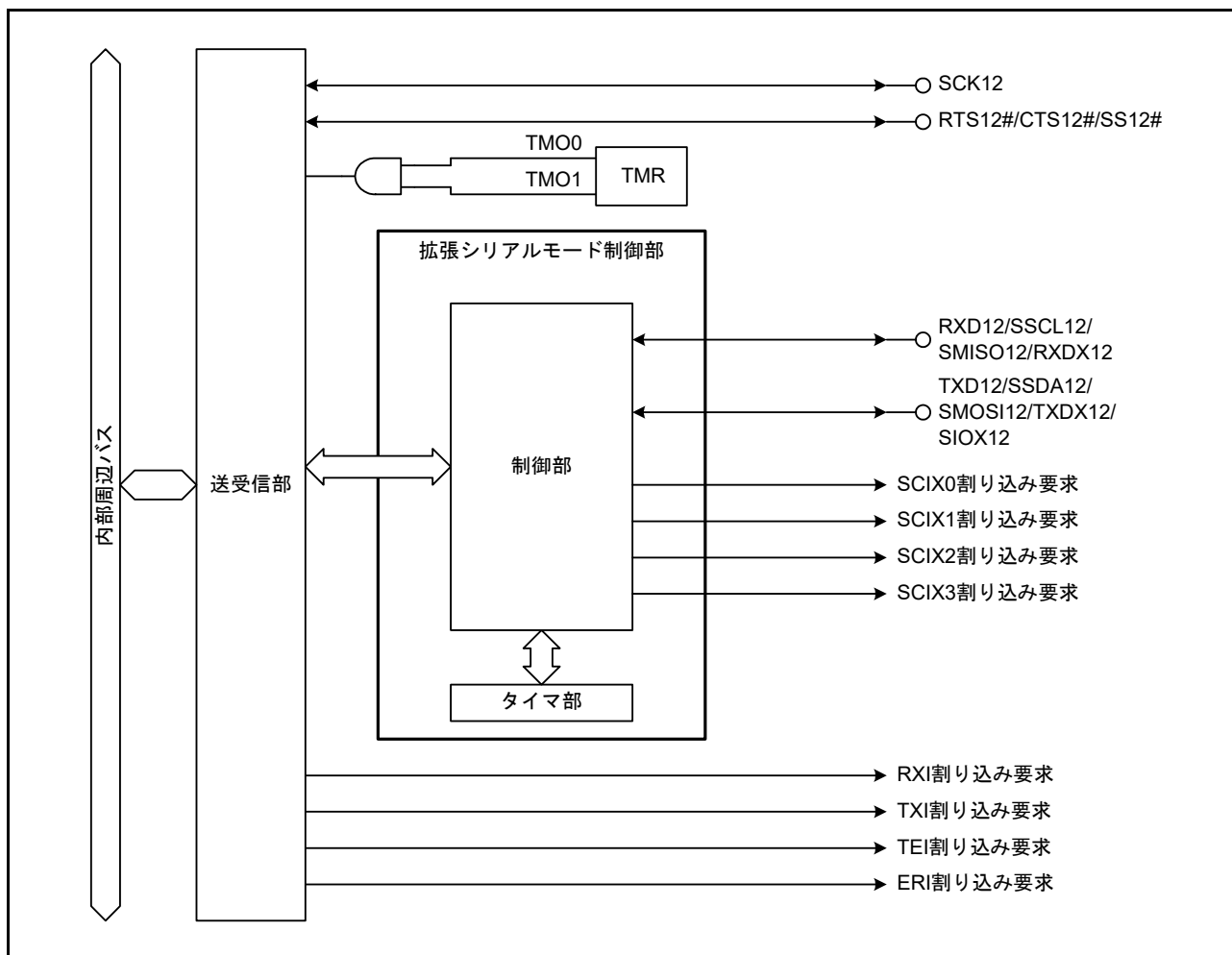
図 41.4 SClh (SCI12) のブロック図
