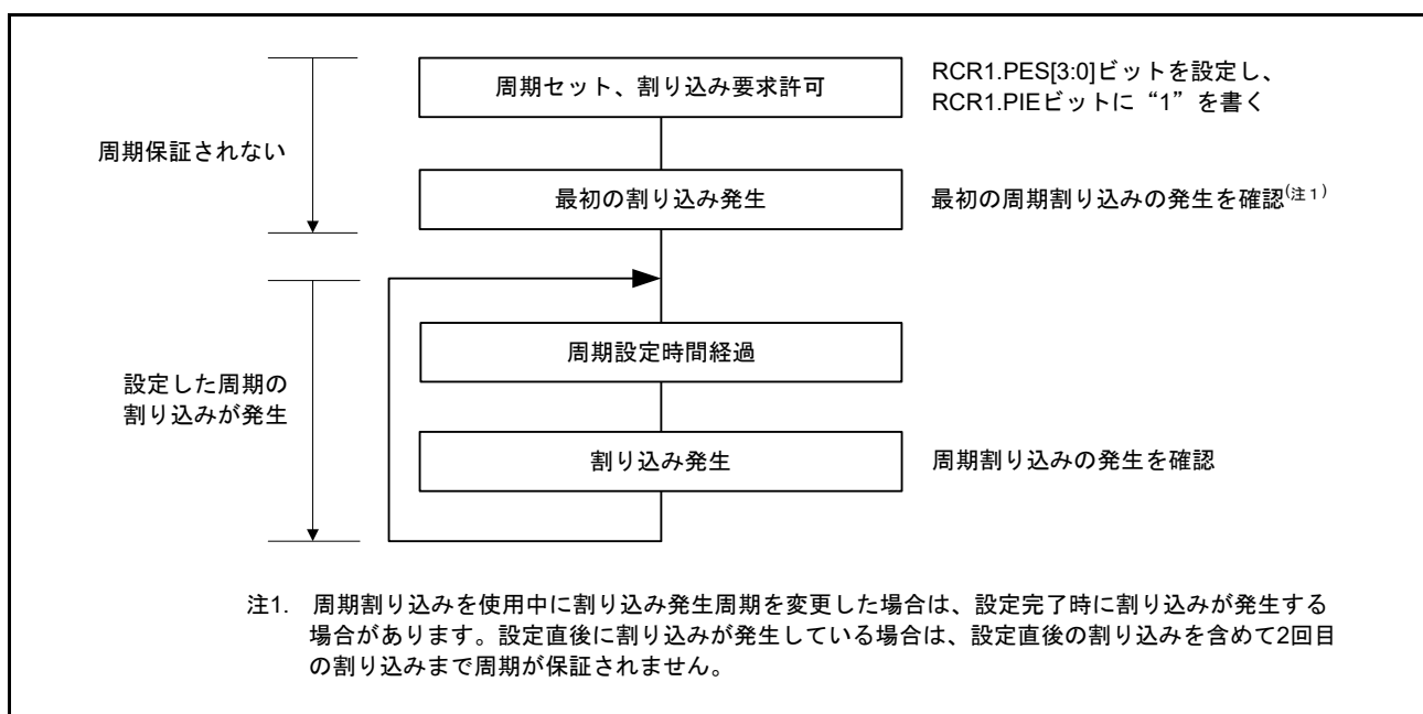
図 33.13 周期割り込み機能の使用方法
