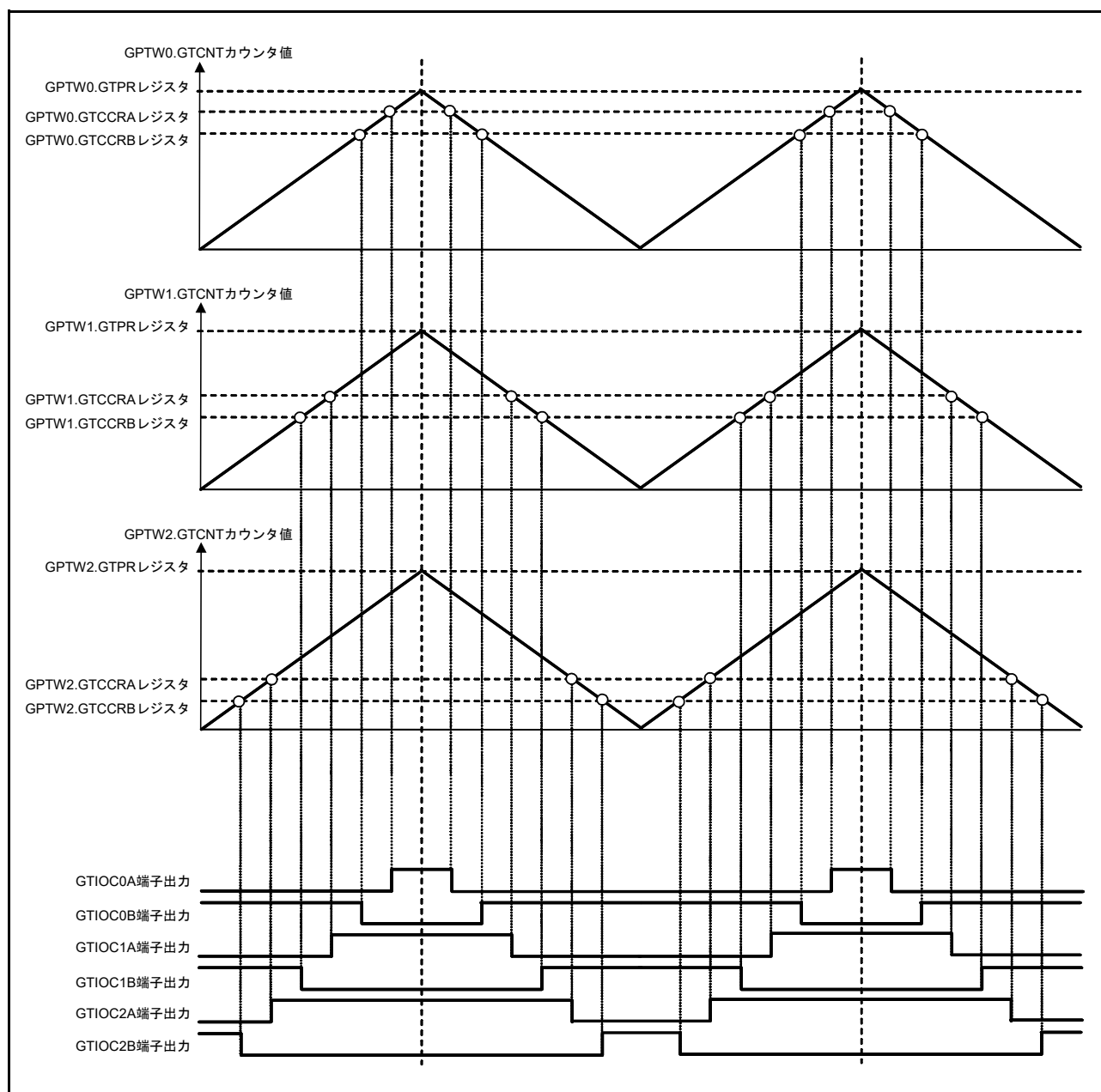
図 26.84 三角波 3 相相補 PWM 出力
