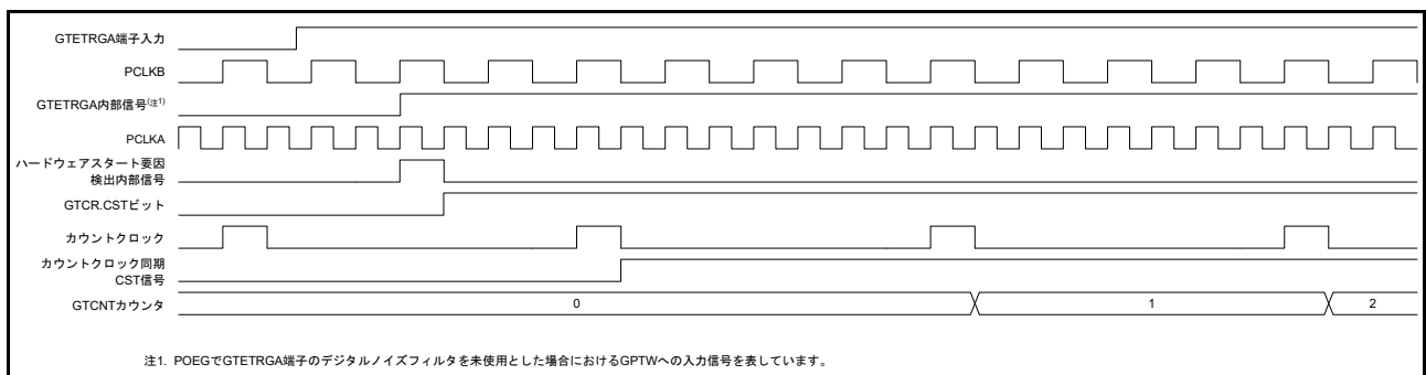
図 26.57 GTETRGA 端子入力の立ち上がりによるカウントスタート動作タイミング例
