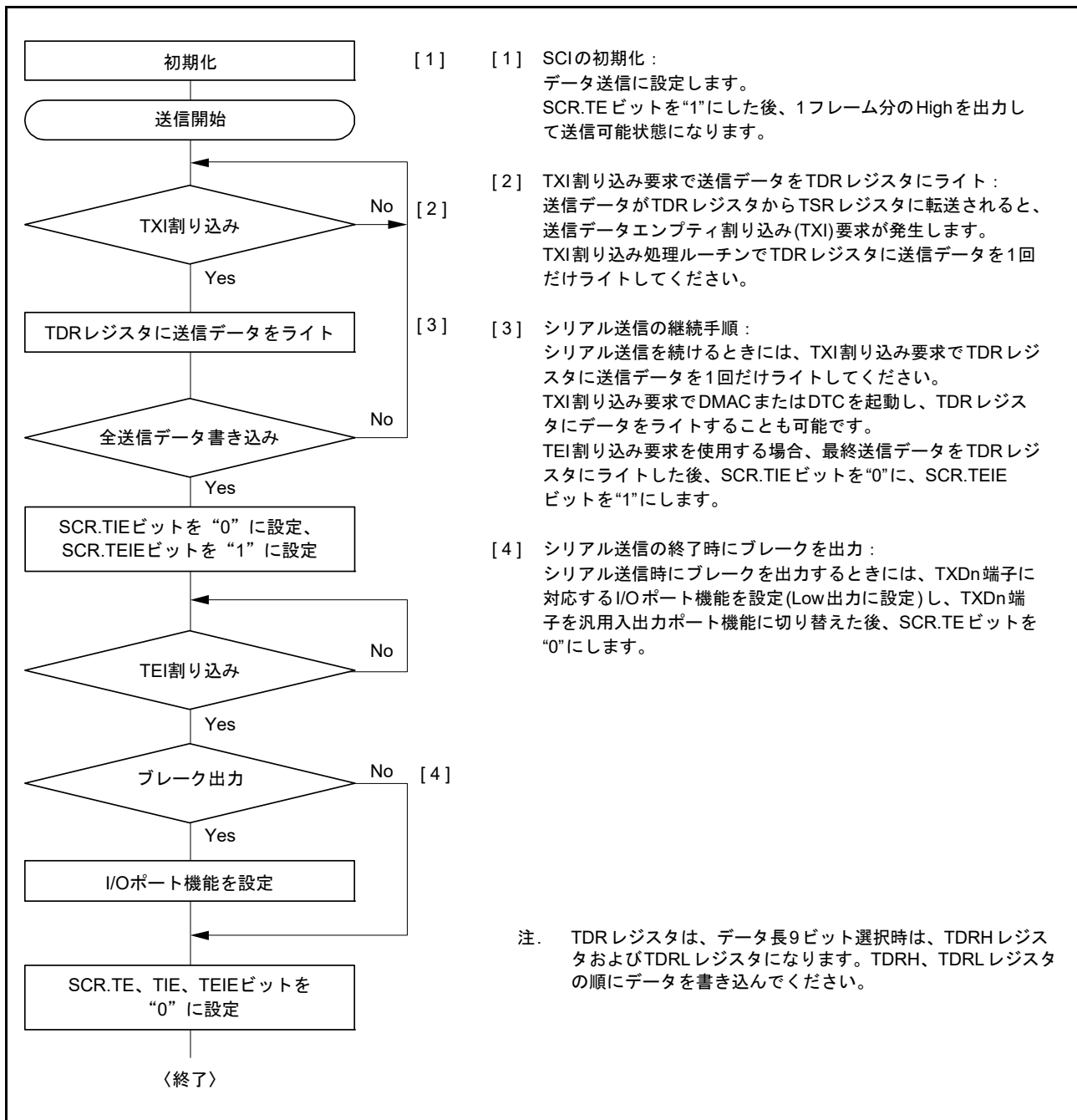
図 41.17 調歩同期式モードのシリアル送信のフローチャート例
