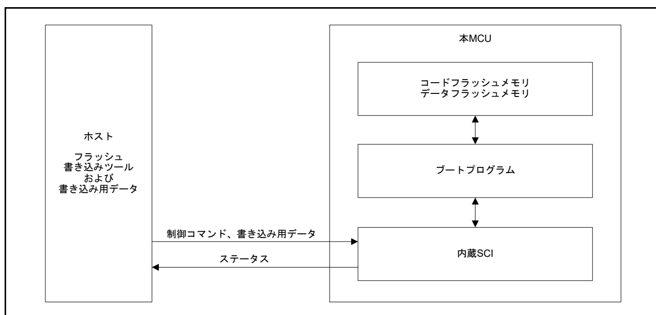
図 62.34 ブートモード (SCI インタフェース) 時のシステム構成
