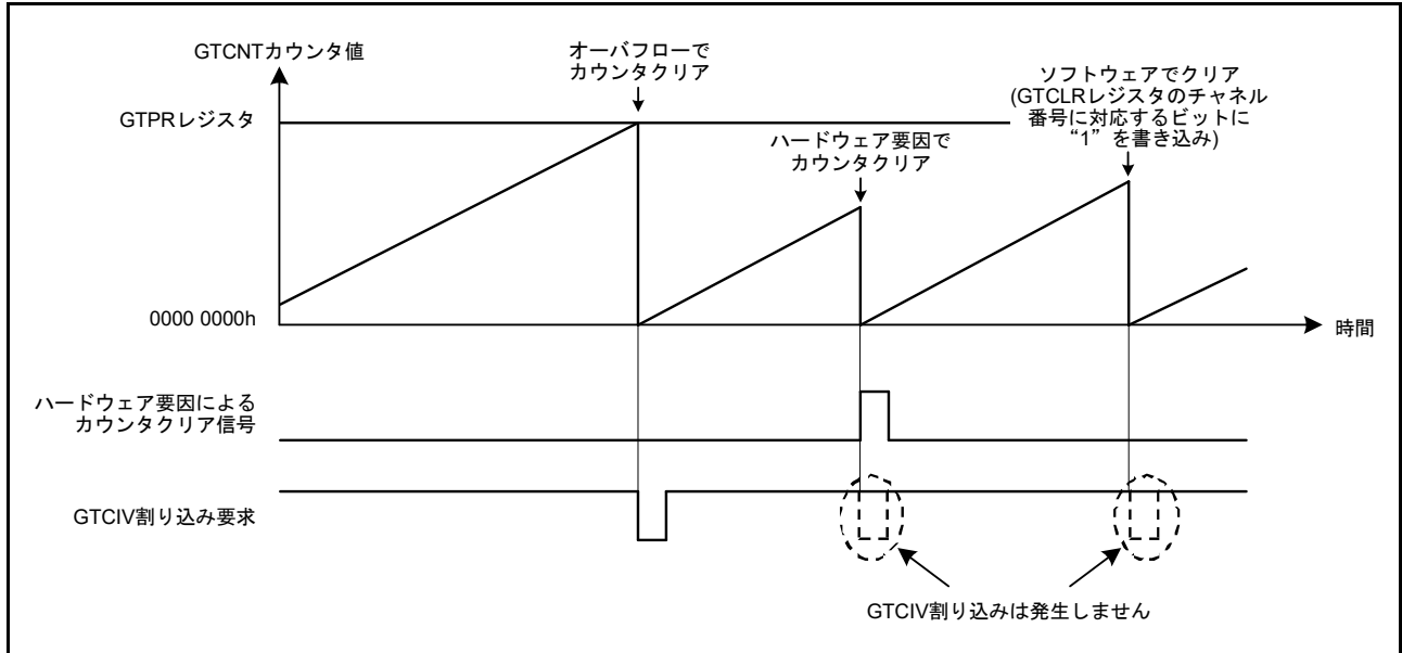
図 26.70 ハードウェア要因によるカウンタクリアと GTCIV 割り込みの関係
