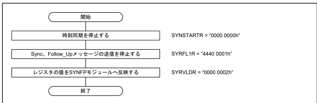
図37.21 P2Pスレーブ動作の停止手順
