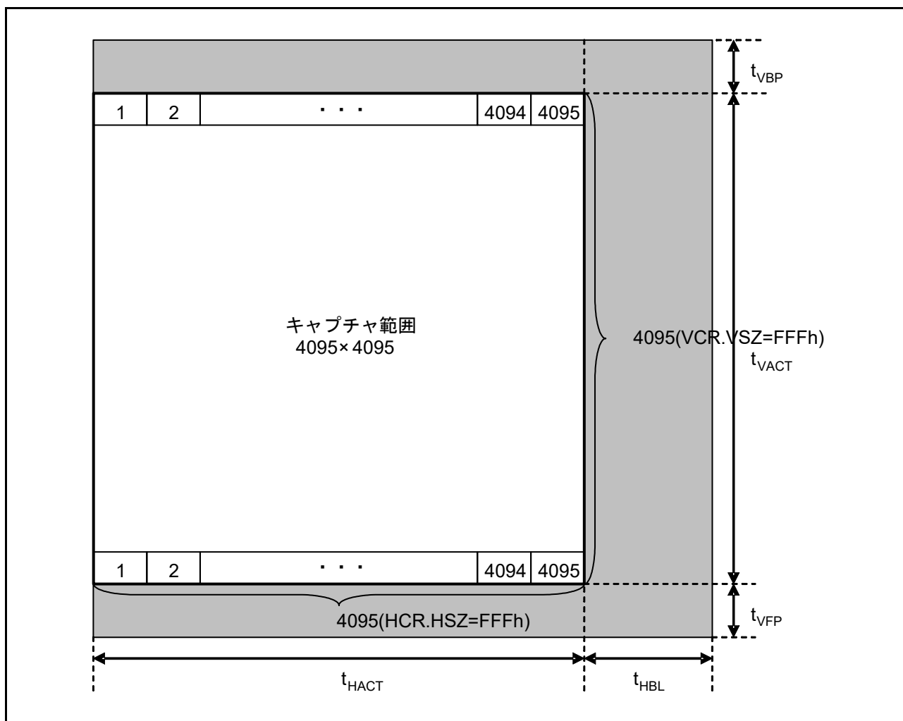
図 50.9 VCR レジスタ、HCR レジスタ設定とキャプチャ範囲 (VCR = 0FFF 0000h, HCR = 0FFF 0000h)
