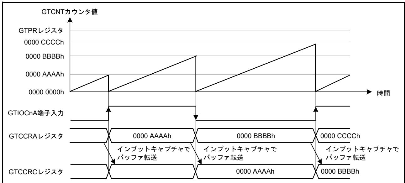
図 26.30 GTCCRA, GTCCRB レジスタのバッファ動作例 (のこぎり波でアップカウント、GTIOcNA 端子入力の両エッジで GTCNT カウンタクリアおよびインプットキャプチャの場合) (n = 0 ~ 3)
