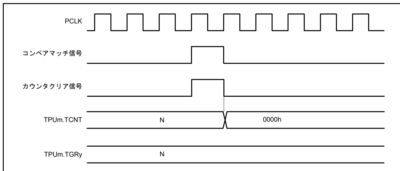
図 28.35 カウンタクリアタイミング (コンペアマッチ)
