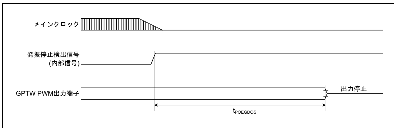
図 63.51 POEG 出力ディセーブル時間 (発振停止検出)
