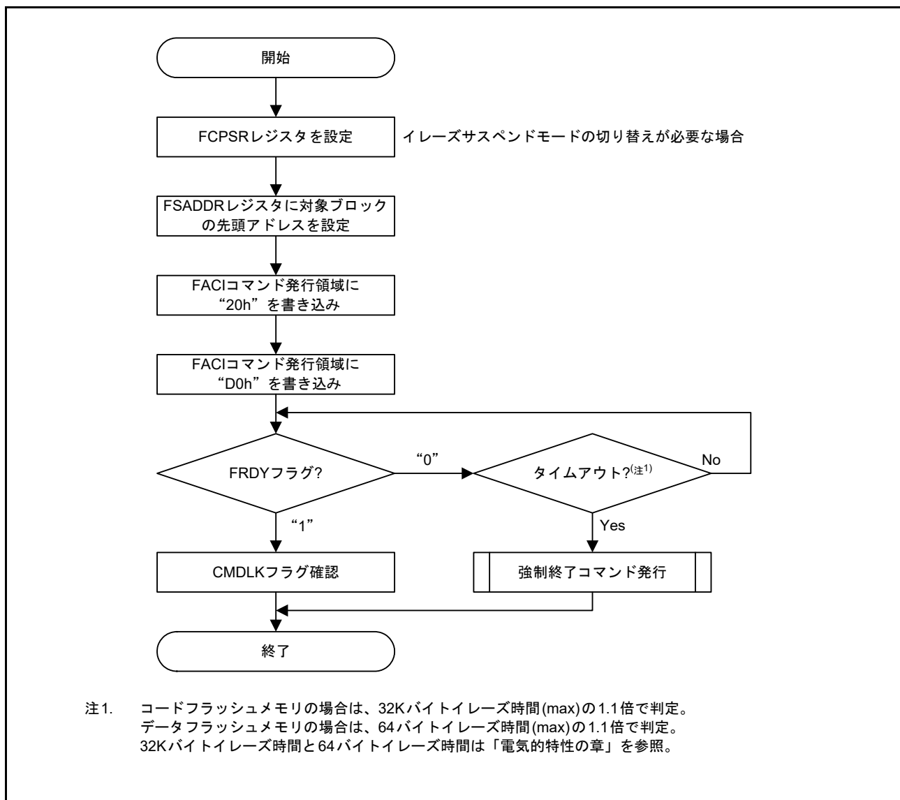
図 62.15 ブロックイレーズコマンドの使用法
