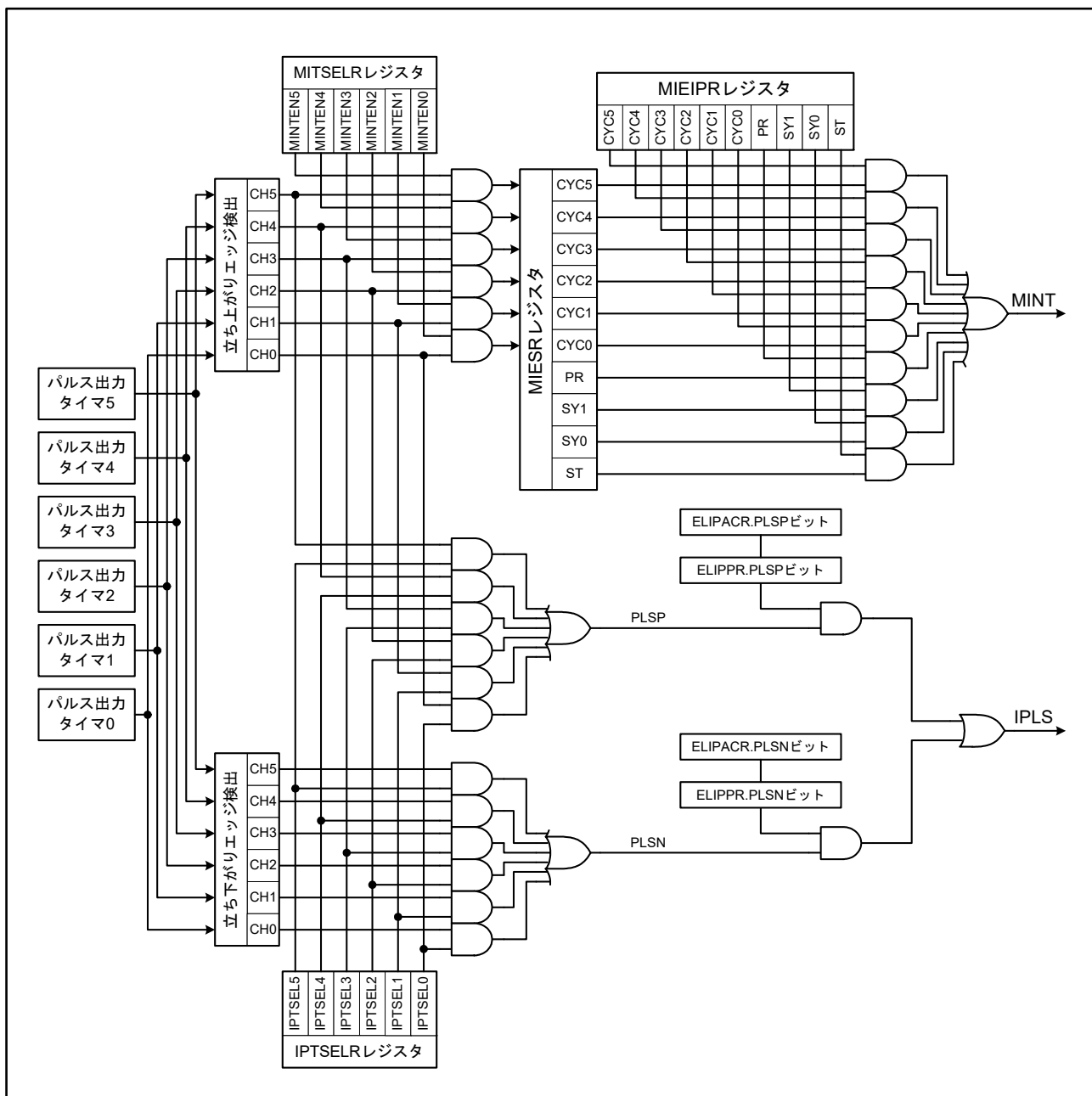
図37.37 パルス出力タイマの割り込み要求の詳細
