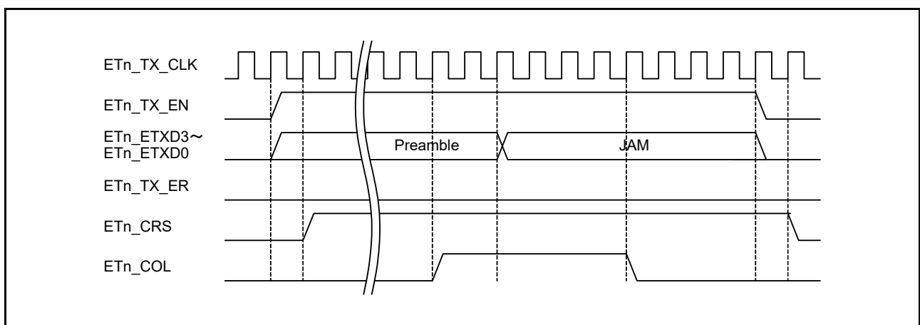
図 36.7 MII フレーム送信タイミング (衝突発生)
