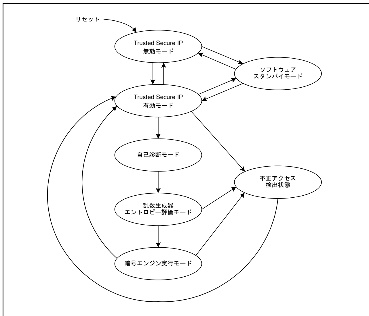
図 55.2 Trusted Secure IP の動作モード状態遷移図
