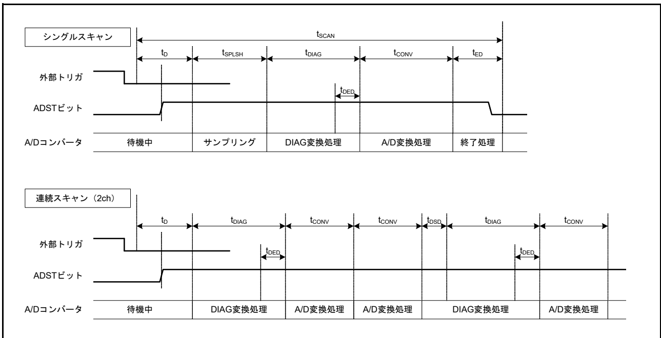
図 56.39 スキャン変換のタイミング (非同期トリガ起動の場合)
