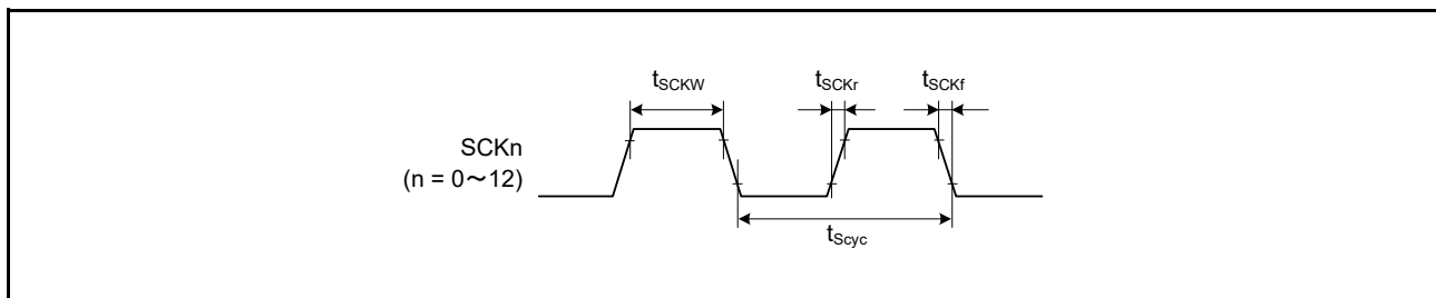
図 63.54 SCK クロック入力タイミング
