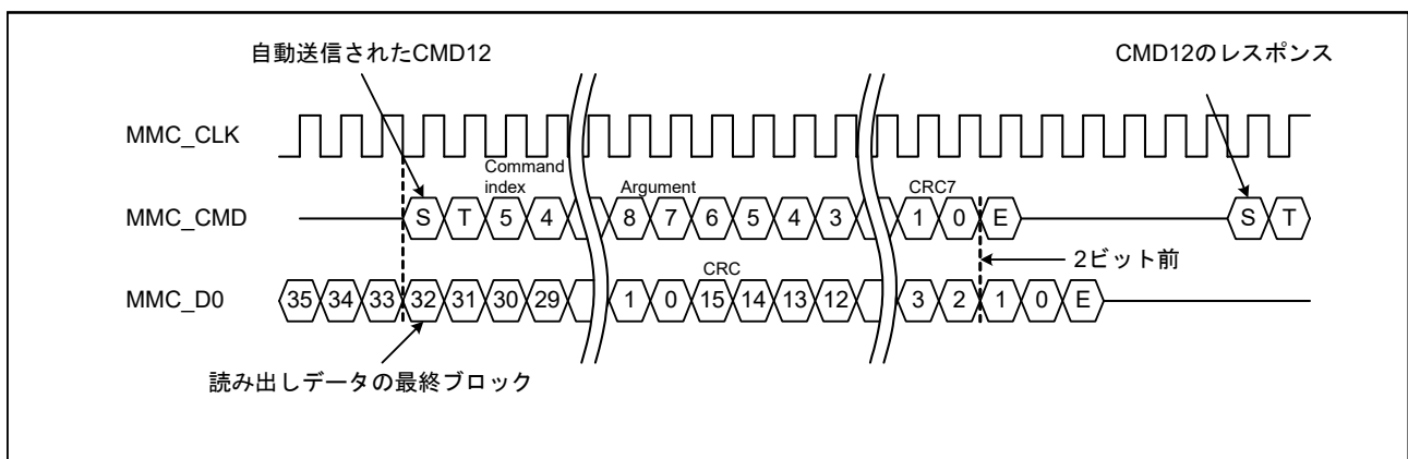
図 49.8 マルチブロックリード時の CMD12 自動送信タイミング (1ビットモード時)
