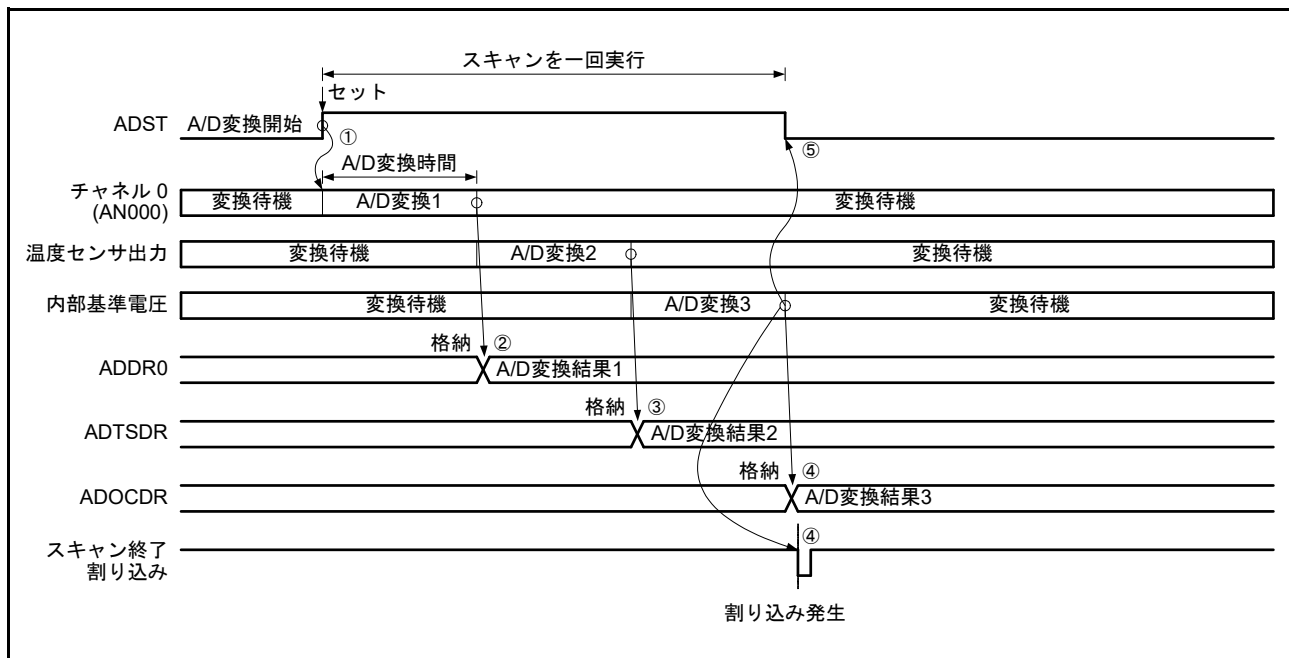
図 56.12 シングルスキャンモードの動作例 (基本動作 : AN000、温度センサ出力、内部基準電圧選択)
