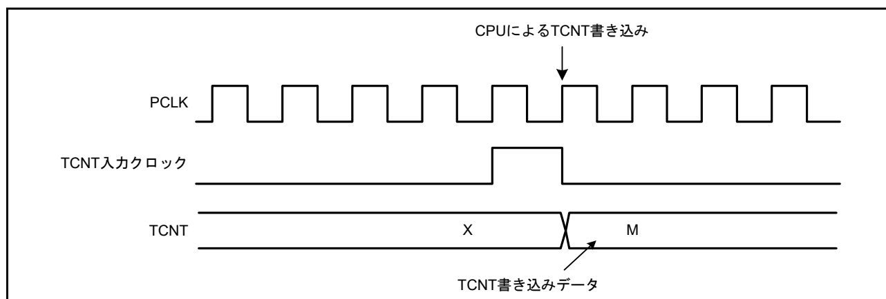
図 28.45 TPUm.TCNT への書き込みとカウントアップの競合
