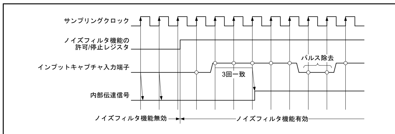
図 26.118 ノイズフィルタのタイミングチャート
