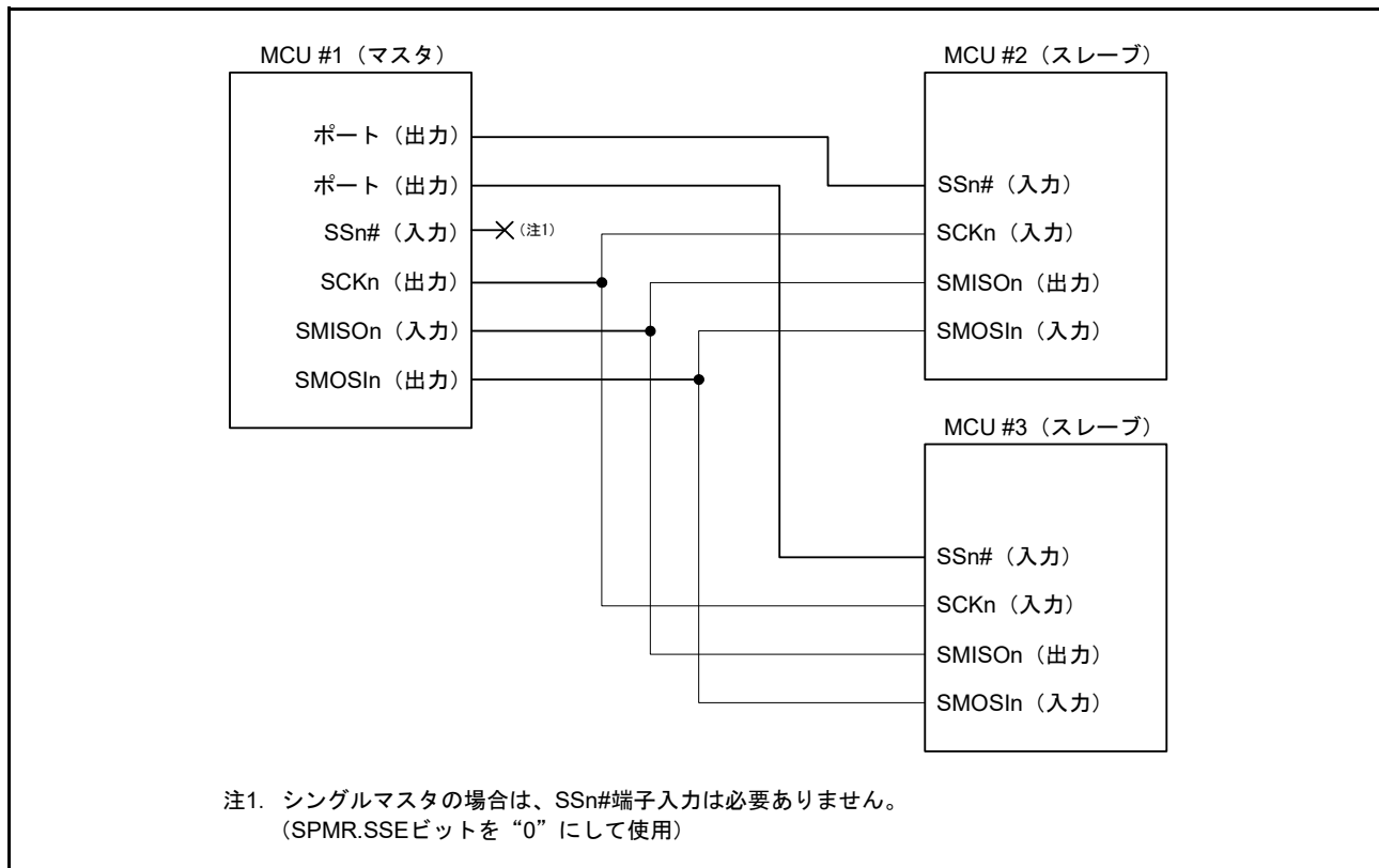
図 41.61 簡易 SPI モードの接続例 (シングルマスタ時 (SPMR.SSE ビット = 0))
