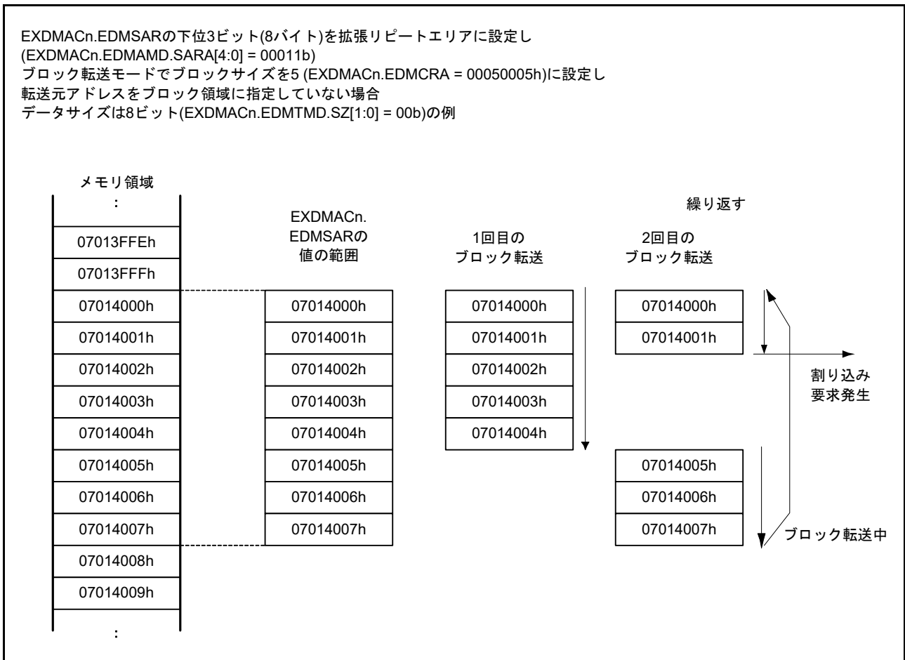
図 19.7 ブロック転送モードと拡張リポートエリア機能を併用した例
