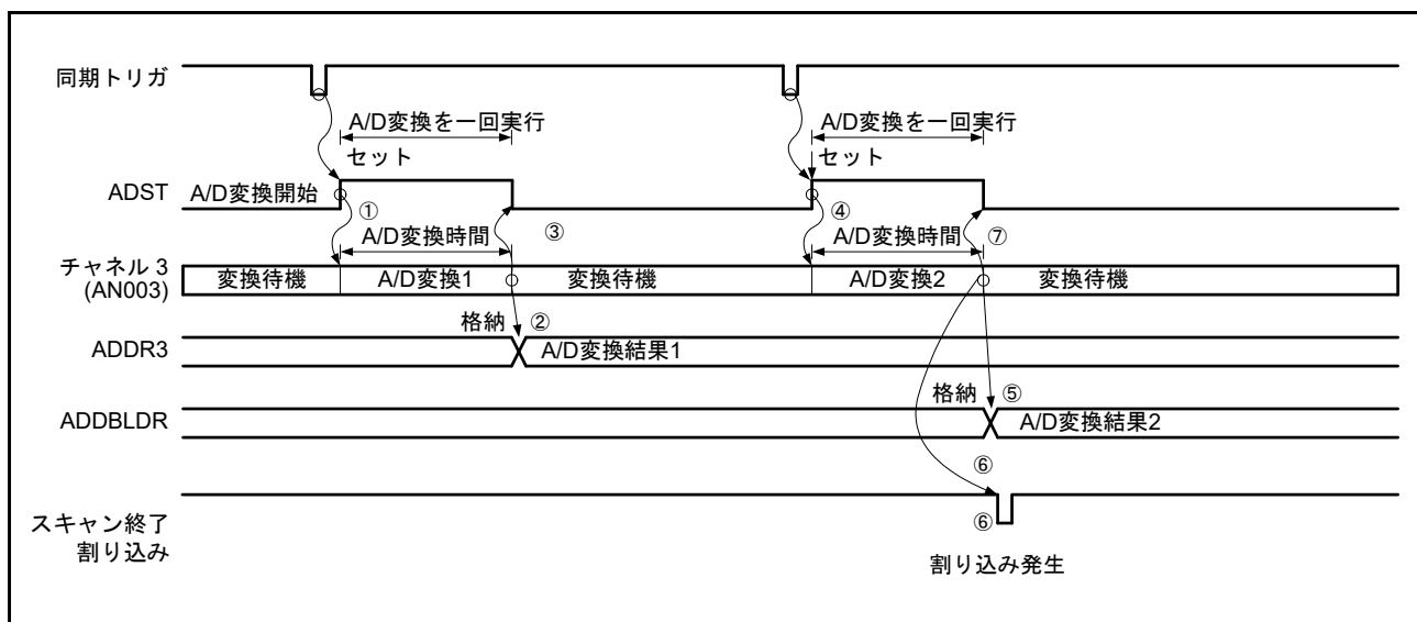
図 56.13 シングルスキャンモードの動作例 (ダブルトリガモード選択、AN003 を二重化)
