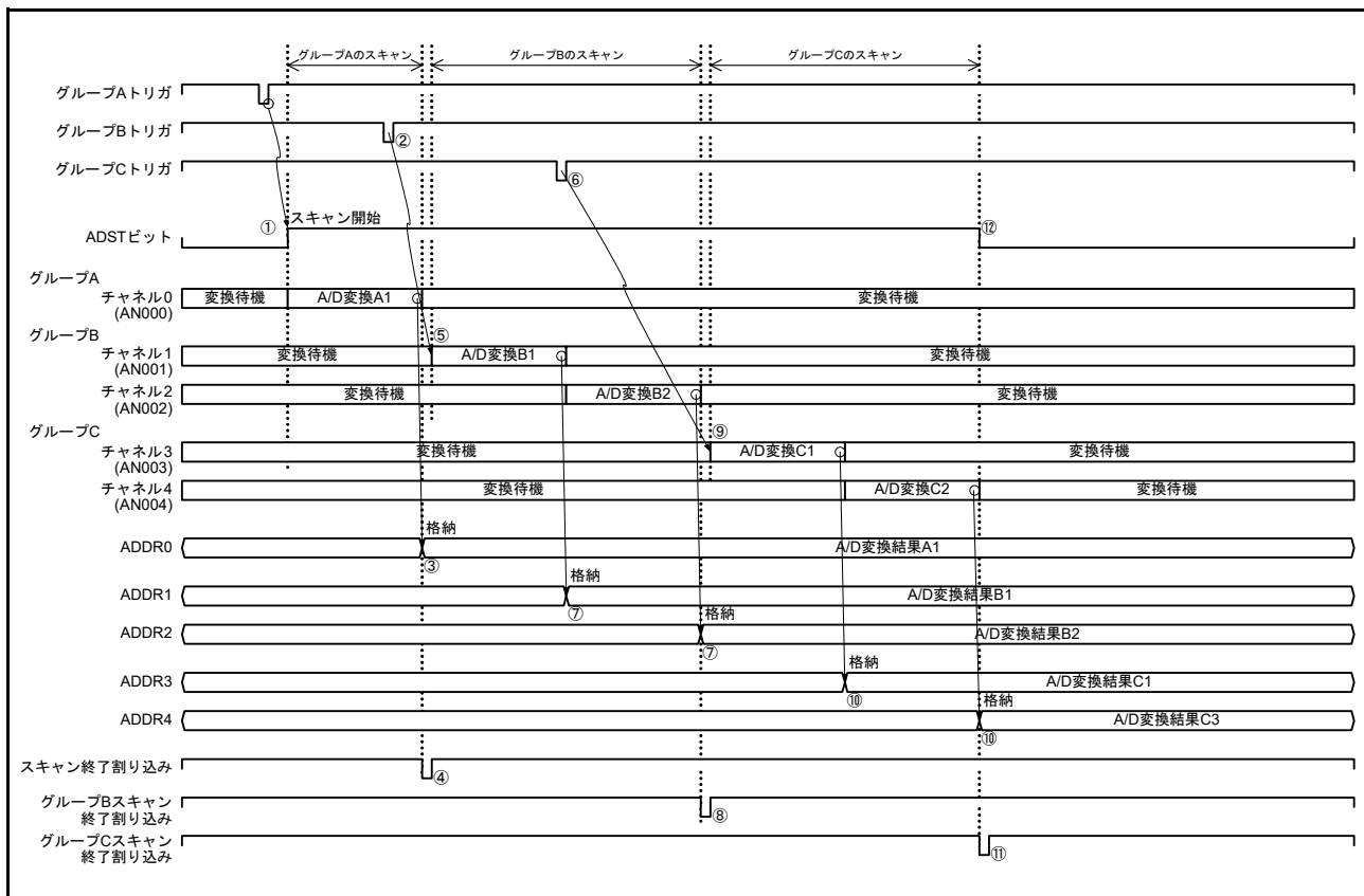
図 56.32 グループ優先動作の例 3「優先グループスキャン中の低優先グループトリガ入力」再スキャンあり (ADGSPCR.GBRSCN = 1, ADGSPCR.GBRP = 0, ADGSPCR.LGRRS = 1, ADGCTRGR.GRCE = 1 時の動作)
