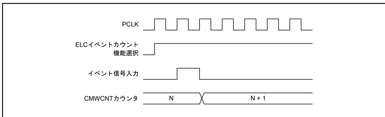
図 32.18 イベント受け付けによるイベントカウント動作
