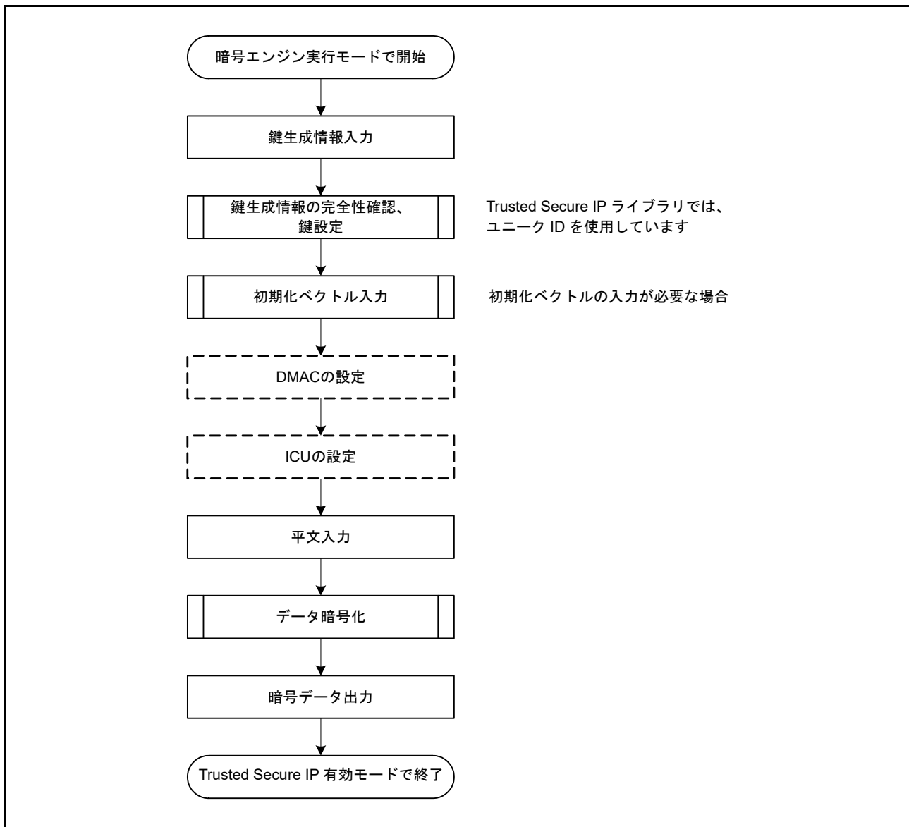
図 55.7 暗号化フロー
