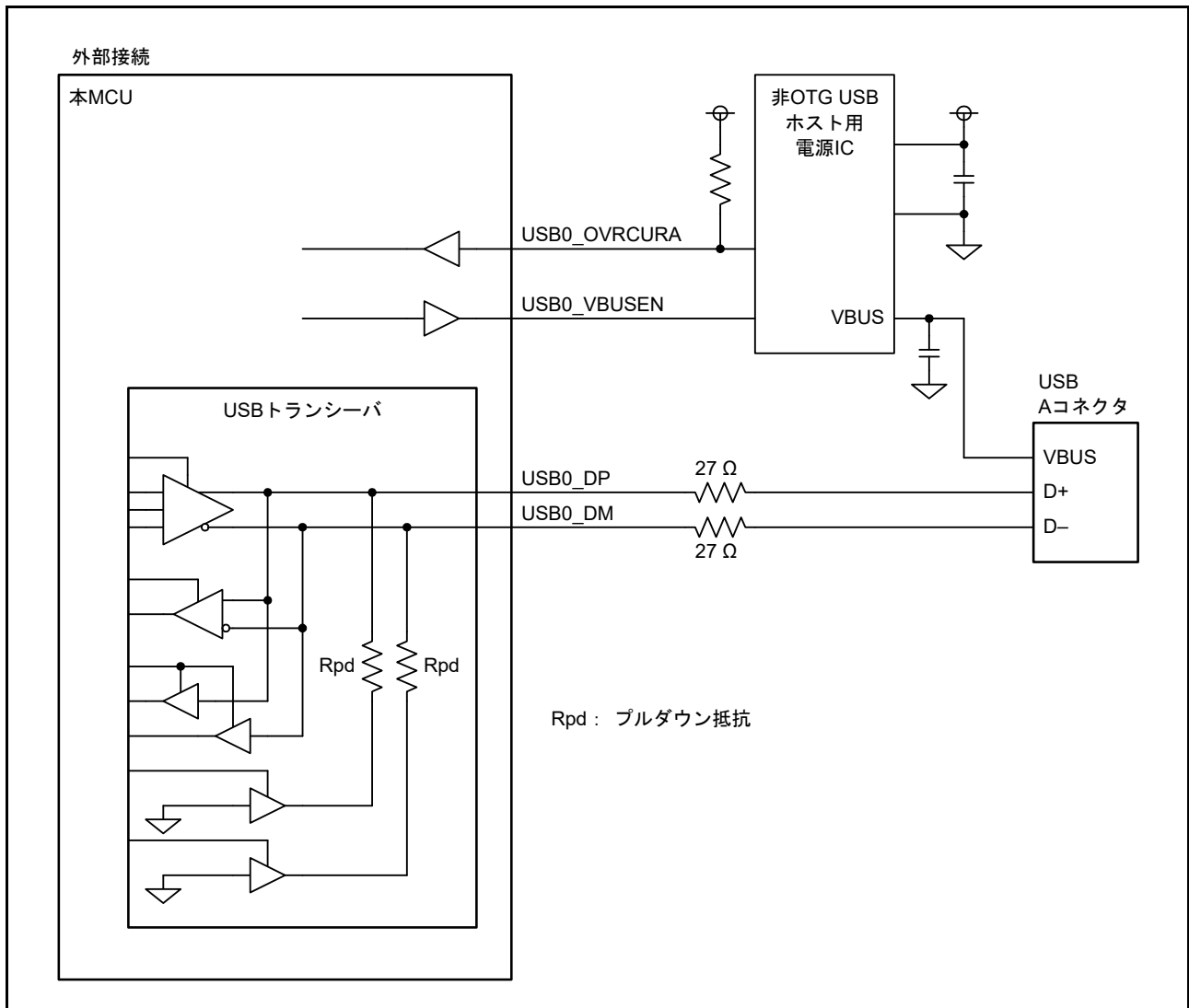
図 40.4 ホストコントローラと USB コネクタとの接続例
