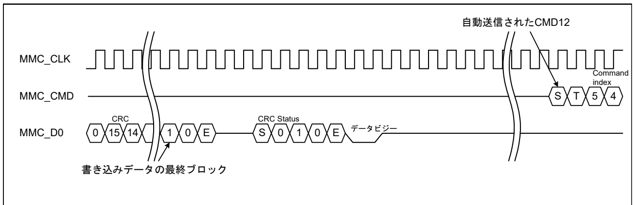
図 49.9 マルチブロックライト時の CMD12 自動送信タイミング (1 ビットモード時)
