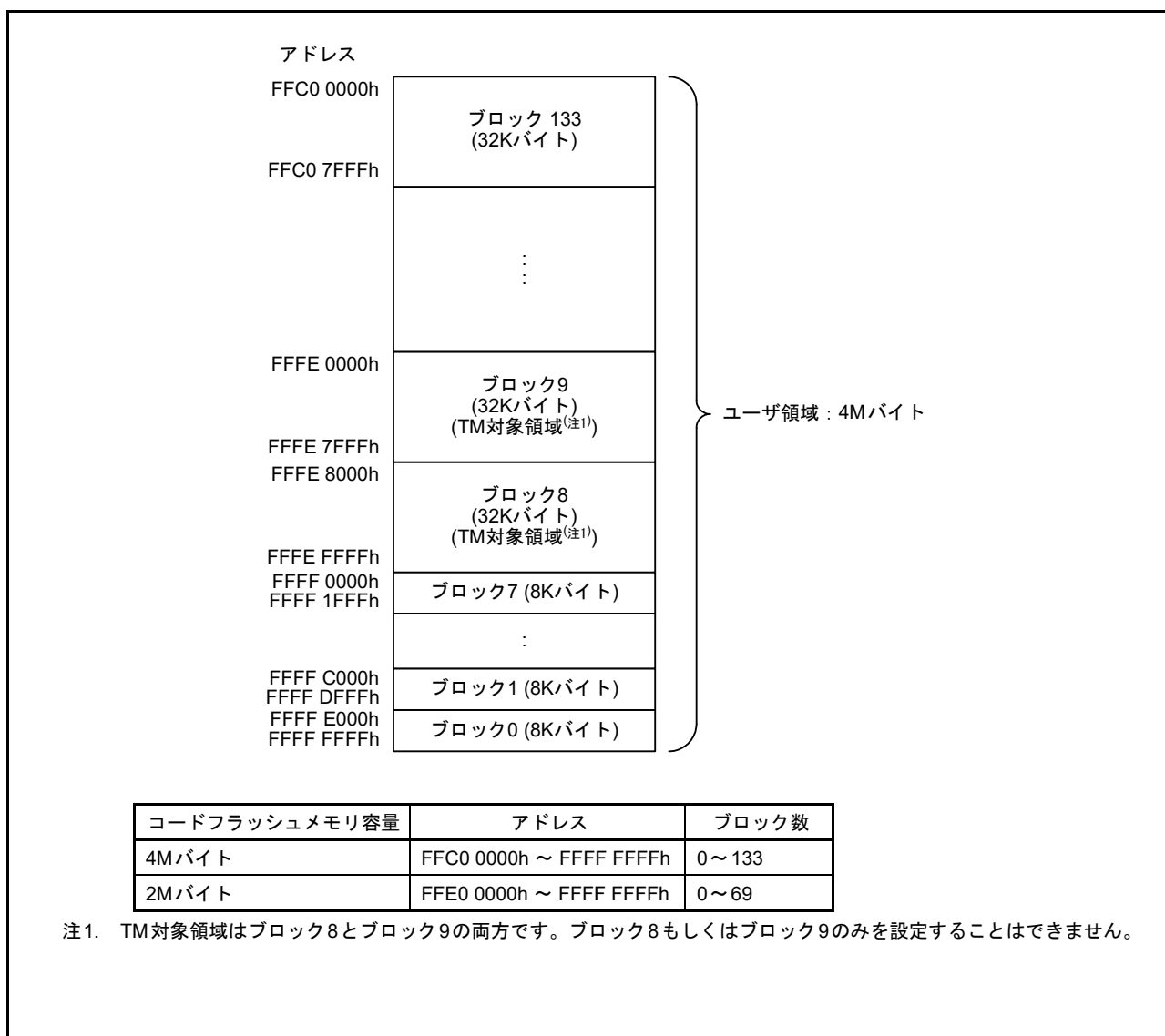
図 62.2 リニアモード時のコードフラッシュメモリマッピング
