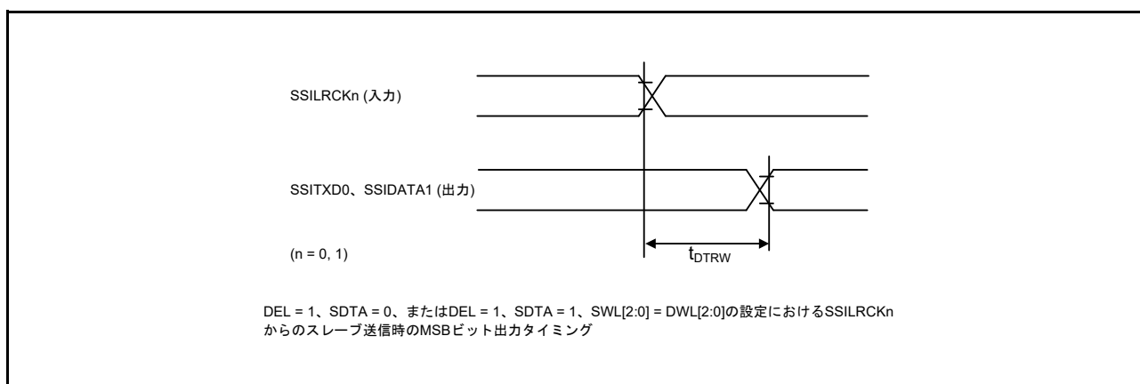
図 63.77 SSILRCKn 変化時からの SSIE データ出力遅延
