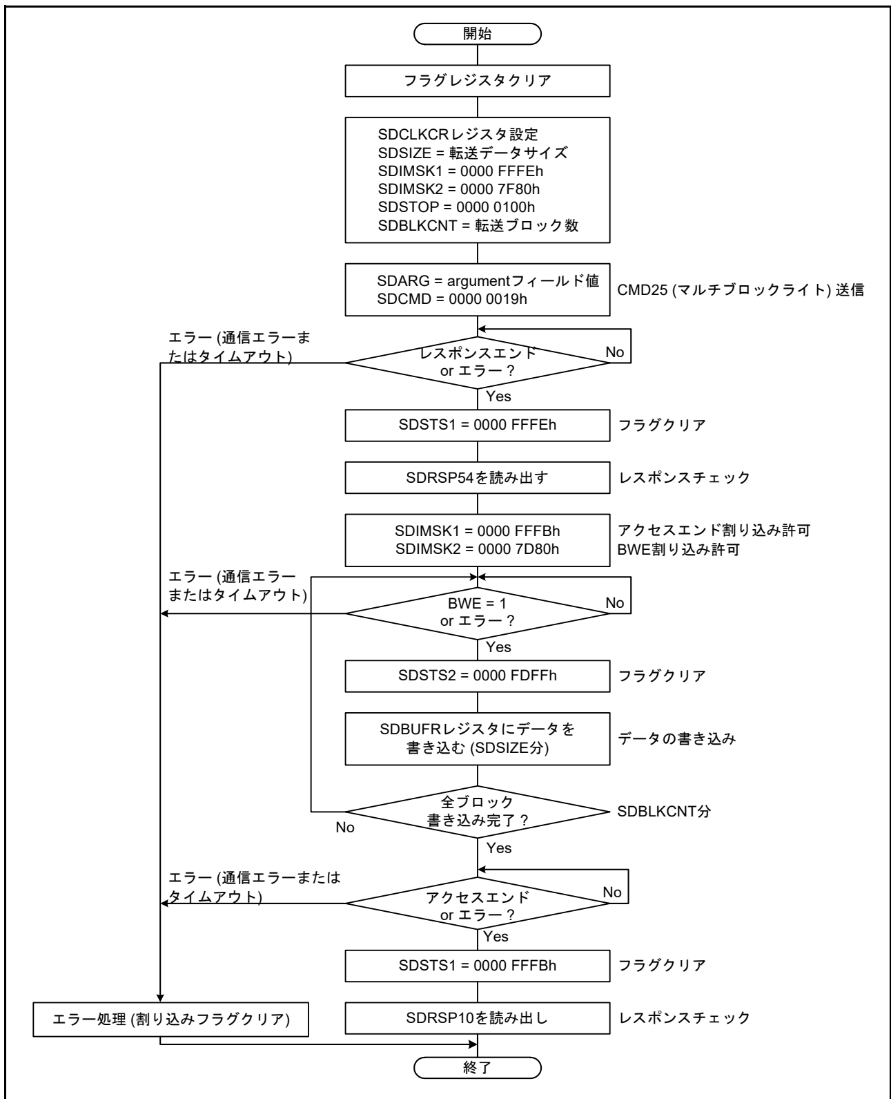
図 48.13 マルチブロックライトコマンドの送信例
