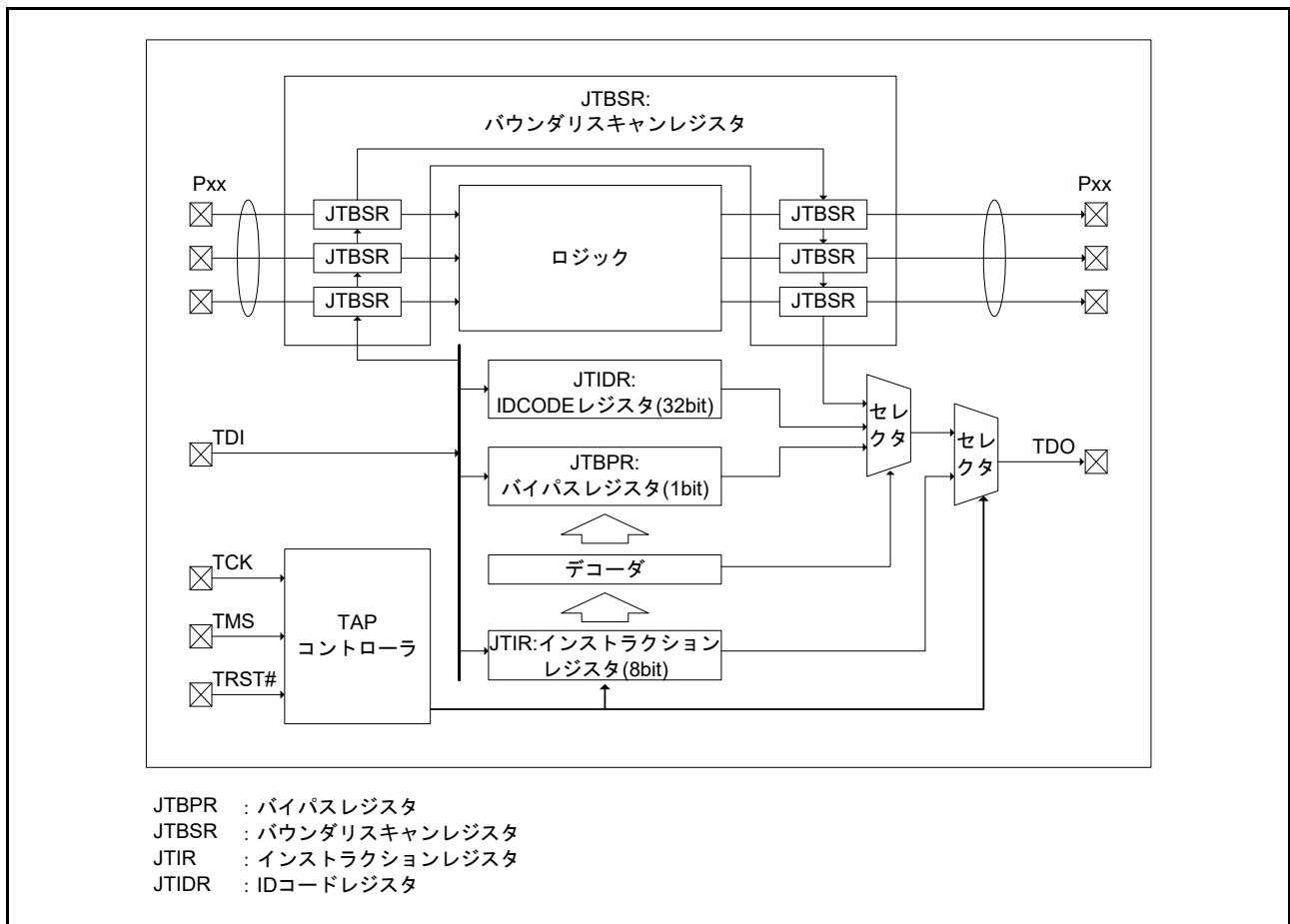
図 53.1 JTAG ブロック図
