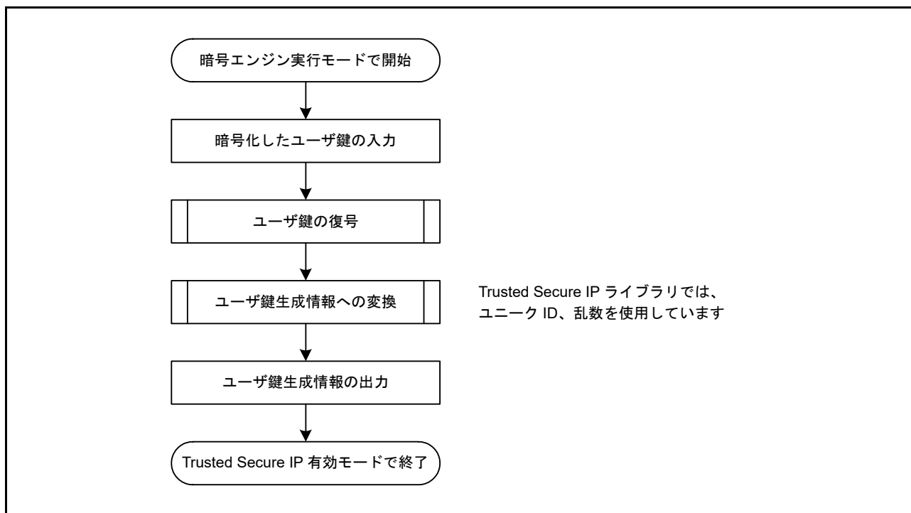
図 55.5 鍵インストールフロー
