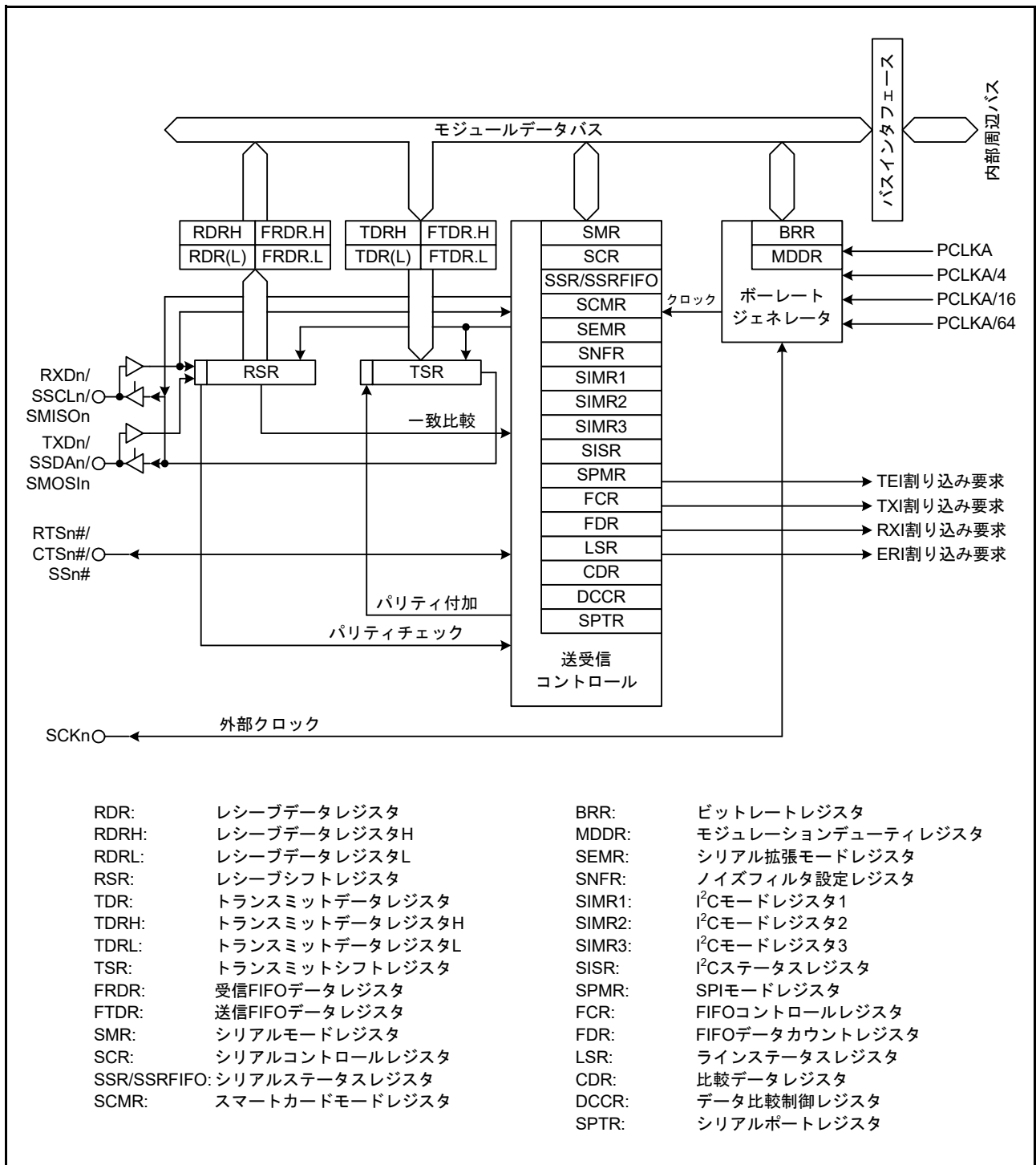
図 41.3 SCli (SCI7 ~ SCI11) のブロック図
