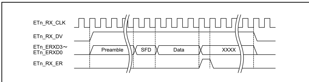
図 36.9 MII フレーム受信タイミング (受信エラー (1) 受信エラー通知)
