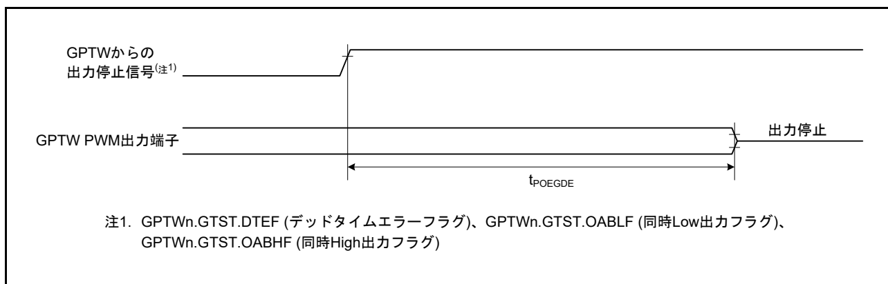
図 63.49 POEG 出力ディセーブル時間 (GPTW からの出力停止信号検出)
