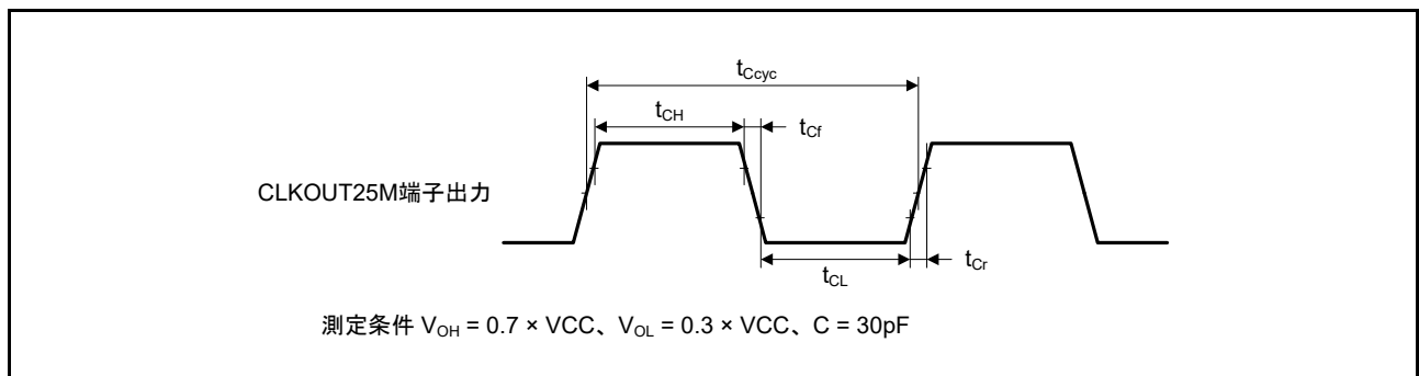
図 63.13 CLKOUT25M 端子出力タイミング
