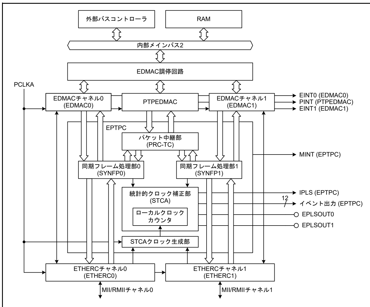
図 37.1 EPTPCの構成
