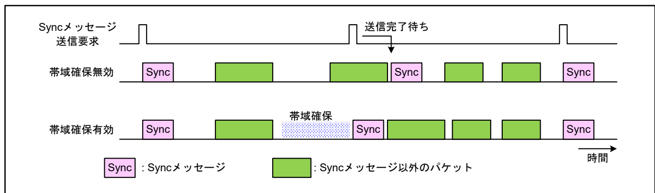
図37.35 Syncメッセージ送信帯域確保機能
