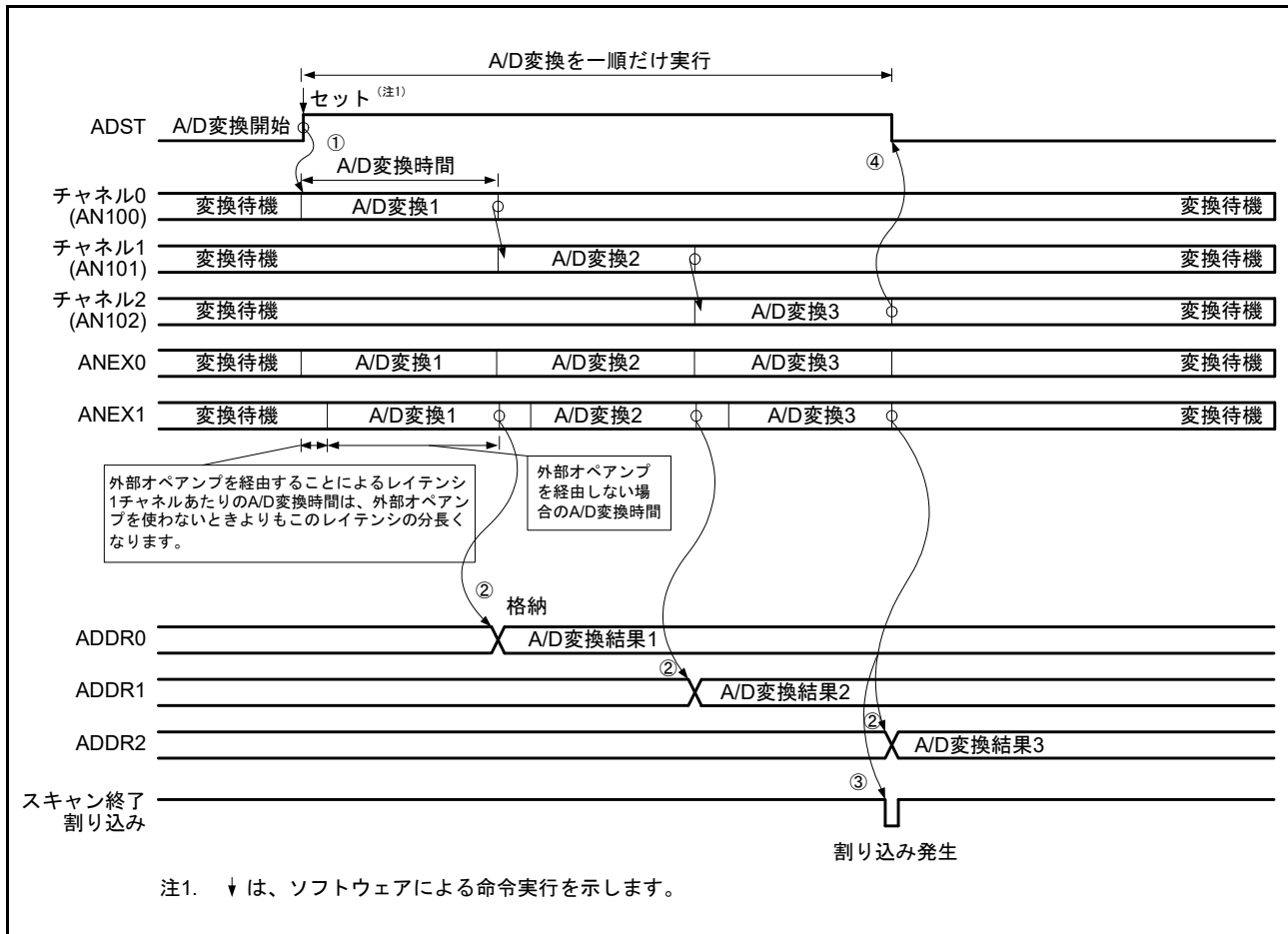
図 56.36 ANEX1 入力の動作例 (シングルスキャンモード)
