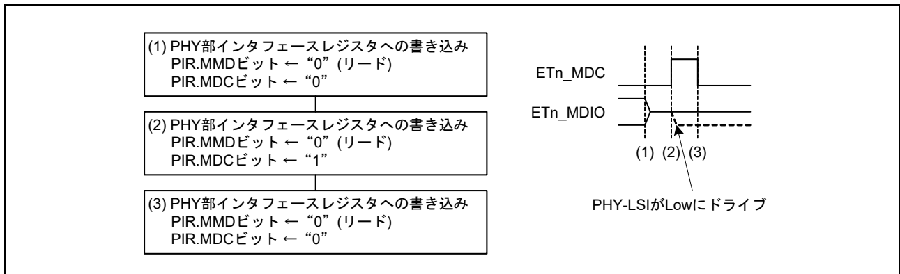
図 36.15 バス解放フロー (表 36.3 中のリード時の TA)
