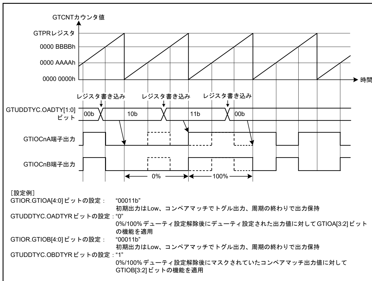
図 26.54 デューティ 0%/100% 出力機能の動作例 (n = 0 ~ 3)
