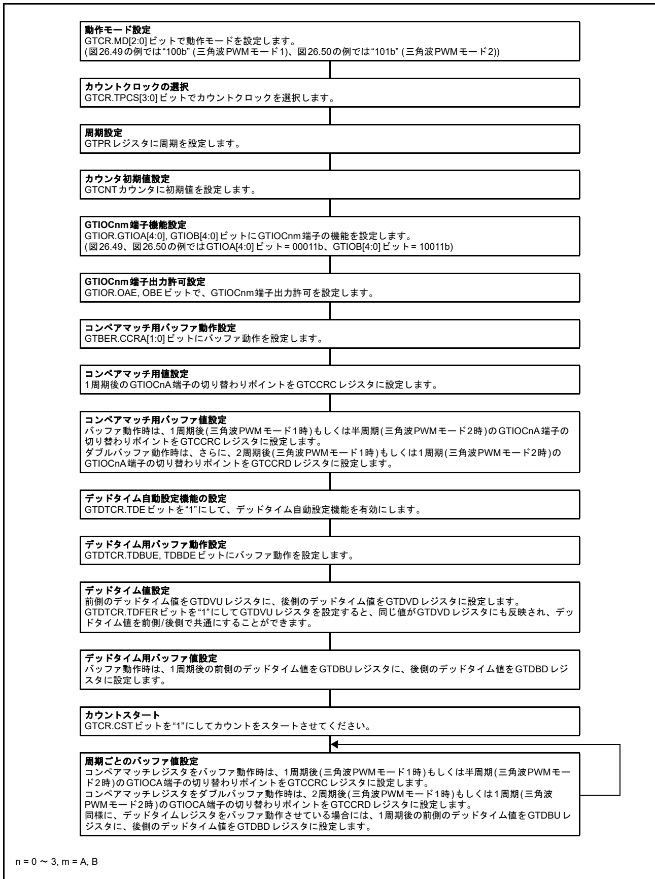
図 26.52 デッドタイム自動設定機能の設定例 (三角波 PWM モード 1/2 時)
