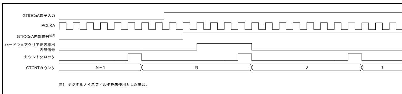
図 26.72 GTIOCnA 端子入力の立ち上がりによるカウンタクリア動作タイミング例 (PCLKA の分周クロックによるカウンタ動作時)
