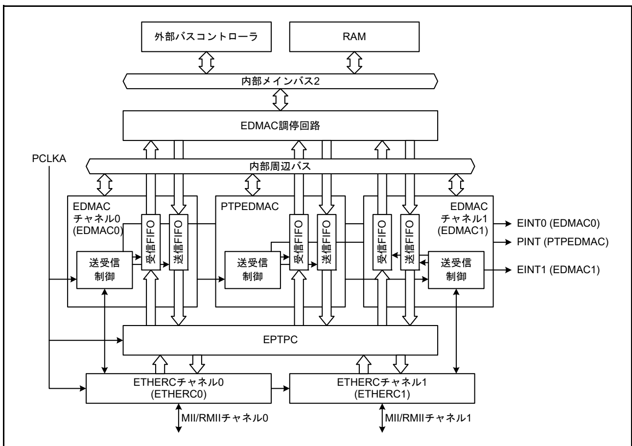
図 38.1 EDMAC の構成
