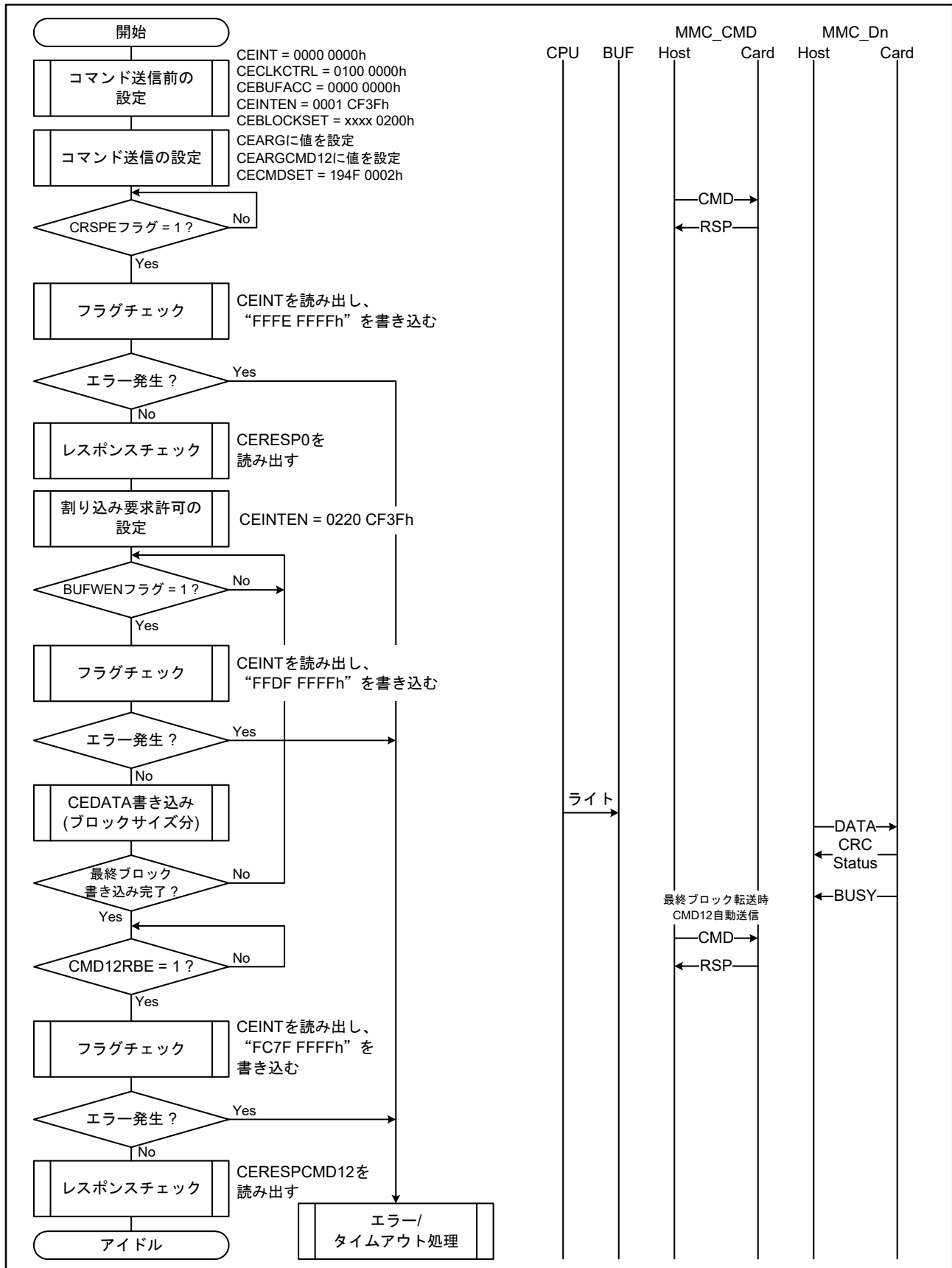
図 49.20 マルチブロックライトの送信例 (CMD25 Open-ended)
