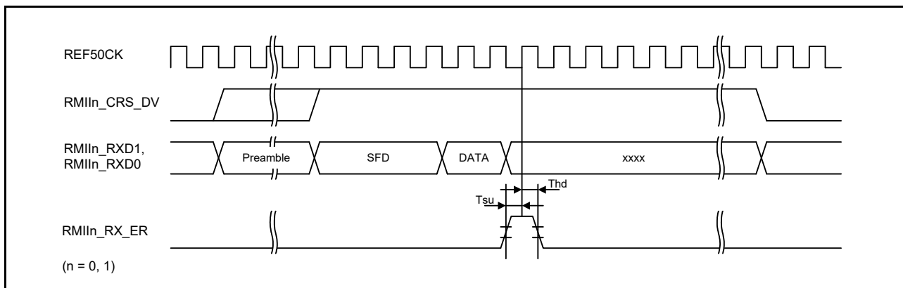
図 63.84 RMIIn 受信タイミング (エラー発生ケース)
