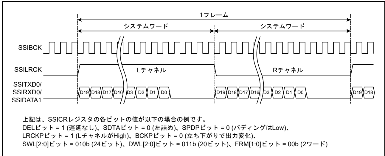
図 47.10 左詰めフォーマットの例
