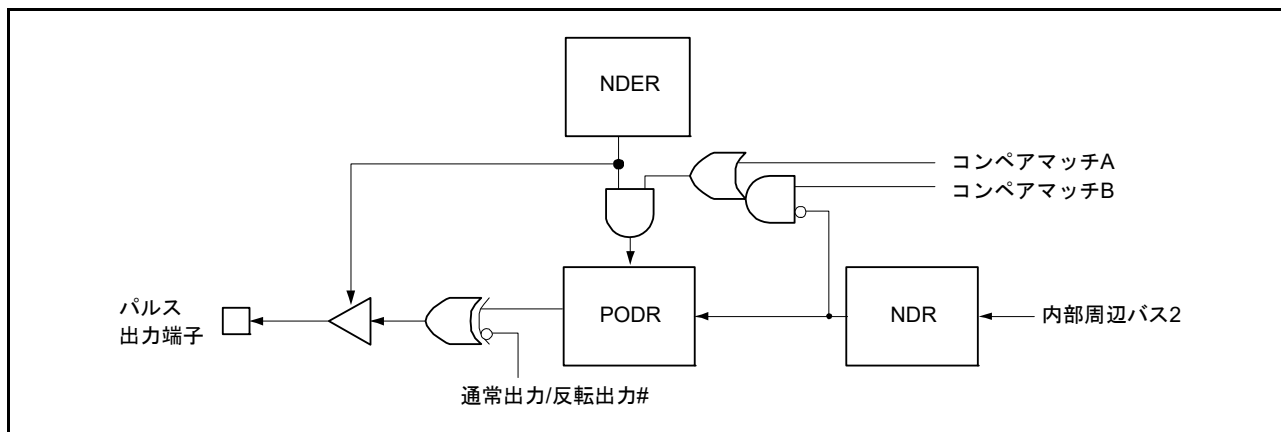
図 29.9 パルス出力ノンオーバーラップ動作
