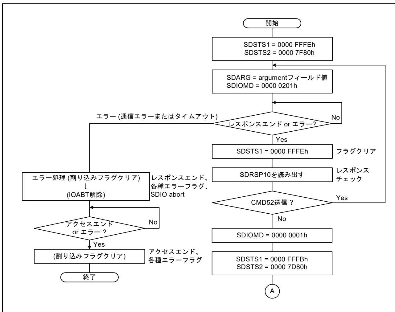
図 48.20 IO_RW_EXTENDED コマンド (CMD53/ マルチブロックライト) のシーケンス中に SDIO none abort (CMD52) を送信する例
