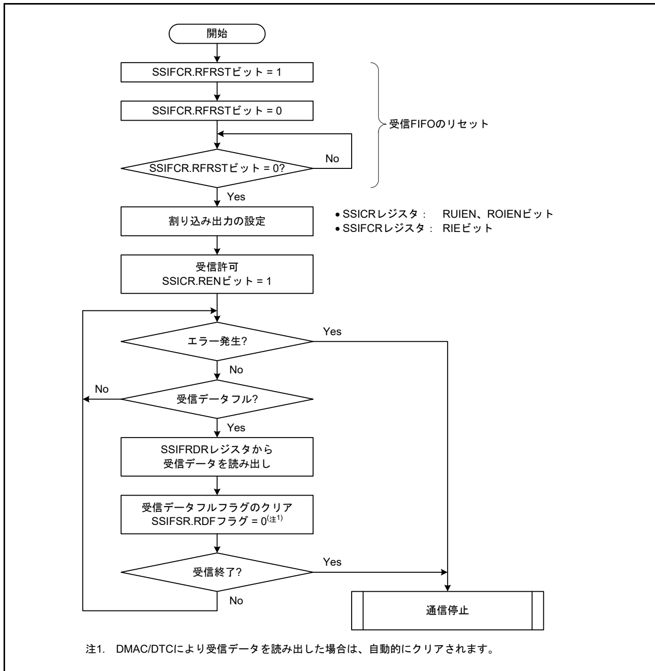
図 47.24 受信フロー例
