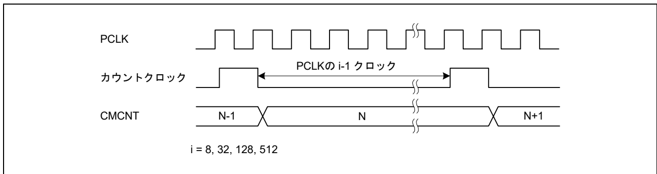
図 31.3 CMCNT カウンタのカウントタイミング
