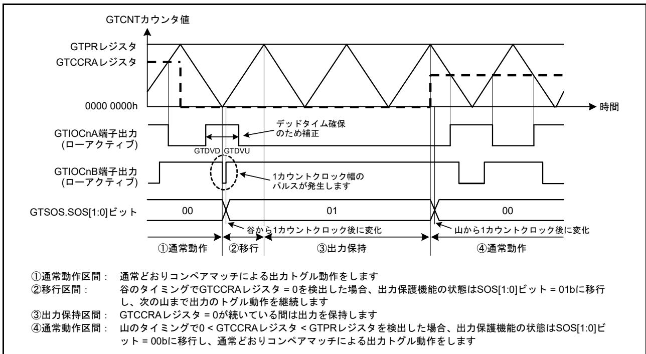
図 26.130 山のバッファ転送で GTCCRA レジスタが“0000 0000h”である場合の出力保護機能の動作例 (山のバッファ転送で 0 < \text{GTCCRA レジスタ} < \text{GTPR レジスタ} に復帰、アクティブレベルは Low の場合) ( n = 0 \sim 3 )
