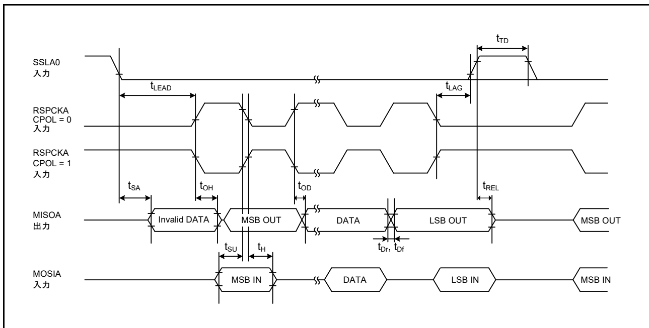
図 63.69 RSPi タイミング (スレーブ、CPHA = 1)
