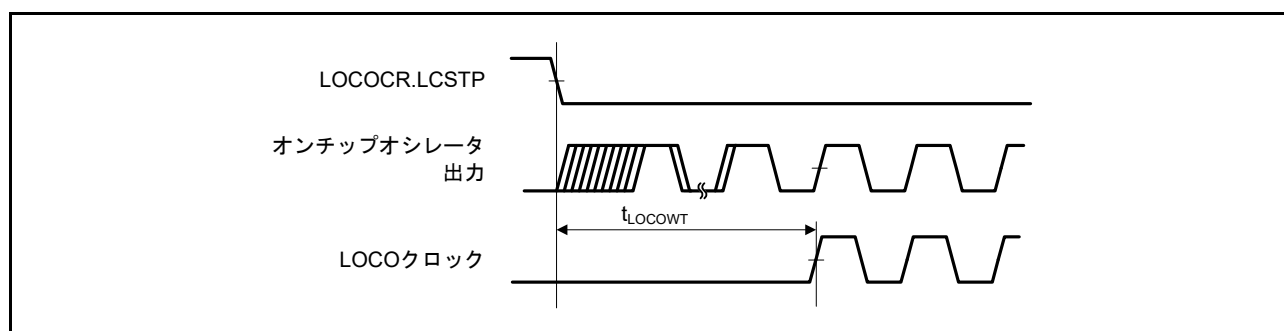
図 63.6 LOCO クロック発振開始タイミング
