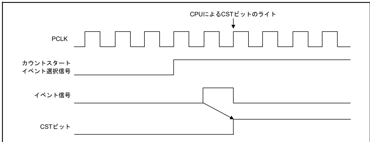
図 28.59 CSTn ビットへのライトサイクルとカウントスタート動作信号の競合
