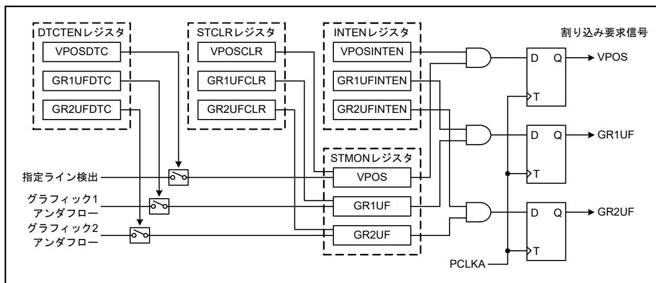
図 51.25 割り込み要求信号生成回路
