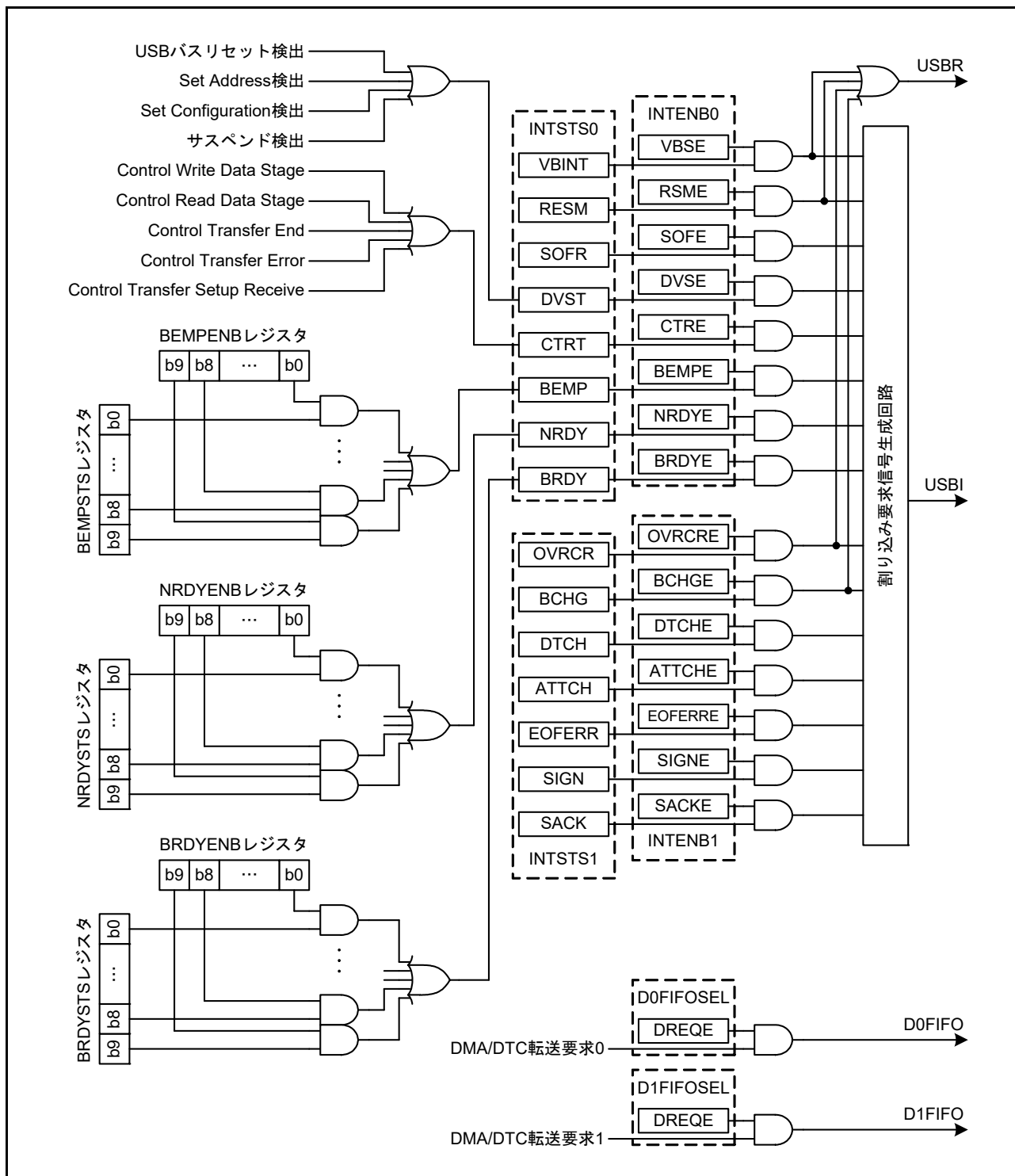
図 40.10 USB 割り込みの関連図
