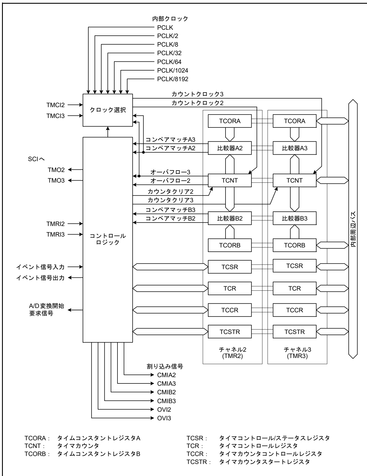
図 30.2 TMR (ユニット1) のブロック図
