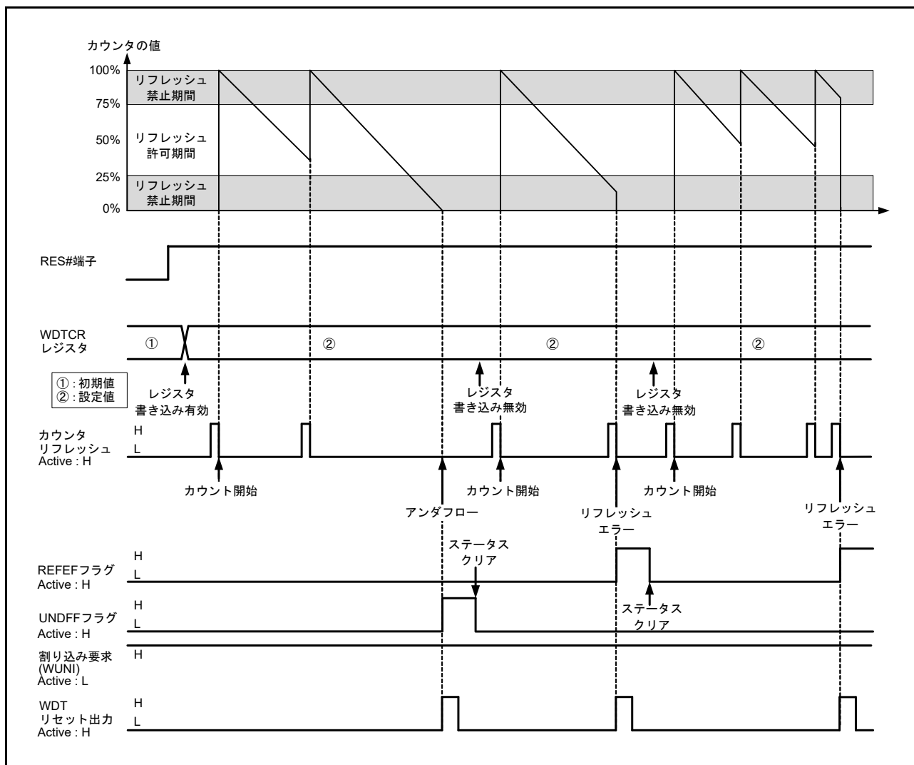
図 34.3 レジスタスタートモード動作例
