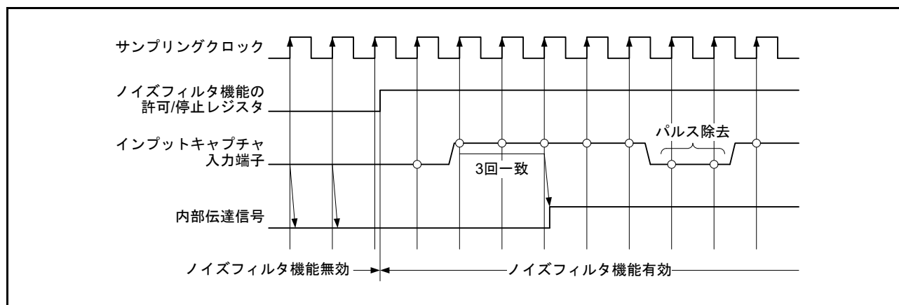
図 28.30 ノイズフィルタのタイミングチャート
