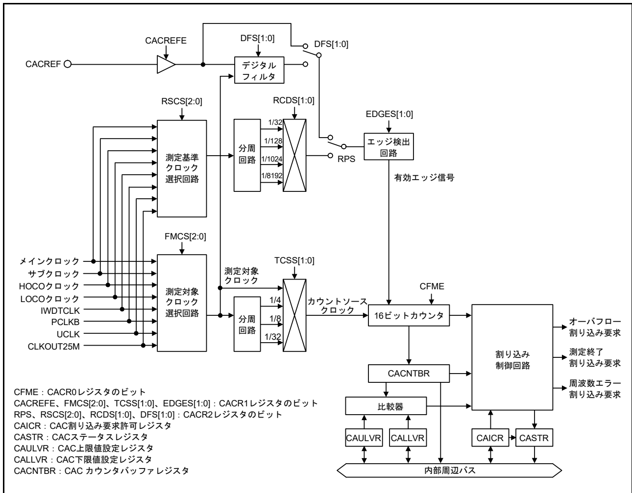
図 10.1 CAC のブロック図
