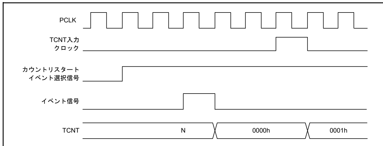
図 28.57 イベント信号入力によるカウントリスタート動作
