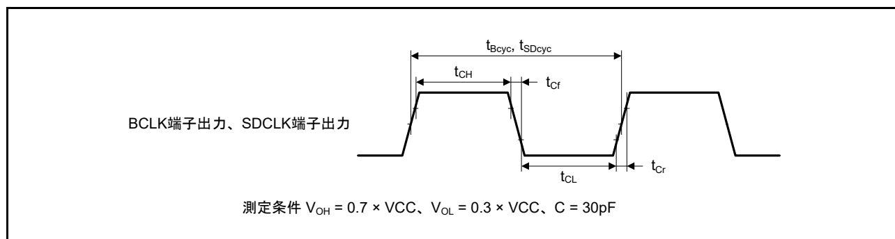
図 63.3 BCLK 端子出力、SDCLK 端子出力タイミング
