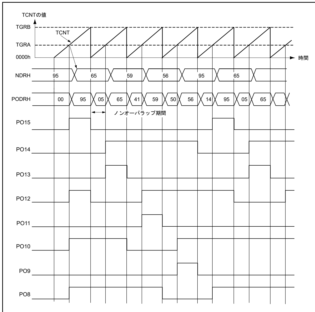
図 29.13 パルス出力ノンオーバーラップ動作例 (4相の相補ノンオーバーラップ出力)
