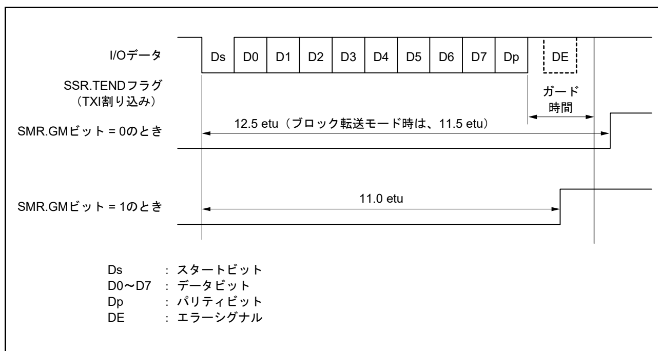
図 41.46 送信時の SSR.TEND フラグの発生タイミング
