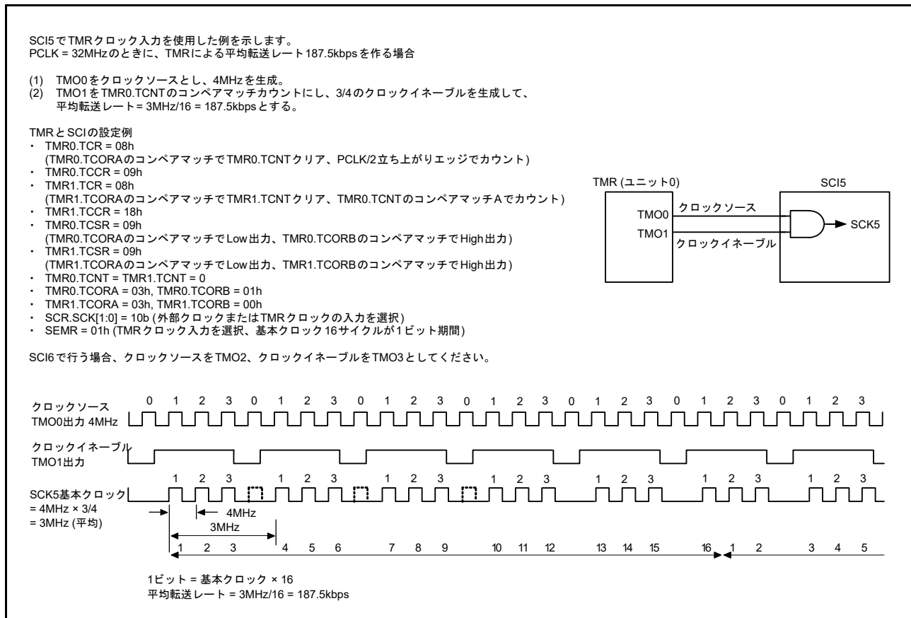
図 41.5 TMR クロック入力時の平均転送レート設定例
