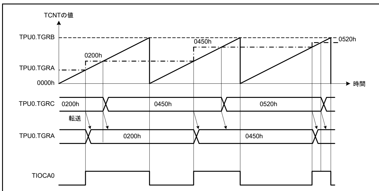
図 28.15 バッファ動作例 (1)
