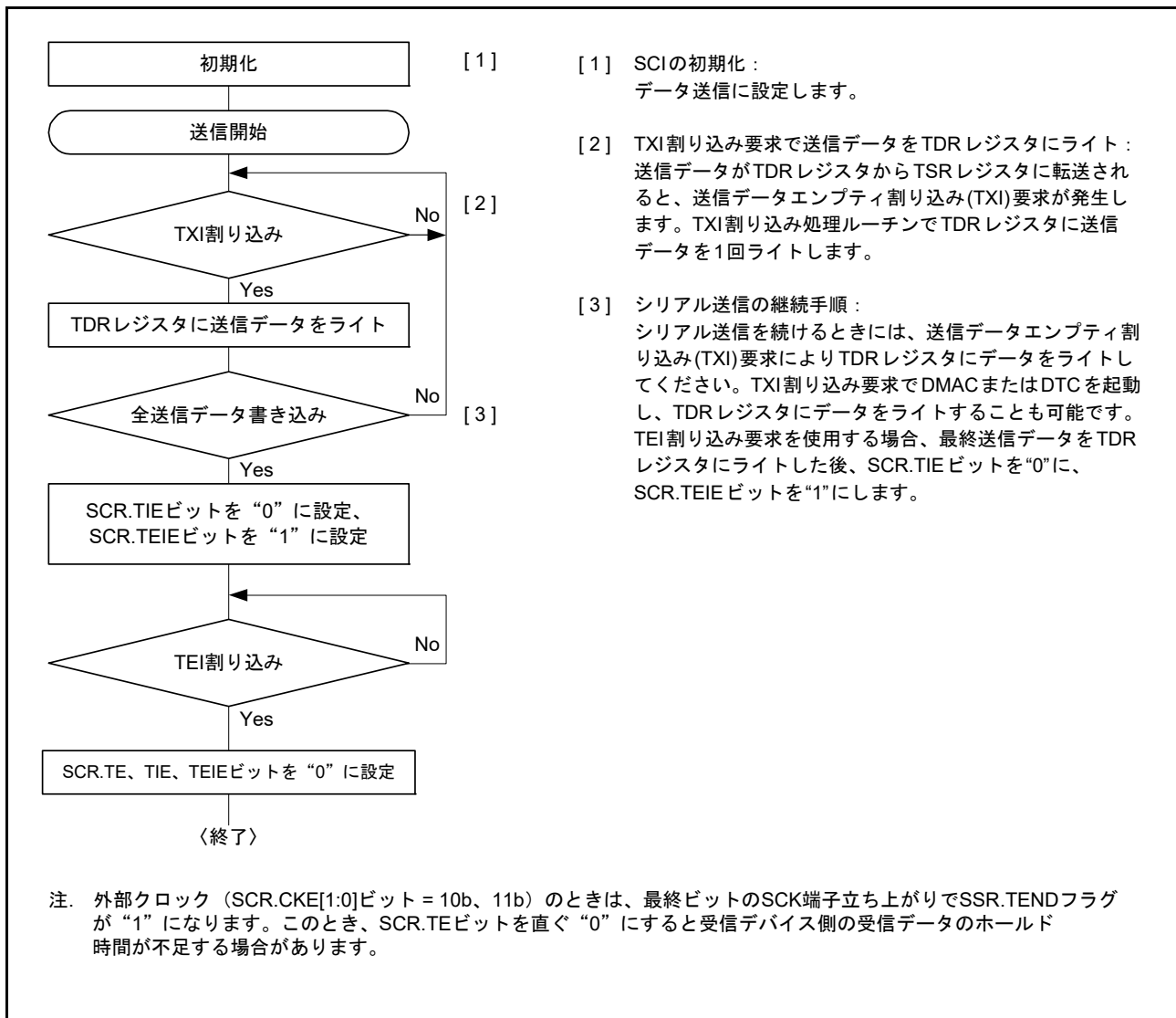
図 41.32 クロック同期式モードのシリアル送信のフローチャート例
