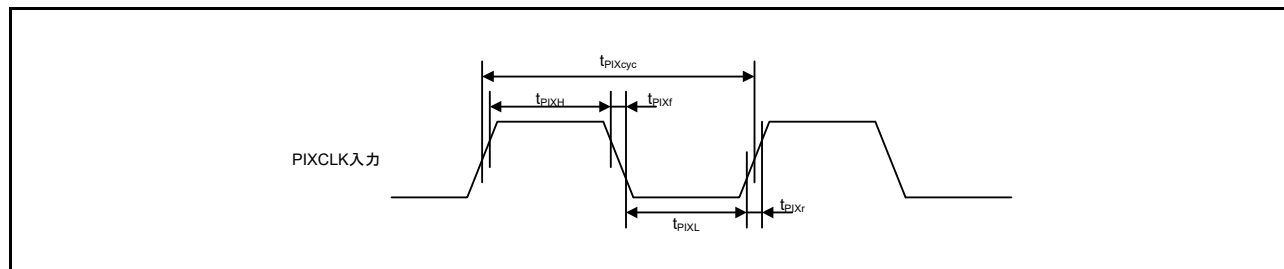
図 63.91 PDC 入力クロックタイミング
