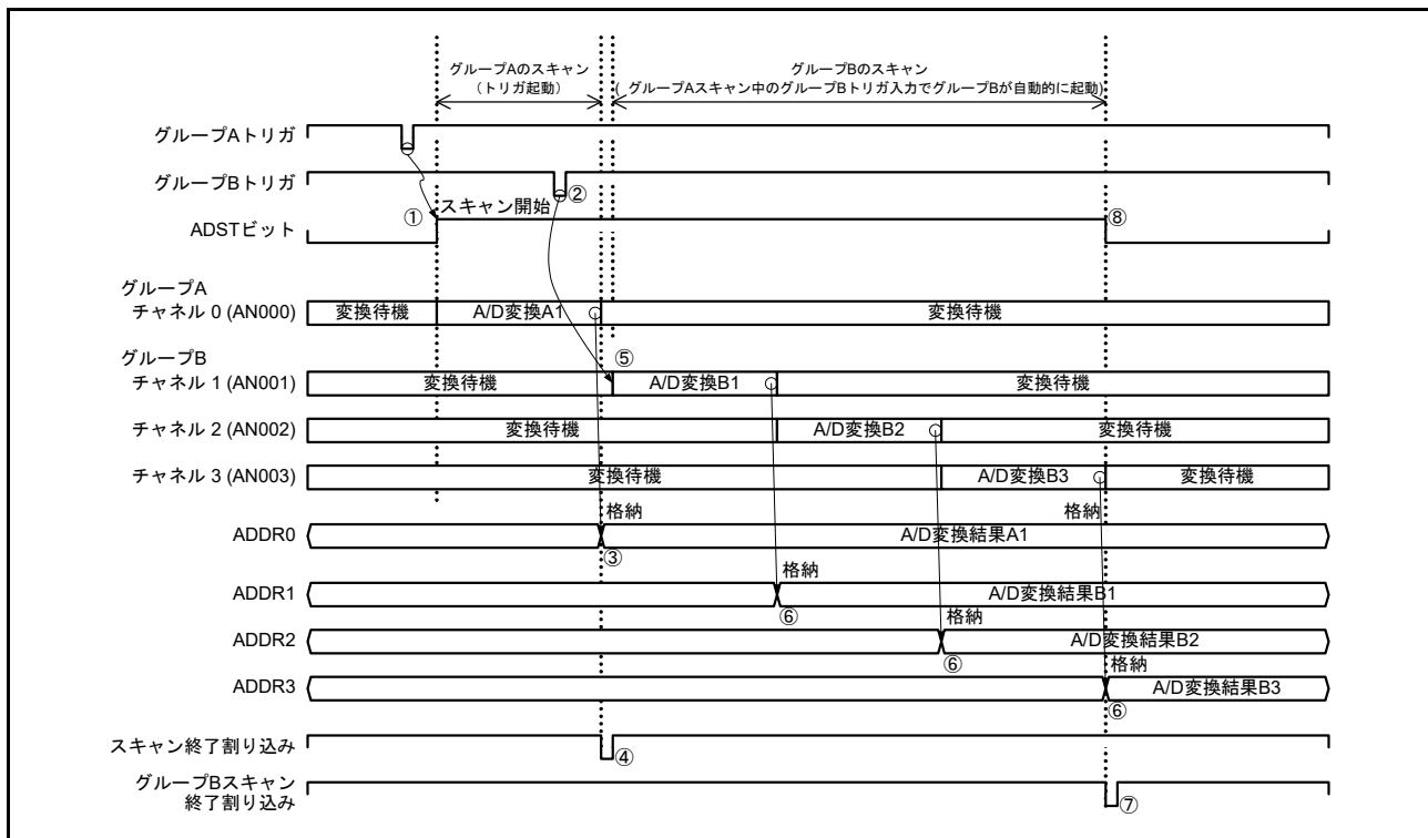
図 56.27 グループ優先動作の例3「グループA スキャン中のグループB トリガ入力」再スキャンあり (ADGSPCR.GBRSCN = 1, ADGSPCR.GBRP = 0, ADGSPCR.LGRRS = 0 設定時)
