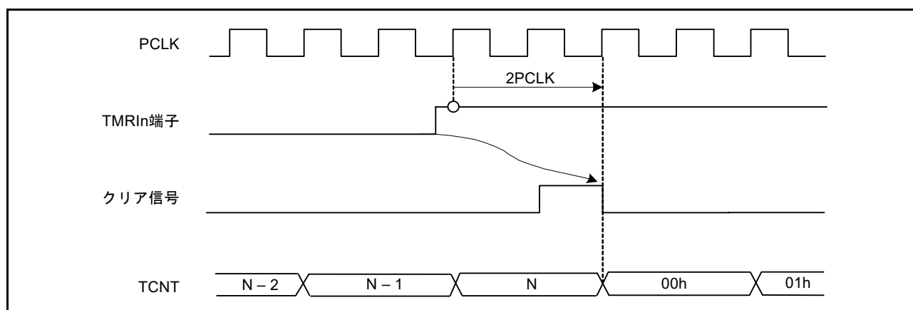
図 30.10 外部カウンタリセット信号によるクリアタイミング (立ち上がりエッジ)
