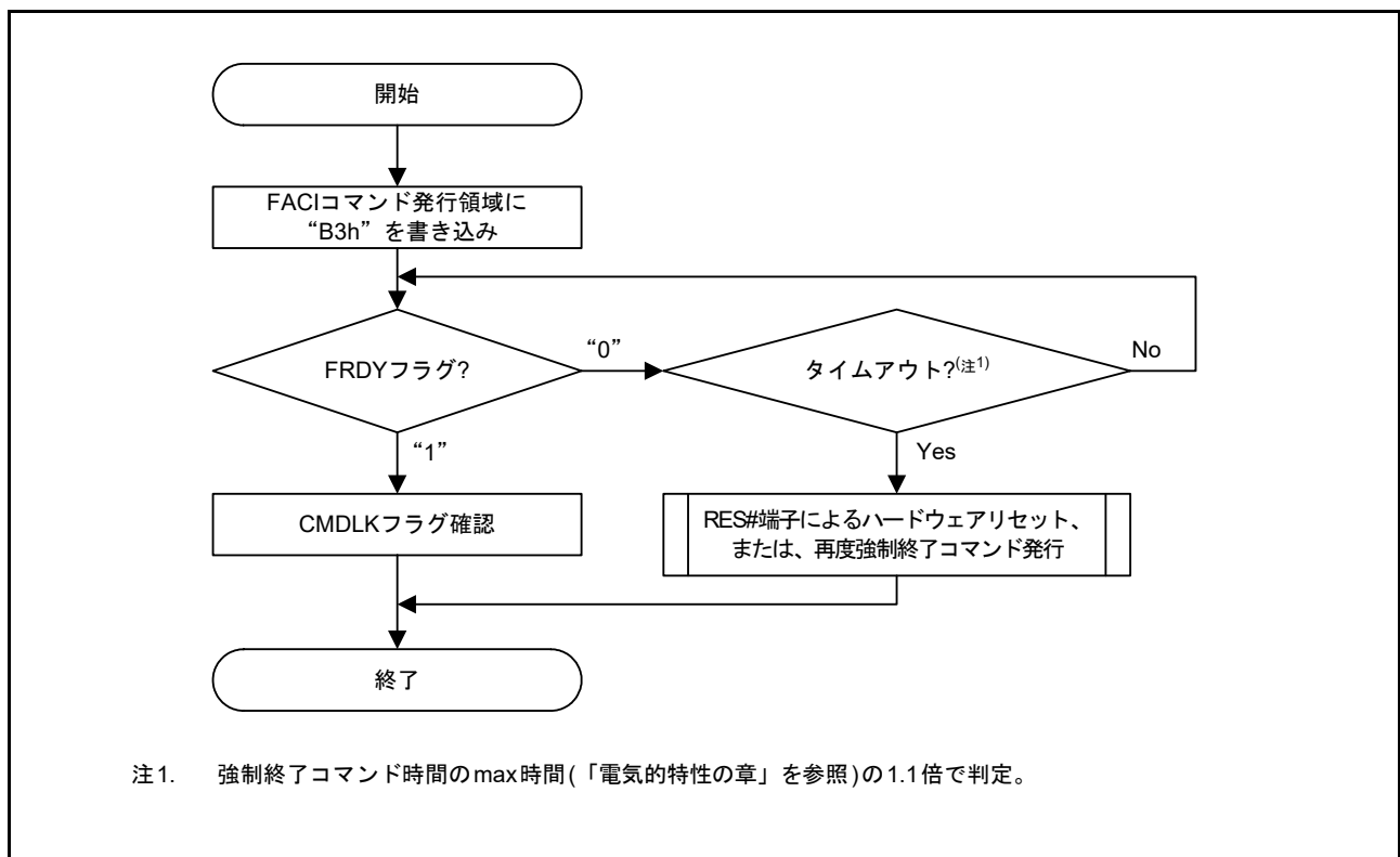
図 62.23 強制終了コマンドの使用方法
