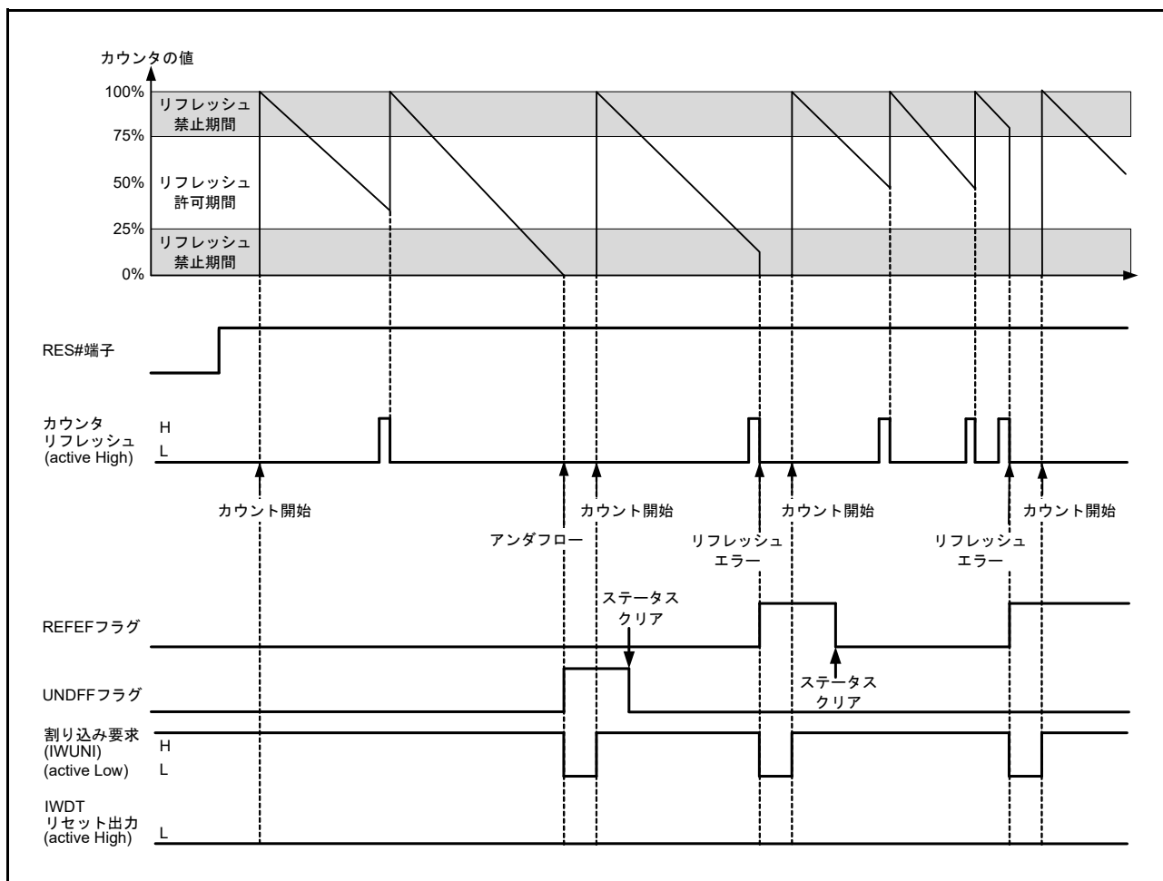
図 35.4 オートスタートモード動作例
