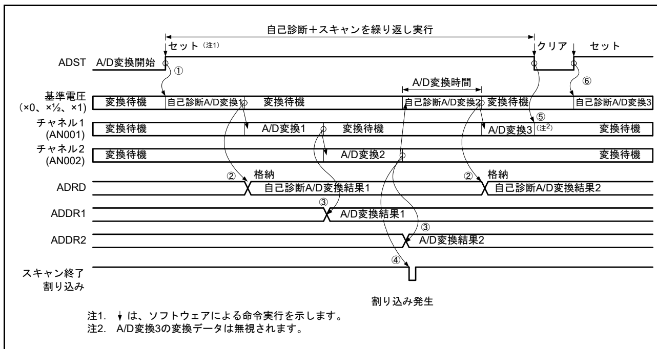
図 56.18 連続スキャンモードの動作例 (基本動作 : AN001, AN002 選択 + 自己診断)
