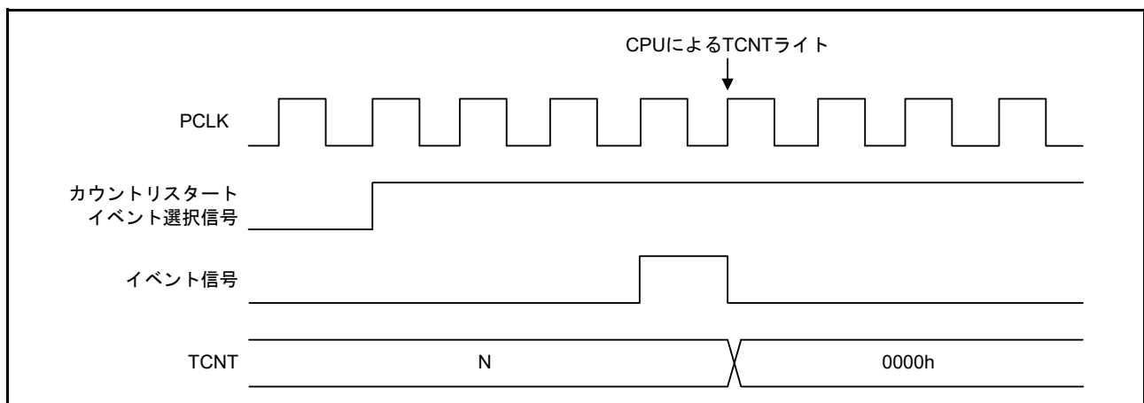
図 28.60 TCNTn へのライトサイクルとカウントリスタート動作の競合
