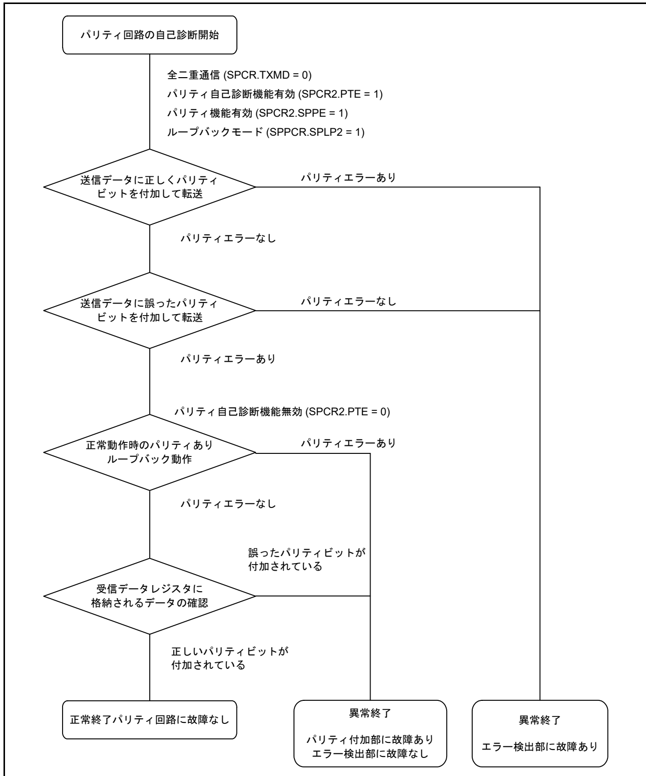
図 44.51 パリティ回路の自己判断フロー
