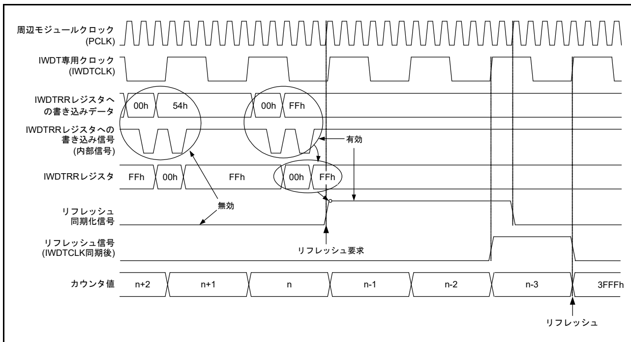
図 35.6 IWDT リフレッシュ動作波形 (IWDTCR.CKS[3:0] = 0000b、IWDTCR.TOPS[1:0] = 11b)
