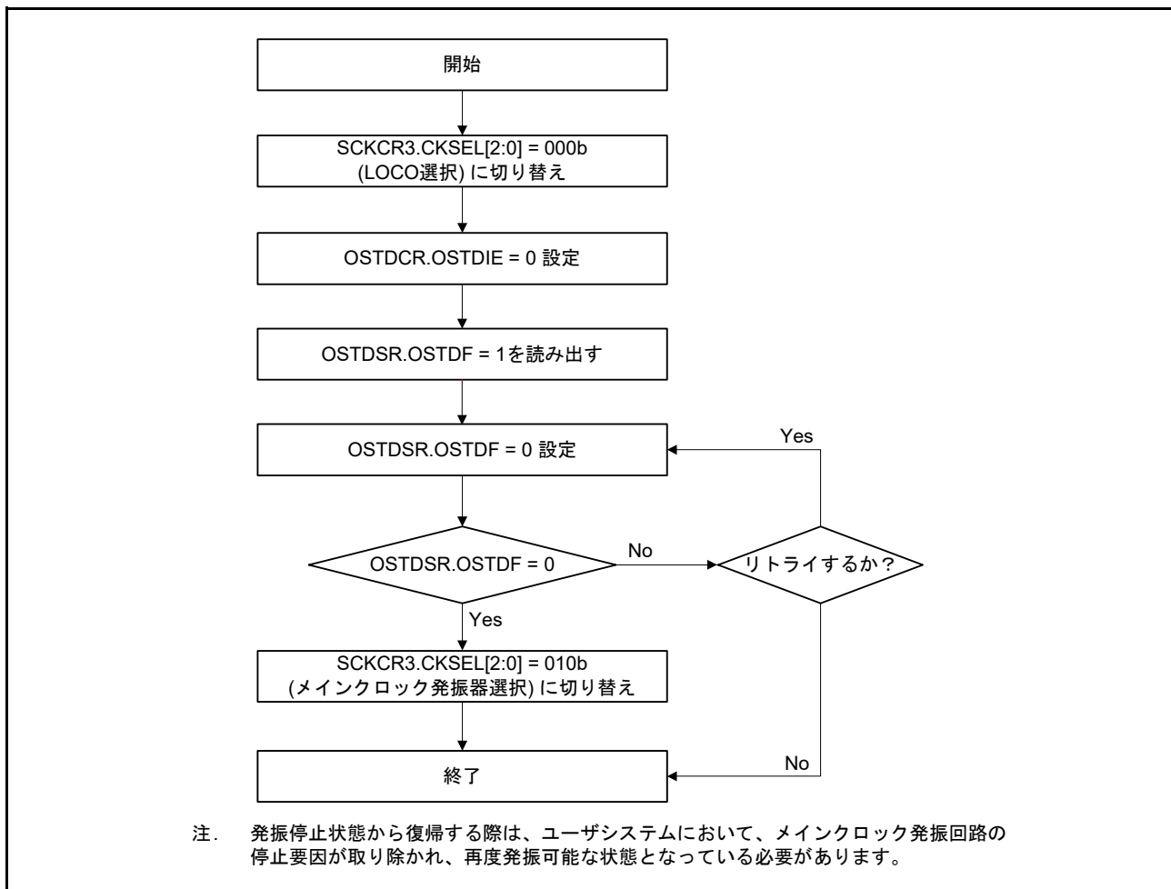
図 9.11 発振停止検出からの復帰のフローチャート例
