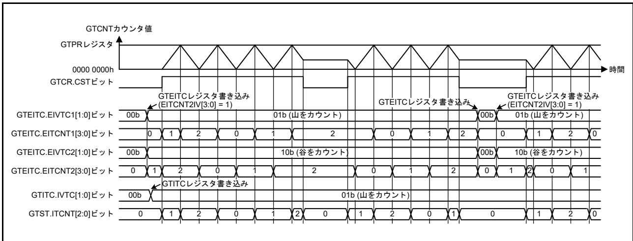
図 26.103 割り込み間引きのカウンタの動作
