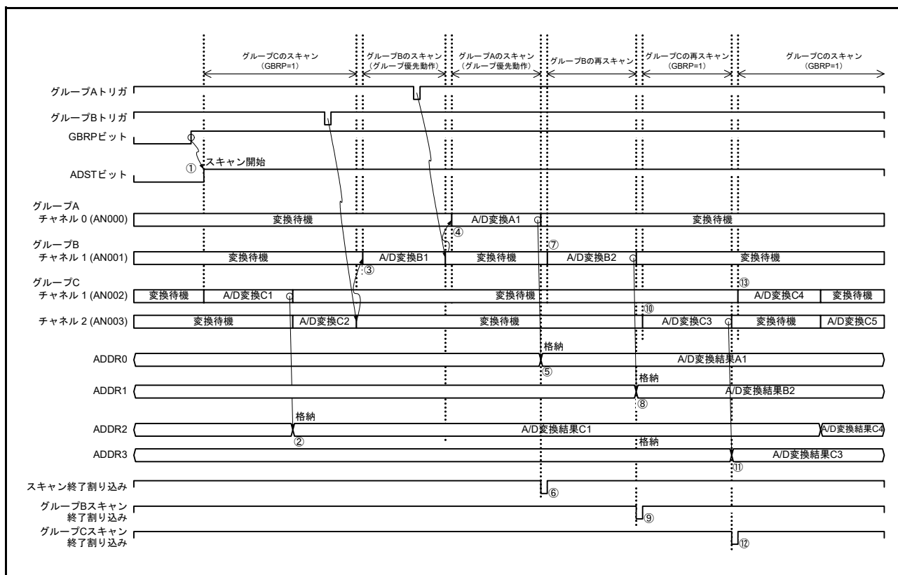
図 56.34 グループ優先動作の例 5「グループ C のシングルスキャン連続動作」 (ADGSPCR.GBRP = 1, ADGSPCR.LGRRS = 1 設定時)
