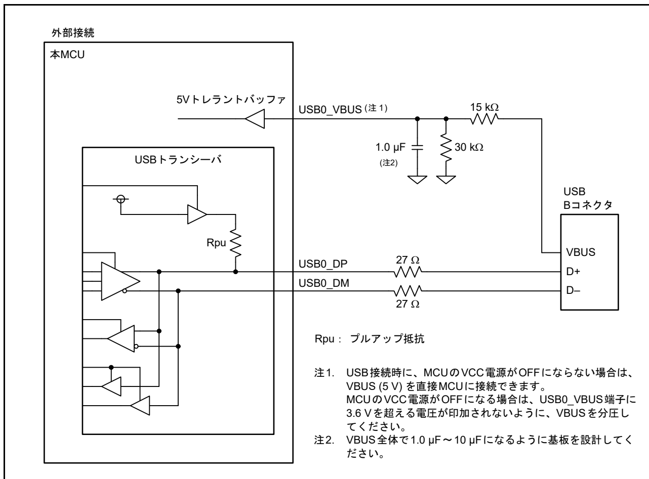
図 40.3 セルフパワー時のファンクションコントローラと USB コネクタとの接続例
