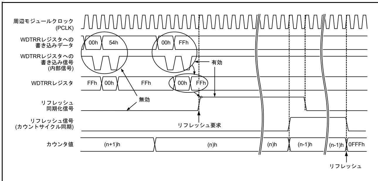
図 34.6 WDT リフレッシュ動作波形 (WDTCR.CKS[3:0] = 0100b、WDTCR.TOPS[1:0] = 01b)
