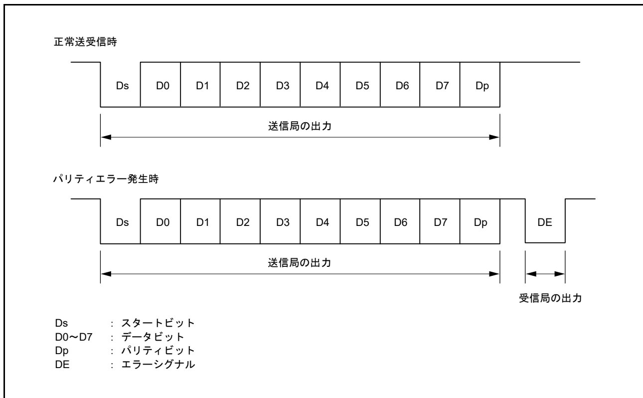
図 41.38 スマートカードインタフェースモードのデータフォーマット
