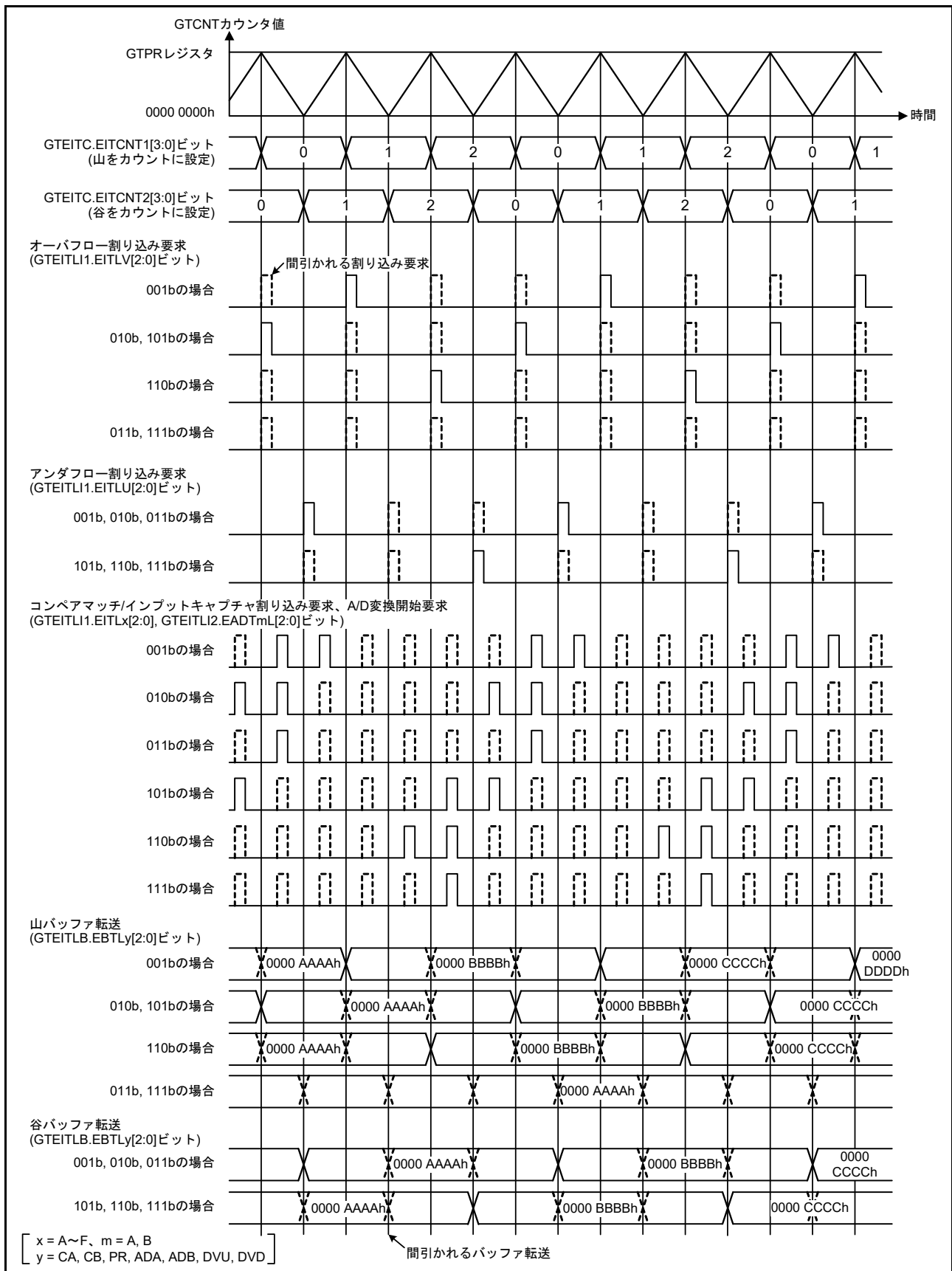
図 26.106 拡張割り込み間引き機能の動作例 (三角波、拡張割り込み間引き 1 間引き回数 2 で山をカウント、拡張割り込み間引き 2 間引き回数 2 で谷をカウント、拡張割り込み間引きカウンタ 2 初期値 "1" の場合)
