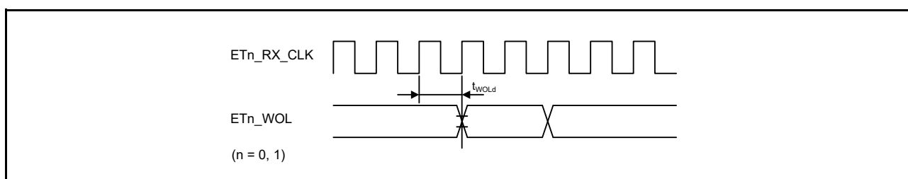
図 63.90 WOL 出カタイミング (MII)
