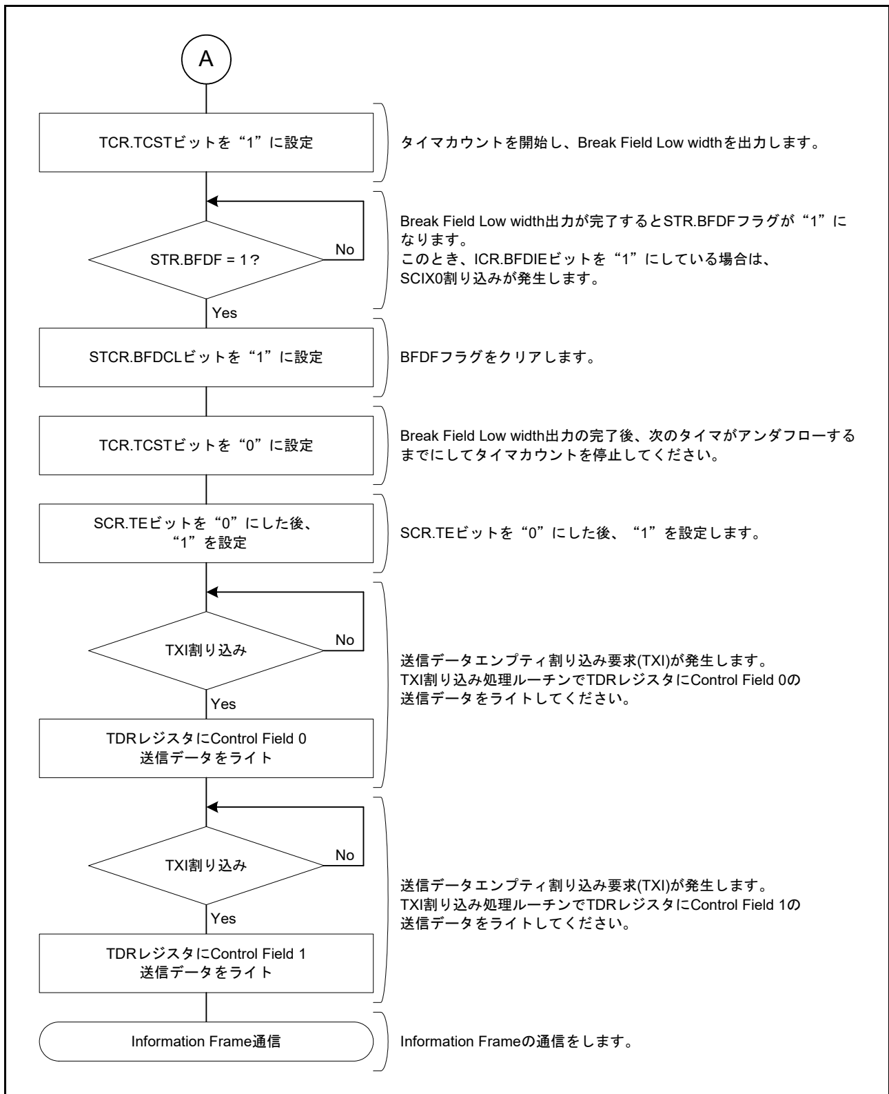
図 41.67 Start Frame 送信フローチャート例 (2)
