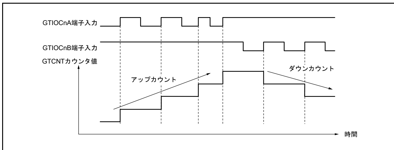
図 26.92 位相計数モード3の動作例 (n = 0 ~ 3)
