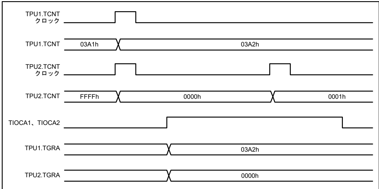
図 28.18 カスケード接続動作例 (1)
