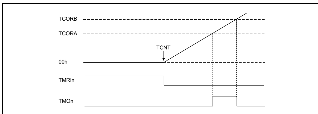
図 30.4 外部カウンタリセット信号入力例 (n = 0 ~ 3)
