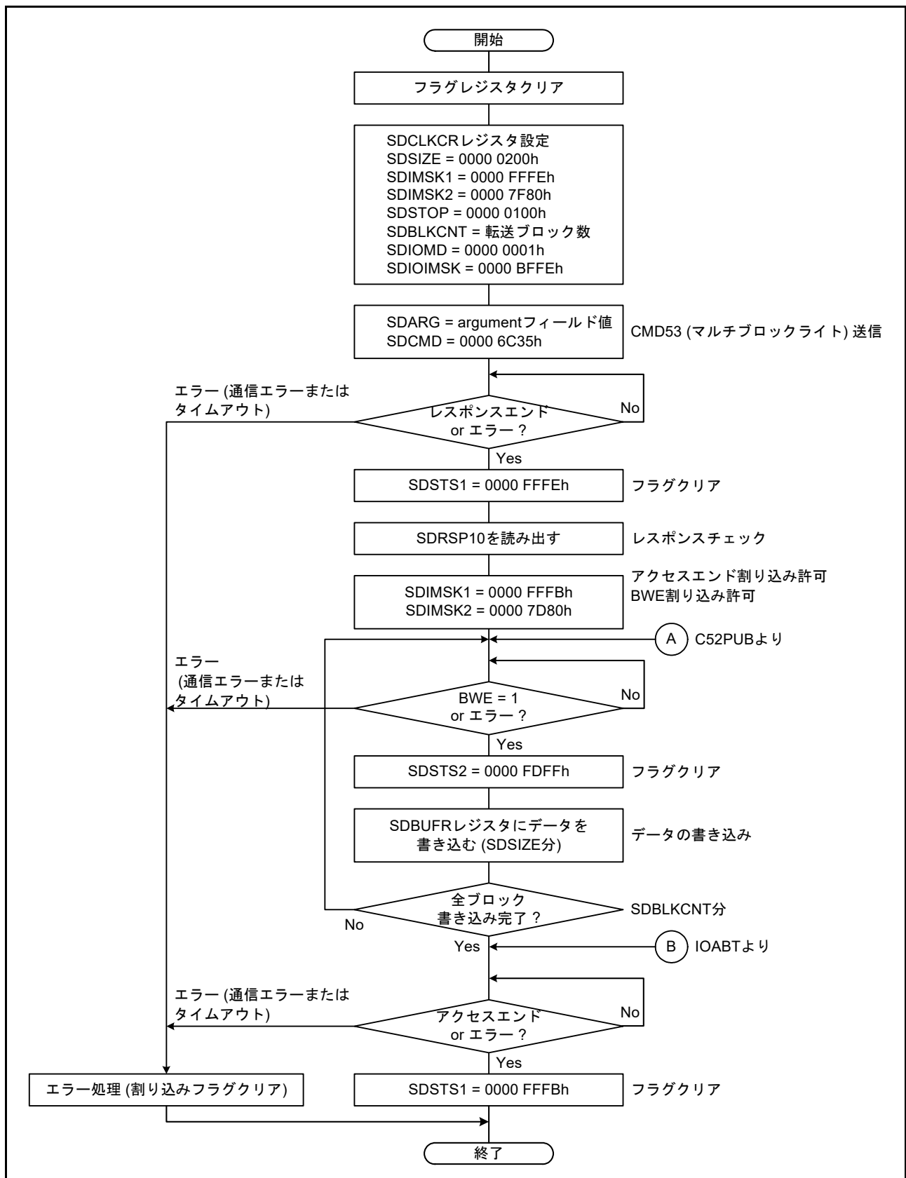
図 48.18 IO_RW_EXTENDED コマンド (CMD53/ マルチブロックライト) の送信例
