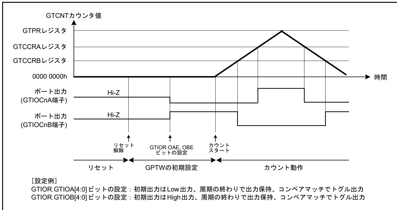
図 26.136 リセット後の端子設定例 (n = 0 ~ 3)
