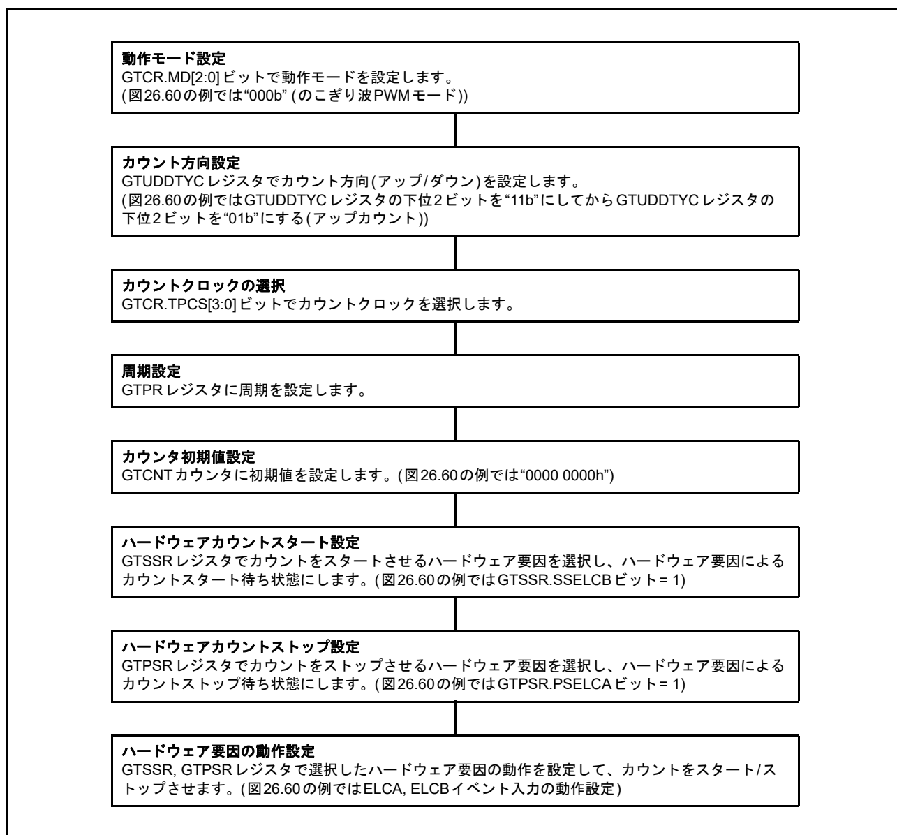
図 26.61 ハードウェア要因によるカウントストップ動作設定例
