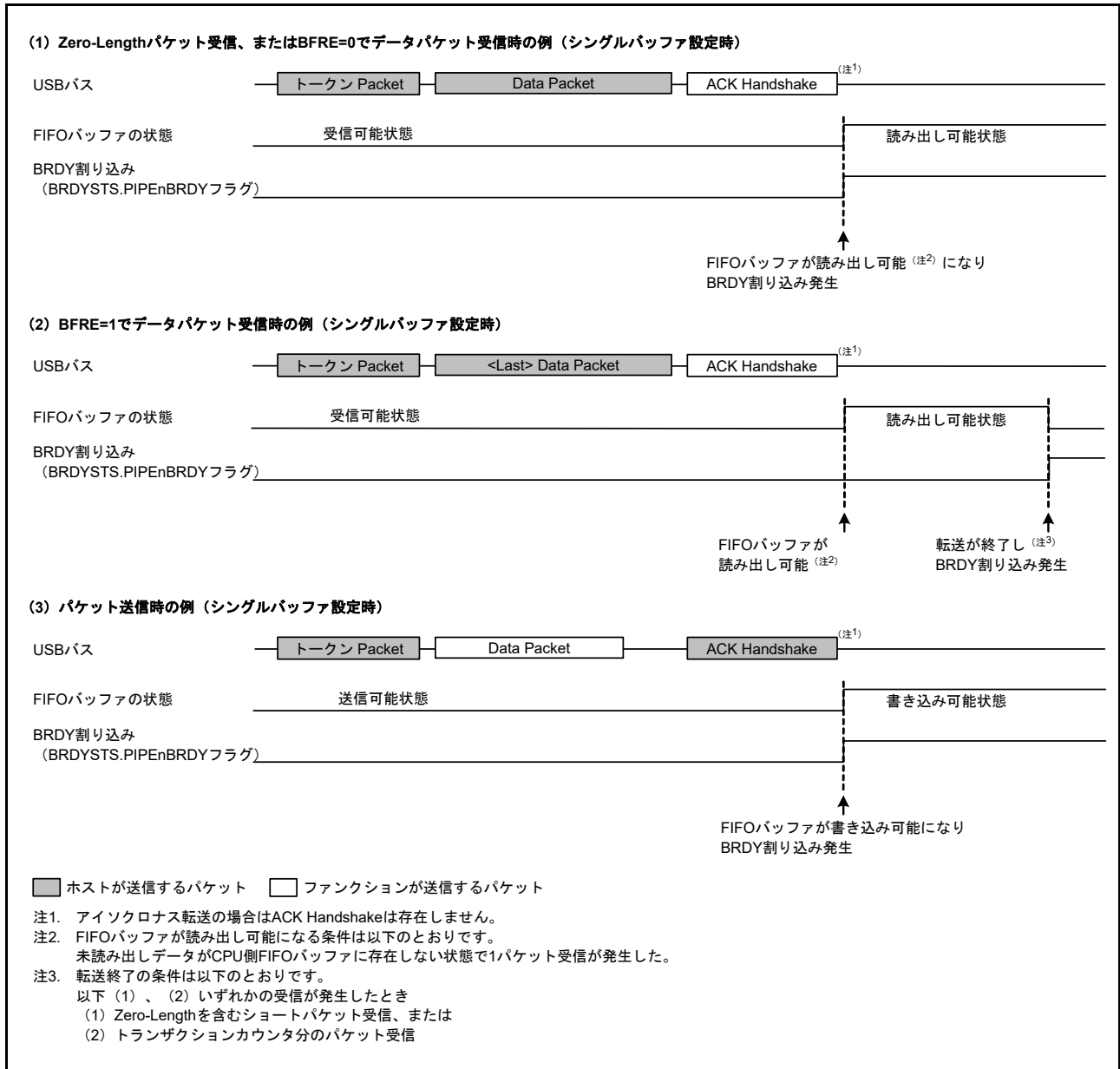
図 40.11 BRDY 割り込み発生タイミング図
