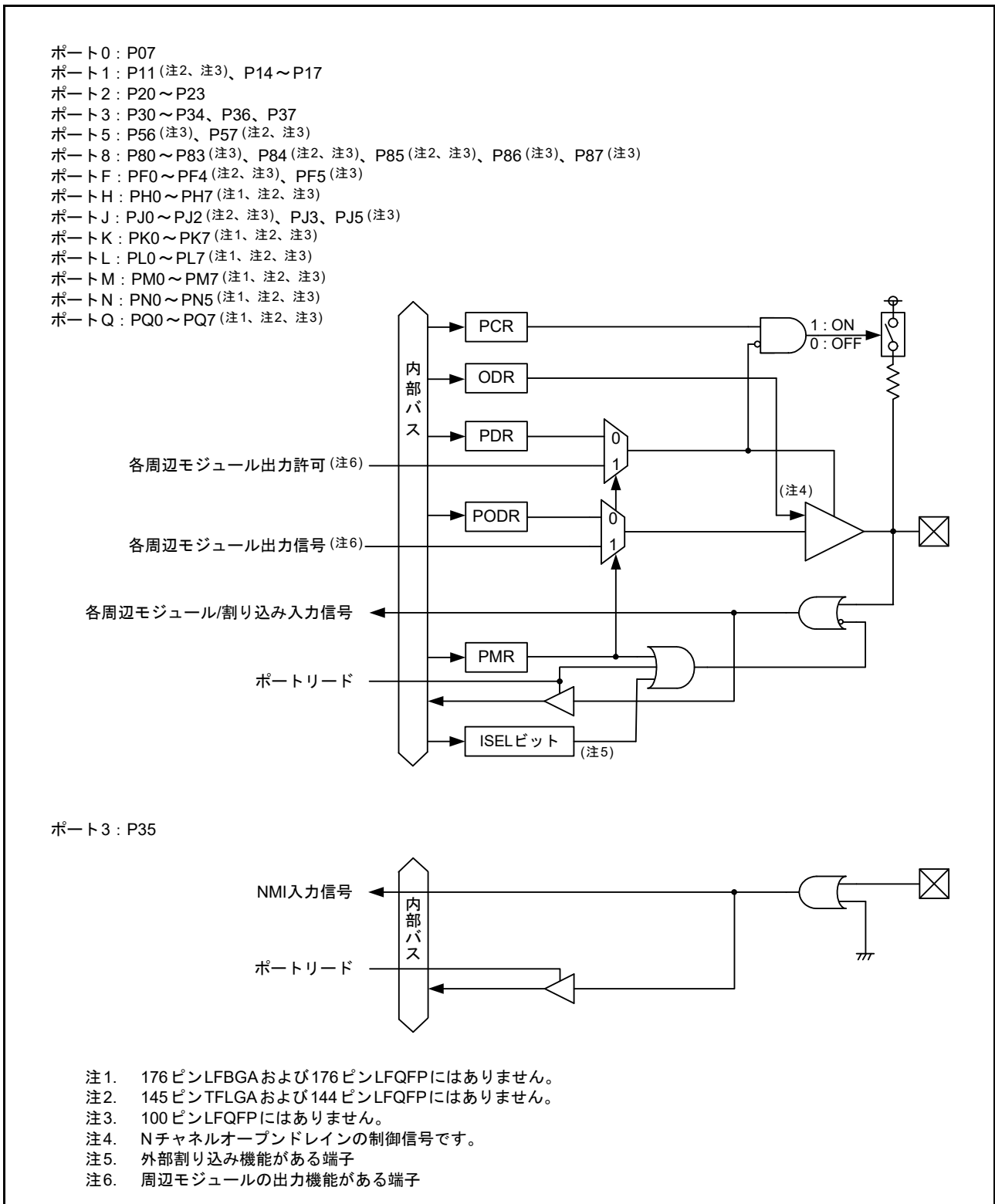
図 22.2 入出力ポートの構成 (2)
