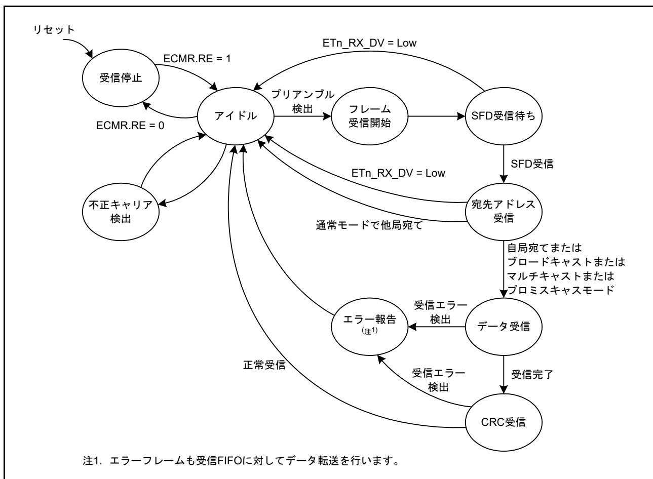
図 36.5 ETHERC 受信部状態遷移図
