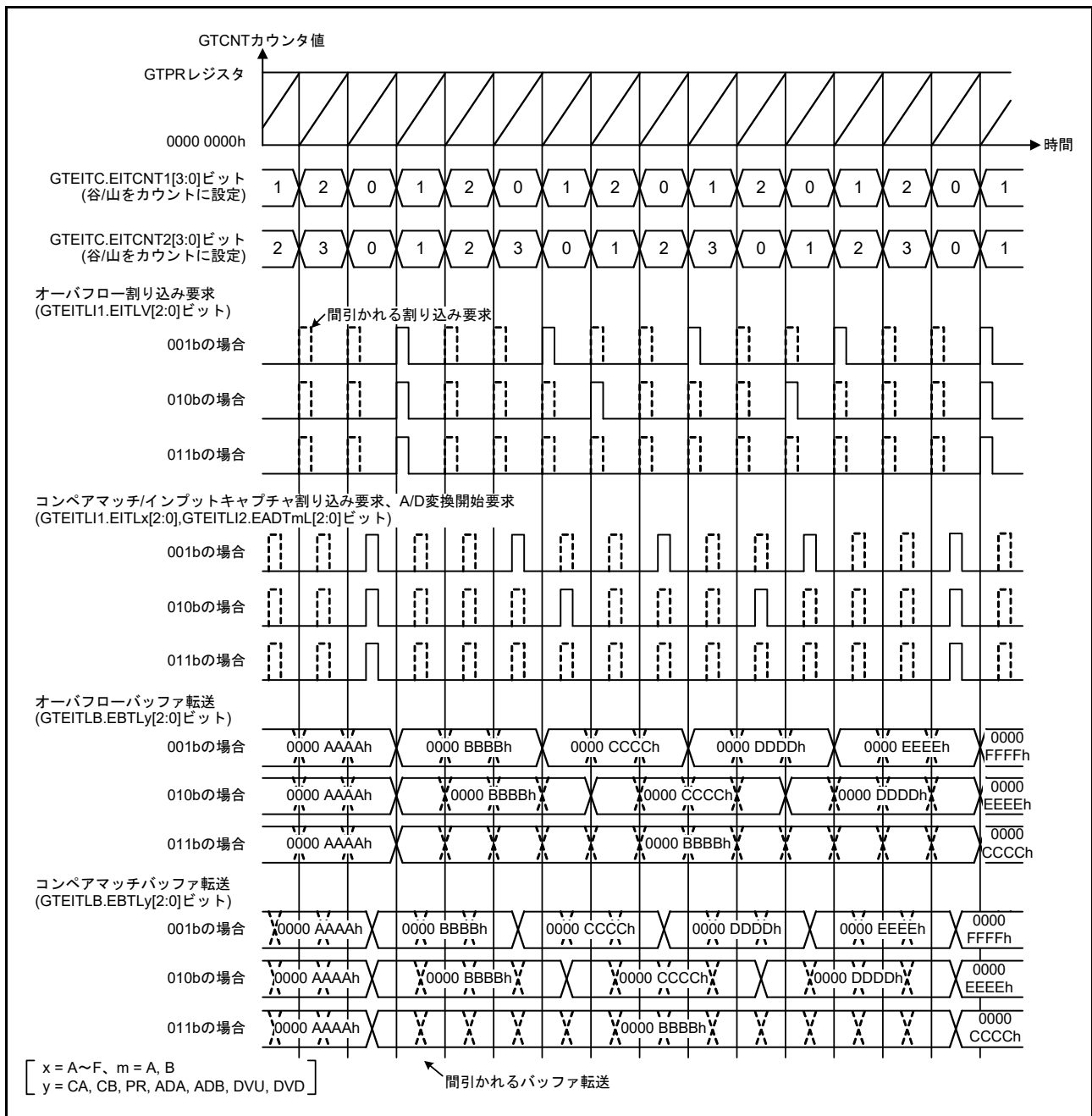
図 26.111 拡張割り込み間引き機能の動作例 ( のこぎり波アップカウント、拡張割り込み間引き 1 間引き回数 2 でオーバーフローをカウント、拡張割り込み間引き 2 間引き回数 3 でオーバーフローをカウント、拡張割り込み間引きカウンタ 2 初期値 "0"、GTEITC.EITCNTk ビット (k = 1, 2) が "0" 以外の期間で間引く場合)
