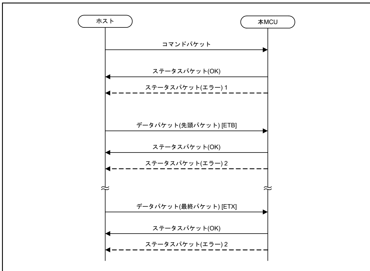
図 62.46 プログラムコマンドの通信シーケンス
