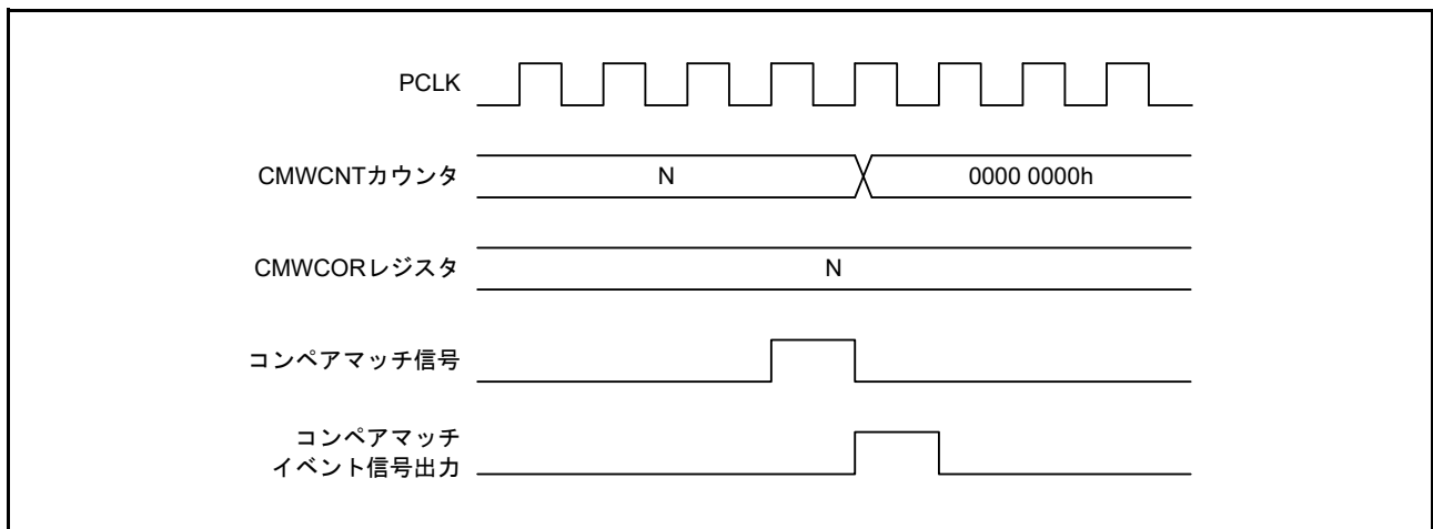
図 32.16 コンペアマッチイベント発行タイミング
