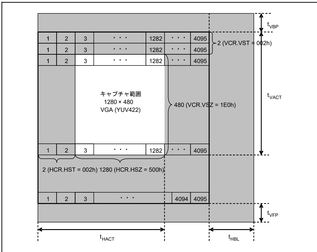
図 50.10 VCR レジスタ、HCR レジスタ設定とキャプチャ範囲 (VCR = 01E0 0002h, HCR = 0500 0002h)
