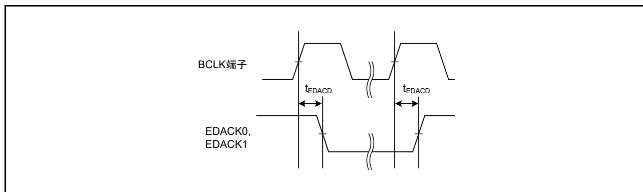
図 63.34 EDACK0、EDACK1 シングルアドレス転送タイミング (SDRAM 領域)
