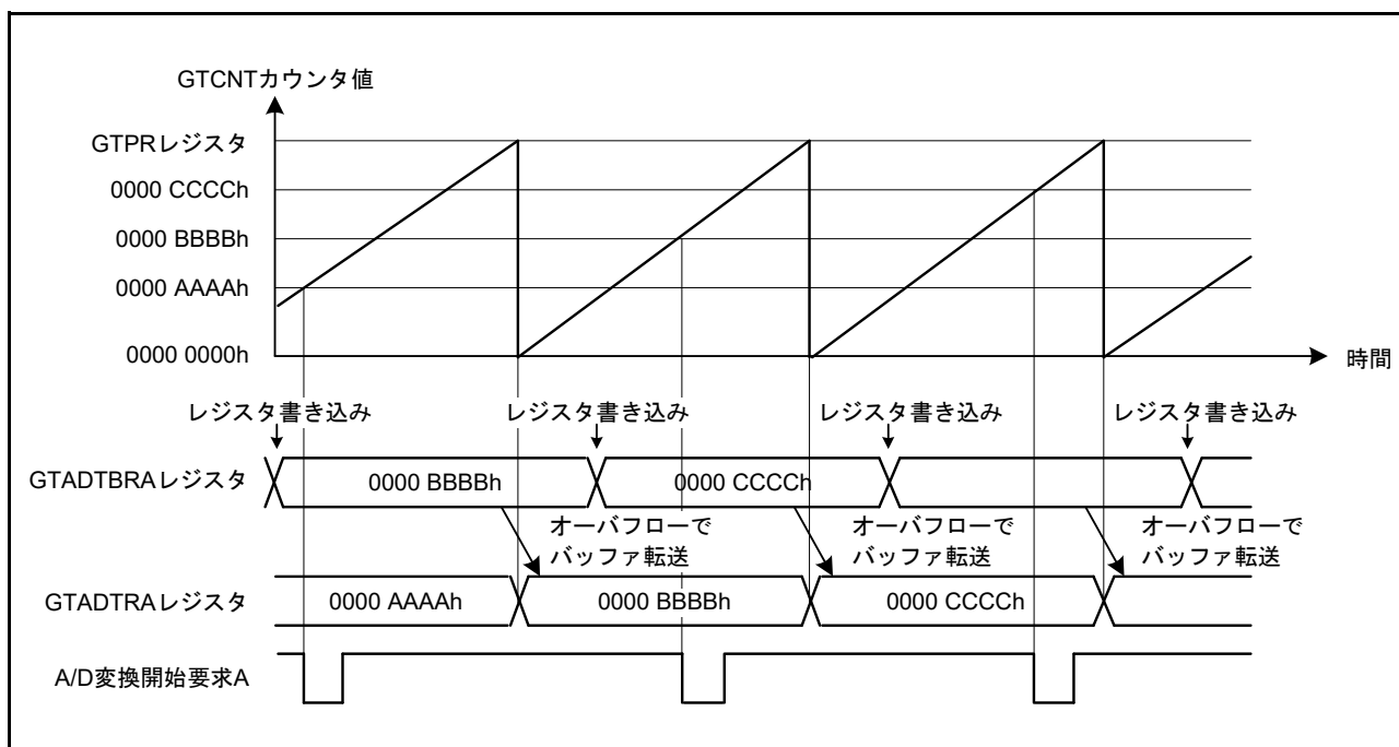
図 26.33 GTADTRA, GTADTRB レジスタのバッファ動作例 (のこぎり波でアップカウント、アップカウントで A/D 変換開始要求発生の場合)
