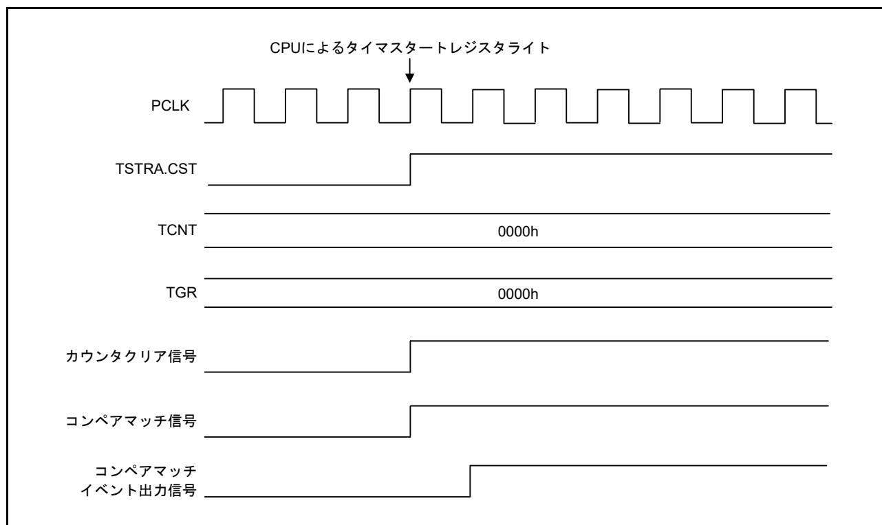
図 28.63 コンペアマッチイベント出力信号の連続出力
