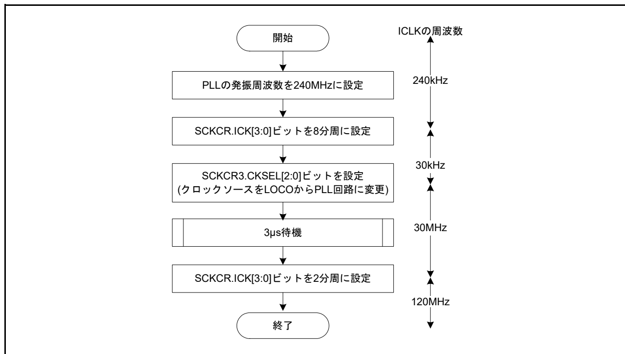
図 9.16 ICLK を LOCO クロック (240kHz) から PLL クロック (240MHz) の 2 分周設定で 120MHz に変更する変更手順例
