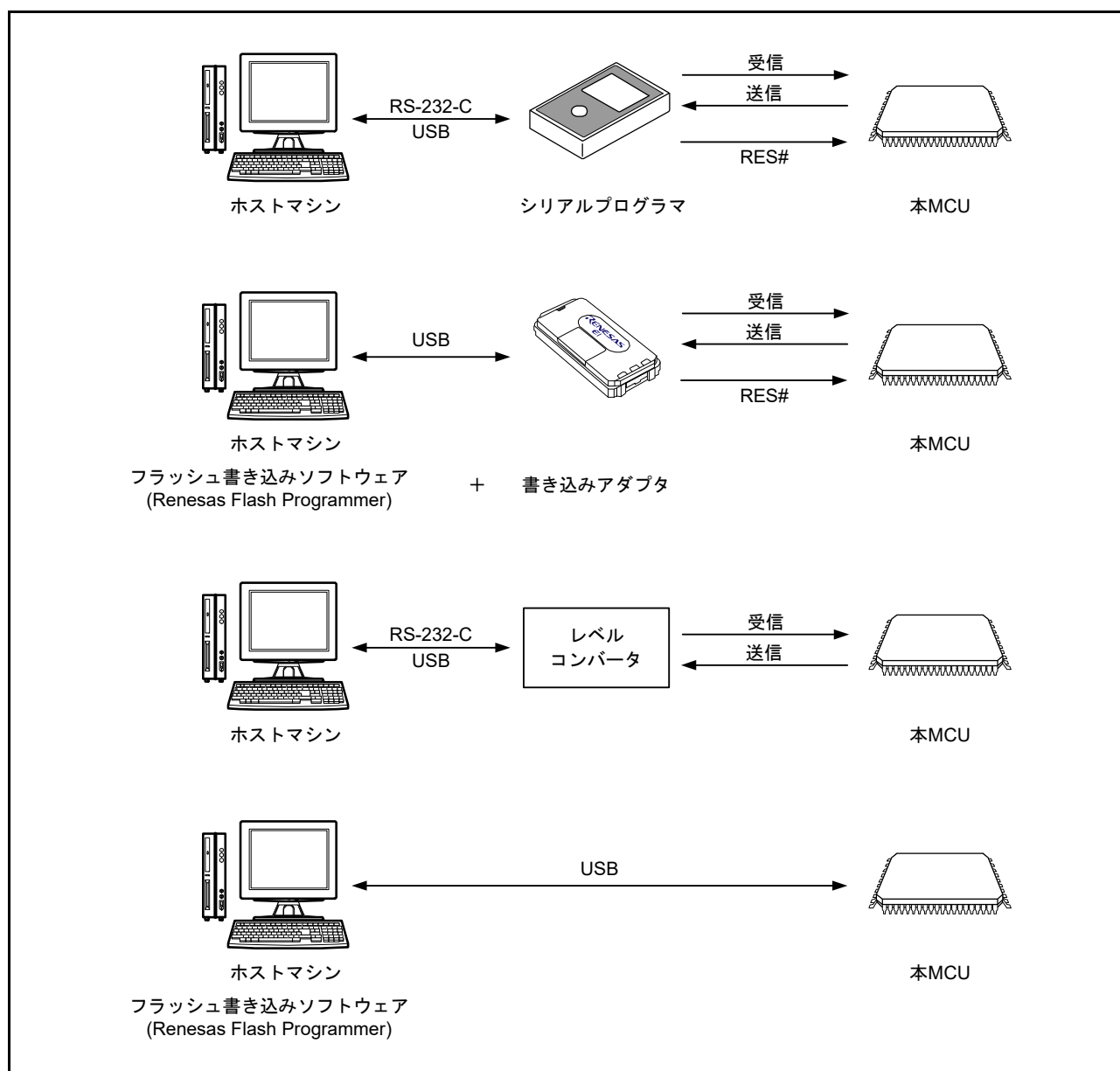
図 62.53 フラッシュメモリを書き換えるための環境
