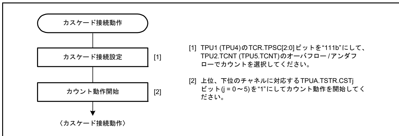
図 28.17 カスケード接続動作設定手順例
