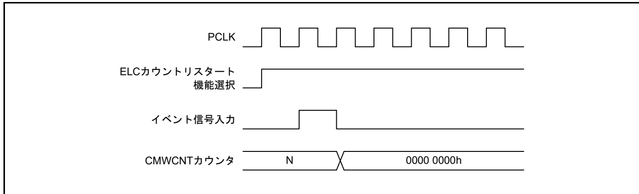
図 32.19 イベント受け付けによるカウントリスタート動作
