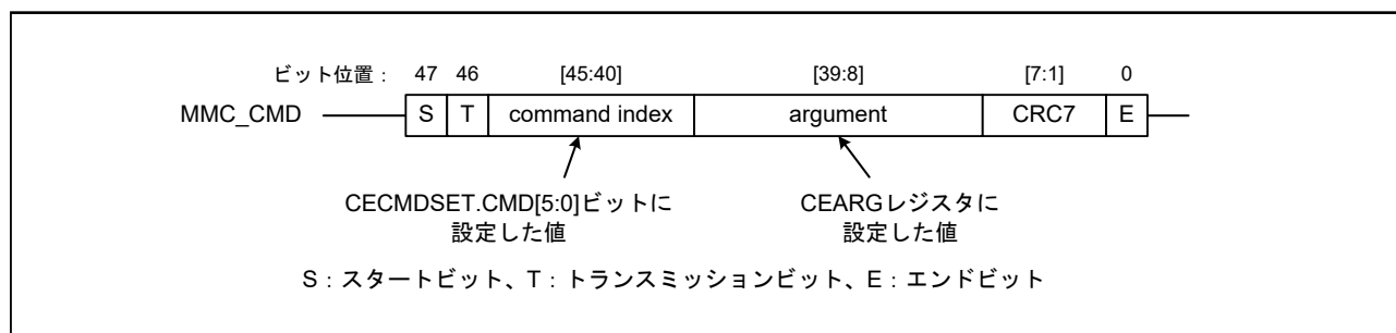
図 49.2 コマンドのフォーマット
