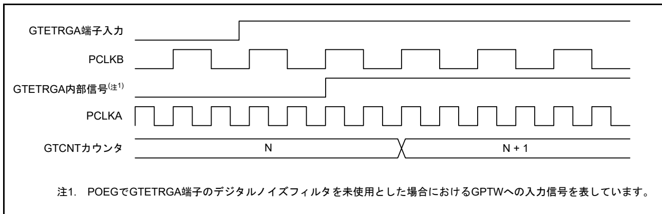
図 26.6 イベントカウント動作例 (GTETRGA 端子入力の立ち上がりによるアップカウント)
