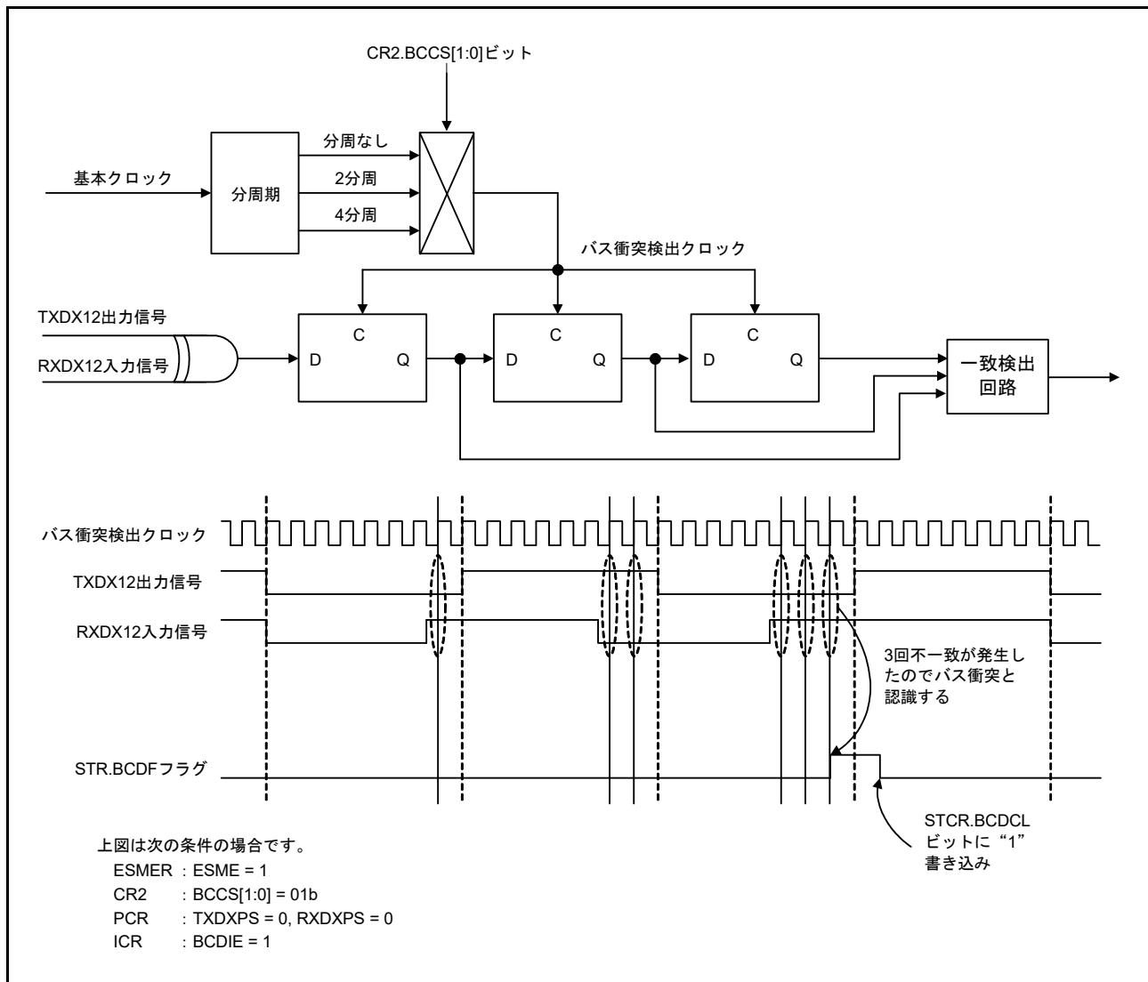
図 41.73 バス衝突検出機能の動作例
