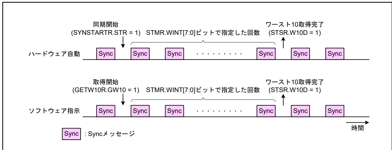
図37.28 傾き差分値収集の概念
