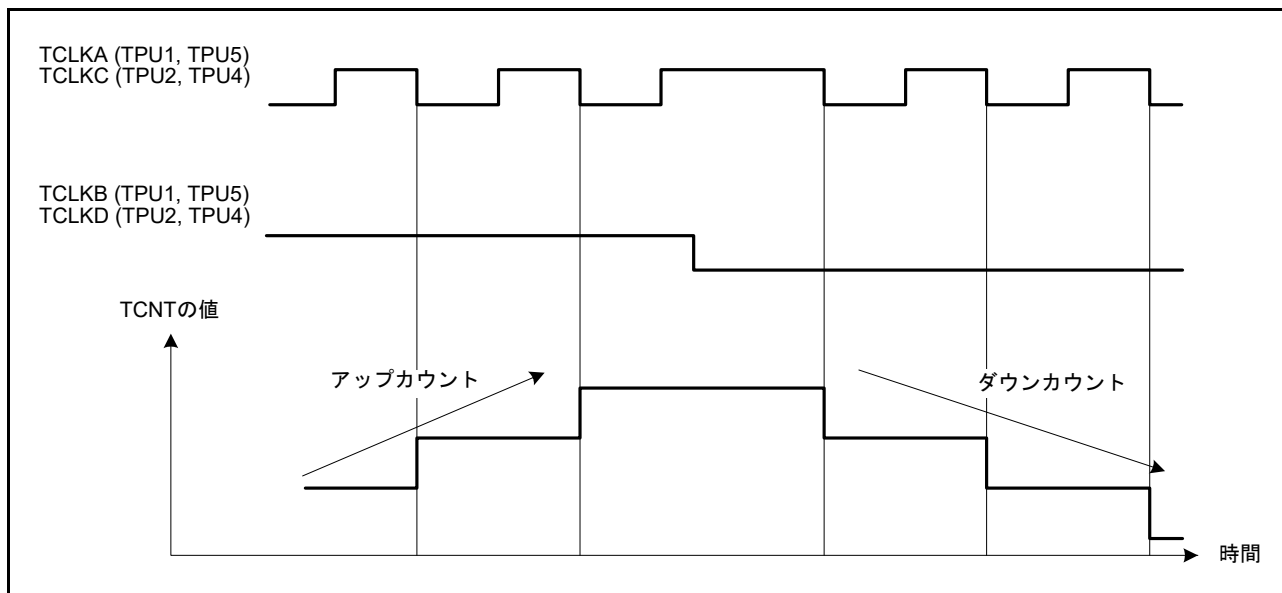
図 28.26 位相計数モード2の動作例
