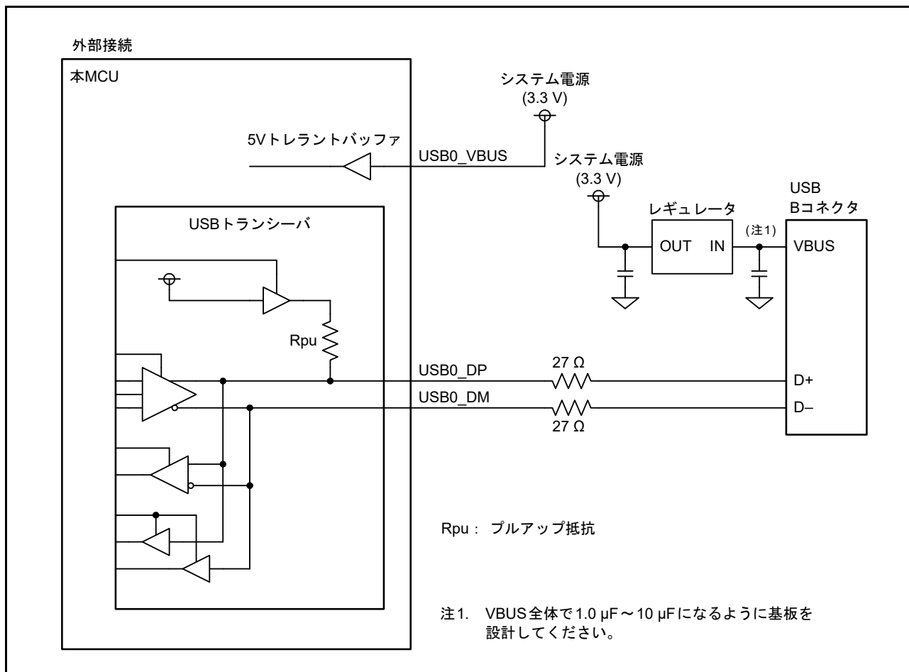
図 40.5 バスパワー時のファンクションコントローラと USB コネクタとの接続例
