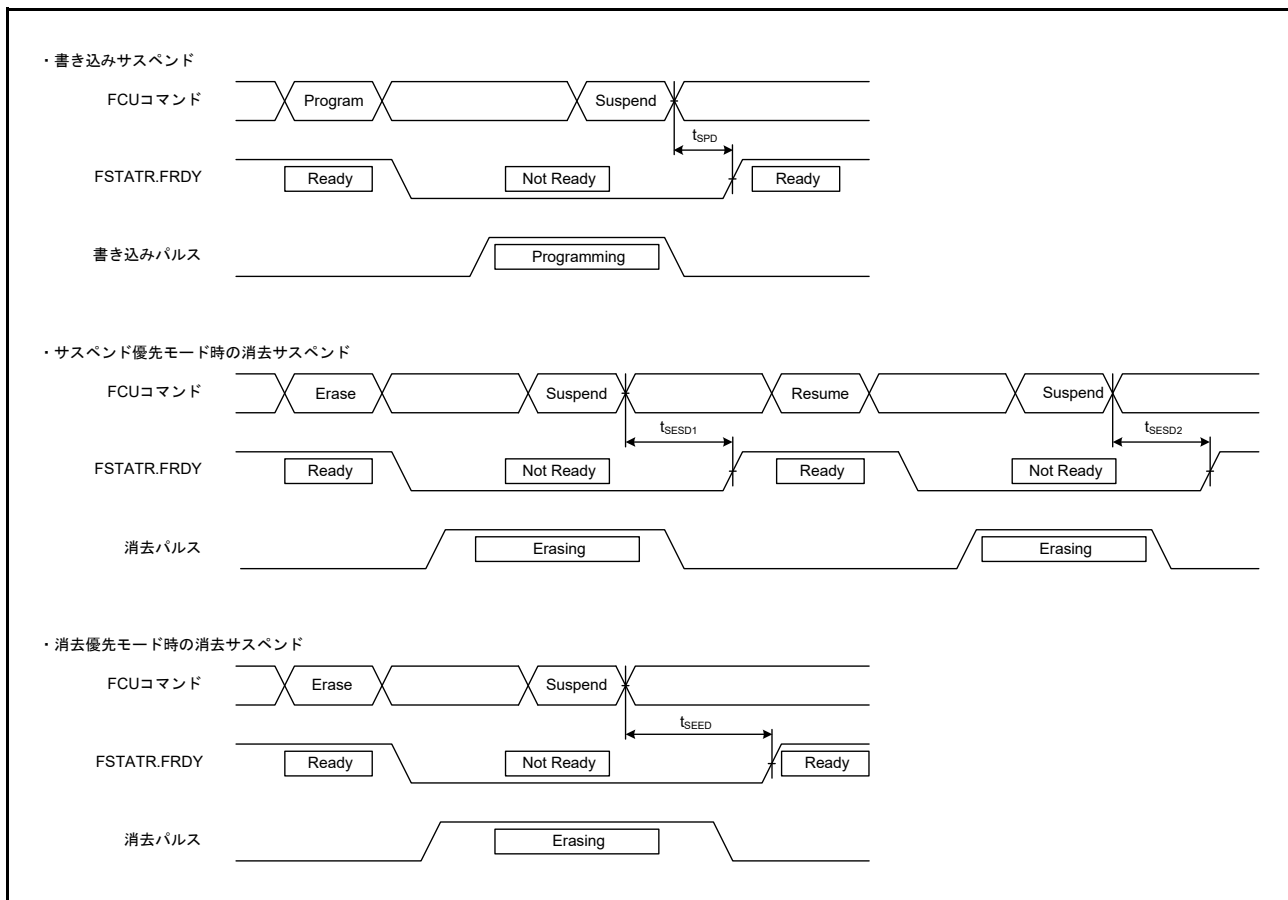
図 63.108 フラッシュメモリプログラム/イレーズサスペンドタイミング
