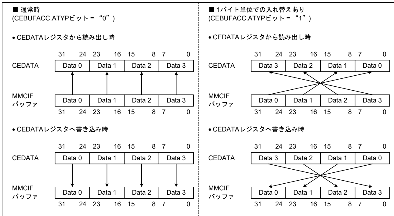
図 49.7 1バイト単位でのデータ入れ替えの概念 (32ビットアクセス)
