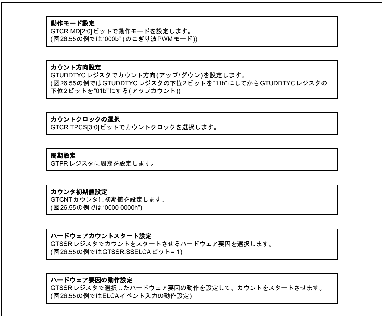
図 26.56 ハードウェア要因によるカウントスタート動作設定例
