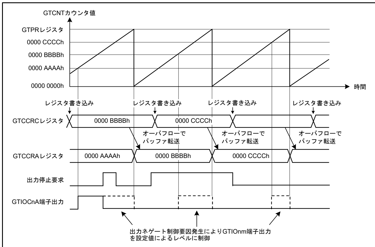
図 26.125 GTIOCnm 端子出力の出力ネゲート制御動作例 ( のこぎり波でアップカウント、バッファ動作、アクティブレベルは High (GTCCRA レジスタのコンペアマッチで High 出力、周期の終わりで Low 出力)、出力ネゲート時に Low 出力 ) (n = 0 ~ 3, m = A, B)
