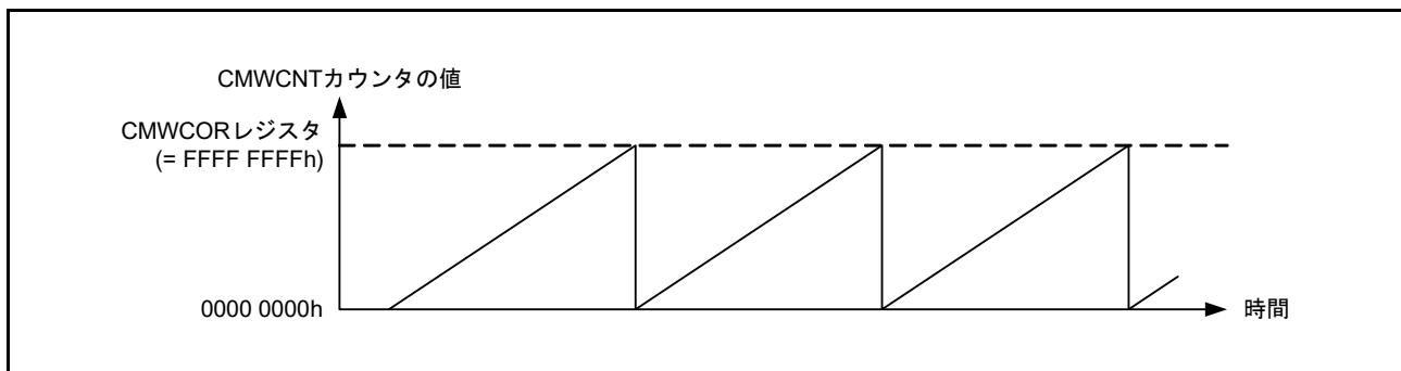
図 32.5 コンペアマッチ動作例 (オーバーフロー検出時)
