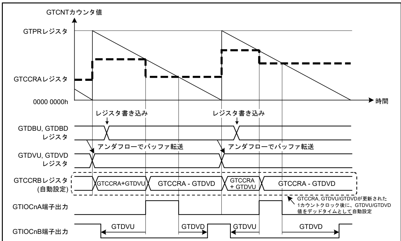
図 26.48 デッドタイム自動設定機能の動作例 ( のこぎり波ワンショットパルスモード、ダウンカウント、GTDVU/GTDVD レジスタはバッファ動作、アクティブレベルは High の場合 ) (n = 0 ~ 3)
