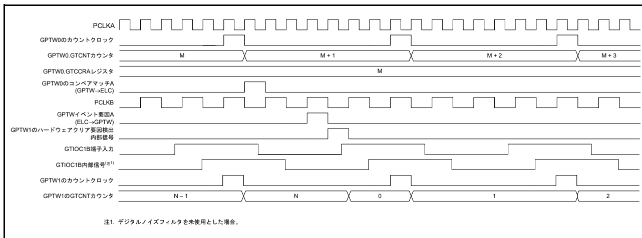
図 26.76 ELCA イベント入力によるカウンタクリア動作タイミング例 (ハードウェア要因によるカウント動作時)
