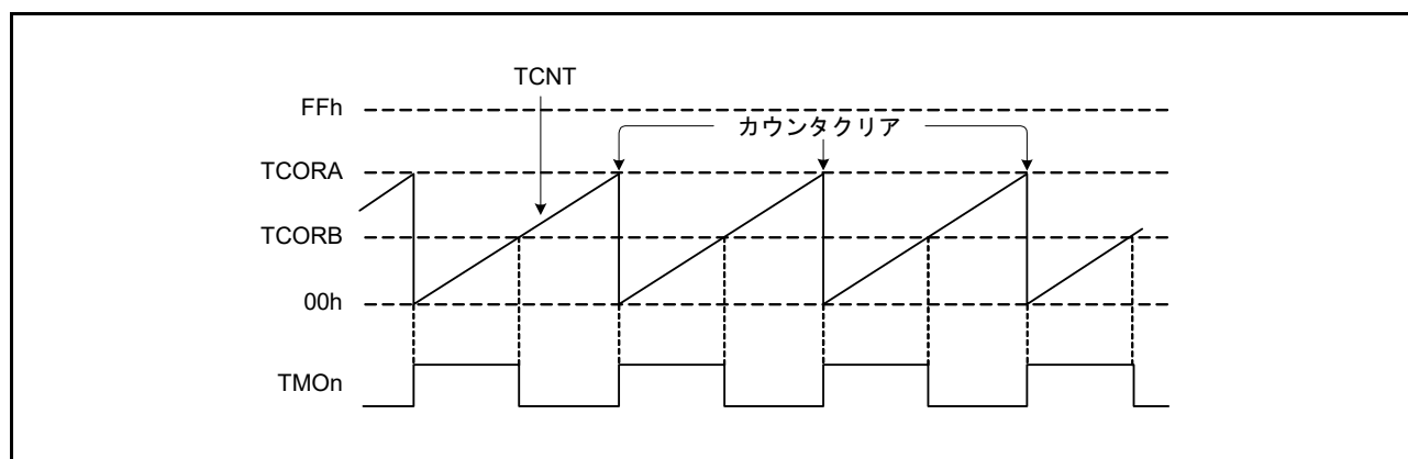
図 30.3 パルス出力例 (n = 0 ~ 3)
