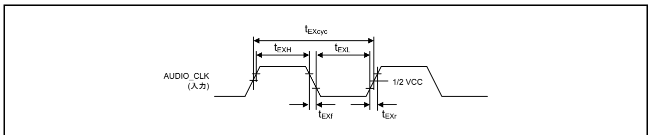
図63.73 クロック入力タイミング
