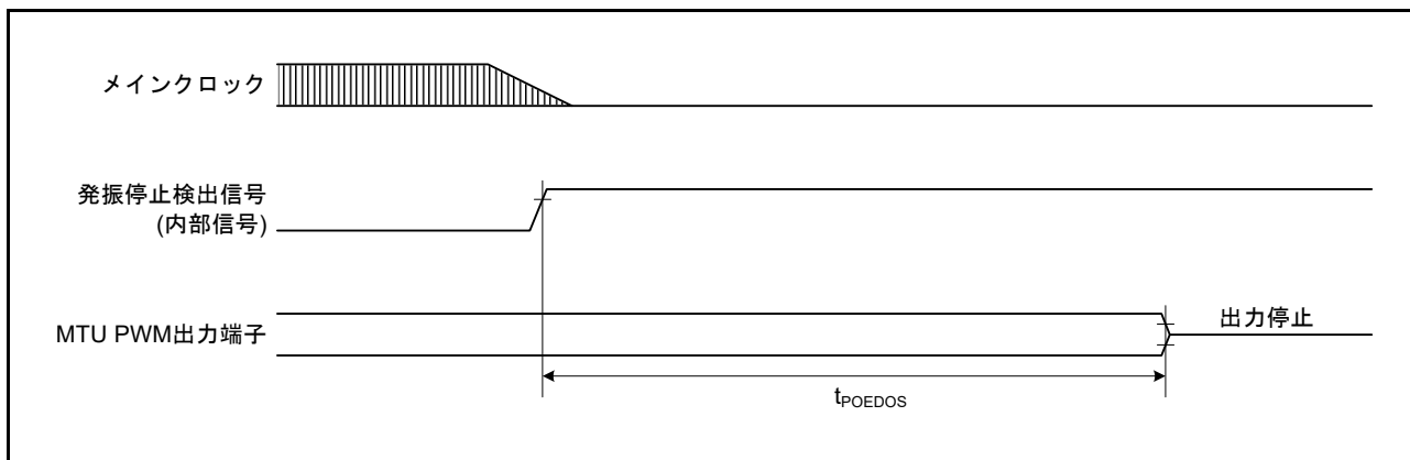
図 63.46 POE 出力ディセーブル時間 (発振停止検出)
