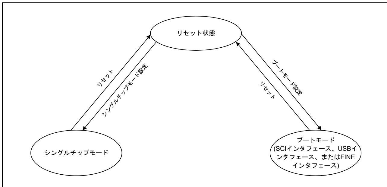
図 62.6 フラッシュメモリに関するモード遷移図
