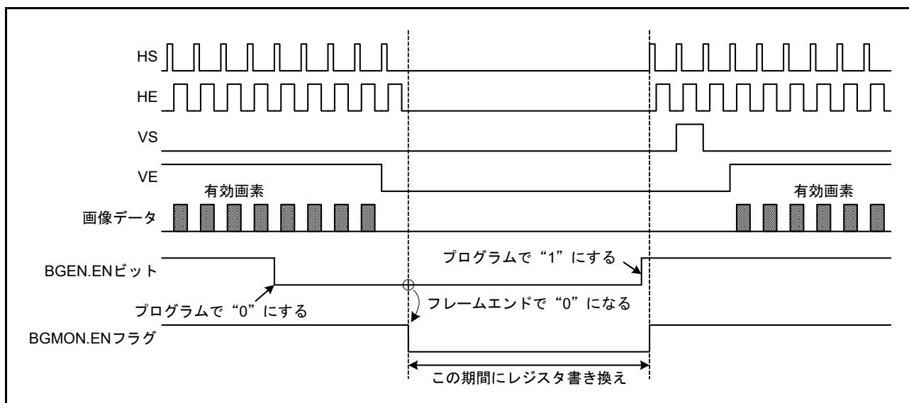
図 51.23 正常動作時の停止と再開
