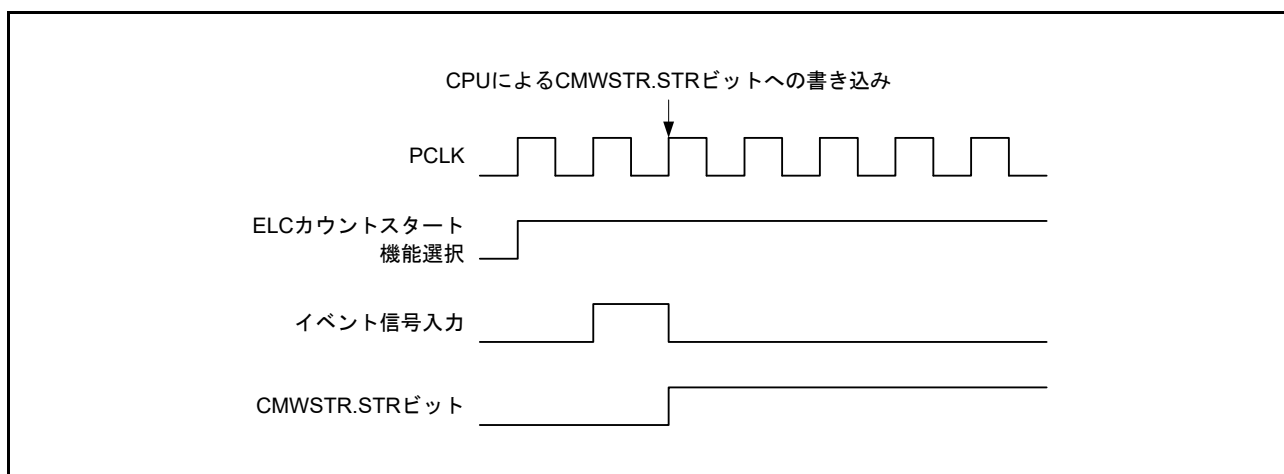
図 32.20 カウントスタート動作でのイベント受け付けとレジスタアクセスの競合
