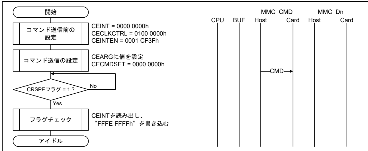
図 49.11 レスポンス受信およびデータ転送を行わないコマンドの送信例 (CMD0)
