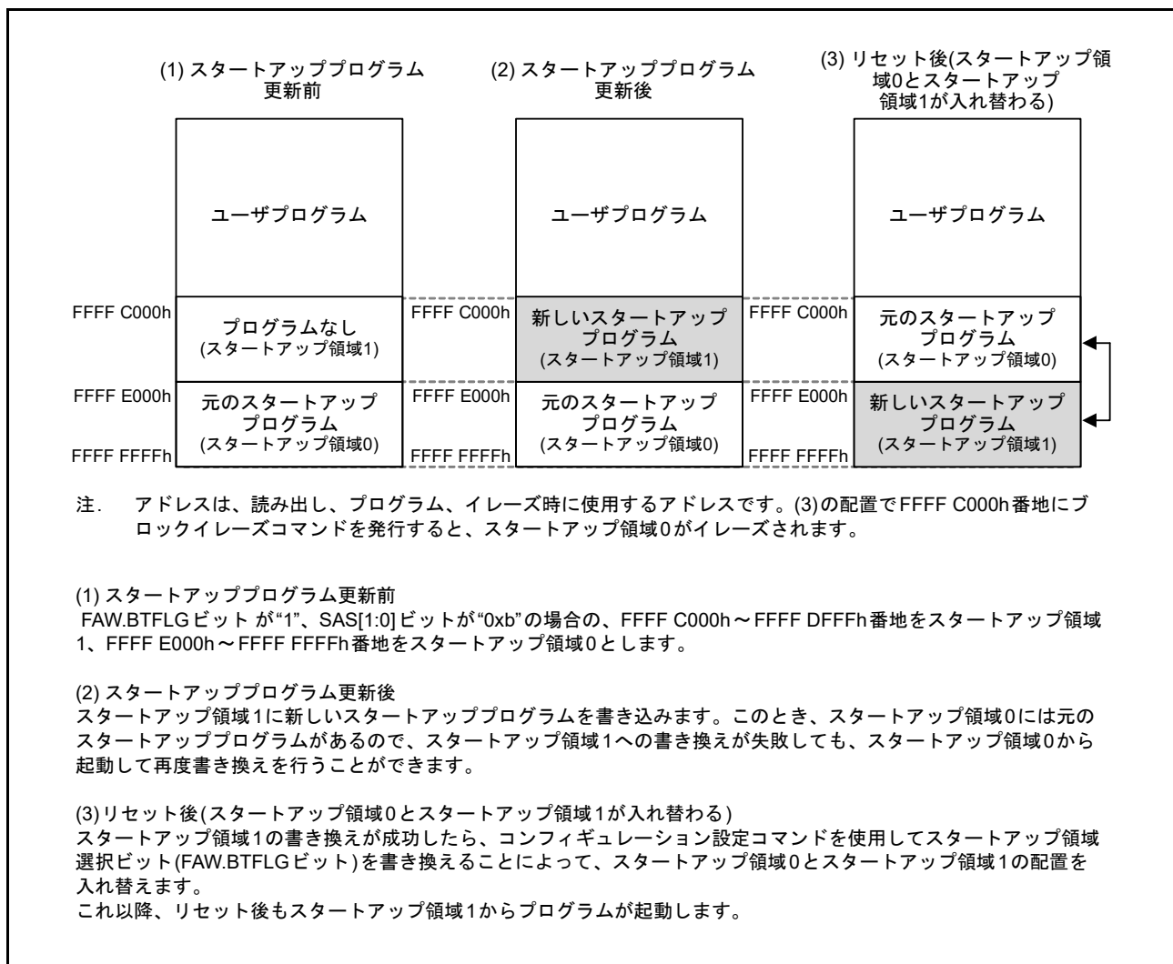
図 62.26 スタートアッププログラム保護機能の概念
