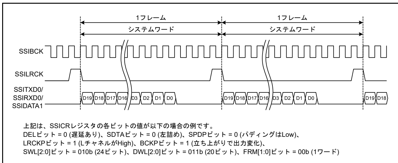
図 47.13 モノラルフォーマットの例 (2) (SSICR.DEL ビット = 0、パディングあり)
