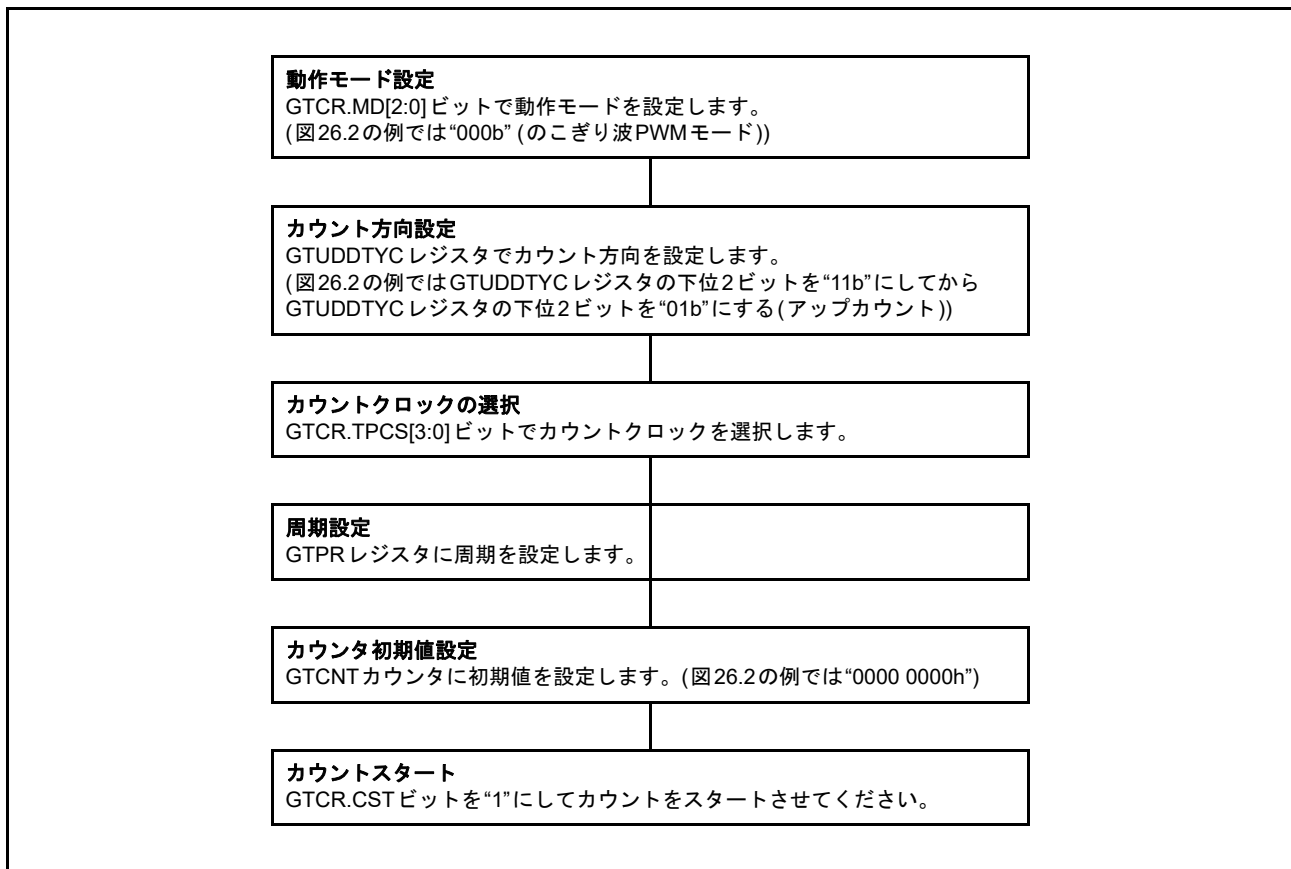
図 26.3 サイクルカウント動作設定例 ( カウントクロックによるアップカウント時 )
