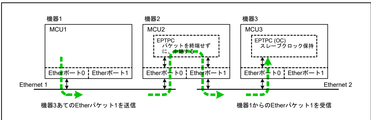
図37.3 本MCUを使用したネットワーク構成例
