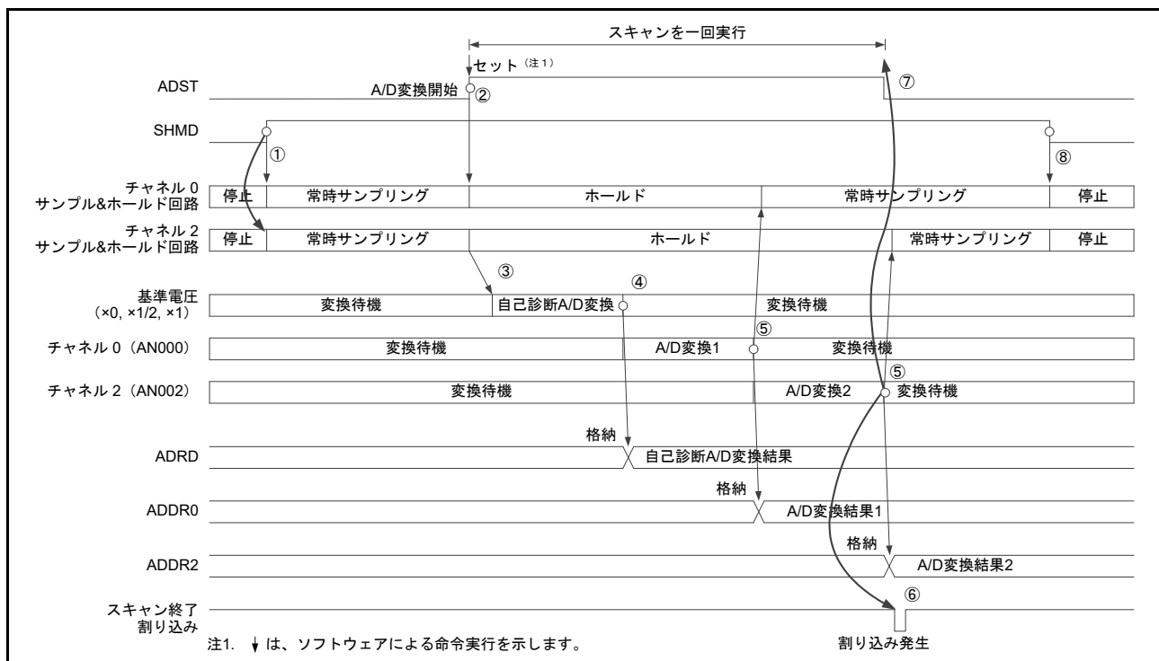
図 56.11 シングルスキャンモードの動作例 (チャンネル専用サンプル & ホールド回路使用 : AN000, AN002 選択 + 自己診断、常時サンプリング有効)
