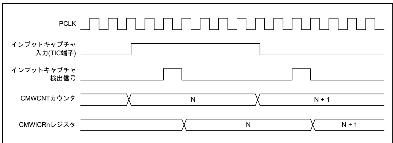
図 32.12 インプットキャプチャタイミング (ユニット 0、両エッジ検出) ( n=0, 1 )
