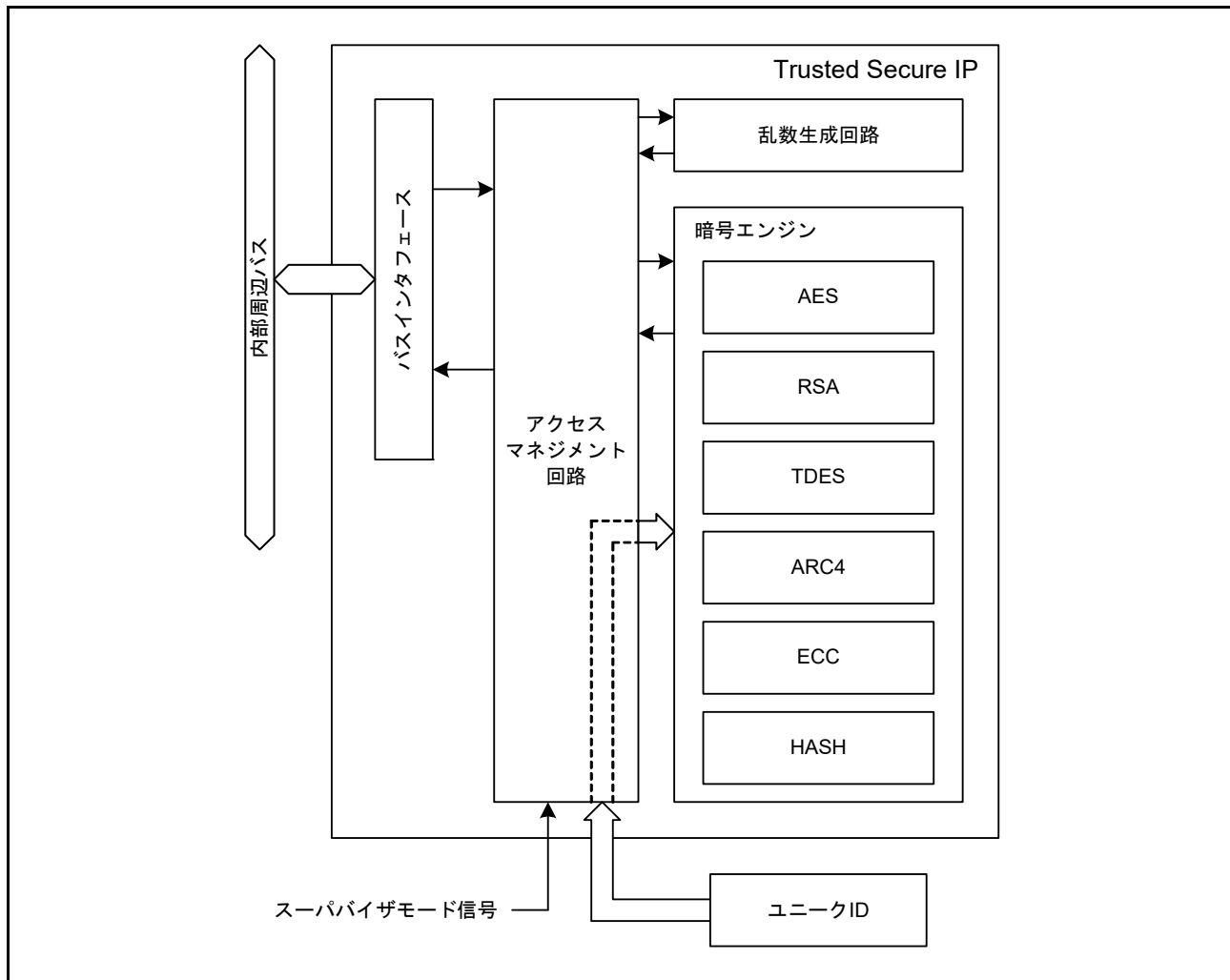
図 55.1 Trusted Secure IPのブロック図
