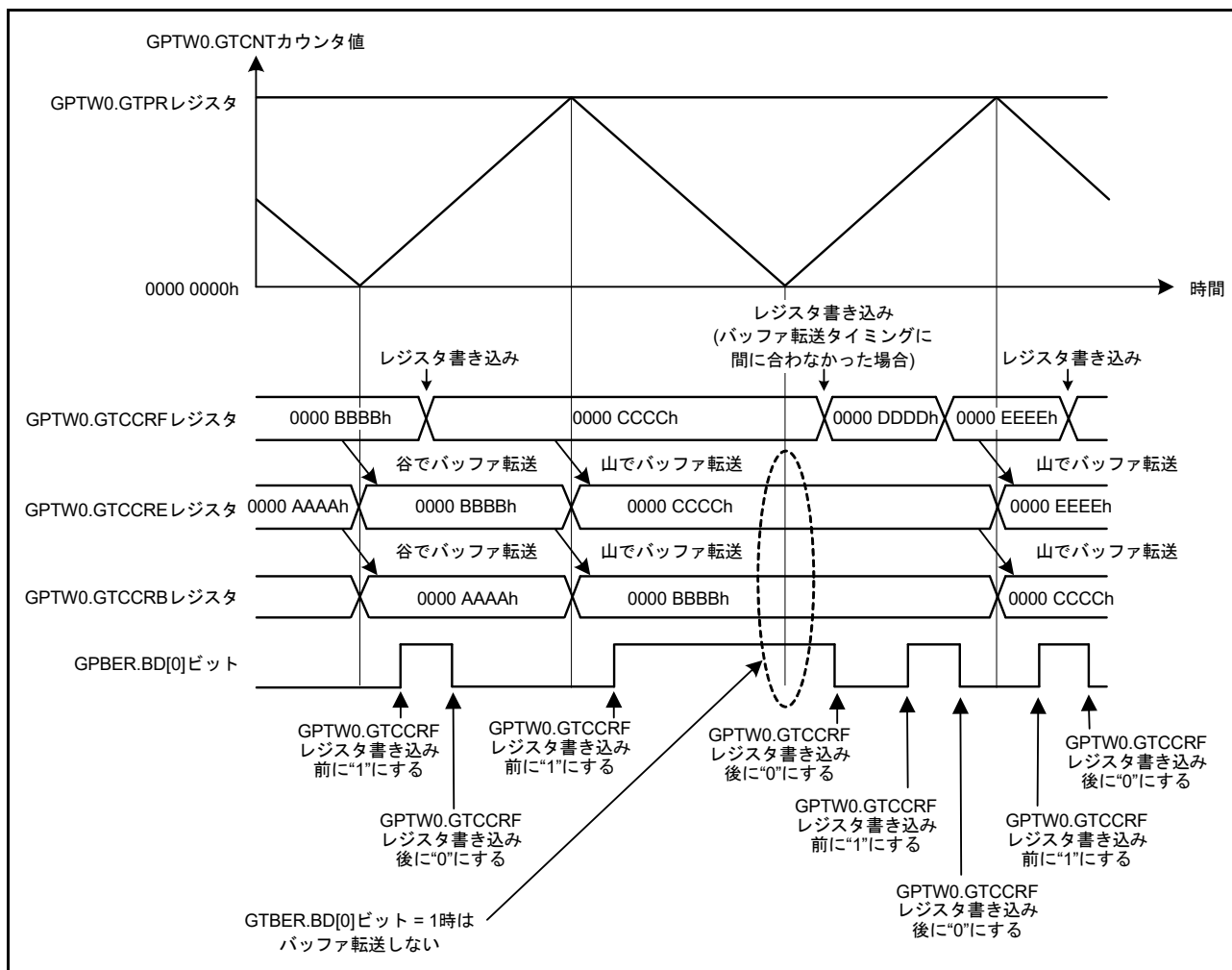
図 26.119 バッファ動作の抑止動作例 ( 三角波、ダブルバッファ動作、谷 / 山両方でバッファ転送の場合 )
