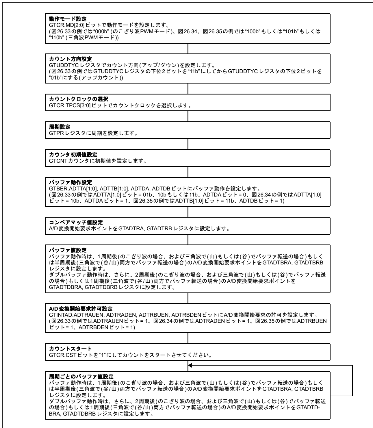
図 26.36 GTADTRA, GTADTRB レジスタのバッファ動作設定例
