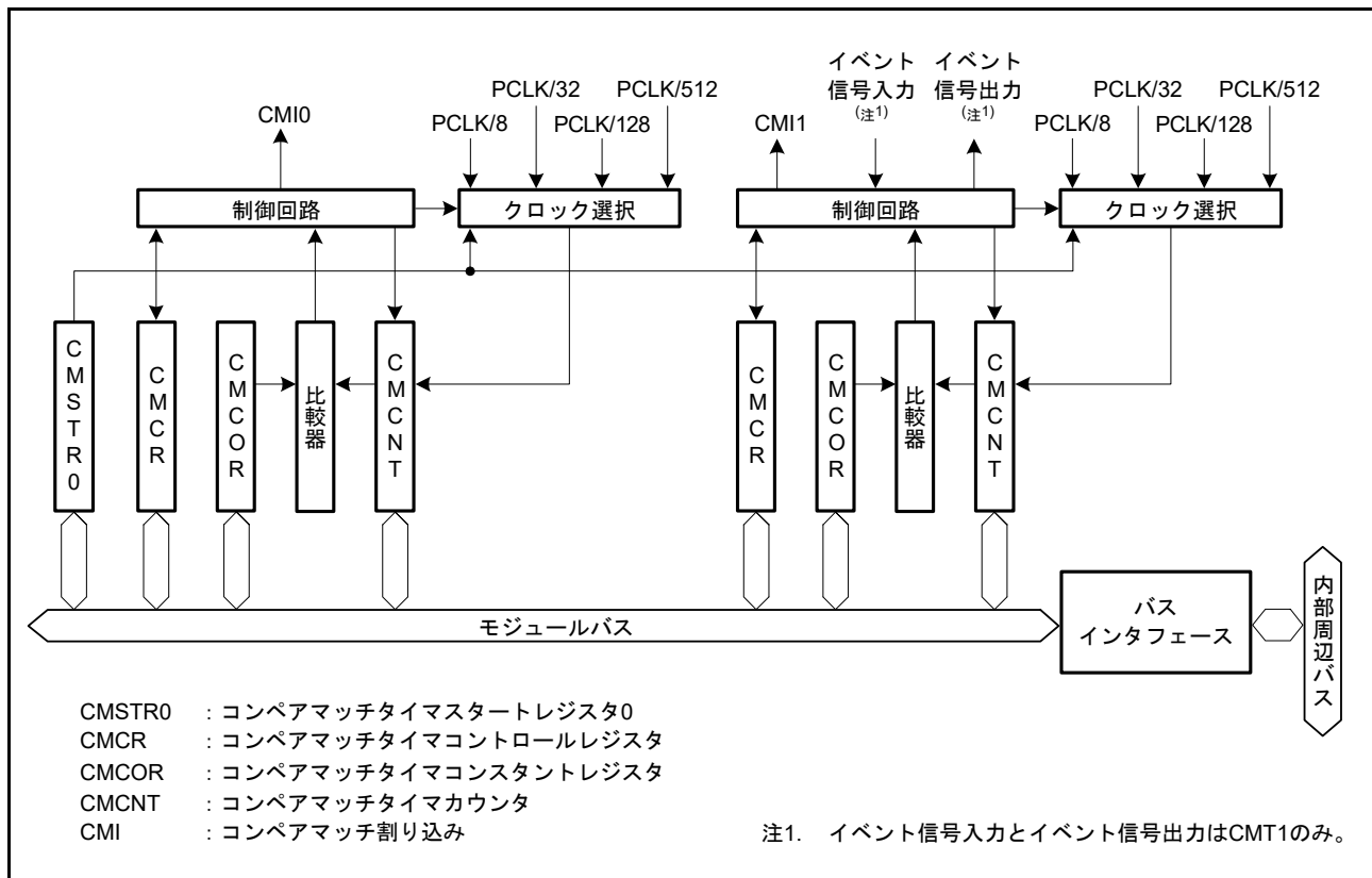
図 31.1 CMT (ユニット 0) のブロック図
