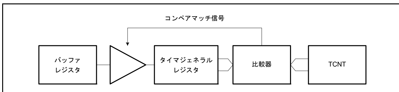
図 28.12 コンペアマッチバッファ動作
