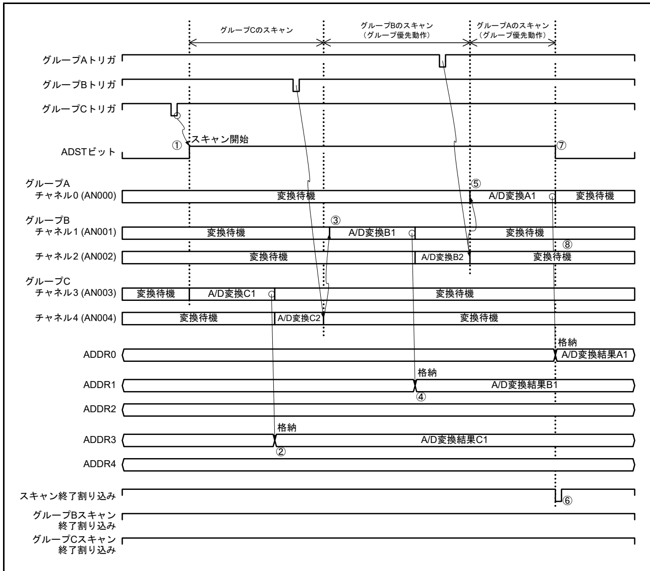
図 56.33 グループ優先動作の例 4 「低優先グループスキャン中の優先グループトリガ入力」再スキャンなし (ADGSPCR.GBRSCN = 0, ADGSPCR.GBRP = 0, ADGSPCR.LGRRS = 1 設定時)
