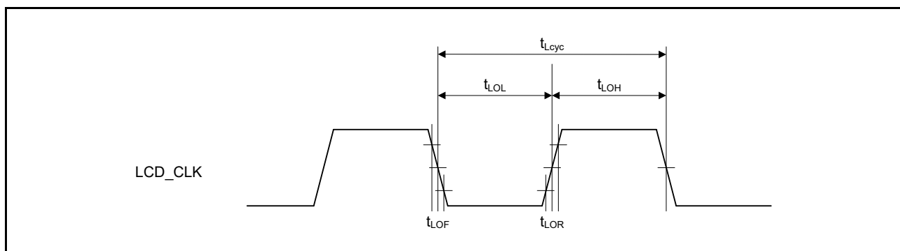
図 63.95 LCD_CLK クロック出カタイミング
