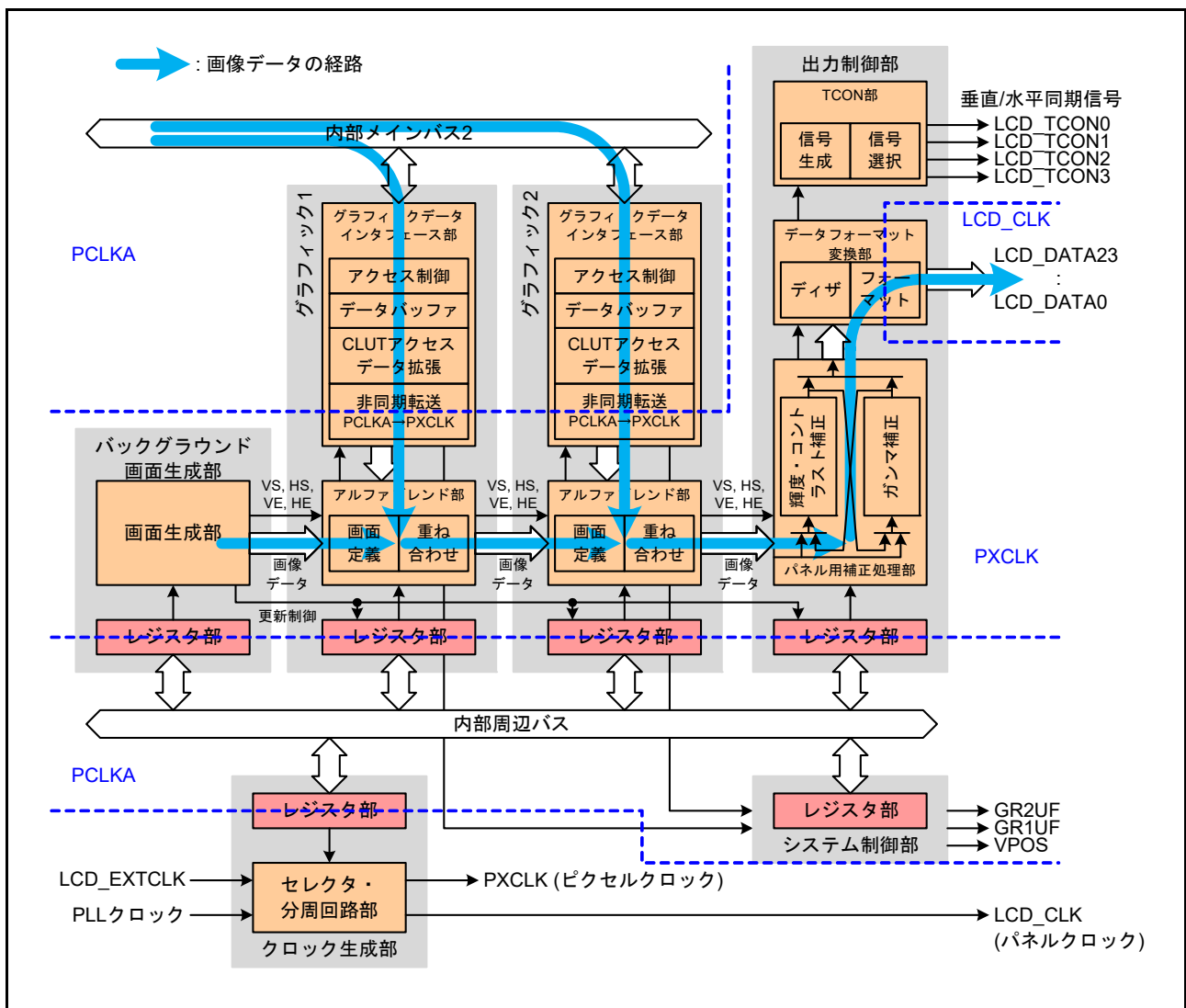
図 51.20 GLCDC の構成
