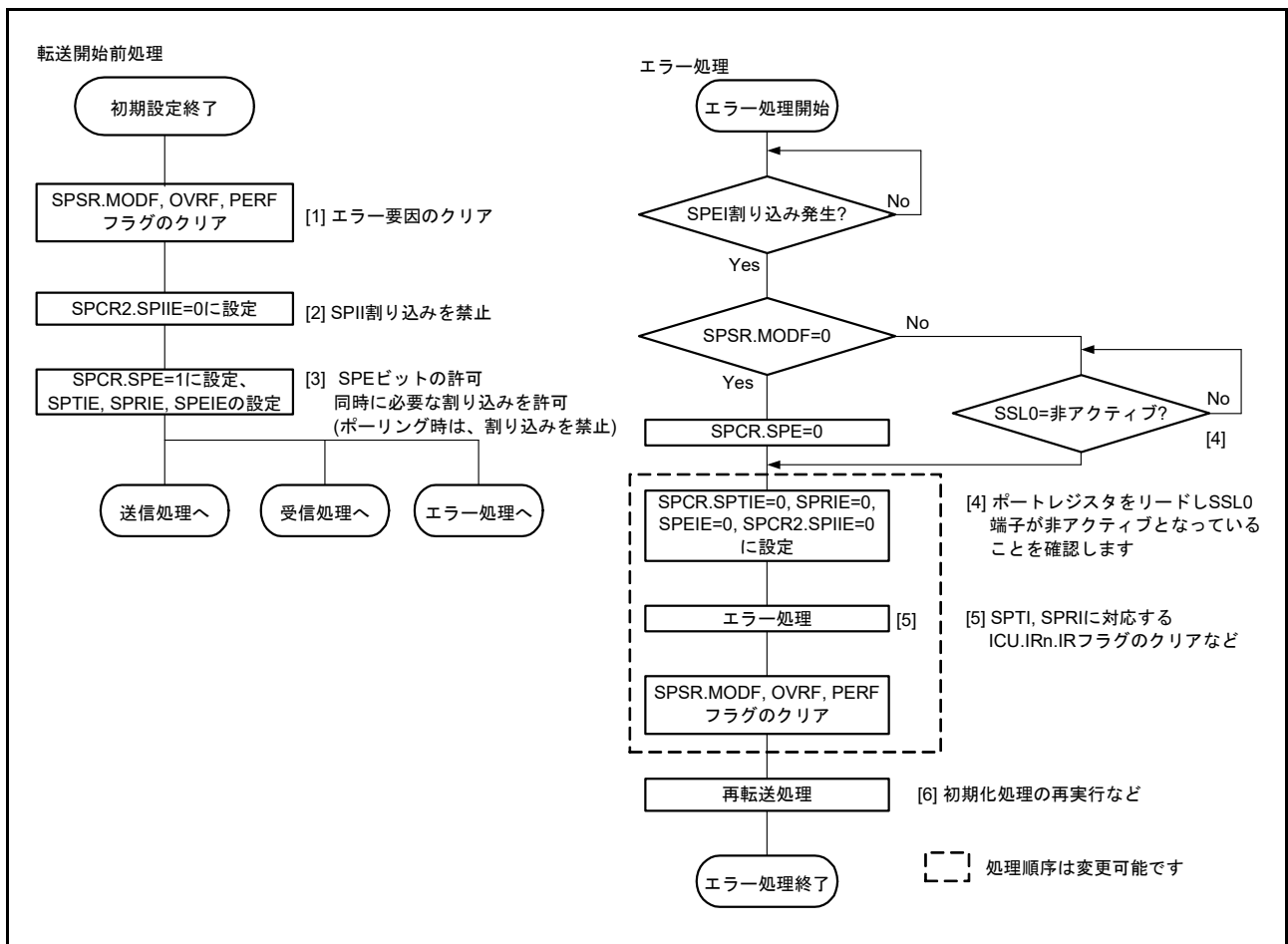
図 44.40 マスタモード時のフローチャート (エラー)
