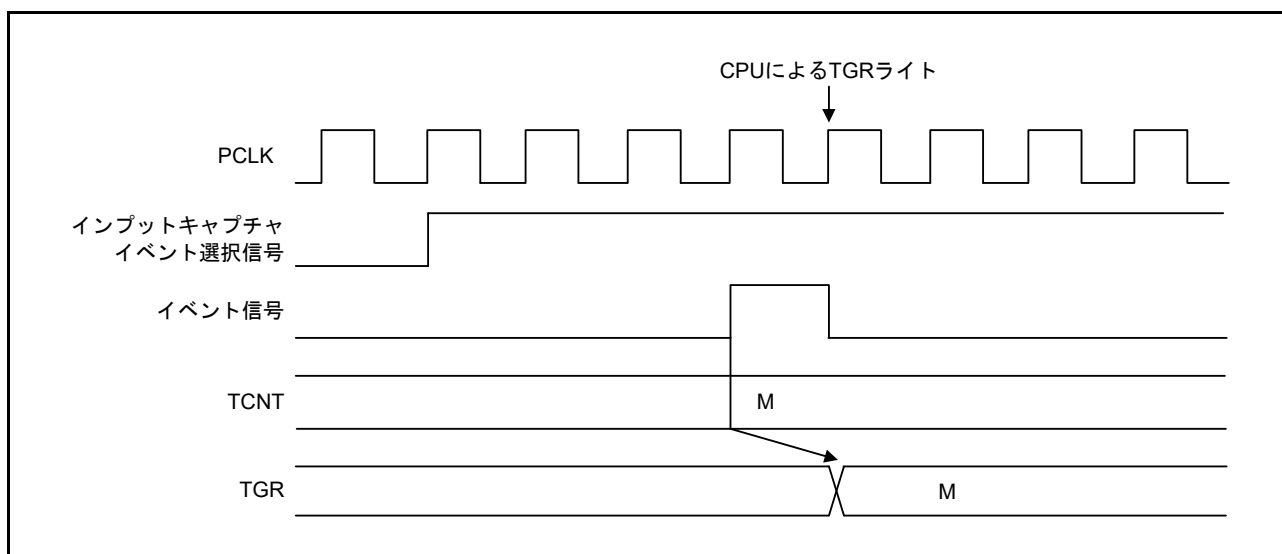
図 28.62 TGR へのライトサイクルとインพุットキャプチャ動作の競合
