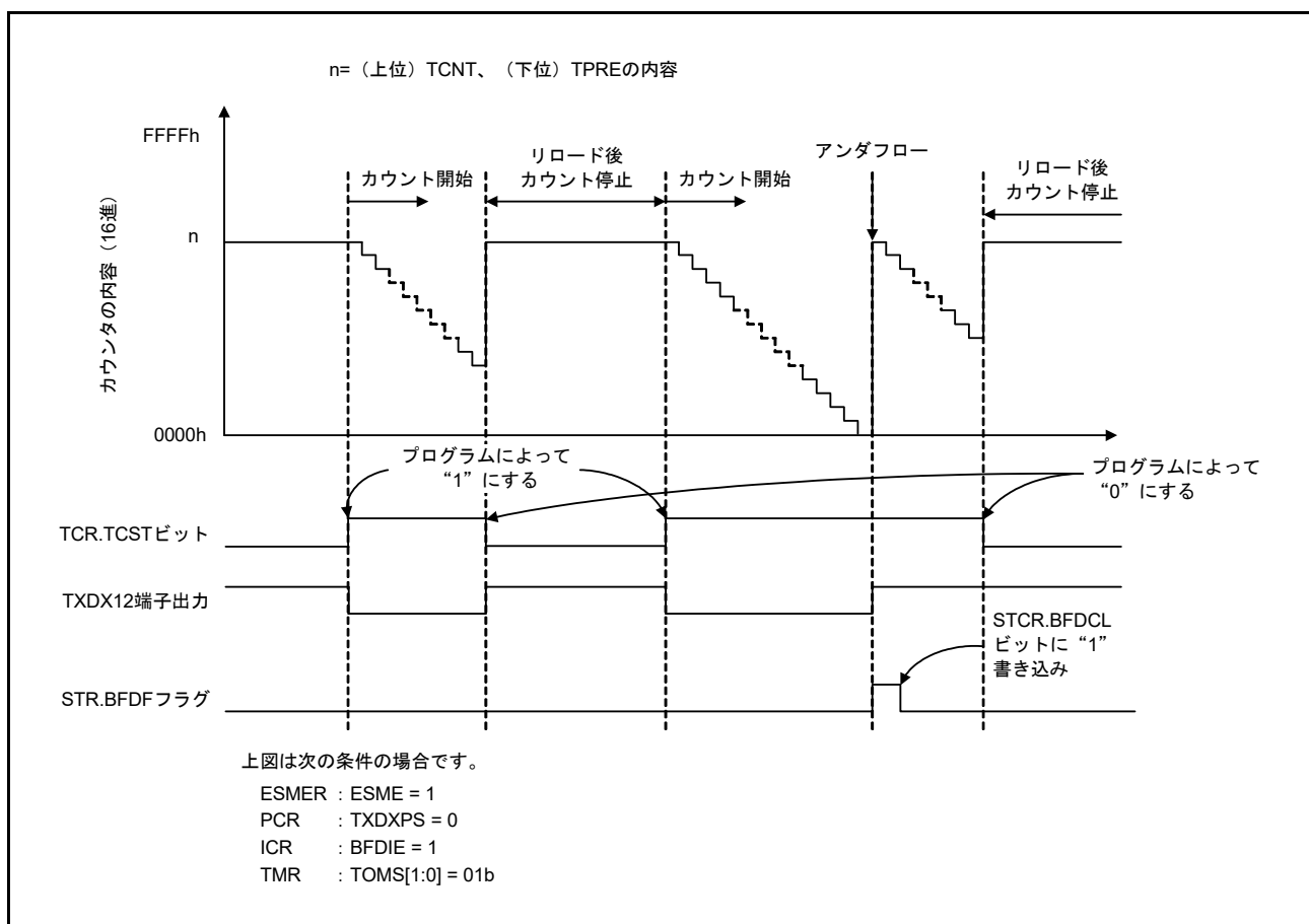
図 41.77 Break Field Low width 出力モードの動作例
