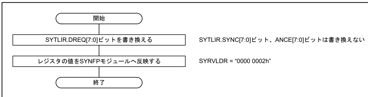
図37.11 Delay_RespメッセージのlogMessageIntervalフィールド値の変更手順
