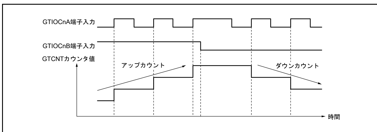
図 26.89 位相計数モード2の動作例 (n = 0 ~ 3)
