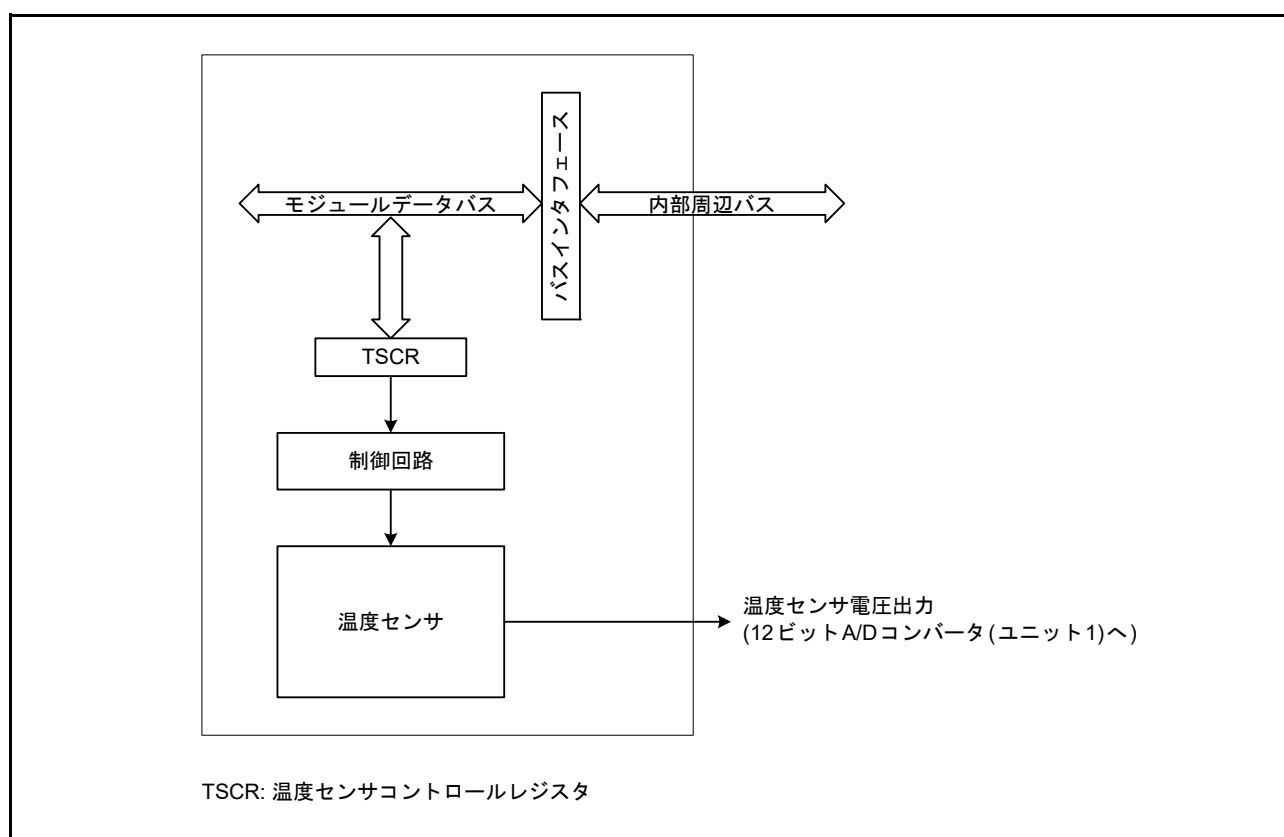
図 58.1 温度センサのブロック図
