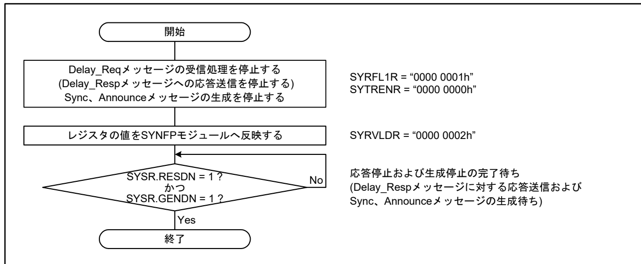
図37.12 E2E マスタ動作の停止手順
