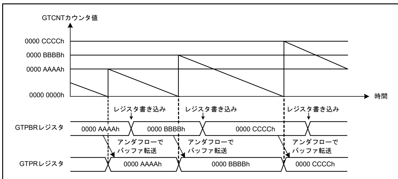
図 26.23 GTPR レジスタのバッファ動作例 (のこぎり波でダウンカウントの場合)
