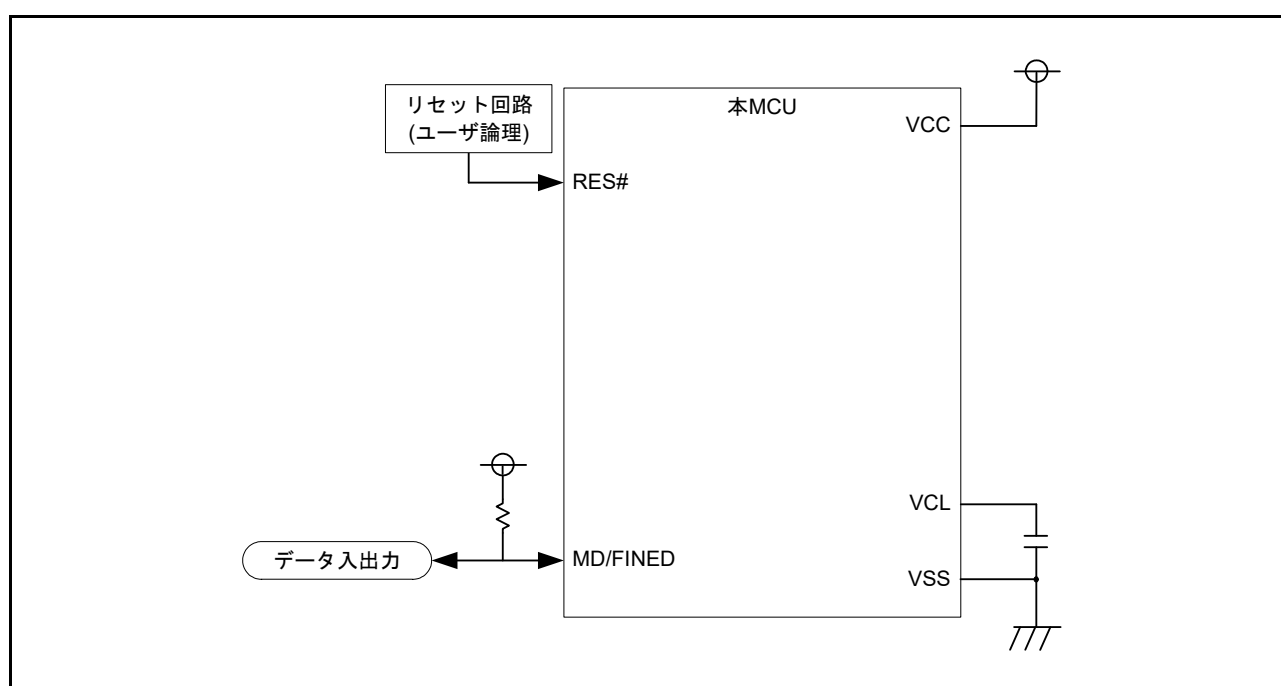
図 62.36 ブートモード (FINE インタフェース) 時の端子接続例
