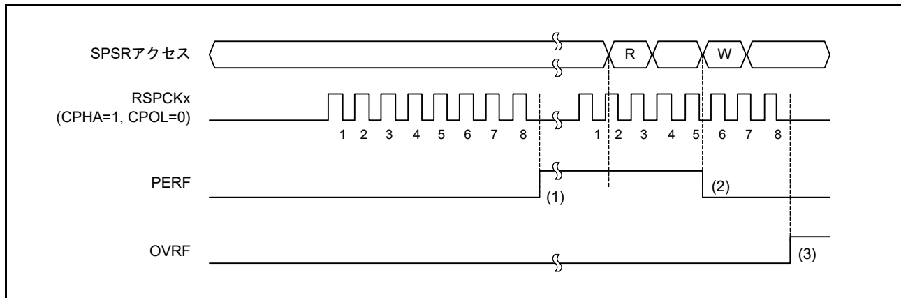
図 44.32 PERF フラグの動作例
