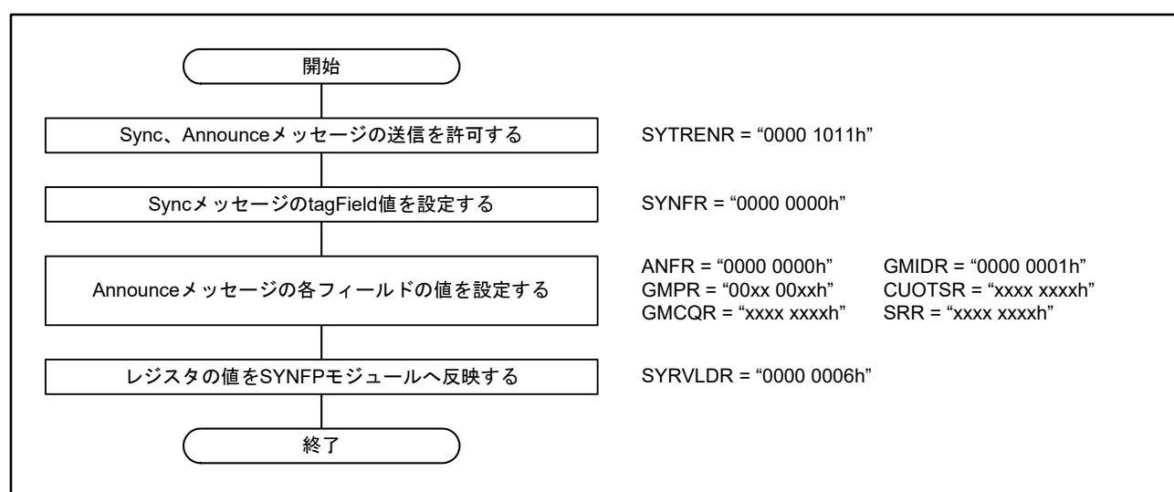
図37.18 P2Pマスタ動作の開始手順
