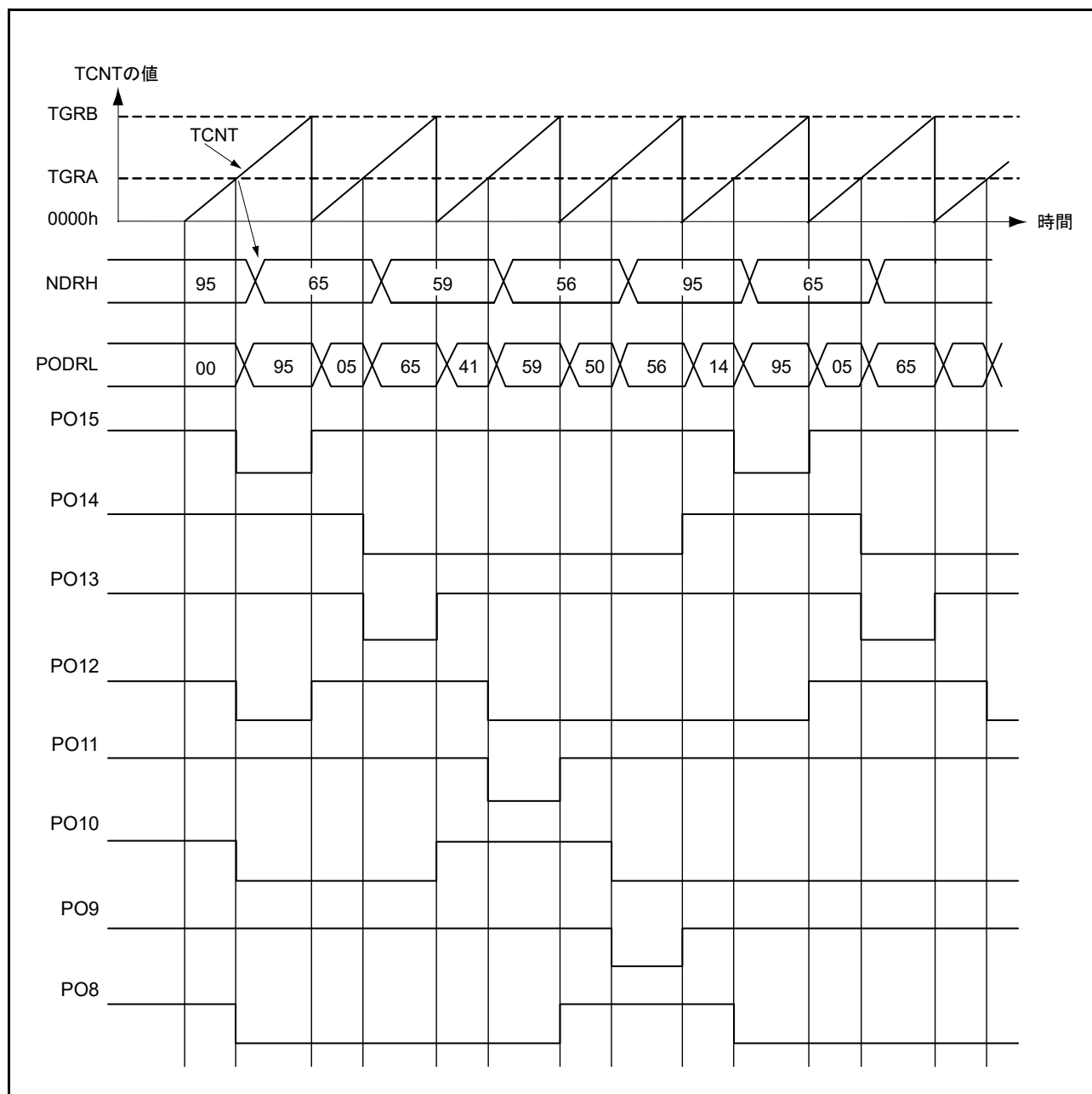
図 29.14 パルス反転出力例
