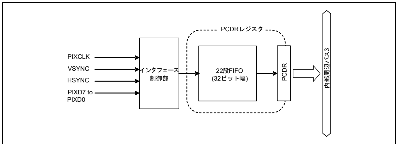
図 50.2 PCDR レジスタの構造図
