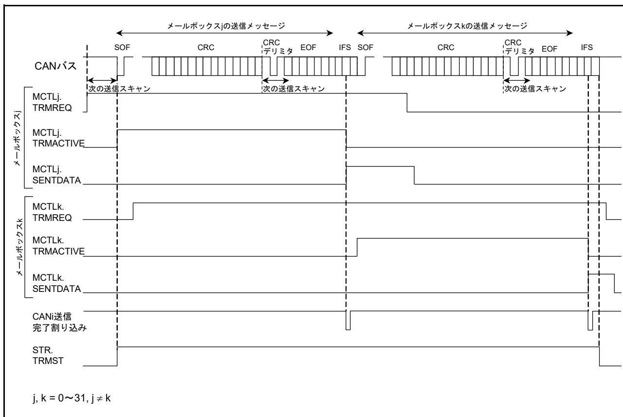
図 43.20 データフレーム送信時の動作例
