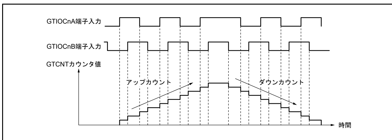
図 26.87 位相計数モード 1 の動作例 (n = 0 ~ 3)
