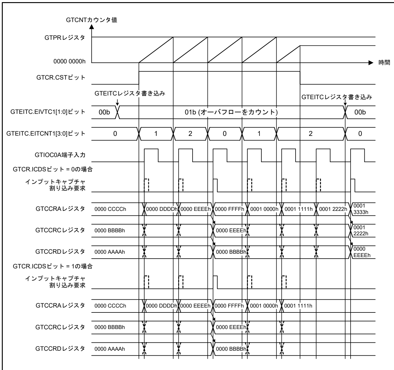
図 26.113 拡張割り込み間引き機能のインプットキャプチャ動作例 (のこぎり波アップカウント、拡張割り込み間引き 1 間引き回数 2 でオーバーフローをカウント、EITCNT1 が “0” 以外の期間で間引く、入力の立ち上がりでインプットキャプチャの場合)
