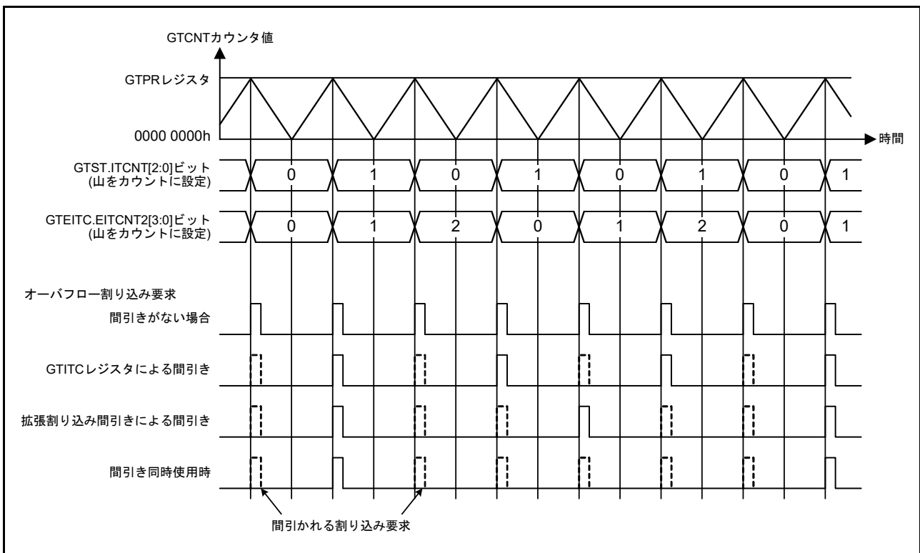
図 26.104 割り込み間引きの動作例 (GTITC レジスタによる間引き : 山をカウント、拡張割り込み間引き : EIVTC1[1:0] ビット = 00b、EIVTC2[1:0] ビット = 01b、EITLV[2:0] ビット = 010b)
