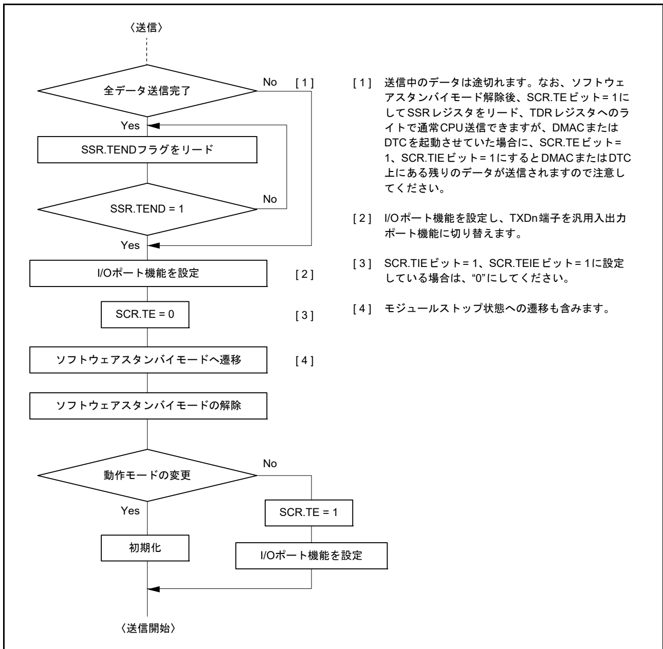
図 41.81 送信時のソフトウェアスタンバイモード遷移フローチャートの例
