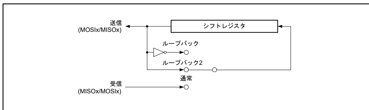
図 44.50 ループバックモード時のシフトレジスタ入出力構成 (マスターモード)
