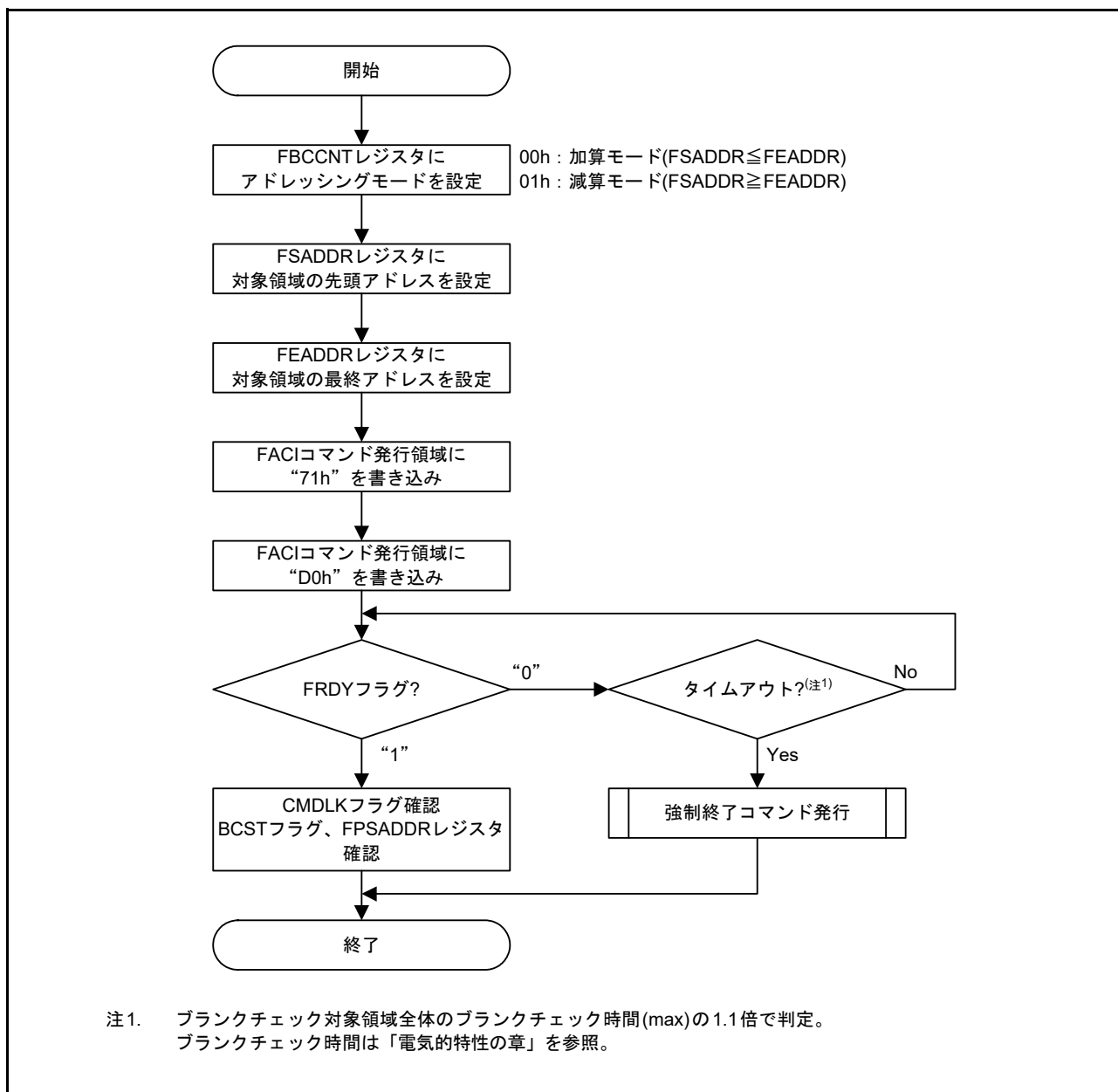
図 62.24 ブランクチェックコマンドの使用方法
