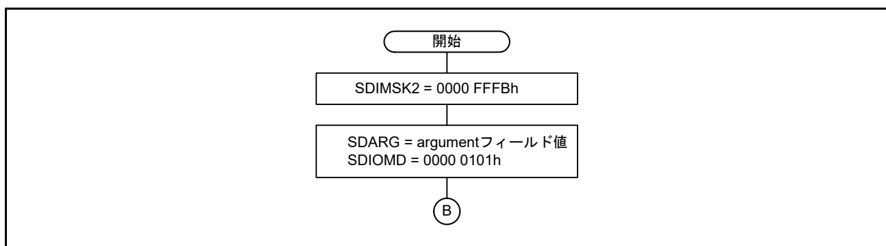
図 48.16 IO_RW_EXTENDED コマンド (CMD53/ マルチブロックリード) のシーケンス中に SDIO abort コマンド (CMD52) を送信する例
