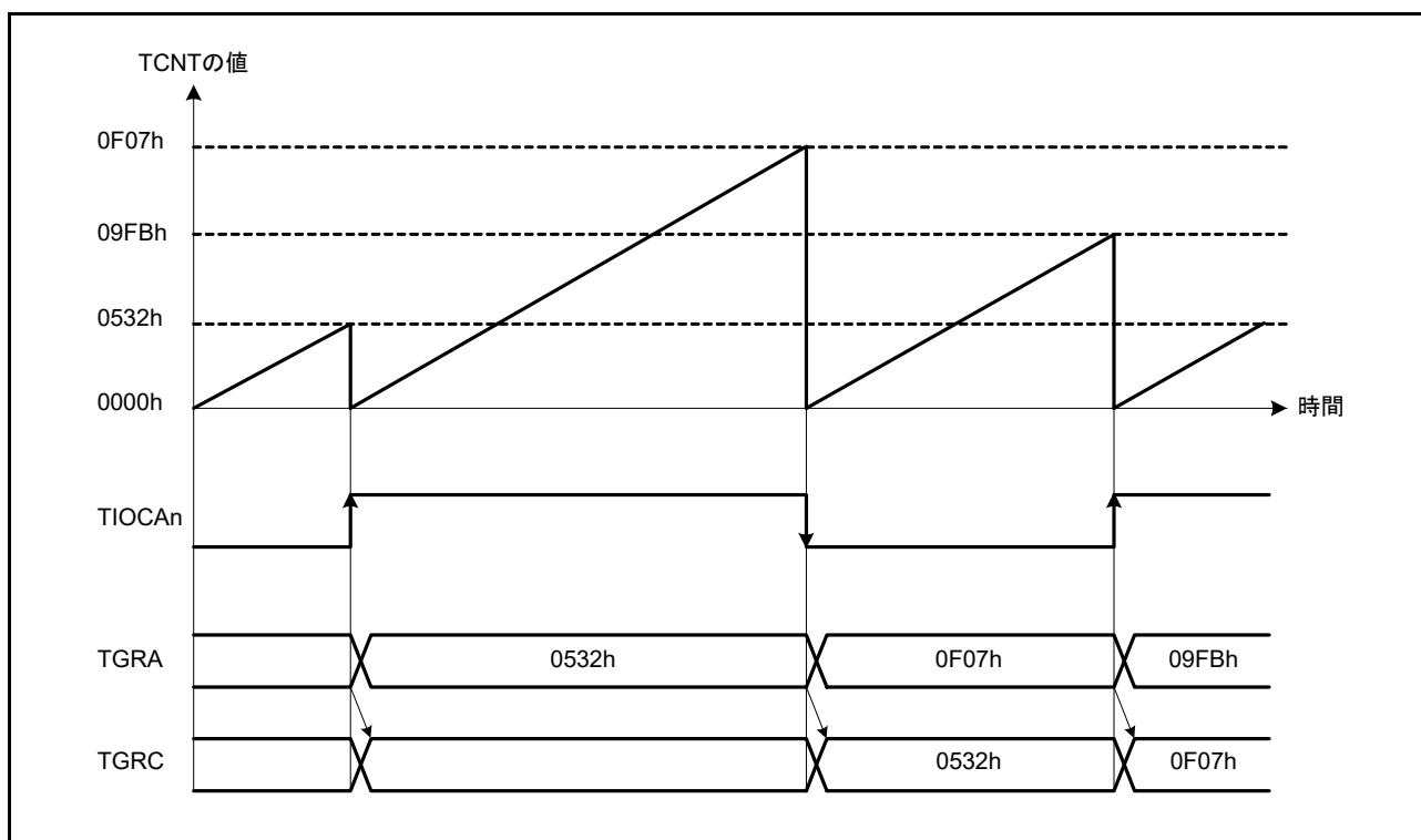
図 28.16 バッファ動作例 (2) (n = 0 ~ 5)
