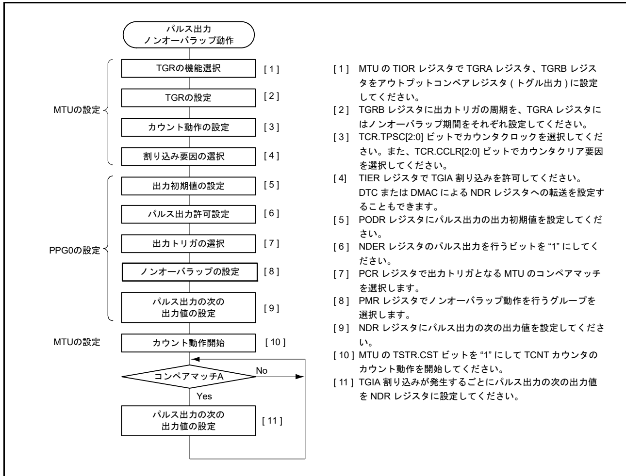
図 29.11 パルス出力ノンオーバーラップ動作の設定手順例 (PPG0 の設定)
