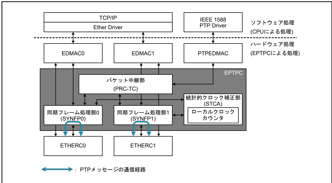
図37.7 ハードウェアによるPTPメッセージの生成と応答の経路
