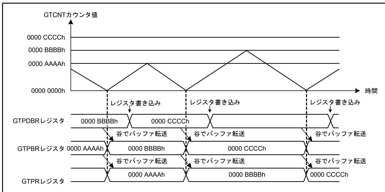
図 26.24 GTPR レジスタのダブルバッファ動作例 (三角波の場合)
