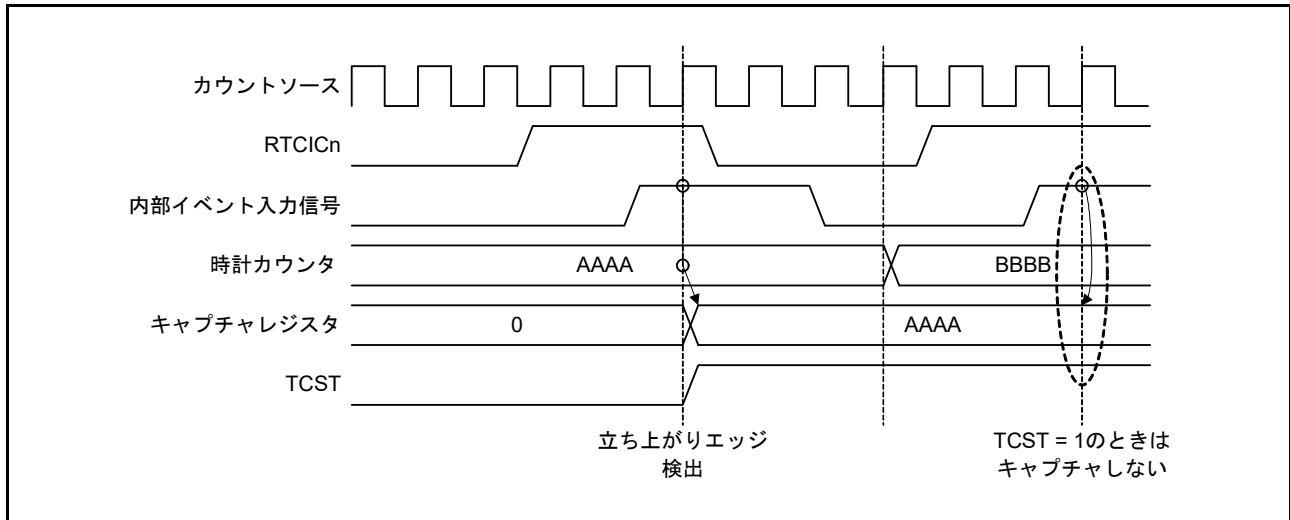
図 33.9 時間キャプチャ機能動作タイミング (フィルタ OFF) (n = 0 ~ 2)
