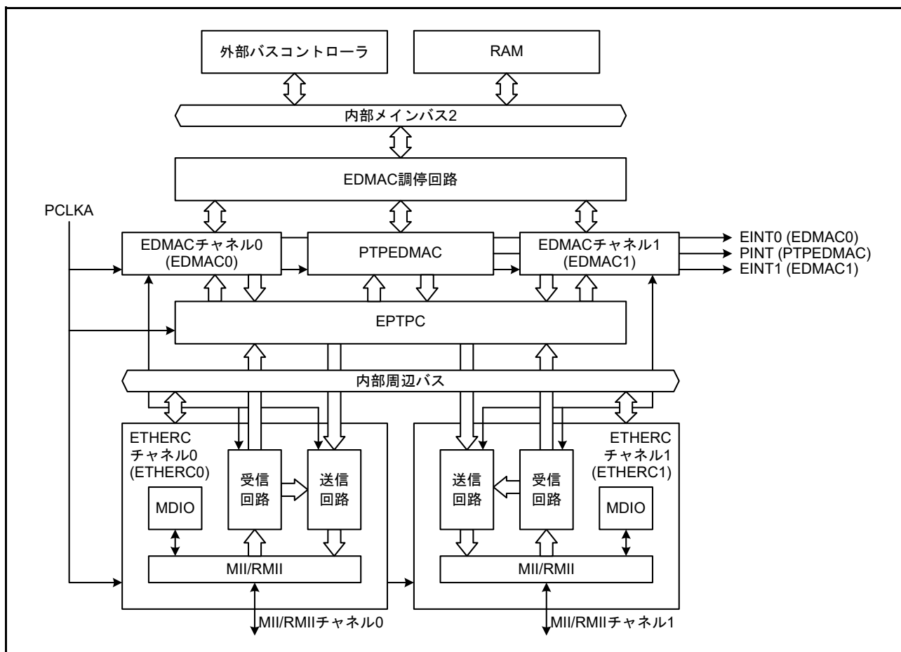
図 36.1 ETHERC の構成
