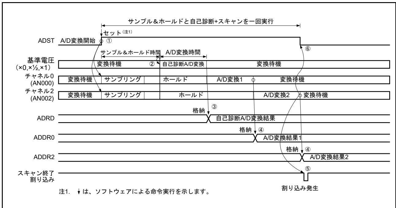
図 56.10 シングルスキャンモードの動作例 (チャンネル専用サンプル & ホールド回路使用チャンネル AN000, AN002 選択 + 自己診断、常時サンプリング無効)
