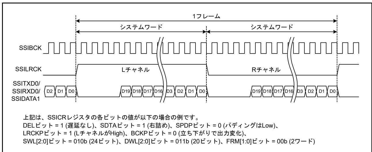
図 47.11 右詰めフォーマットの例
