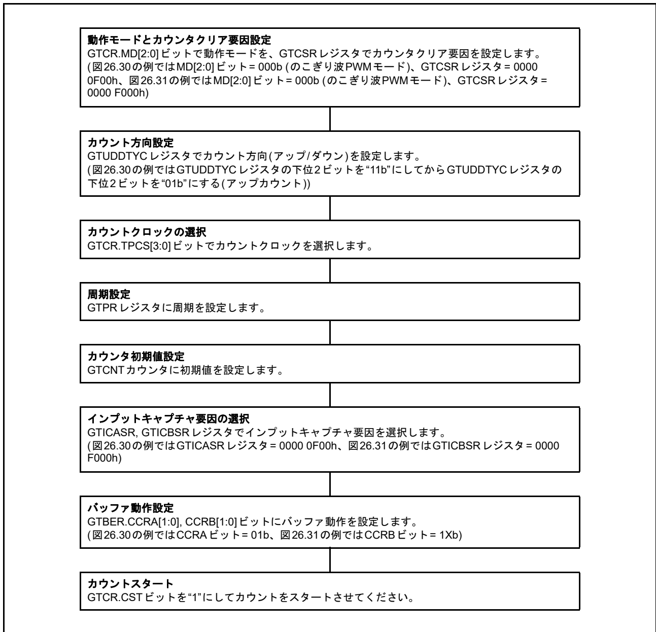
図 26.32 GTCCRA, GTCCRB レジスタのバッファ動作設定例 (インプットキャプチャ時)
