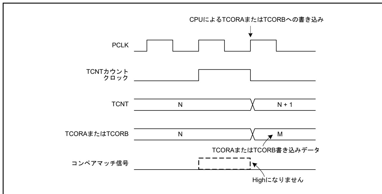
図 30.15 TCORA、TCORB レジスタのライトとコンペアマッチの競合
