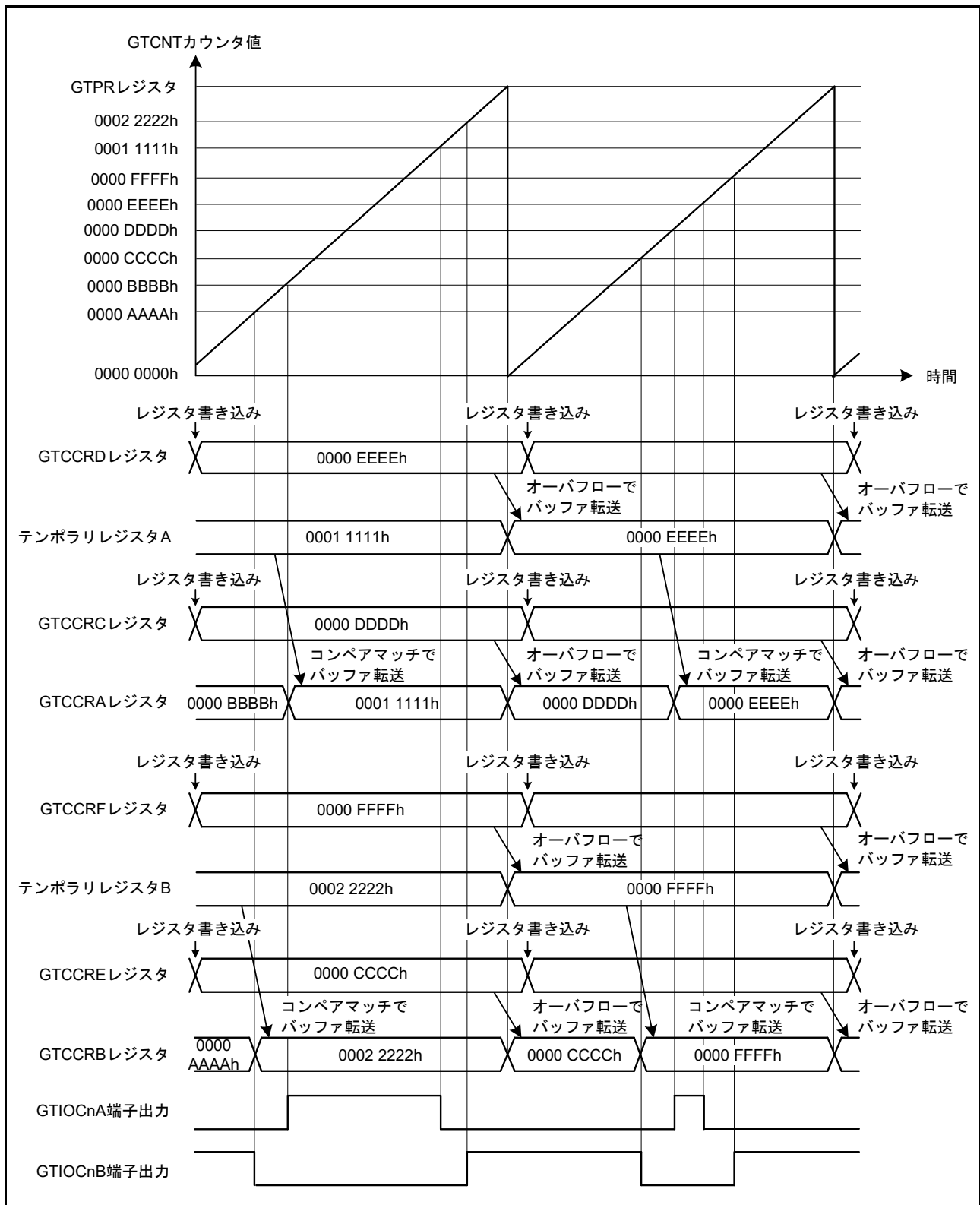
図 26.39 のこぎり波ワンショットパルスモード動作例 ( アップカウント、初期出力で GTIOCnA 端子 = Low 出力 /GTIOCnB 端子 = High 出力、GTCCRA/GTCCRB レジスタのコンペアマッチでトグル出力、周期の終わりで出力保持の場合 ) (n = 0 ~ 3)
