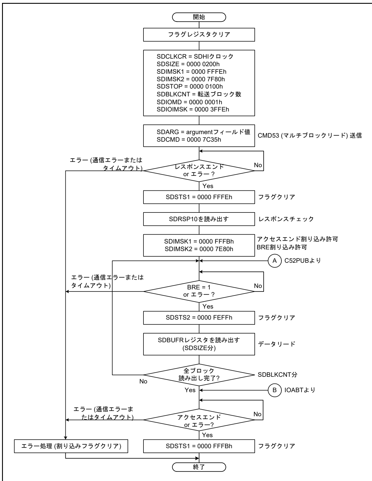
図 48.15 IO_RW_EXTENDED コマンド (CMD53/ マルチブロックリード) の送信例
