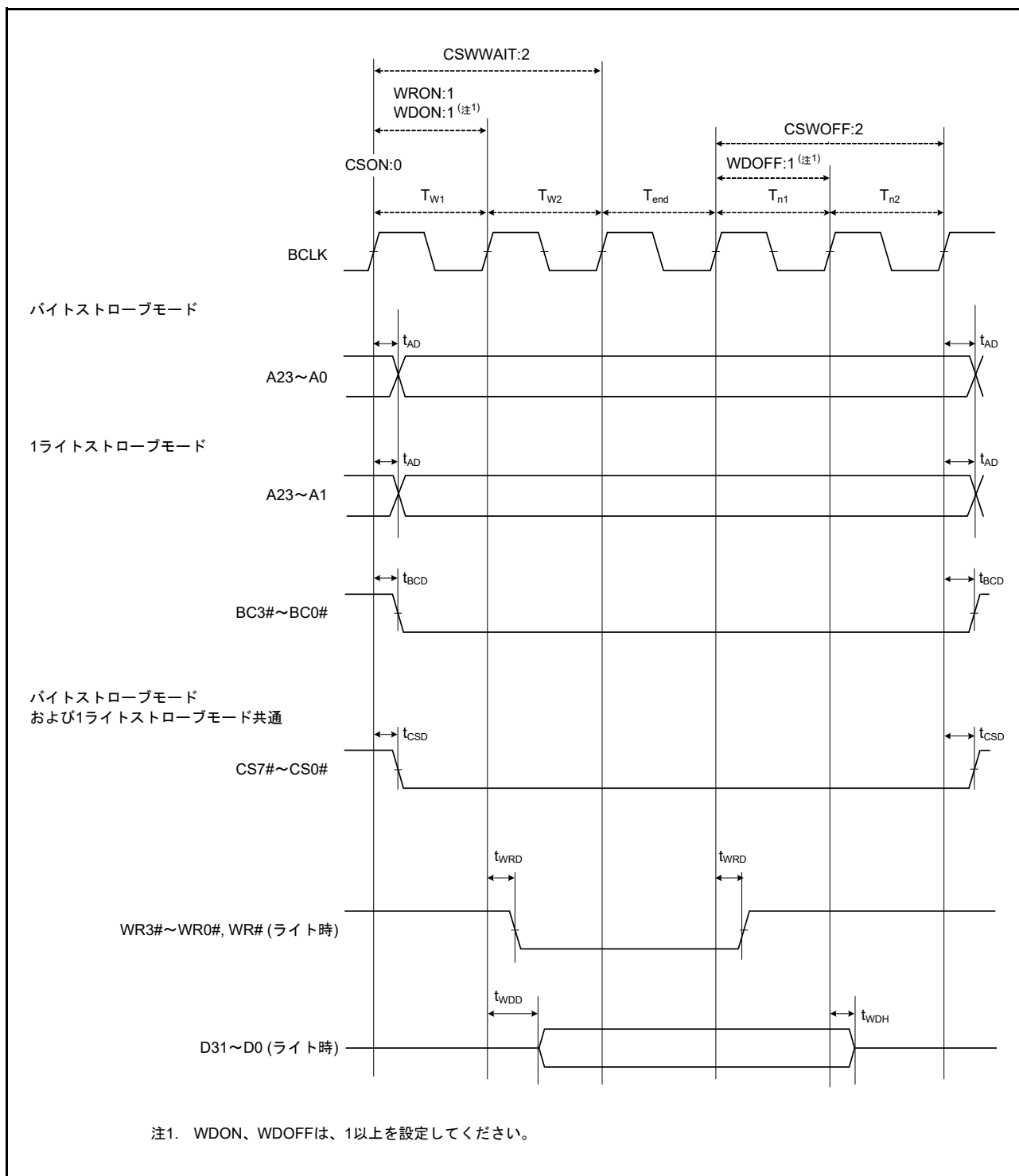
図 63.21 外部バスタイミング / ノーマルライトサイクル (バスクロック同期)
