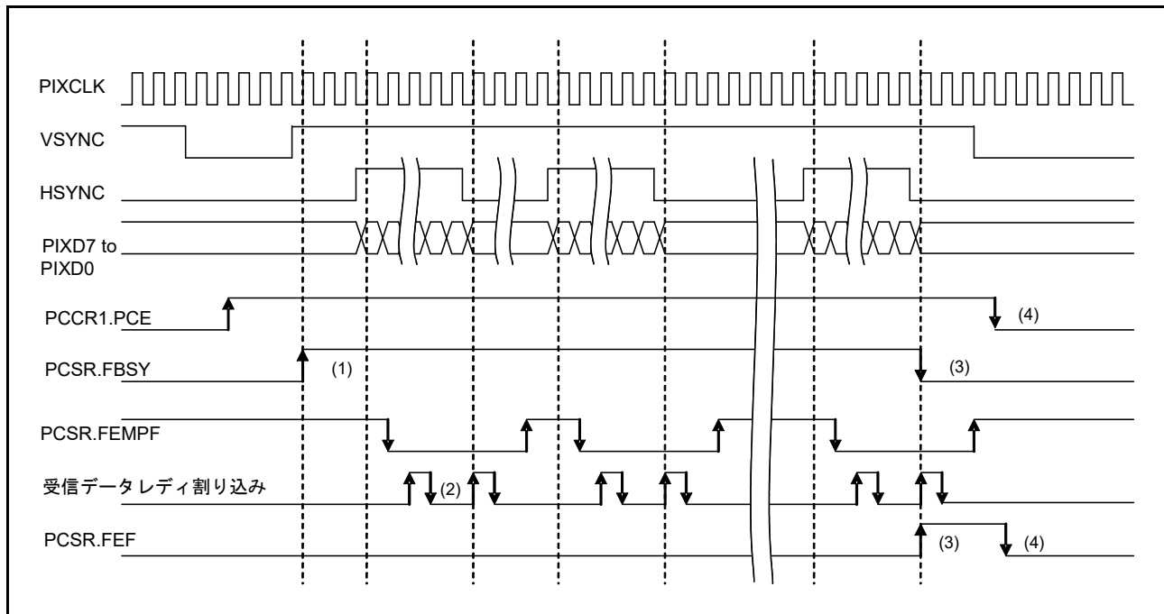
図 50.11 受信動作例
