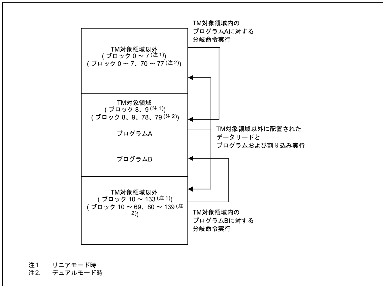
図 62.55 TM 機能有効時、TM 対象領域で CPU が動作可能なケース
