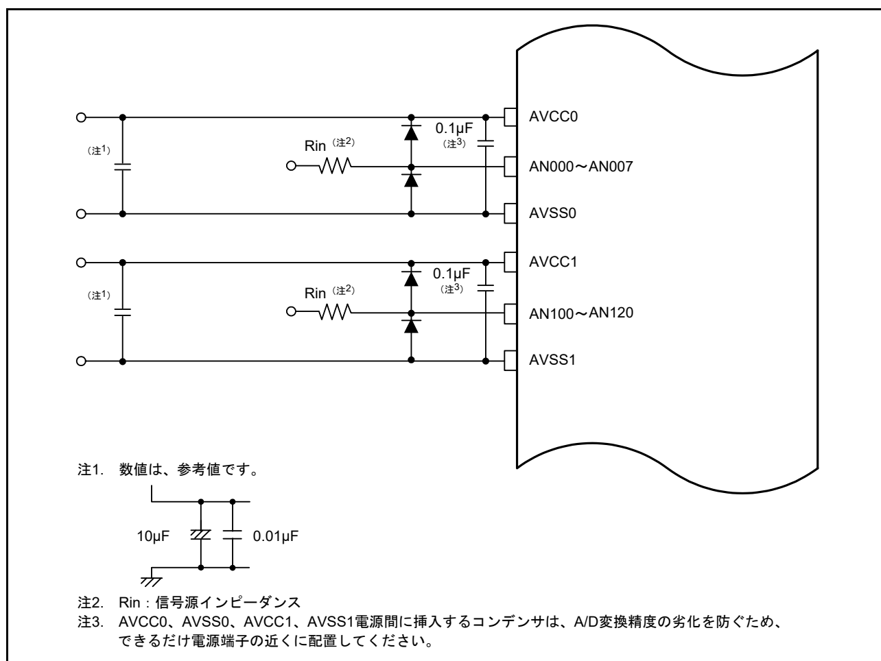
図 56.48 アナログ入力保護回路の例
