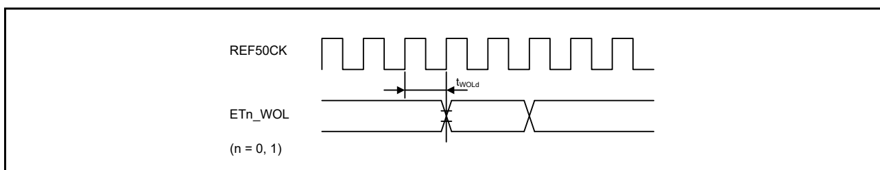
図 63.85 WOL 出カタイミング (RMIIn)
