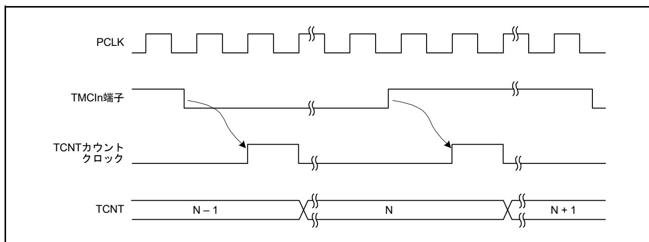
図 30.6 外部クロック動作時のカウンタタイミング (両エッジの場合)
