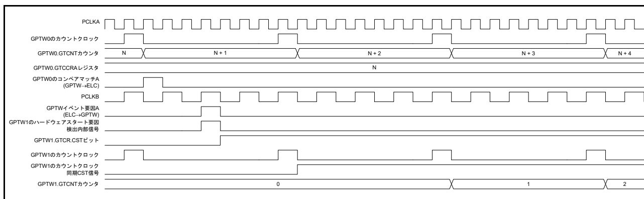
図 26.59 ELCA イベント入力によるカウントスタート動作タイミング例
