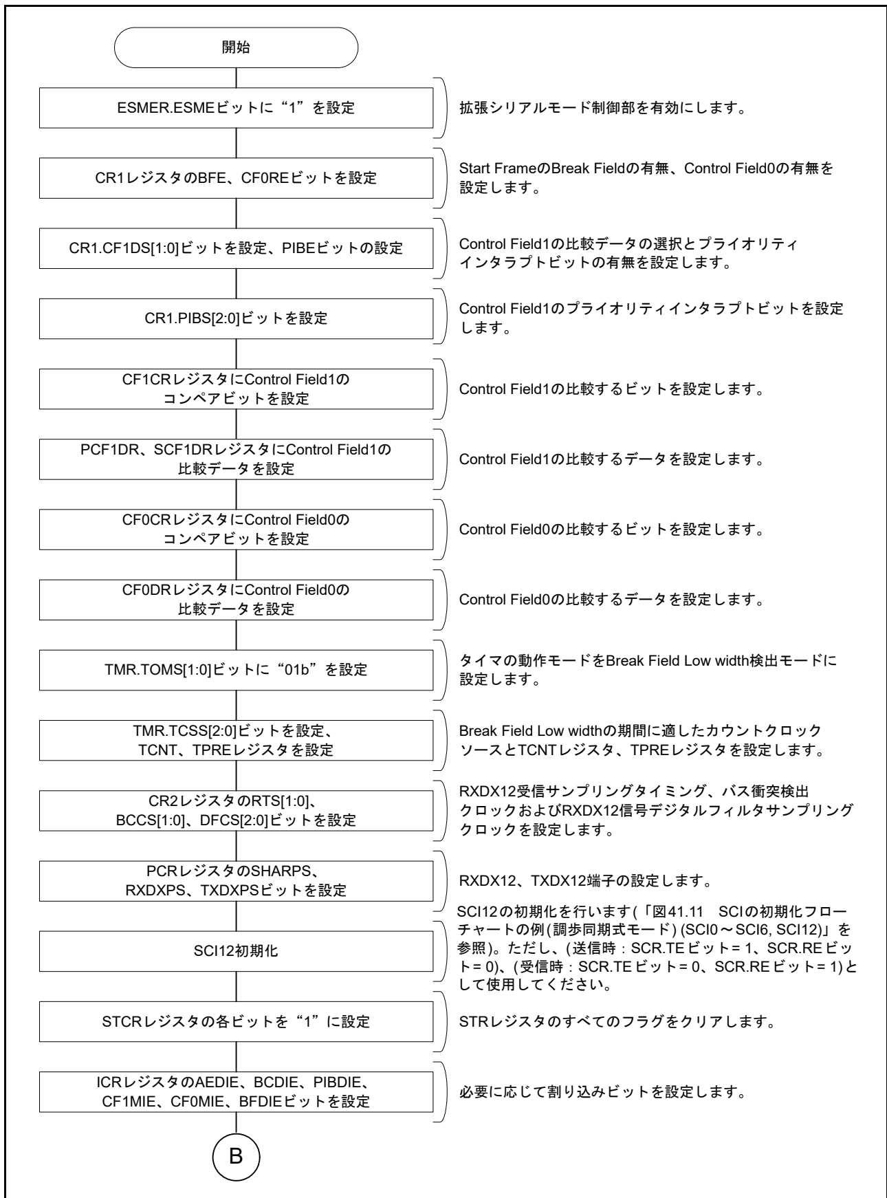
図 41.69 Start Frame 受信フローチャート例 (1)
