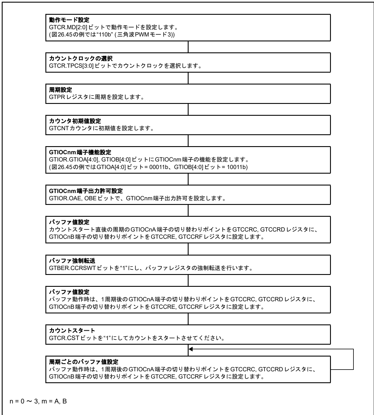
図 26.46 三角波 PWM モード 3 設定例
