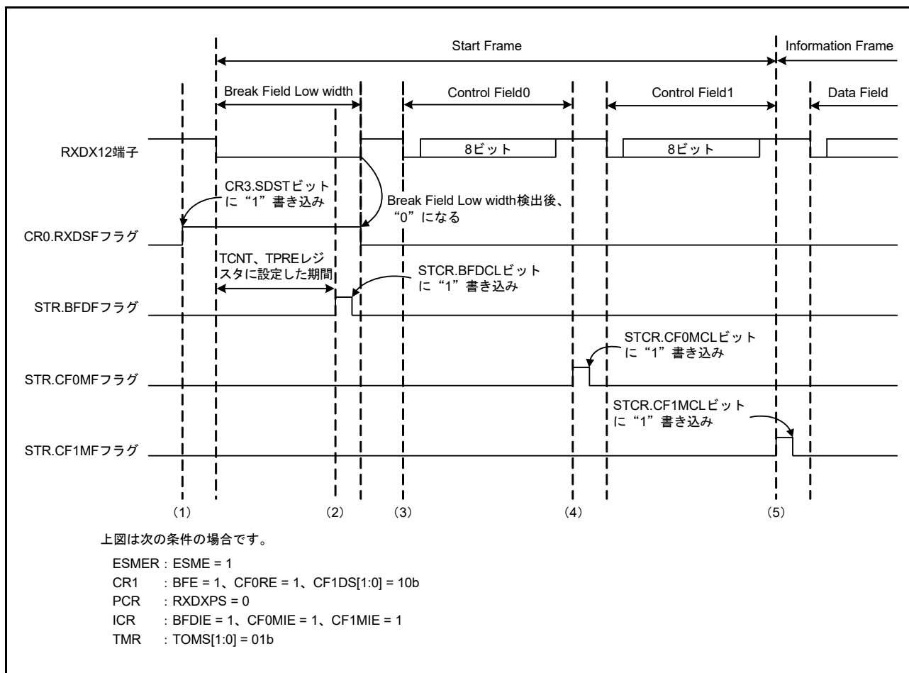
図 41.68 Start Frame 受信時の動作例
