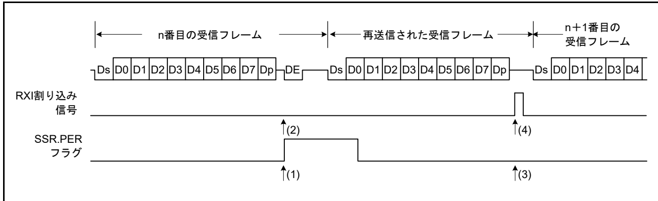
図 41.47 SCI 受信モードの場合の再送信動作 (受信時の再送信動作)
