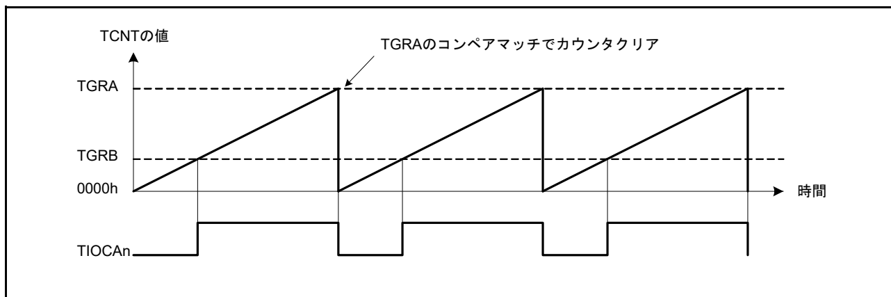
図 28.21 PWM モードの動作例 (1) (n = 0 ~ 5)
