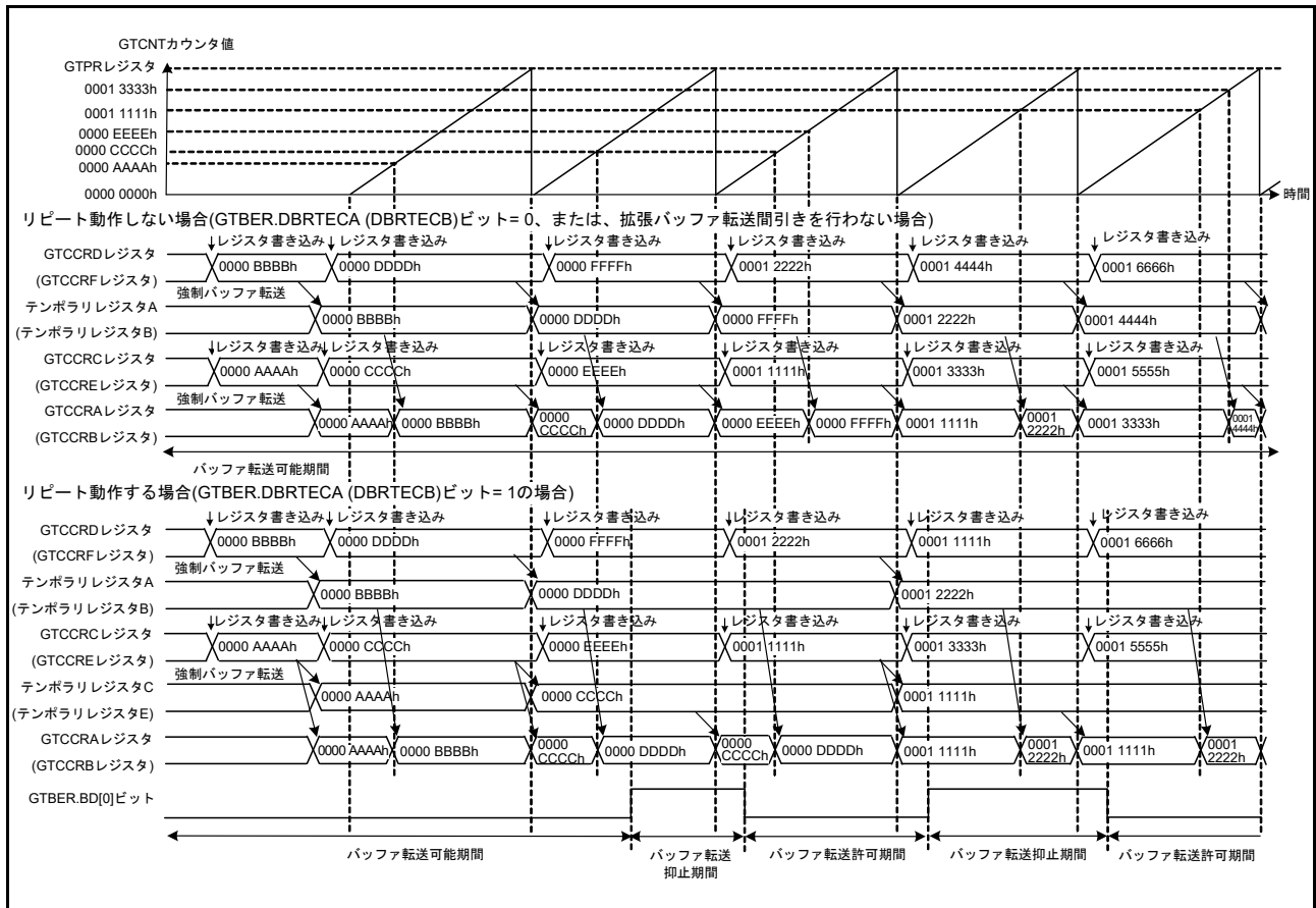
図 26.122 GTCCR バッファ転送抑止時ダブルバッファリポート動作例 (のこぎり波ワンショットパルスモード、GTBER.BD[0] ビットを更新する場合)
