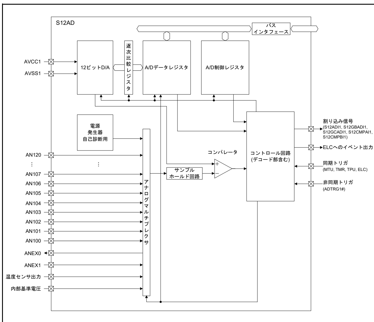
図 56.2 12ビットA/Dコンバータのブロック図 (ユニット1)
