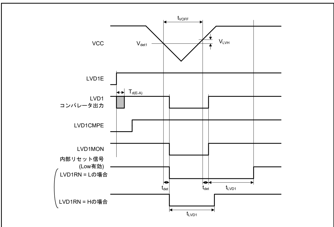
図 63.104 電圧検出回路タイミング ( V_{det1} )
