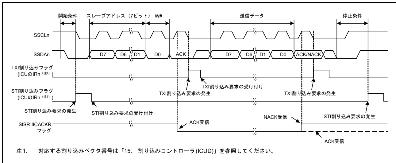
図 41.56 簡易 I 2 C バスモードのマスタ送信の動作例 1 (7 ビットスレーブアドレス、送信割り込み、受信割り込み使用時)
