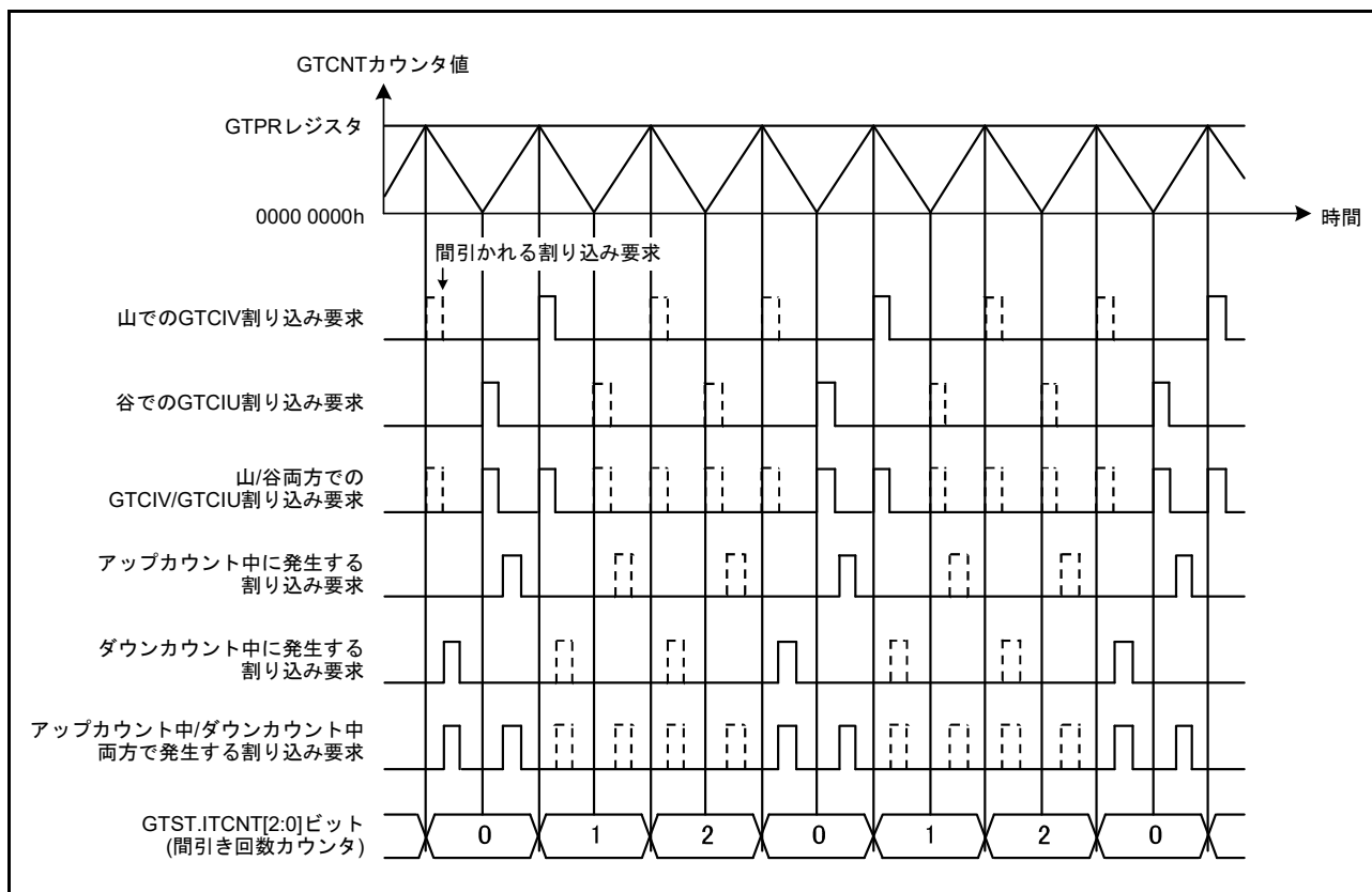
図 26.97 割り込み間引き機能の動作例 (三角波、山をカウントして間引き、間引き回数 2 の場合)
