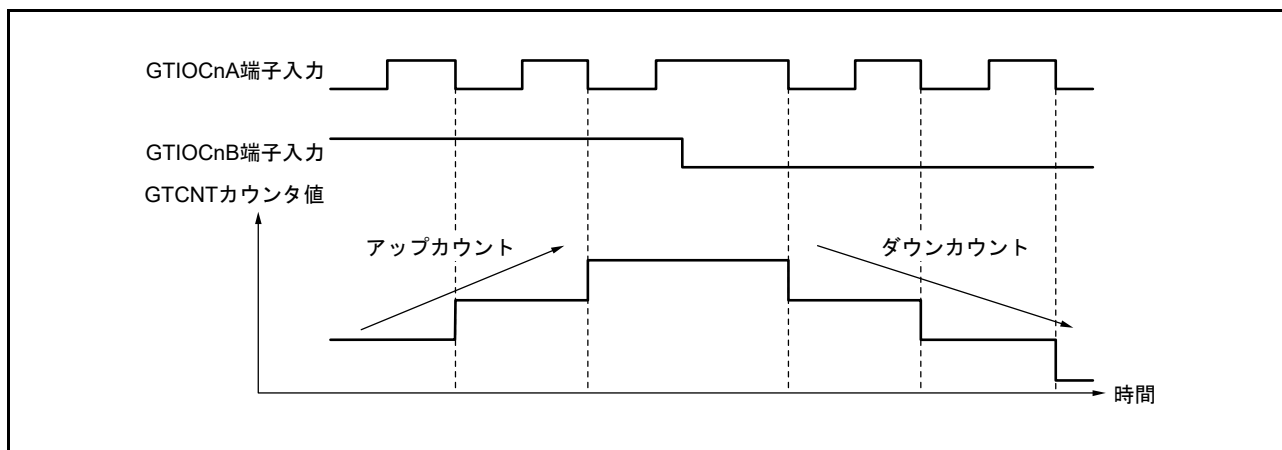
図 26.88 位相計数モード2の動作例 (n = 0 ~ 3)
