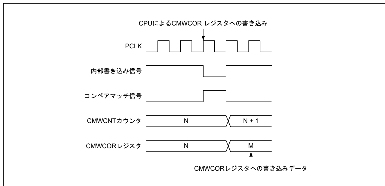
図 32.25 CMWCOR レジスタへの書き込みとコンペアマッチの競合
