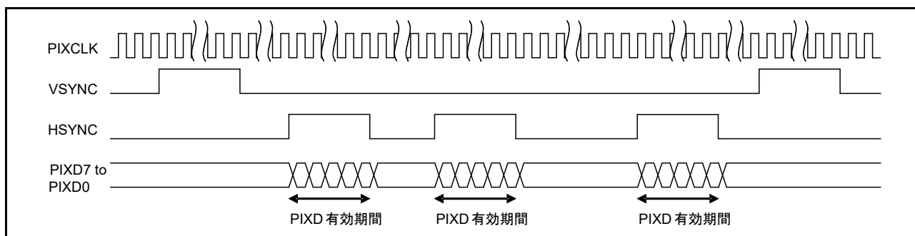
図 50.5 PDC 通信フォーマット (VPS = 1, HPS = 0)
