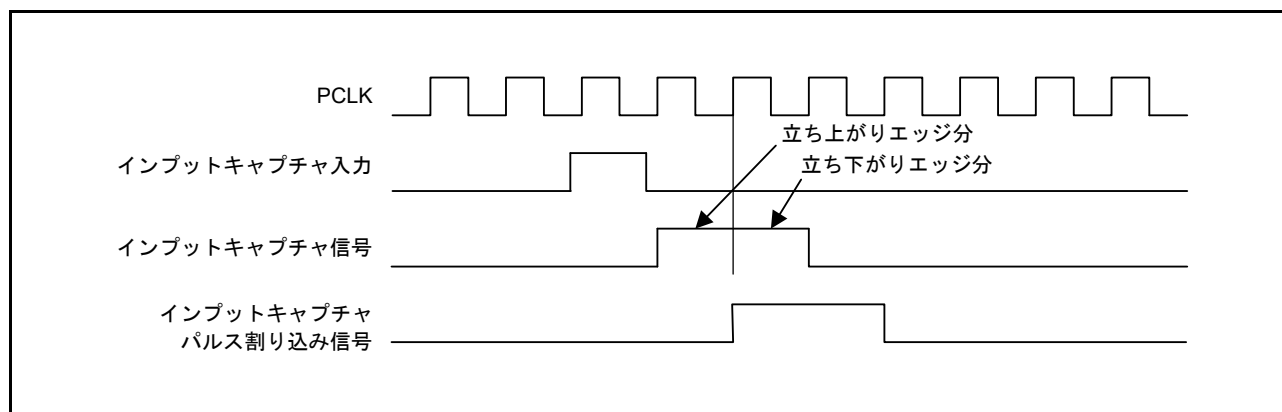
図 28.54 インพุットキャプチャパルス割り込みの連続出力
