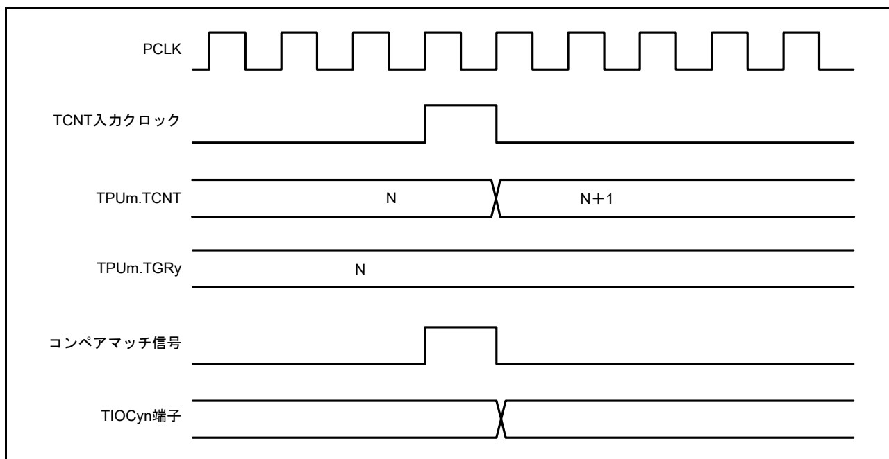
図 28.33 アウトプットコンペア出力タイミング
