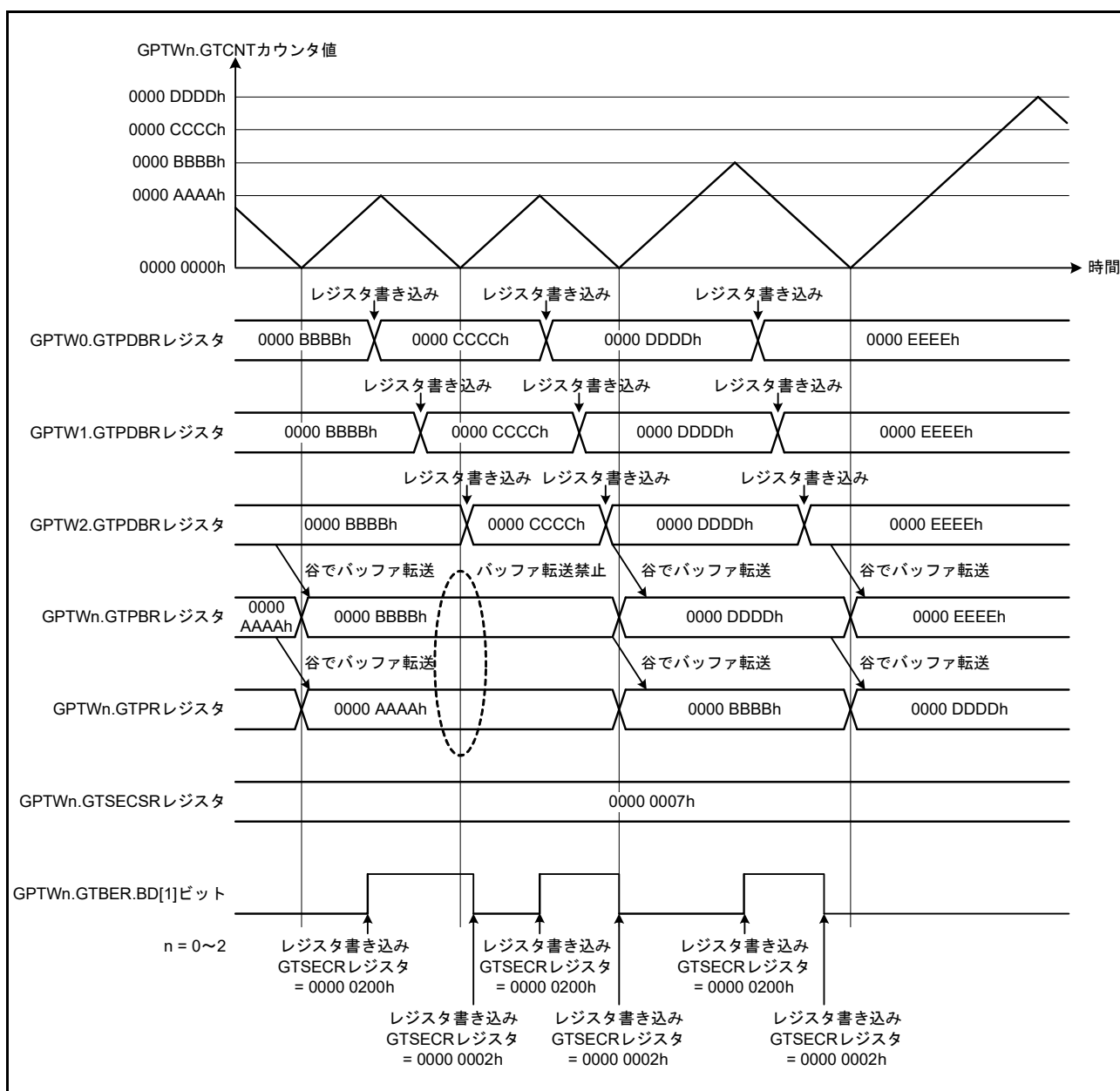
図 26.120 複数チャネルのバッファ動作の抑止動作例 (三角波、ダブルバッファ動作の場合)
