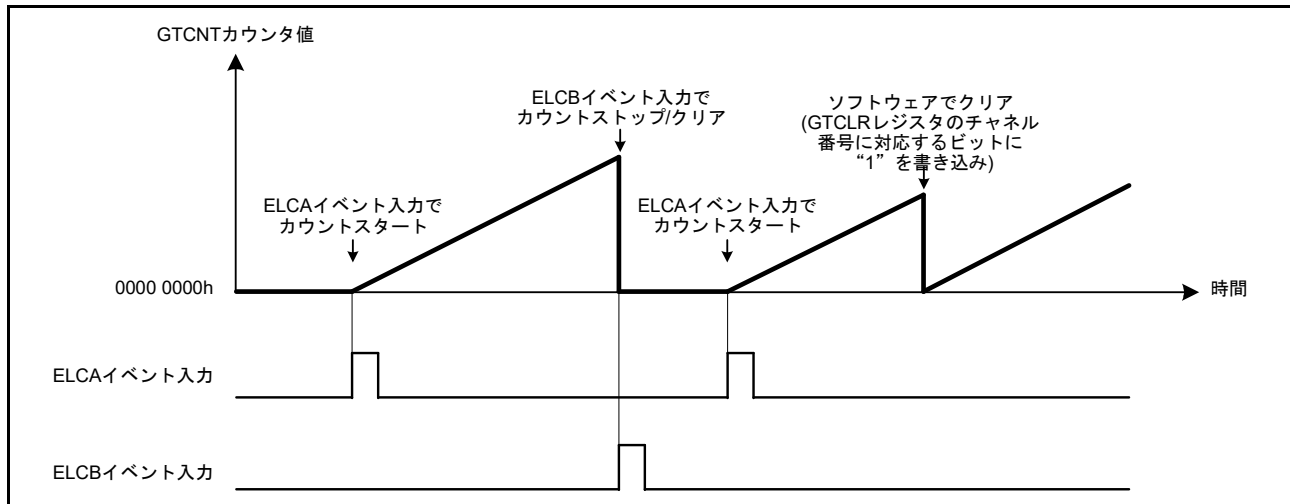
図 26.67 ハードウェア要因によるカウンタクリア動作例 (のこぎり波でアップカウント、ELCA イベント入力でスタート、ELCB イベント入力でカウントストップ/クリア時)
