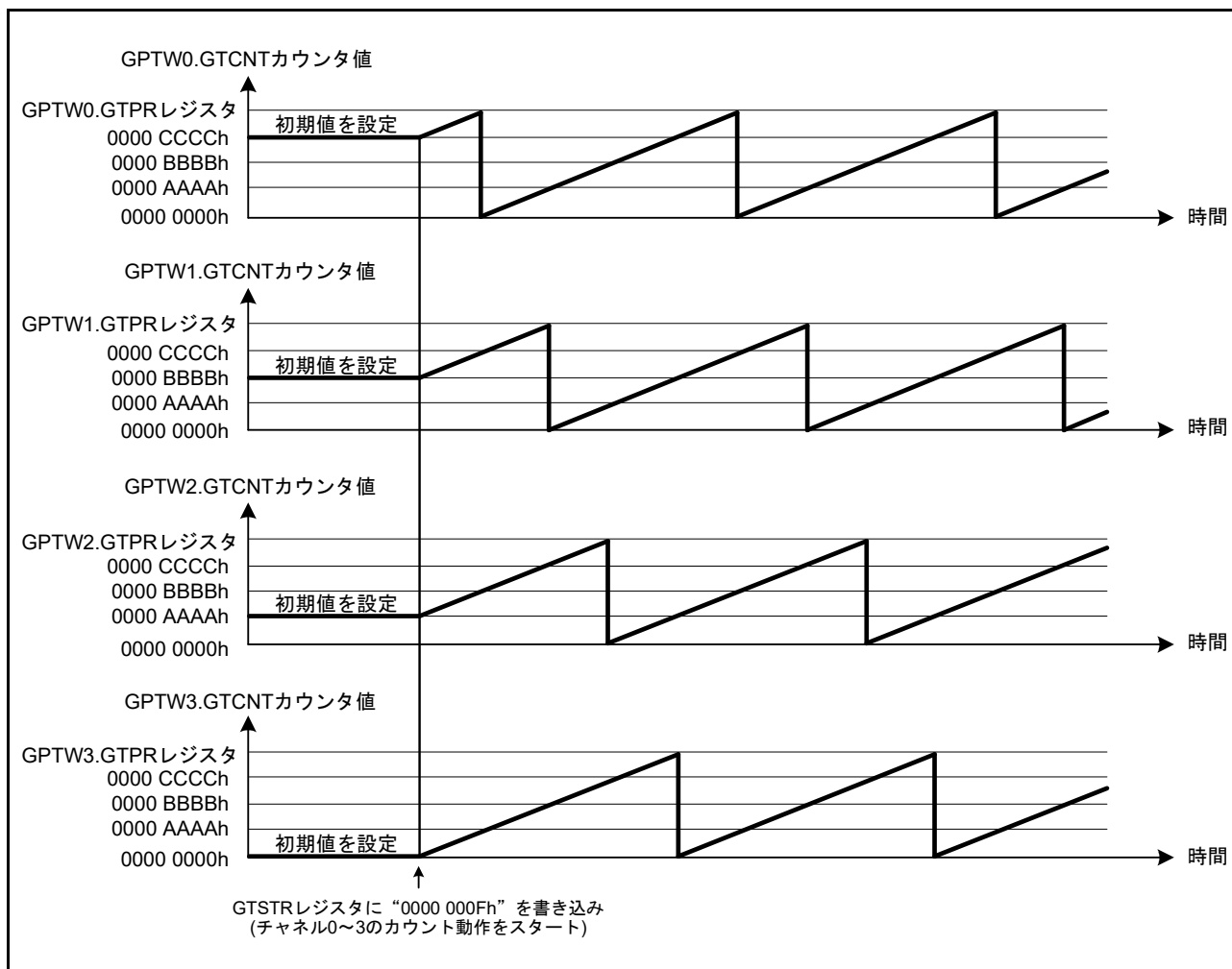
図 26.78 ソフトウェアによる位相シフトスタート動作例 (カウント周期 (GTPR レジスタ値) が同一のとき)
