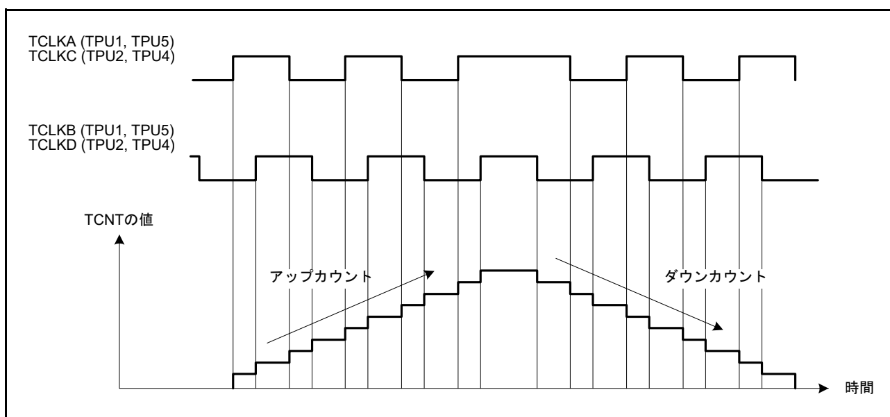
図 28.25 位相計数モード1の動作例
