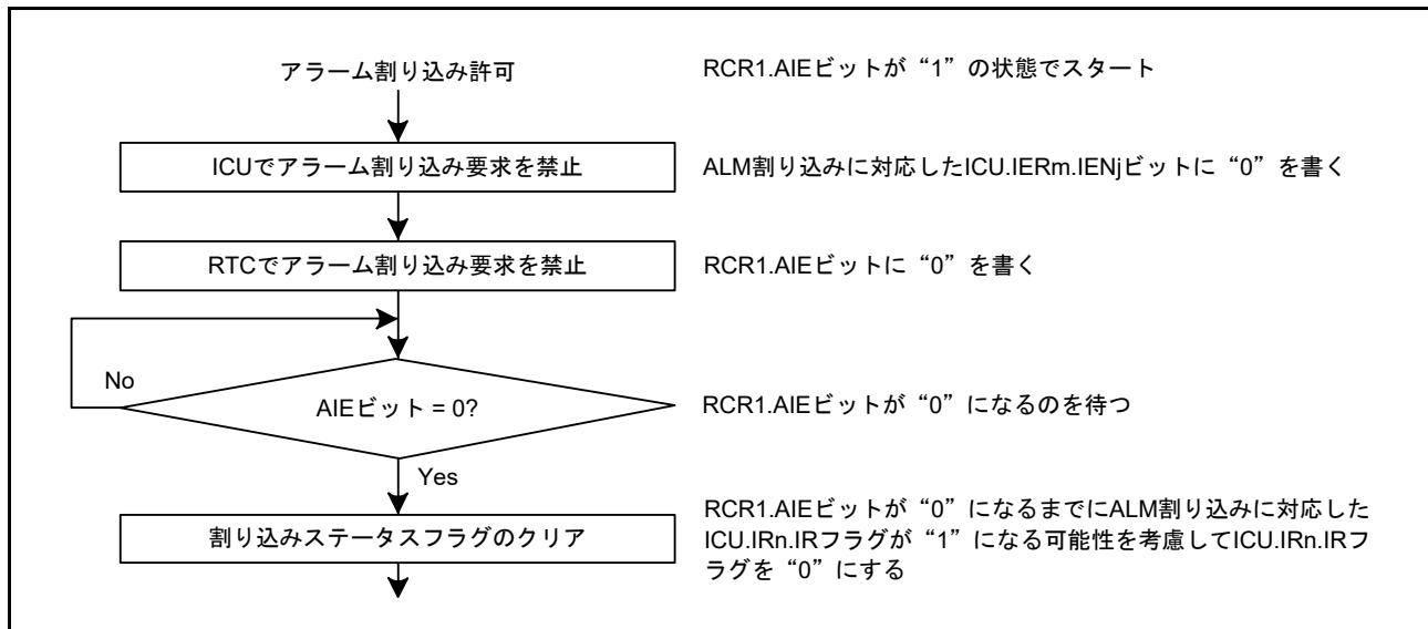
図 33.8 アラーム割り込み要求を禁止する手順
