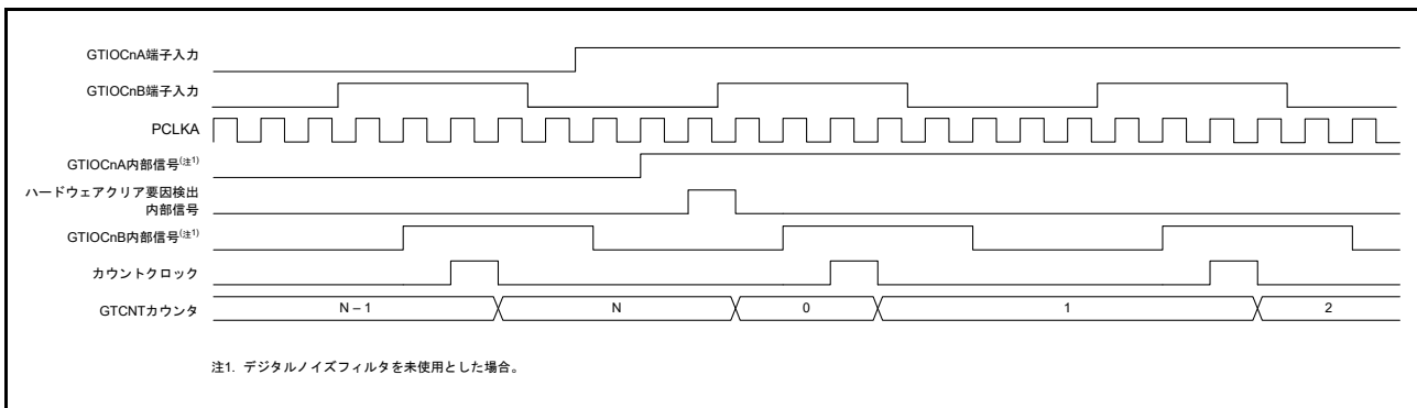
図 26.75 GTIOChA 端子入力の立ち上がりによるカウンタクリア動作タイミング例 (ハードウェア要因によるカウント動作時)
