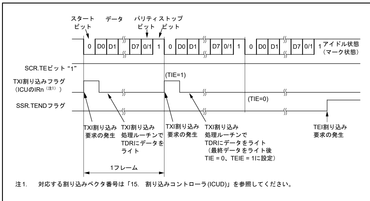
図 41.16 調歩同期式モードのシリアル送信の動作例 (3) (8ビットデータ / パリティあり / 1ストップビット / CTS機能使用しない / 送信中～送信終了時)
