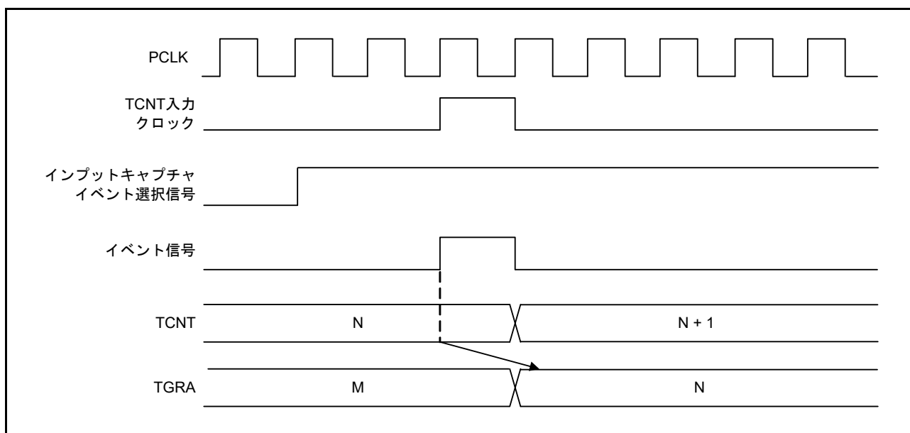
図28.58 イベント信号入力によるインพุットキャプチャ動作
