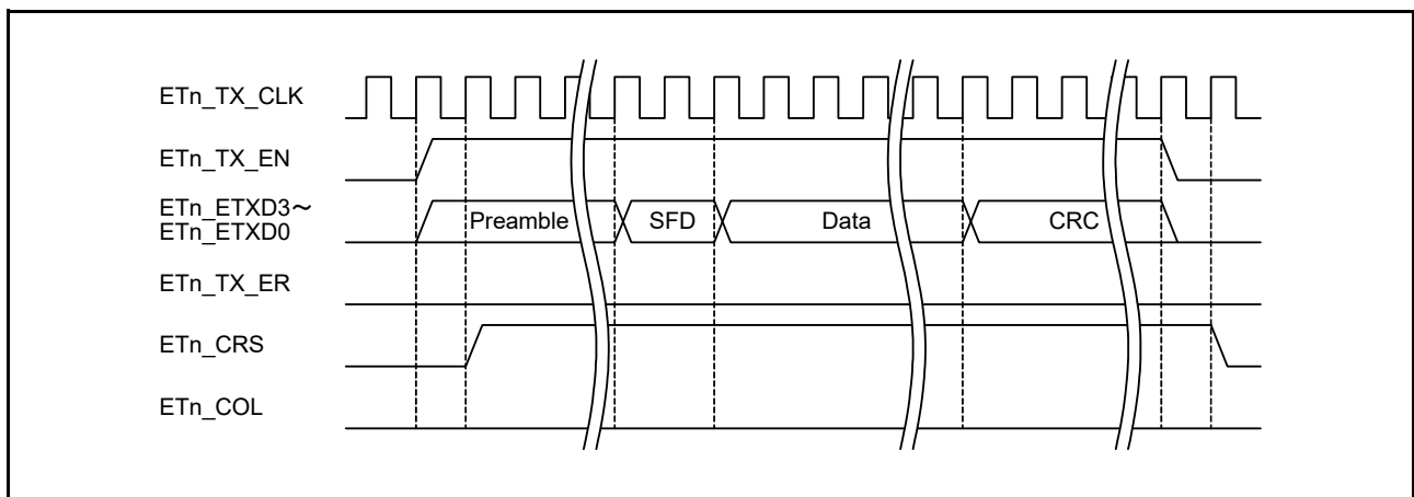
図 36.6 MII フレーム送信タイミング (正常時)
