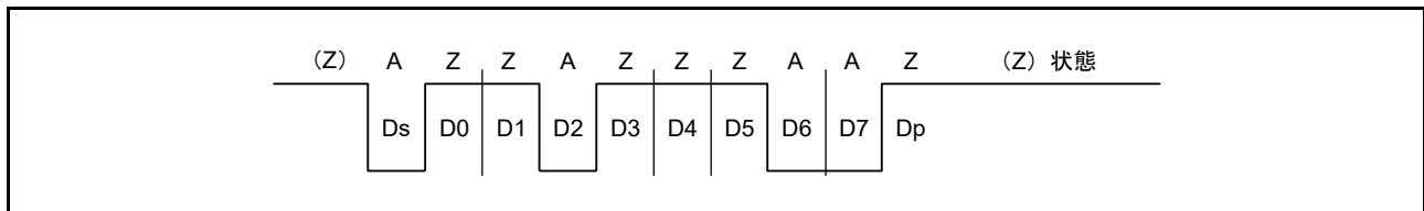
図 41.39 ダイレクトコンベンション (SCMR.SDIR ビット = 0、SCMR.SINV ビット = 0、SMR.PM ビット = 0)
