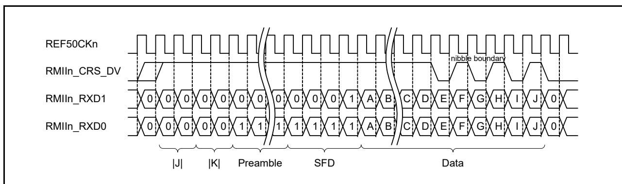
図 36.12 RMII フレーム受信タイミング (正常受信)
