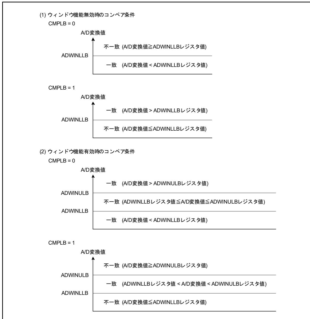
図 56.5 コンペア機能ウィンドウ B コンペア条件説明
