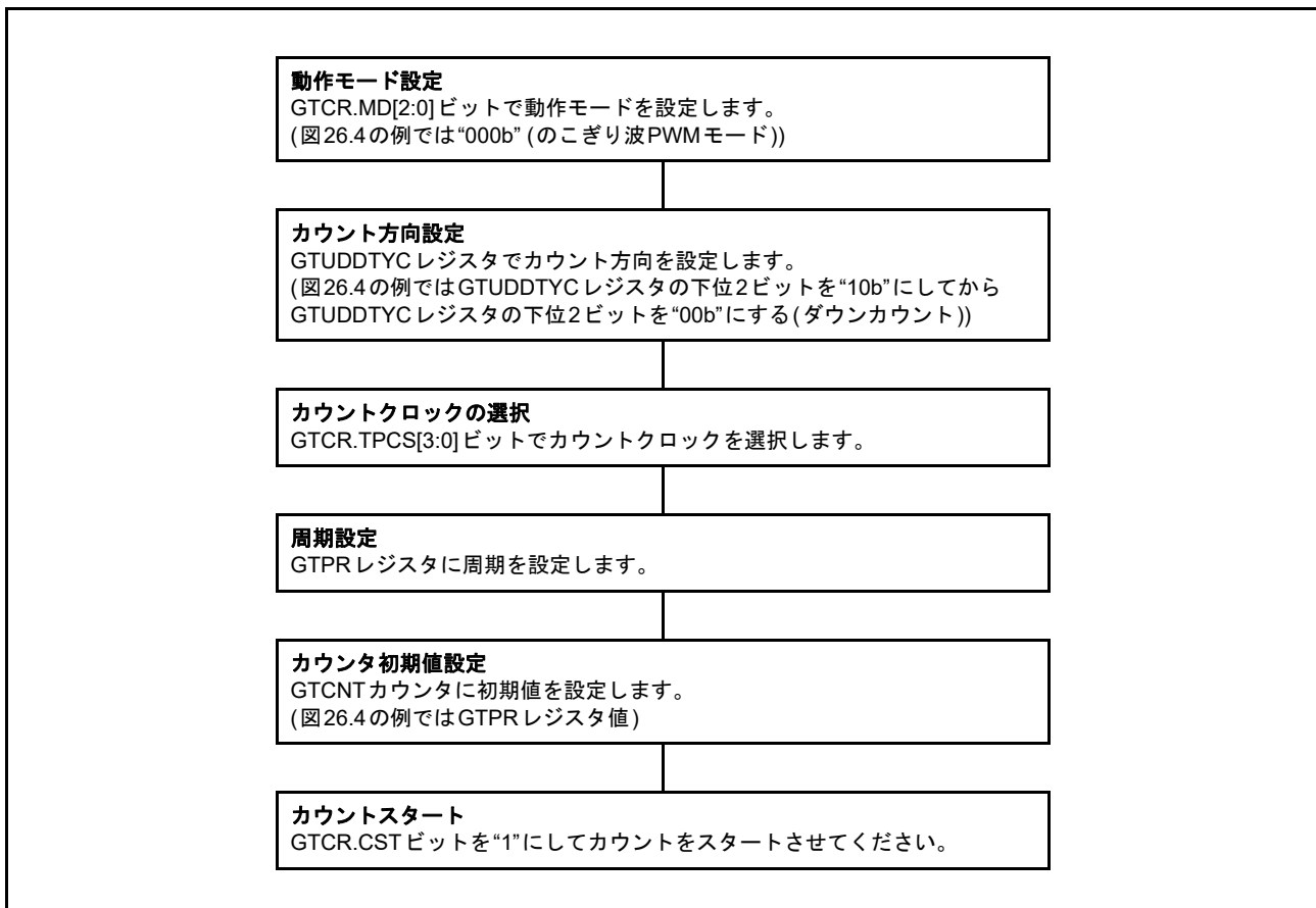
図 26.5 サイクルカウント動作設定例 (カウントクロックによるダウンカウント時)
