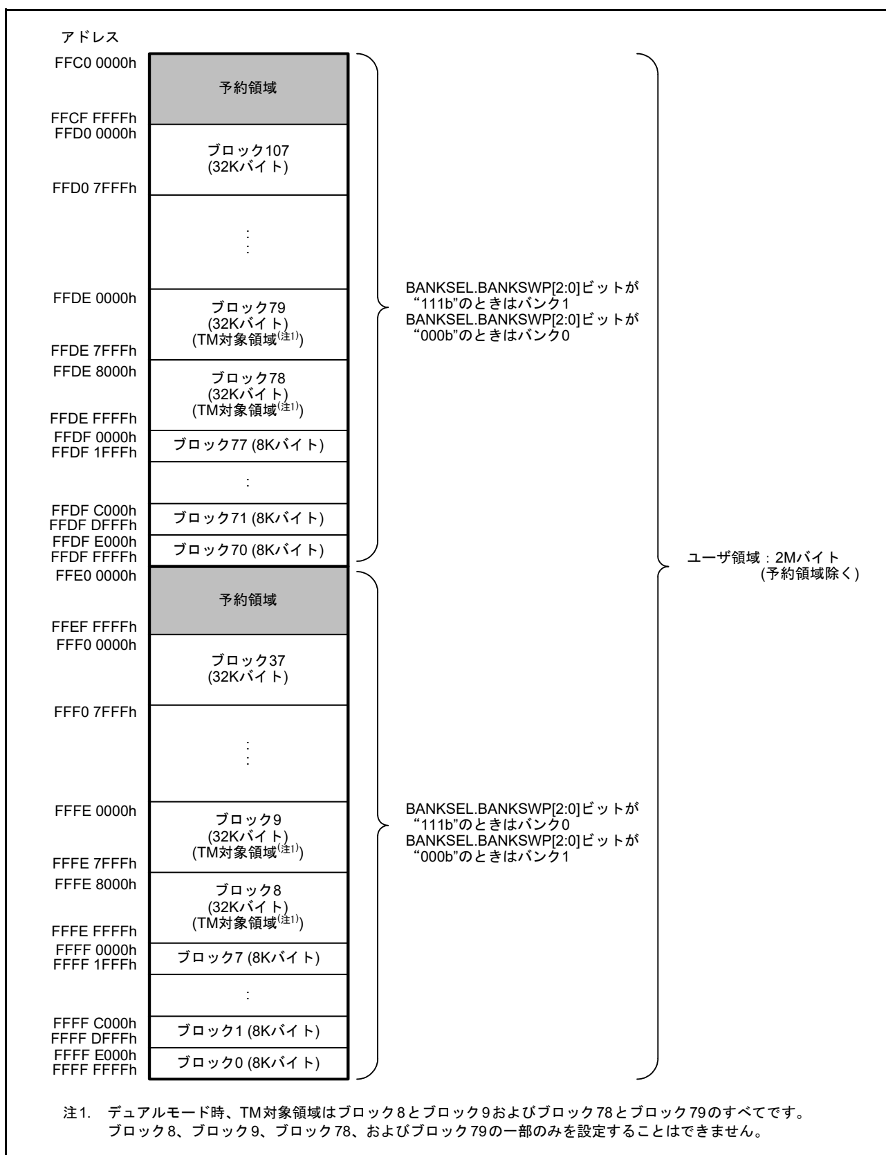
図 62.4 デュアルモード時のコードフラッシュメモリマッピング (コードフラッシュメモリ容量が2Mバイトの製品)
