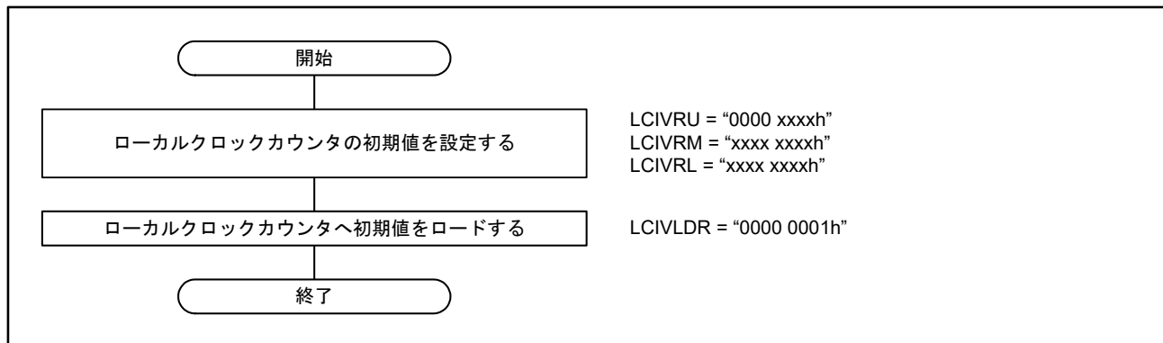
図37.30 ローカルクロックカウンタへの初期値設定の手順
