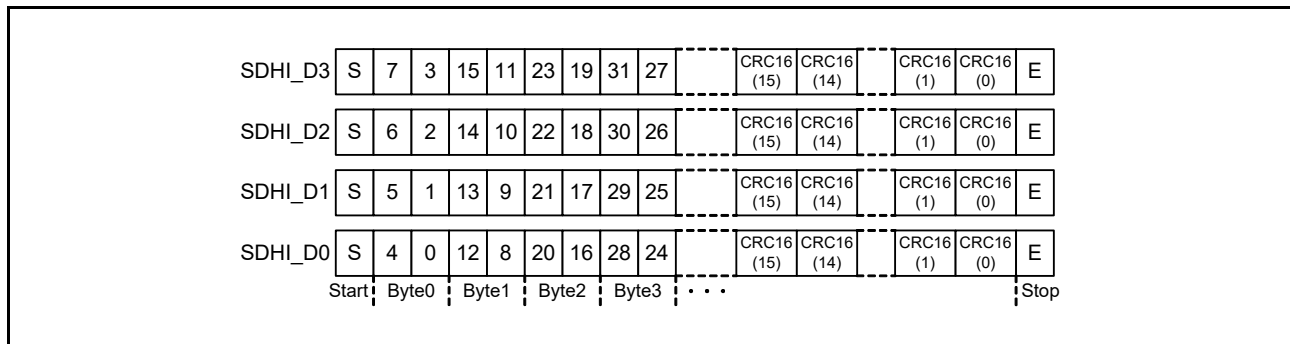
図 48.3 ワイドバスモードの転送フォーマット (SDOPT.WIDTH ビットが“0” のとき )
