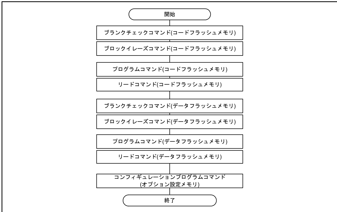
図 62.49 書き換え方法の例
