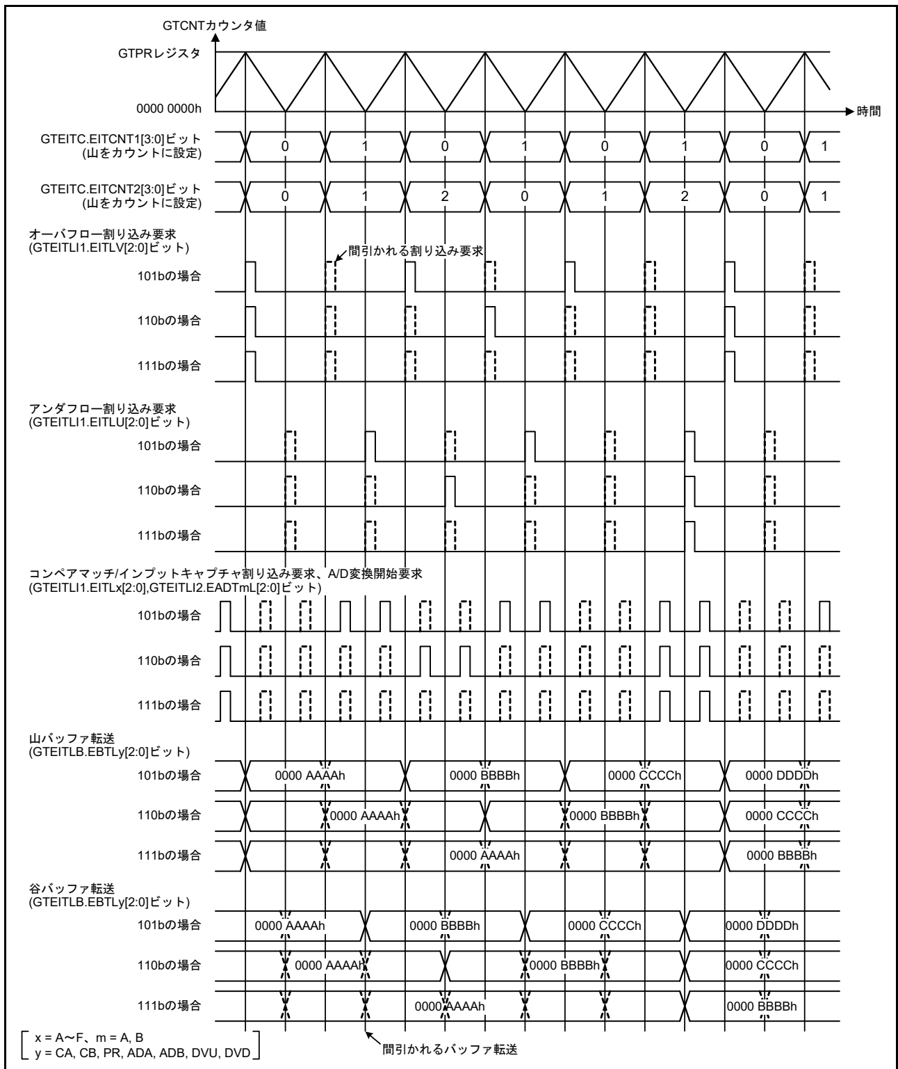
図 26.108 拡張割り込み間引き機能の動作例 (三角波、拡張割り込み間引き 1 間引き回数 1 で山をカウント、拡張割り込み間引き 2 間引き回数 2 で山をカウント、拡張割り込み間引きカウンタ 2 初期値 “0”、GTEITC.EITCNTk ビット (k = 1, 2) が GTEITC.EIVTTk ビット以外の期間で間引く場合)
