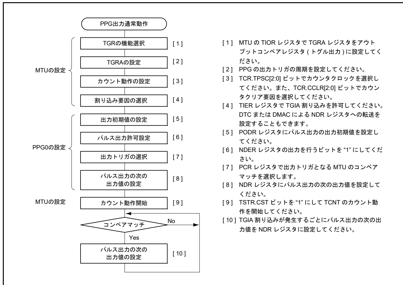
図 29.6 パルス出力通常動作の設定手順例 (PPG0 の設定)
