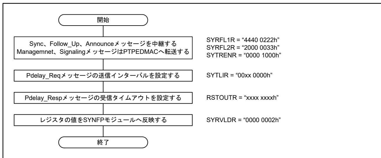
図37.23 P2P TC動作の開始手順
