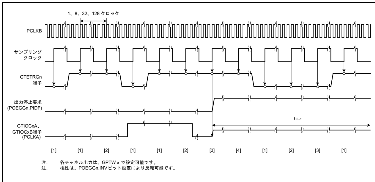
図 27.3 デジタルノイズフィルタの動作例
