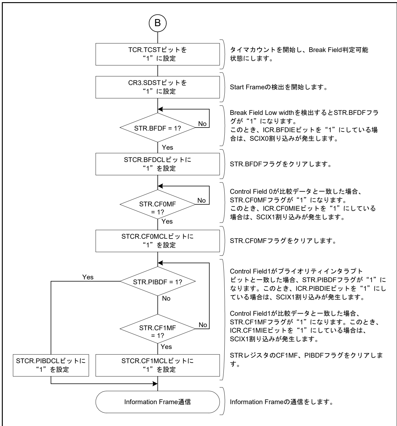
図 41.70 Start Frame 受信フローチャート例 (2)
