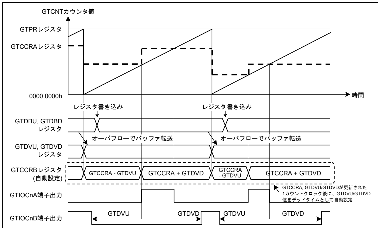
図 26.47 デッドタイム自動設定機能の動作例 ( のこぎり波ワンショットパルスモード、アップカウント、GTDVU/GTDVD レジスタはバッファ動作、アクティブレベルは High の場合 ) (n = 0 ~ 3)
