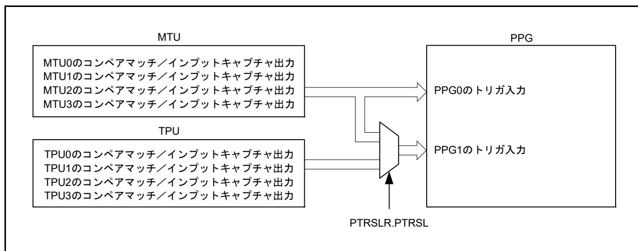
図 29.3 PPGトリガセレクトのブロック図
