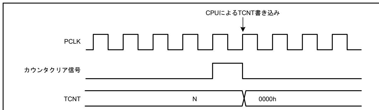
図 28.44 TPUm.TCNT への書き込みとクリアの競合
