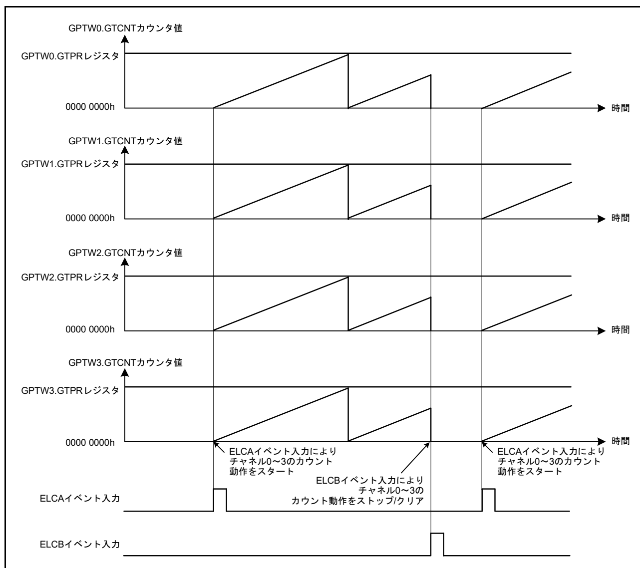
図 26.79 ハードウェア要因による同時スタート/ストップ/クリア動作例 (カウンタ周期 (GTPR レジスタ値) が同一のとき)
