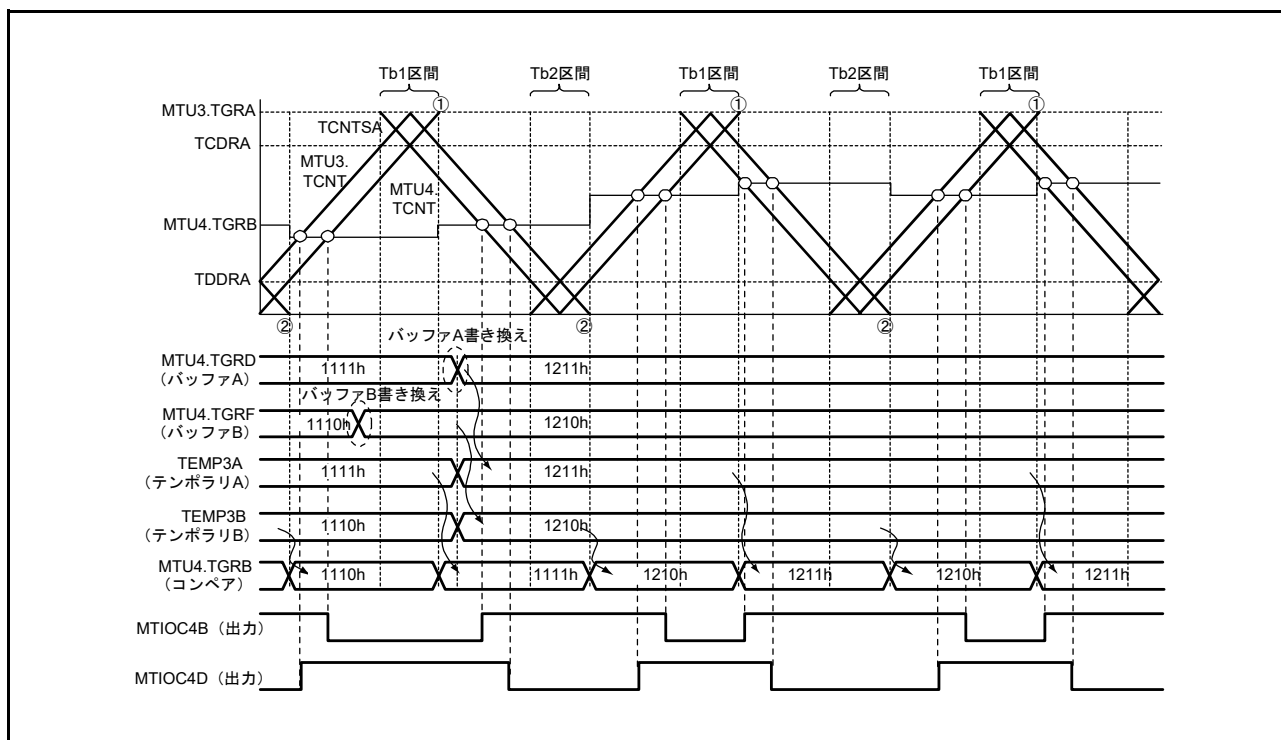
図 24.83 ダブルバッファ機能の動作例
