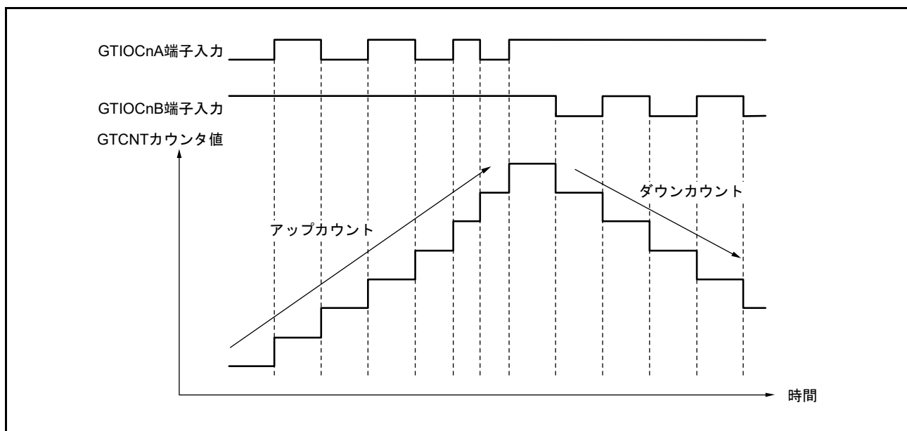
図 26.93 位相計数モード3の動作例 (n = 0 ~ 3)
