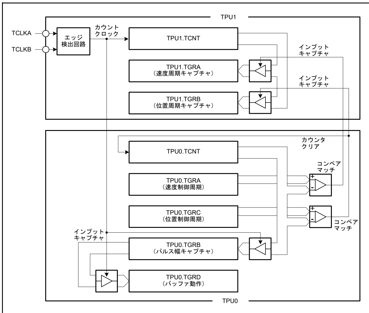
図 28.29 位相計数モードの応用例
