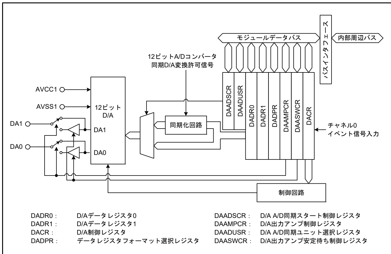
図57.1 12ビットD/Aコンバータのブロック図
