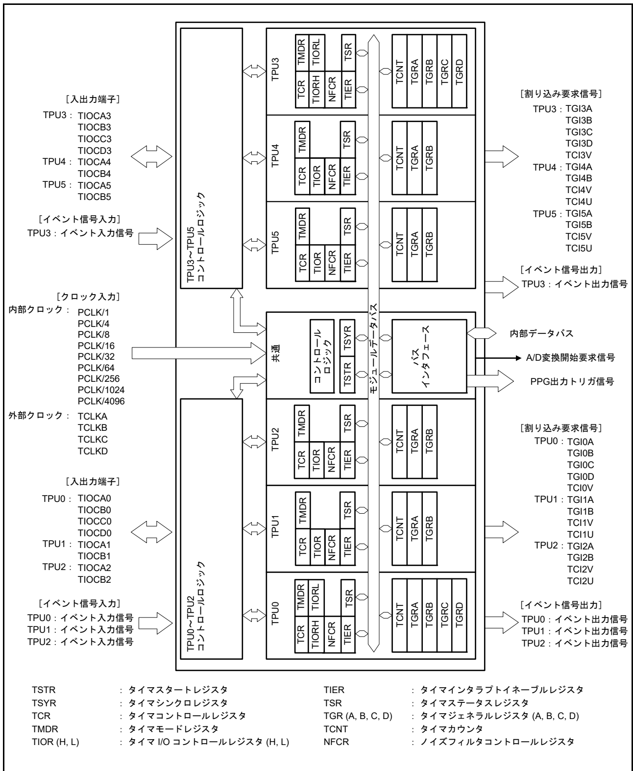
図 28.1 TPU のブロック図
