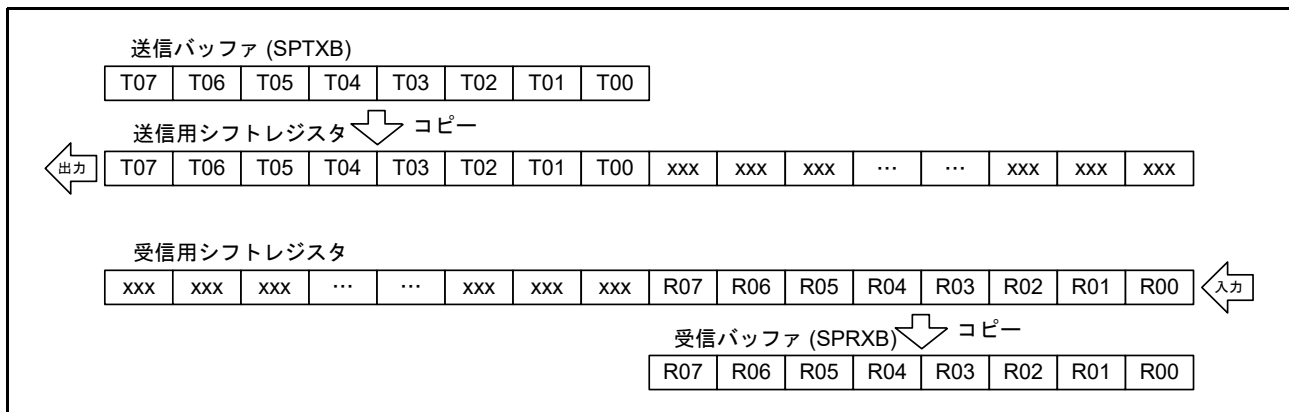
図 45.8 MSB ファースト転送 (8 ビットデータ)
