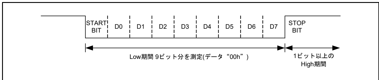
図 62.41 ビットレート自動調整時の SCI 送受信フォーマット
