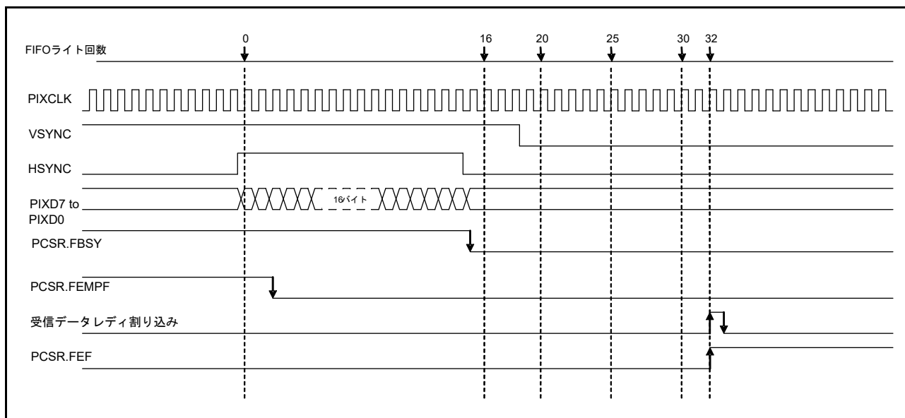
図 50.13 フレームエンド時の継続受信動作例
