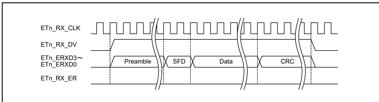
図 36.8 MII フレーム受信タイミング (正常受信)
