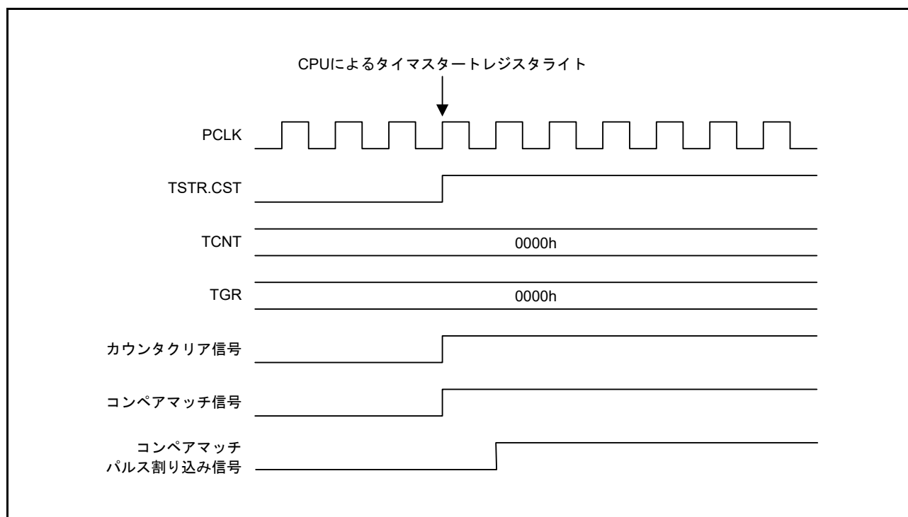
図 28.53 コンペアマッチパルス割り込みの連続出力
