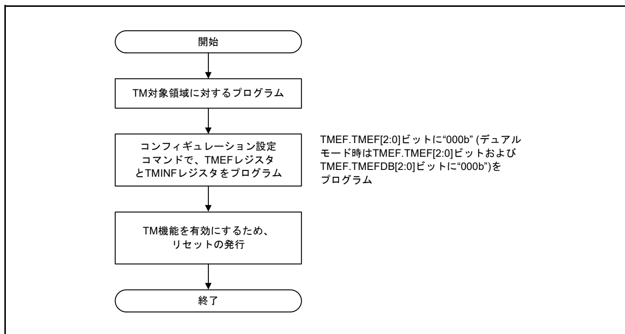
図 62.57 ブートモードで TM 機能を有効にするためのフロー
