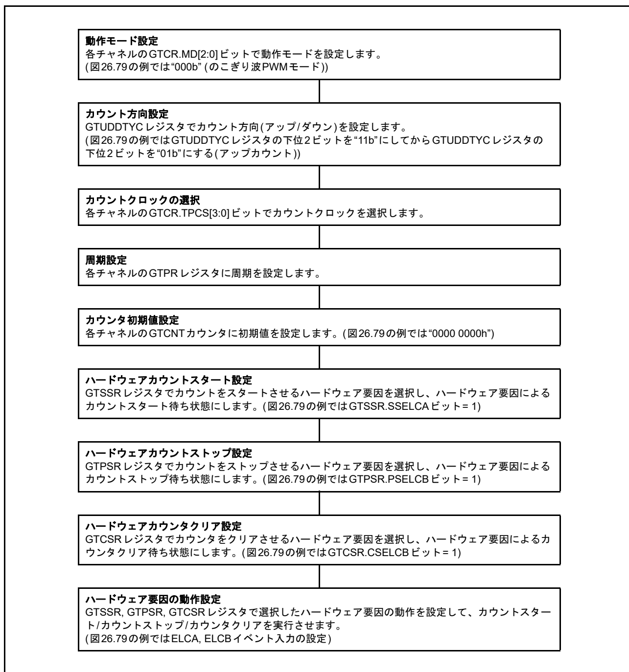
図 26.80 ハードウェア要因による同時スタート設定例
