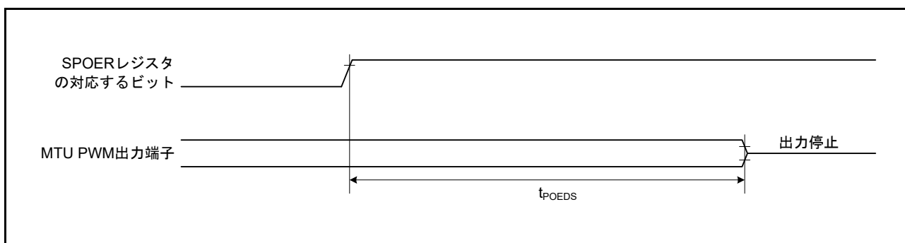
図 63.45 POE 出力ディセーブル時間 (レジスタ設定)
