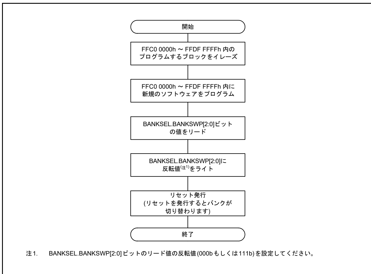
図 62.33 起動バンク選択フロー例 (コードフラッシュメモリ容量が4Mバイトの製品の例)
