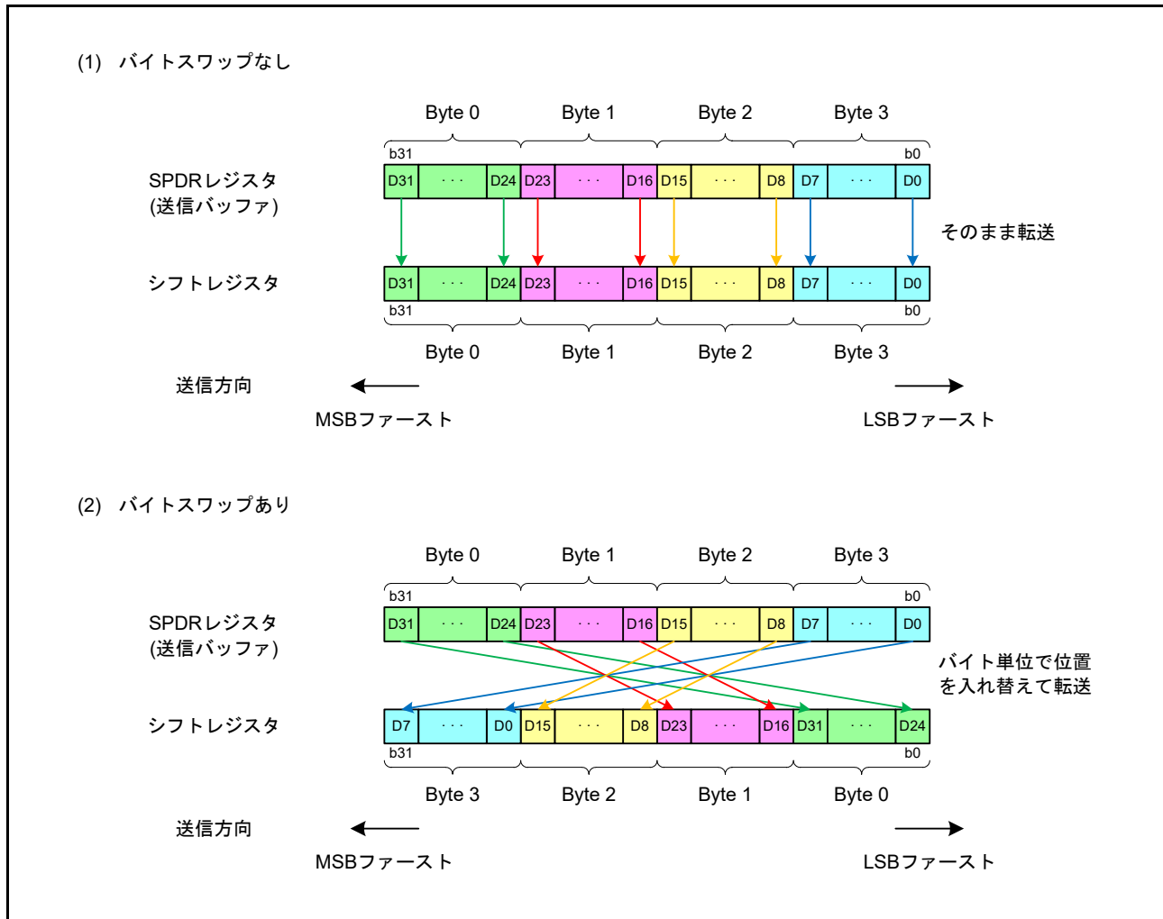
図 44.22 MSB/LSB ファーストとバイトスワップあり/なしの設定と送信データ変換
