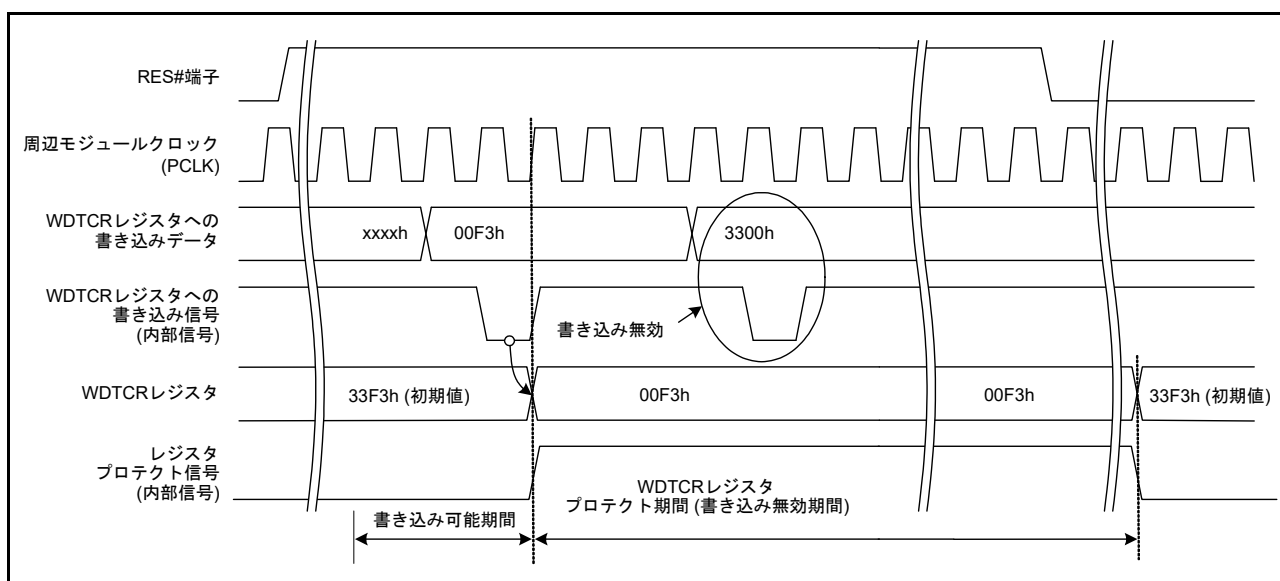
図 34.5 WDTCR レジスタ書き込み制御波形
