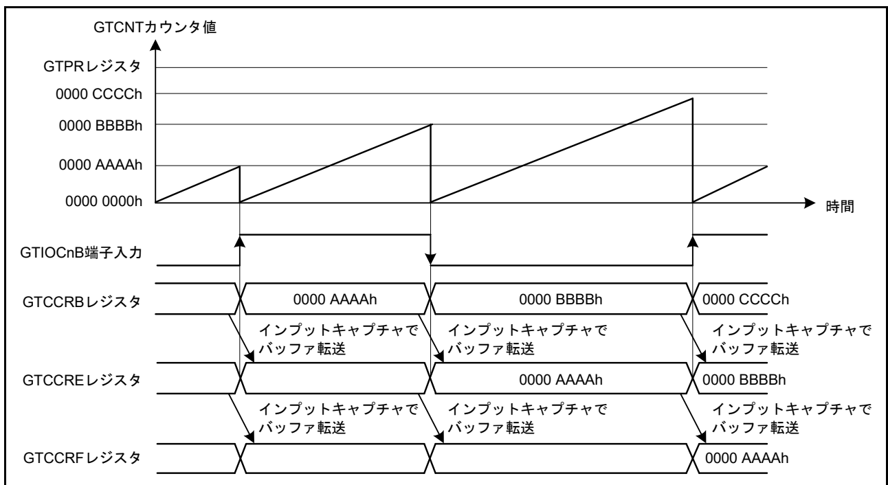
図 26.31 GTCCRA, GTCCRB レジスタのダブルバッファ動作例 (のこぎり波でアップカウント、GTIOcNB 端子入力の両エッジで GTCNT カウンタクリアおよびインプットキャプチャの場合) (n = 0 ~ 3)
