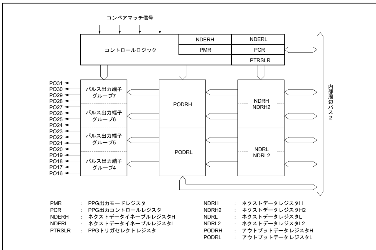
図 29.2 PPG1 のブロック図
