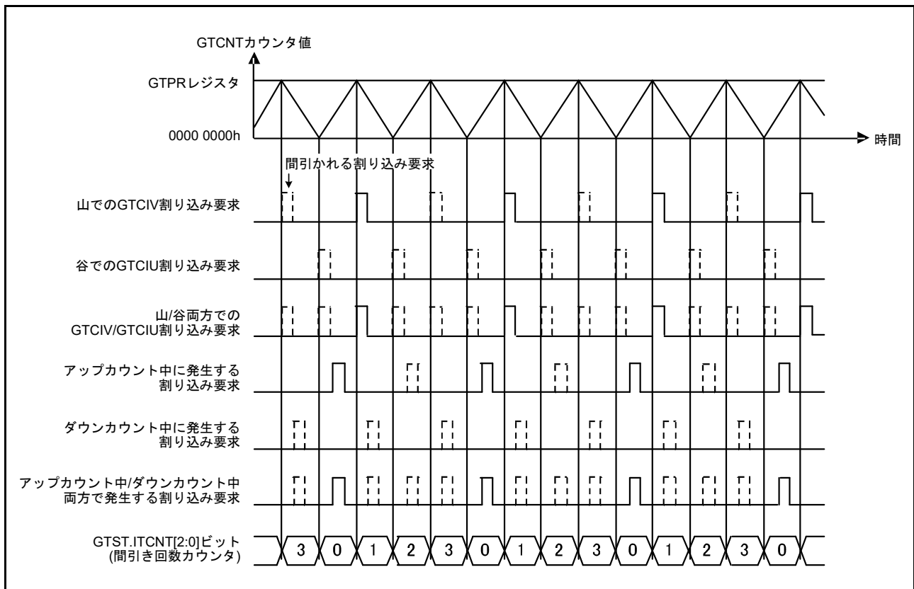
図 26.101 割り込み間引き機能の動作例 (三角波、谷 / 山両方をカウントして間引き、間引き回数 3、ダウンカウントで間引き開始の場合)
