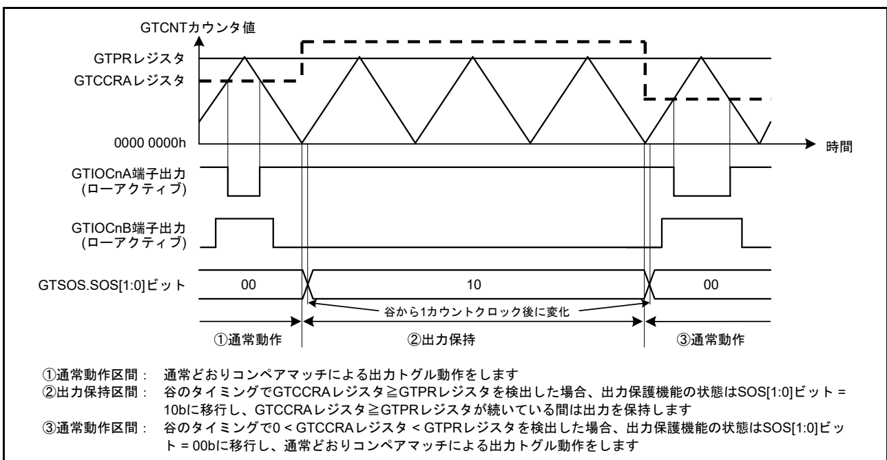
図 26.131 谷のバッファ転送で GTCCRA レジスタ \geq GTPR レジスタが設定された場合の出力保護機能の動作例 (谷のバッファ転送で 0 < \text{GTCCRA レジスタ} < \text{GTPR レジスタ} に復帰、アクティブレベルは Low の場合) ( n = 0 \sim 3 )
