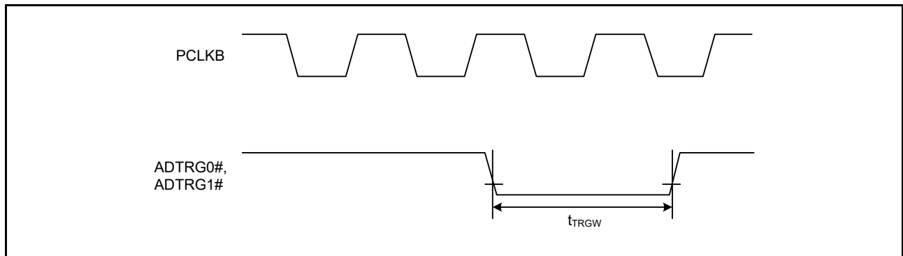
図 63.97 A/Dコンバータトリガ入力タイミング
