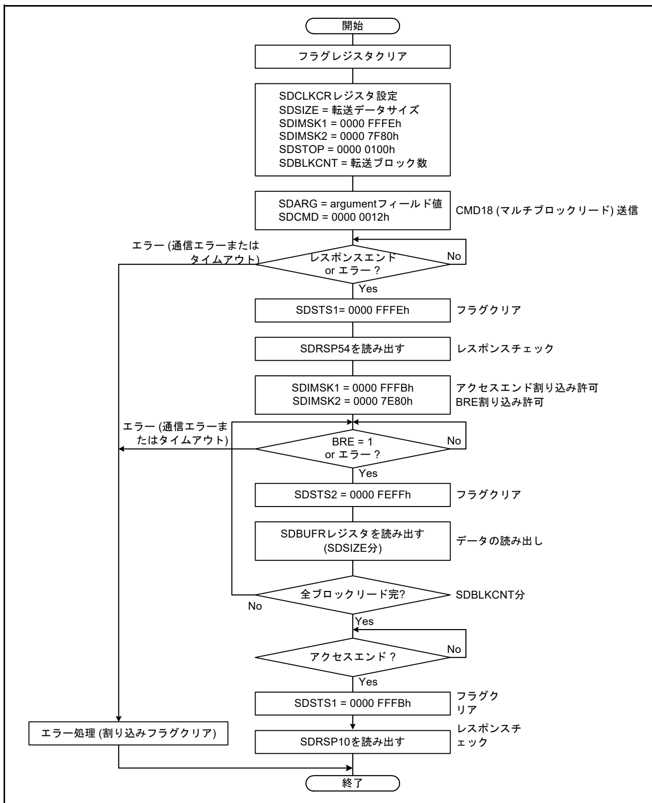
図 48.12 マルチブロックリードコマンドの送信例
