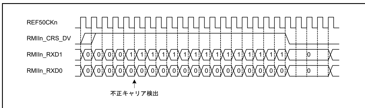
図 36.13 RMII フレーム受信タイミング (不正キャリア検出を伴う受信)
