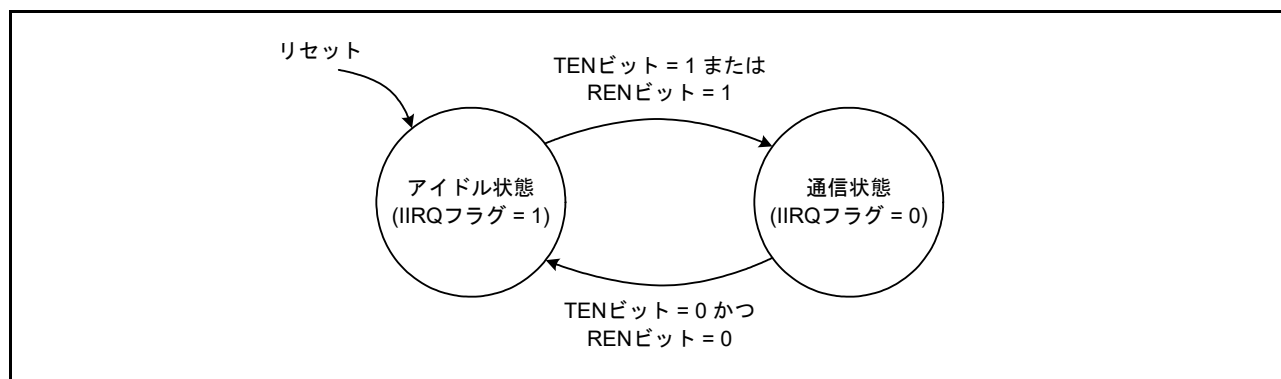
図 47.20 SSIE の状態遷移
