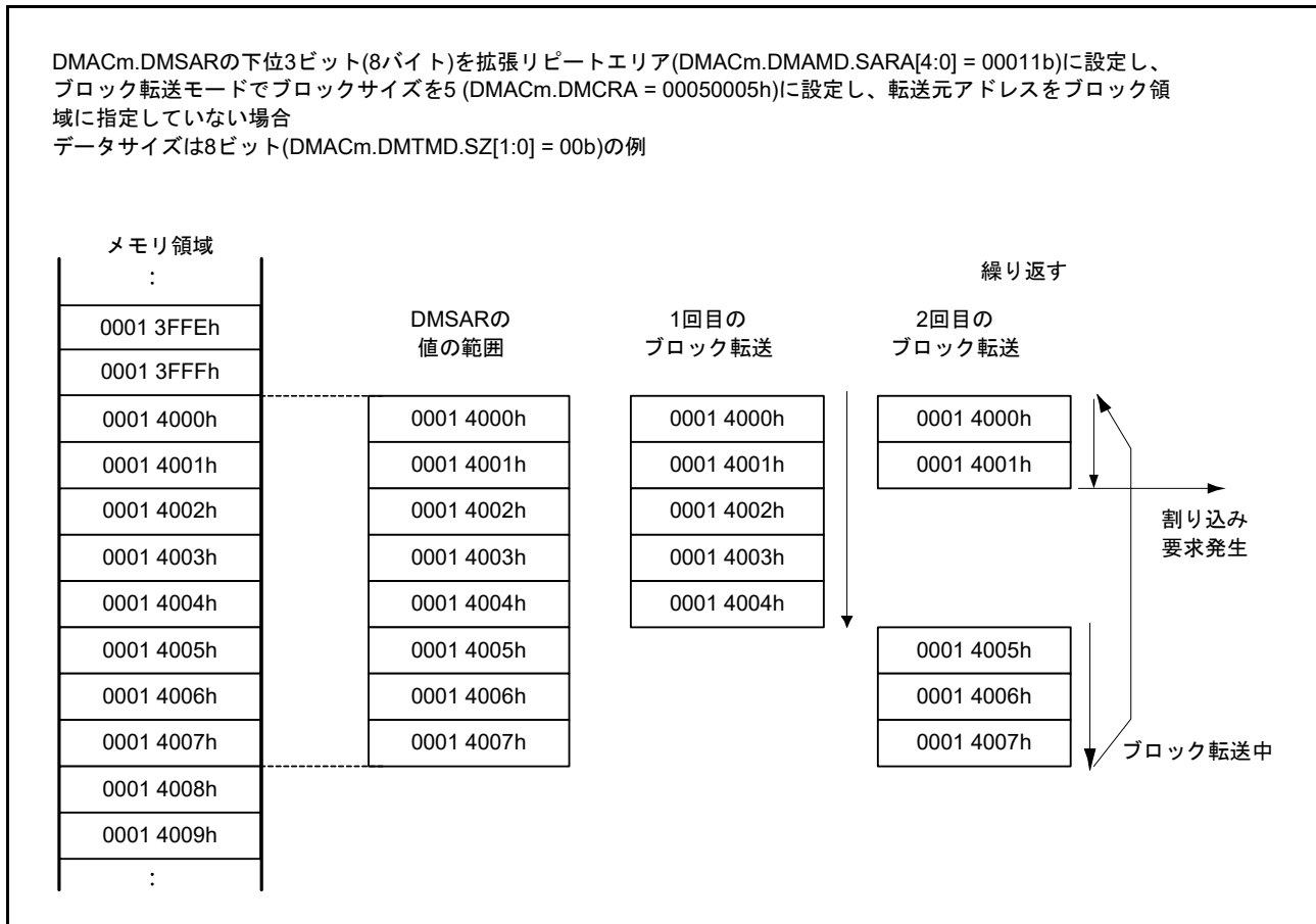
図 18.6 ブロック転送モードと拡張リポートエリア機能を併用した例
