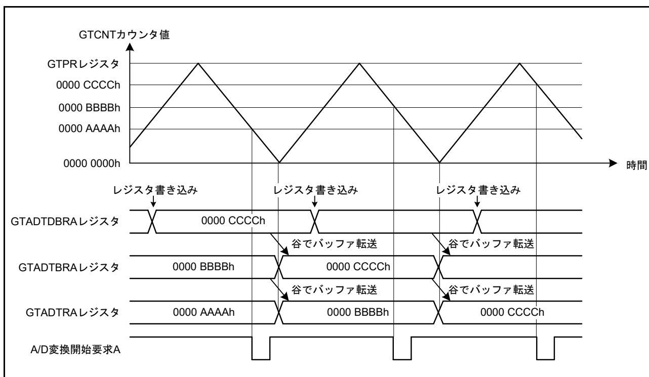
図 26.34 GTADTRA, GTADTRB レジスタのダブルバッファ動作例 (三角波、谷でバッファ転送、ダウンカウントで A/D 変換開始要求発生の場合)
