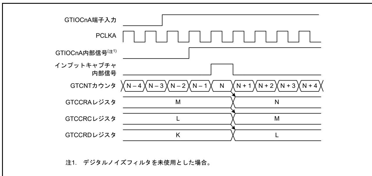
図 26.20 GTIOCnA 端子入力立ち上がりによるインプットキャプチャ動作タイミング例
