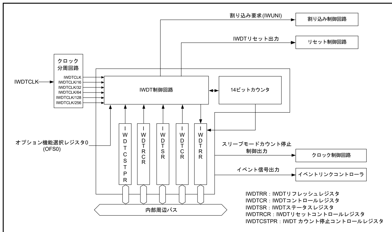
図 35.1 IWDT のブロック図
