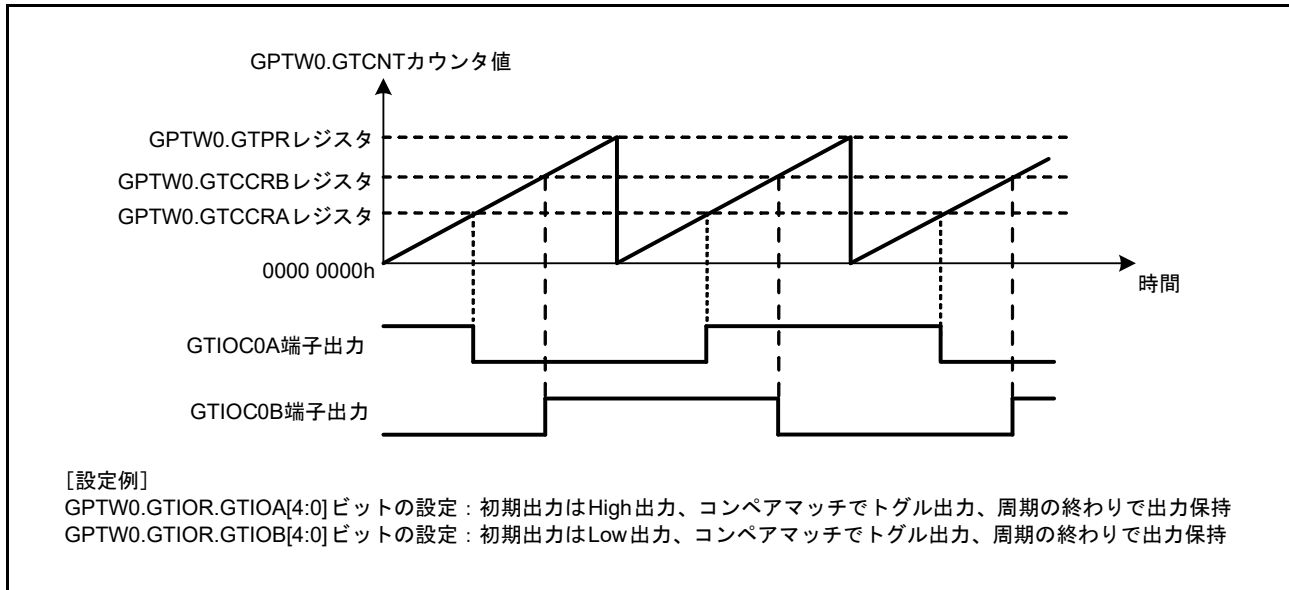
図 26.14 トグル出力動作例 (1)
