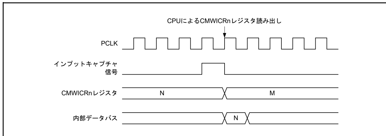
図 32.28 CMWICRn レジスタの読み出しとインプットキャプチャの競合
