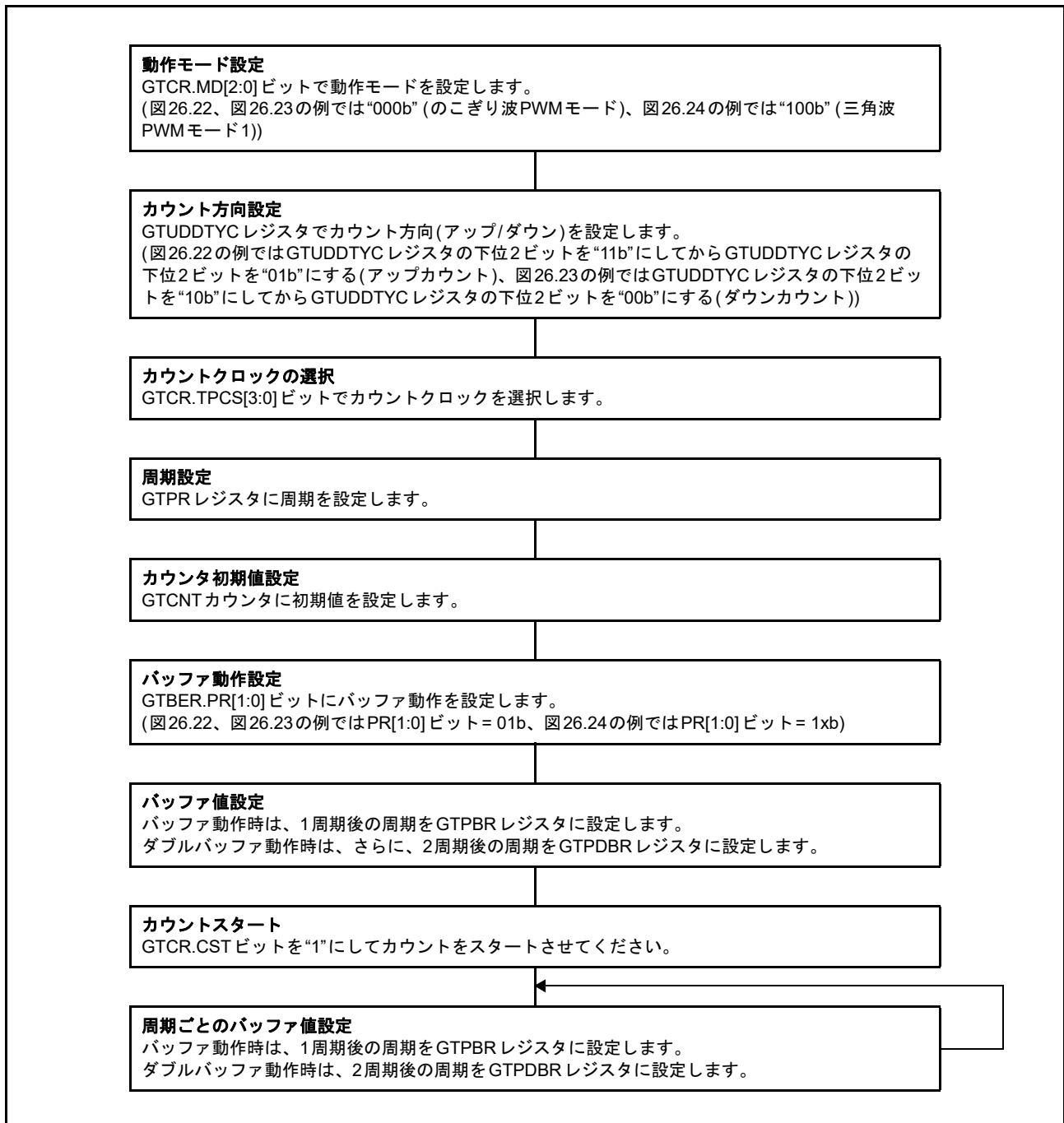
図 26.25 GTPR レジスタのバッファ動作設定例
