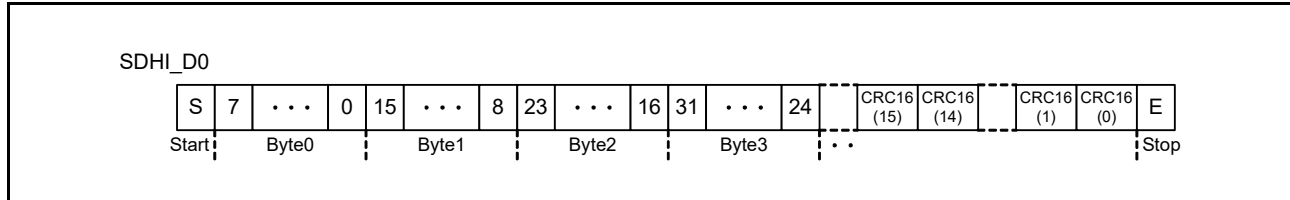
図 48.2 デフォルトバスモードの転送フォーマット (SDOPT.WIDTH ビットが“1” のとき )
