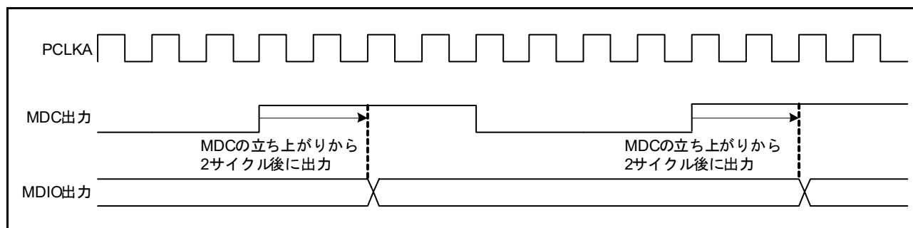
図 39.9 PCLKA の 2 サイクル遅延時のホールド時間調整タイミング
