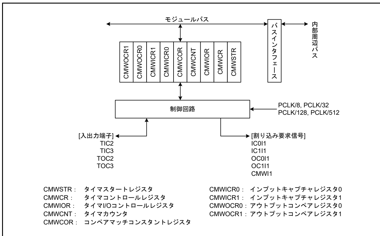
図 32.2 CMTW1 のブロック図
