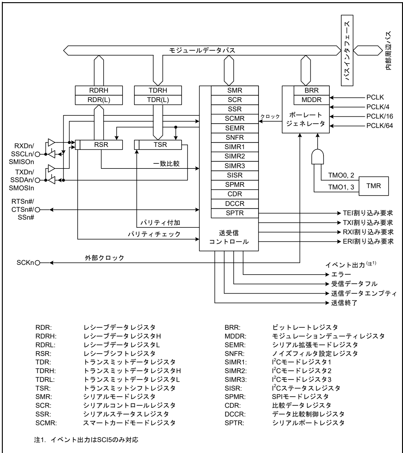
図 41.2 SCIj (SCI5, SCI6) のブロック図
