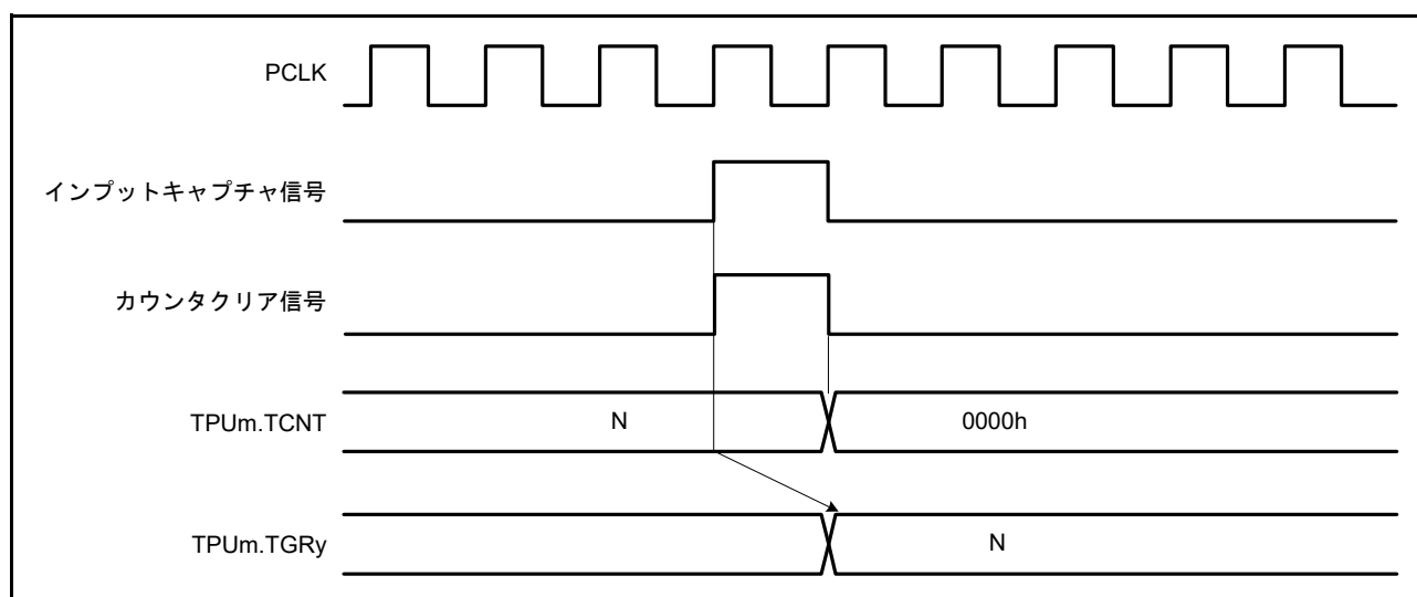
図 28.36 カウンタクリアタイミング (インプットキャプチャ)
