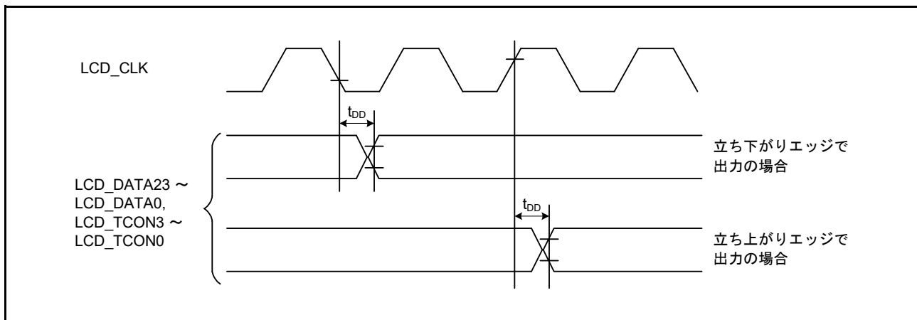
図 63.96 LCD 出力データタイミング
