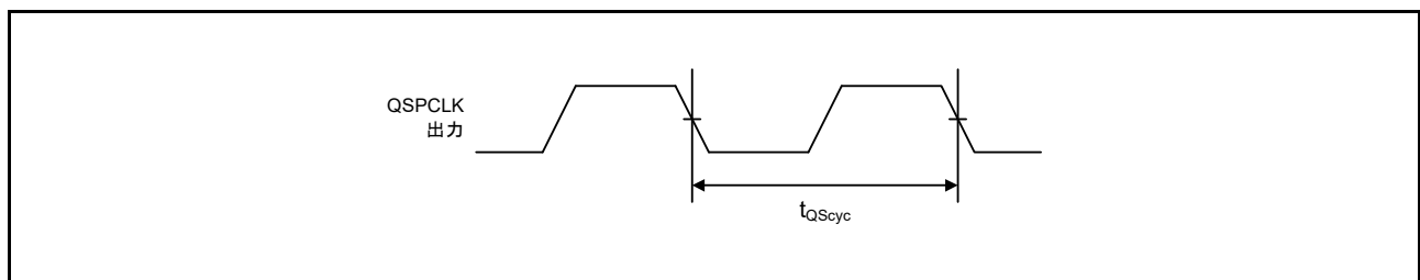
図 63.70 QSPI クロックタイミング
