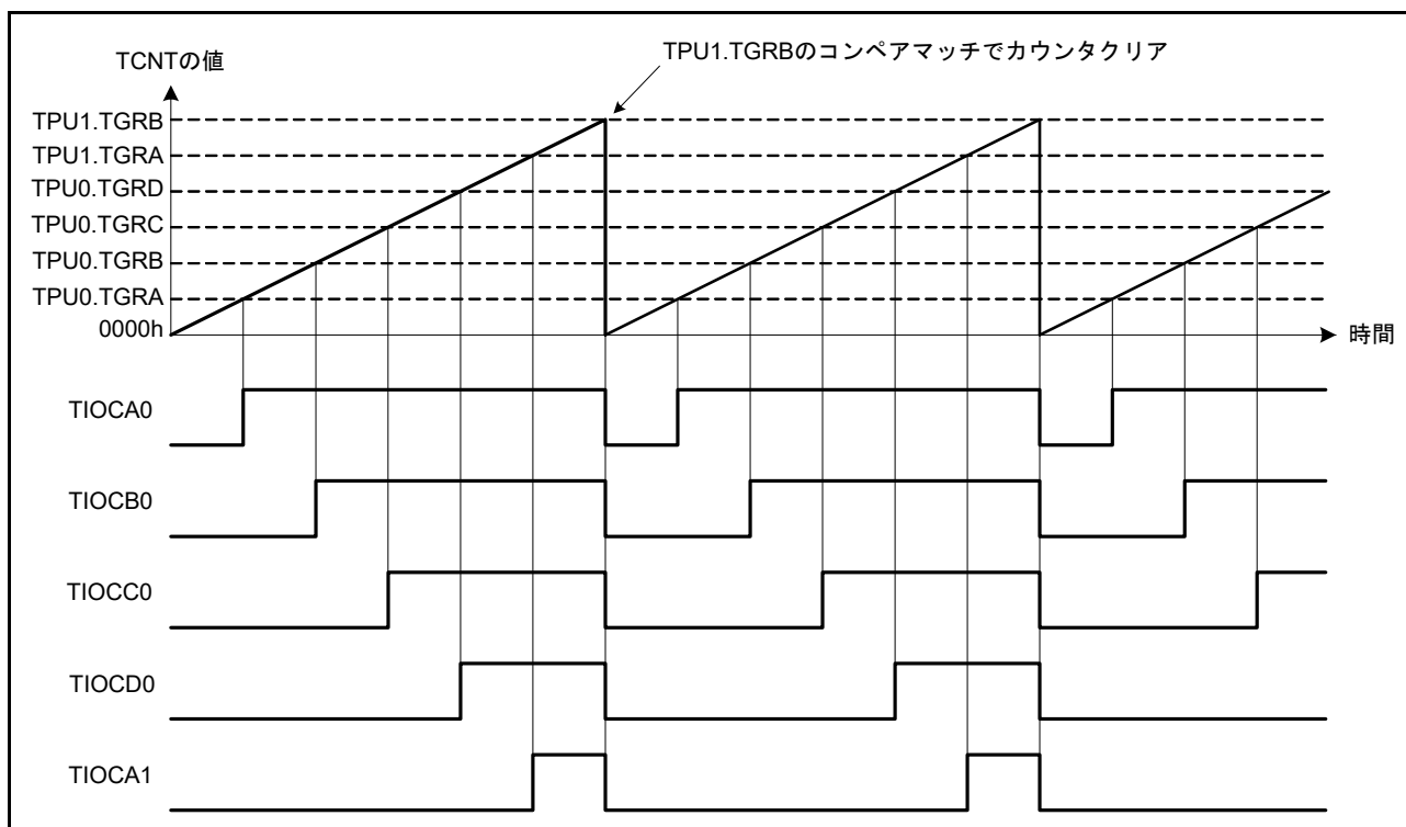
図 28.22 PWM モードの動作例 (2)
