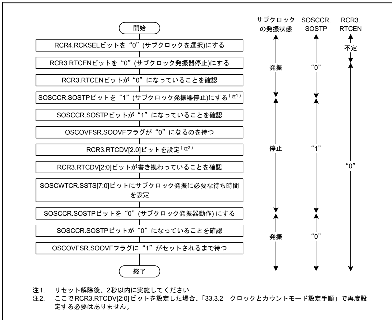
図 9.14 サブクロックをシステムクロックのみに使用する場合の初期化フローチャート例
