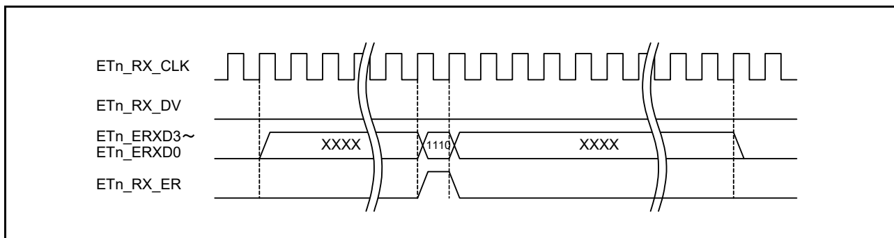
図 36.10 MII フレーム受信タイミング (受信エラー (2) 不正キャリア検出通知)
