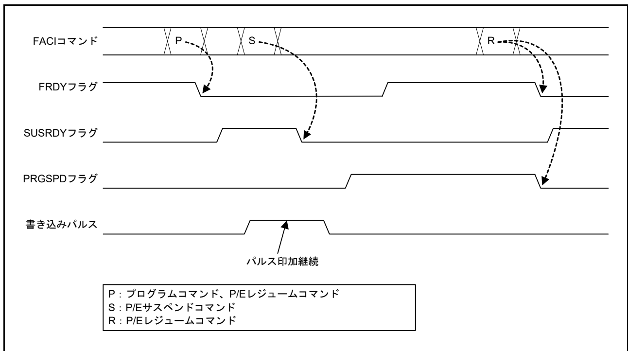
図 62.18 プログラム処理の中断動作
