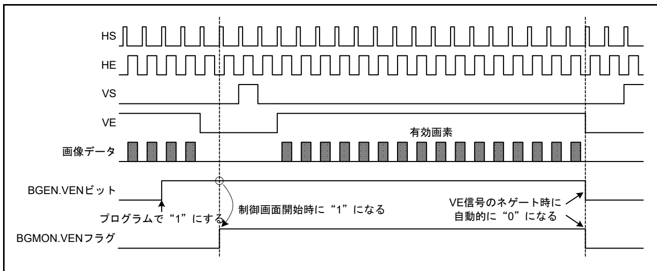
図 51.22 内部動作へのレジスタ値反映制御信号
