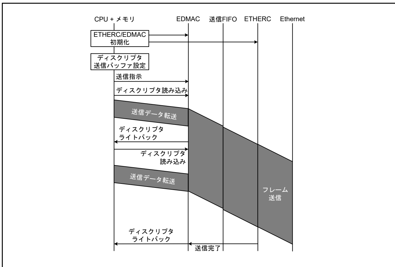
図 38.5 送信フローの例
