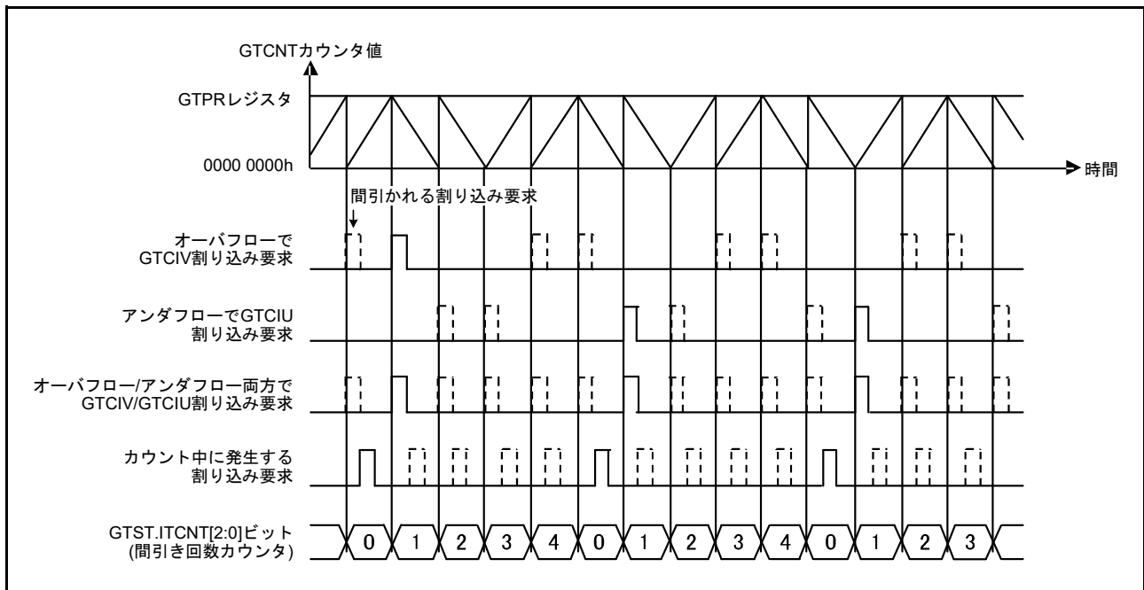
図 26.102 割り込み間引き機能の動作例 (のこぎり波でカウント方向を切替えながら動作、オーバーフロー / アンダフロー両方をカウントして間引き、間引き回数 4 の場合)
