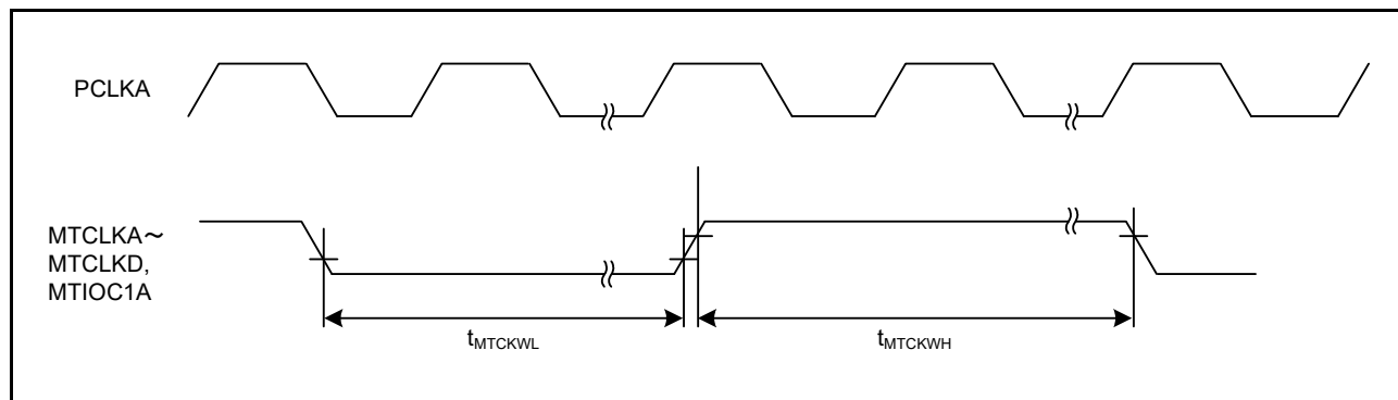
図 63.41 MTU クロック入力タイミング
