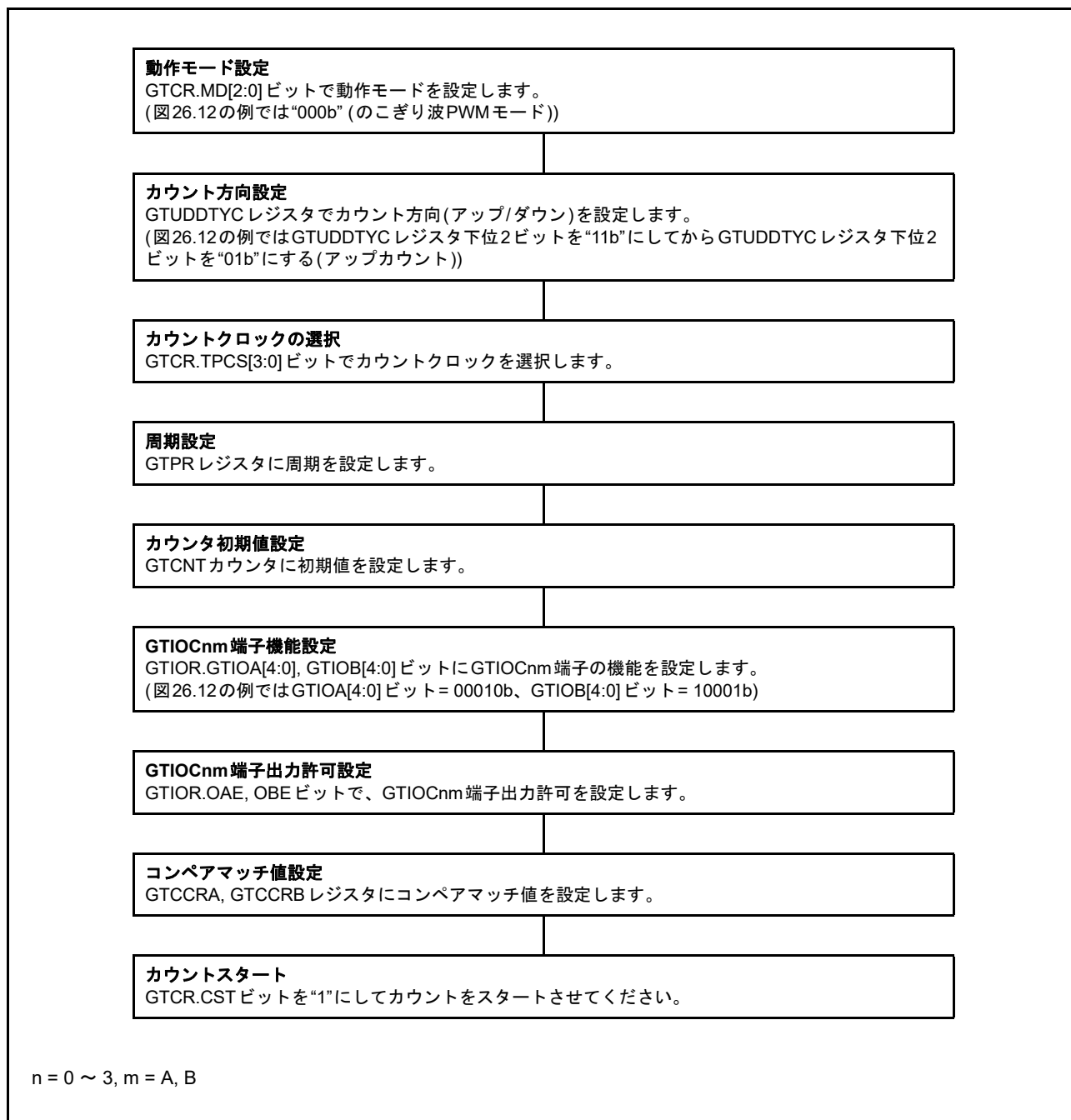
図 26.13 Low 出力 /High 出力動作設定例
