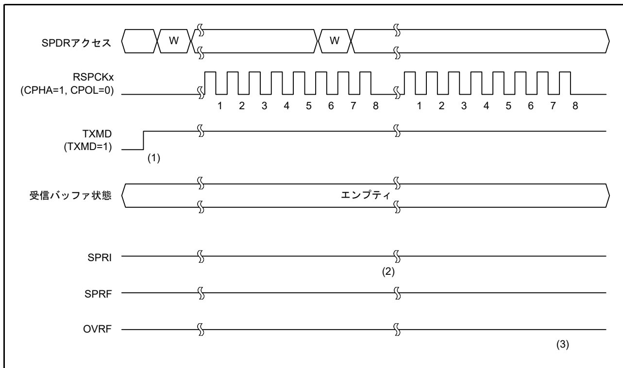
図 44.27 SPCR.TXMD = 1 の動作例
