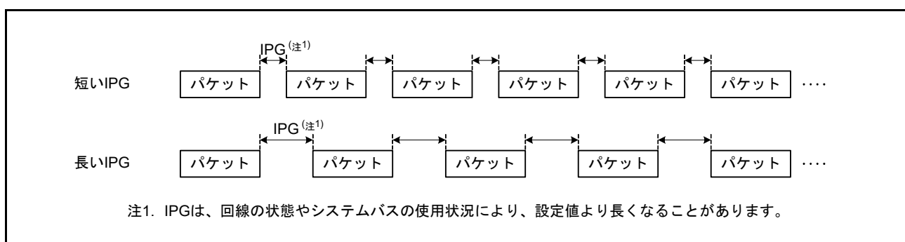
図 36.18 IPG の変更による伝送効率の違い
