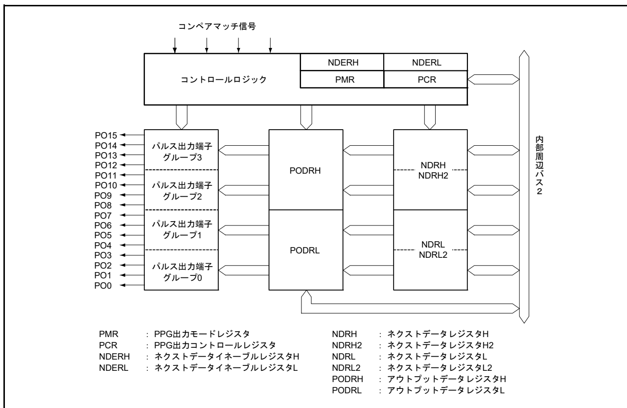
図 29.1 PPG0 のブロック図
