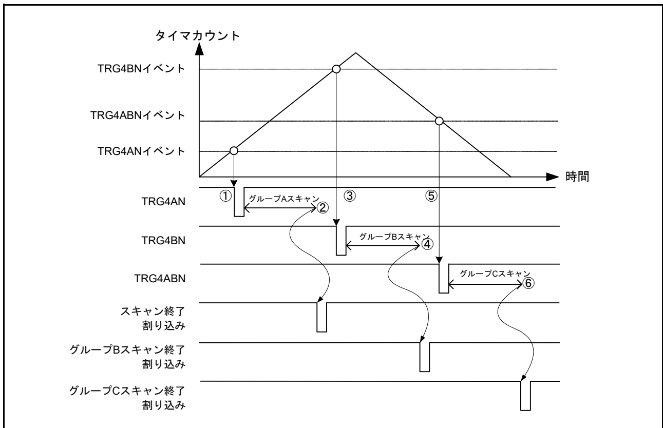
図 56.22 グループスキャンモードの動作例 (MTU からの同期トリガ発生による基本動作)
