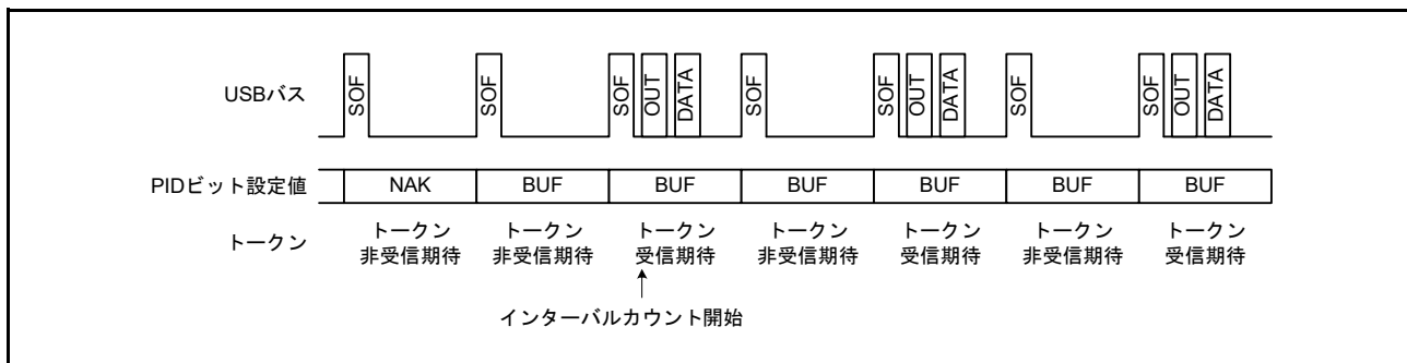
図 40.19 IITV[2:0] = 000b 以外の場合のフレームとトークン受信期待有無の関係
