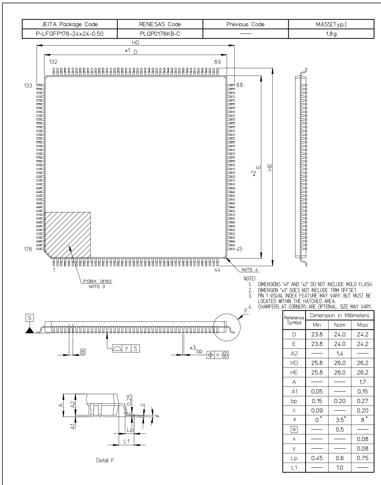
図 C. 176ピン LQFP (PLQP0176KB-C)
