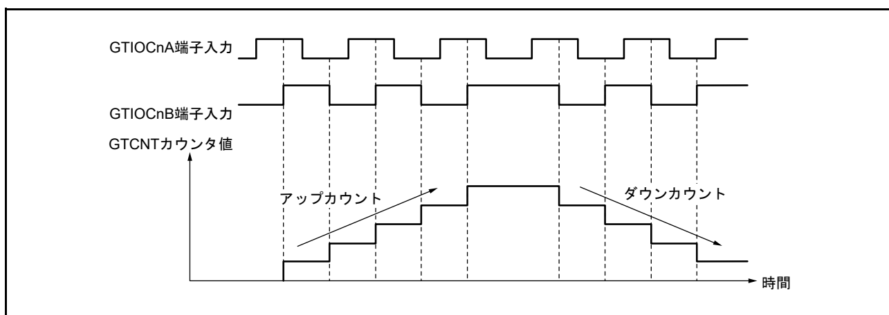
図 26.94 位相計数モード4の動作例 (n = 0 ~ 3)
