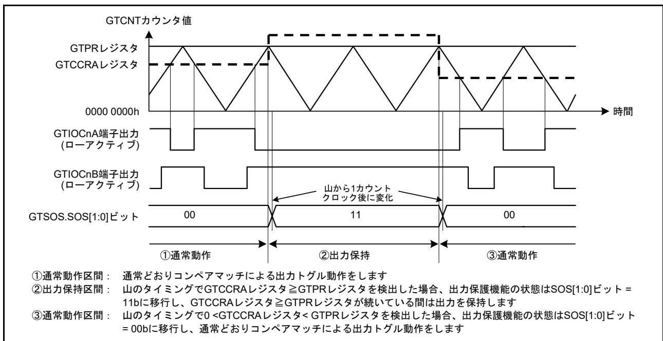
図 26.133 山のバッファ転送で GTCCRA レジスタ \geq GTPR レジスタが設定された場合の出力保護機能の動作例 (山のバッファ転送で 0 < GTCCRA レジスタ < GTPR レジスタに復帰、アクティブレベルは Low の場合) ( n = 0 \sim 3 )
