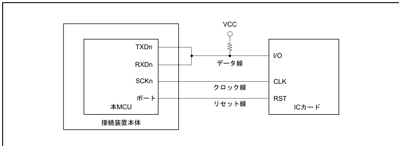
図 41.37 スマートカード (ICカード) との接続例
