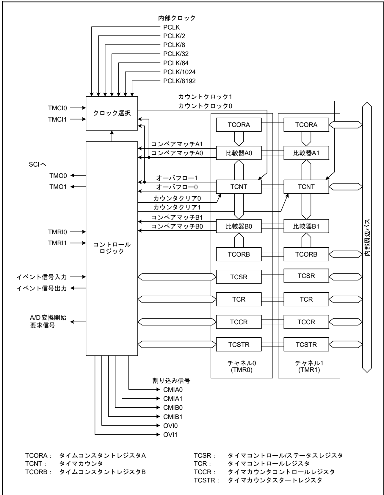
図 30.1 TMR (ユニット0) のブロック図
