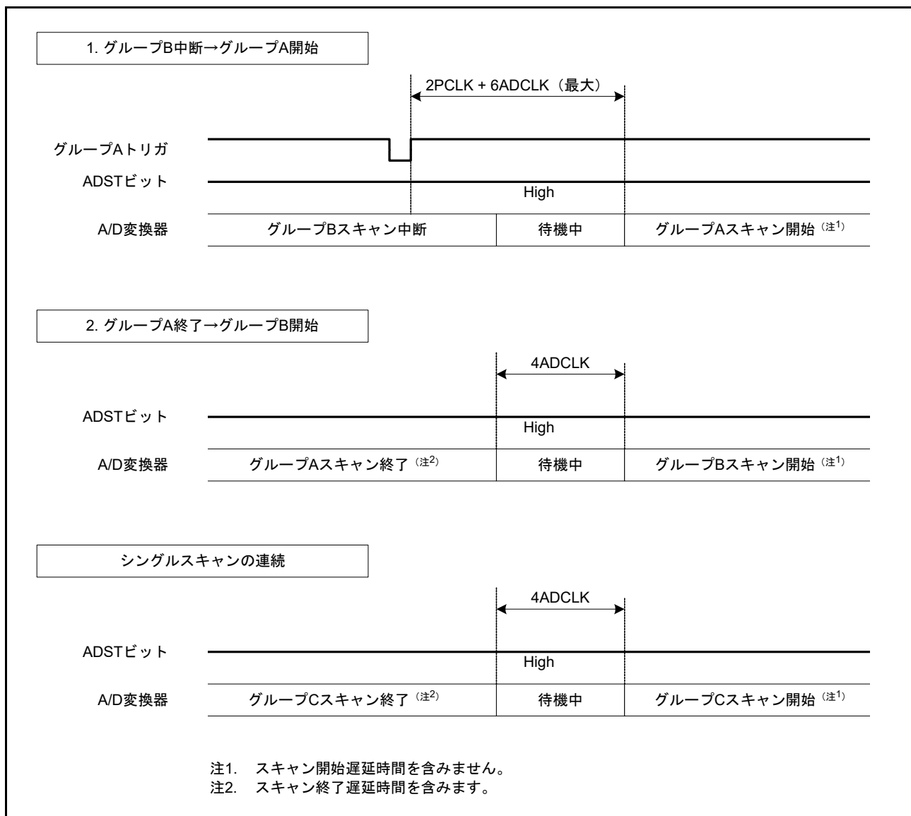
図 56.40 グループ優先でのスキャン停止 / 起動タイミング
