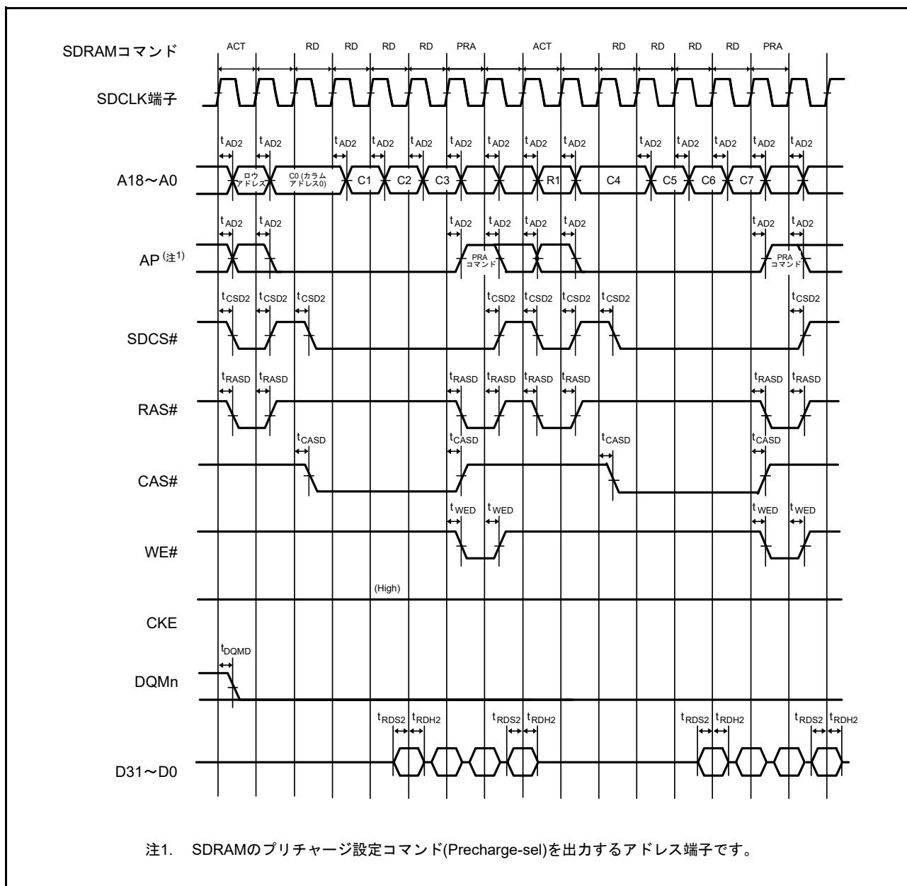
図 63.29 SDRAM 空間複数リード行またぎバスタイミング
