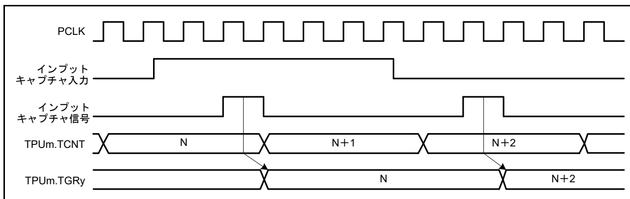
図 28.34 インพุットキャプチャ入力信号タイミング
