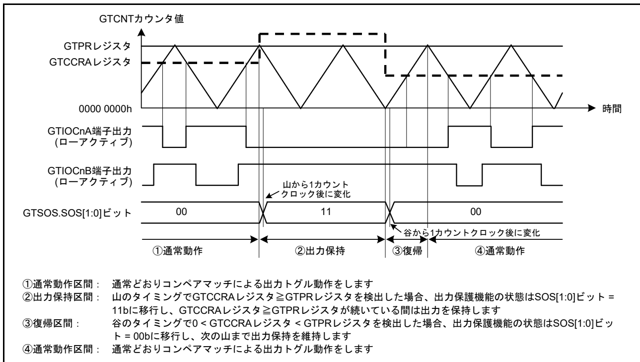
図 26.134 山のバッファ転送で GTCCRA レジスタ \geq GTPR レジスタが設定された場合の出力保護機能の動作例 (谷のバッファ転送で 0 < \text{GTCCRA レジスタ} < \text{GTPR レジスタ} に復帰、アクティブレベルは Low の場合) ( n = 0 \sim 3 )
