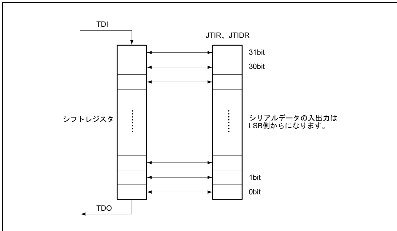
図 53.3 シリアルデータ入出力
