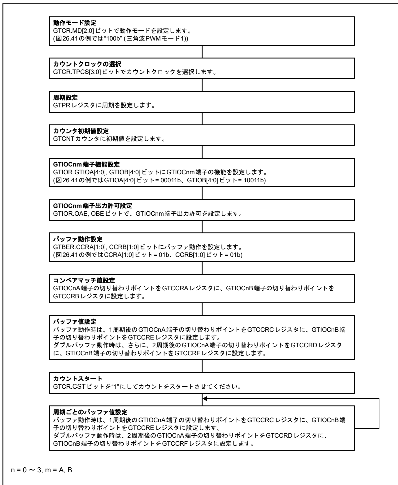
図 26.42 三角波 PWM モード 1 設定例
