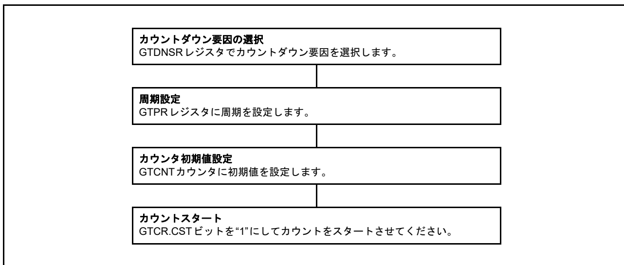
図 26.11 イベントカウント動作設定例 (ハードウェア要因によるダウンカウント時)
