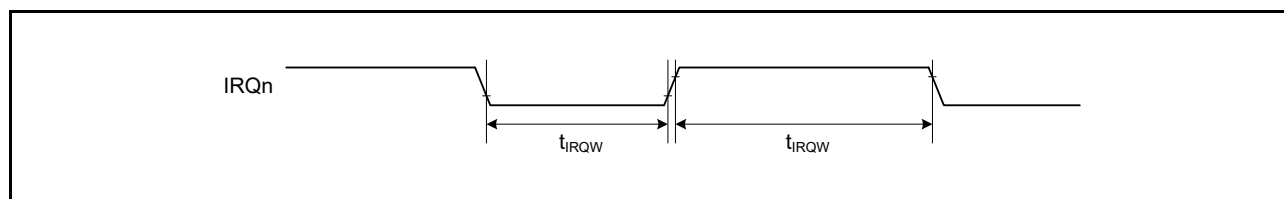
図 63.17 IRQ 割り込み入カタイミング
