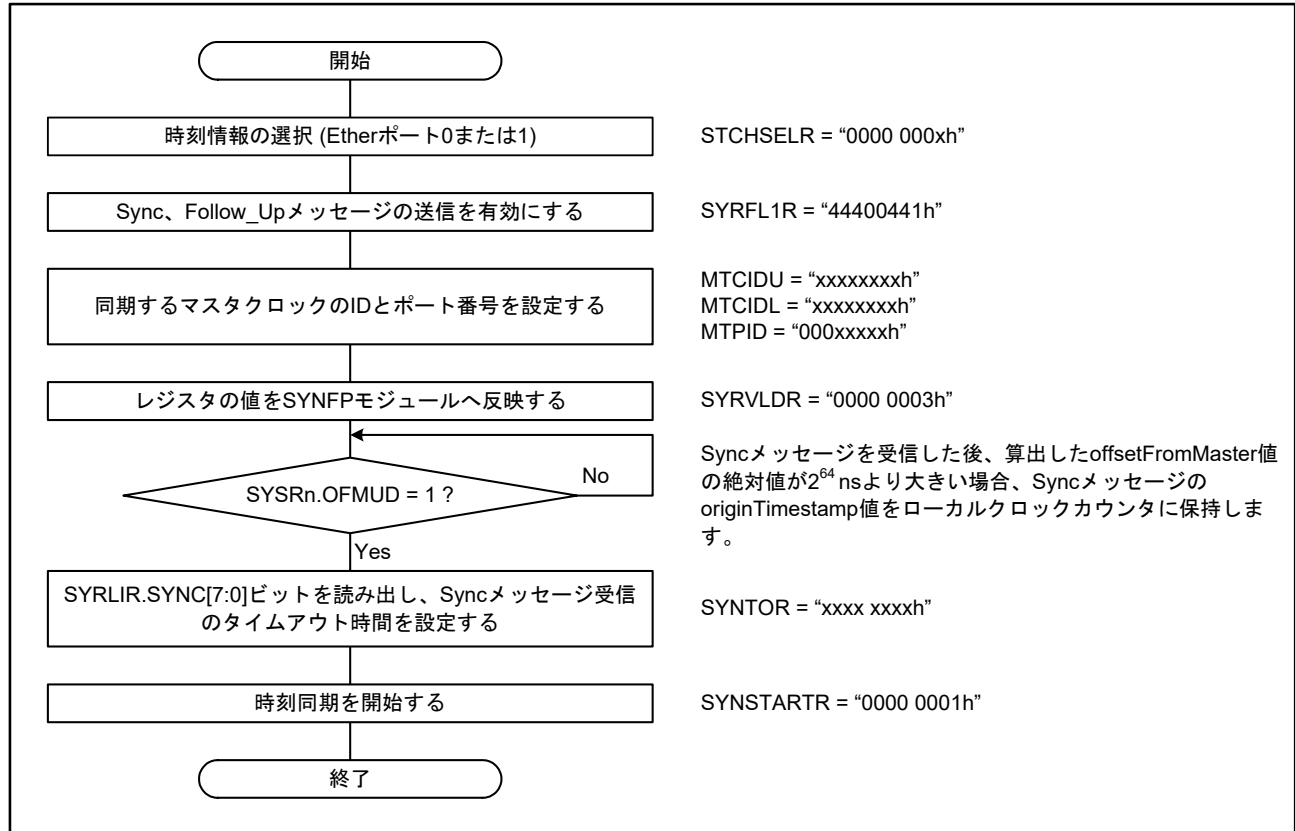
図37.20 P2Pスレーブ動作の開始手順
