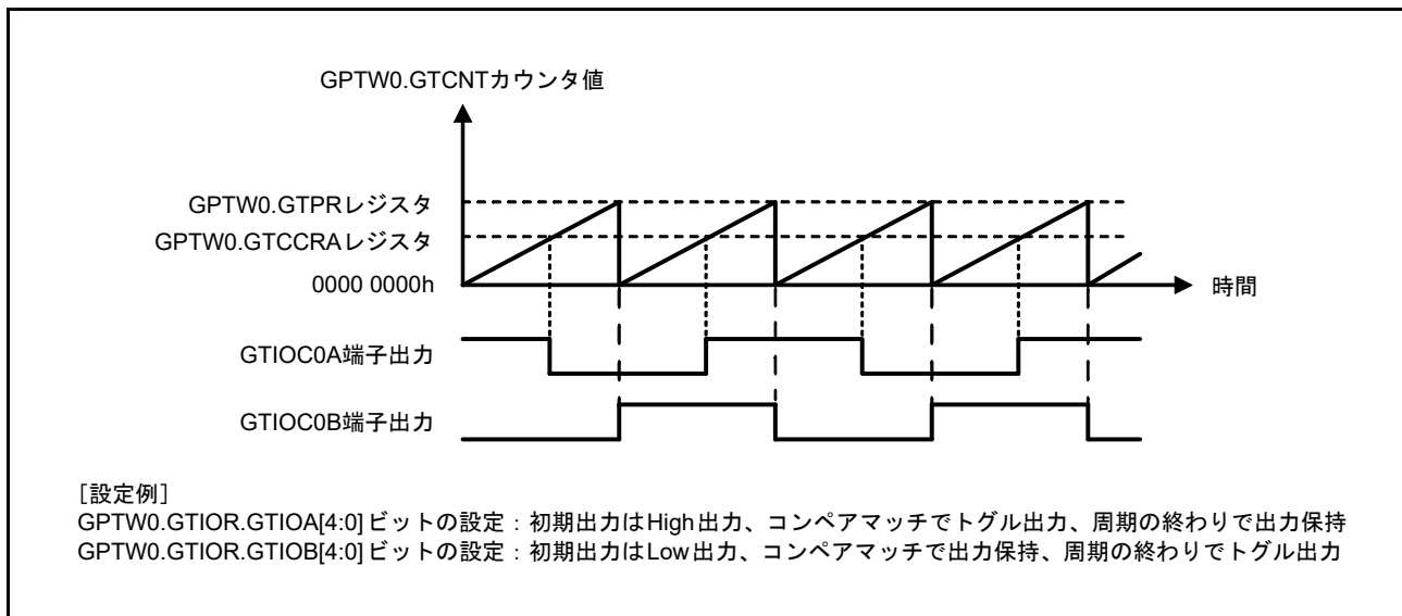
図 26.15 トグル出力動作例 (2)
