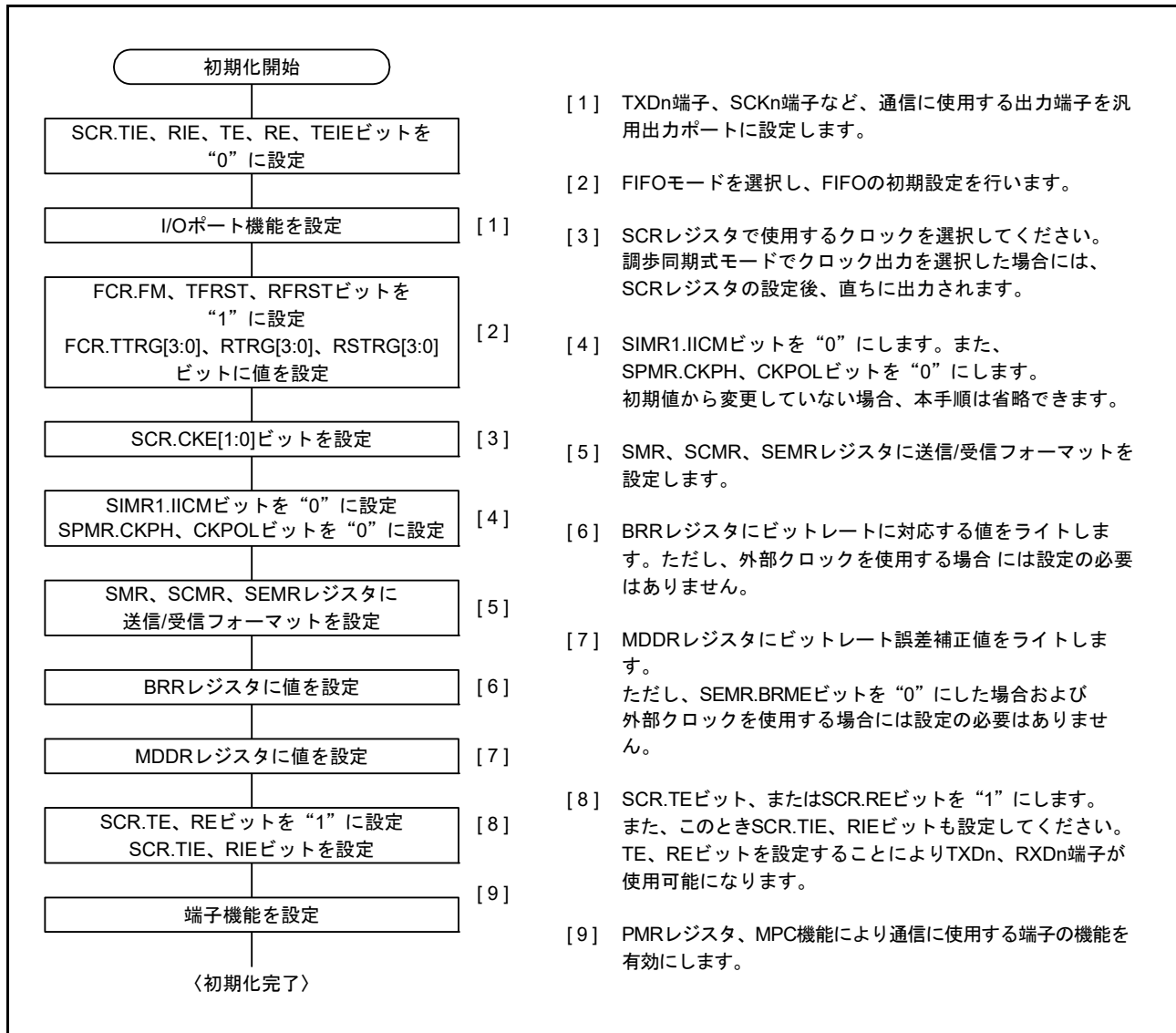
図 41.12 SCI の初期化フローチャートの例 ( 調歩同期式モード、FIFO 使用 ) (SCI7 ~ SCI11)
