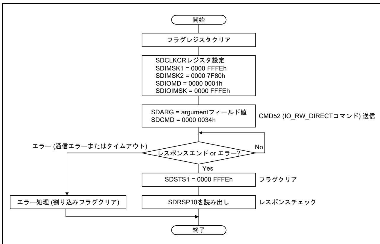
図 48.14 IO_RW_DIRECT コマンドの送信例
