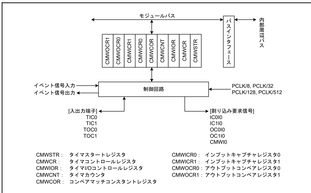
図 32.1 CMTW0 のブロック図
