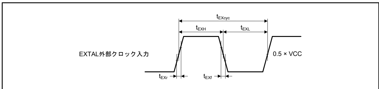
図 63.4 EXTAL 外部クロック入力タイミング
