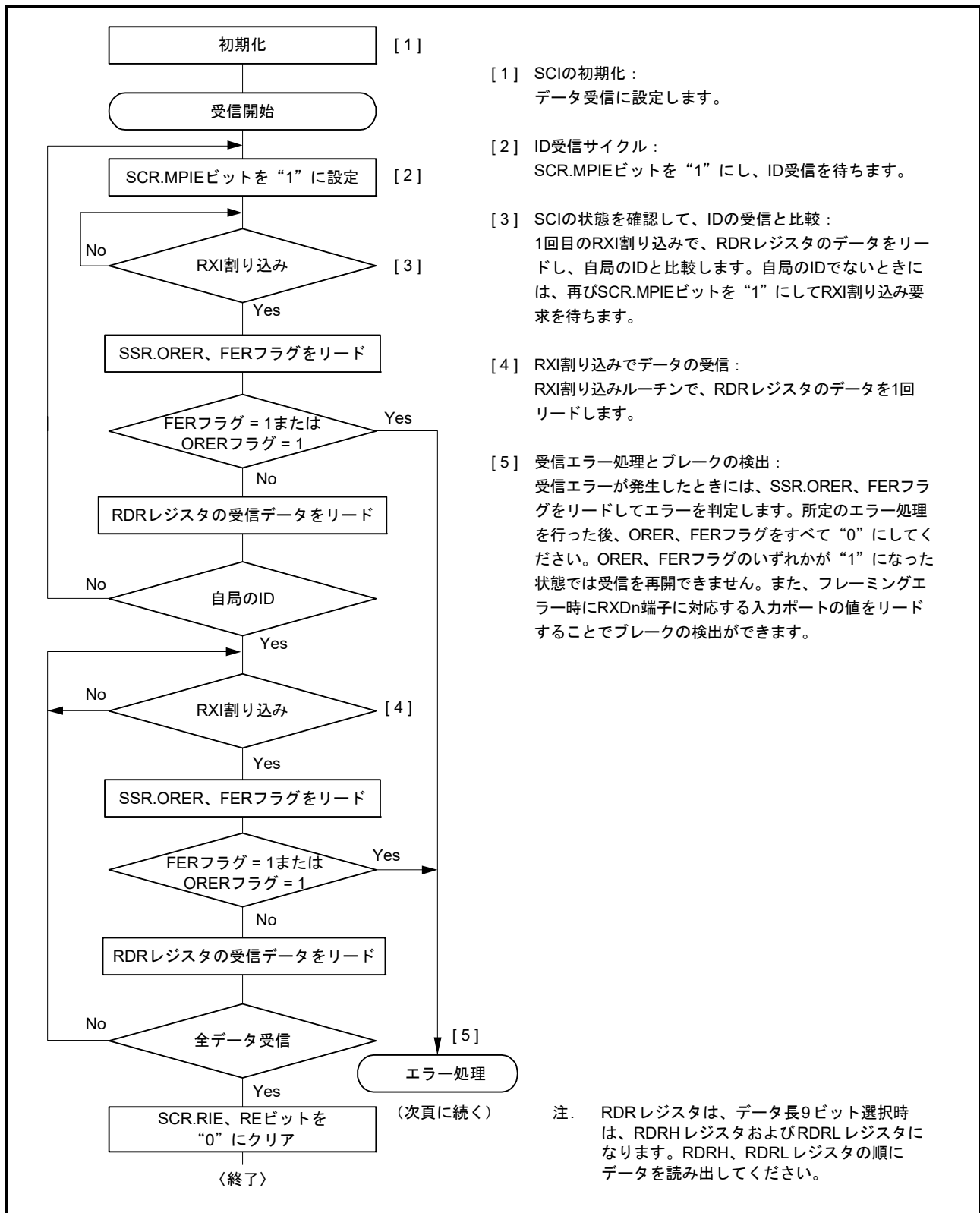
図 41.25 マルチプロセッサシリアル受信のフローチャートの例 (1)
