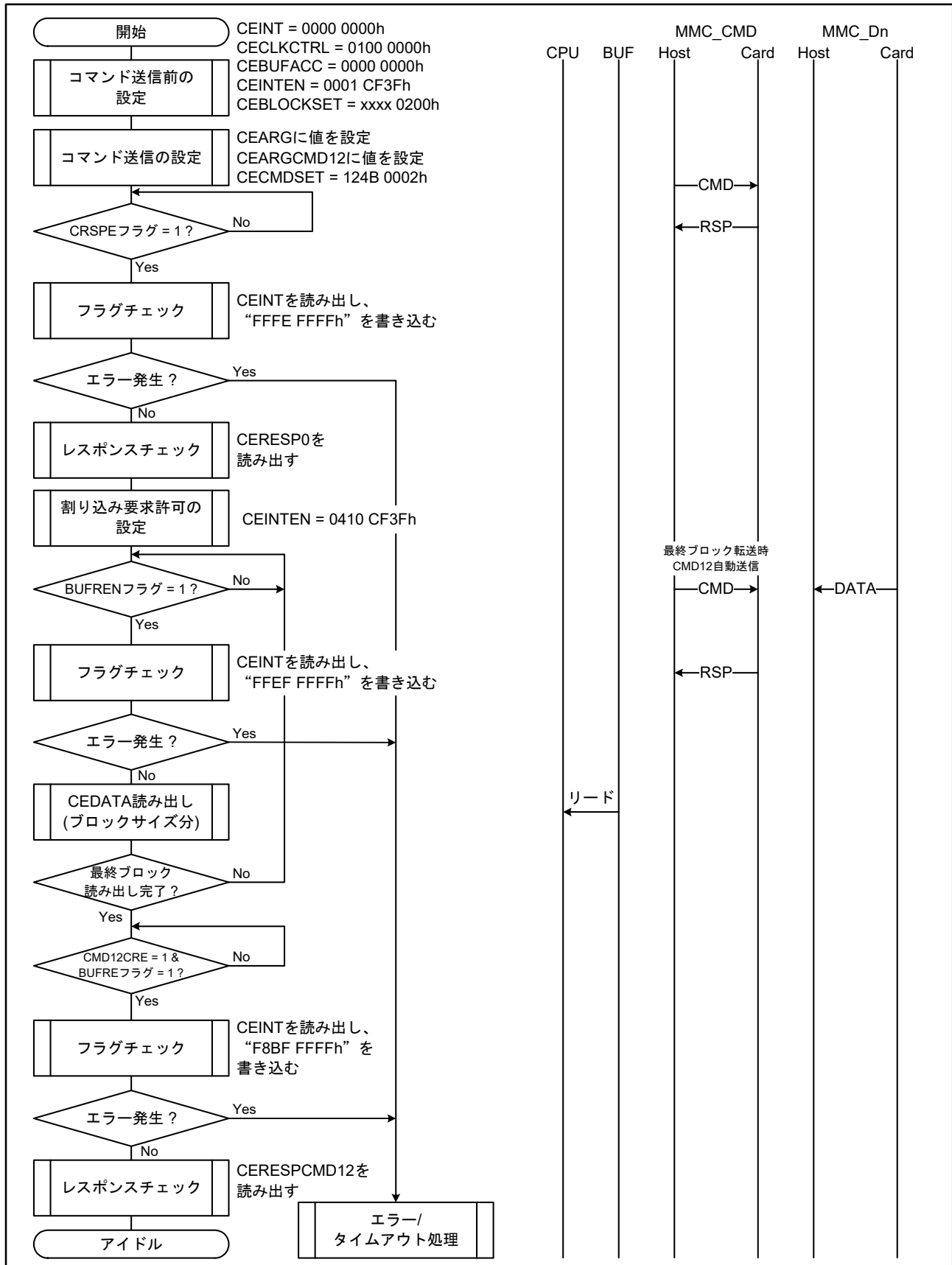
図 49.17 マルチブロックリードコマンドの送信例 (CMD18 Open-ended)
