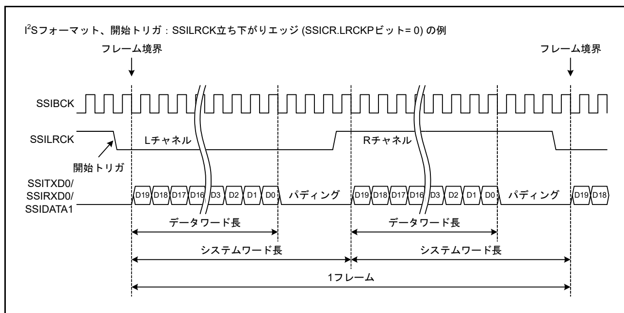
図 47.1 データフォーマットに関する用語の定義
