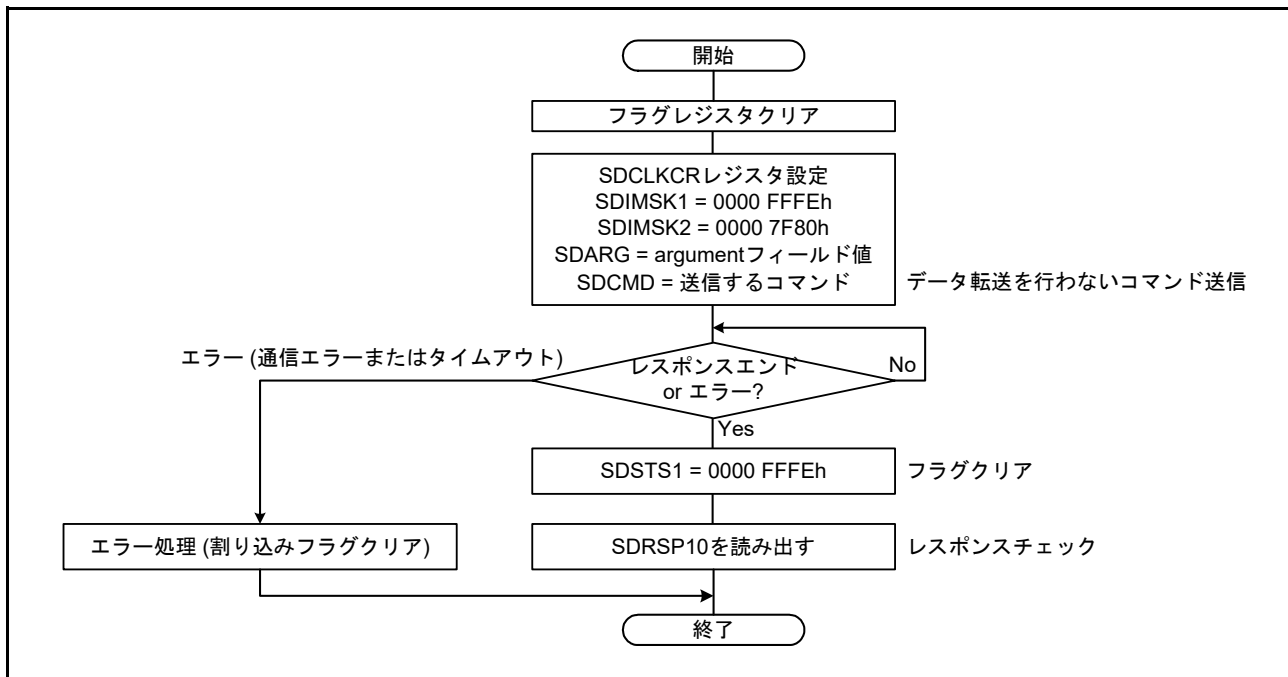
図 48.9 データ転送を行わないコマンドの送信例
