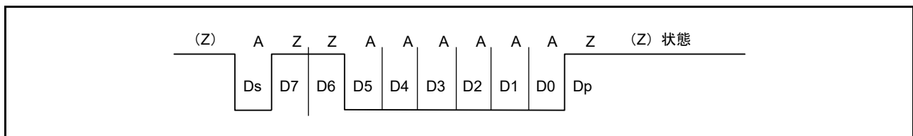
図 41.40 インバースコンベンション (SCMR.SDIR ビット = 1、SCMR.SINV ビット = 1、SMR.PM ビット = 1)
