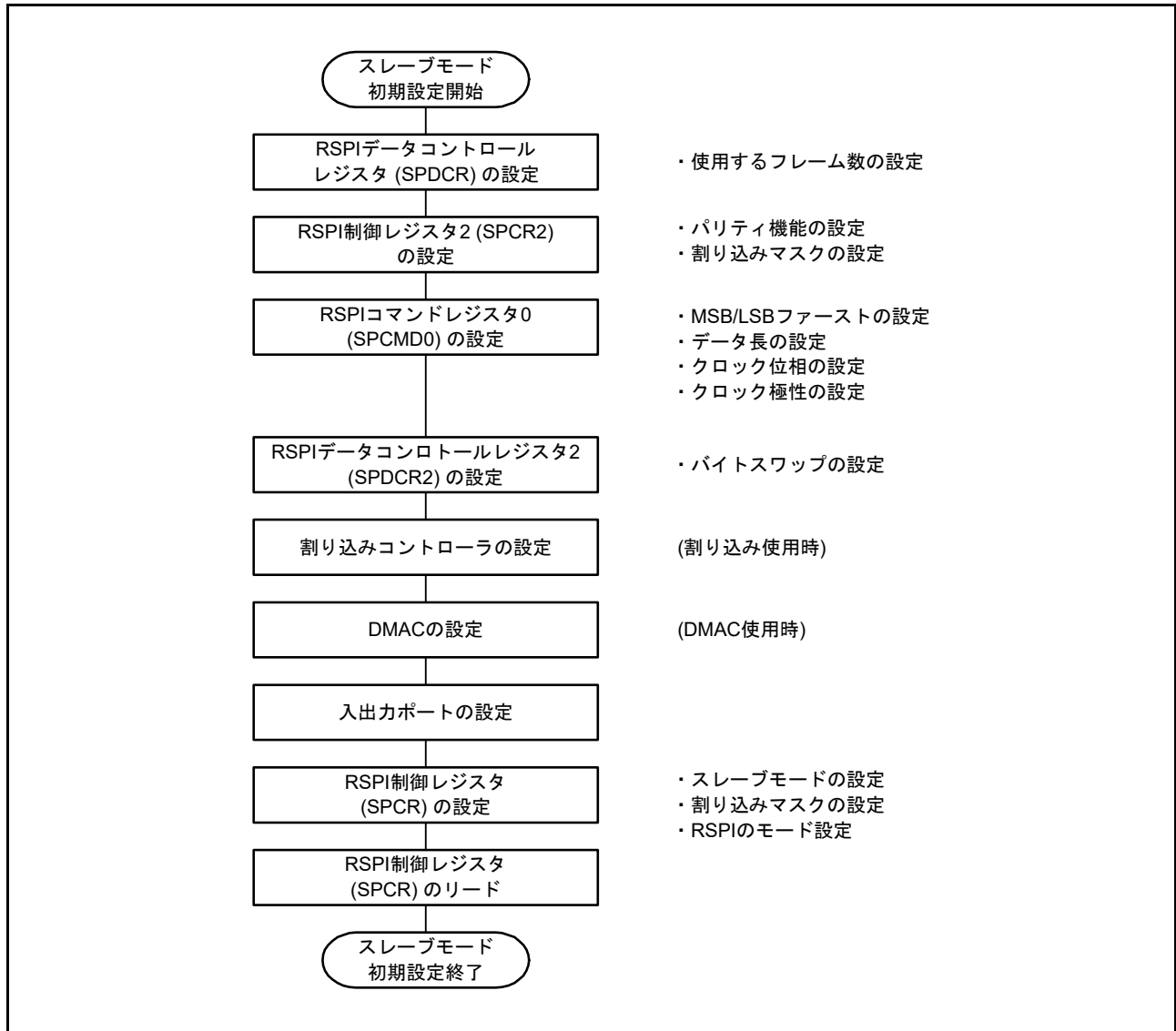
図 44.49 スレーブモード時の初期化フロー例 (クロック同期式動作)
