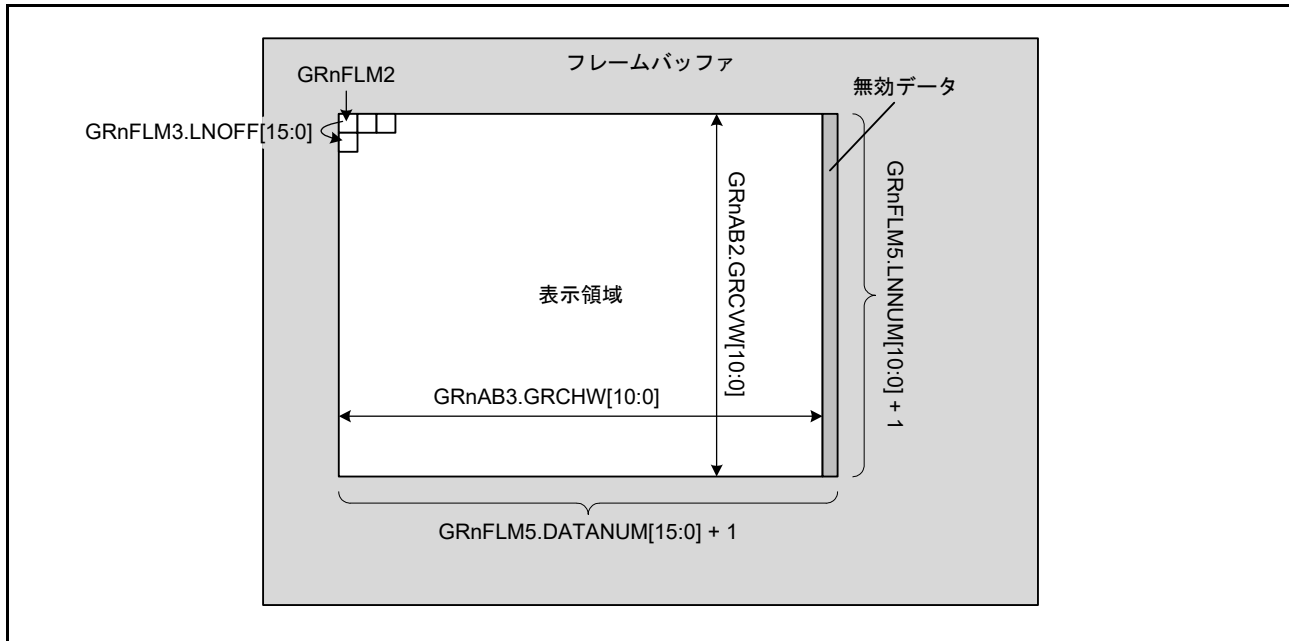
図 51.4 マクロラインを使用しない場合のフレームバッファ設定例
