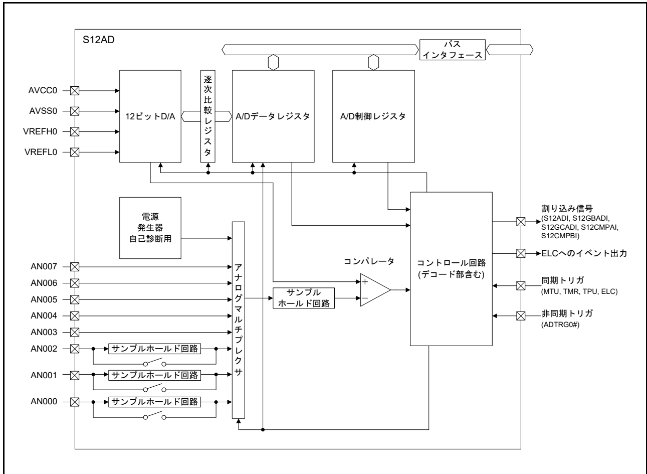
図 56.1 12ビットA/Dコンバータのブロック図 (ユニット0)
