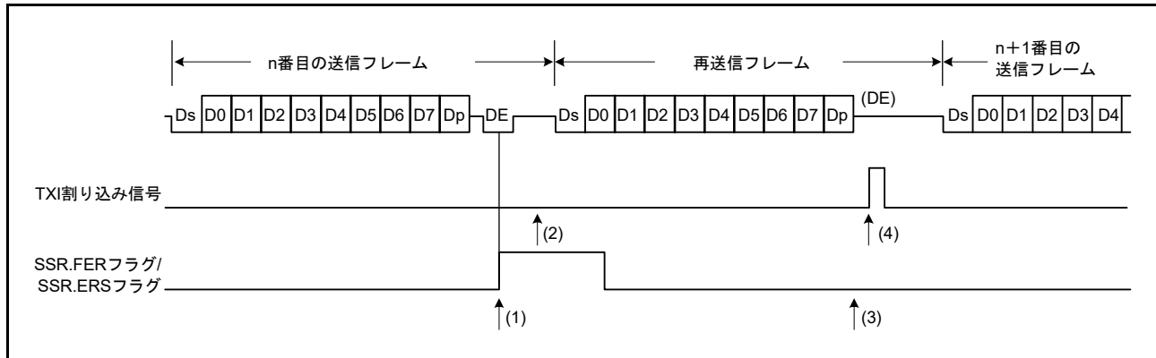
図 41.44 SCI 送信モードの場合の再送信動作 (送信時の再送信動作)
