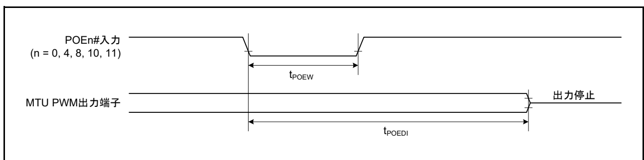
図 63.43 POE 出力ディセーブル時間 (POEn# 端子の変化)
