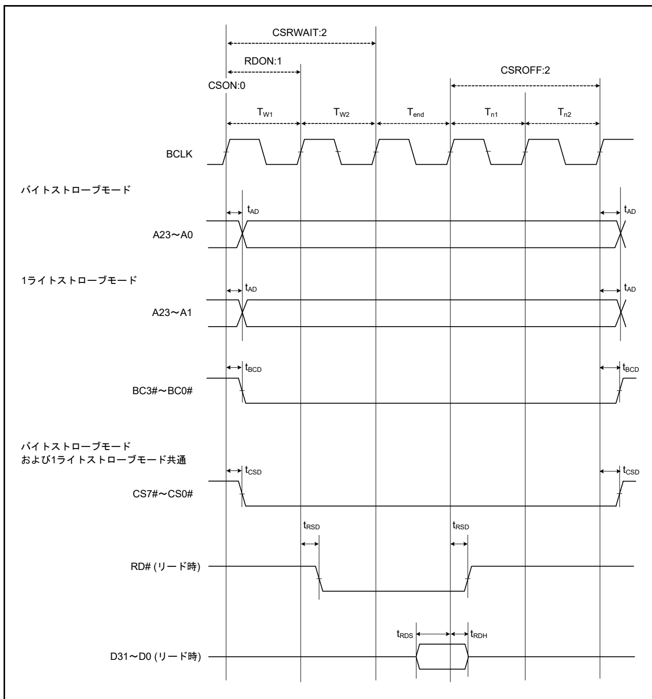
図 63.20 外部バスタイミング / ノーマルリードサイクル (バスクロック同期)
