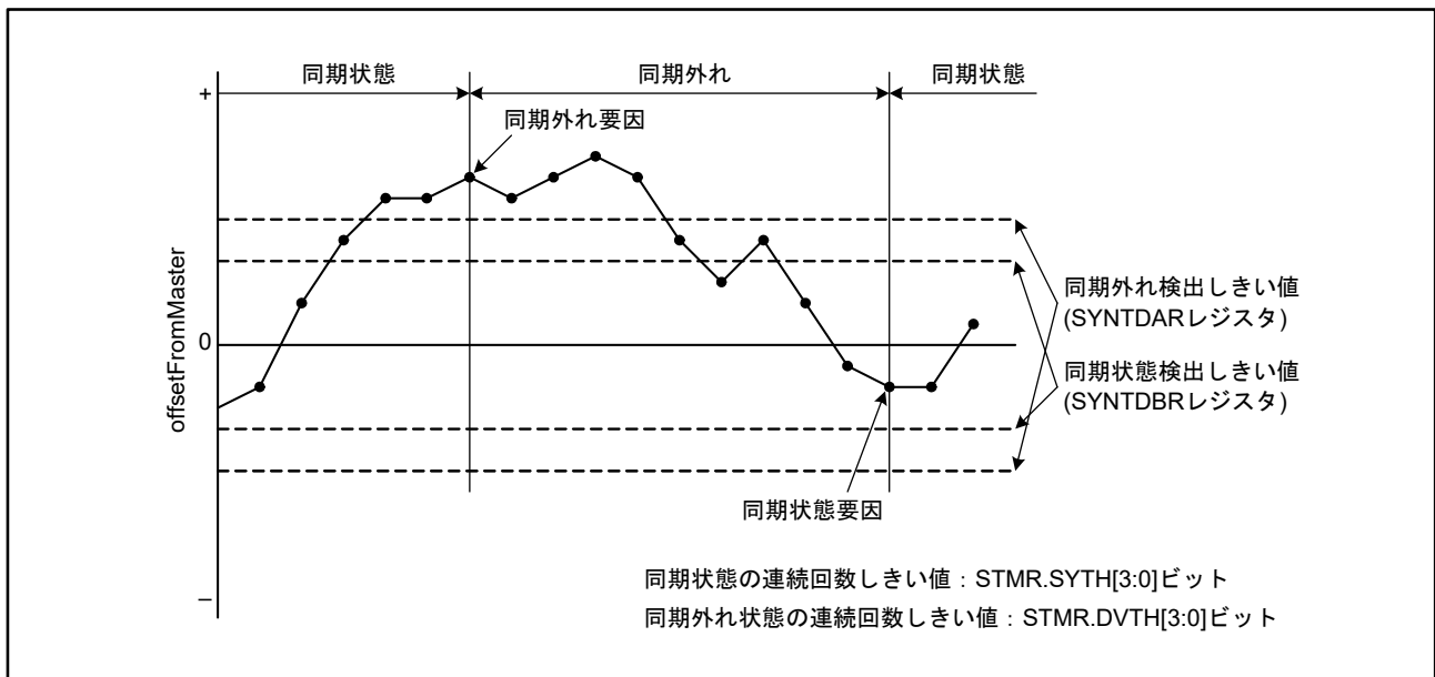
図 37.26 同期外れおよび同期状態の発生例 (STMR.DVTH[3:0] ビットおよびSYTH[3:0] ビットで連続検出回数を3回に指定)
