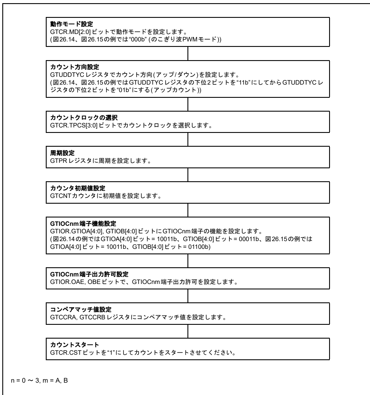
図 26.16 トグル出力動作設定例
