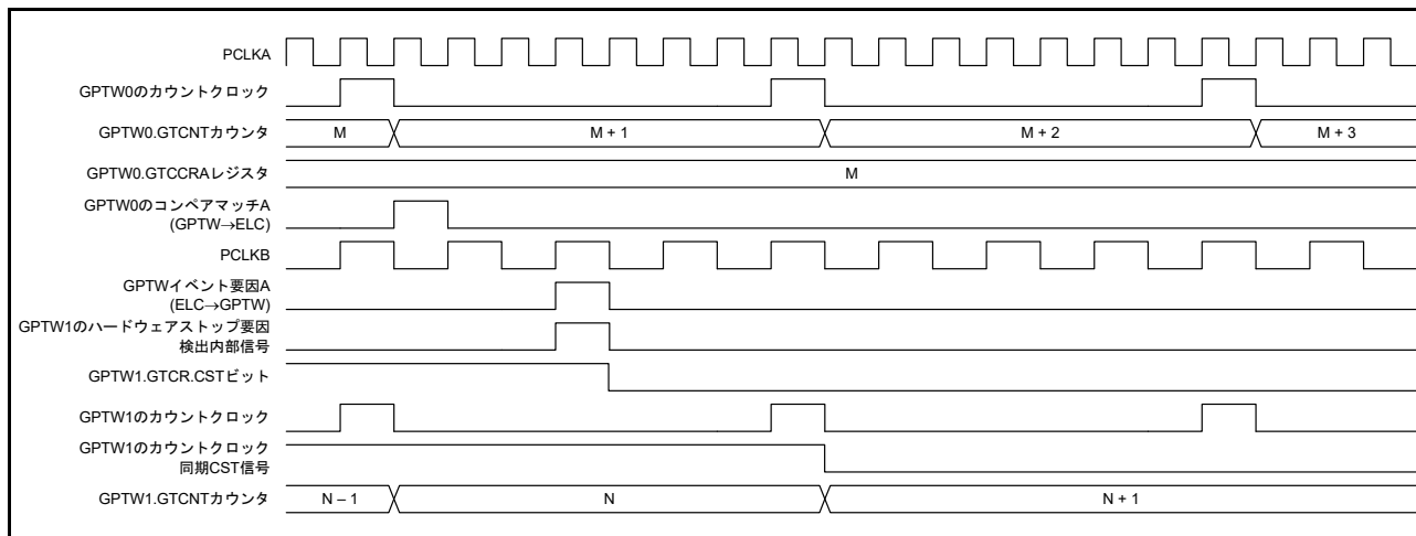
図 26.66 ELCA イベント入力によるカウントストップ動作タイミング例
