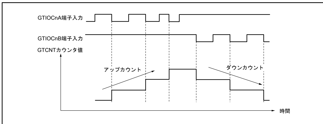
図 26.91 位相計数モード3の動作例 (n = 0 ~ 3)
