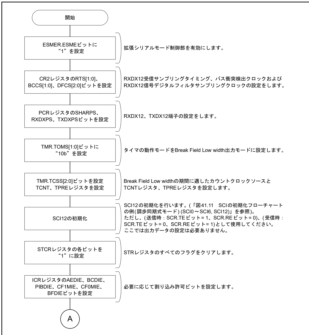
図 41.66 Start Frame 送信フローチャート例 (1)
