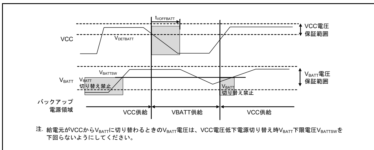
図 63.107 バッテリバックアップ機能特性
