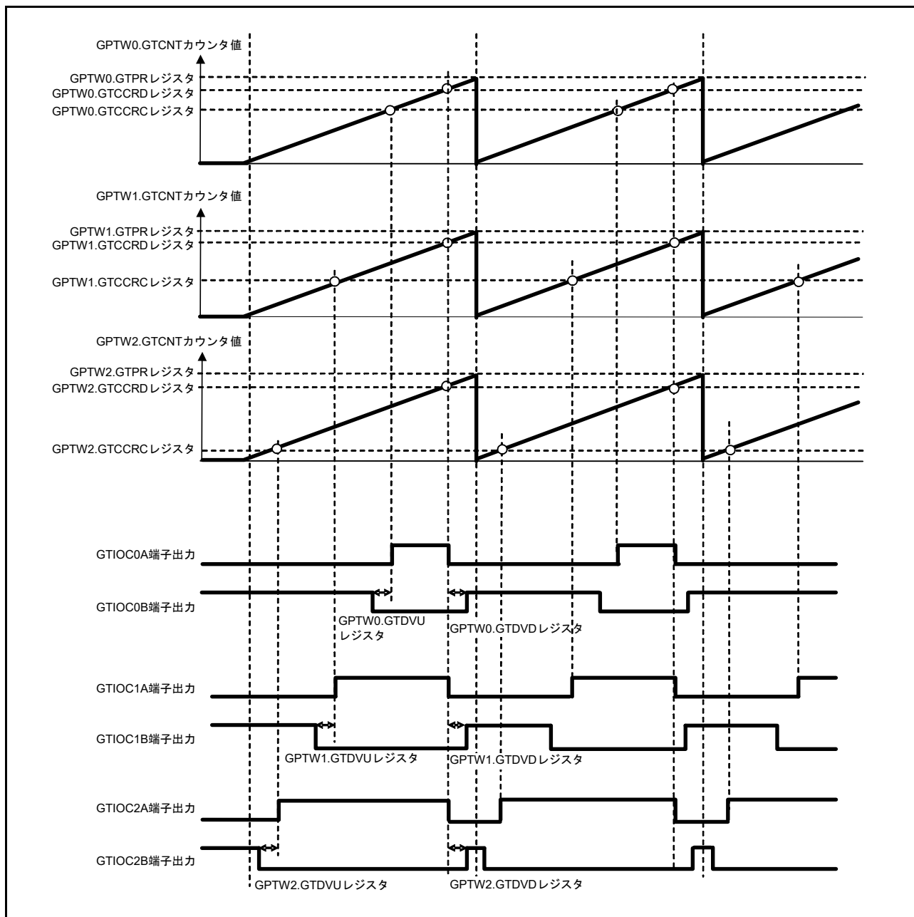
図 26.83 のこぎり波 3 相相補 PWM 出力例 (デッドタイム自動設定)
