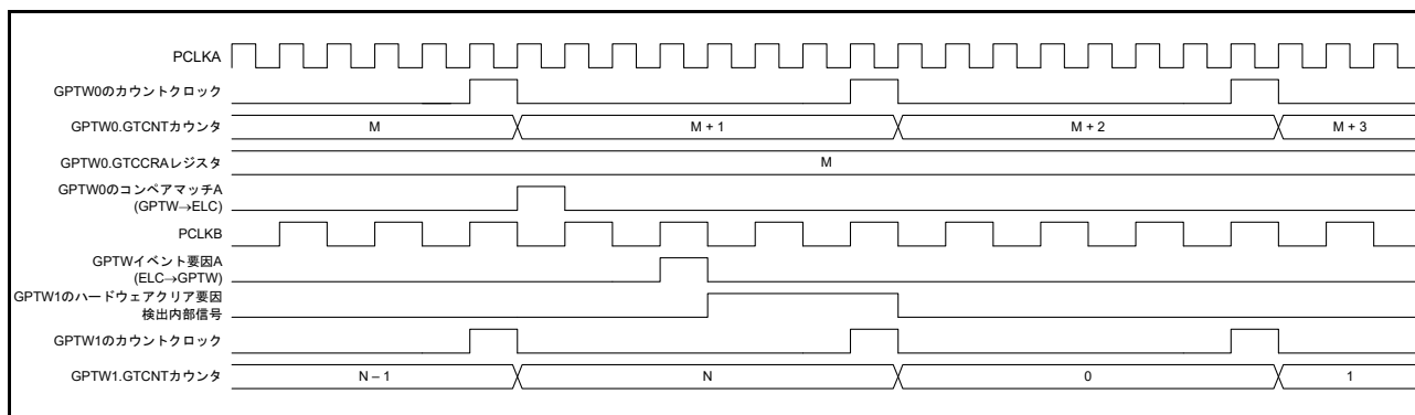
図 26.73 ELCA イベント入力によるカウンタクリア動作タイミング例 (PCLKA の分周クロックによるカウンタ動作時)
