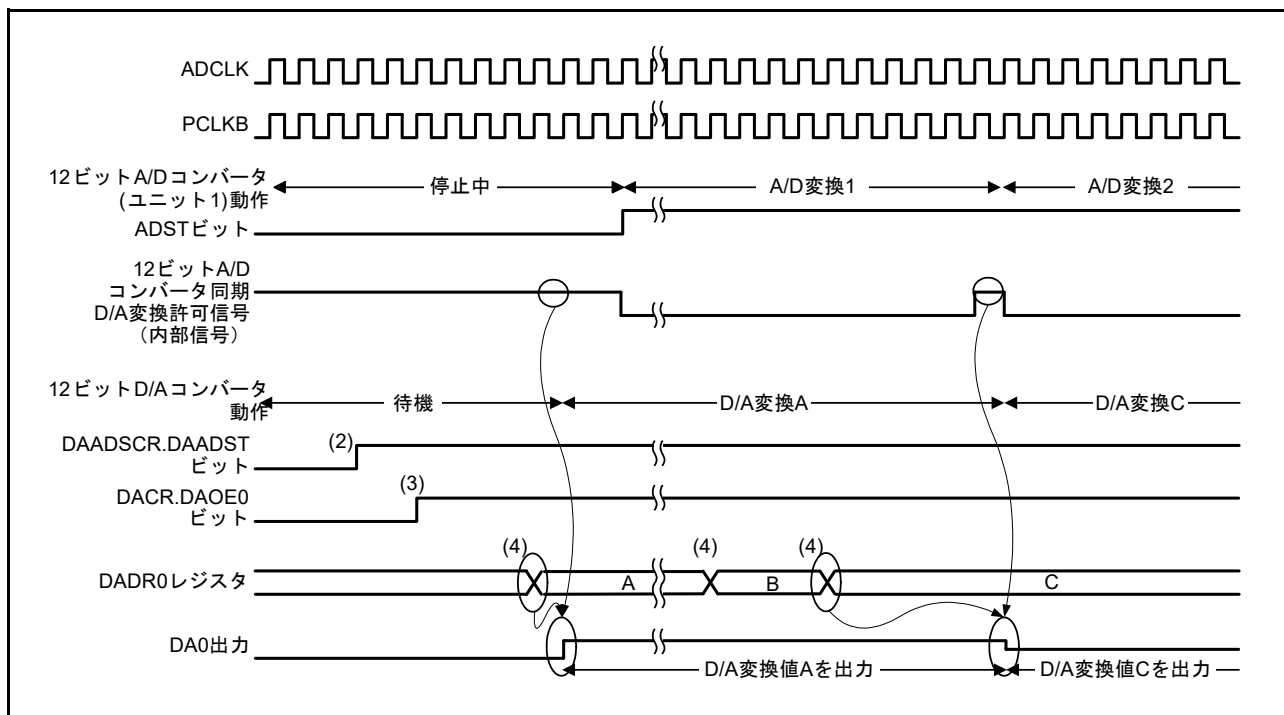
図 57.3 12ビットD/Aコンバータを12ビットA/Dコンバータ(ユニット1)に同期して変換する例
