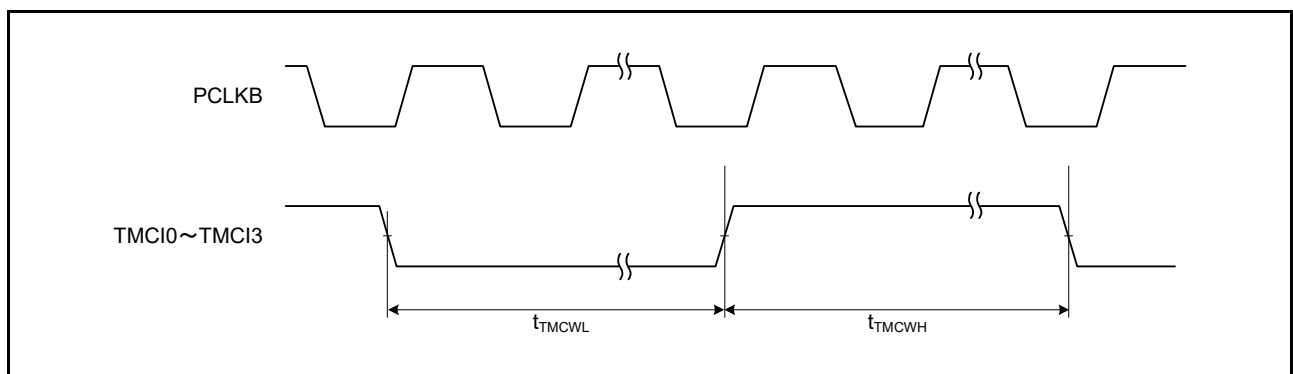
図 63.38 TMR クロック入力タイミング
