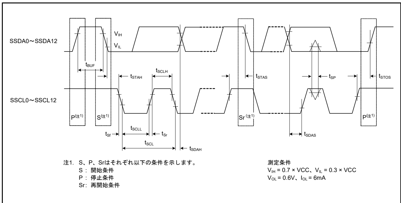
図 63.56 簡易 IIC バスインタフェース入出力タイミング
