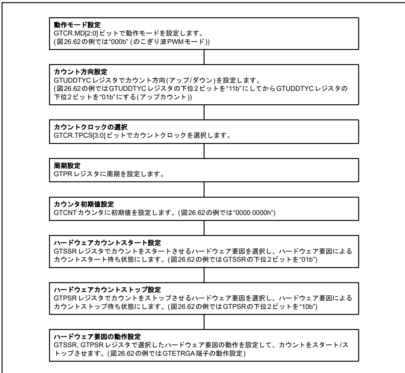
図 26.63 ハードウェア要因によるカウントスタート/ストップ動作設定例
