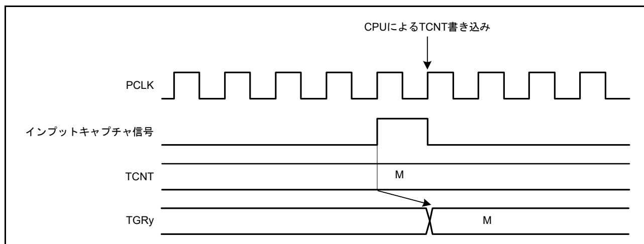
図 28.49 TPUm.TGRy レジスタへの書き込みとインプットキャプチャの競合
