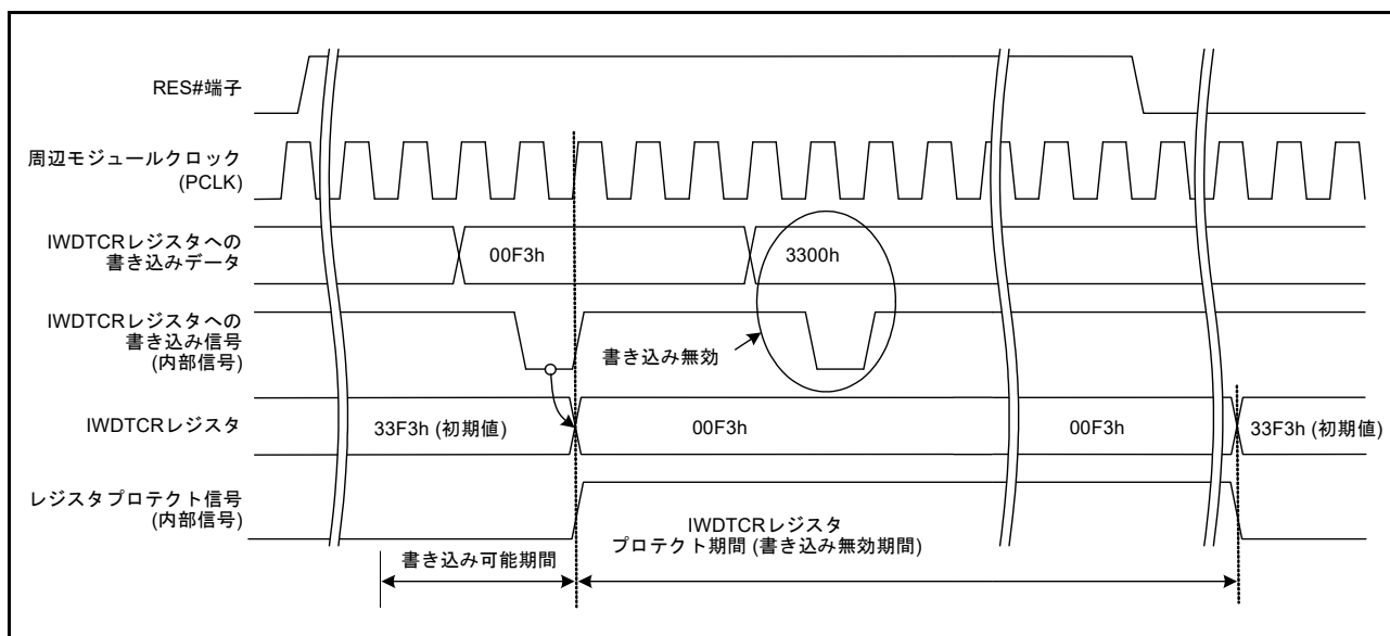
図 35.5 IWDTCR レジスタ書き込み制御波形
