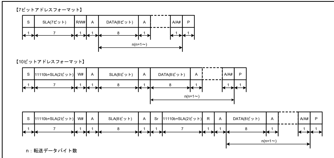
図 42.2 I 2 C バスフォーマット
