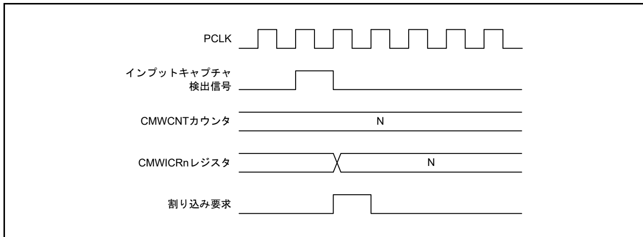
図 32.15 インพุットキャプチャ割り込みの発生タイミング (n = 0, 1)
