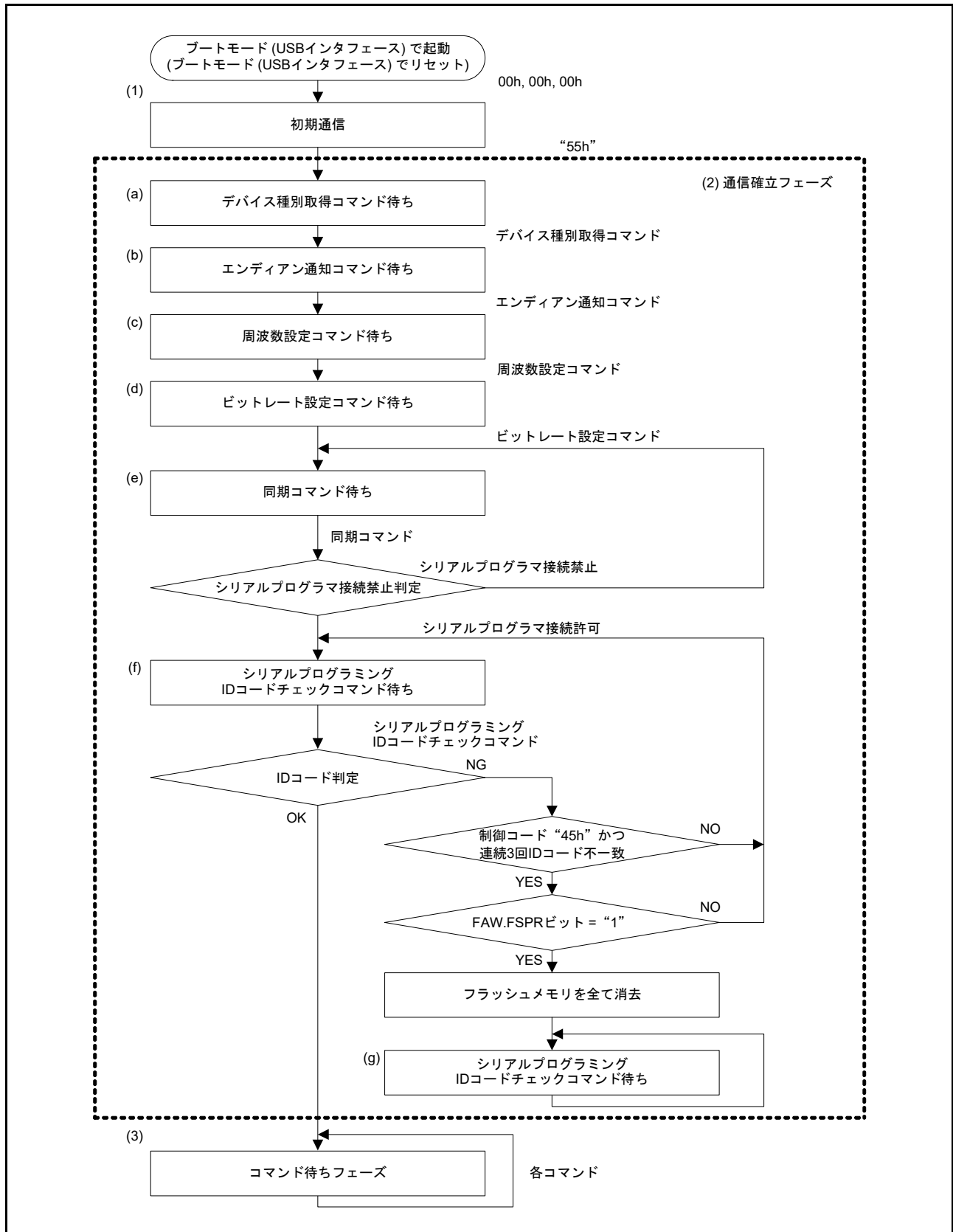
図 62.39 ブートモード (USB インタフェース) の状態遷移フロー
