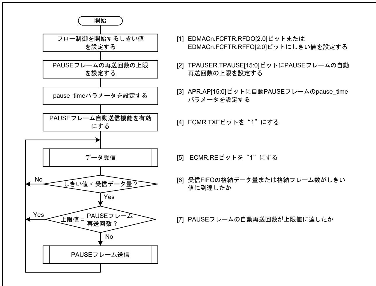
図 36.19 PAUSE フレーム自動送信の設定手順例
