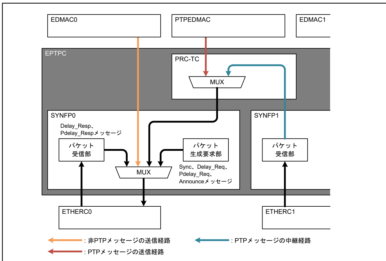
図37.34 送信メッセージのアービトレーション
