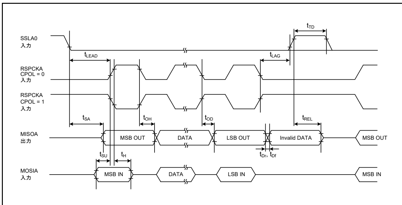
図 63.68 RSPI タイミング ( スレーブ、CPHA = 0)
