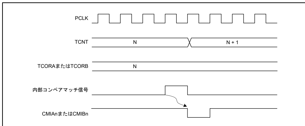
図 30.7 コンペアマッチ時の割り込みタイミング (n = 0 ~ 3)
