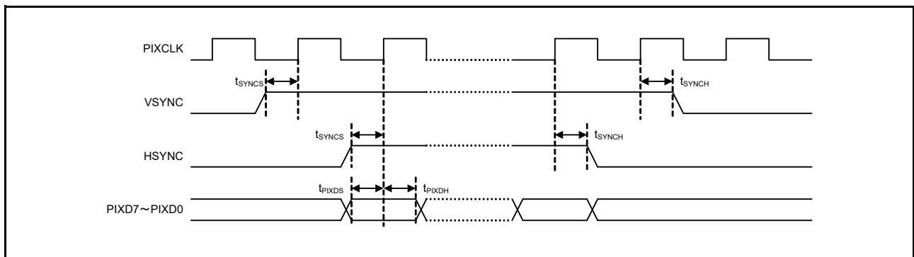
図 63.93 PDC AC タイミング
