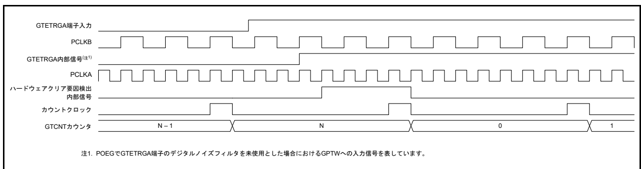
図 26.71 GTETRGA 端子入力の立ち上がりによるカウンタクリア動作タイミング例 (PCLKA の分周クロックによるカウント動作時)
