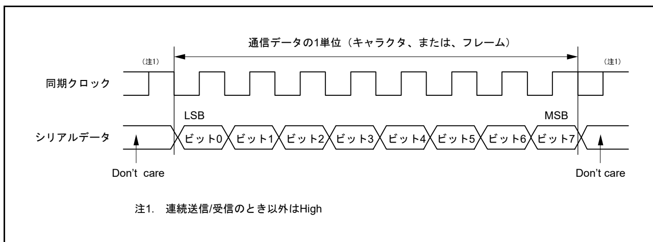
図 41.27 クロック同期式シリアル通信のデータフォーマット (LSB ファーストの場合)
