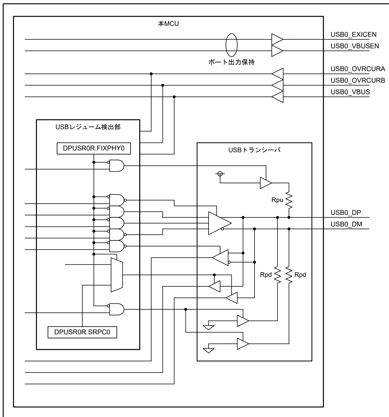
図 40.6 USB レジューム検出部と USB0 用入出力端子の接続概略図
