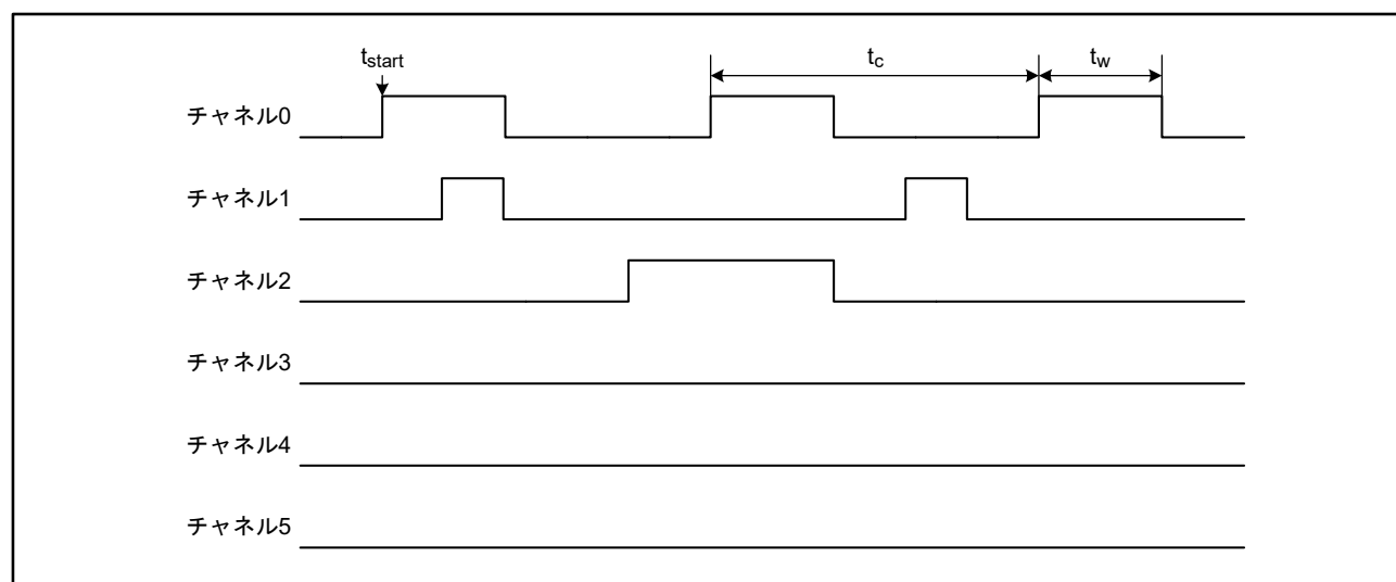
図37.32 パルス出力タイマの動作タイミング
