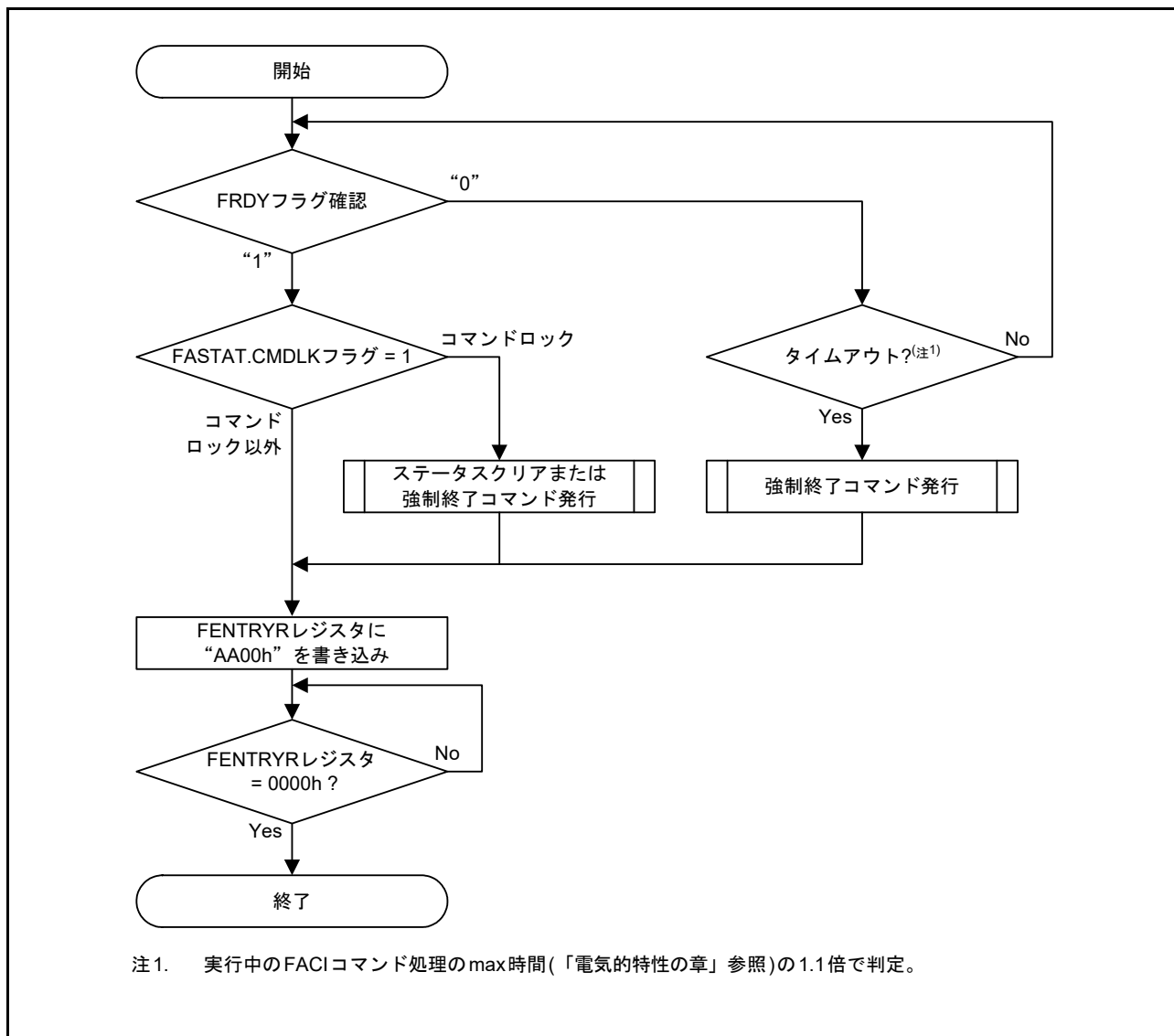
図 62.11 リードモード移行フロー
