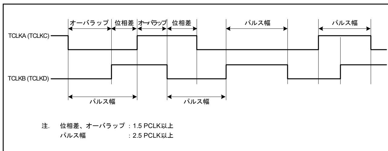
図 28.43 位相計数モード時の位相差、オーバーラップ、およびパルス幅
