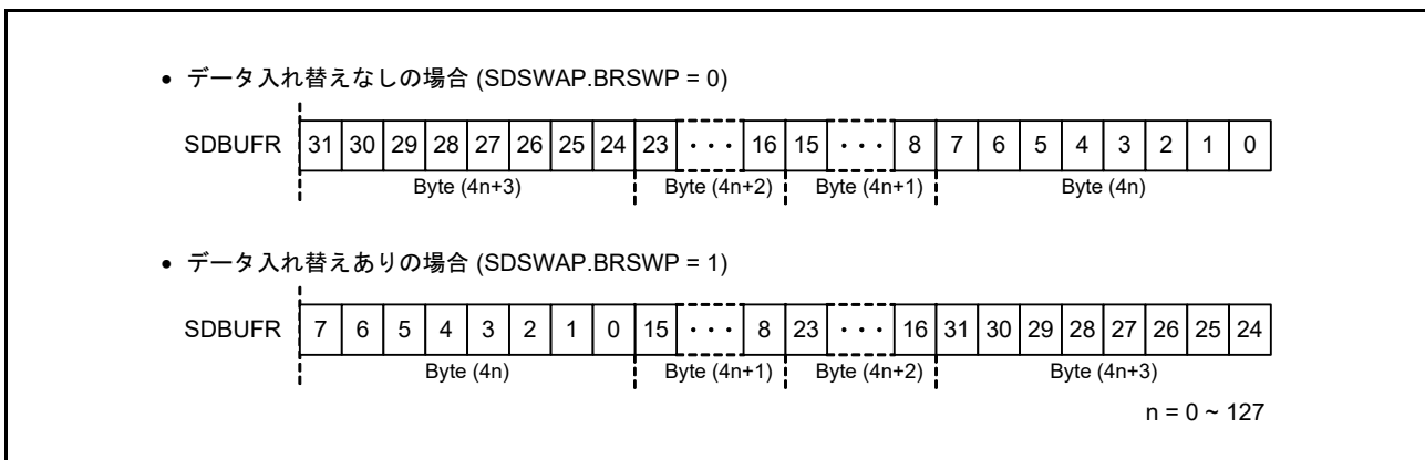
図 48.5 SDBUFRレジスタ読み出し時のデータ配置
