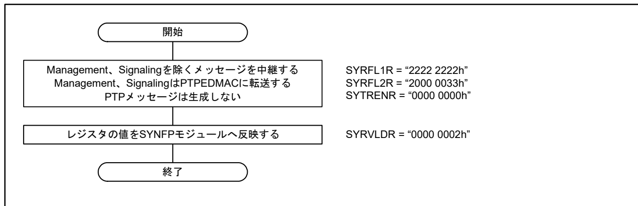
図37.22 E2E TC動作の開始手順
