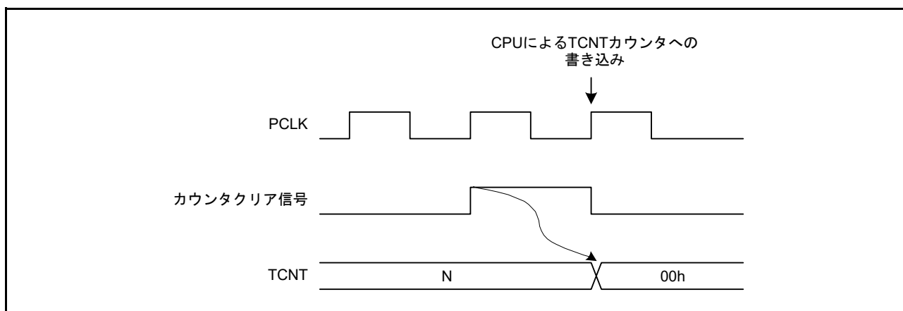
図 30.13 TCNTカウンタへの書き込みとカウンタクリアの競合
