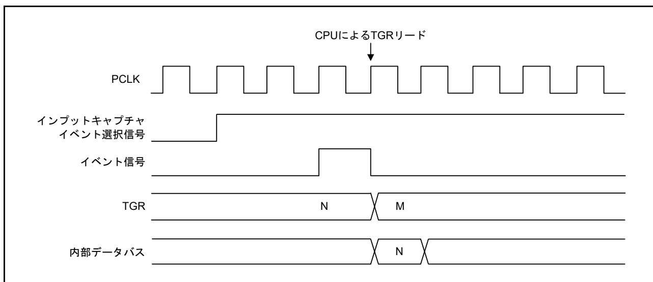
図 28.61 TGR へのリードサイクルとインพุットキャプチャ動作の競合
