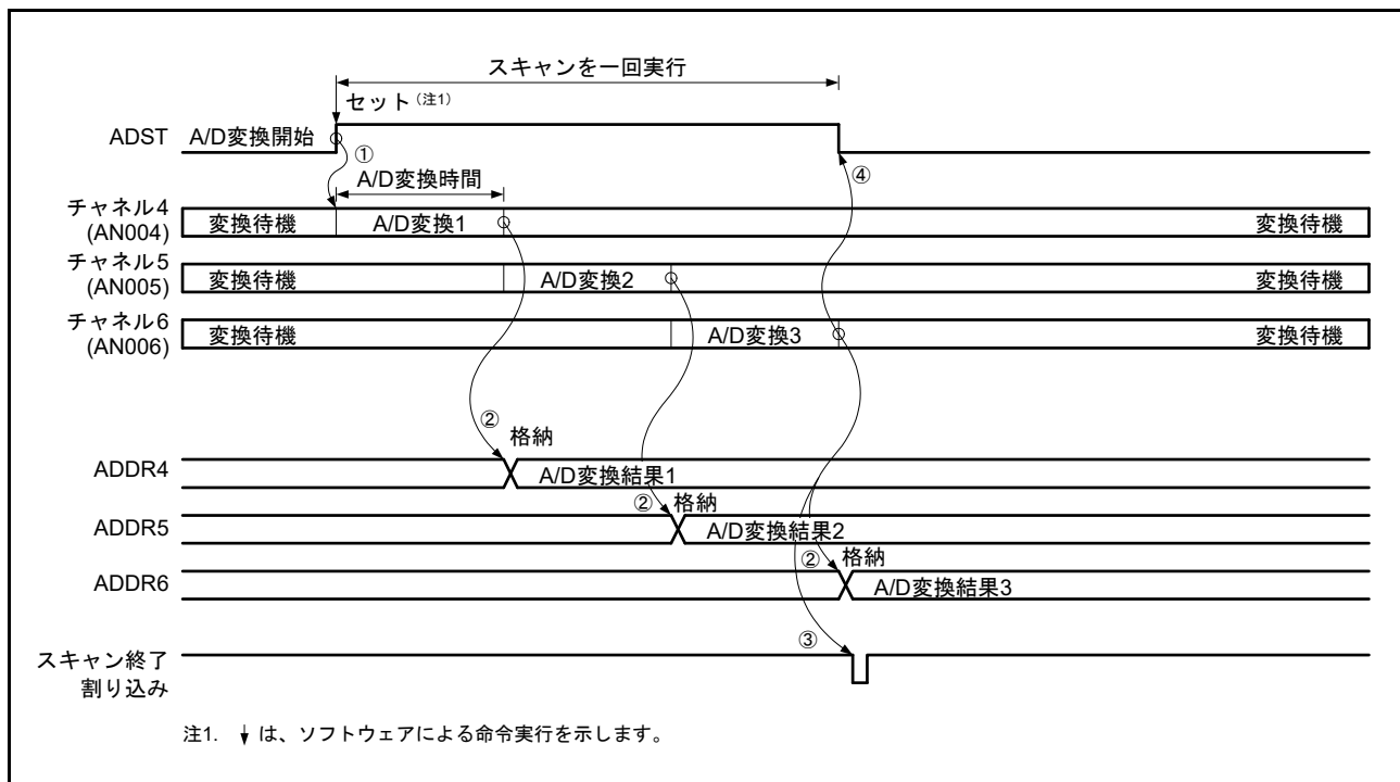
図 56.6 シングルスキャンモードの動作例 (基本動作 : AN004, AN005, AN006 選択)
