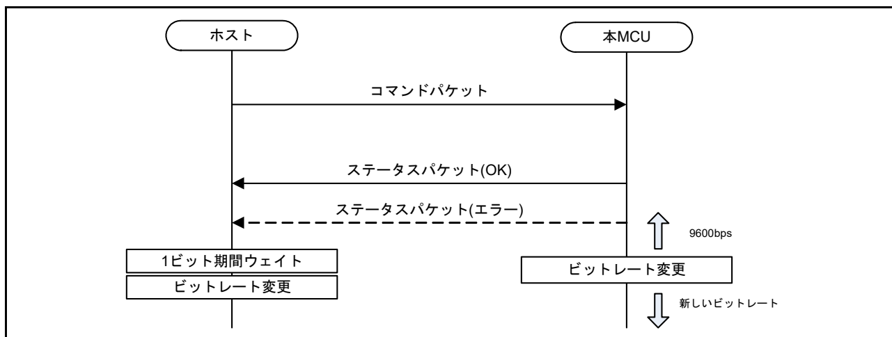
図 62.45 ビットレート設定コマンドの通信シーケンス
