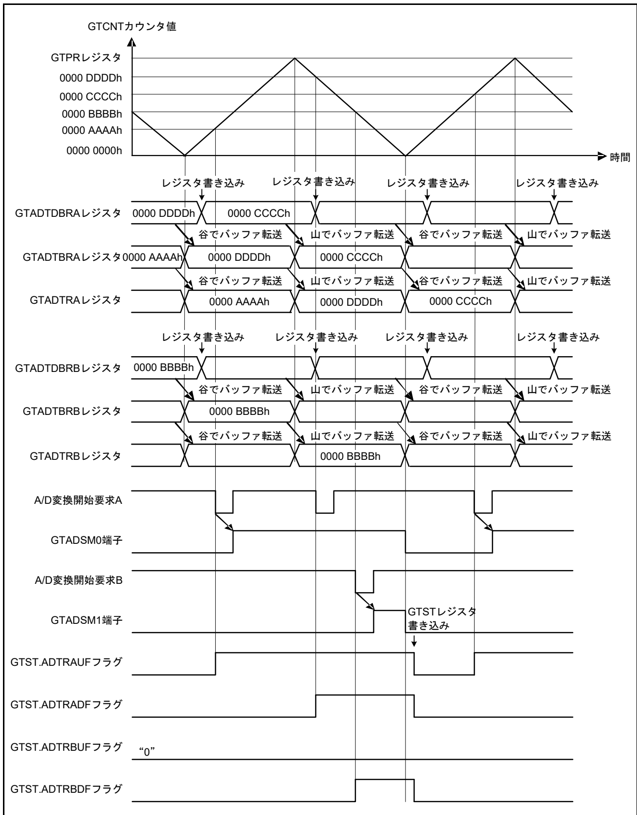
図 26.115 A/D 変換開始要求の動作例
