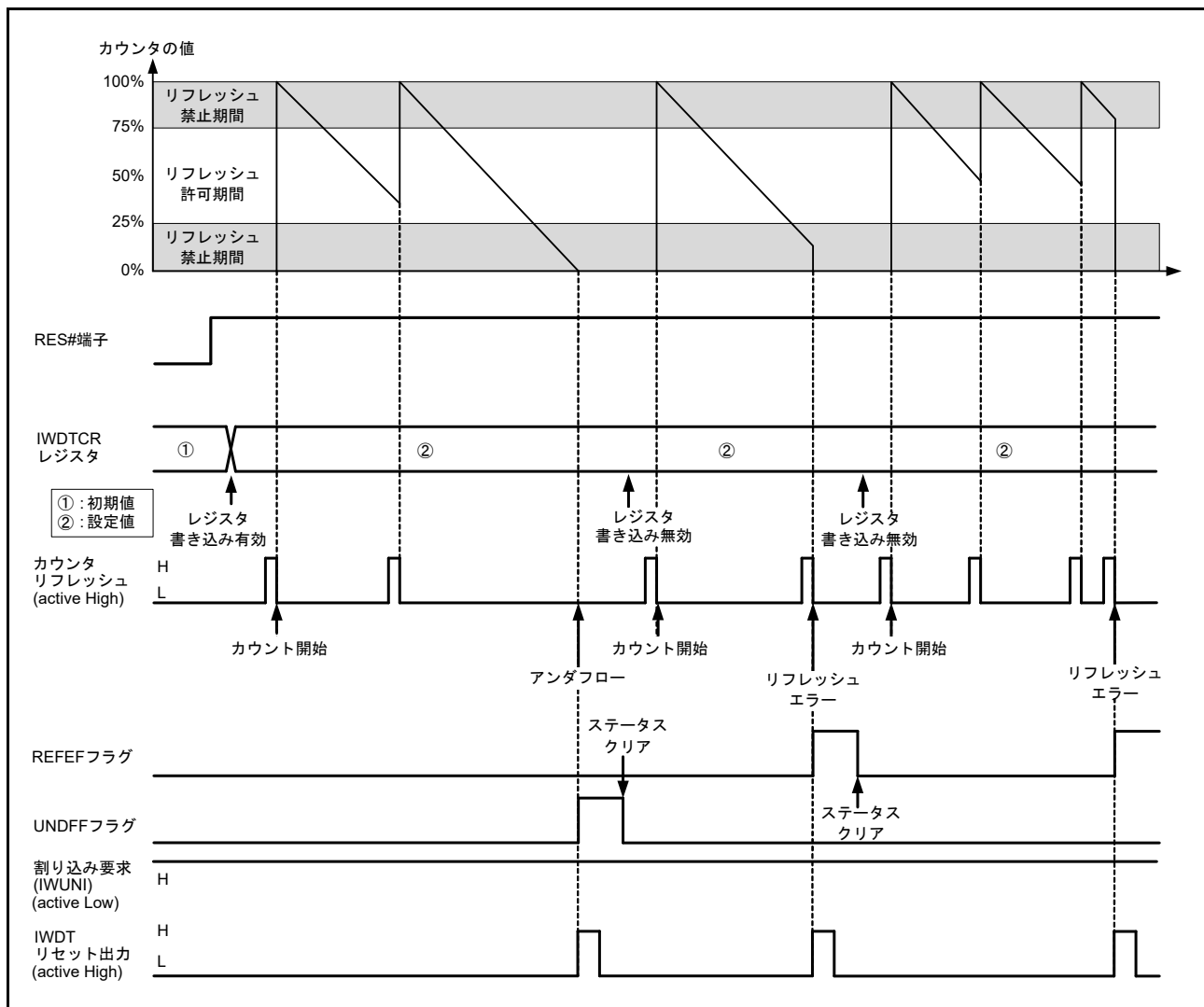
図 35.3 レジスタスタートモード動作例
