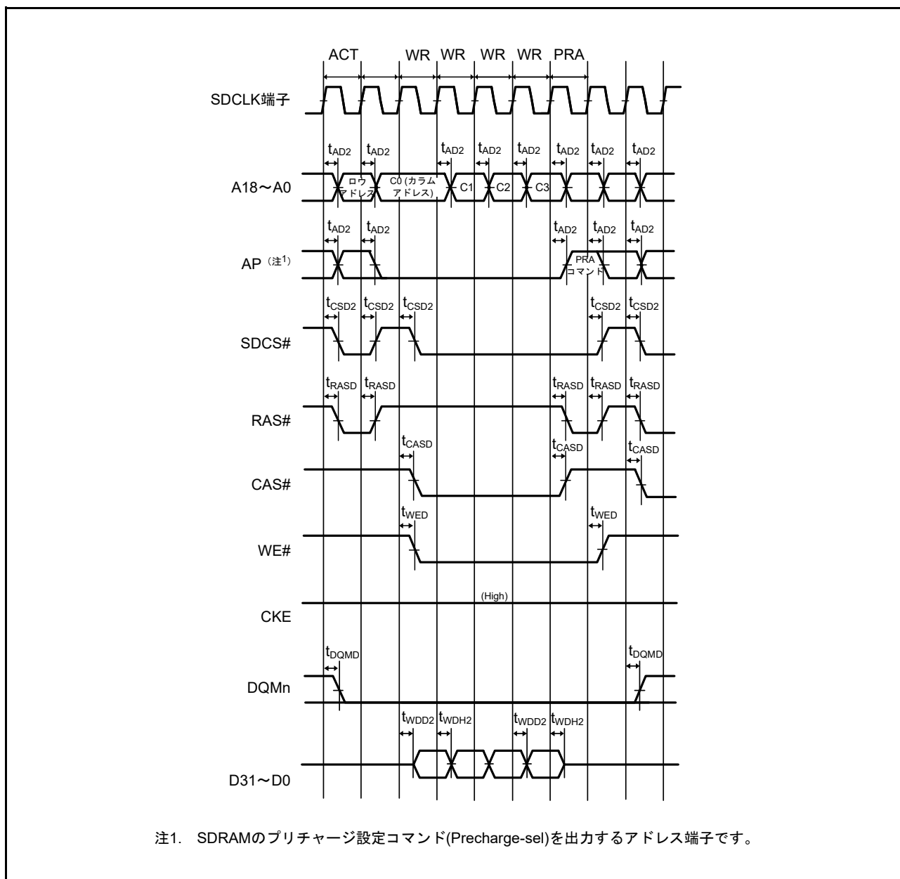
図 63.28 SDRAM 空間複数ライトバスタイミング
