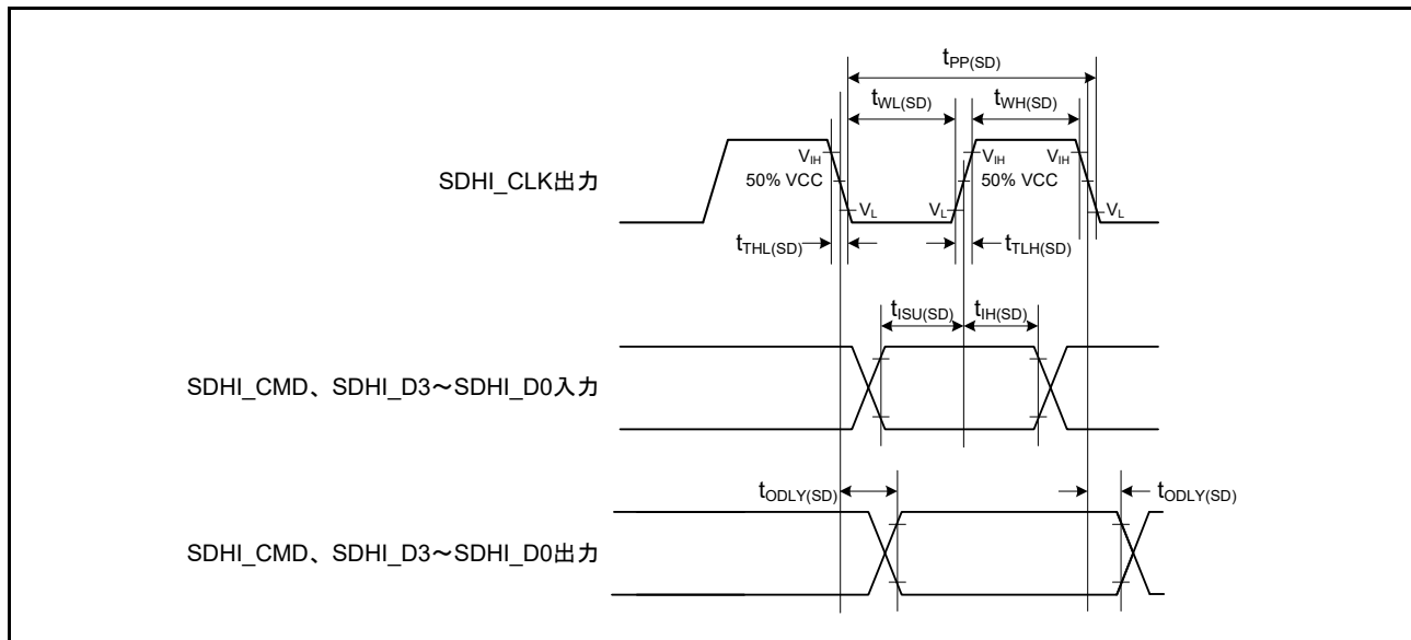
図 63.80 SD ホストインタフェース入出力信号タイミング
