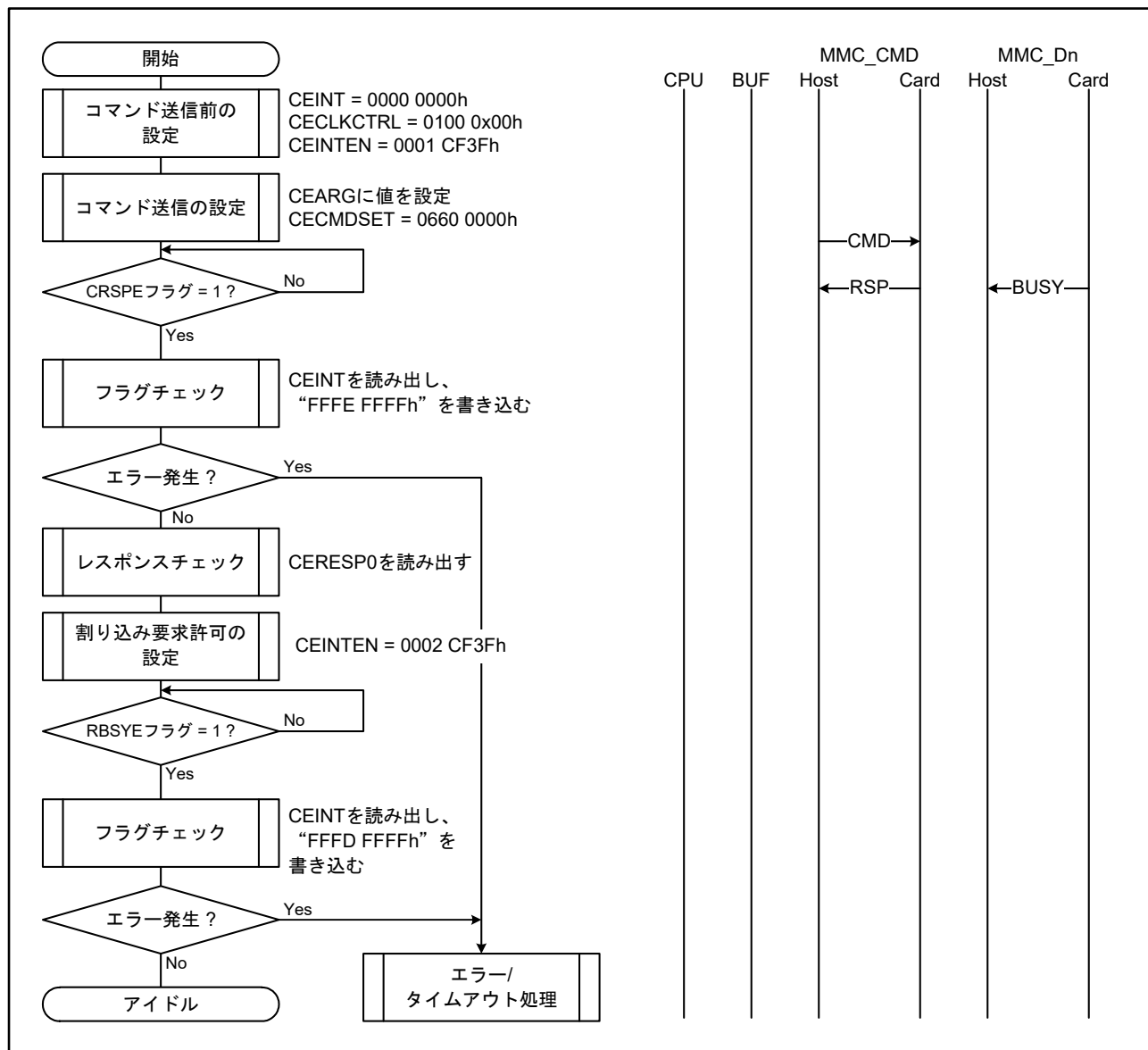
図 49.13 データ転送を行わないコマンド (レスポンスビジーあり) の送信例 (CMD6)
