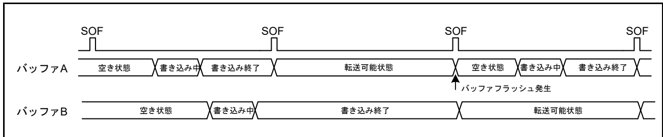
図 40.21 バッファフラッシュ機能動作例
