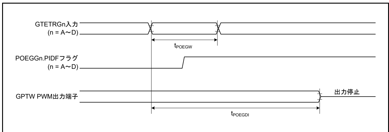
図 63.48 POEG 出力ディセーブル時間 (GTETRGn 端子の入力レベル検出 (フラグ経由))
