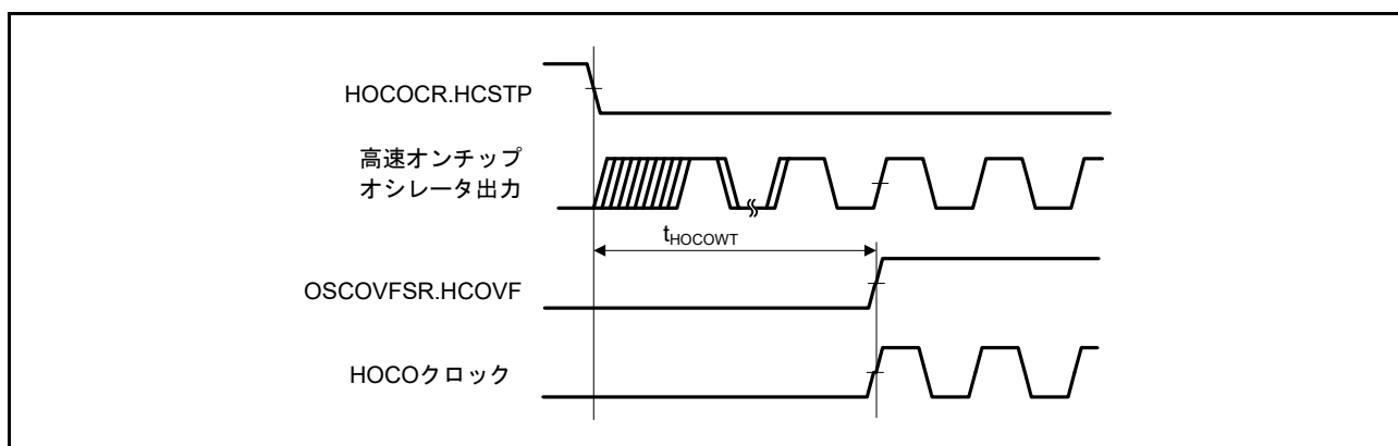
図 63.8 HOCO クロック発振開始タイミング (HOCOCR.HCSTP 設定による発振開始)
