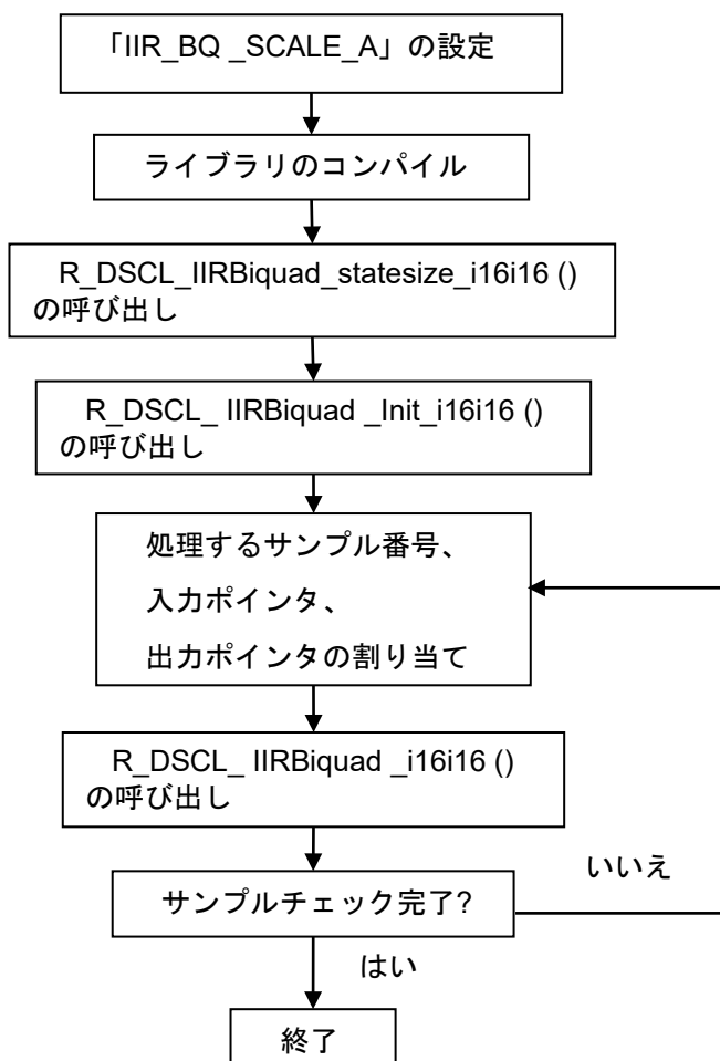
図4 処理フロー
