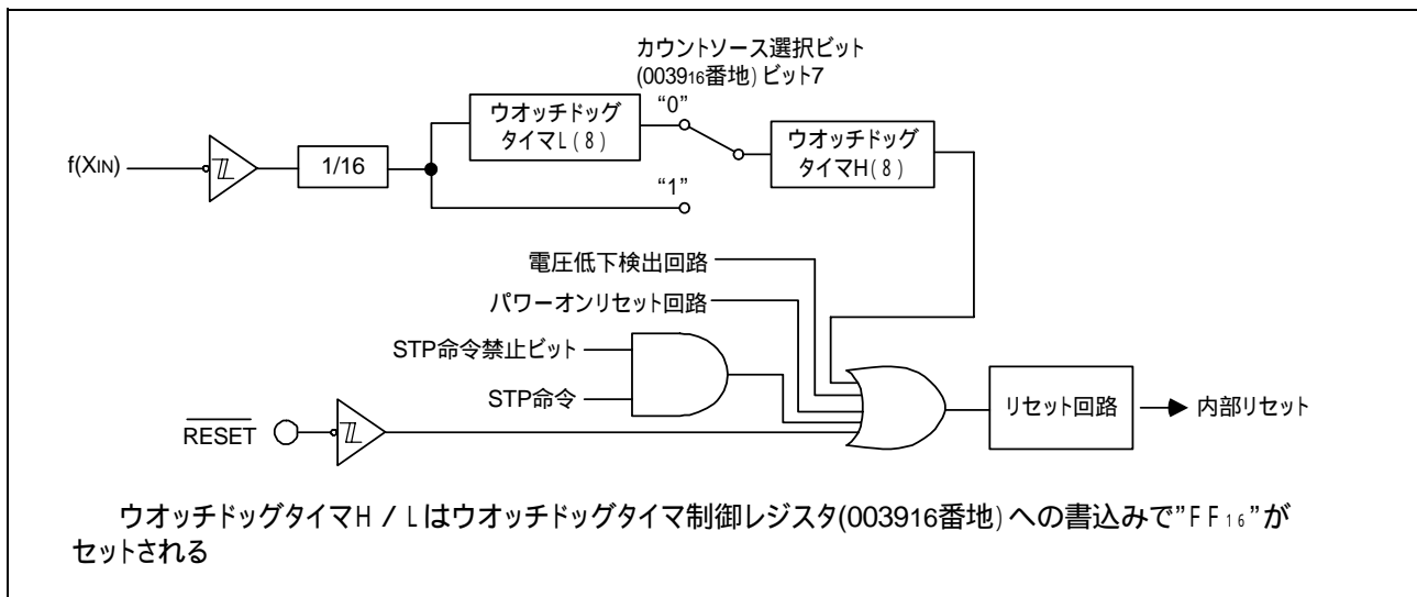
図 3.1 接続と分周比の設定
