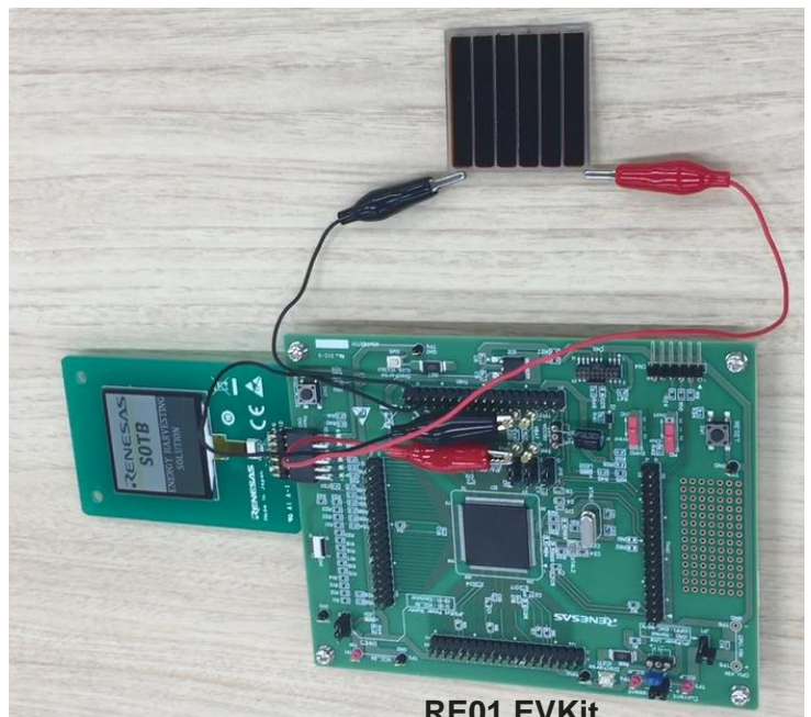
RE01 EVKit
