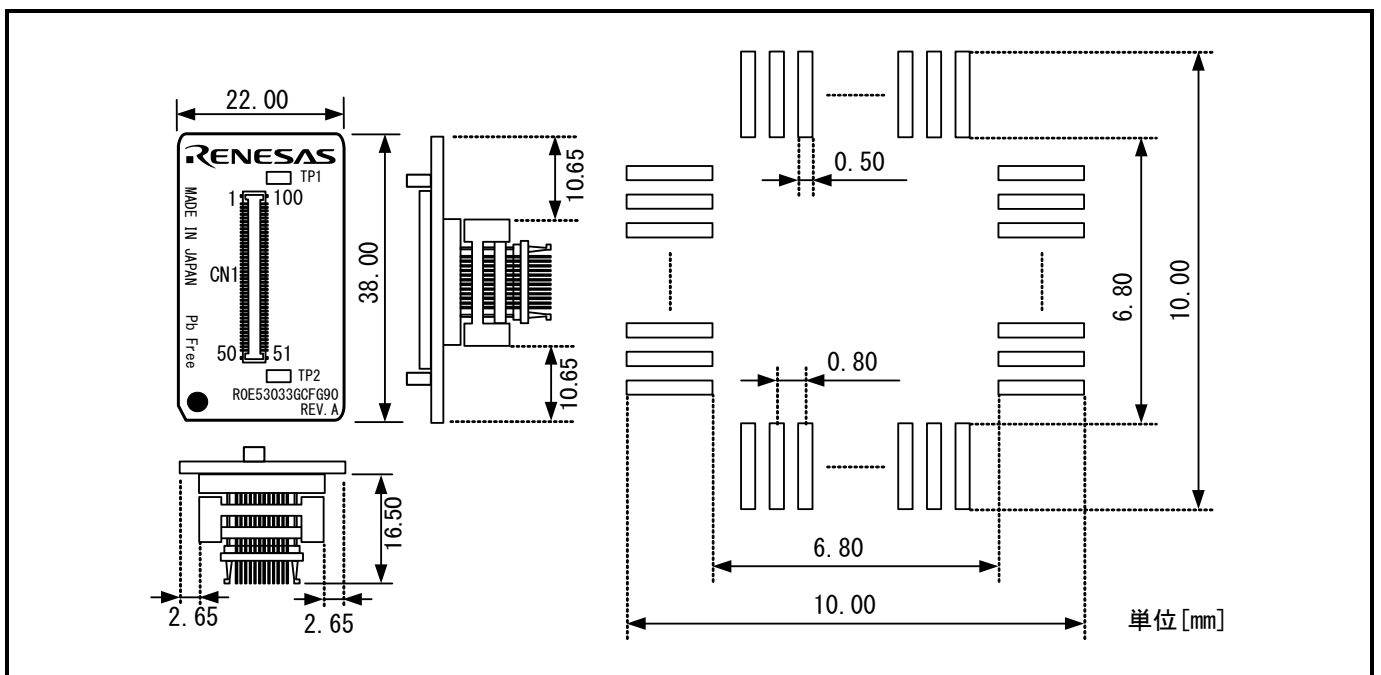
図7.6 ROE53033GCFG90ユーザーシステム接続部の寸法図および参考フットパターン
