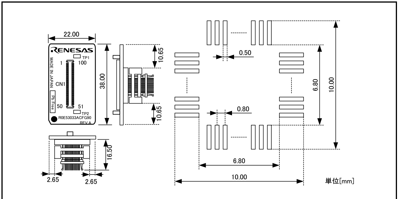
図7.5 ROE53033ACFG90ユーザーシステム接続部の寸法図および参考フットパターン
