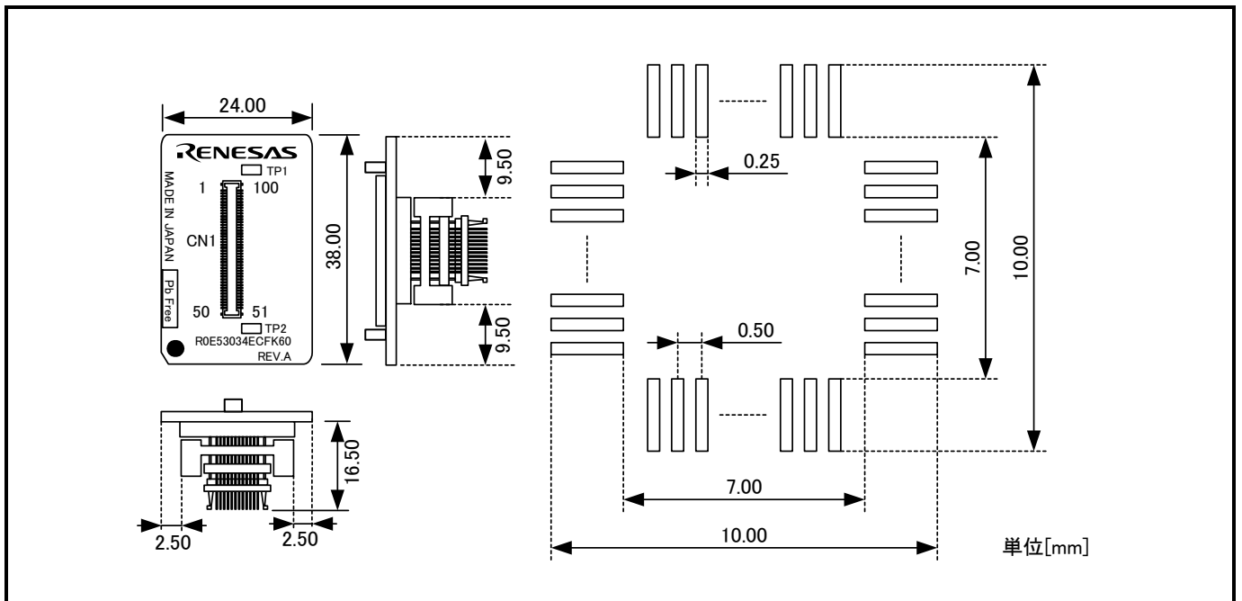
図7.8 ROE53034ECFK60ユーザーシステム接続部の寸法図および参考フットパターン
