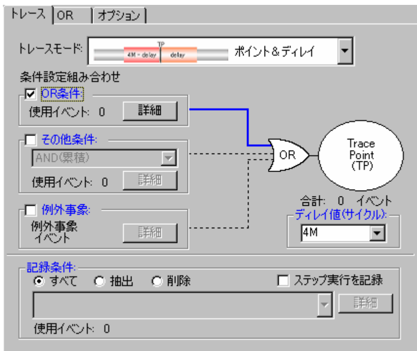
図5.50 [トレース条件設定]ダイアログボックス
