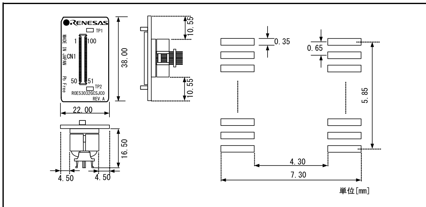
図7.4 ROE53032GCSJC0ユーザーシステム接続部の寸法図および参考フットパターン
