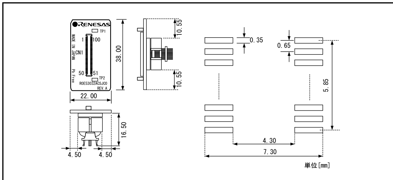
図7.3 ROE53032ACSJC0ユーザーシステム接続部の寸法図および参考フットパターン
