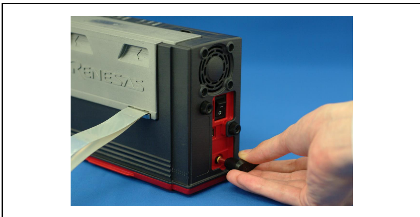
図2.5 エミュレータ用電源の接続
