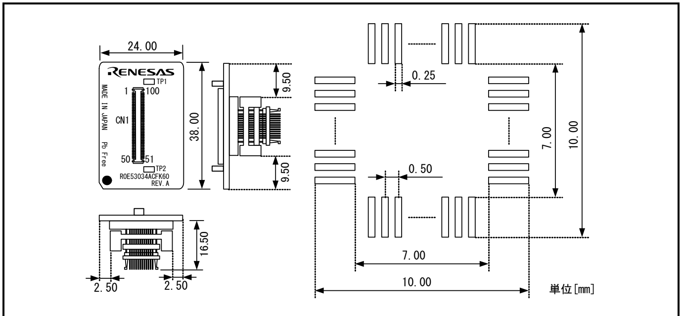
図7.7 ROE53034ACFK60ユーザーシステム接続部の寸法図および参考フットパターン
