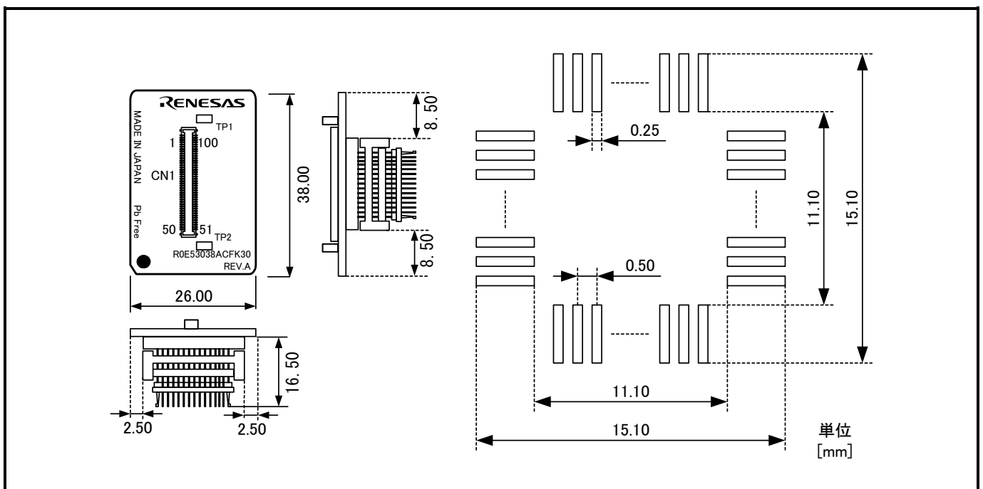
図7.12 R0E53038ACFK30ユーザーシステム接続部の寸法図および参考フットパターン
