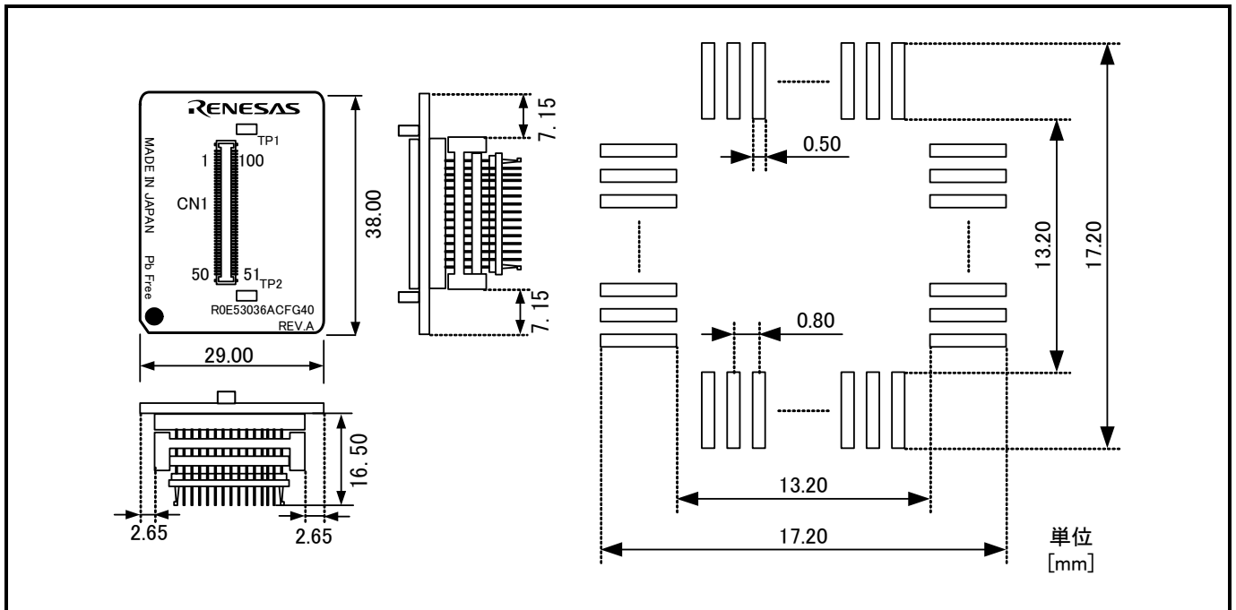
図7.11 R0E53036ACFG40ユーザーシステム接続部の寸法図および参考フットパターン
