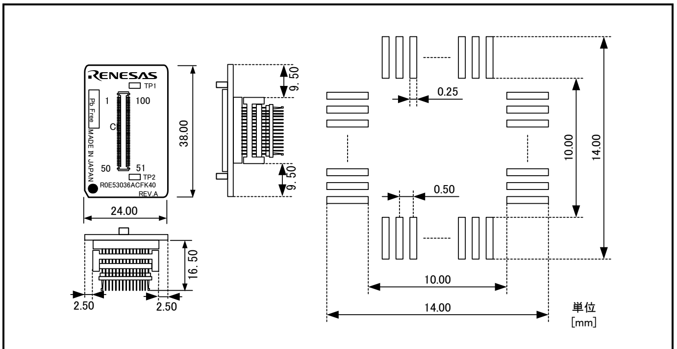
図7.10 R0E53036ACFK40ユーザーシステム接続部の寸法図および参考フットパターン
