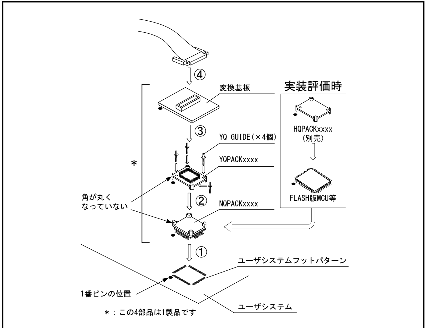
図2.11 ユーザシステムへの接続
