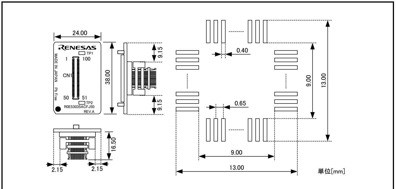
図7.9 R0E53035ACFJ50ユーザーシステム接続部の寸法図および参考フットパターン
