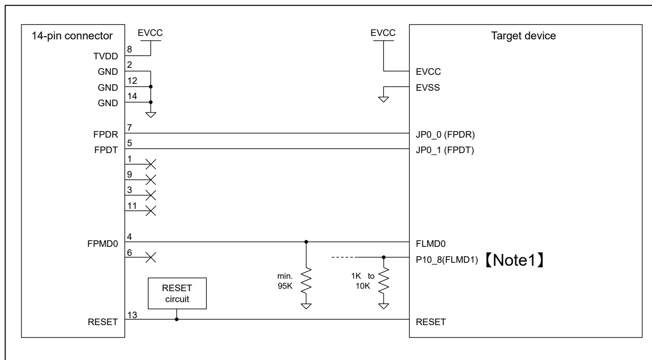
図 2-7 接続例
