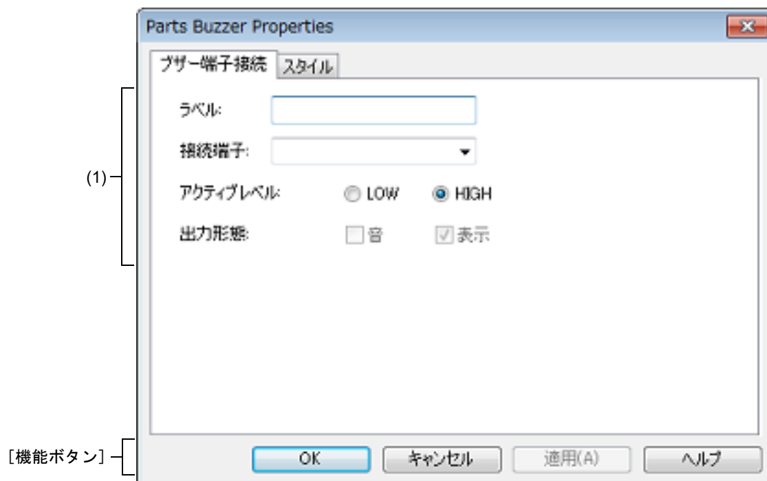
図 A.87 Parts Buzzer Properties ダイアログ : [ブザー端子接続] タブ
