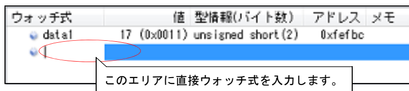
図 2.63 ウォッチ式のエントリ・ボックス
