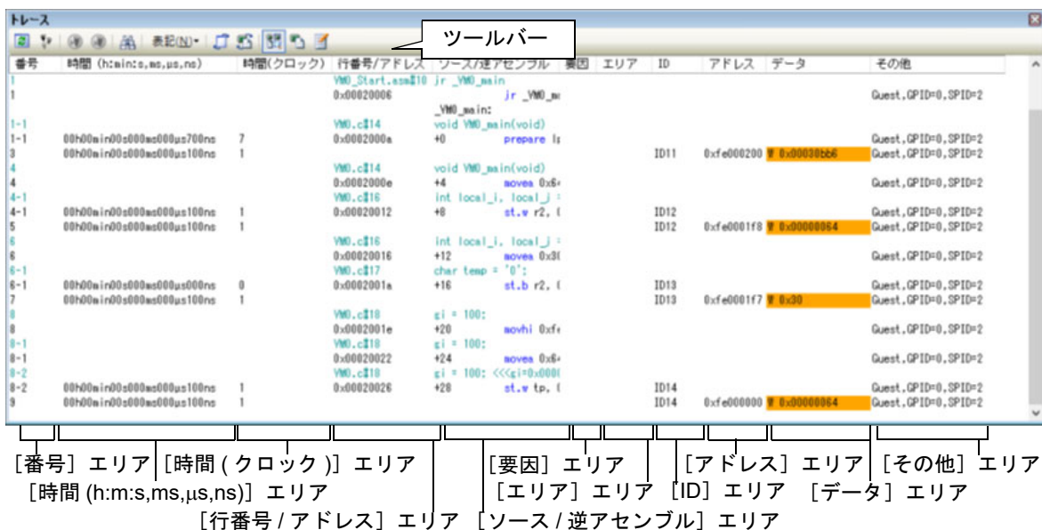
図 2.70 トレース・データの表示（トレース パネル【Full-spec emulator】【E1】【E20】）
