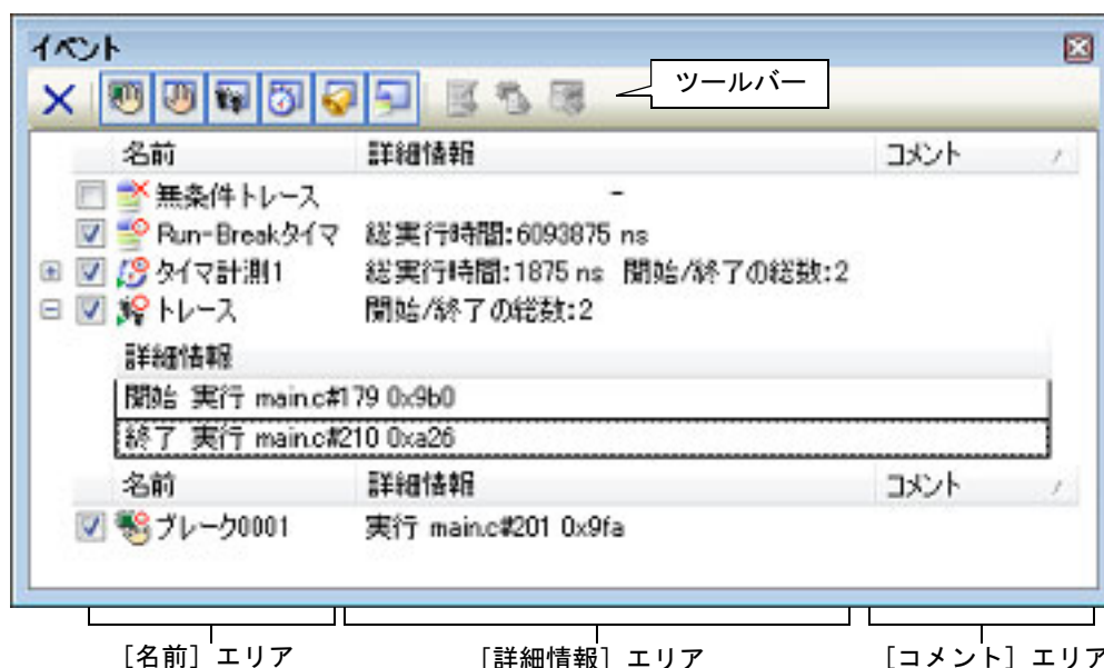
図 2.93 設定したイベントの表示（イベントパネル）
