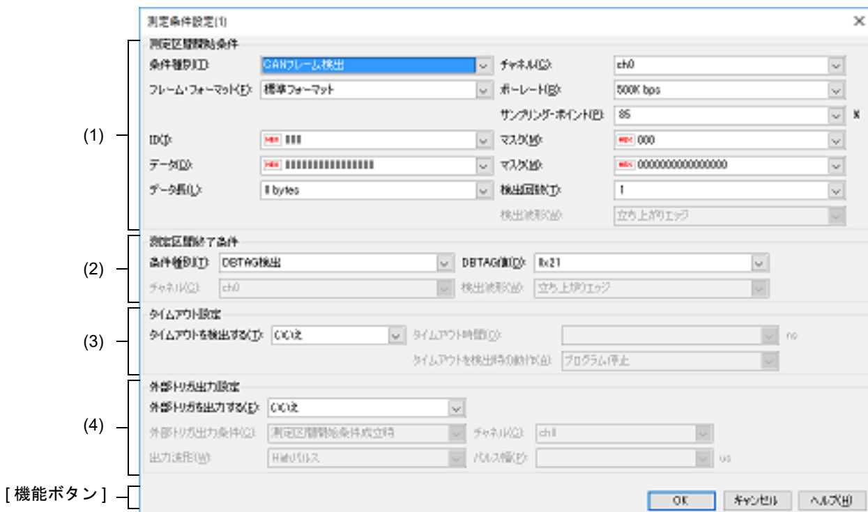
図 A.66 CAN 受信処理時間測定条件設定 ダイアログ
