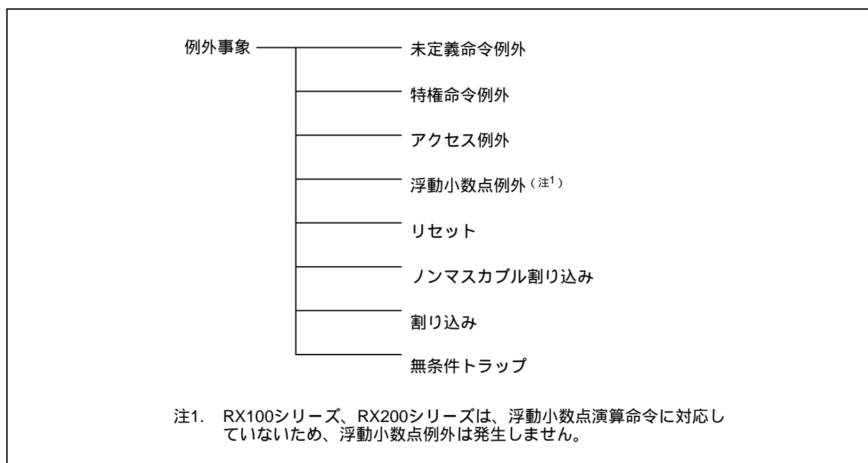
図 5.1 例外事象の種類
