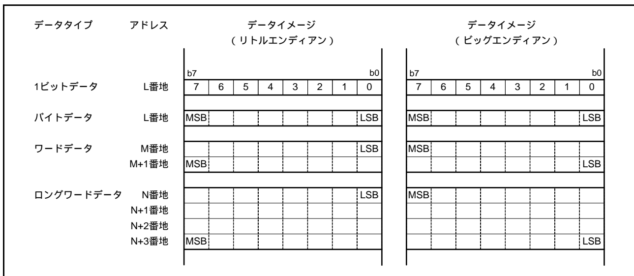
図 1.7 メモリ上のデータ配置
