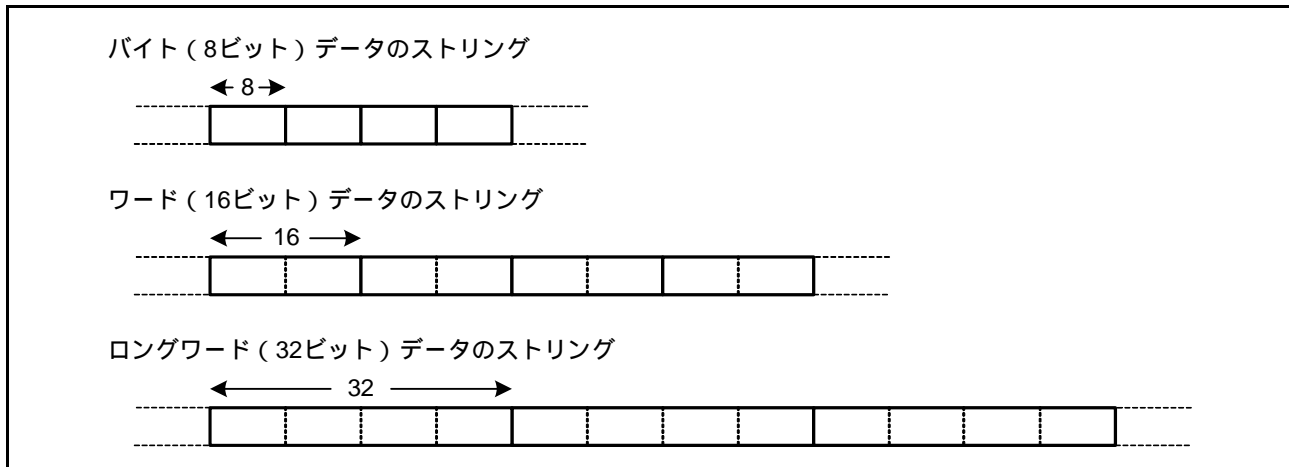
図 1.5 ストリング
