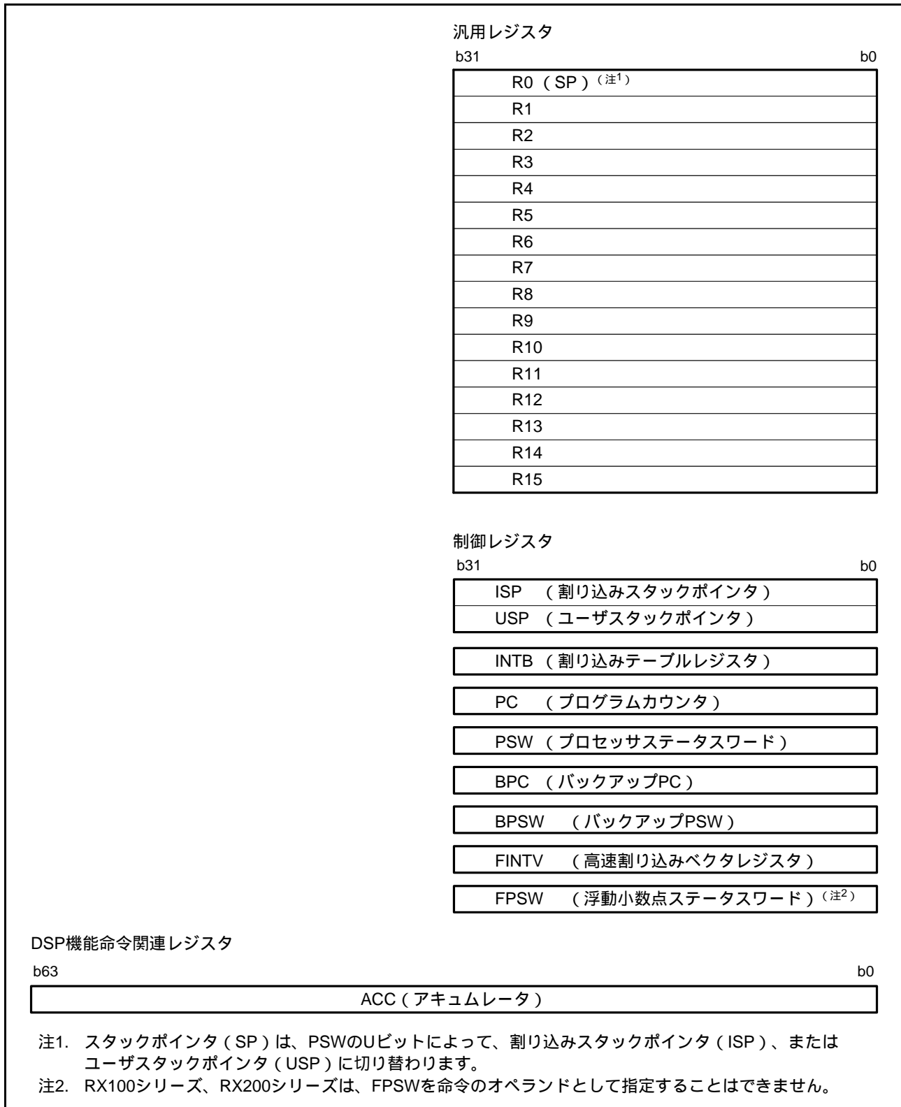
図 1.1 CPUレジスタセット
