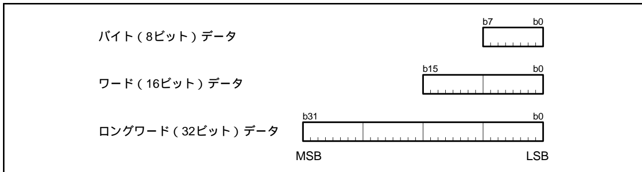
図 1.6 レジスタのデータ配置
