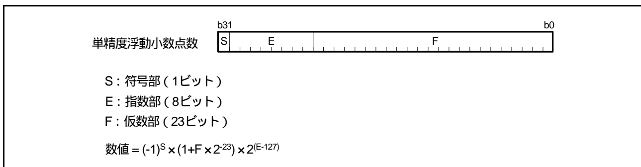
図 1.3 浮動小数点数
