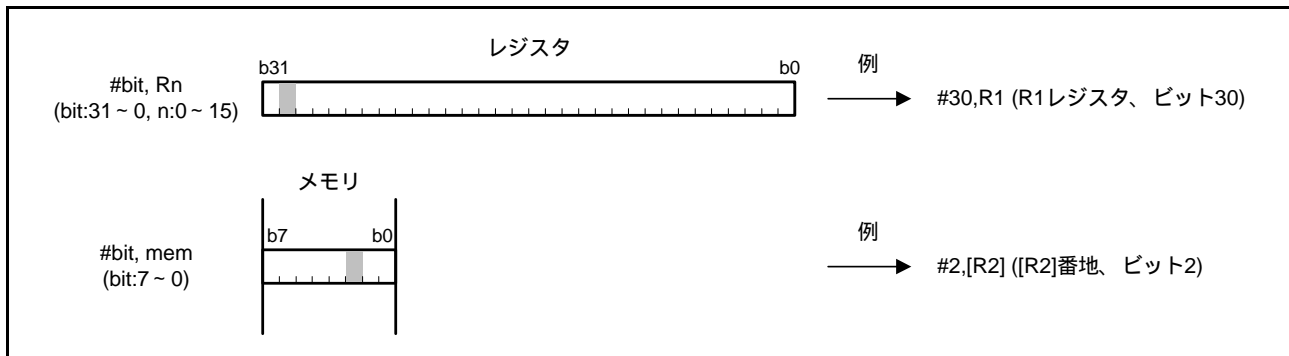
図 1.4 ビット
