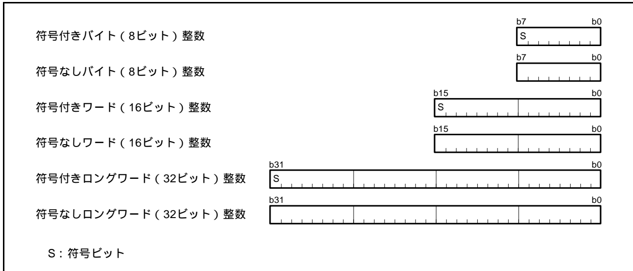
図 1.2 整数
