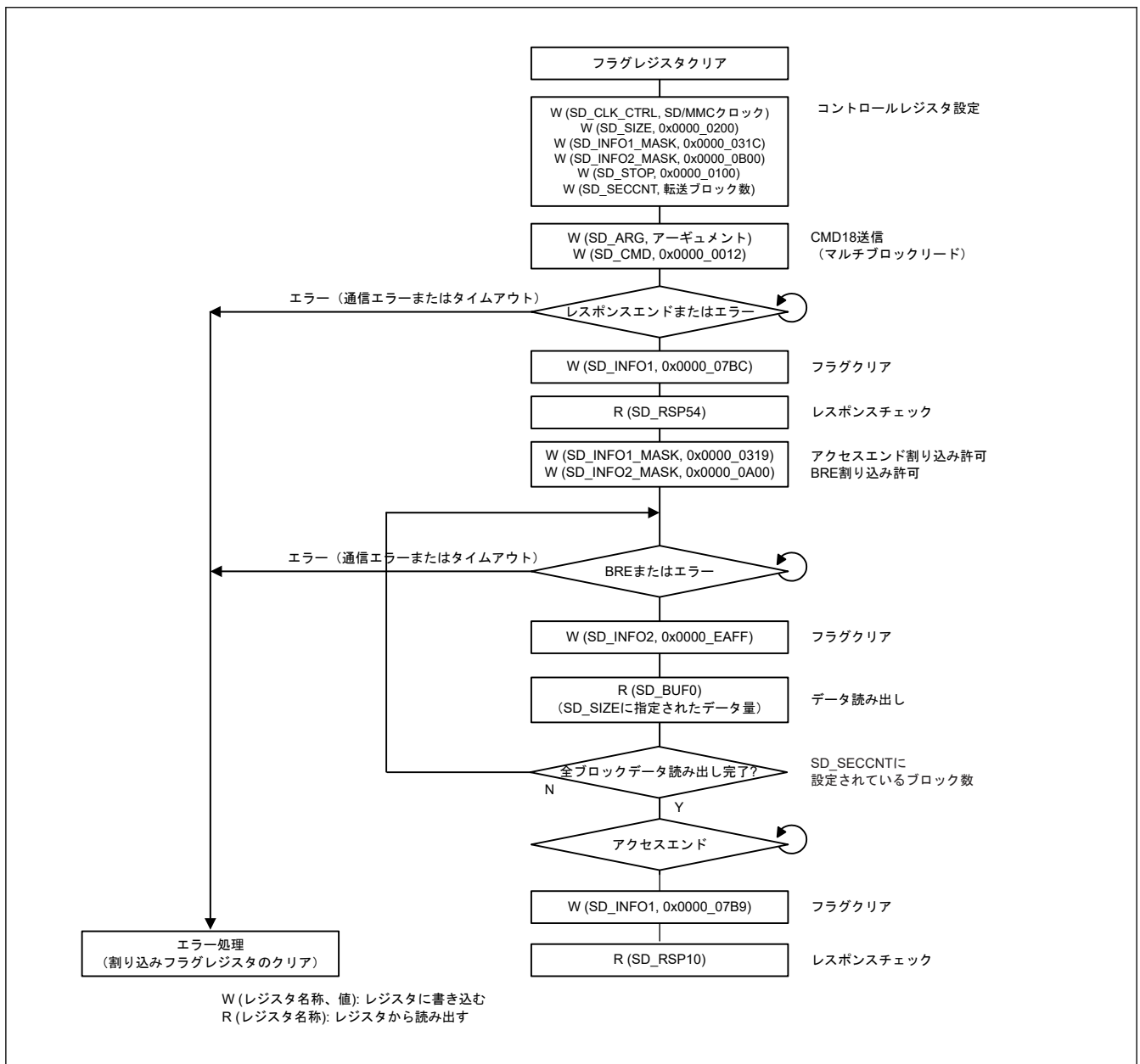
図 33.13 マルチブロックリード動作の例
