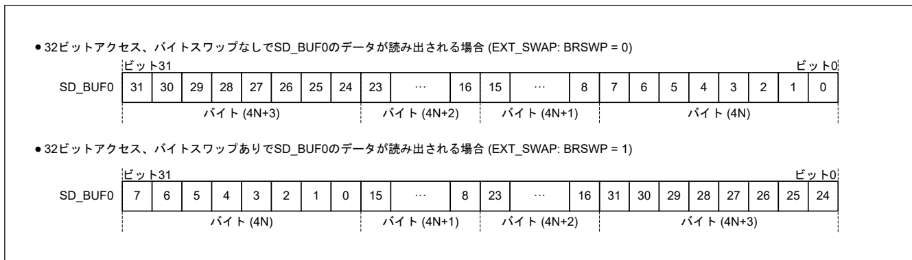
図 33.6 SD_BUF0 からの読み出し
