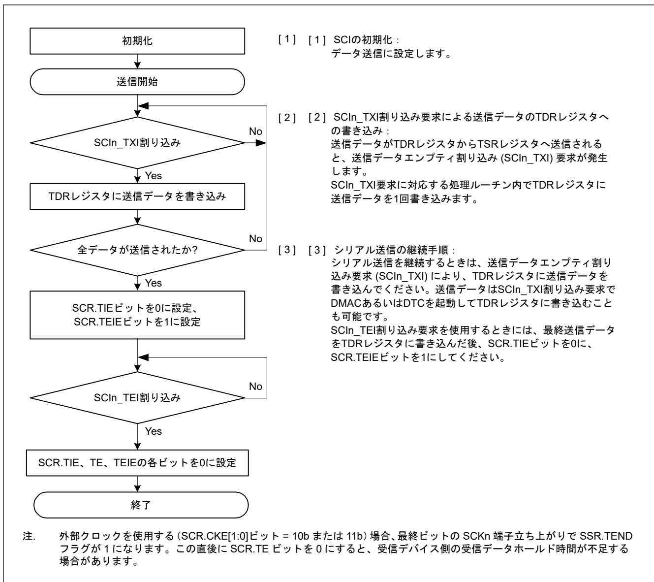
図 27.69 クロック同期式モードにおけるシリアル送信のフローチャート例 (非 FIFO 選択時)
