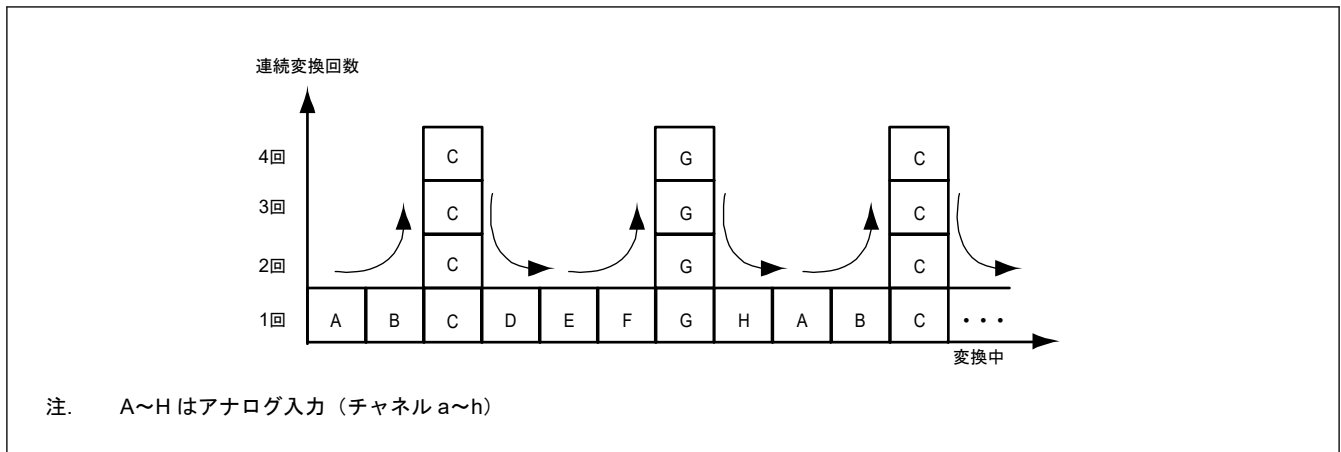
図 37.3 ADADC.ADC[2:0] = 011b および ADADS0/1 によるアナログ入力 C と G を 1 に選択時のスキャン変換シーケンス
