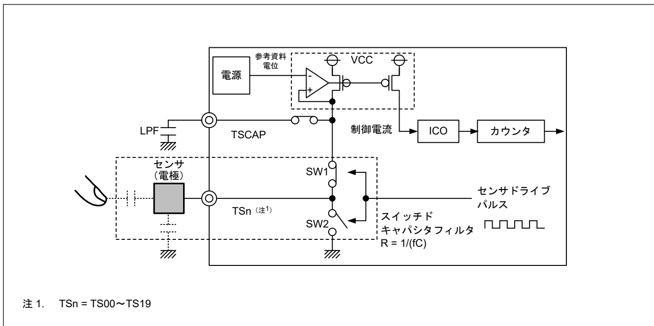
図 40.4 計測部回路
