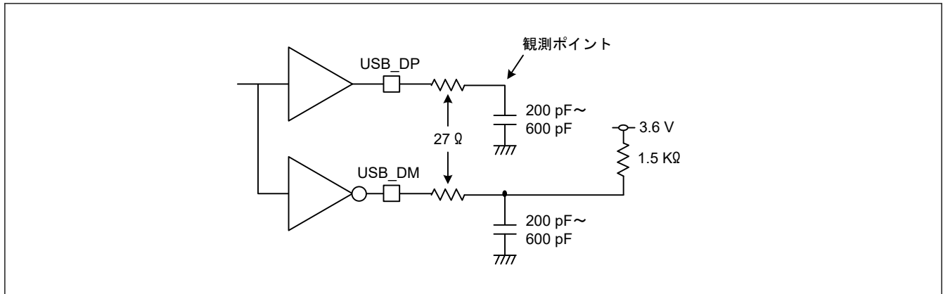
図 47.51 Low-speed モードにおける測定回路
