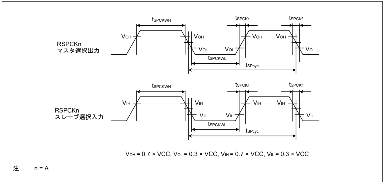
図 47.34 SPI クロックタイミング
