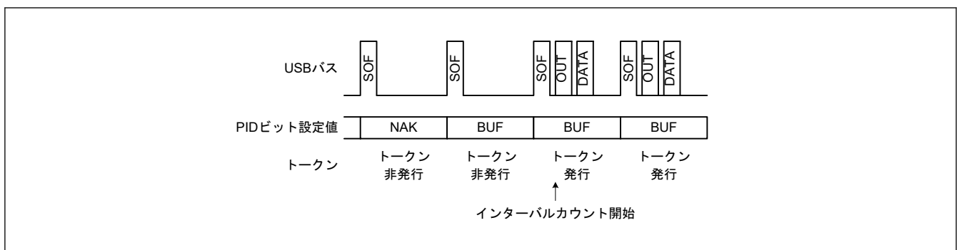
図 26.17 IITV[2:0] = 0 の場合のトークン発行の有無
