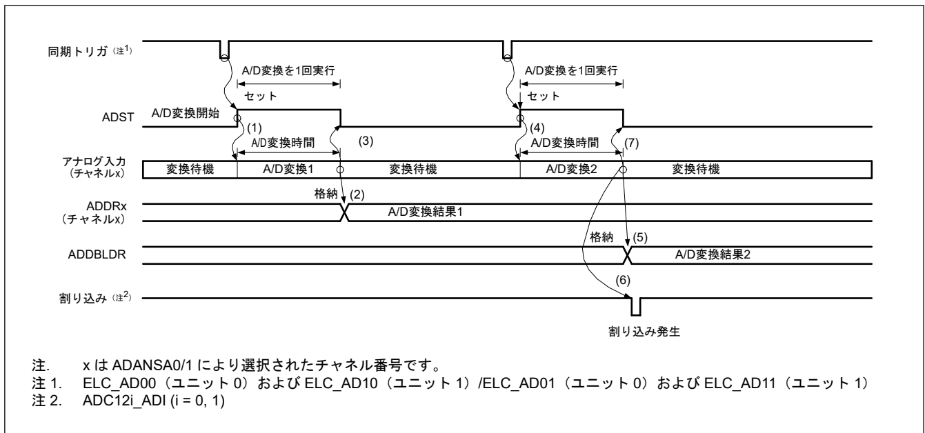
図 37.11 シングルスキャンモードの動作例 (ダブルトリガモード選択、アナログ入力 (チャンネル x) を2重化)
