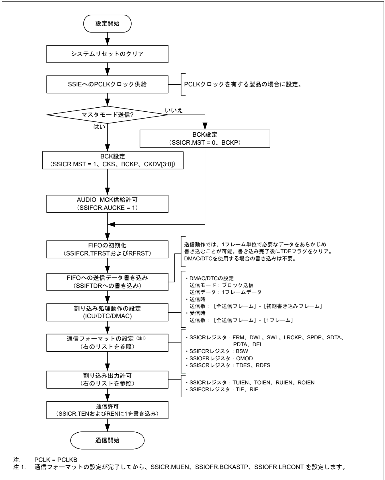
図 32.53 通信開始手順 (CPU 動作手順)
