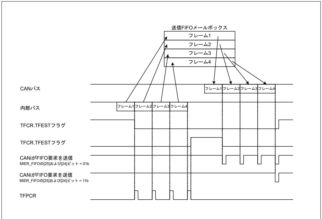
図 29.3 MIER_FIFO のビット[25]および[24]が 01b または 11b の場合の送信 FIFO メールボックスの動作説明
