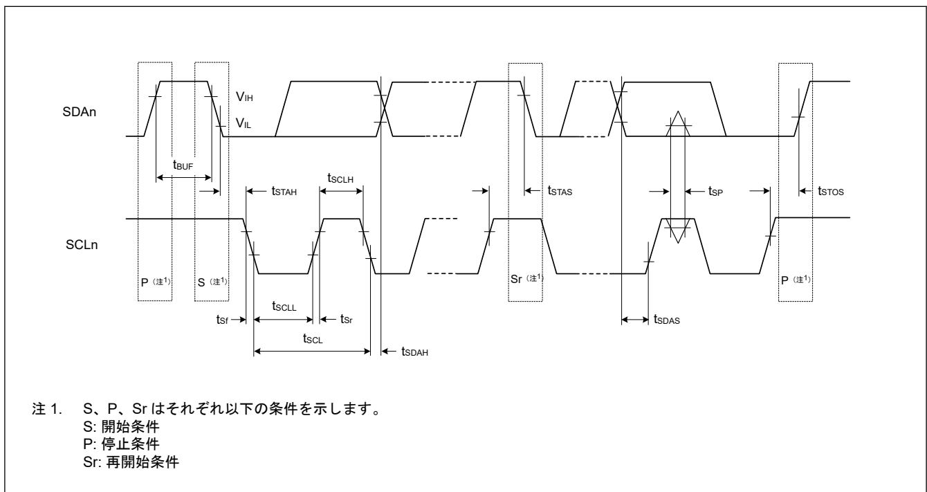
図 47.43 I 2 C バスインタフェース入出力タイミング
