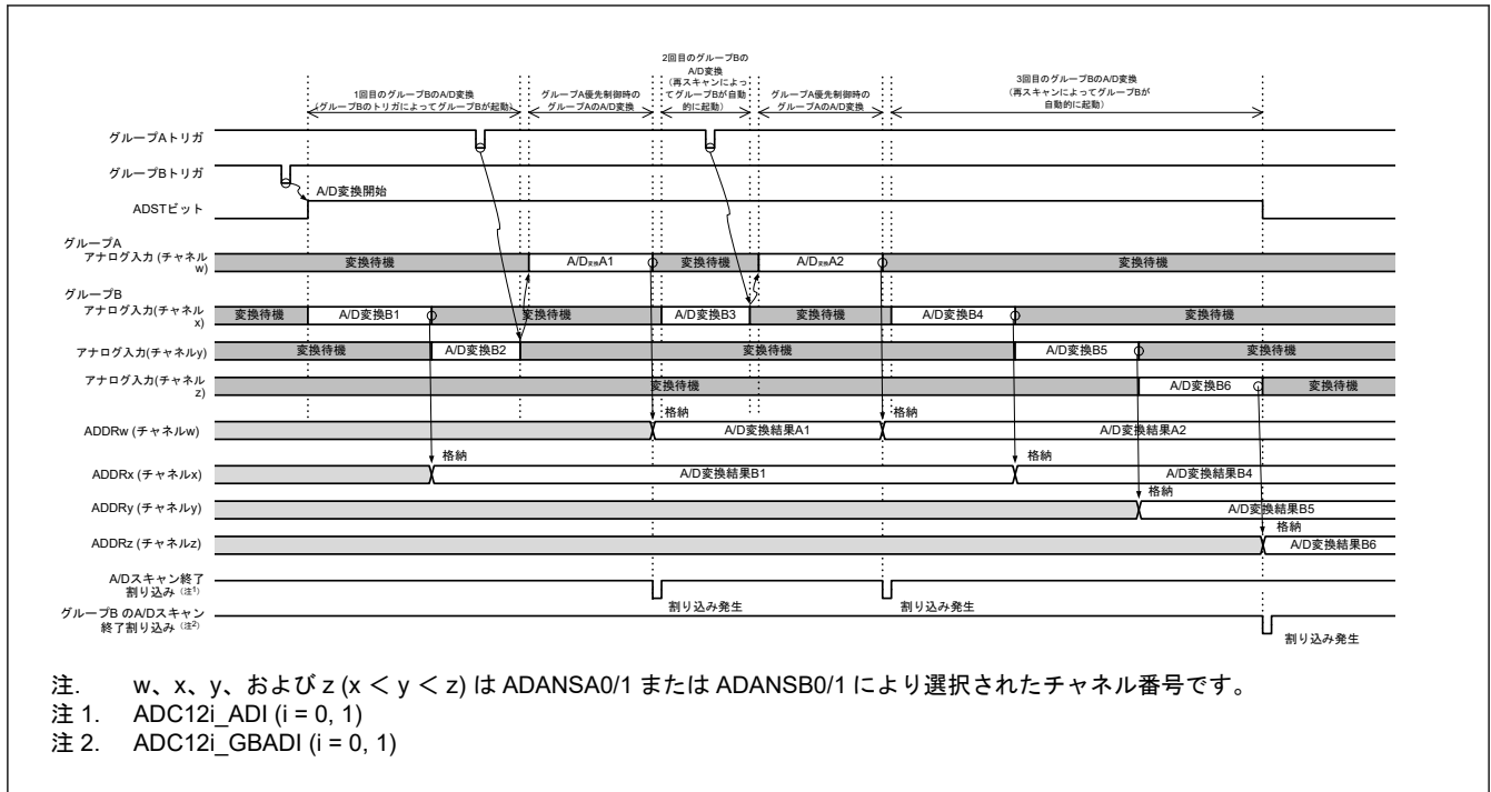
図 37.20 グループ優先動作の例 1-2 : グループ B 再スキャン中のグループ A トリガ入力、再スキャンあり (ADGSPCR.GBRSCN = 1、ADGSPCR.GBRP = 0、および ADGSPCR.LGRRS = 0 の場合)
