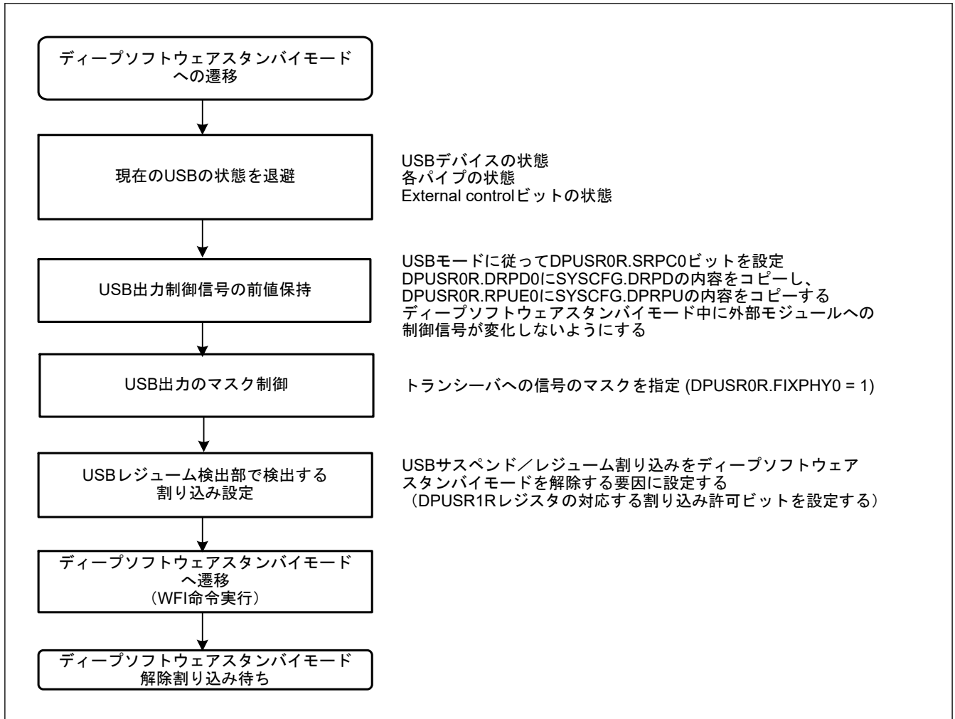
図 26.8 ホストコントローラ機能またはデバイスコントローラ機能選択時におけるディープソフトウェアスタンバイモード遷移時の USBFS 設定フロー
