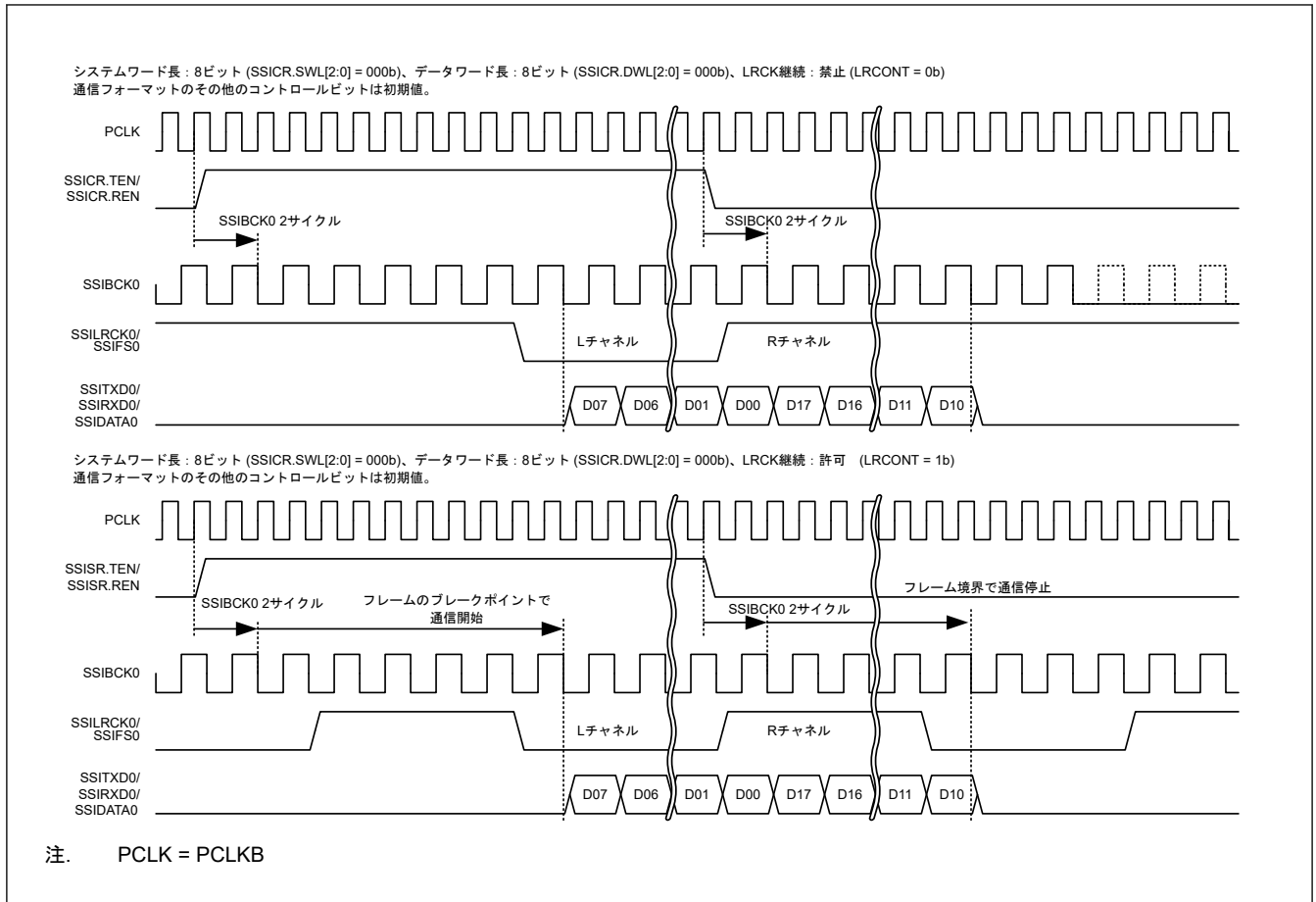
図 32.33 LR クロック/フレーム同期継続の動作例
