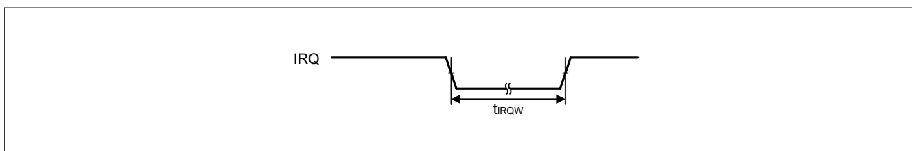
図 47.18 IRQ 割り込み入力タイミング
