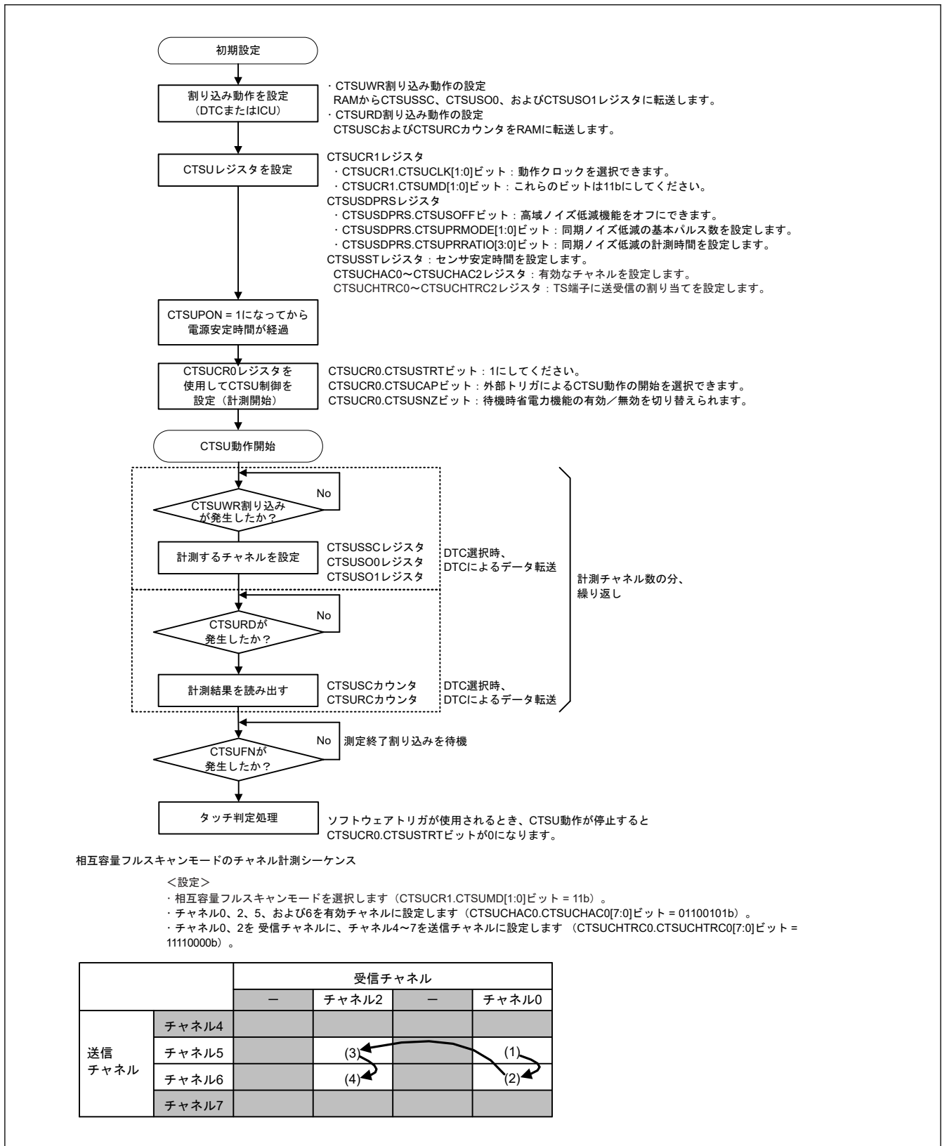
図 40.16 相互容量フルスキャンモードのソフトウェアフローと動作例
