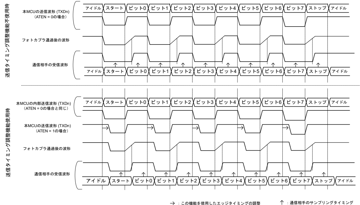
図 27.37 フォトカプラを経由する送信波形の説明
