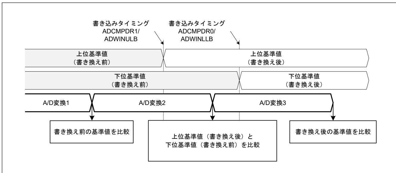
図 37.6 書き換え前後の上側基準値と下側基準値の比較
