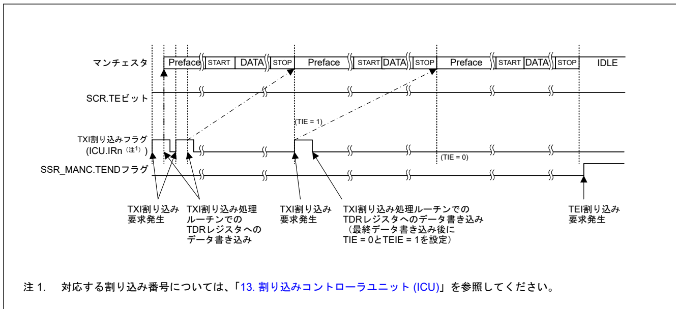
図 27.58 マンチェスタモードにおけるシリアル送信の終了動作の例（プレフィスあり、CTS 機能なし）
