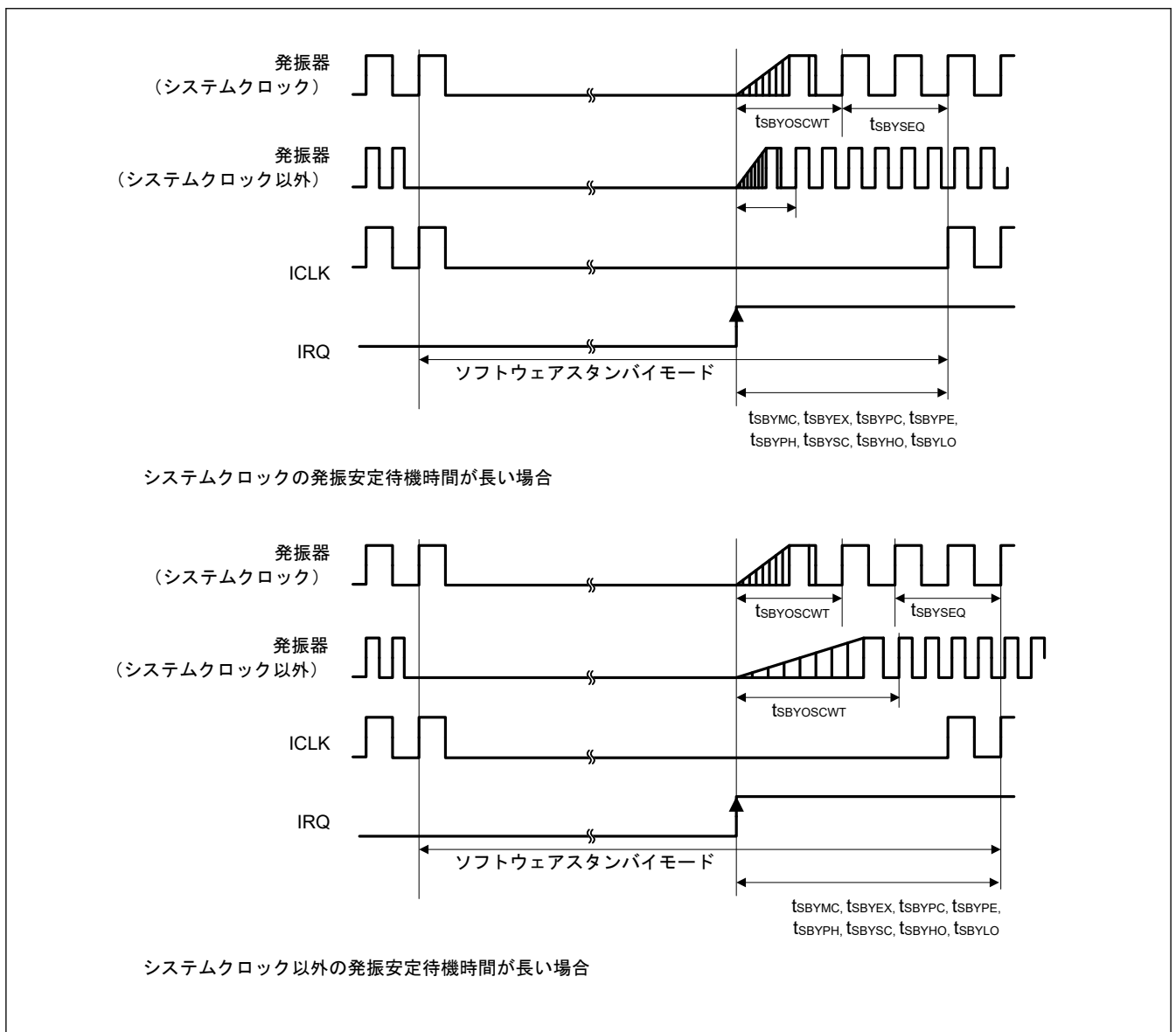
図 47.14 ソフトウェアスタンバイモード解除タイミング
