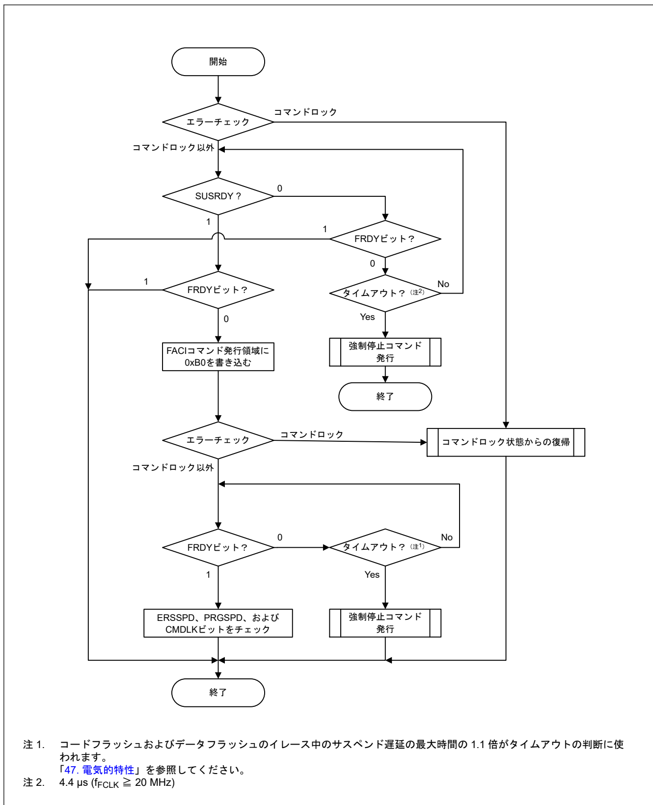
図 44.16 P/E サスペンドコマンドの使用フロー
