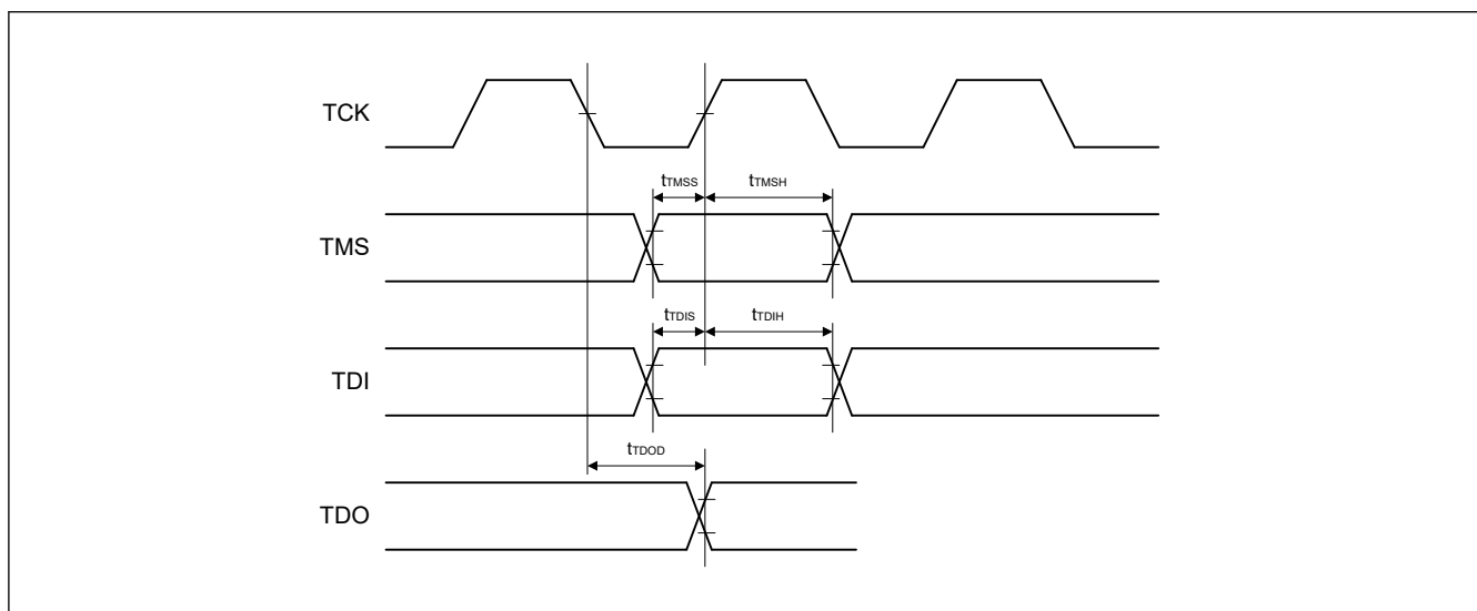
図 47.64 バウンダリスキャン入出カタイミング
