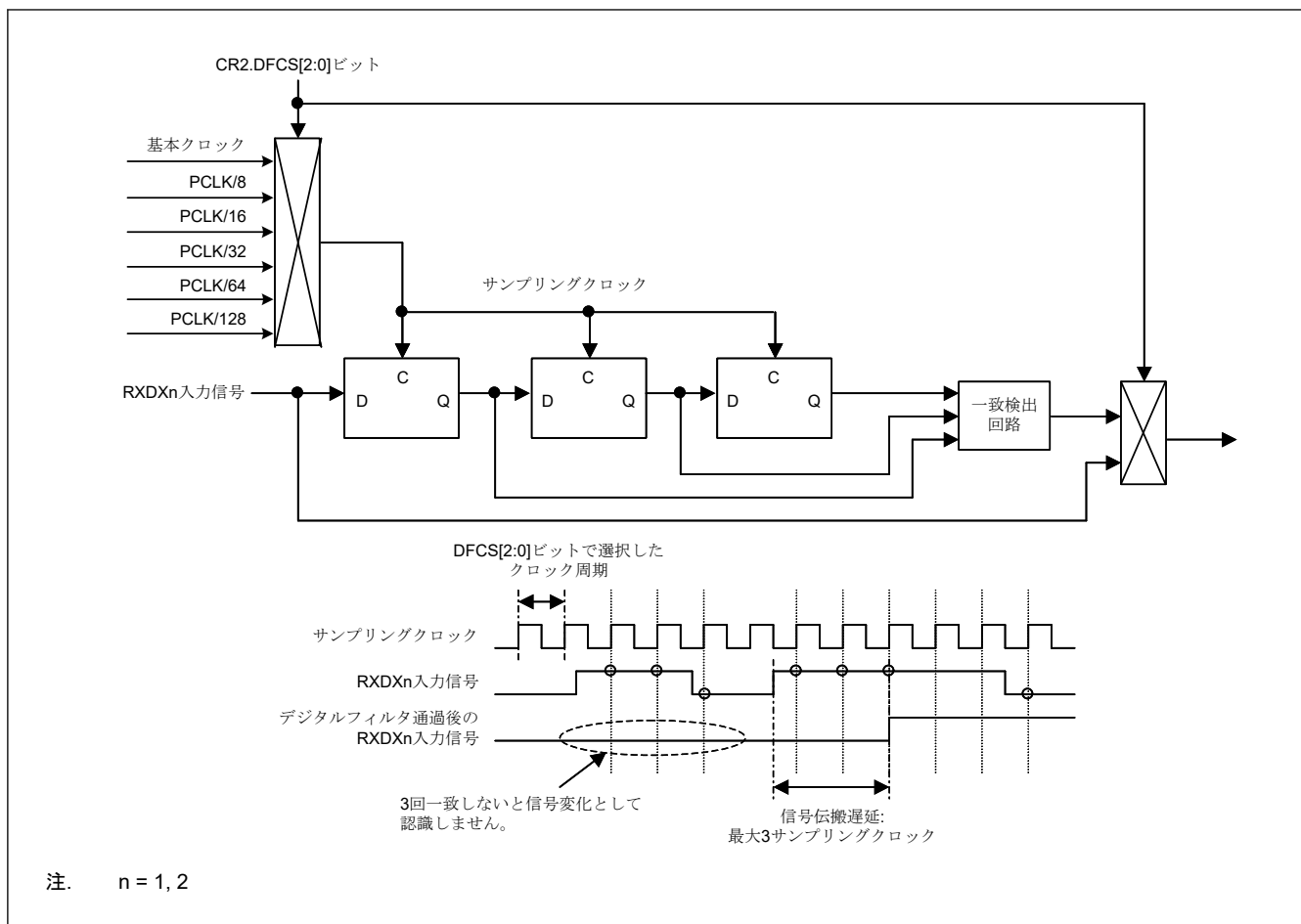
図 27.112 デジタルフィルタ機能の動作例
