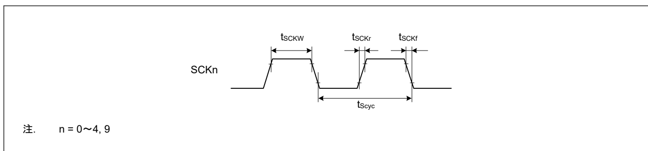
図 47.26 SCK クロック入出力タイミング
