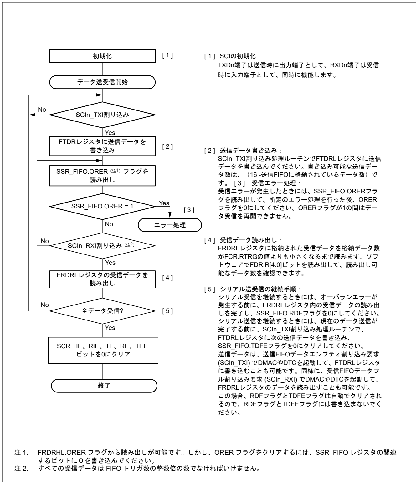
図 27.76 クロック同期式モードにおけるシリアル同時送受信動作のフローチャート例 (FIFO 選択時)
