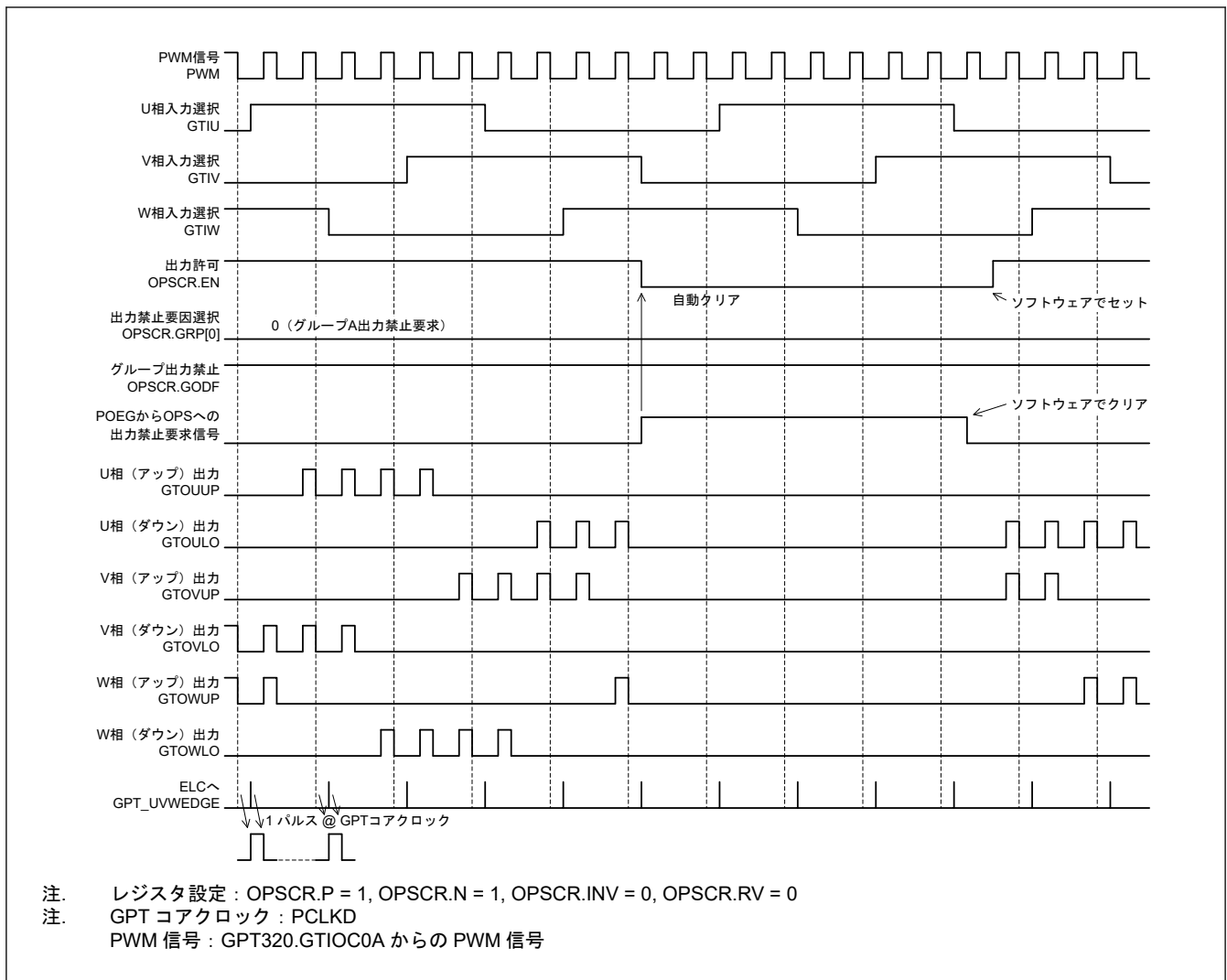
図 21.60 グループ出力禁止制御動作例
