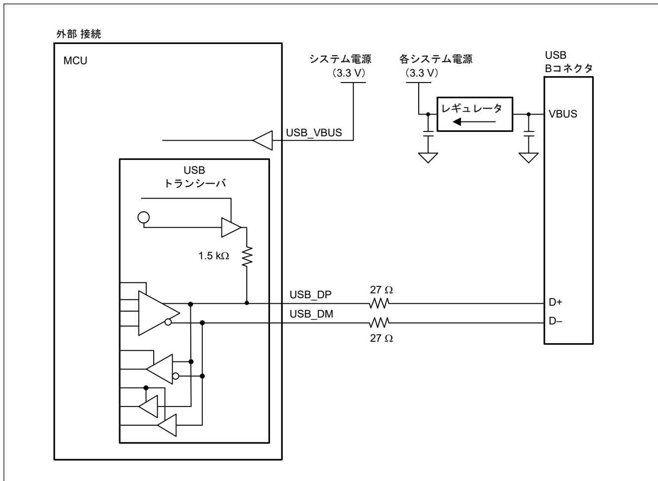
図 26.5 バスパワー状態でのデバイス接続例
