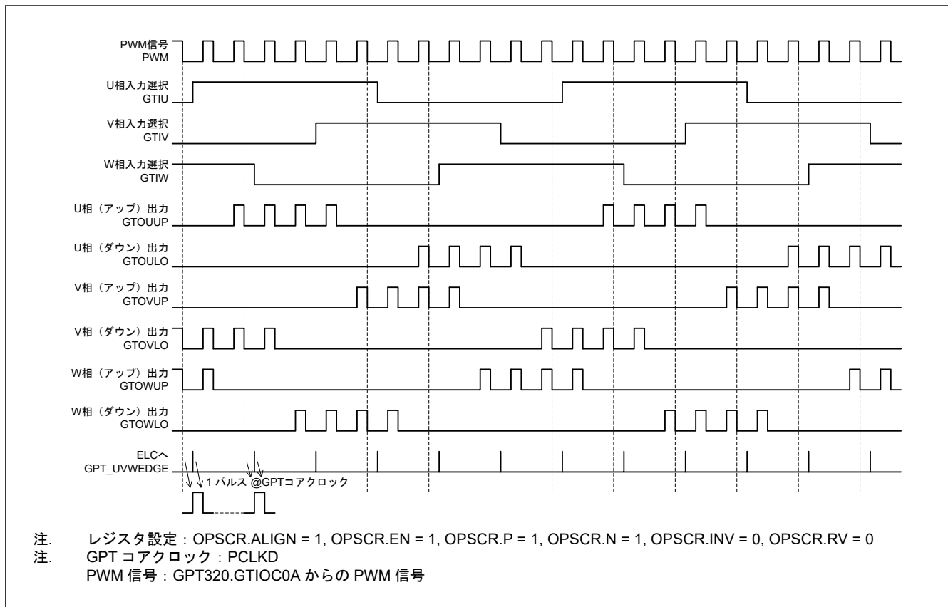
図 21.59 6相 PWM 出力動作例 (チョップ制御)
