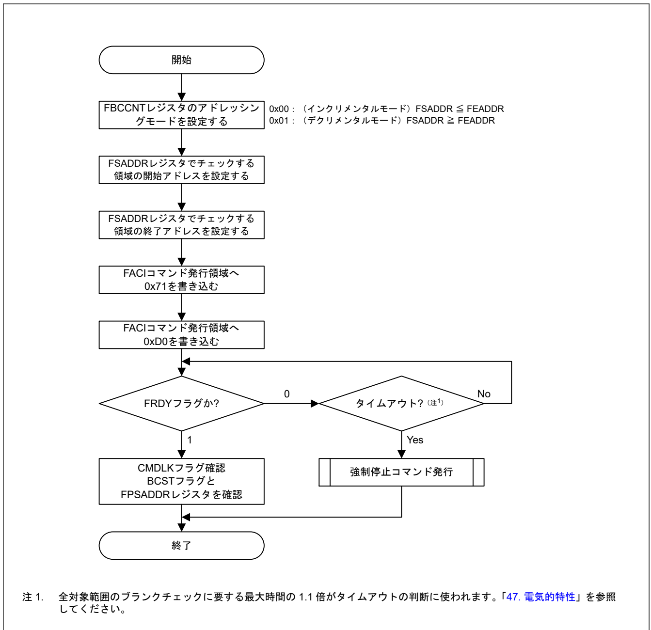
図 44.23 ブランクチェックコマンドの使用フロー
