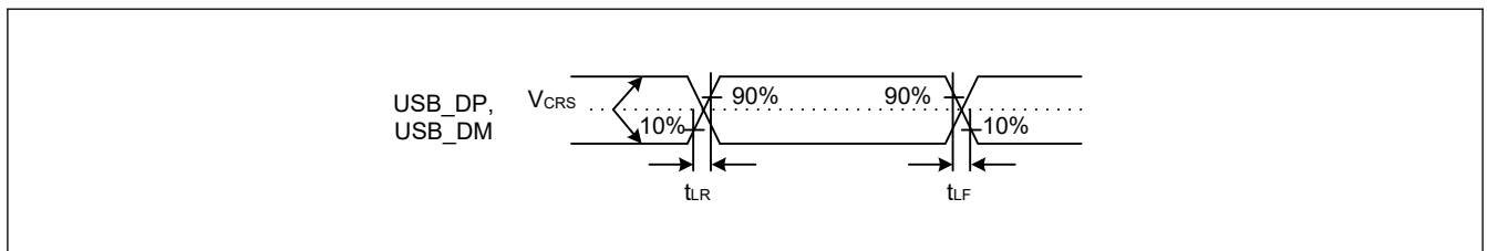
図 47.50 Low-speed モードにおける USB_DP、USB_DM の出力タイミング
