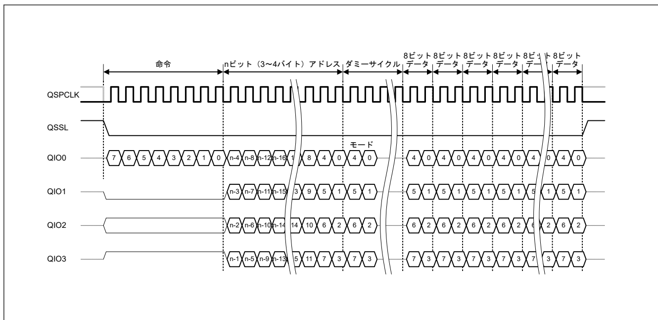
図 31.5 拡張 SPI プロトコル例 (ファストリード Quad I/O)
