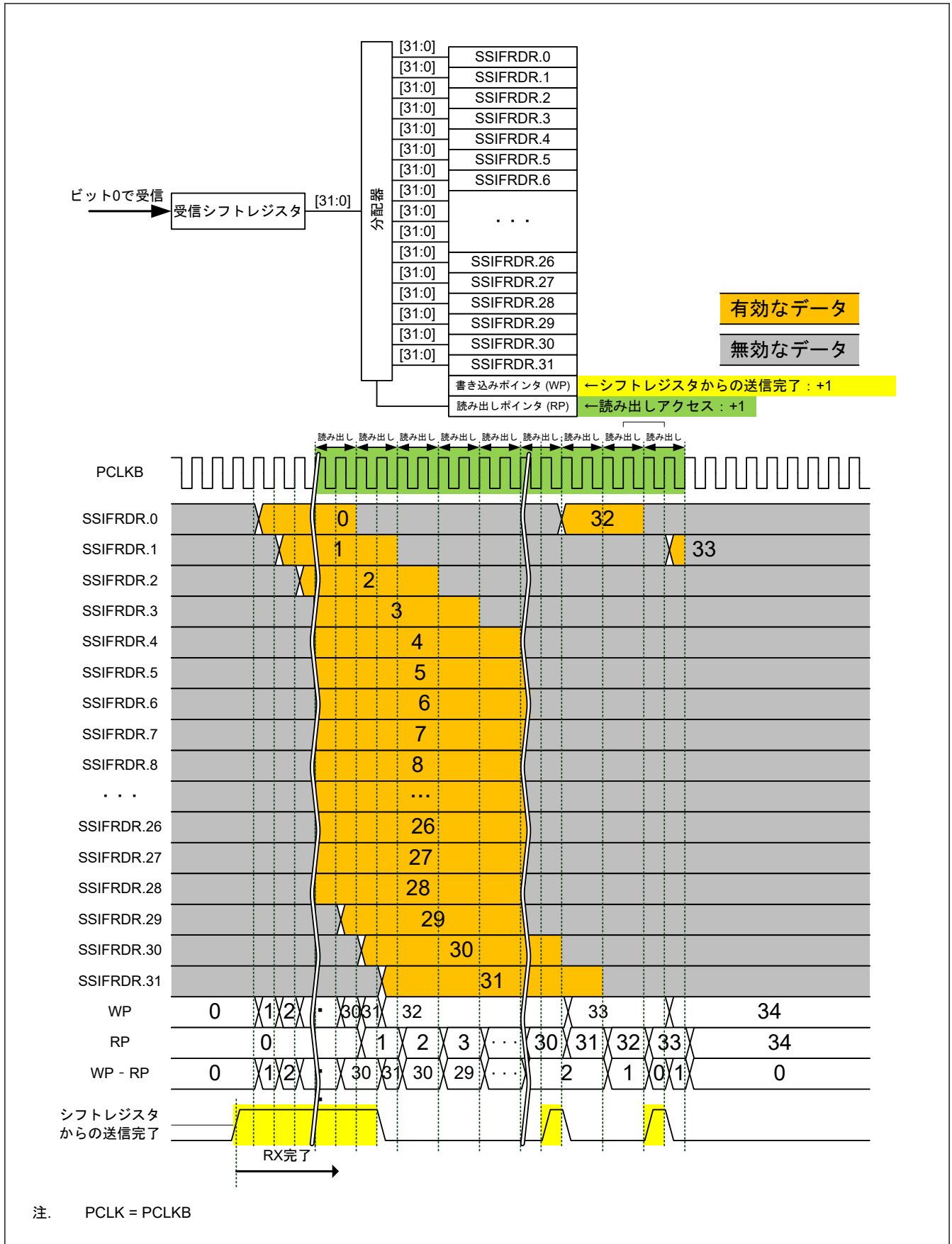
図 32.32 受信 FIFO データレジスタと受信シフトレジスタの構成、および FIFO の動作例
