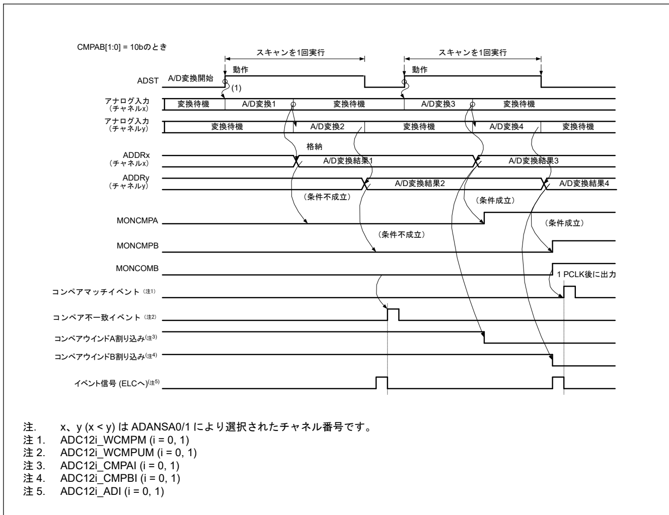
図 37.30 コンペア機能のイベント出力の動作例 (アナログ入力 (チャンネル x, y) を比較)
