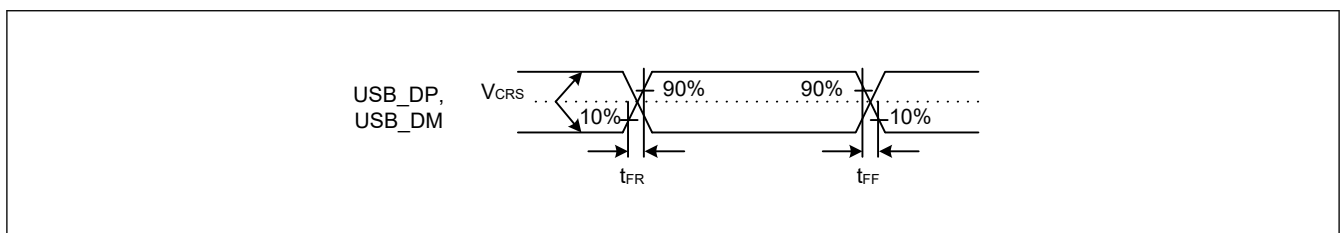
図 47.52 フルスピードモードにおける USB_DP、USB_DM の出力タイミング
