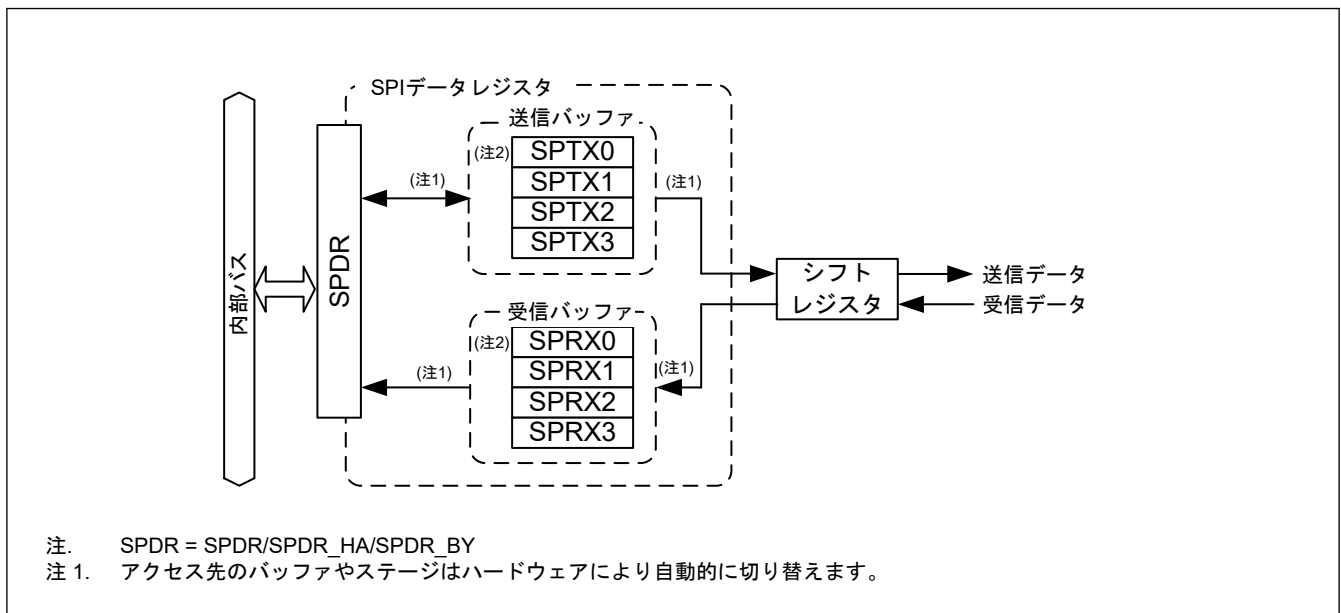
図 30.2 SPDR/SPDR_HA/SPDR_BY レジスタの構成図
