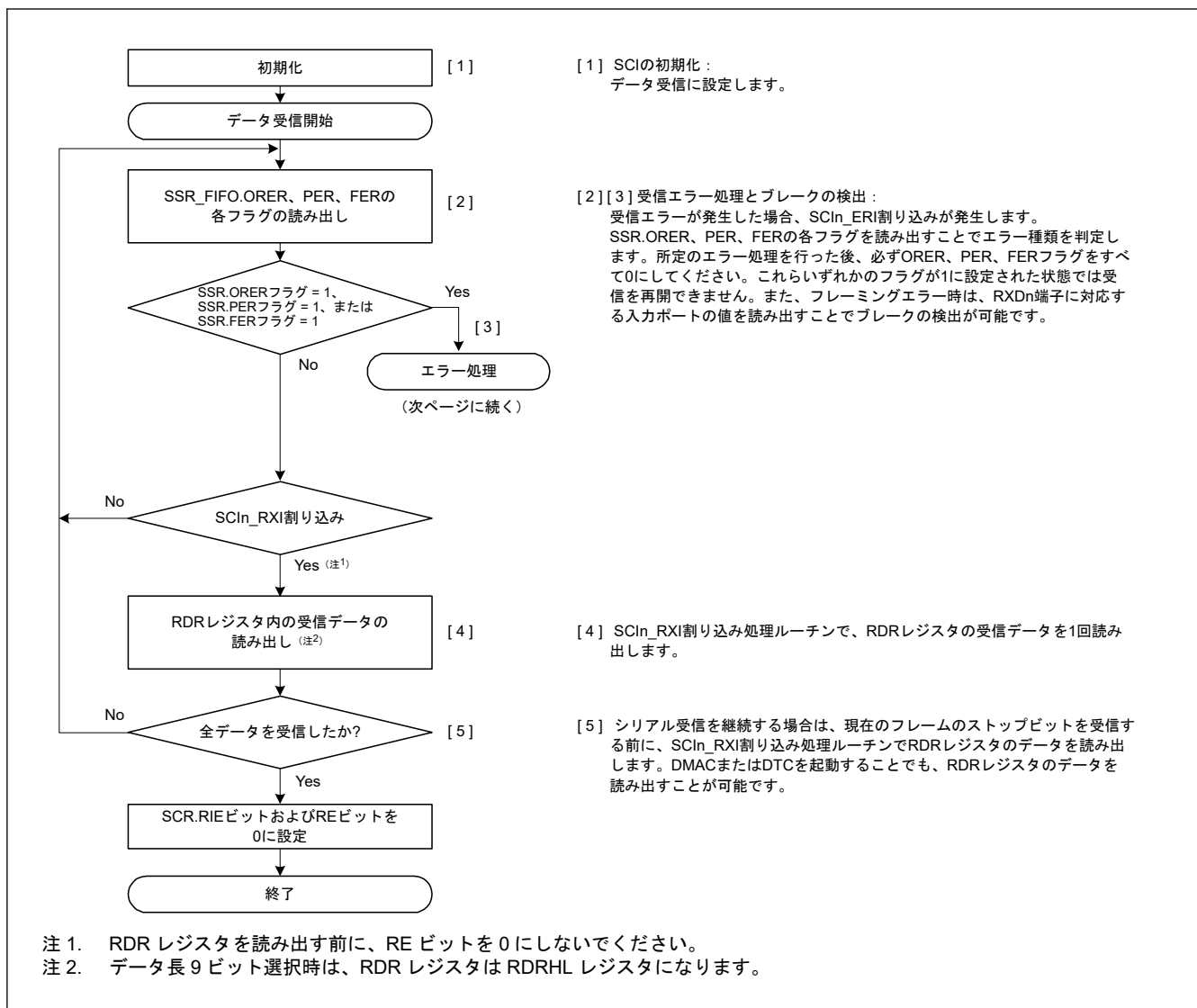
図 27.20 調歩同期式モードにおけるシリアル受信のフローチャート例（非 FIFO 選択、アドレス一致検出無効時）(1)
