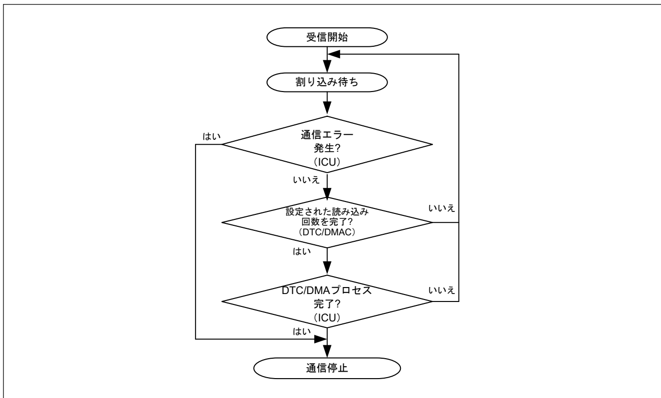
図 32.55 受信手順
