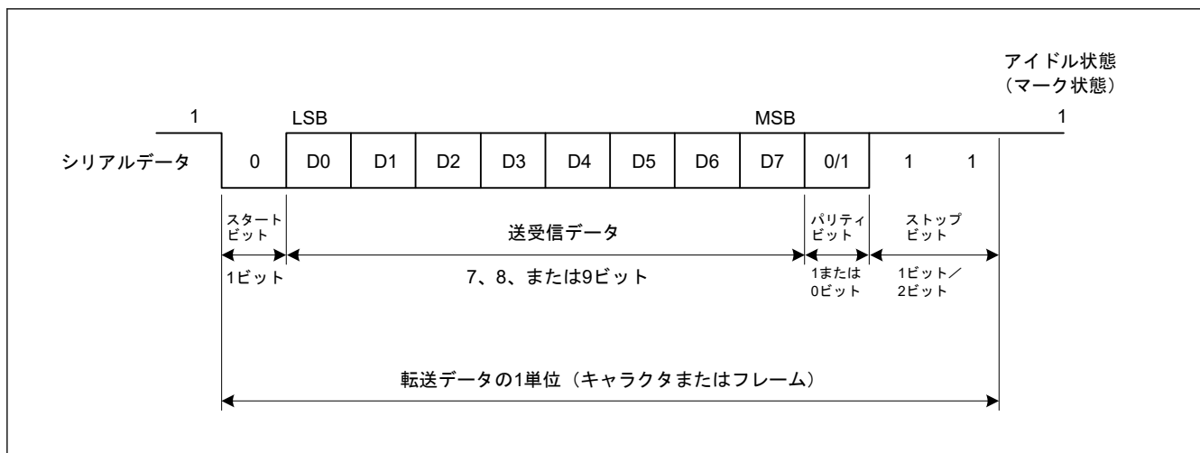
図 27.6 調歩同期式シリアル通信のデータフォーマット (8 ビットデータ/パリティあり/2 ストップビットの場合)
