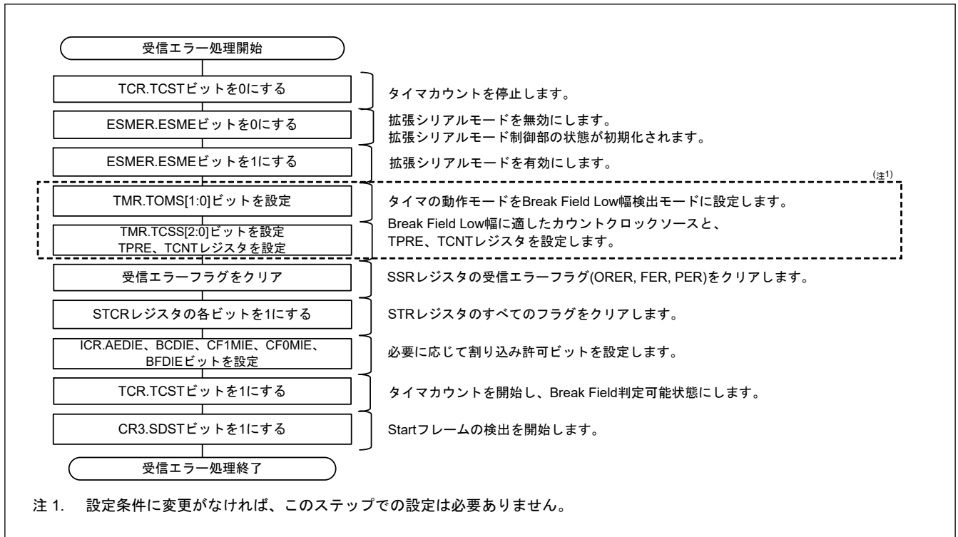
図 27.125 受信エラー処理のフローチャートの例 (スタートフレーム受信時)
