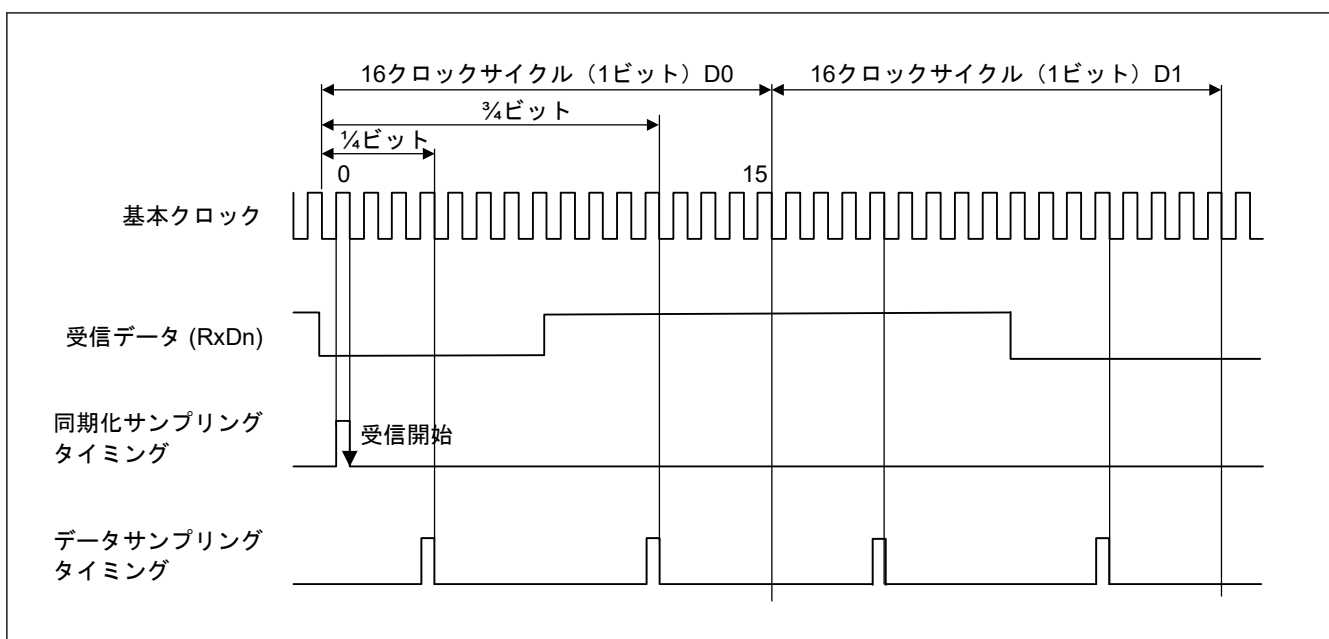
図 27.59 マンチェスタモードでのデータ受信サンプリングタイミング
