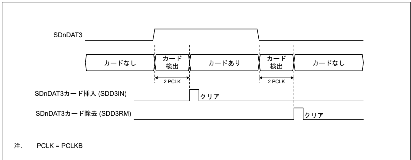
図 33.8 SDnDAT3 による SD カード検出
