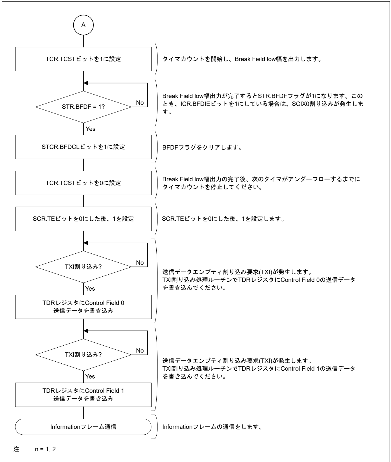
図 27.104 Start Frame 送信フローチャート例 (2/2)
