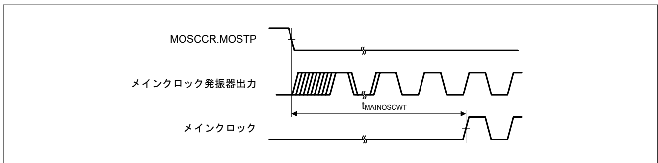
図 47.8 メインクロック発振開始タイミング
