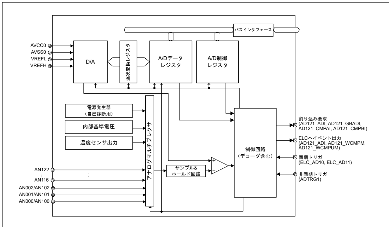
図 37.2 ADC12 のブロック図 (ユニット 1)
