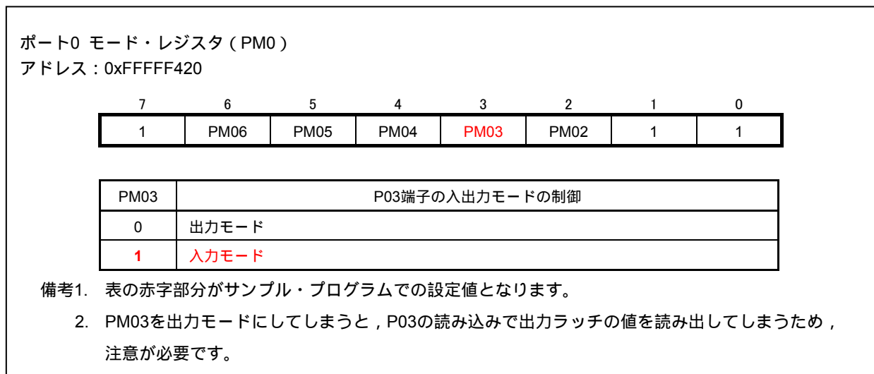
図4 - 1 PM0レジスタのフォーマット
