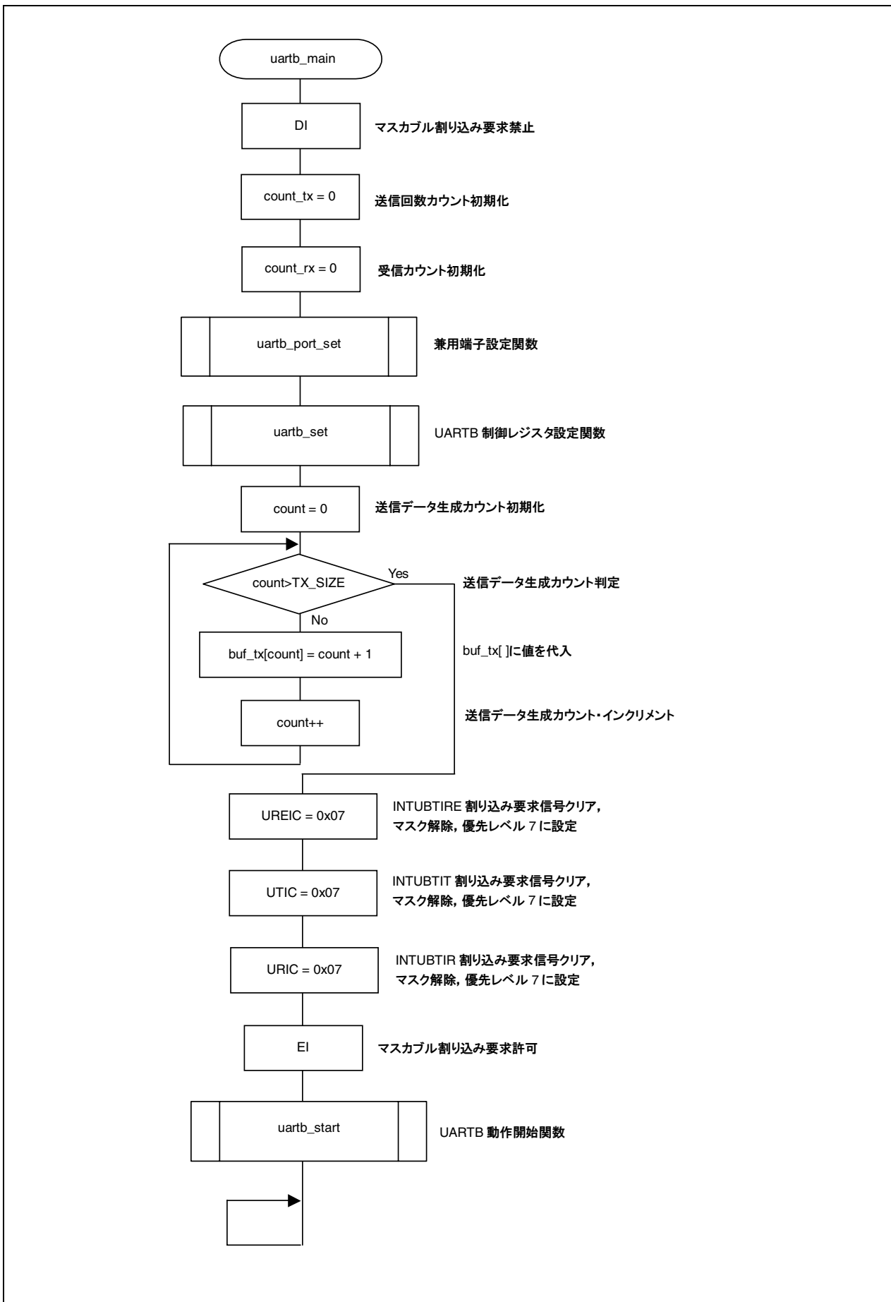
図2 - 1 FIFOモード (1/4)
