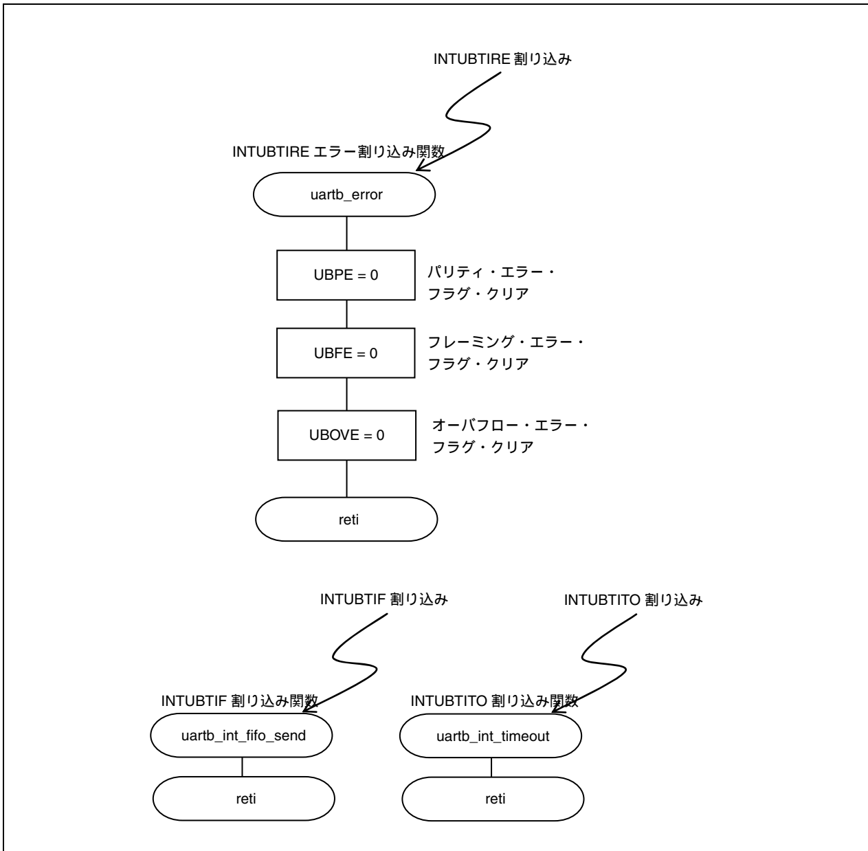
図2 - 1 FIFOモード (4/4)
