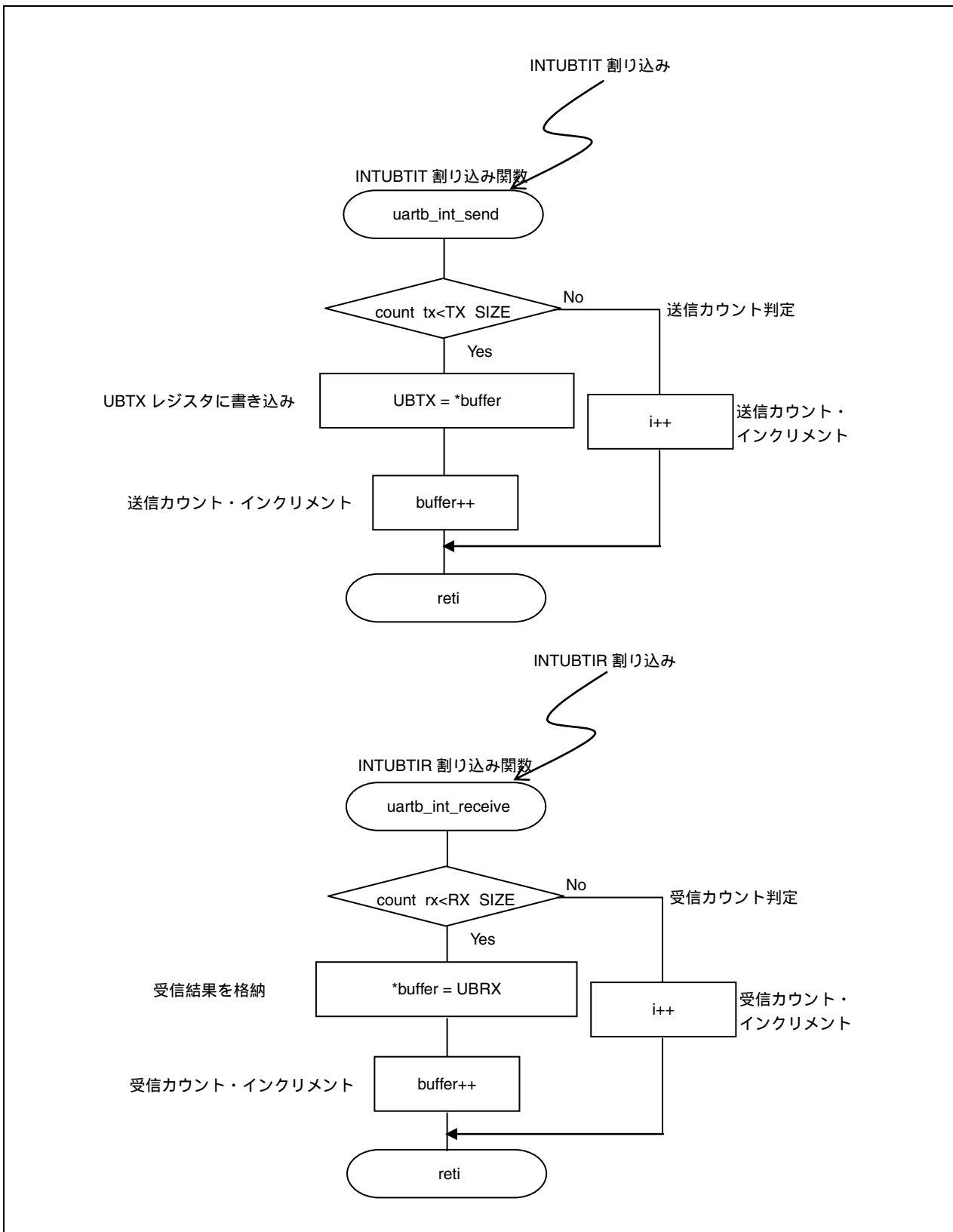
図2 - 1 FIFOモード (3/4)
