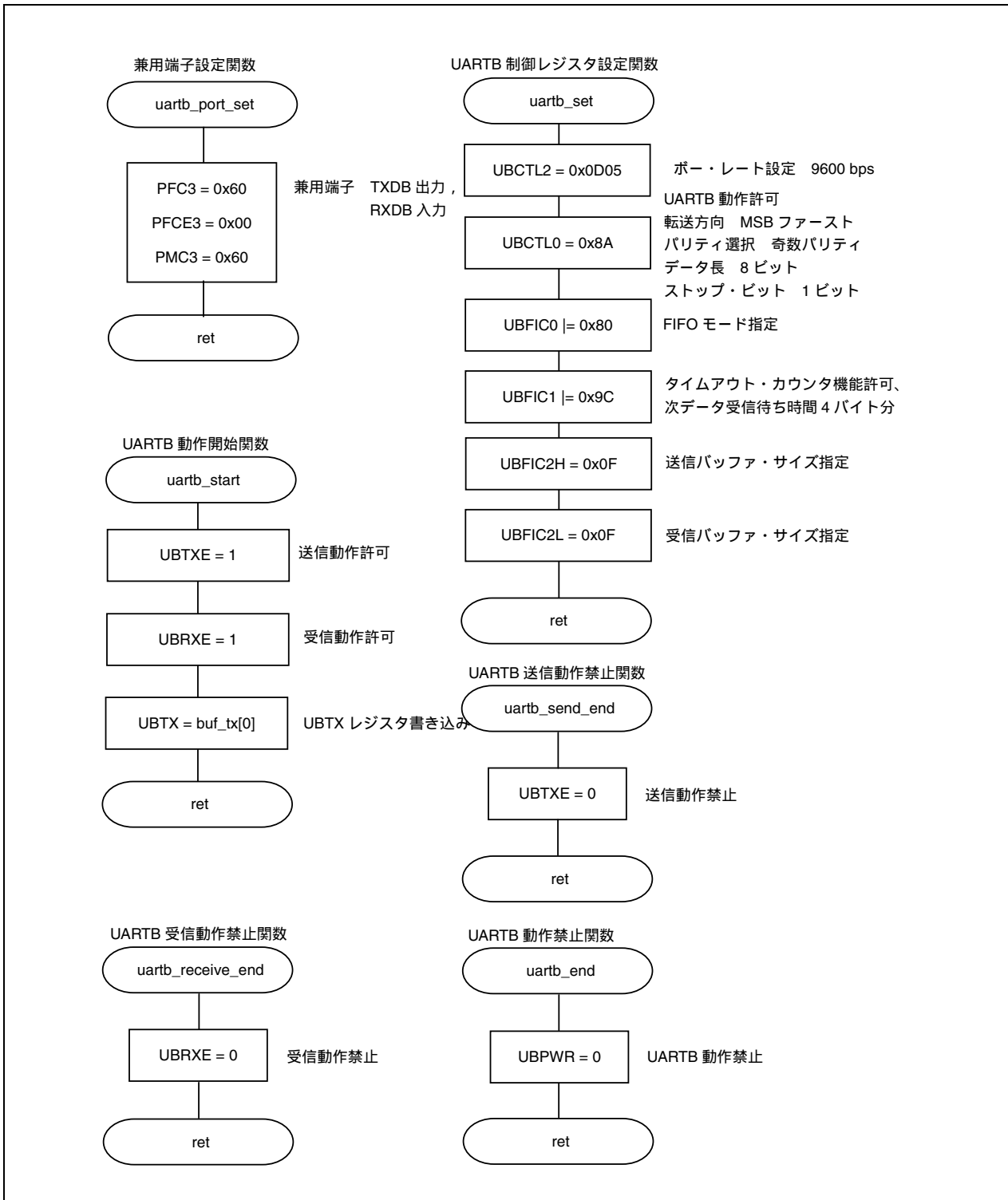
図2 - 1 FIFOモード (2/4)
