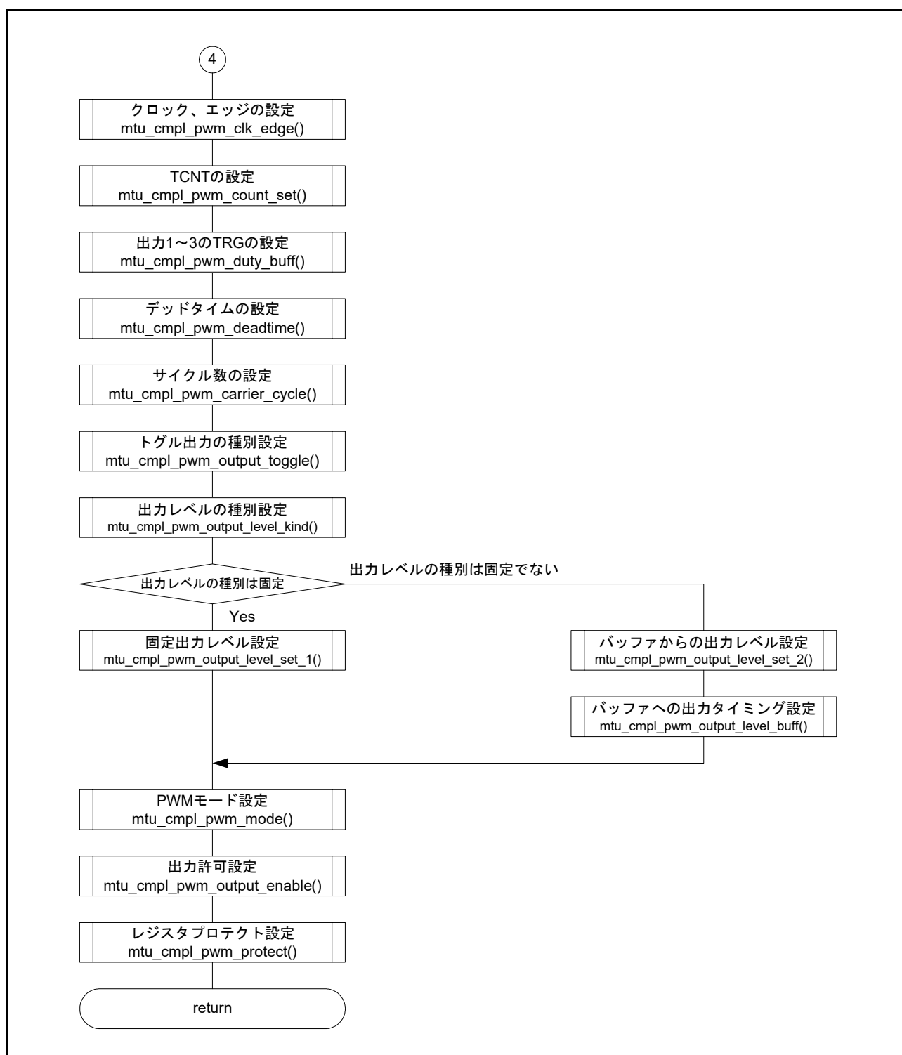
図 6.21 相補 PWM モード終了処理 (5)
