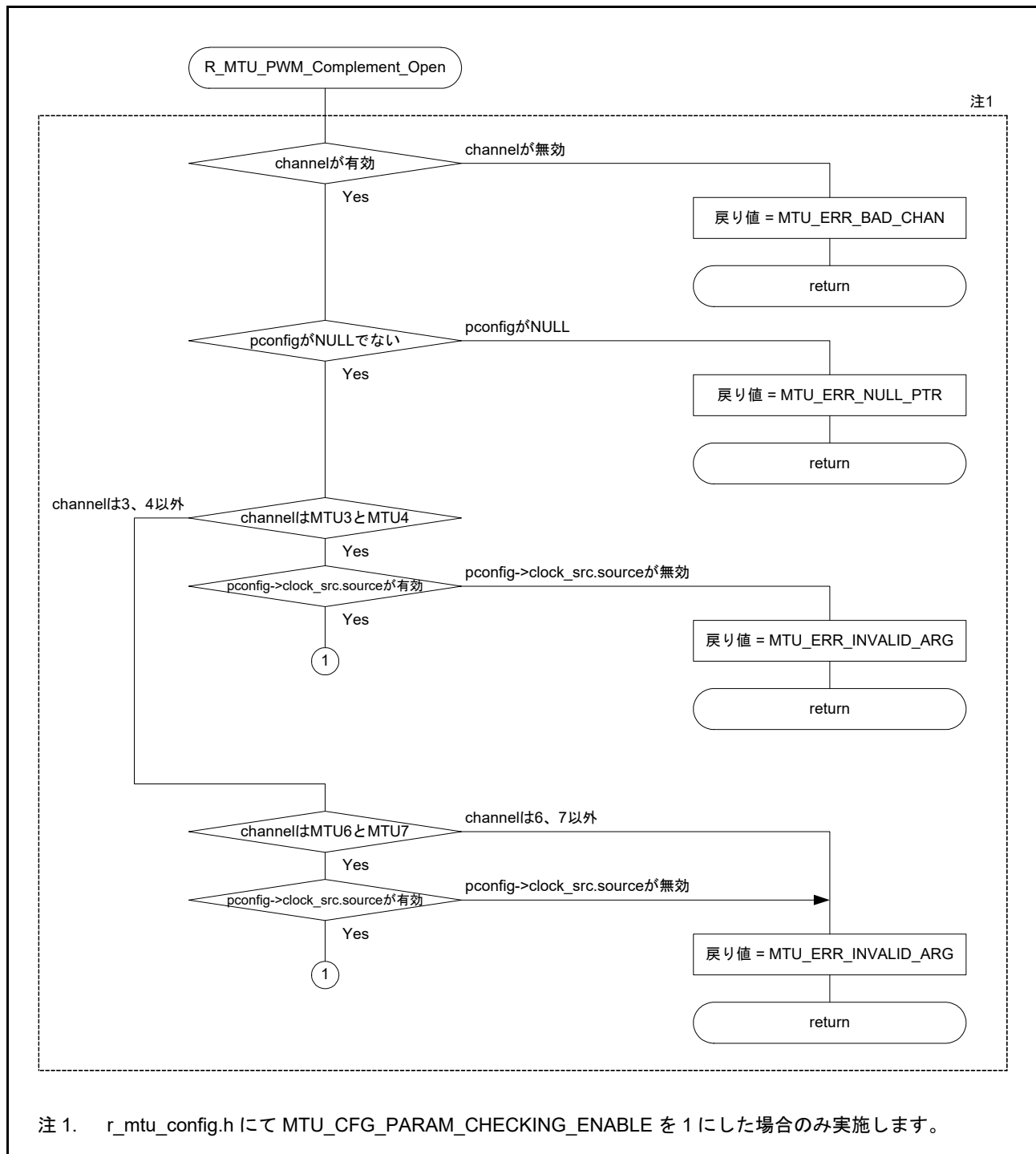
図 6.17 相補 PWM モード設定処理 (1)
