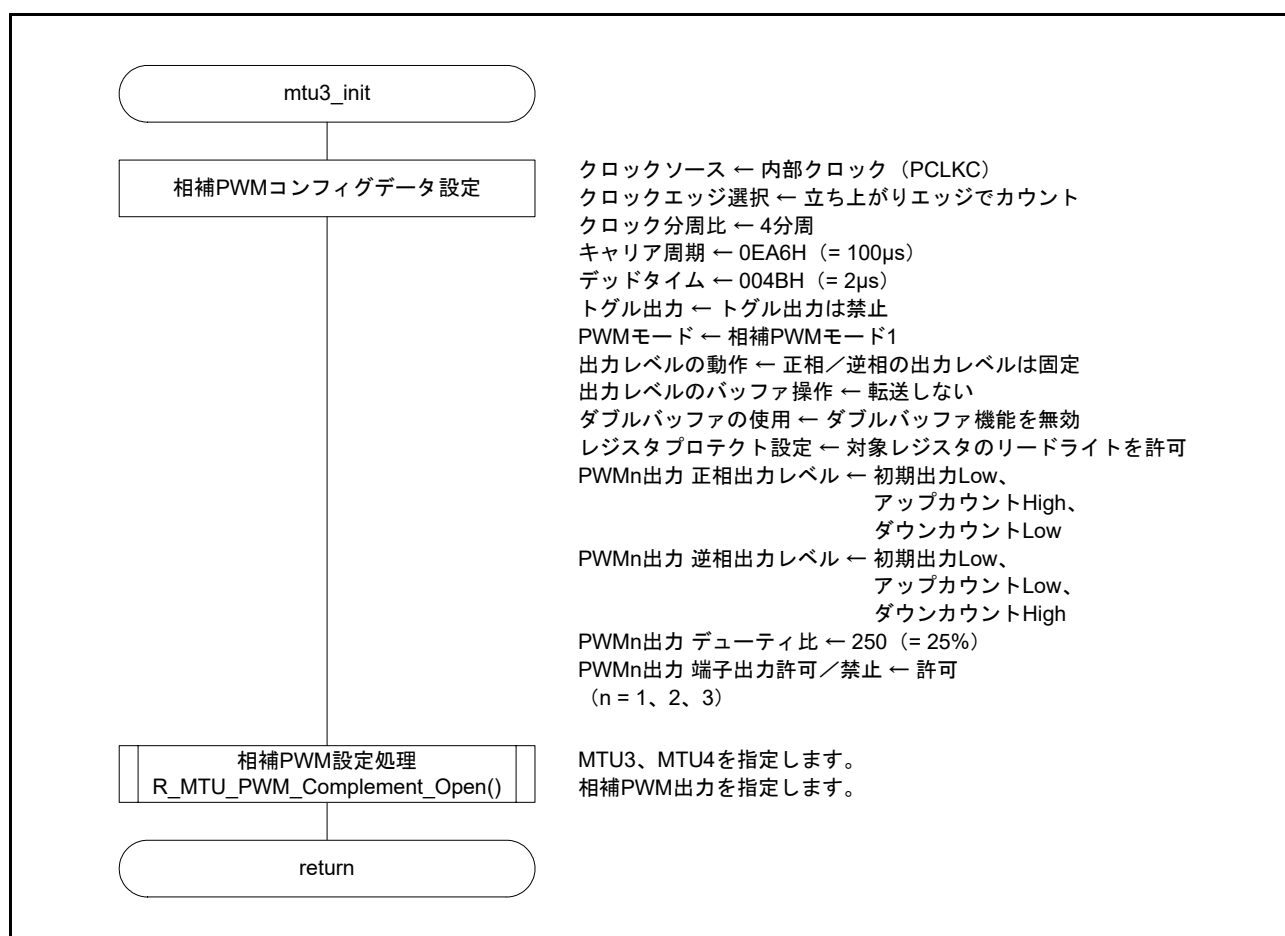
图 6.16 MTU 初期化处理
