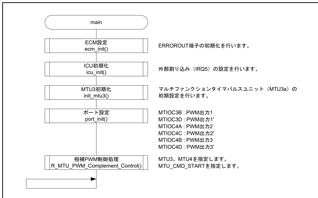
図 6.15 メイン処理
