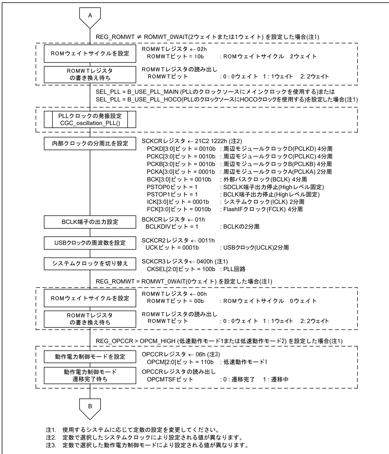
図 3.5 クロック初期設定(2/3)
