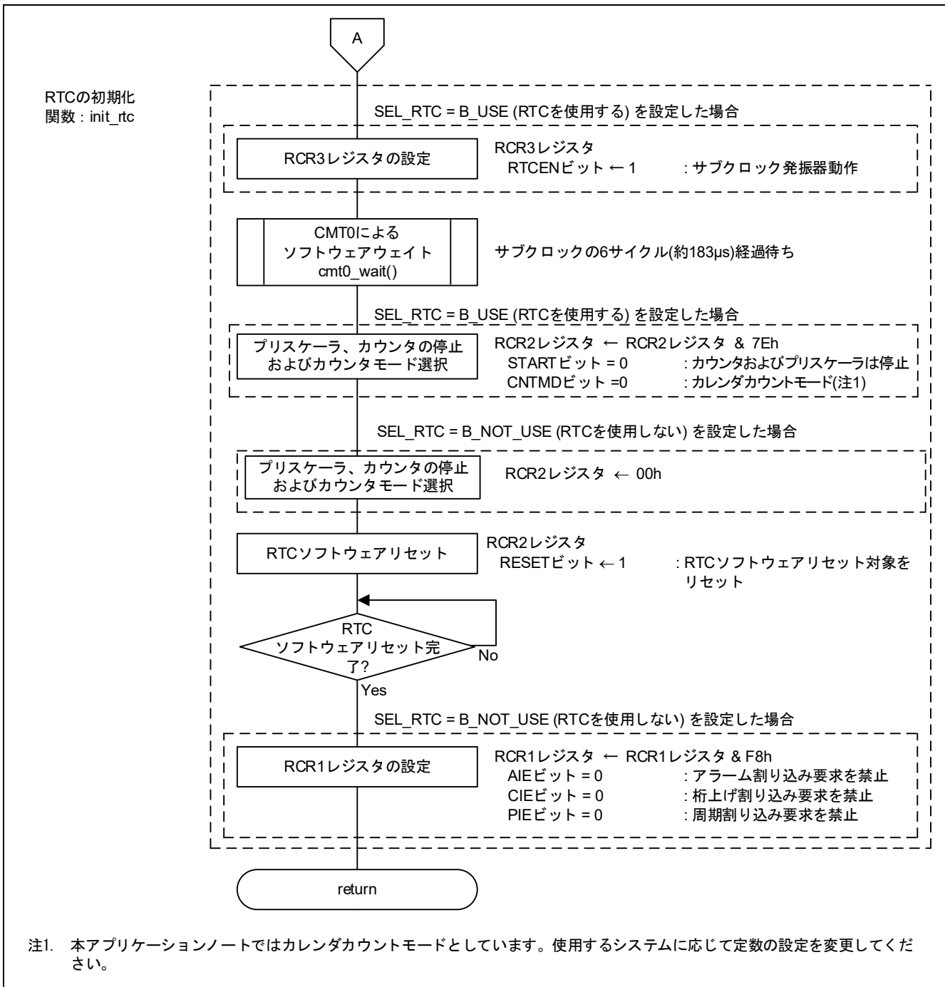
図 3.11 サブクロックの発振設定(2/2)
