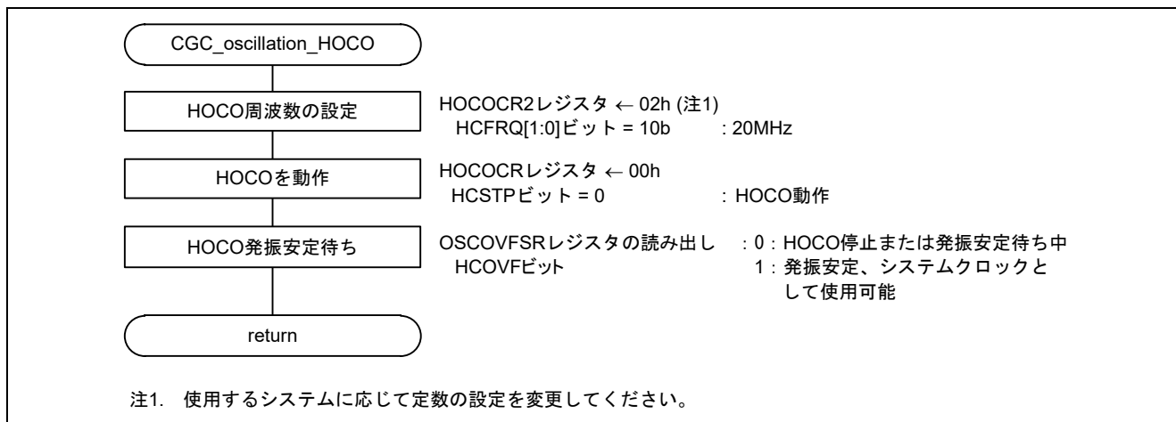
図 3.9 HOCO クロックの発振設定
