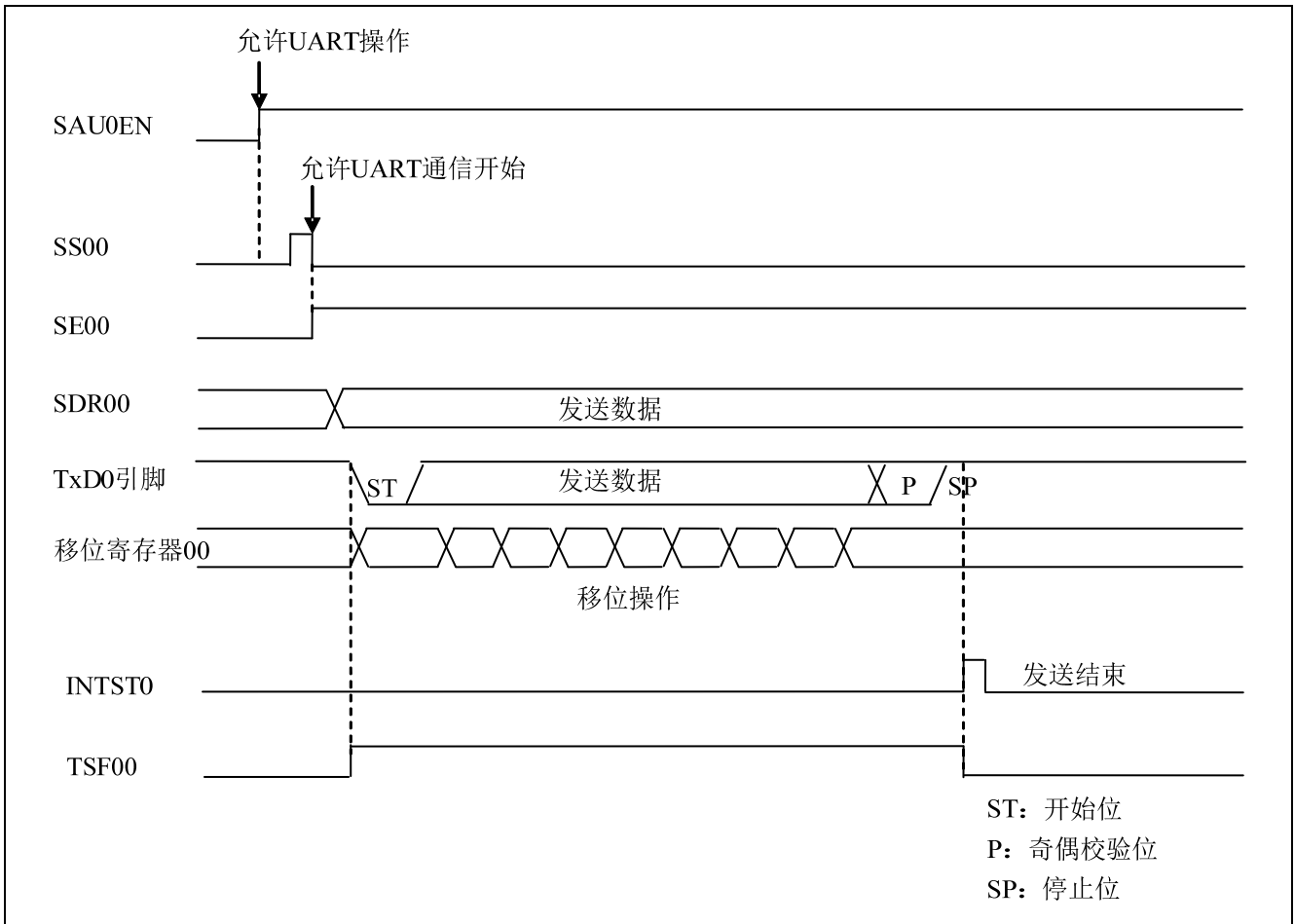
图 1.2 UART 发送时序图
