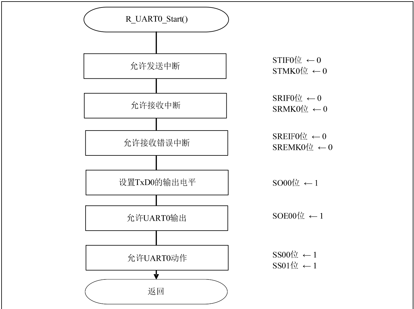
图 5.13 UART0 动作开始处理
