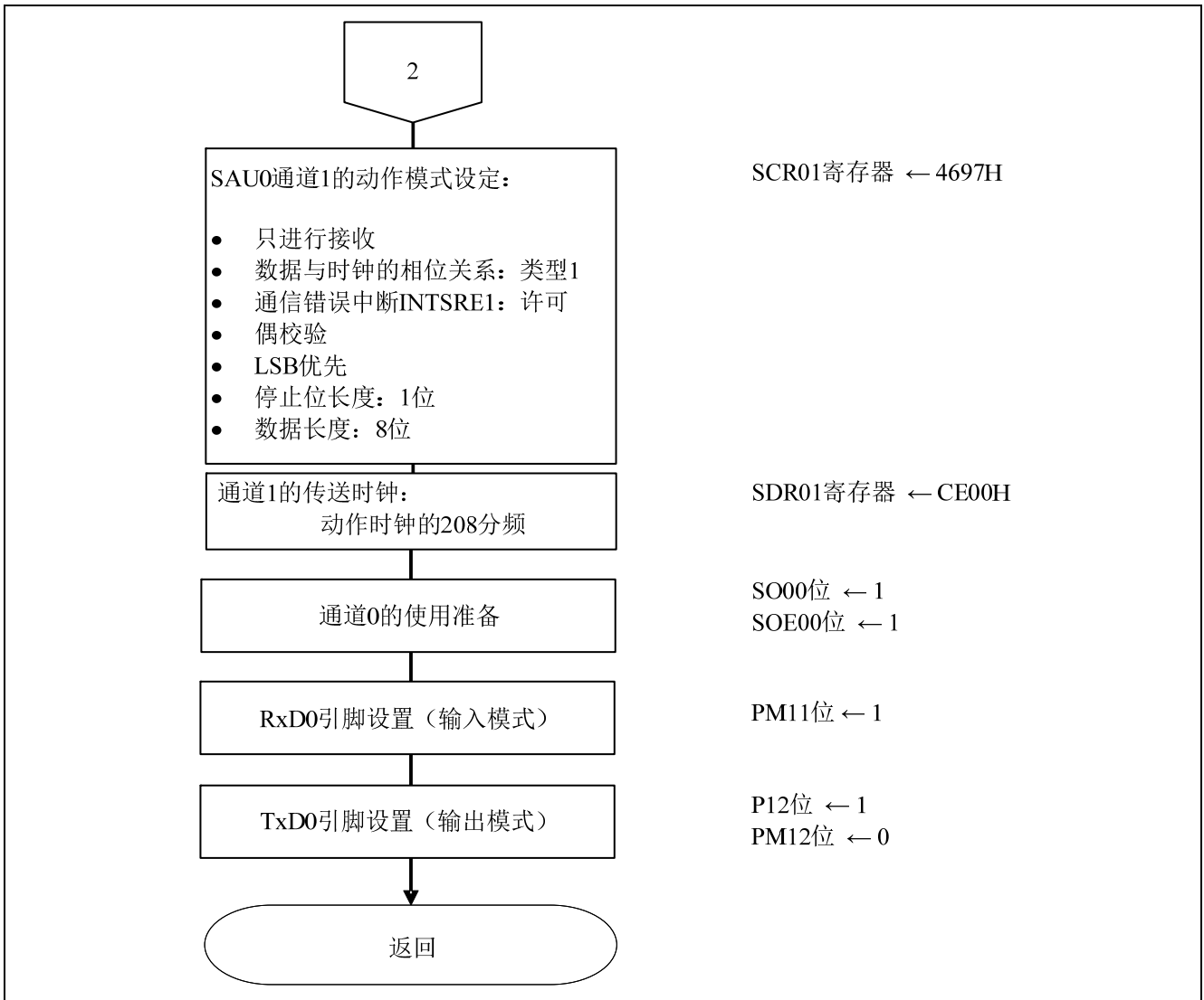
图 5.9 UART0 的设置 (3/3)
