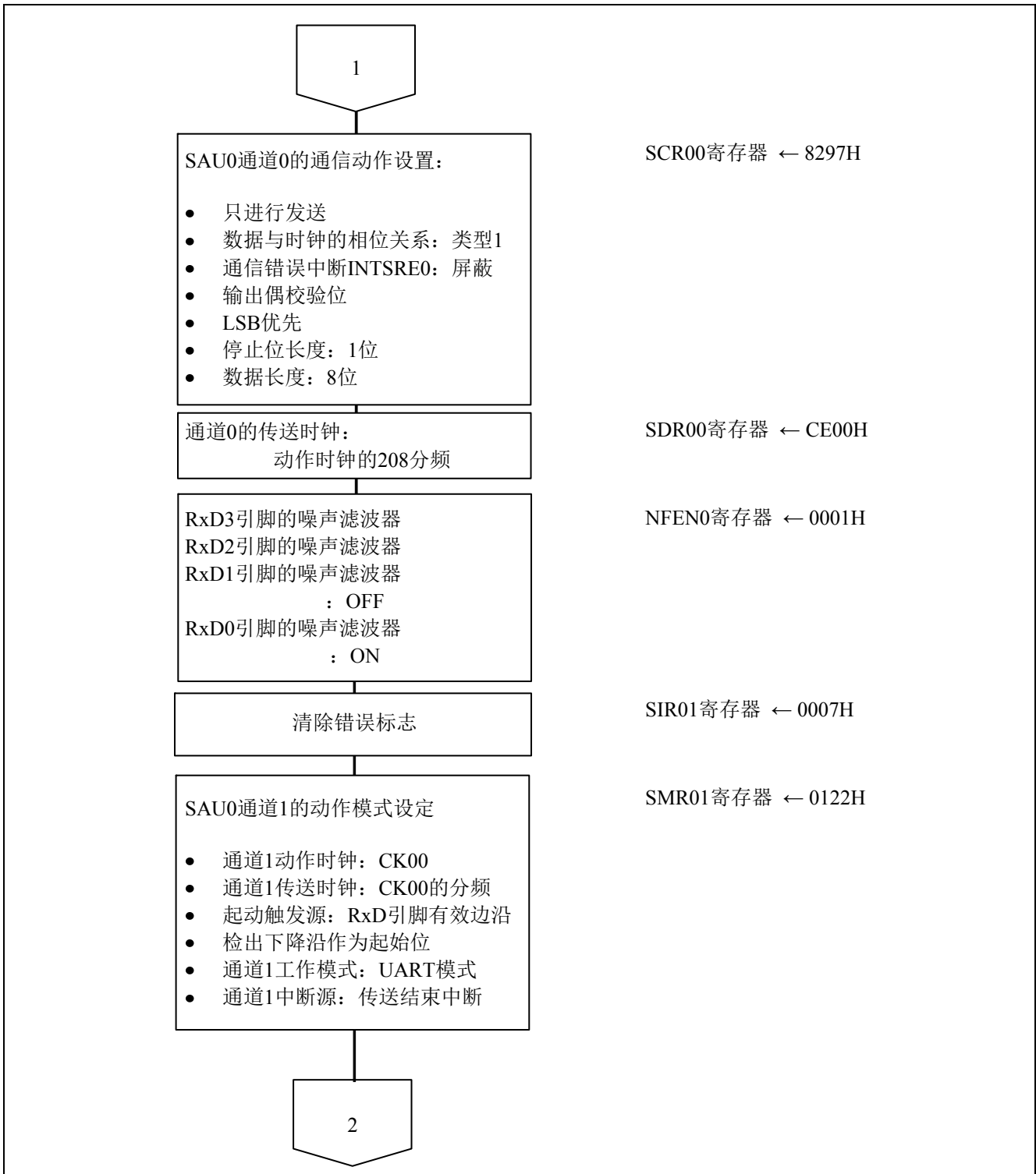
图 5.8 UART0 的设置 (2/3)
