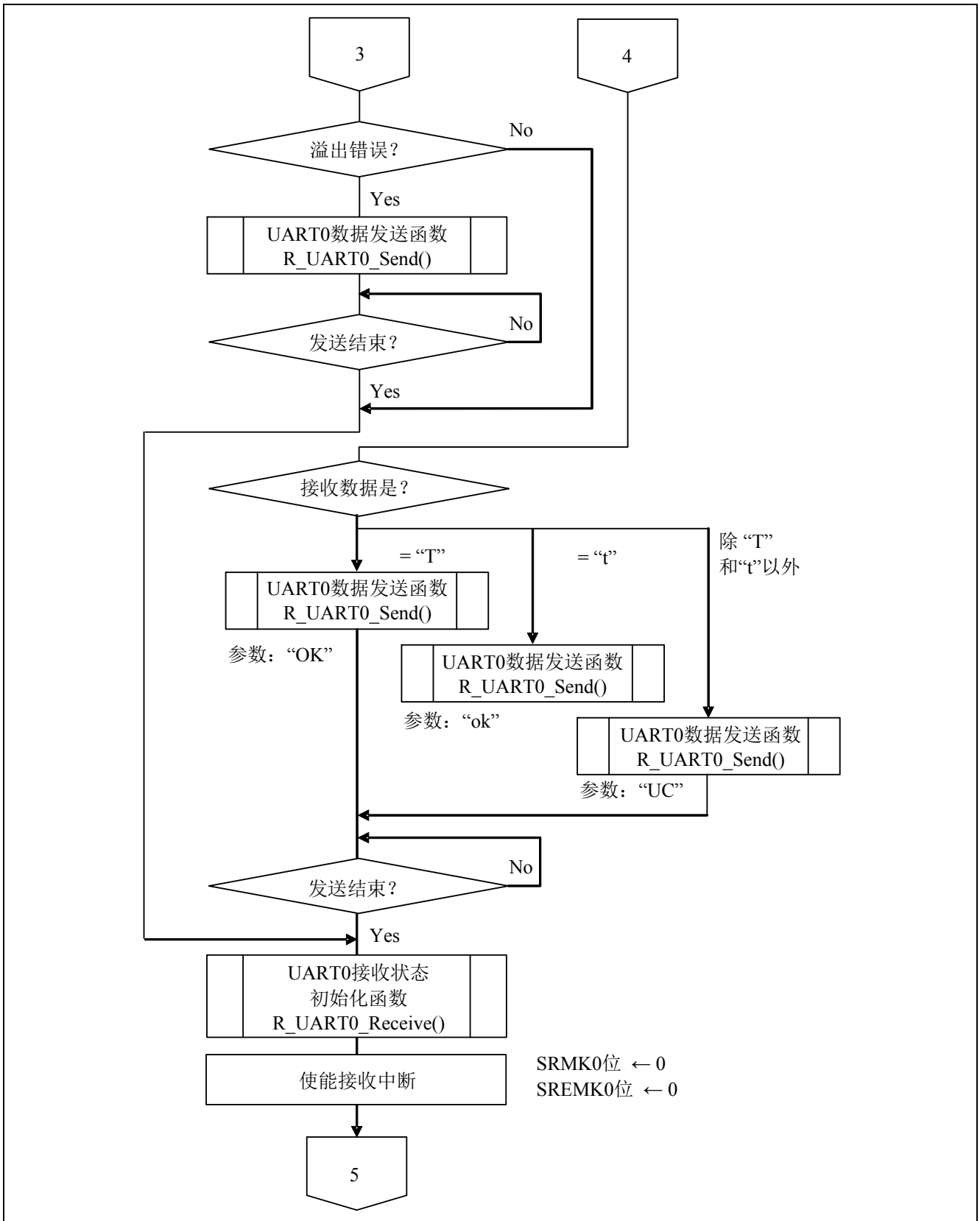
图 5.11 主函数处理 (2/2)
