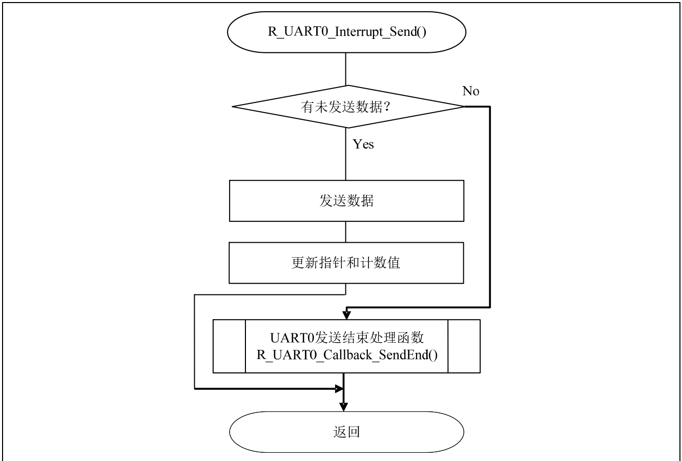
图 5.19 INTST0 中断处理函数
