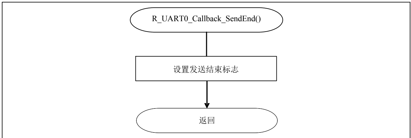
图 5.20 UART0 发送结束处理函数
