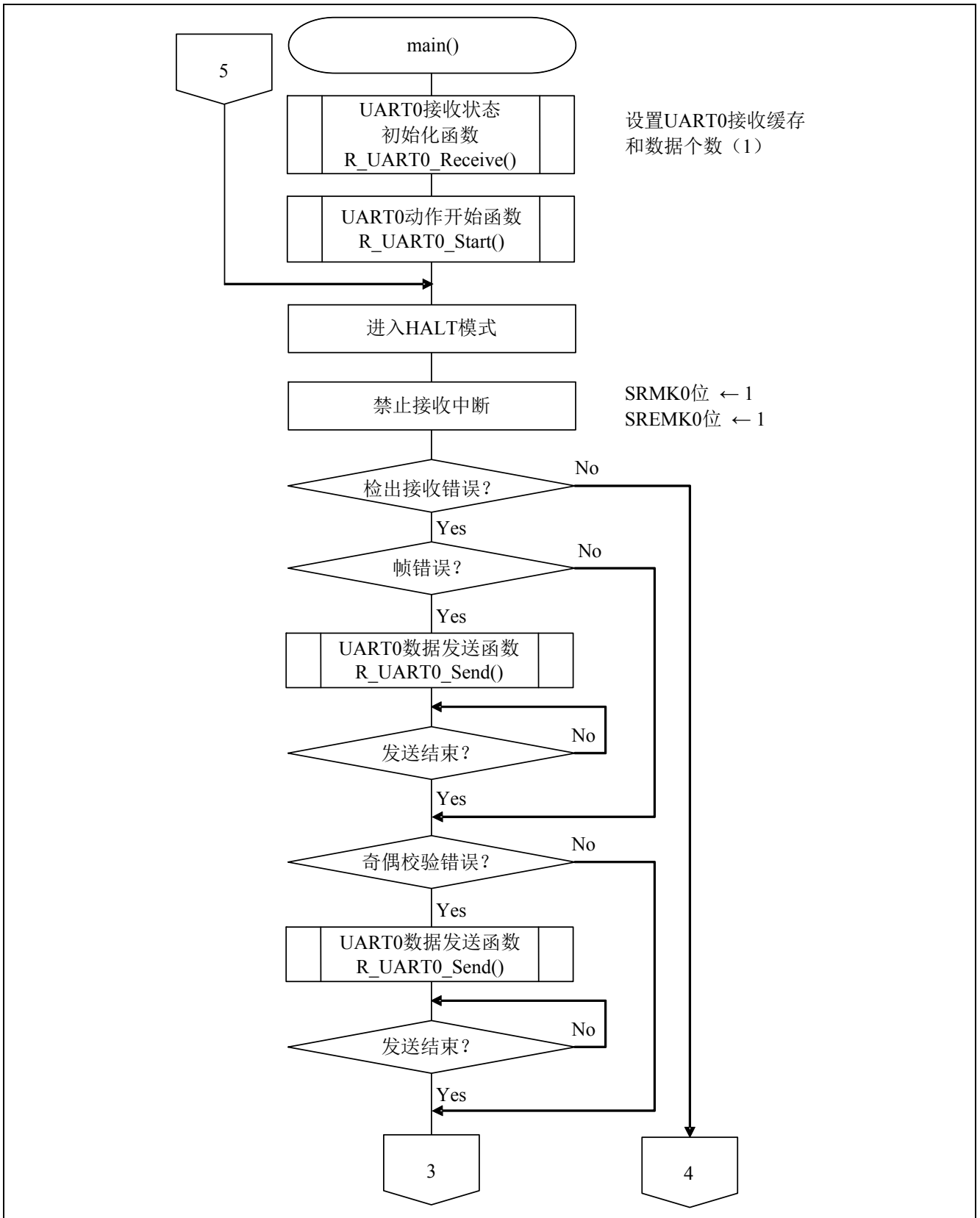
图 5.10 主函数处理 (1/2)
