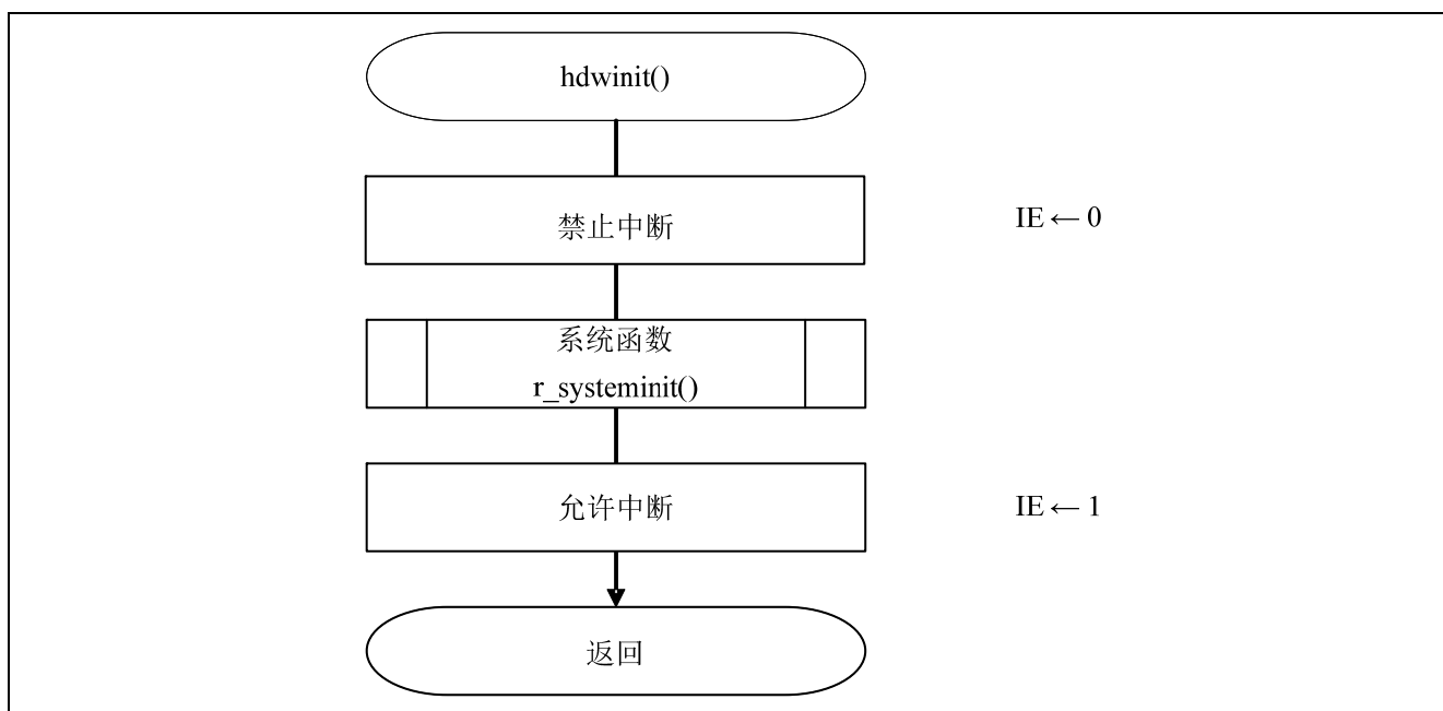
图 5.2 初始化函数
