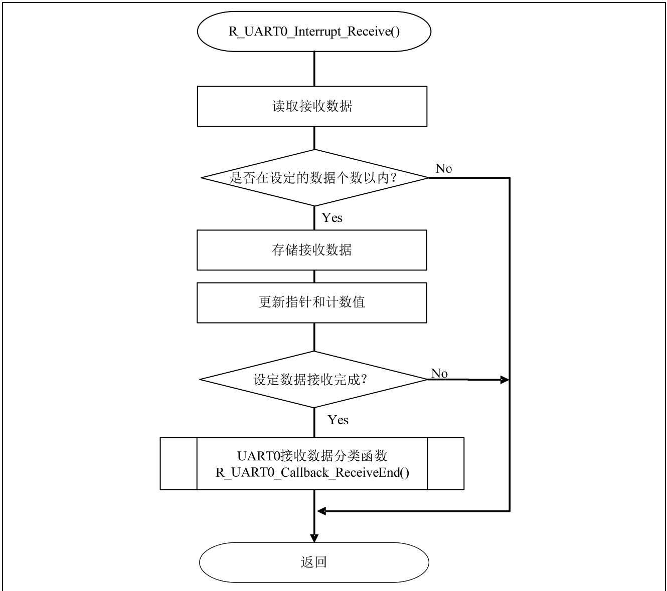
图 5.14 INTSR0 中断处理函数
