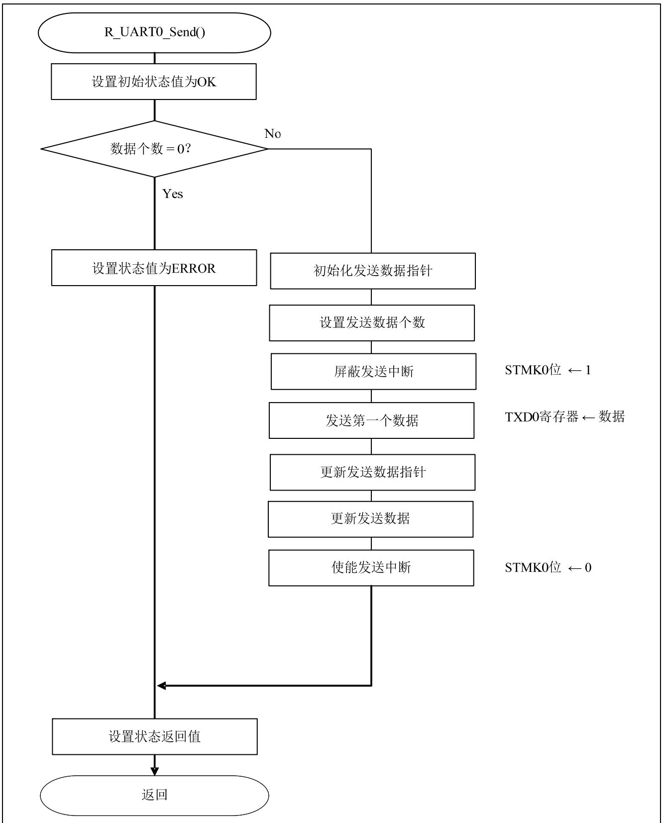
图 5.15 UART0 数据发送函数
