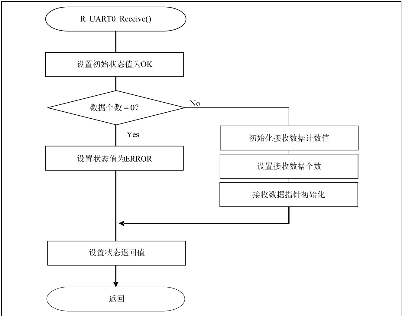
图 5.12 UART0 接收状态初始化函数
