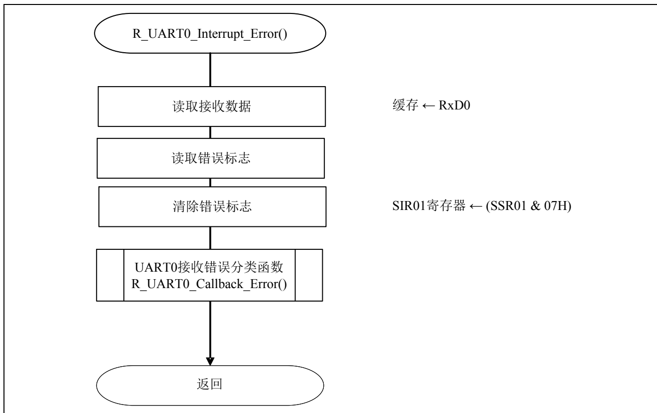
图 5.17 UART0 接收错误中断函数
