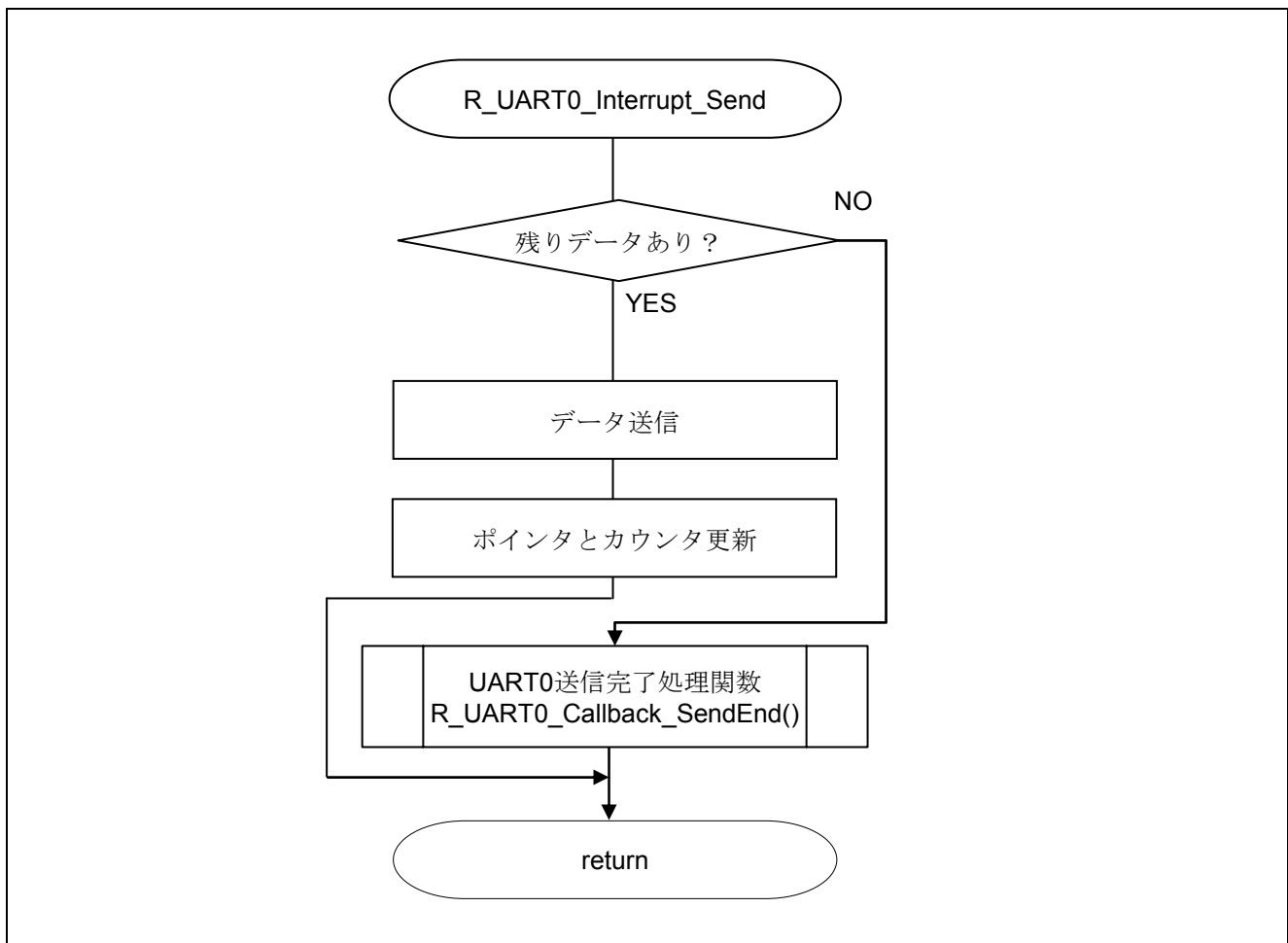
図 5.19 INTST0 割り込みサービスルーチン
