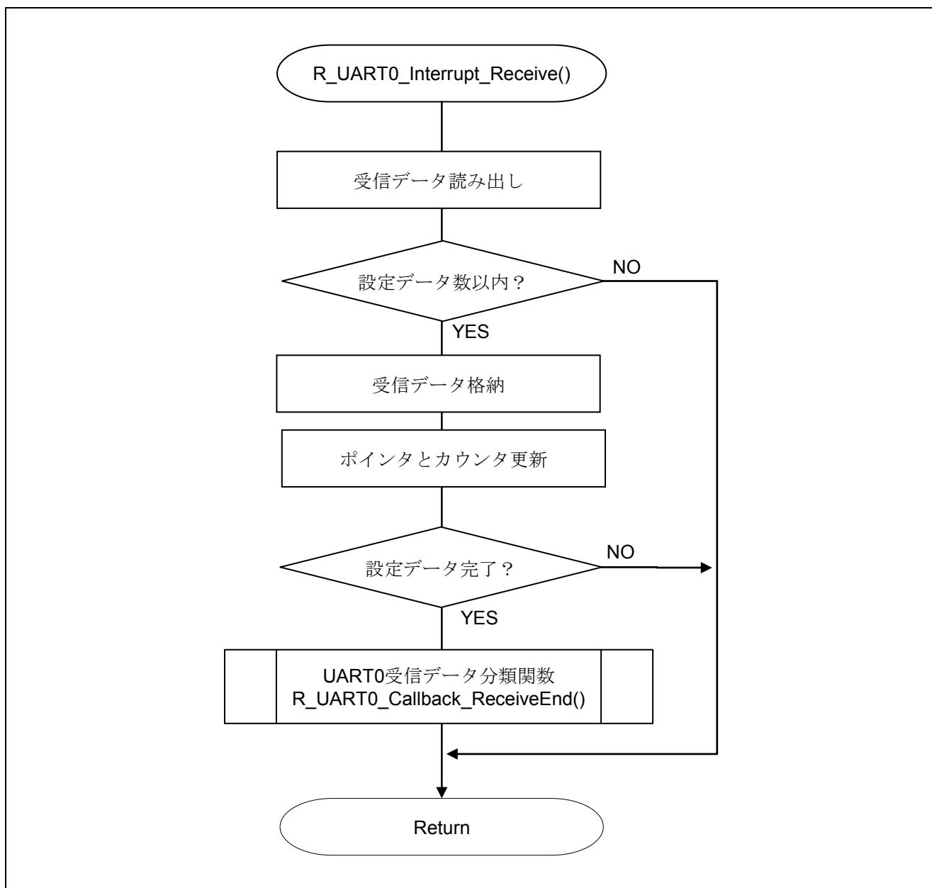
図 5.14 INTSR0 割り込みサービスルーチン
