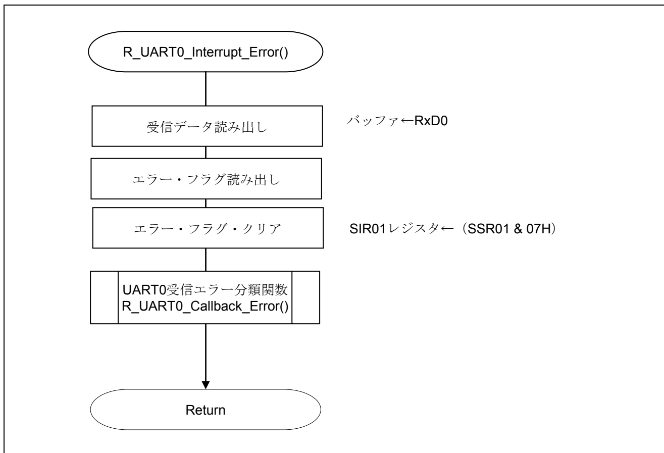
図 5.17 UART0 受信エラー割り込み関数
