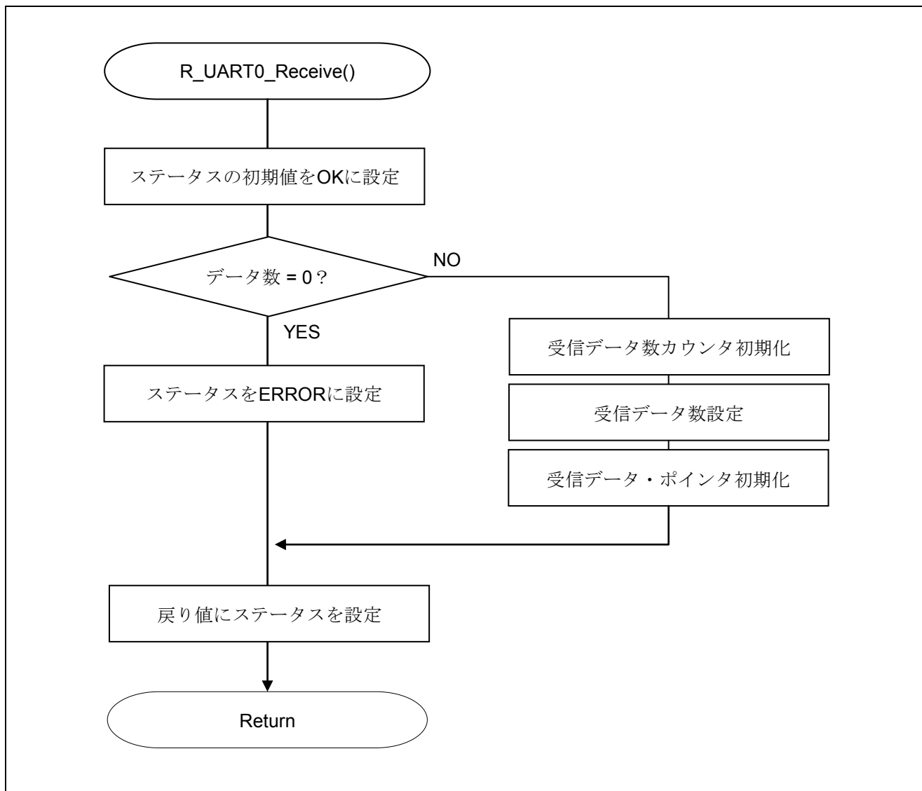
図 5.12 UART0 受信ステータス初期化関数
