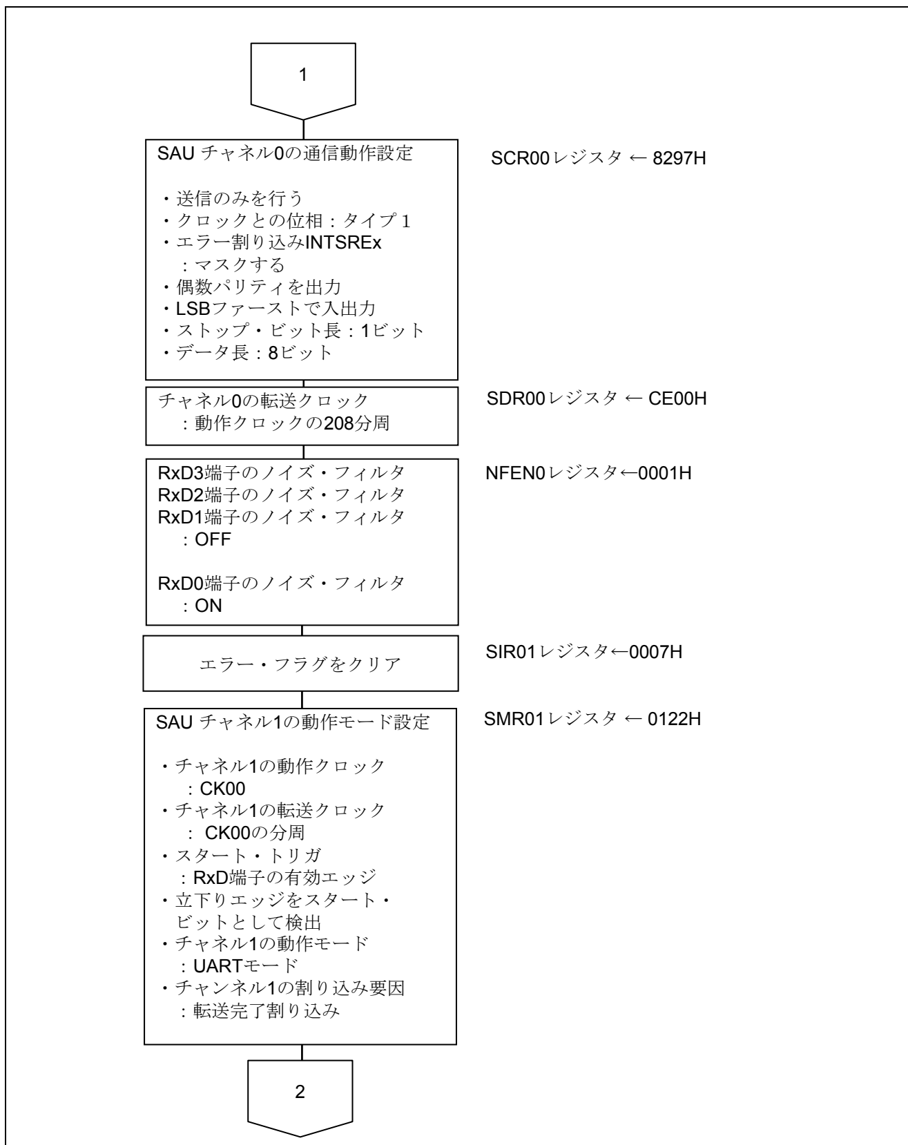
図 5.8 UART0 の設定 (2/3)
