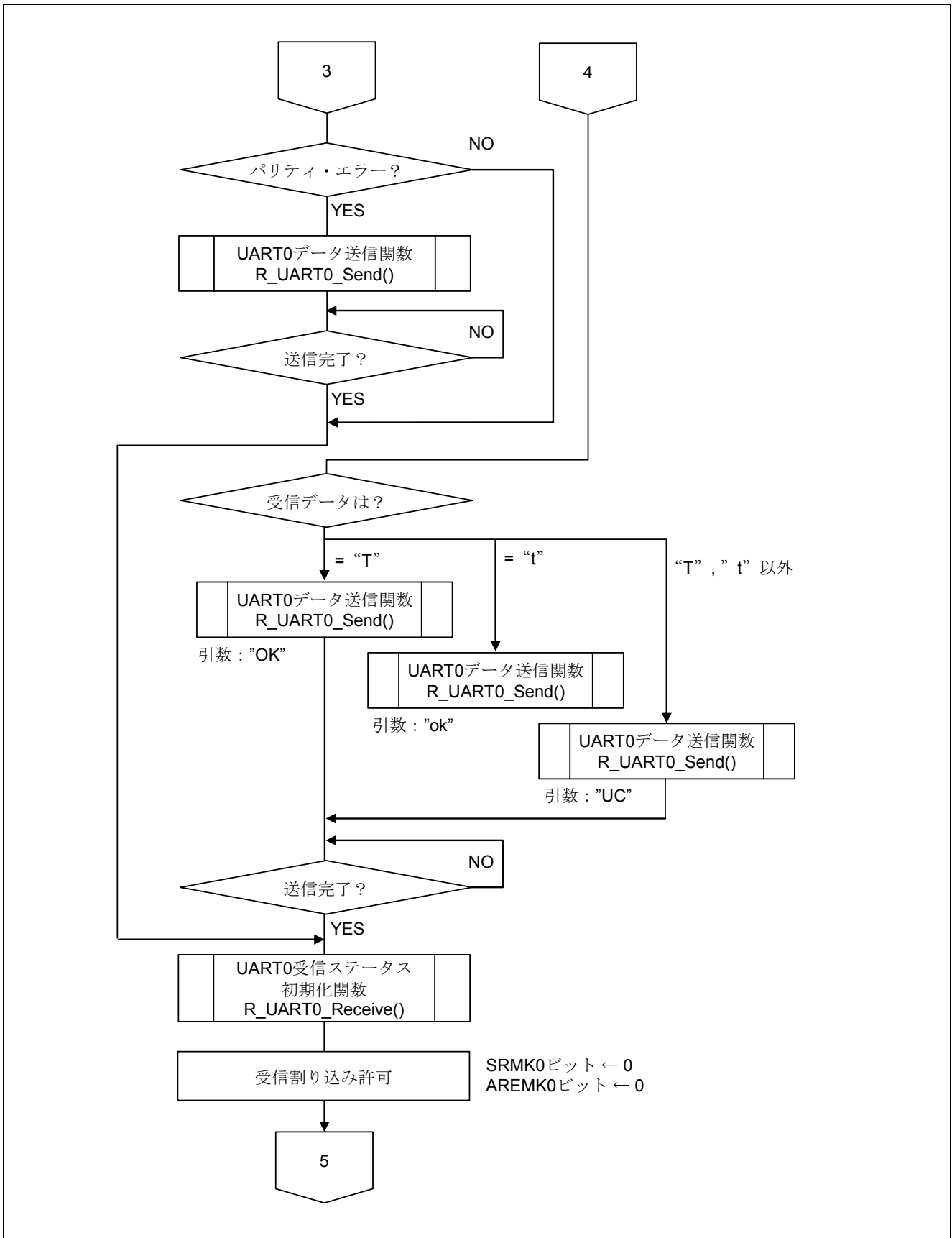
図 5.11 メイン関数 (2/2)
