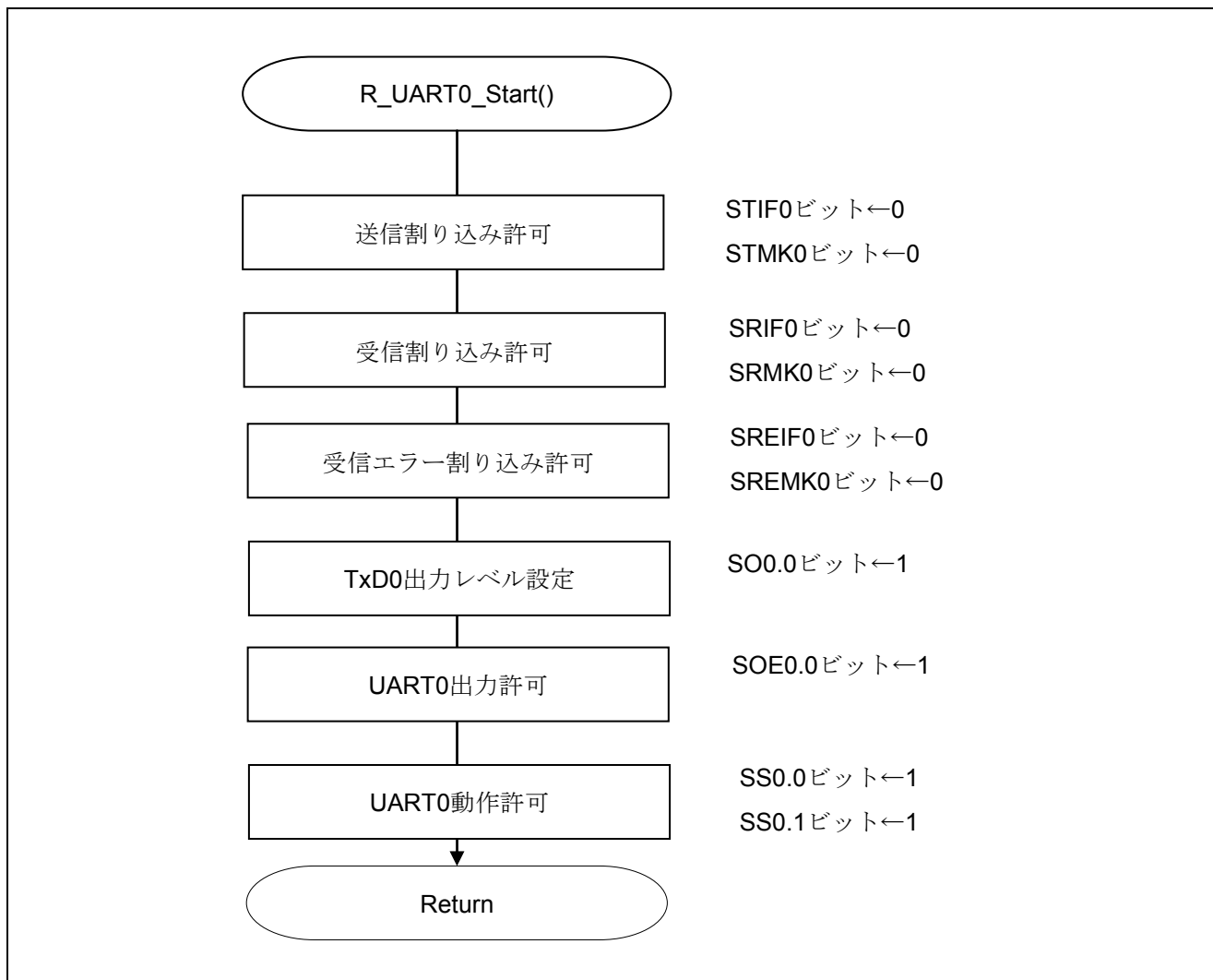
図 5.13 UART0 動作開始関数
