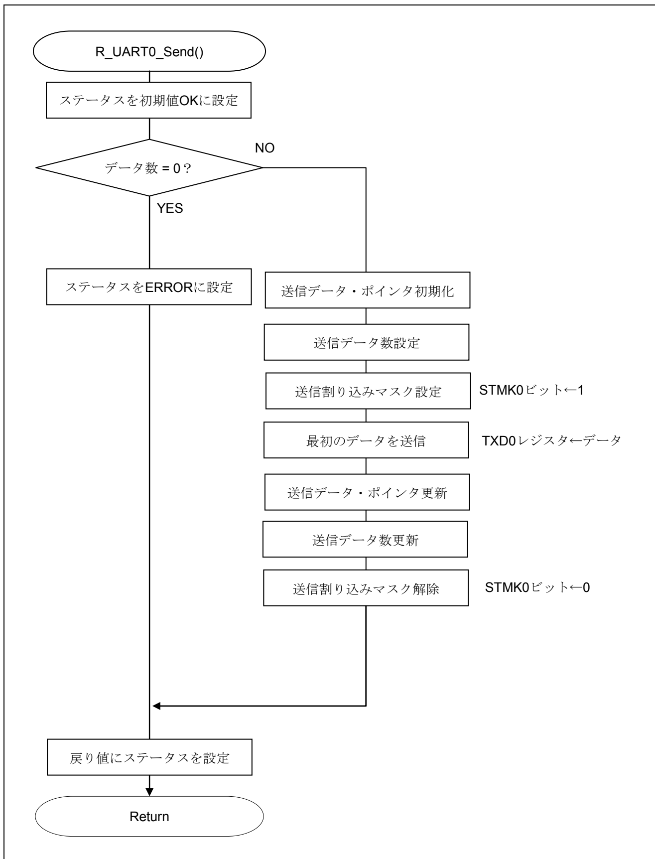
図 5.16 UART0 データ送信関数
