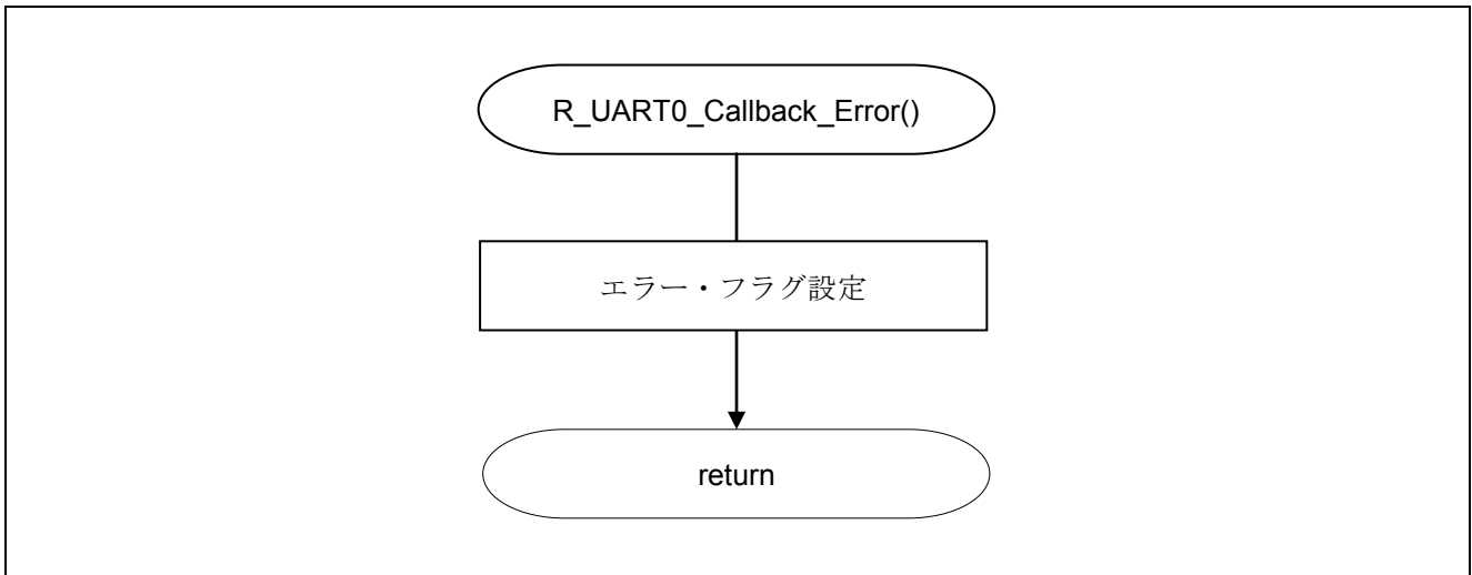
図 5.18 UART0 受信エラー分類関数
