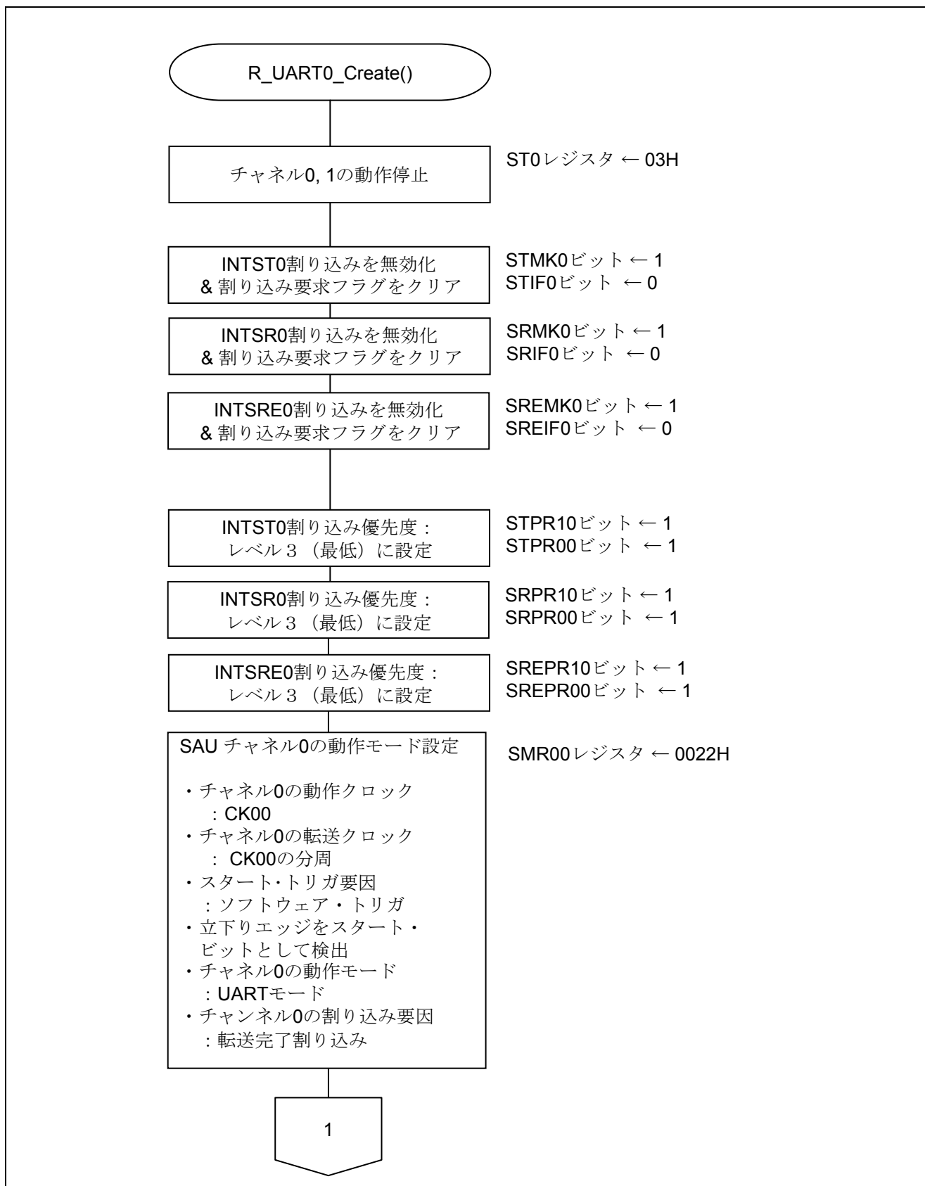
図 5.7 UART0 の設定 (1/3)
