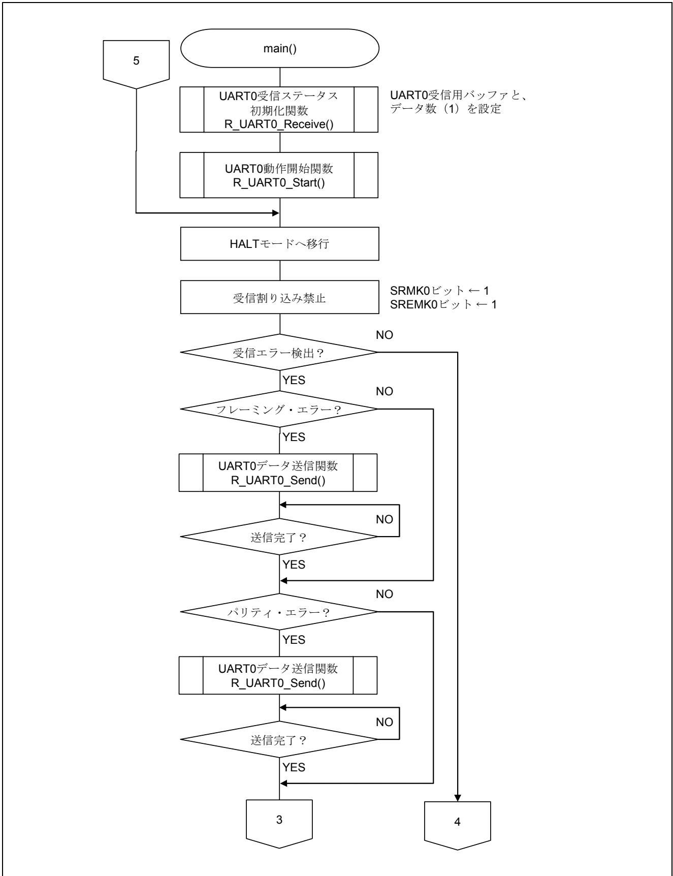
図 5.10 メイン関数 (1/2)
