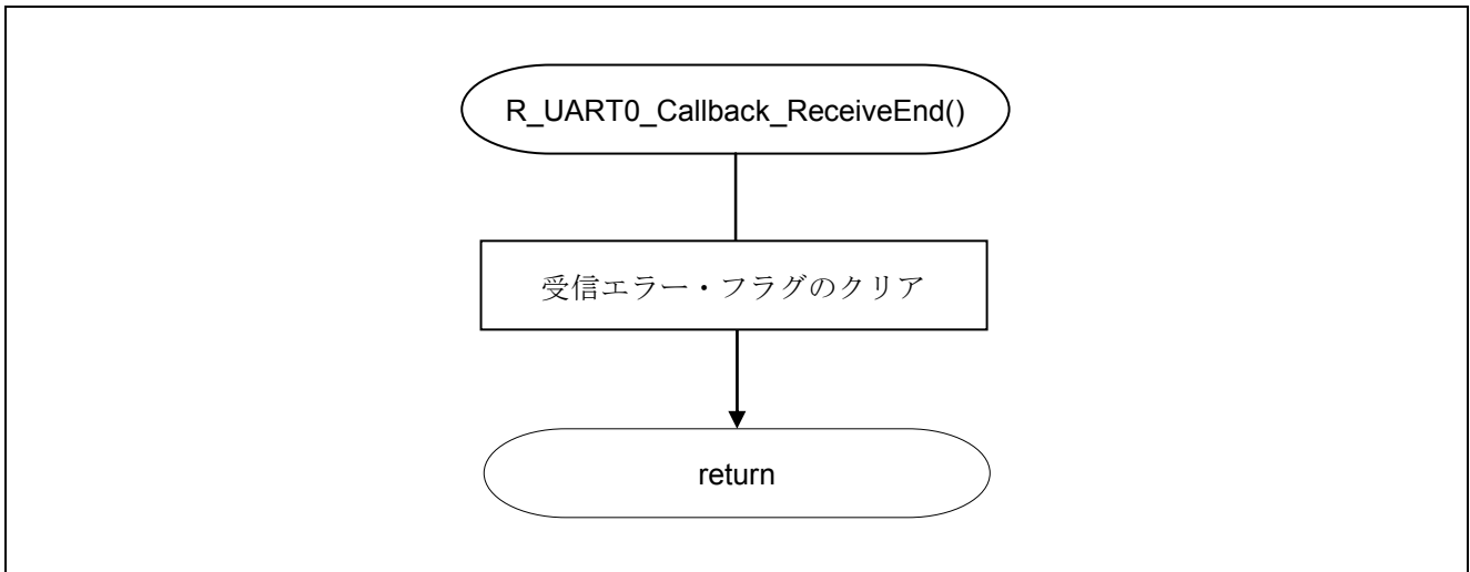
図 5.15 UART0 受信データ分類関数
