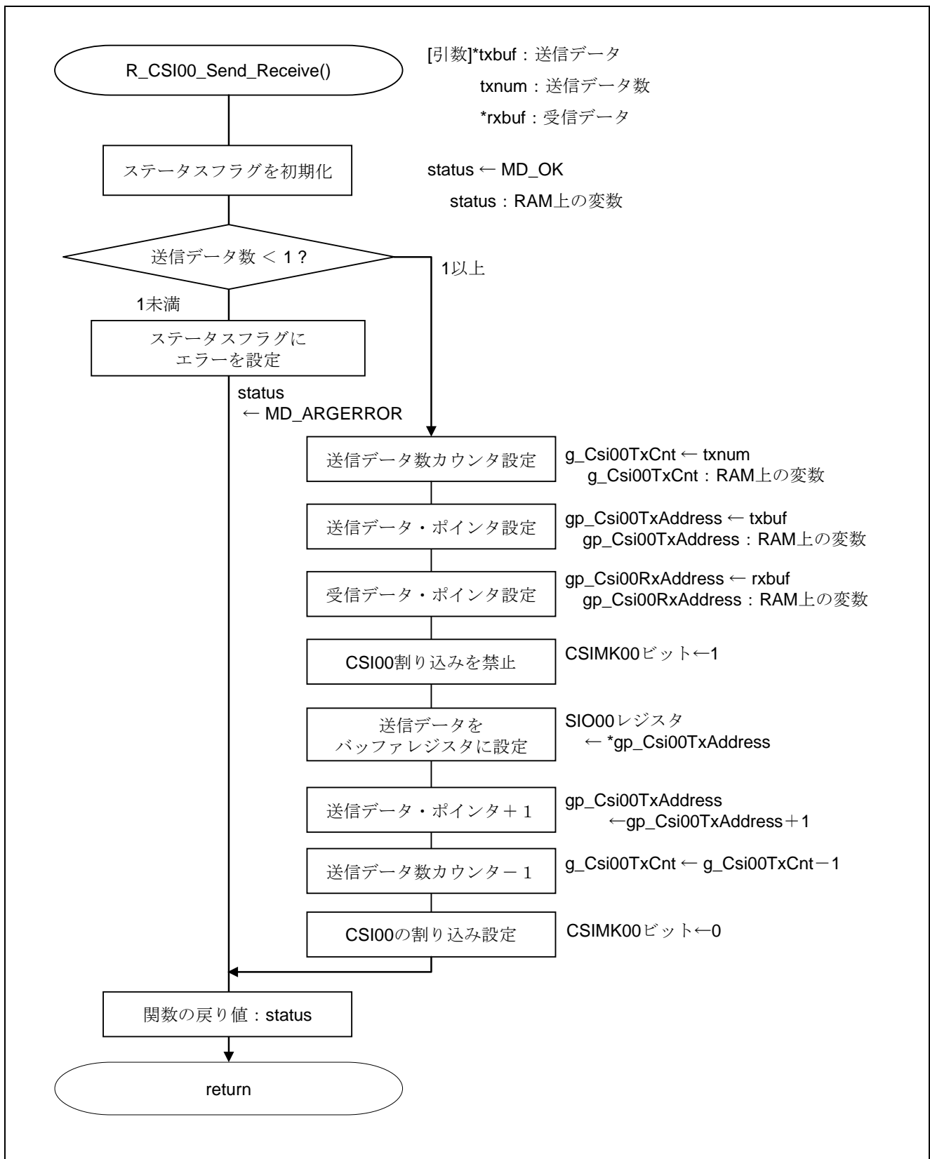
図 5.13 CSI00 データ送受信開始処理
