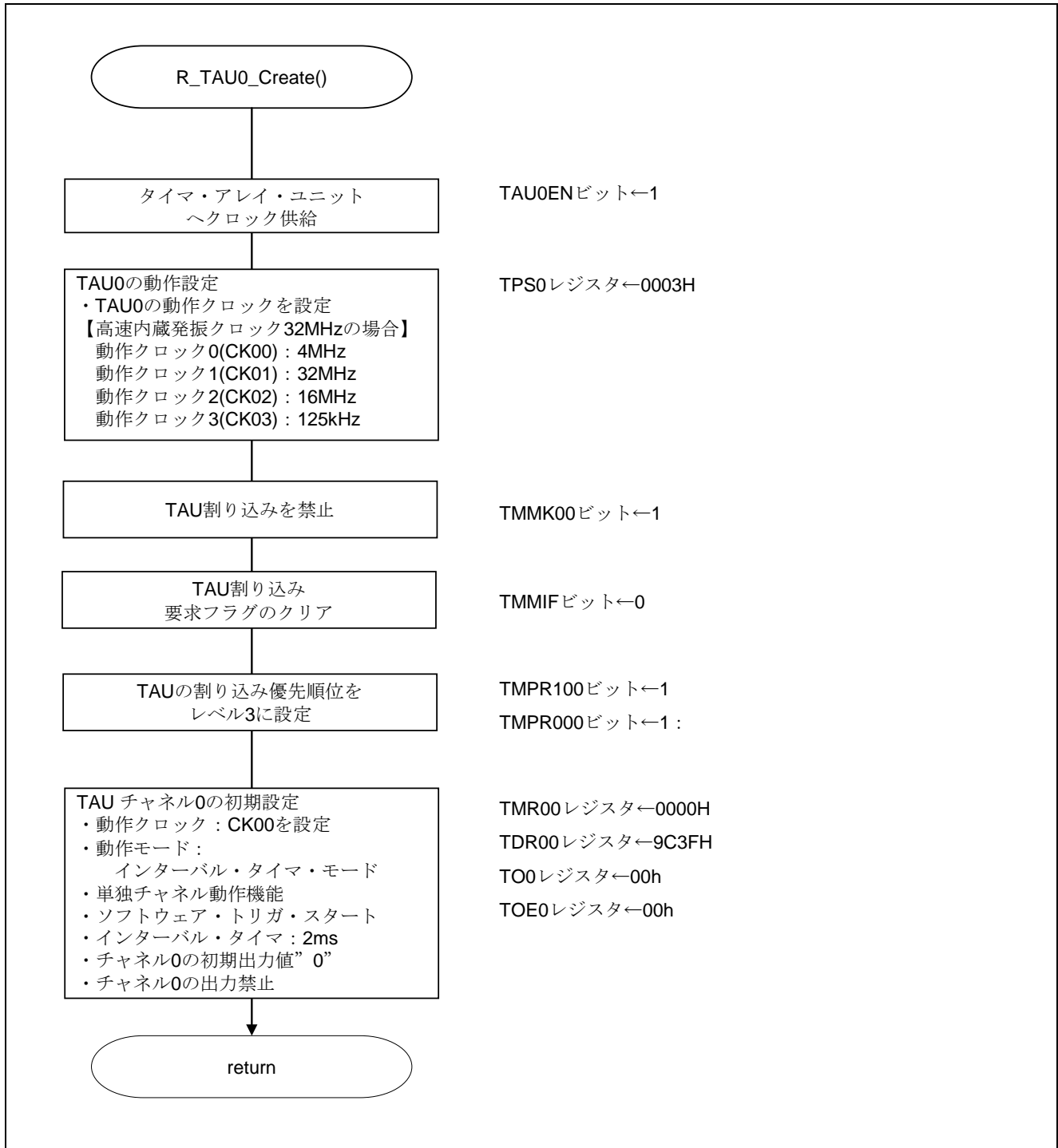
図 5.8 TAU0 の設定
