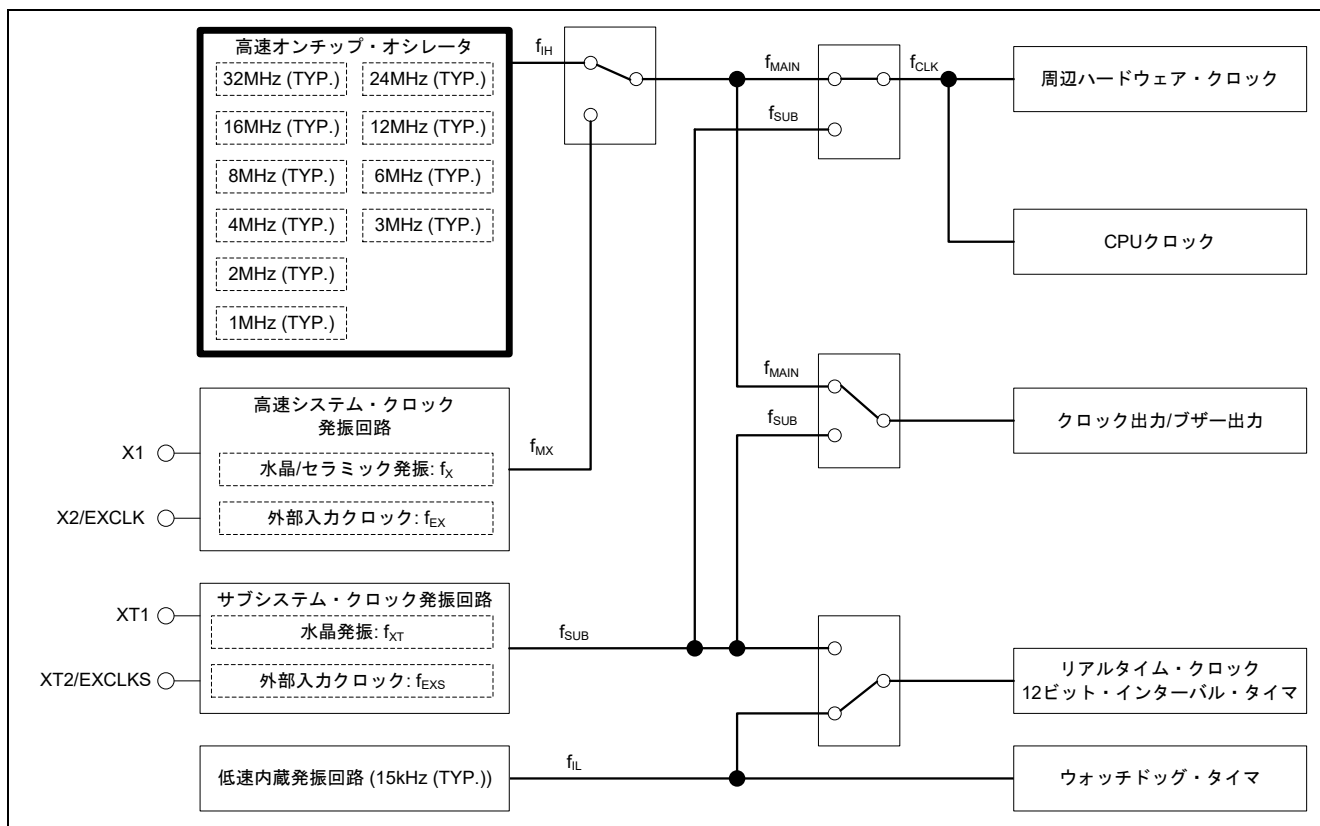
図 1.2 RL78/G13 のクロック発生回路のブロック図
