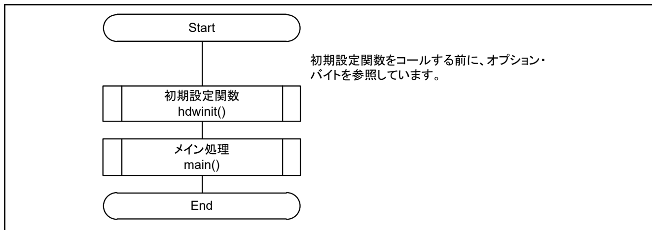
図 5.1 全体フロー
