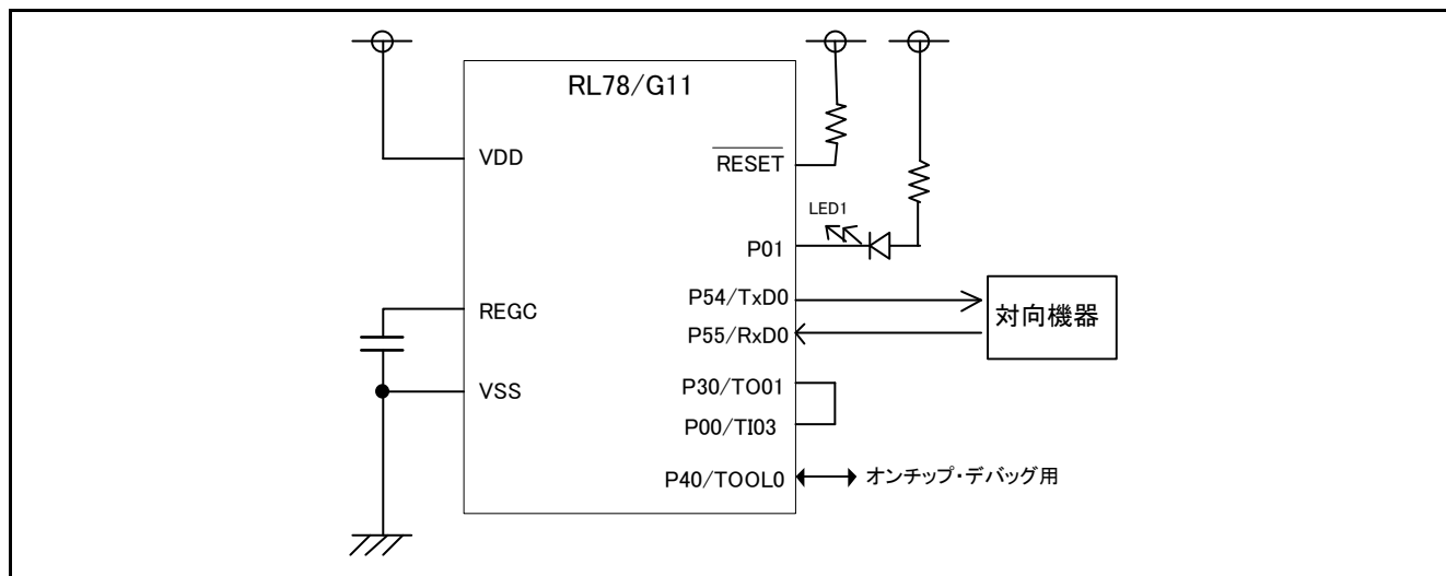
図 4.1 接続例
