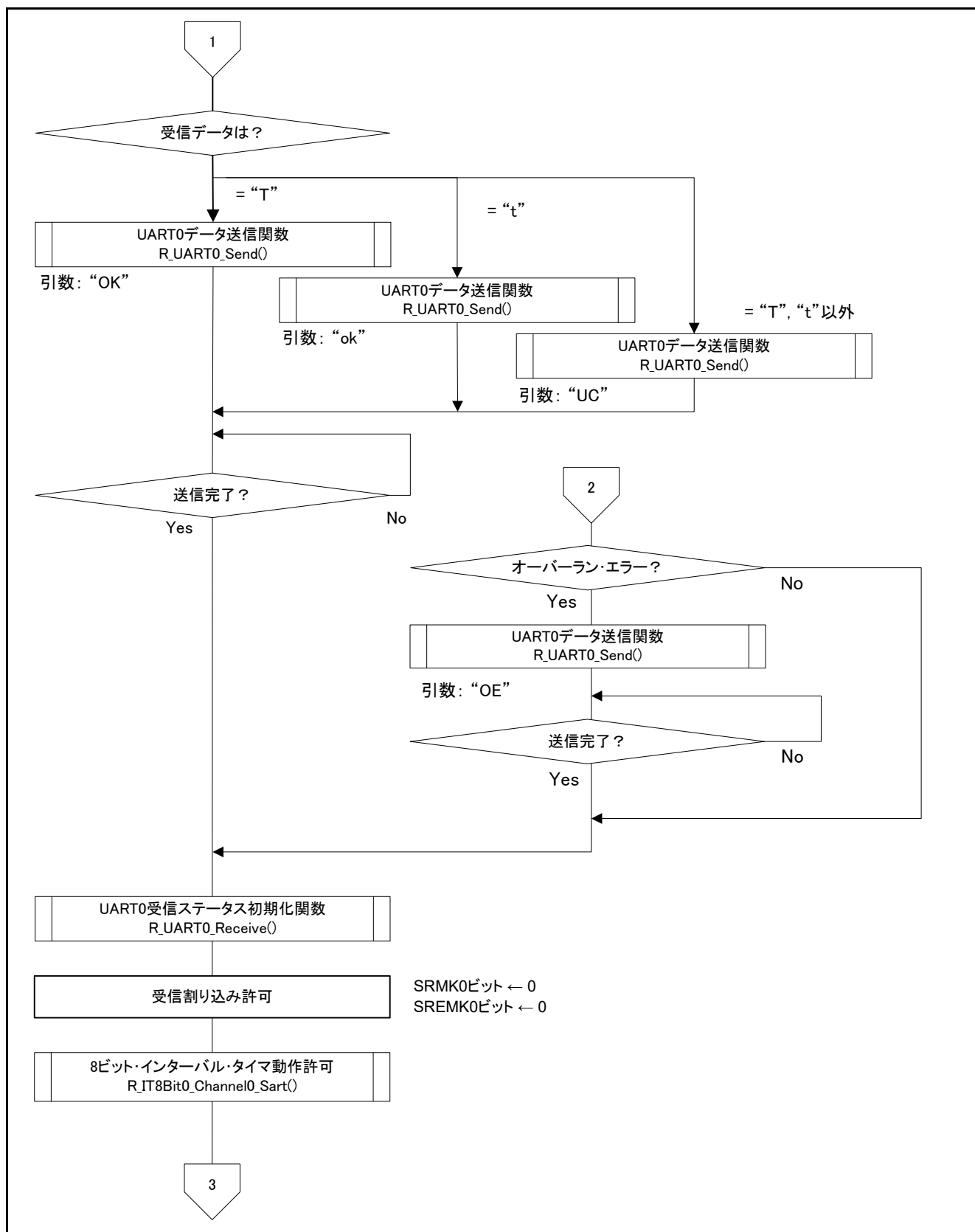
図 5.13 メイン処理 (2/2)
