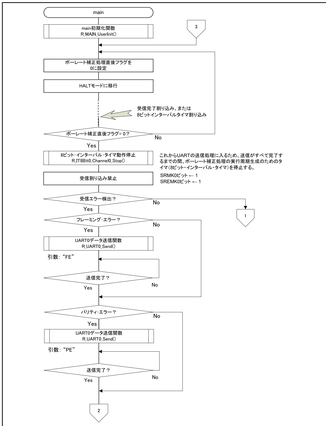
図 5.12 メイン関数 (1/2)
