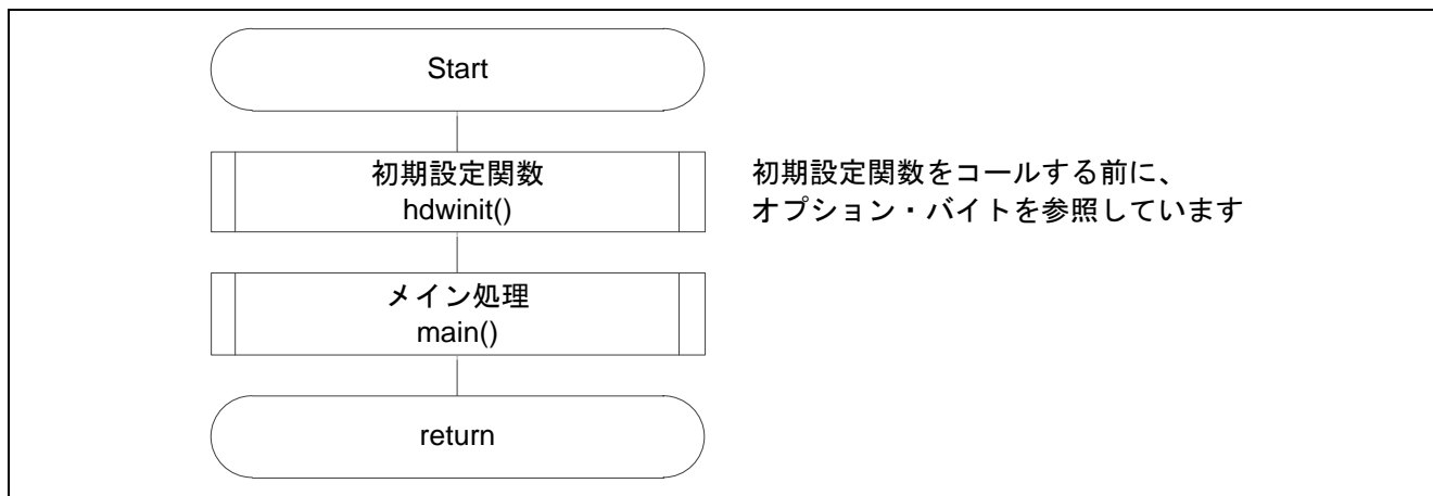
図 5.1 全体フロー
