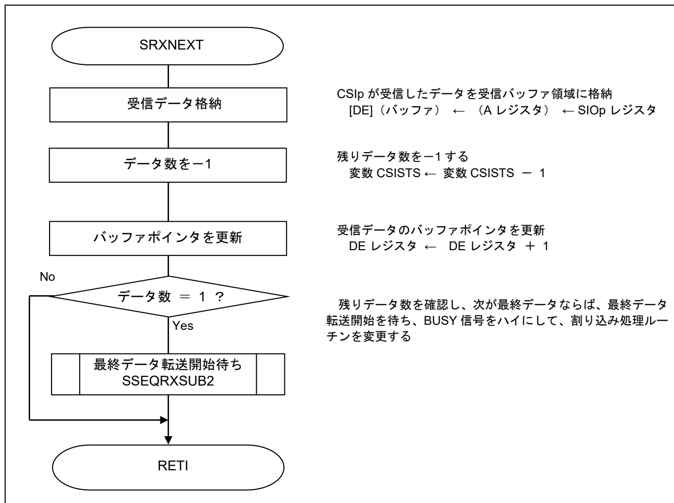
図 5.19 連続受信時データ受信完了割り込み処理
