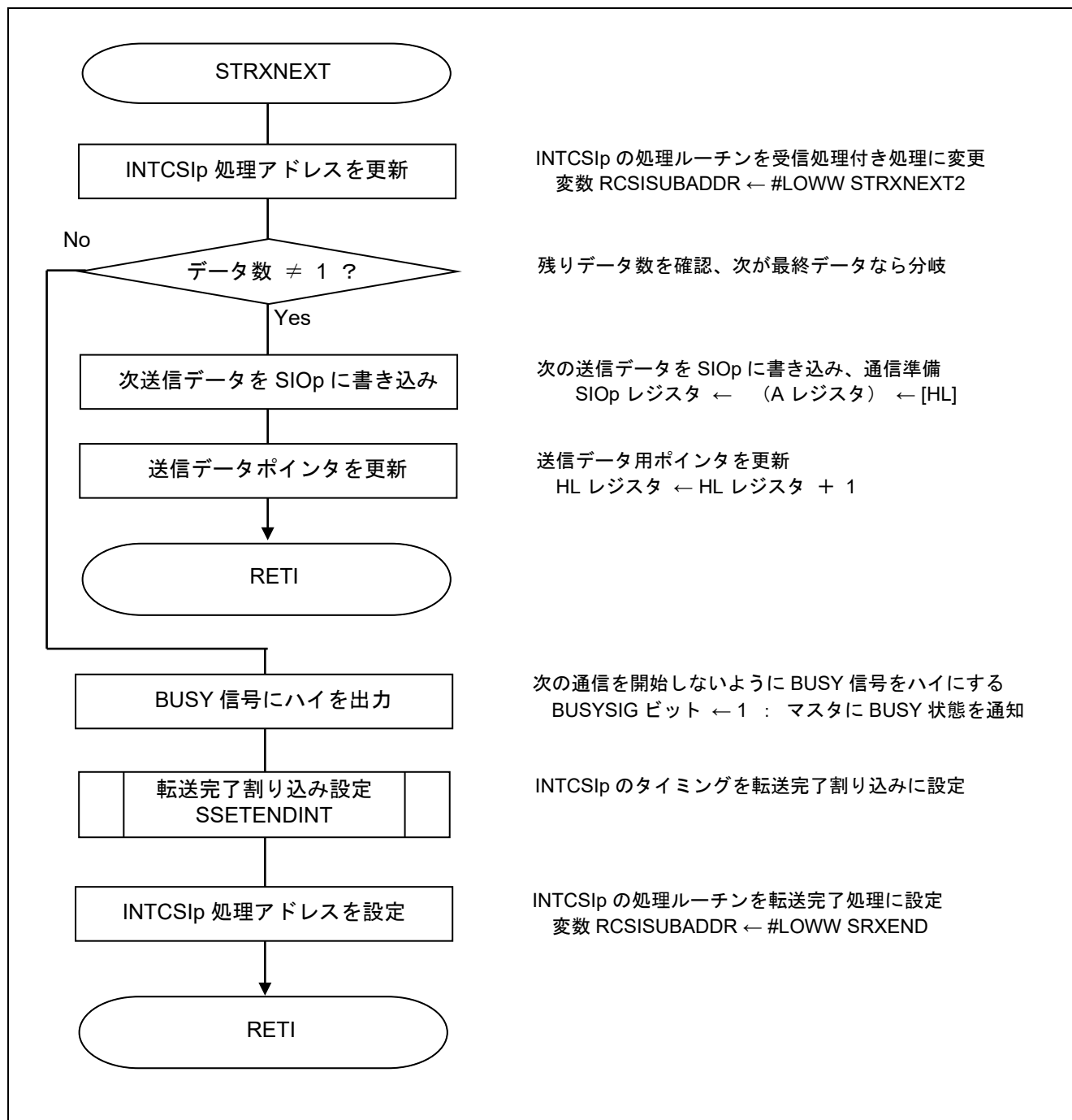
図 5.23 連続送受信時通信開始割り込み処理
