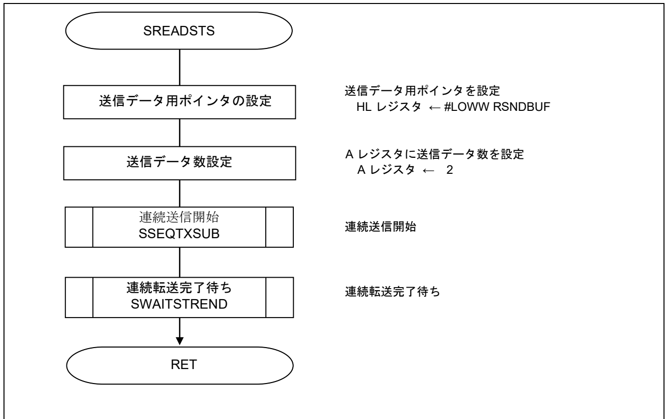
図 5.10 ステータス確認コマンド処理関数
