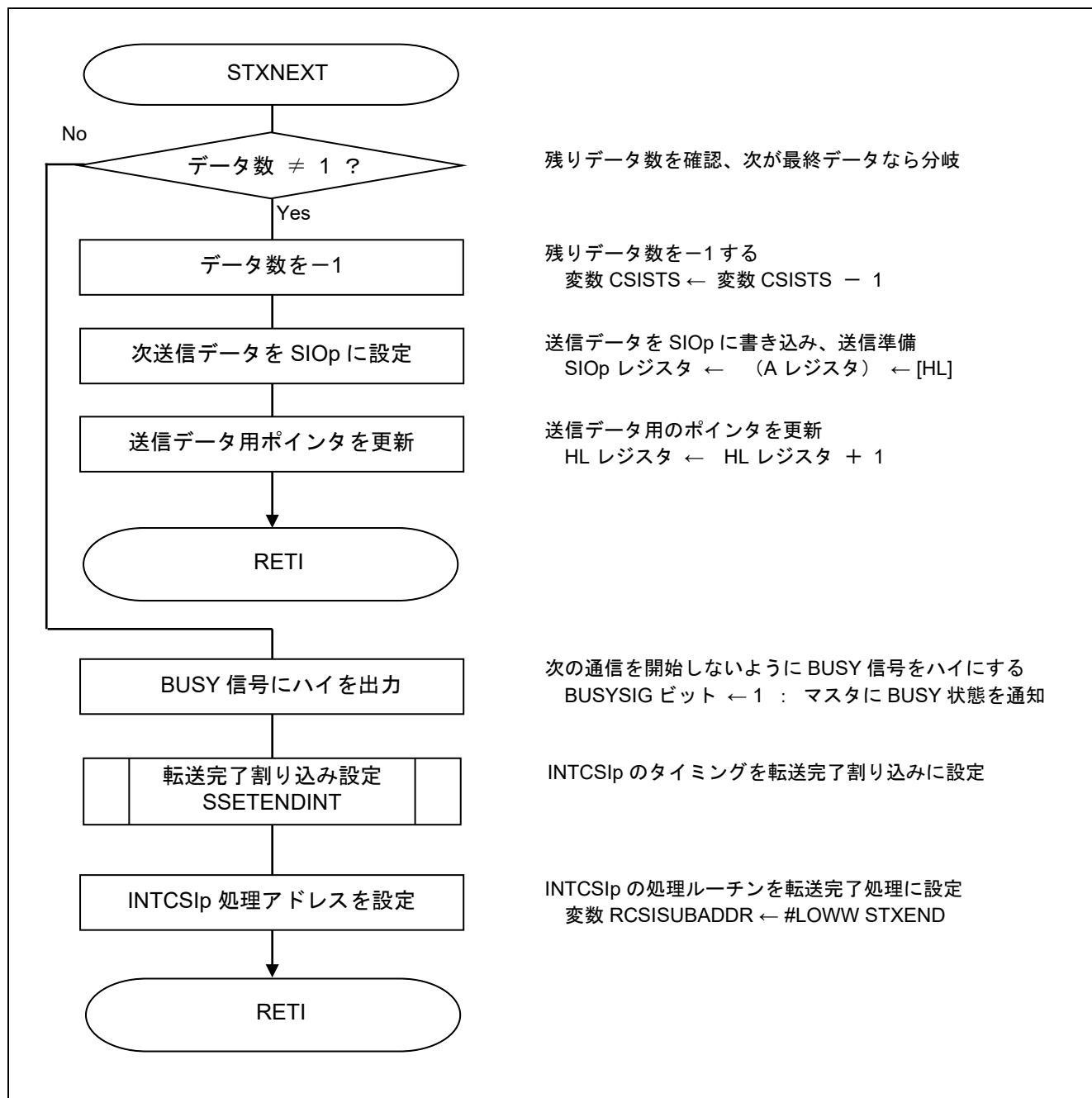
図 5.20 連続送信時データ送信完了割り込み処理
