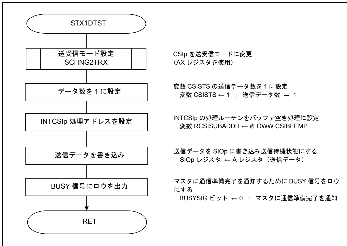
図 5.26 1 キャラクタ送信開始処理関数
