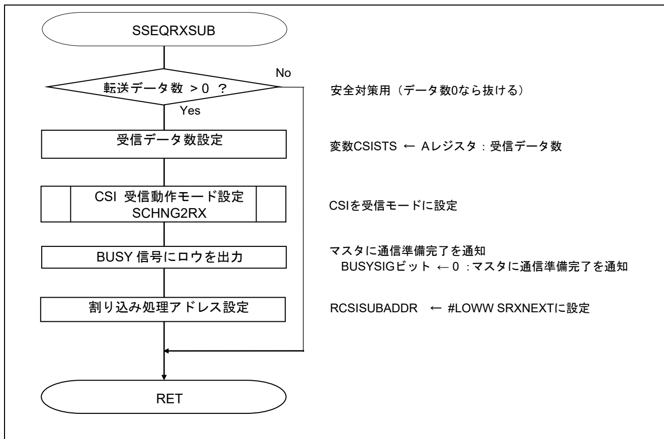
図 5.30 連続受信開始処理
