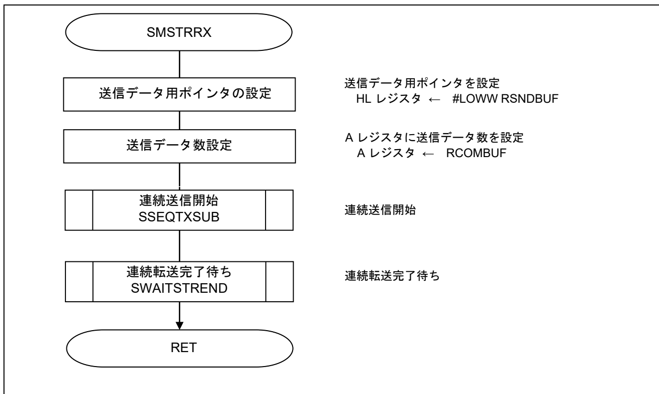
図 5.11 マスタ受信コマンド処理関数
