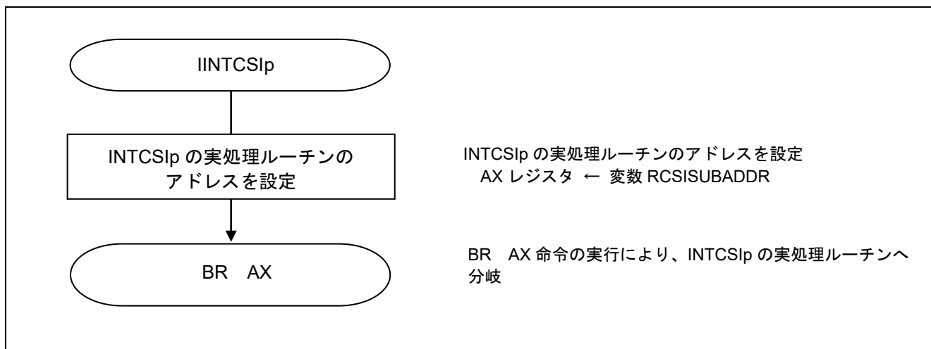
図 5.16 INTCSIp 割り込みエントリ処理
