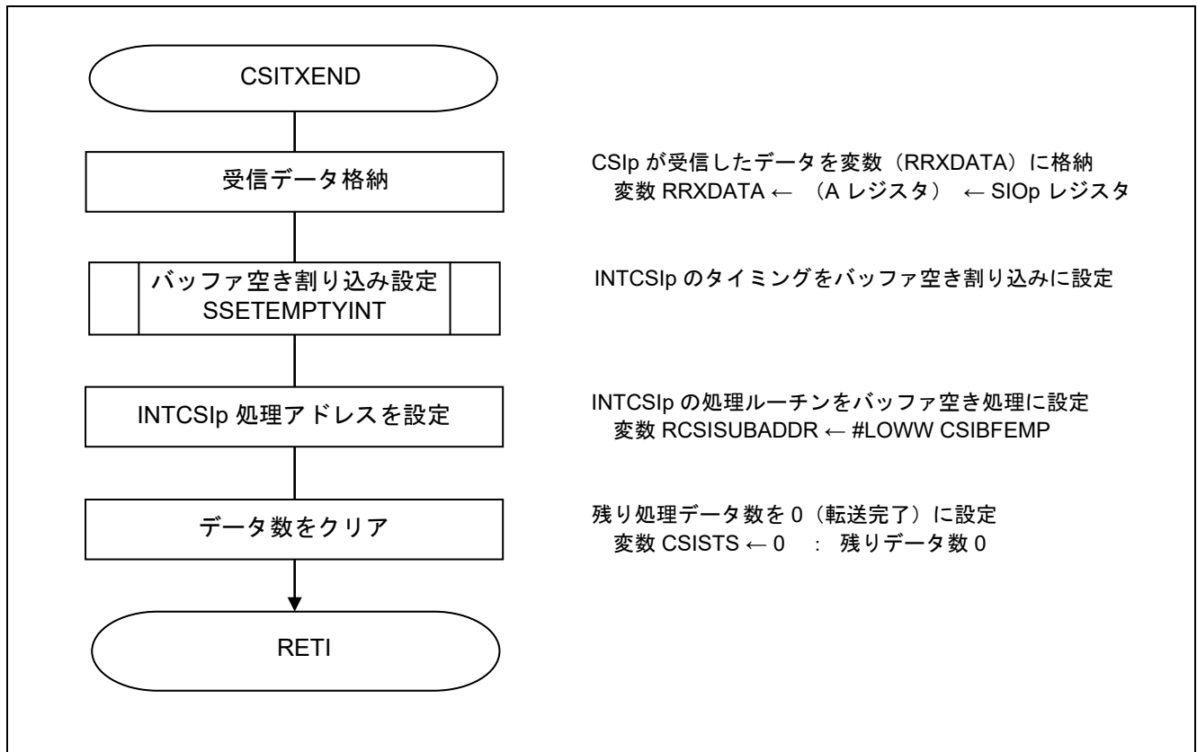
図 5.18 1 キャラクタ送信完了割り込み処理
