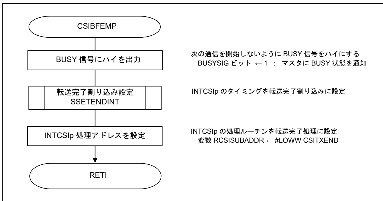
図 5.17 1 キャラクタ転送開始割り込み処理
