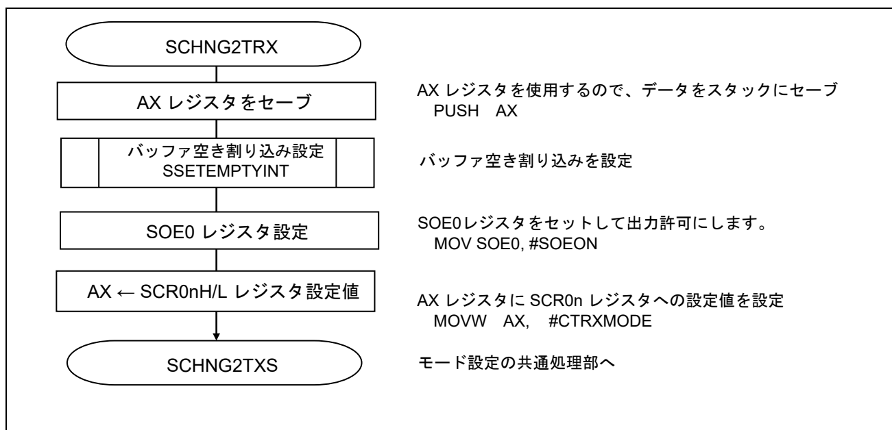
図 5.38 送受信モード設定処理
