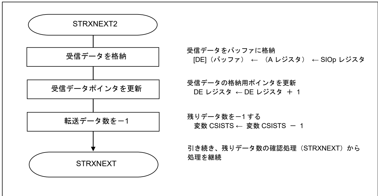
図 5.24 連続送受信時バッファ空き割り込み処理
