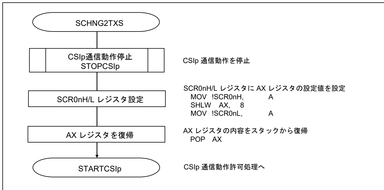
図 5.39 モード設定共通処理
