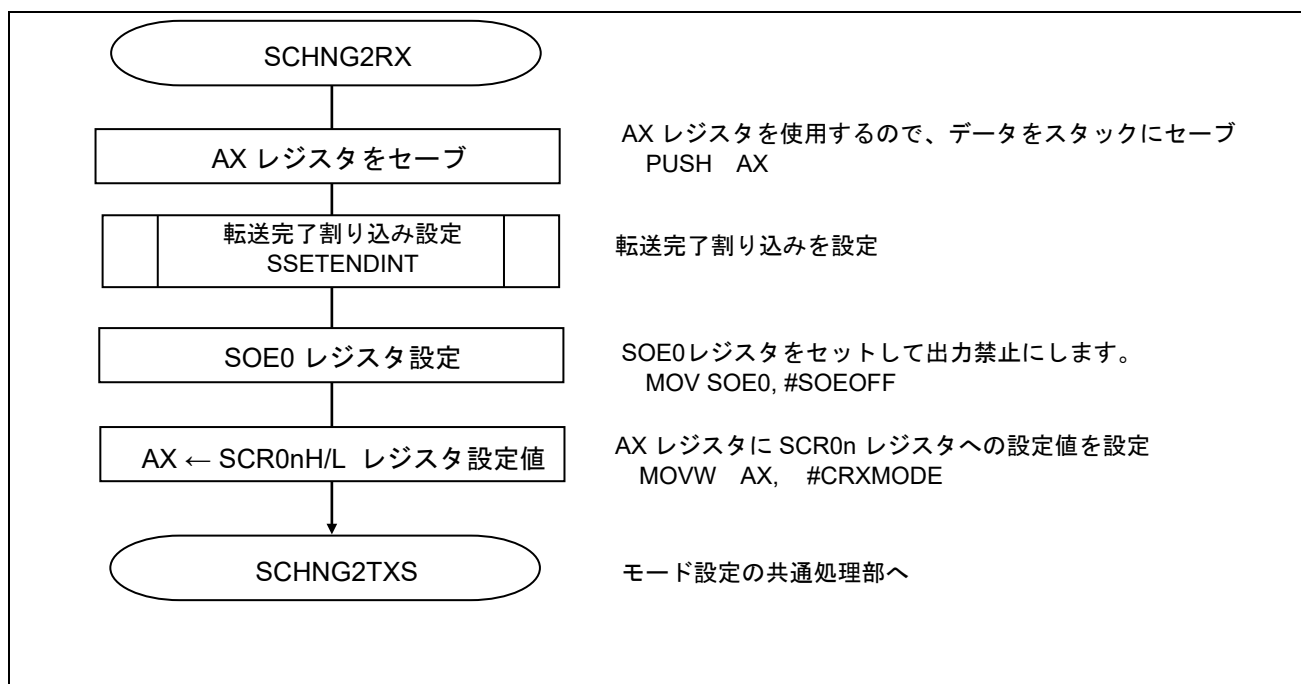
図 5.37 送信モード設定処理
