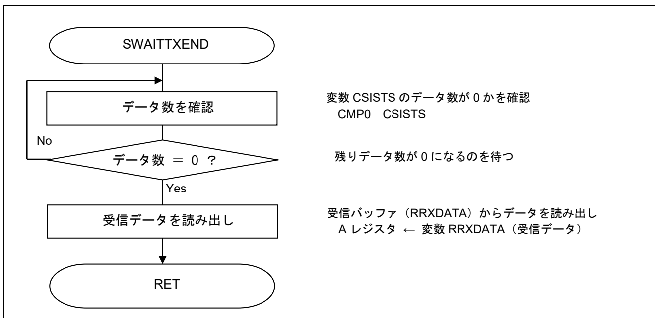
図 5.28 1 キャラクタ送受信完了待ち処理関数
