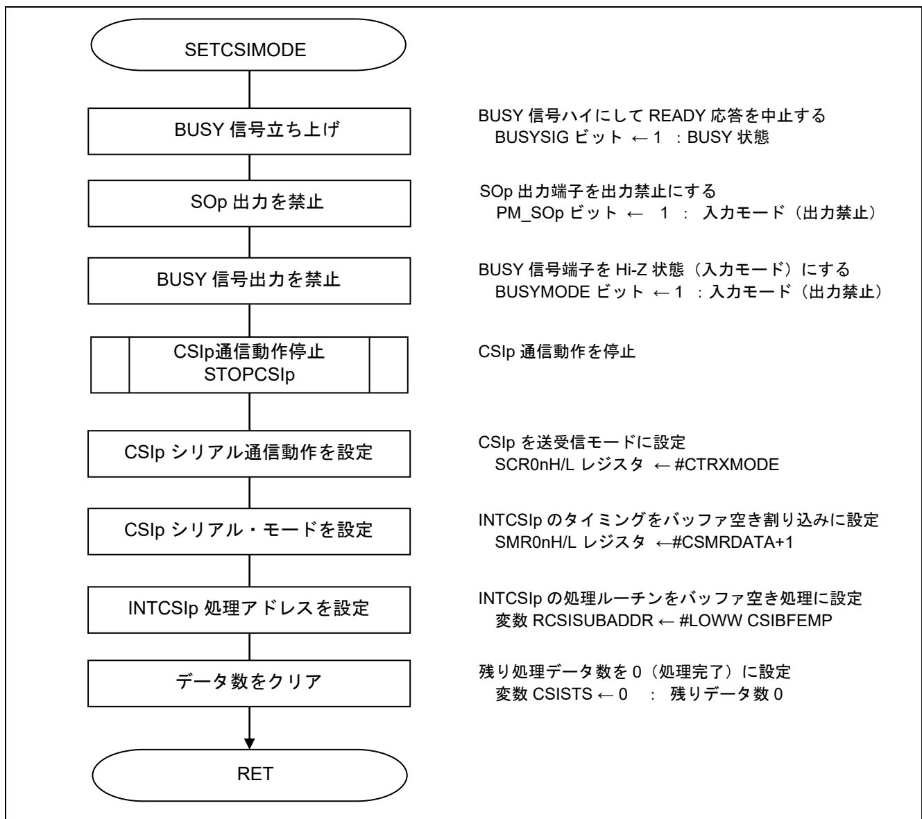
図 5.9 CSIp 選択解除処理関数
