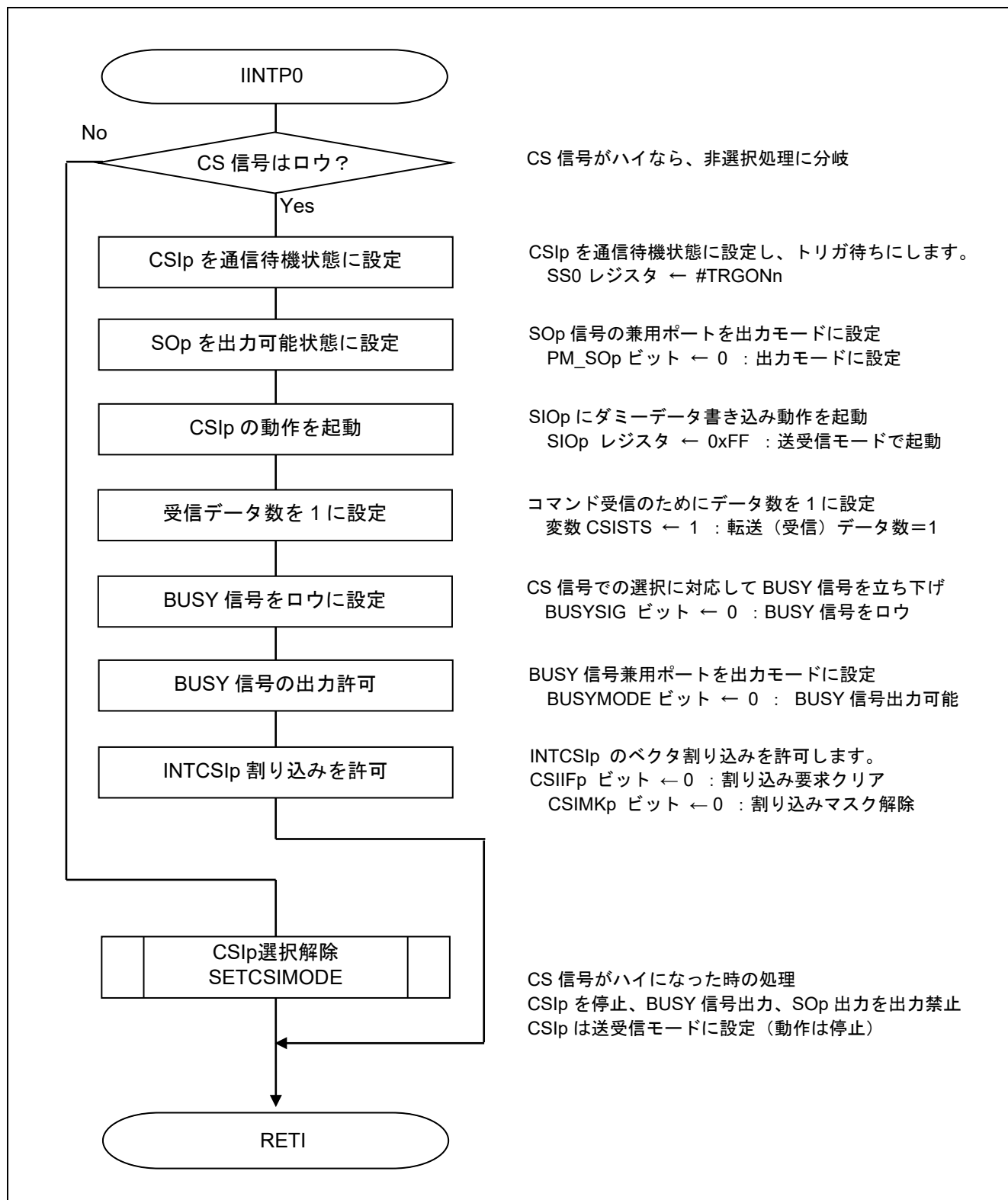
図 5.15 INTP0 割り込み処理関数
