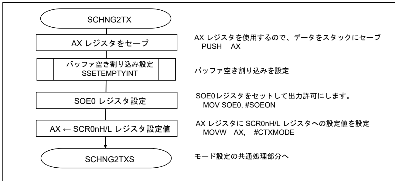
図 5.36 送信モード設定処理
