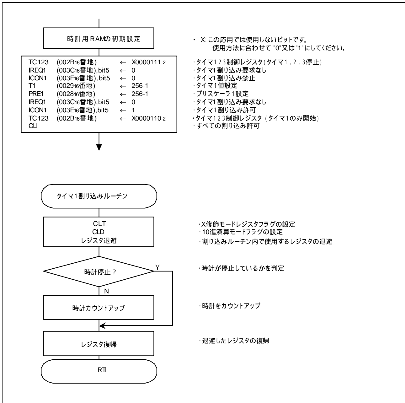
図 3.3 制御手順
